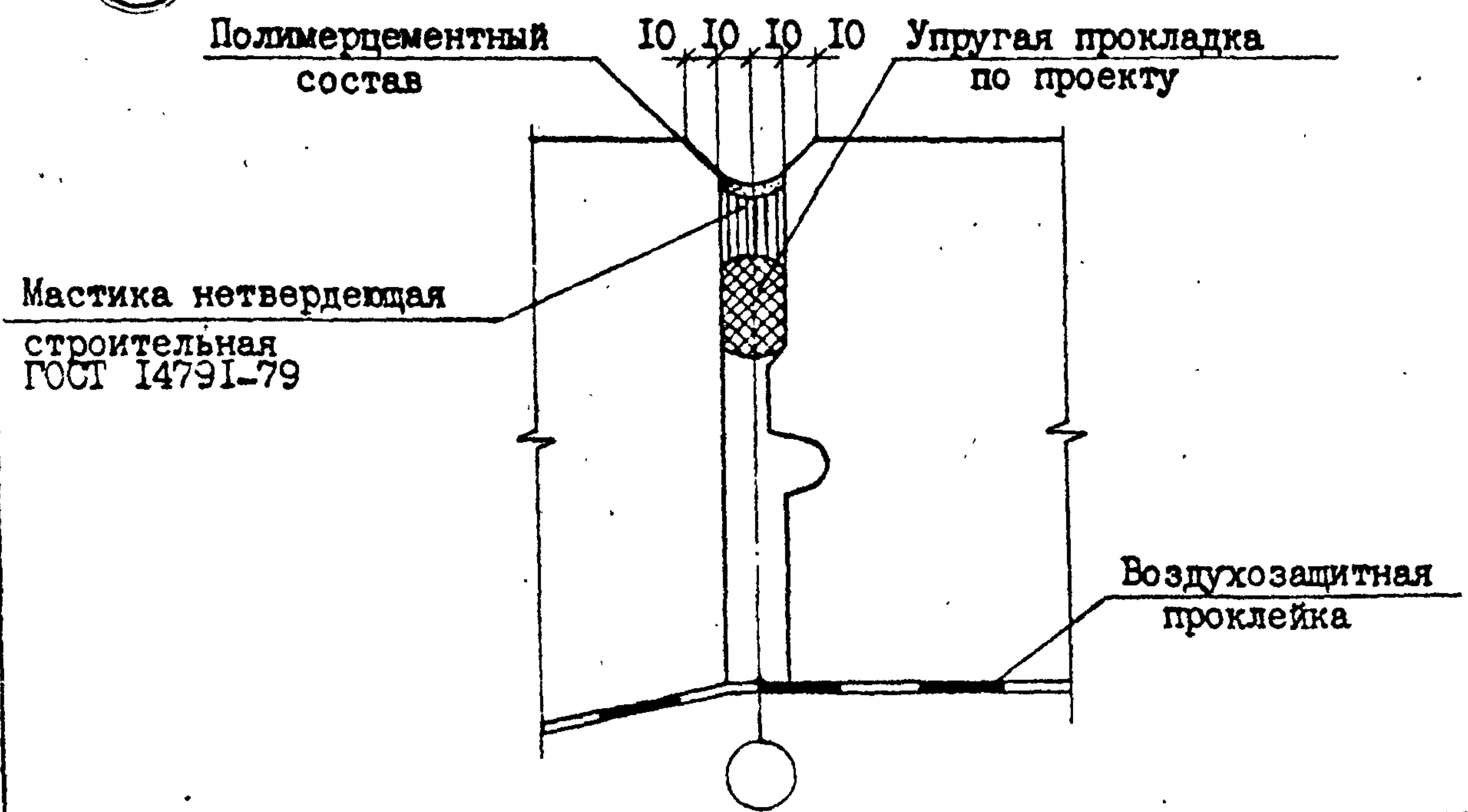
А ВАРИАНТ ЗАДЕЛКИ СТЫКА НЕТВЕРДЕЮЩЕЙ МАСТИКОЙ РИС.1
