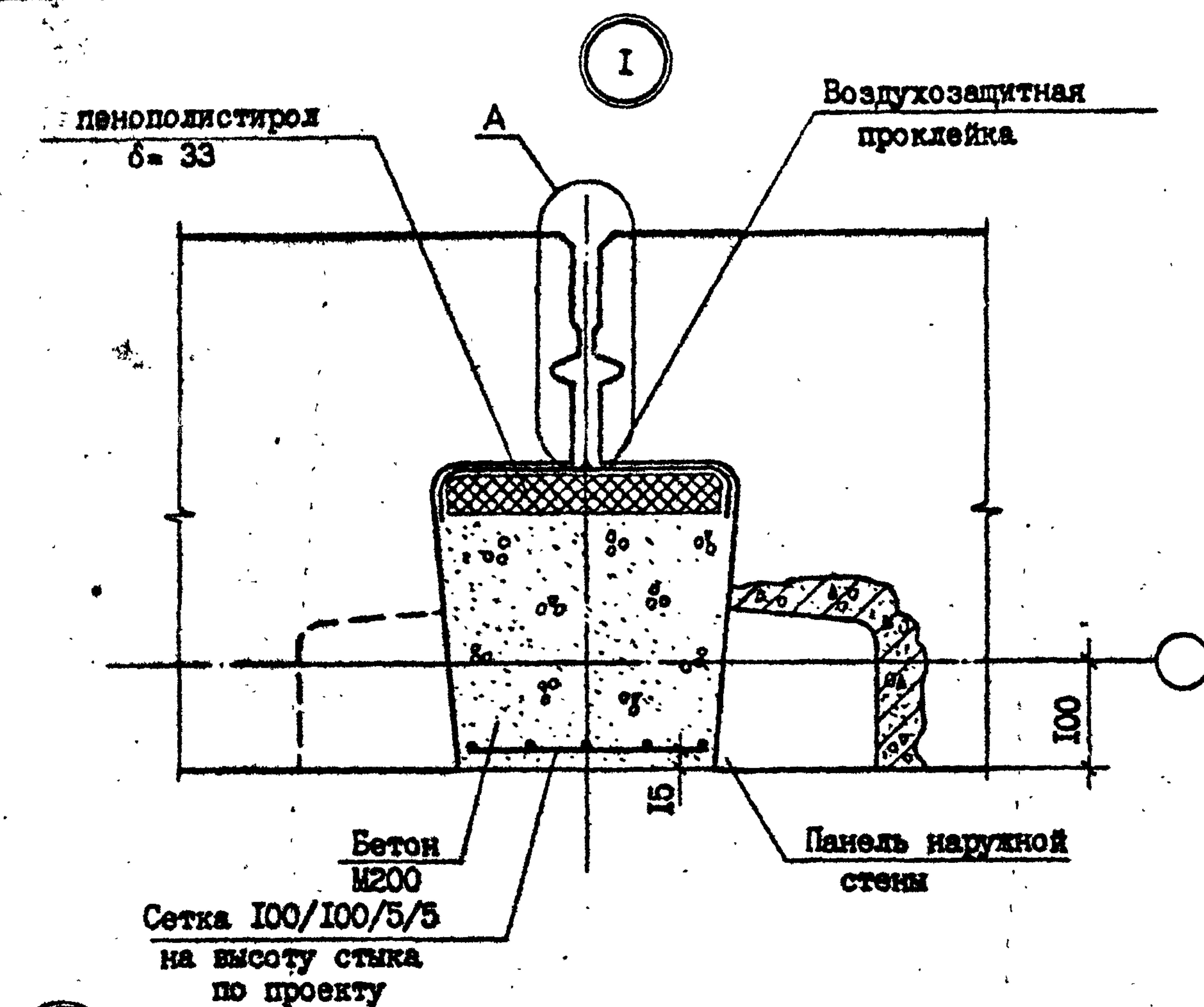
ВАРИАНТ ЗАДЕЛКИ СТЫКОВ НЕТВЕРДЕЮЩЕЙ МАСТИКОЙ РИС.1
