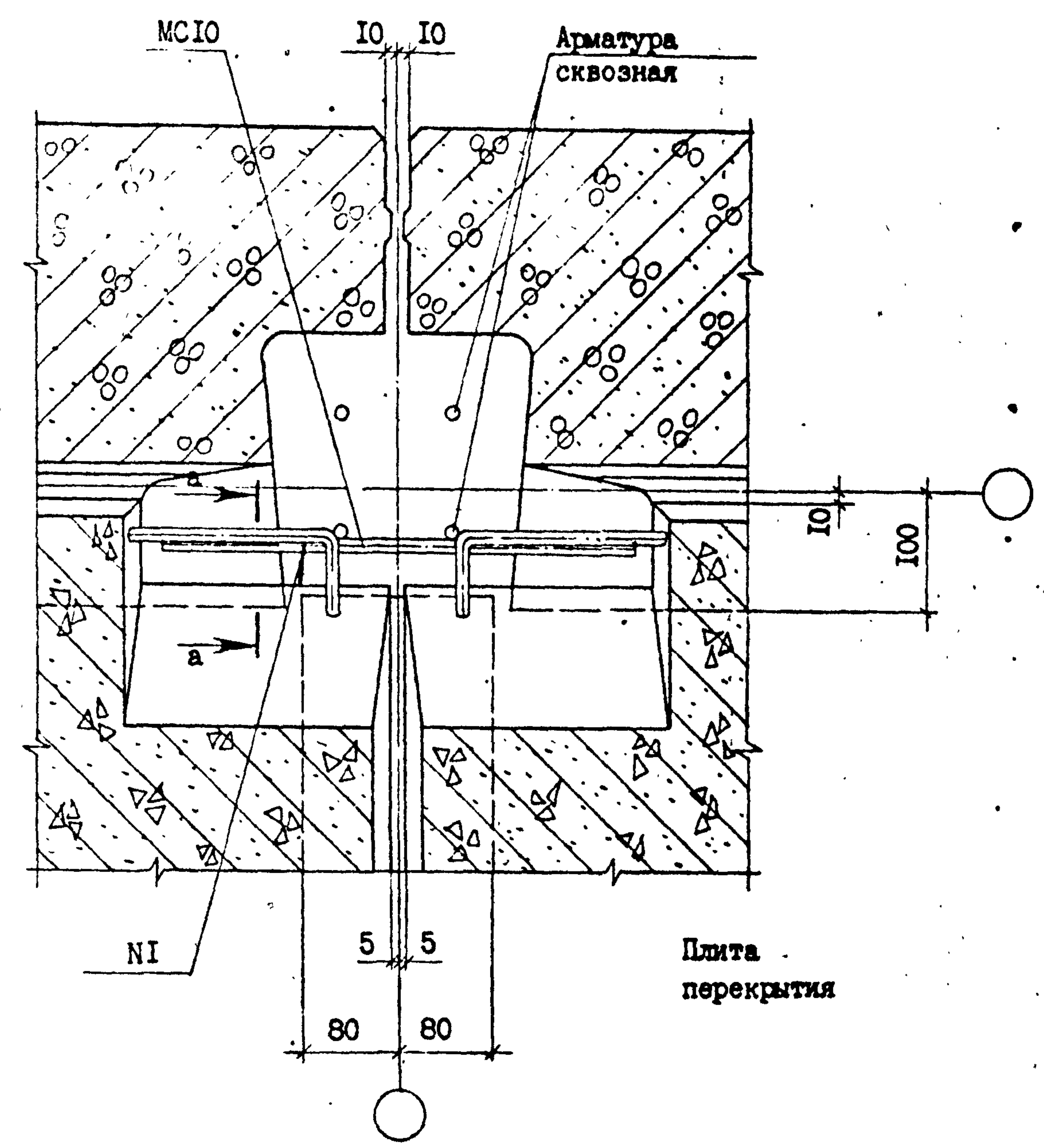
Сечение а-а см. лист I
