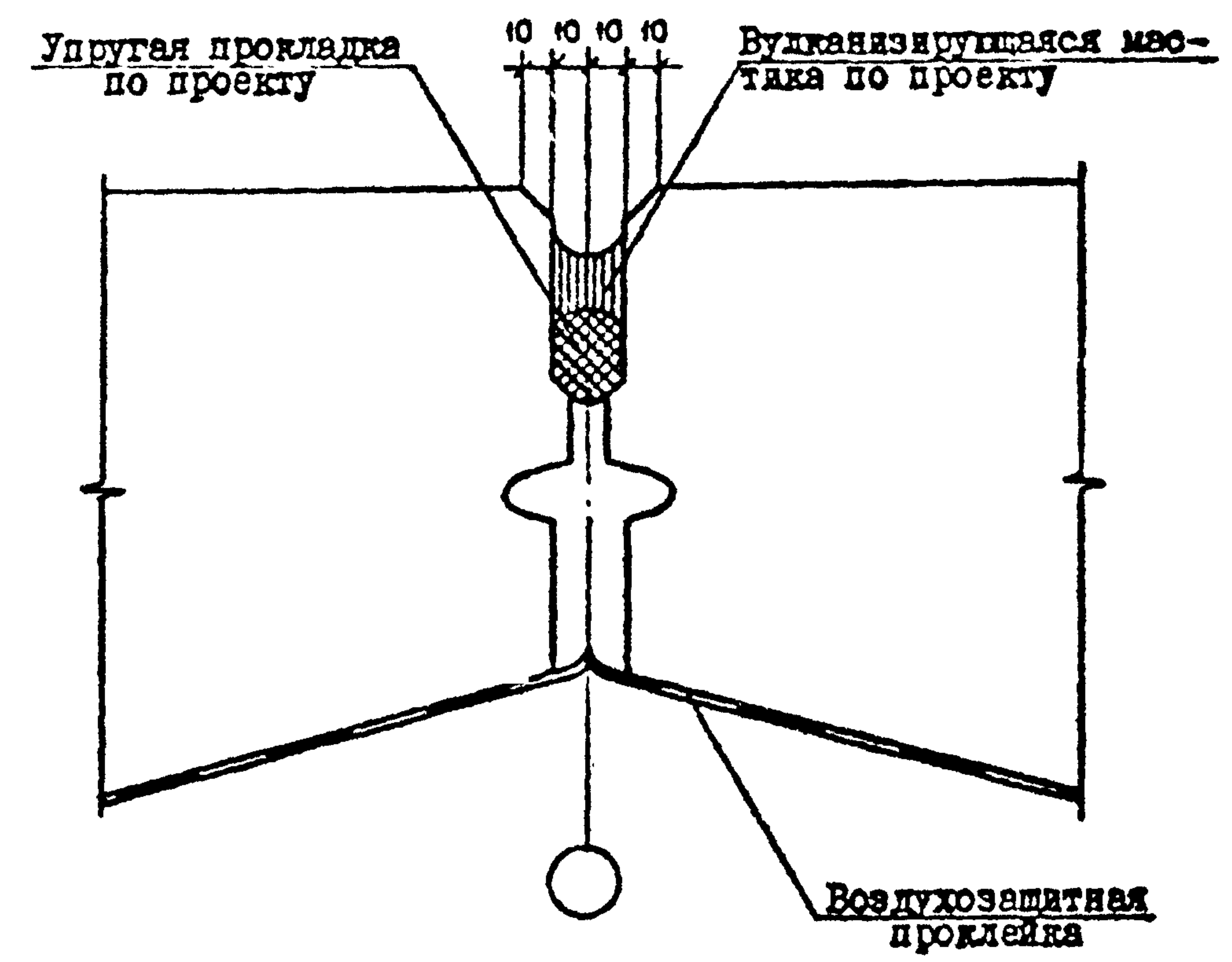
А ВАРИАНТ ЗАДЕЛКИ СТЫКОВ ВУЛКАНИЗИРУЮЩЕЙ МАСТИКОЙ РИС. 2
