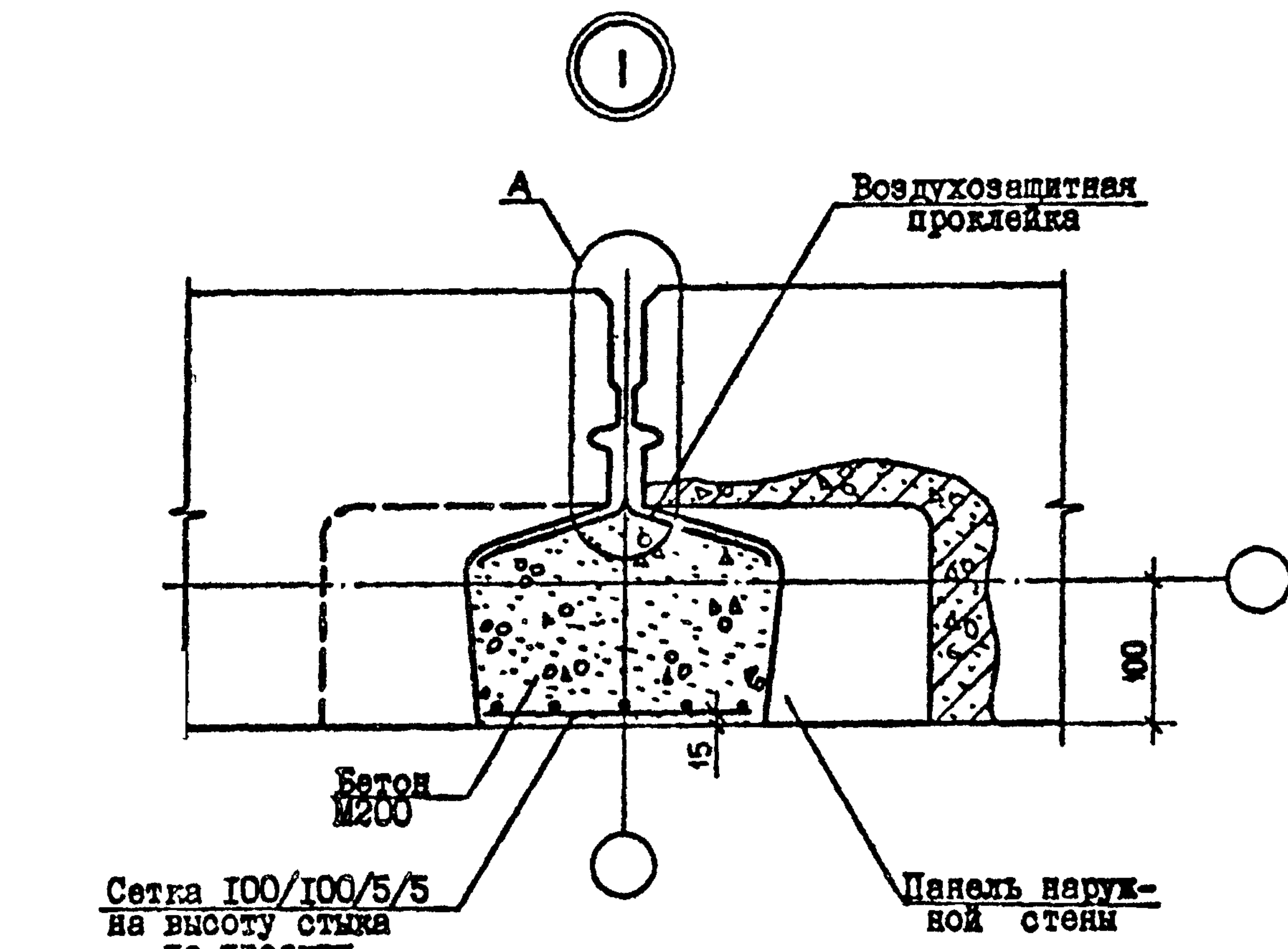
А ВАРИАНТ ЗАДЕЛКИ СТЫКОВ НЕТВЕРДЕЮЩЕЙ МАСТИКОЙ РИС. 1
