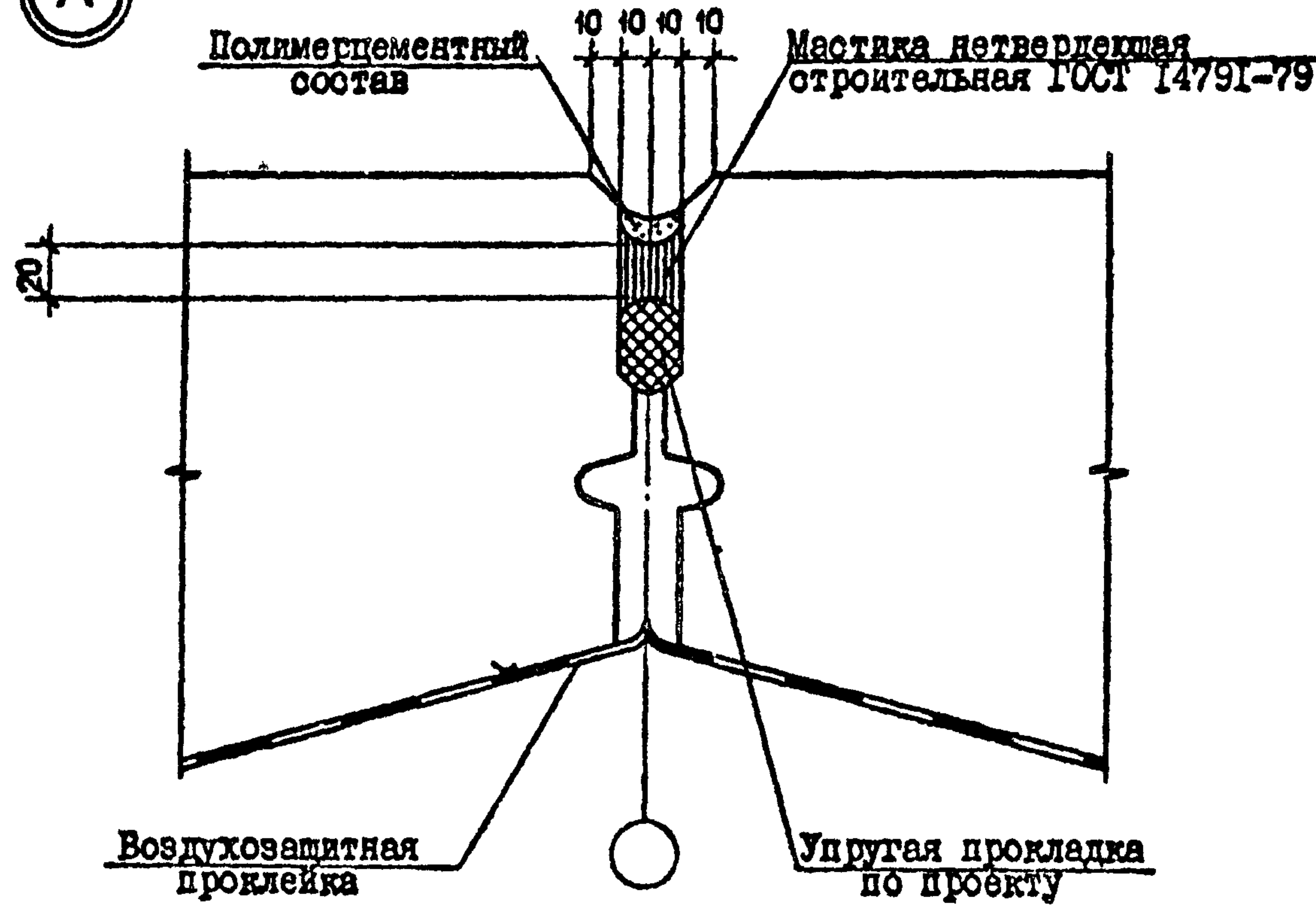
А ВАРИАНТ ЗАДЕЛКИ СТЫКОВ НЕТВЕРДЕЮЩЕЙ МАСТИКОЙ РИС. 1
