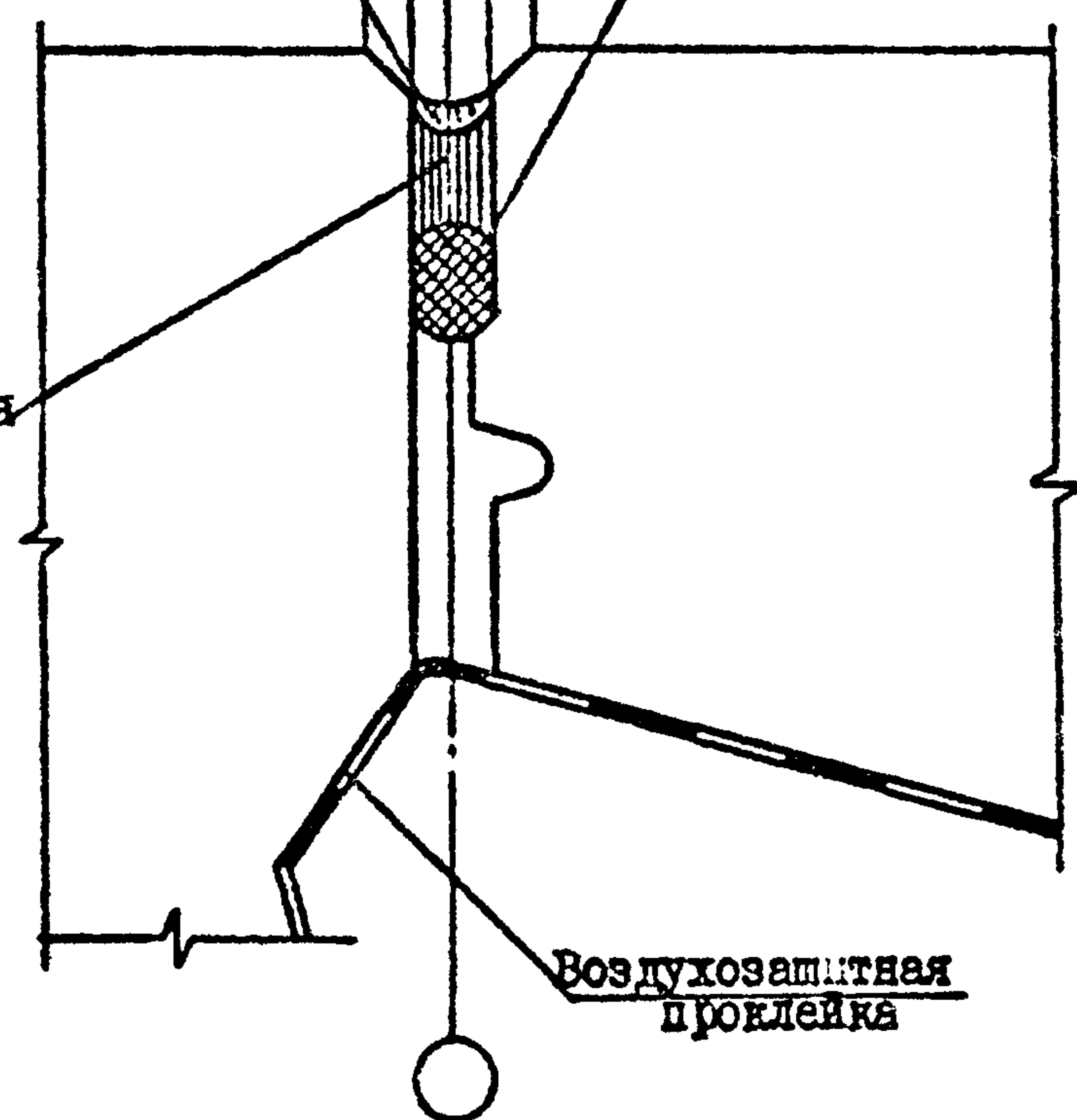
А ВАРИАНТ ЗАДЕЛКИ СТЫКА НЕТВЕРДЕЮЩЕЙ МАСТИКОЙ РИС. 1 Полимерцементный состав 10 10 10 10 Упругая прокладка по проекту
