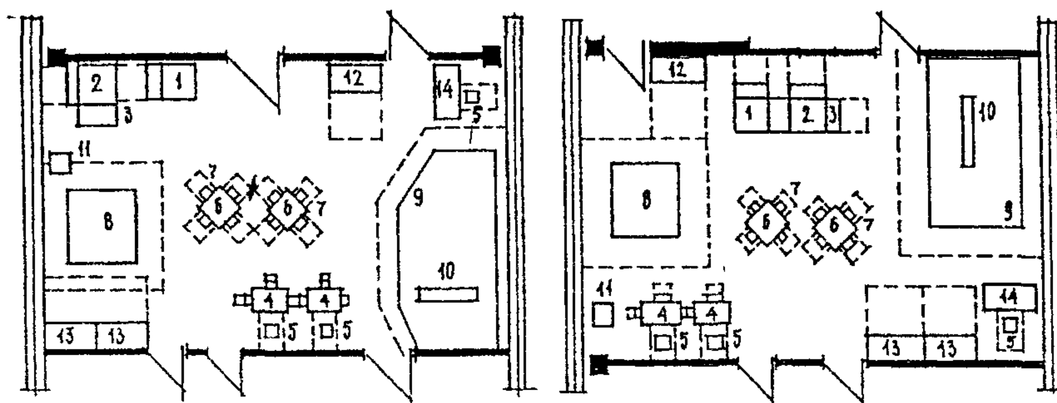
Рис. 29 Различные схемы размещения мебели в групповой детей 0-1 года
