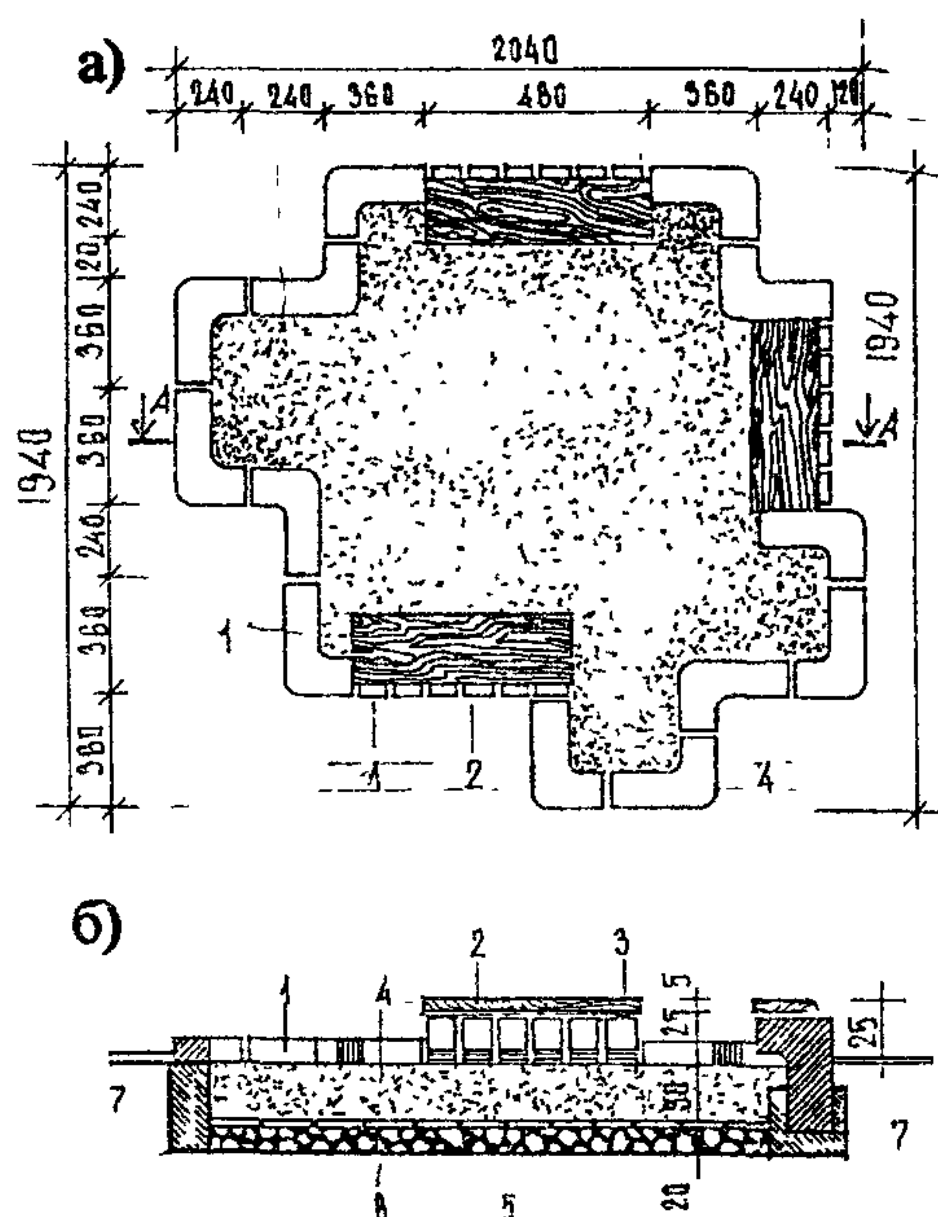
Рис. 11 Пример решения песочного двора (опыт Болгарии)
