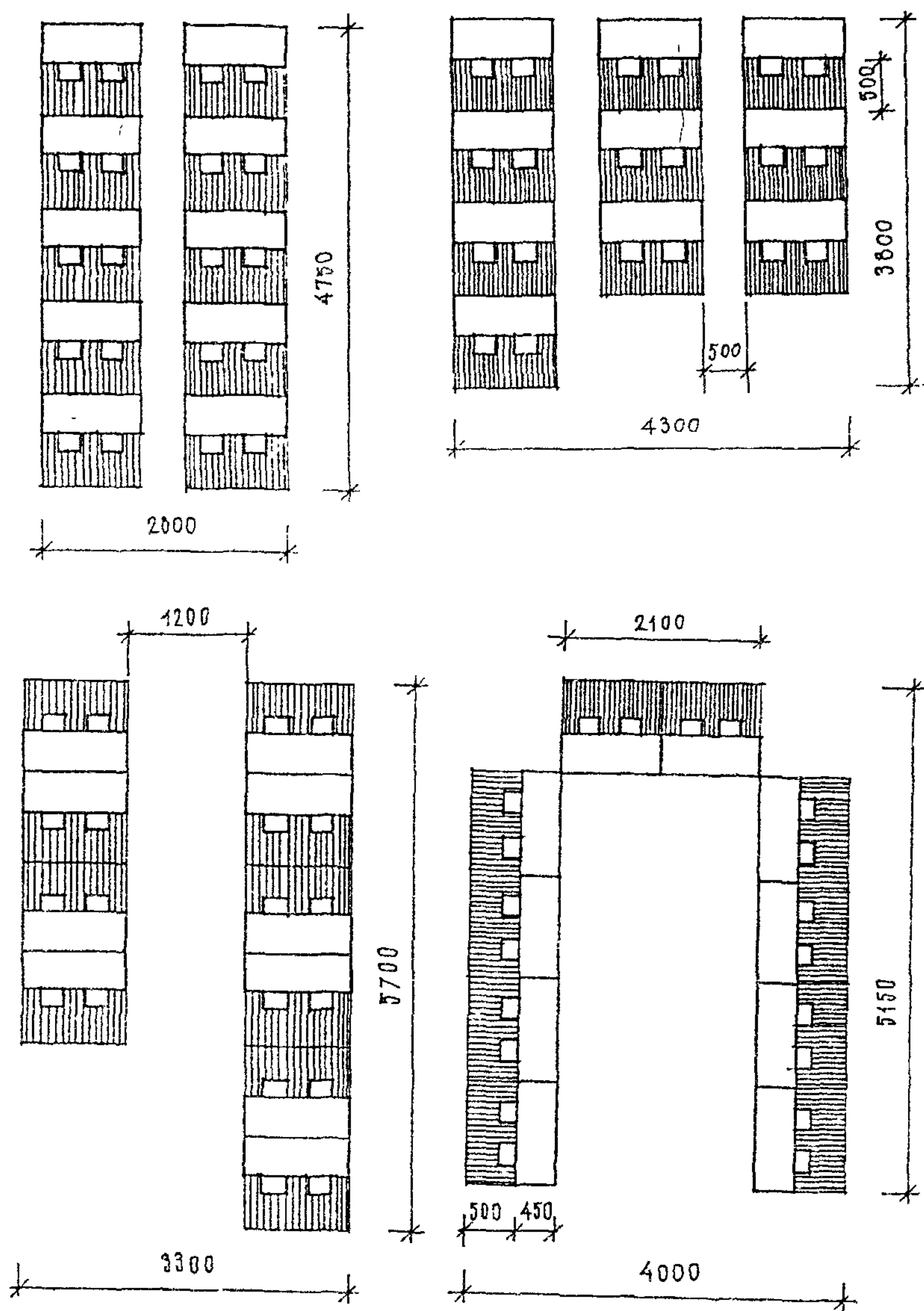
Рис. 31 Разные приемы организации "зоны столиков" в групповых детей 3-6(7) лет во время еды и занятий, для которых данная организация пространства является желательной
