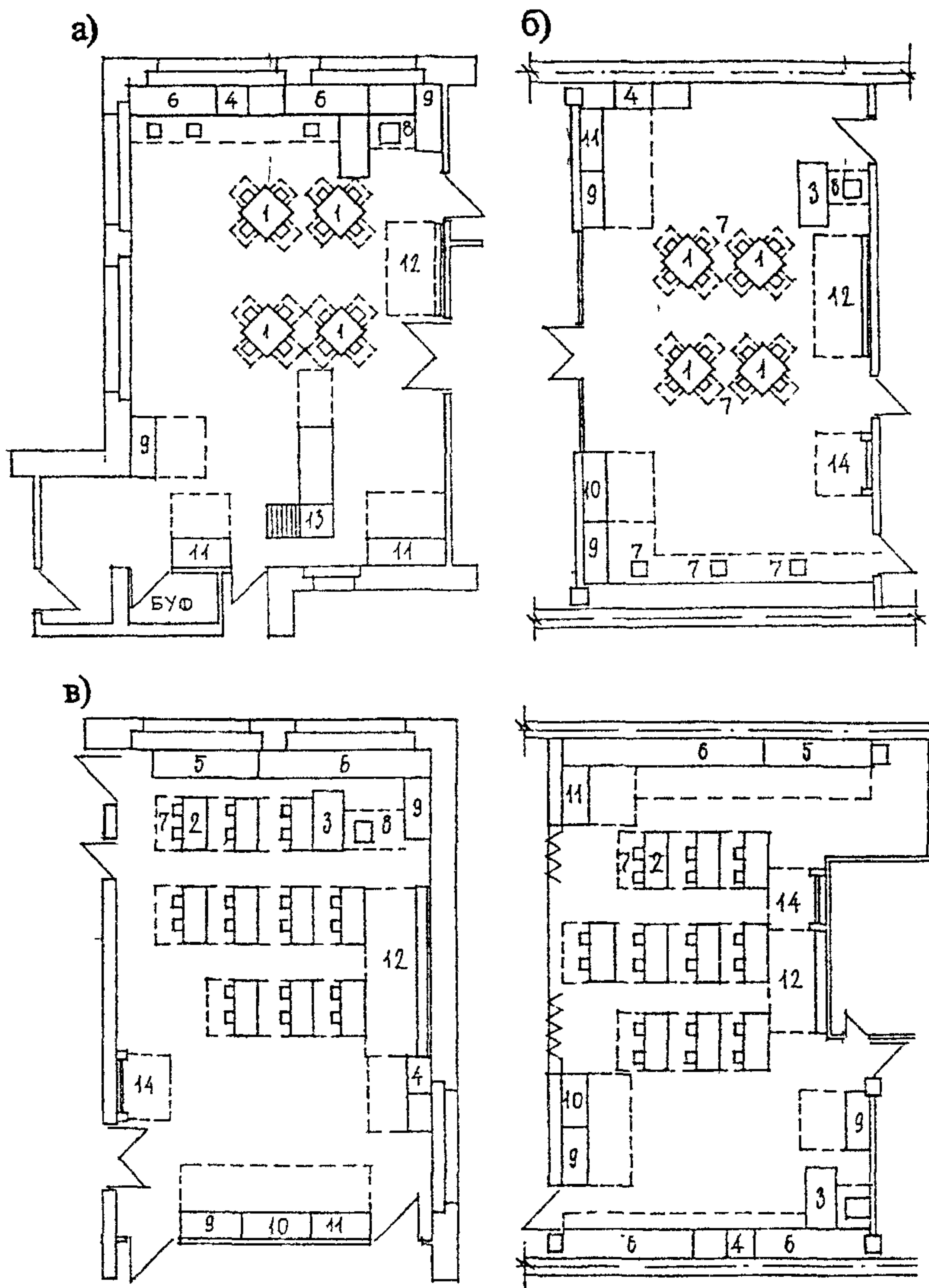
Рис. 32 Примеры размещения мебели в групповых
