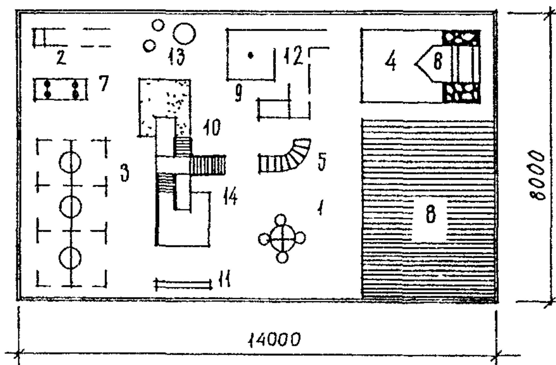
Рис. 12 Групповая площадка для детей с нарушением слуха
