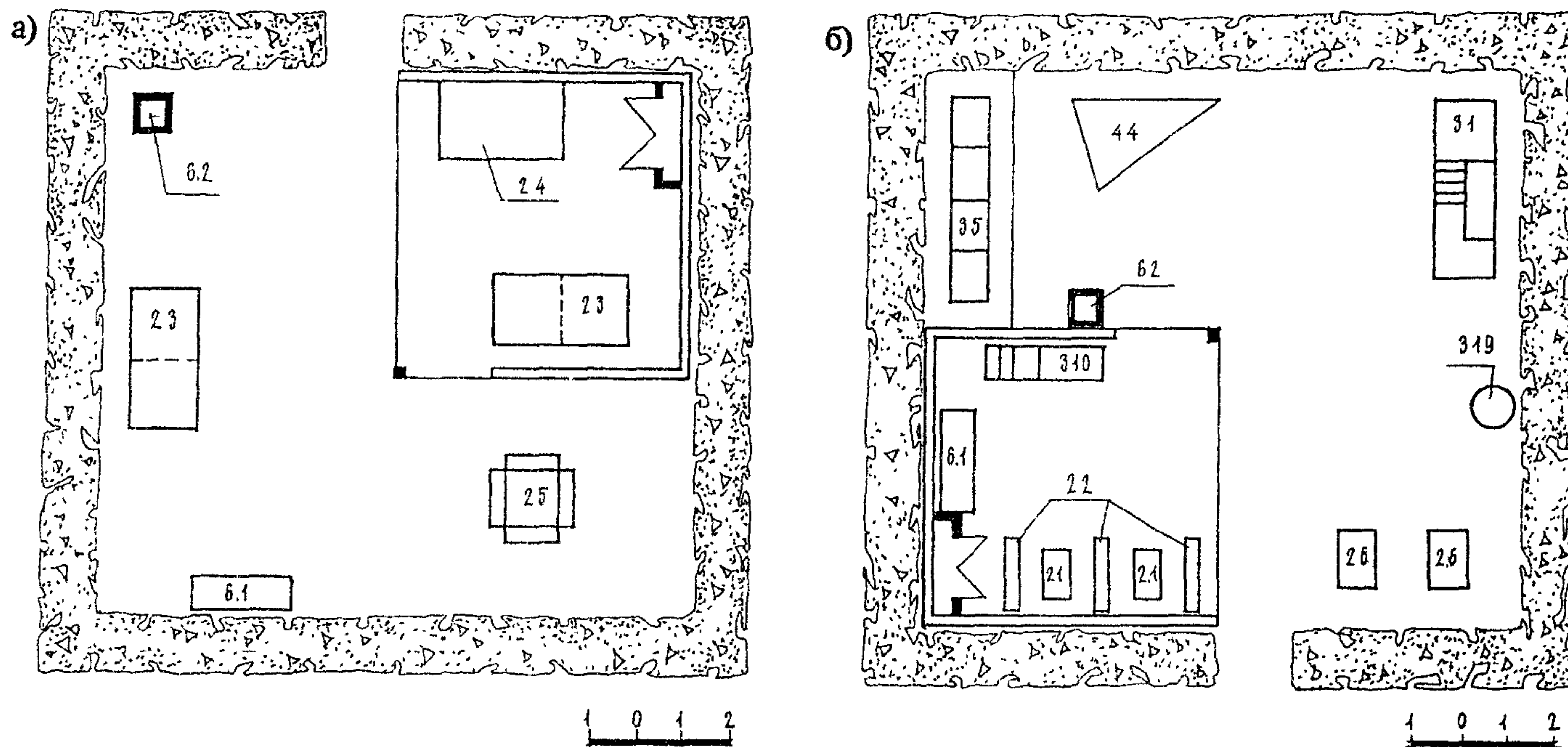
Рис. 3 Размещение оборудования на групповых площадках а - детей 0-1 года; б - детей 1-2 лет
