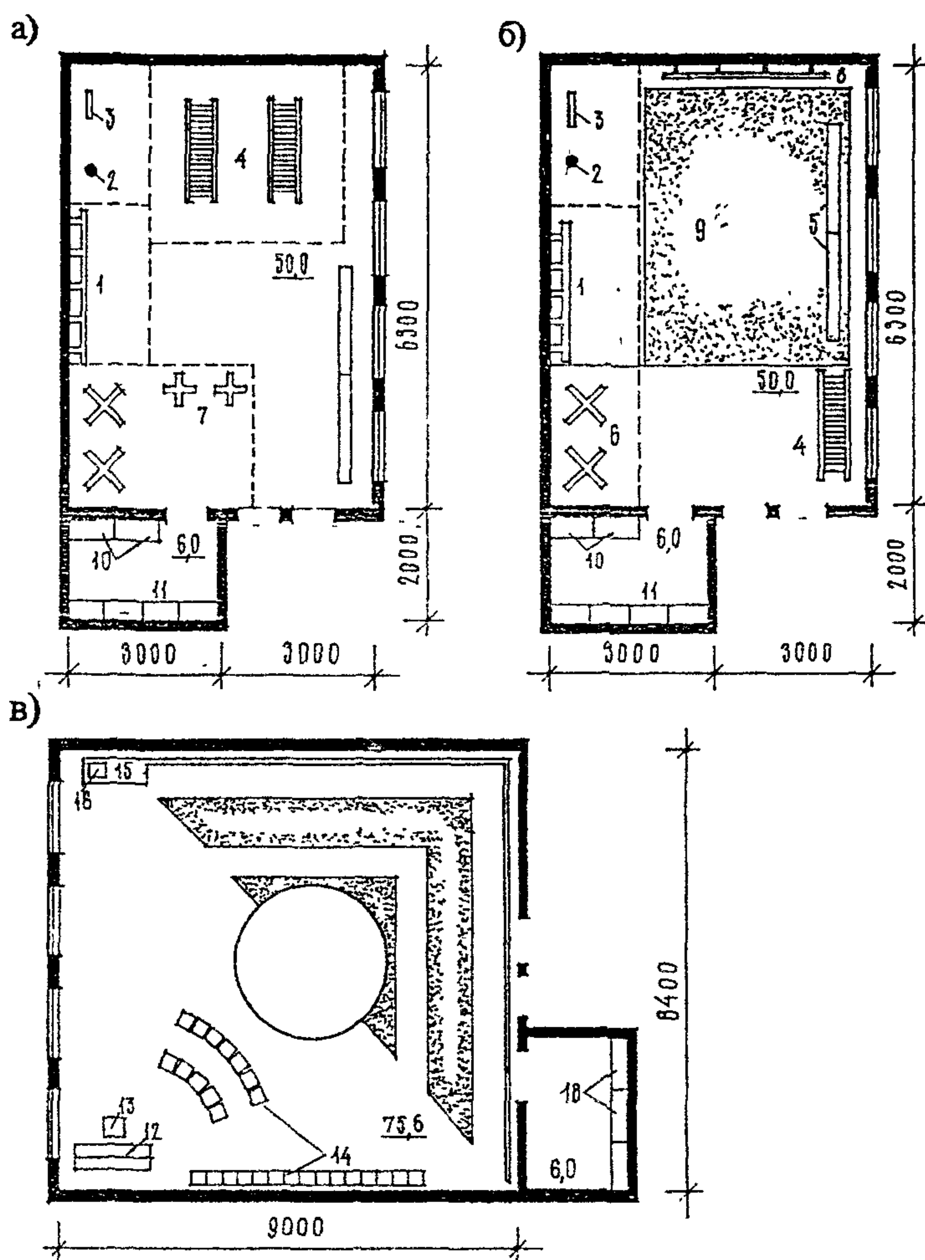
Рис. 41 Расстановка оборудования в залах для музыкальных и физкультурных занятий компенсирующих дошкольных учреждений
