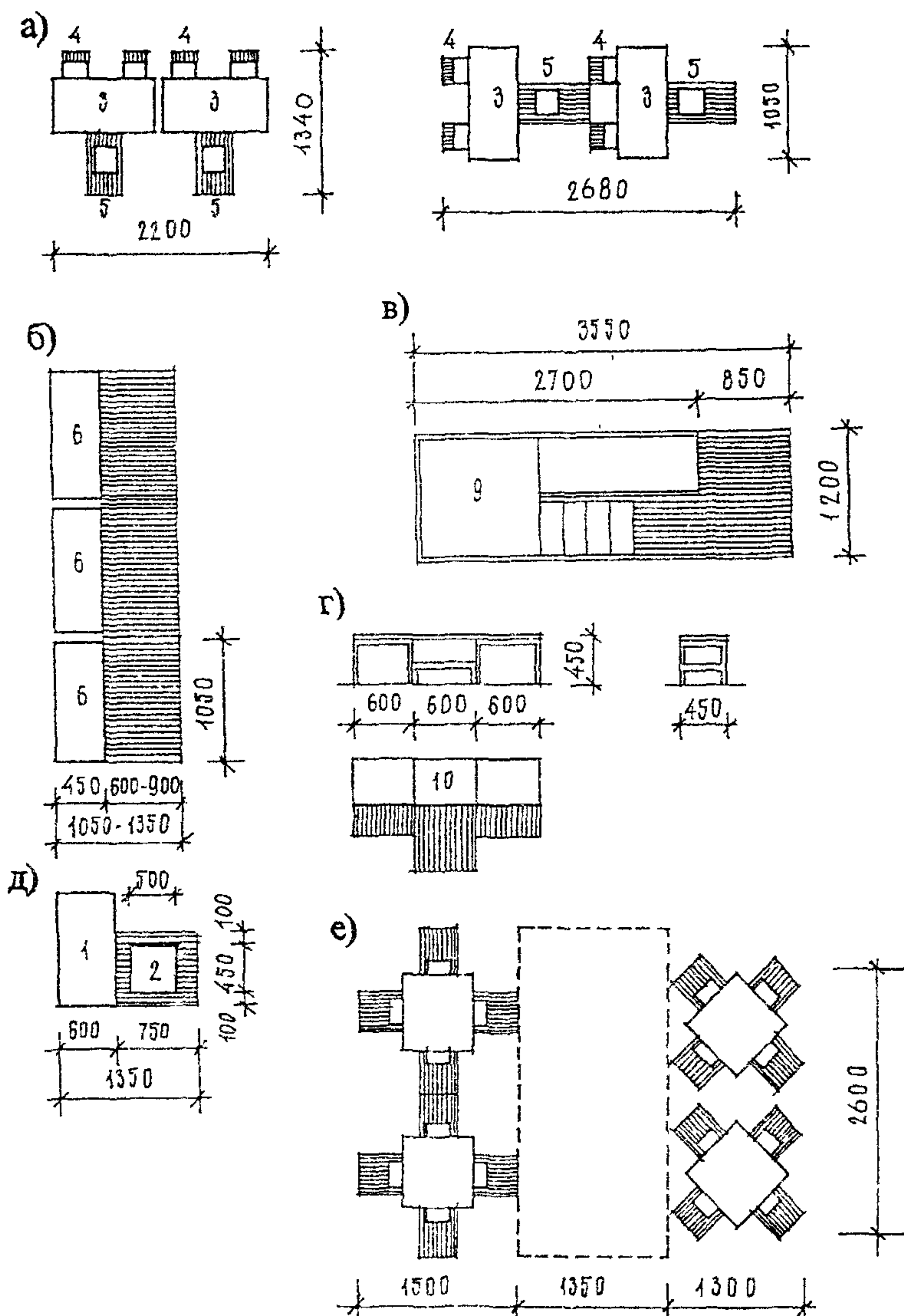
Рис. 28 Различные схемы размещения мебели в функциональных зонах групповой детей 1-2 лет
