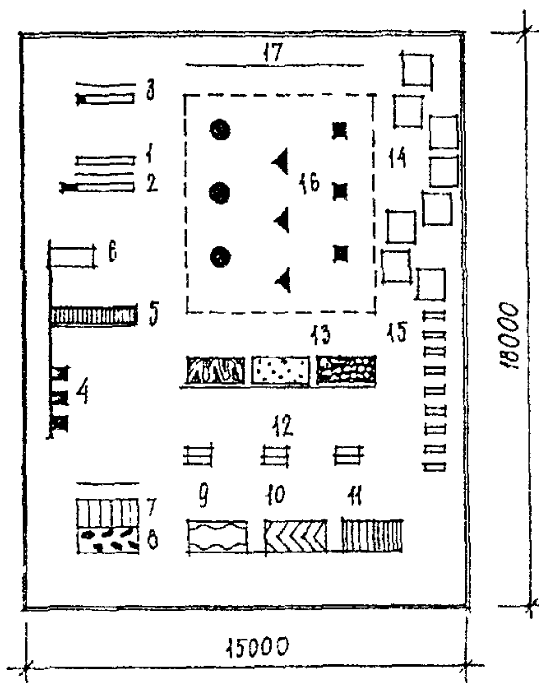
Рис. 13 Лечебно-гимнастическая площадка для детей с нарушением зрения
