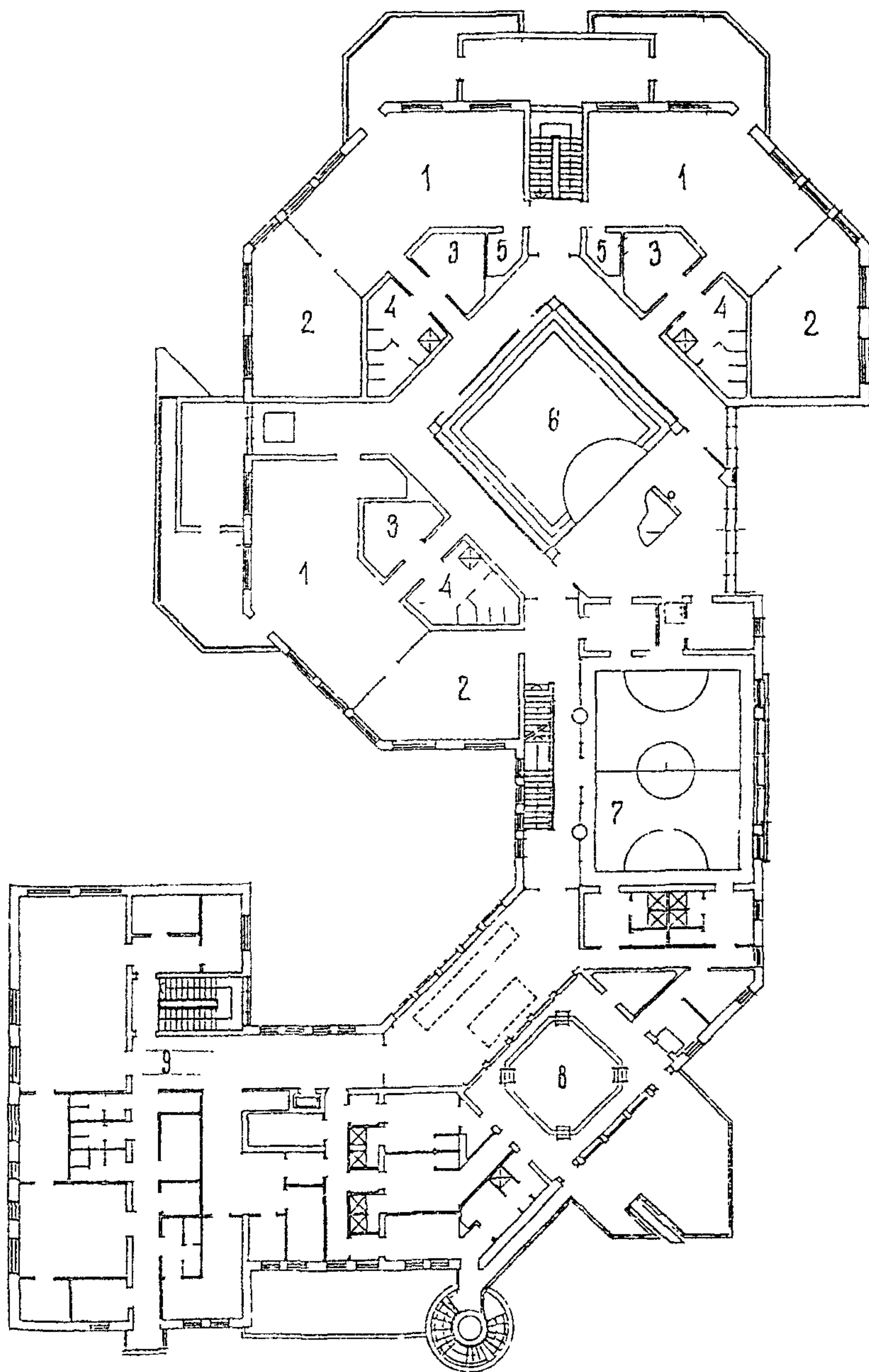
Рис. 53 ЦДВ на 6 групп. Арх. Л.Смывина, Б. Гранцев.
