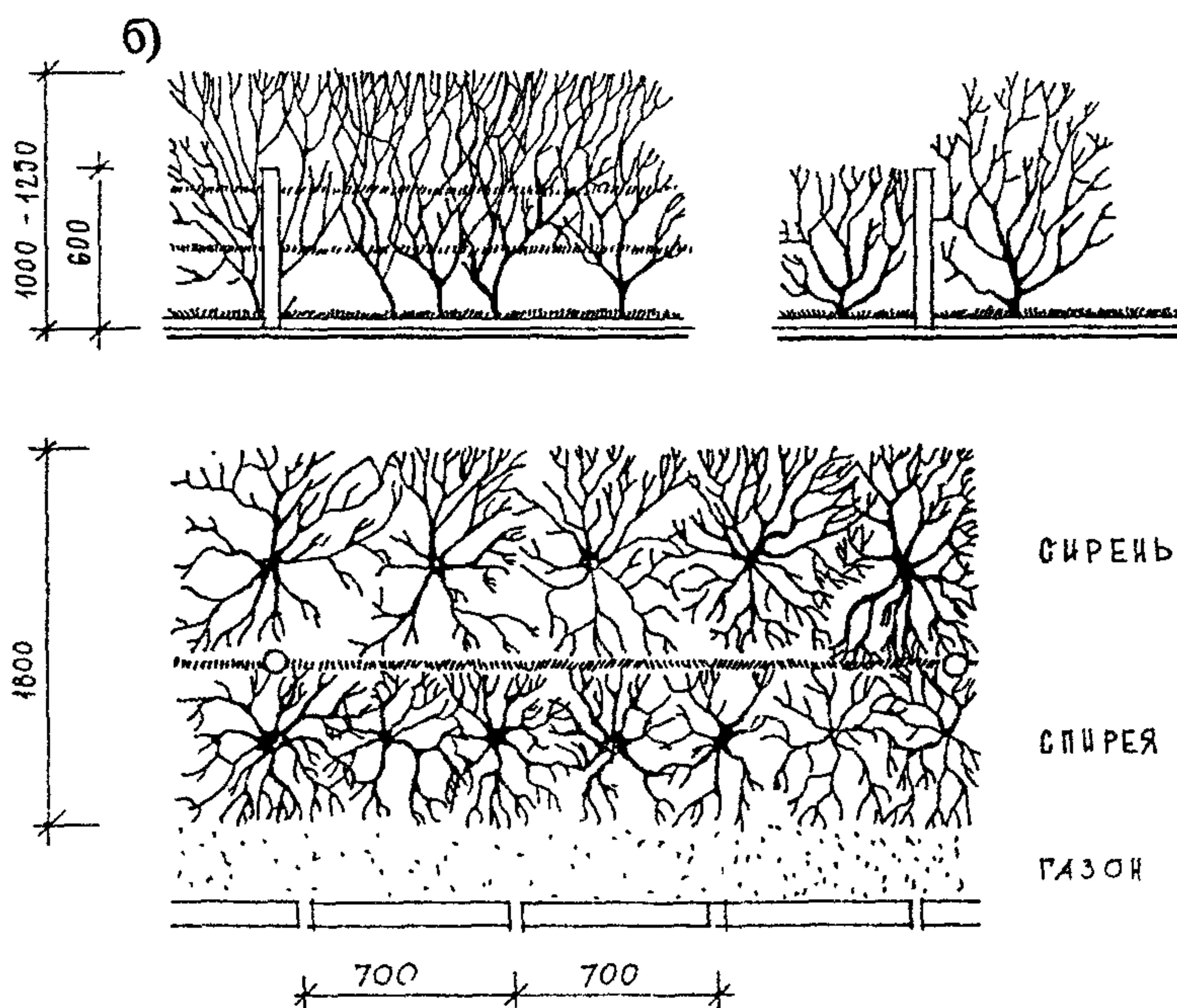
Рис. 19 Посадка кустарников и организация живой изгороди а - однорядная; б - двухрядная
