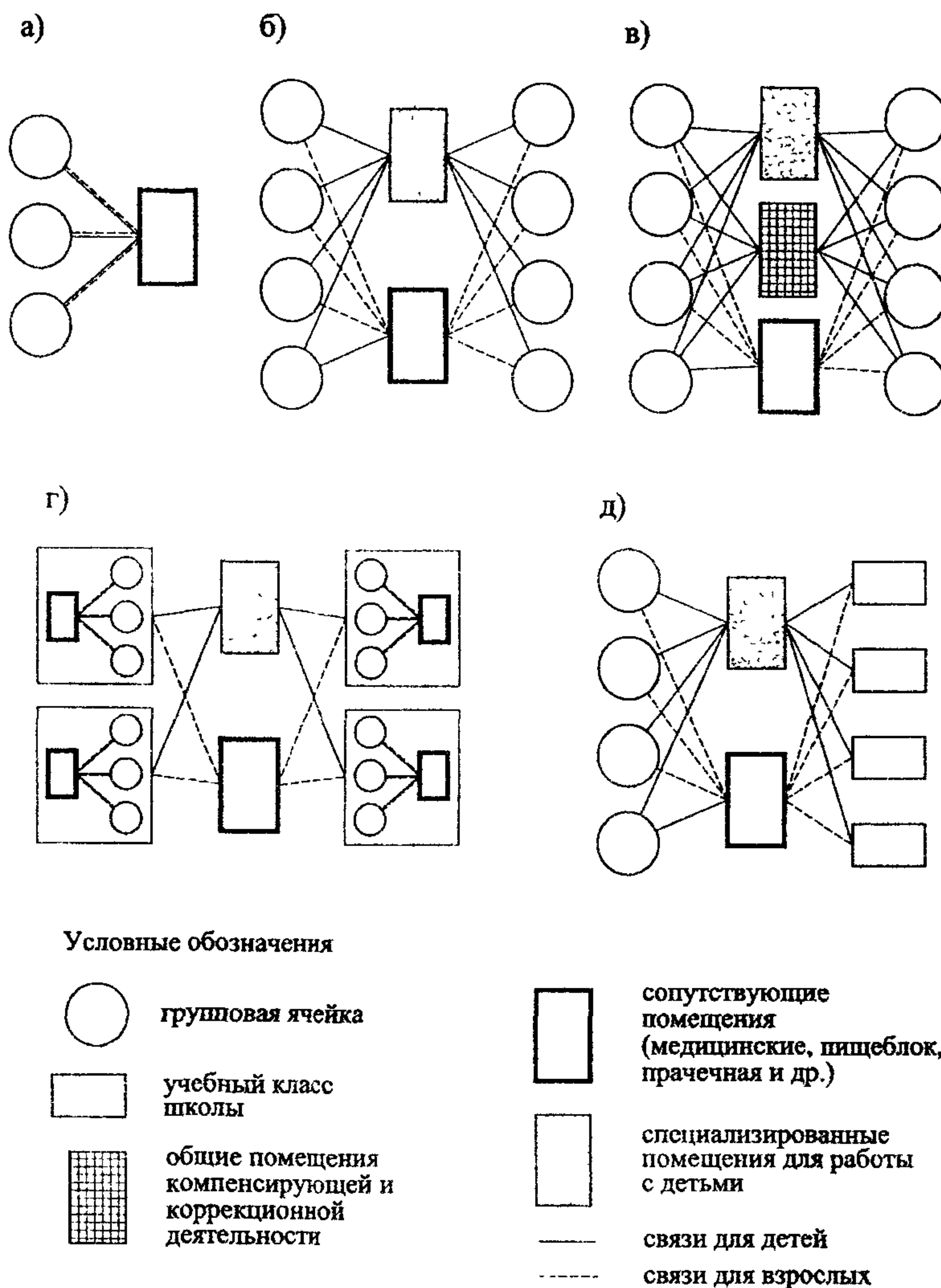
Рис. 21 . Функциональная структура дошкольных образовательных учреждений (состав и взаимосвязь функциональных элементов): а - малые ДОУ; б - ДОУ общего типа; в - ДОУ компенсирующего вида; г - КДВ; д - детский сад - начальная школа
