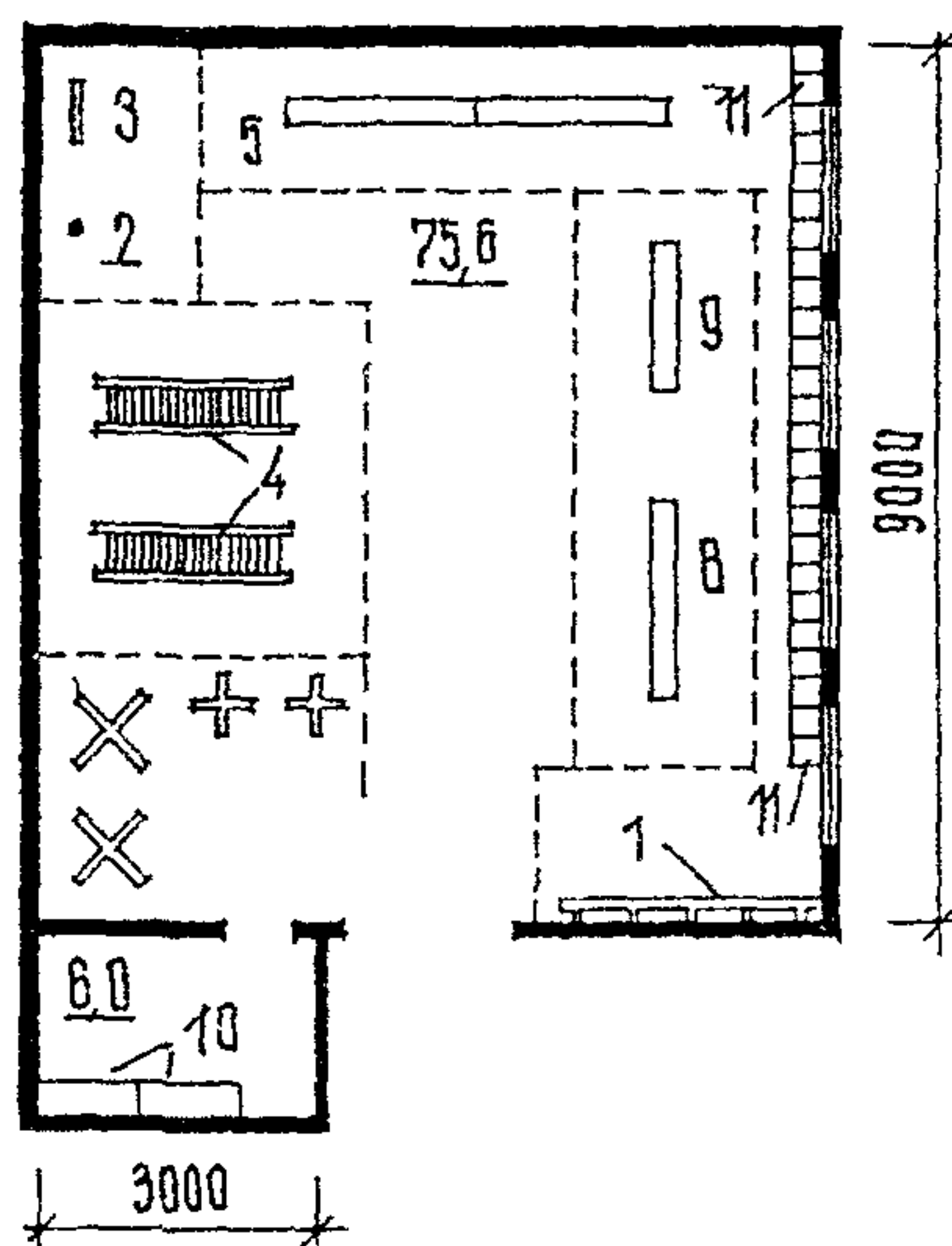
Рис. 40 Расстановка оборудования в залах для музыкальных и физкультурных занятий
