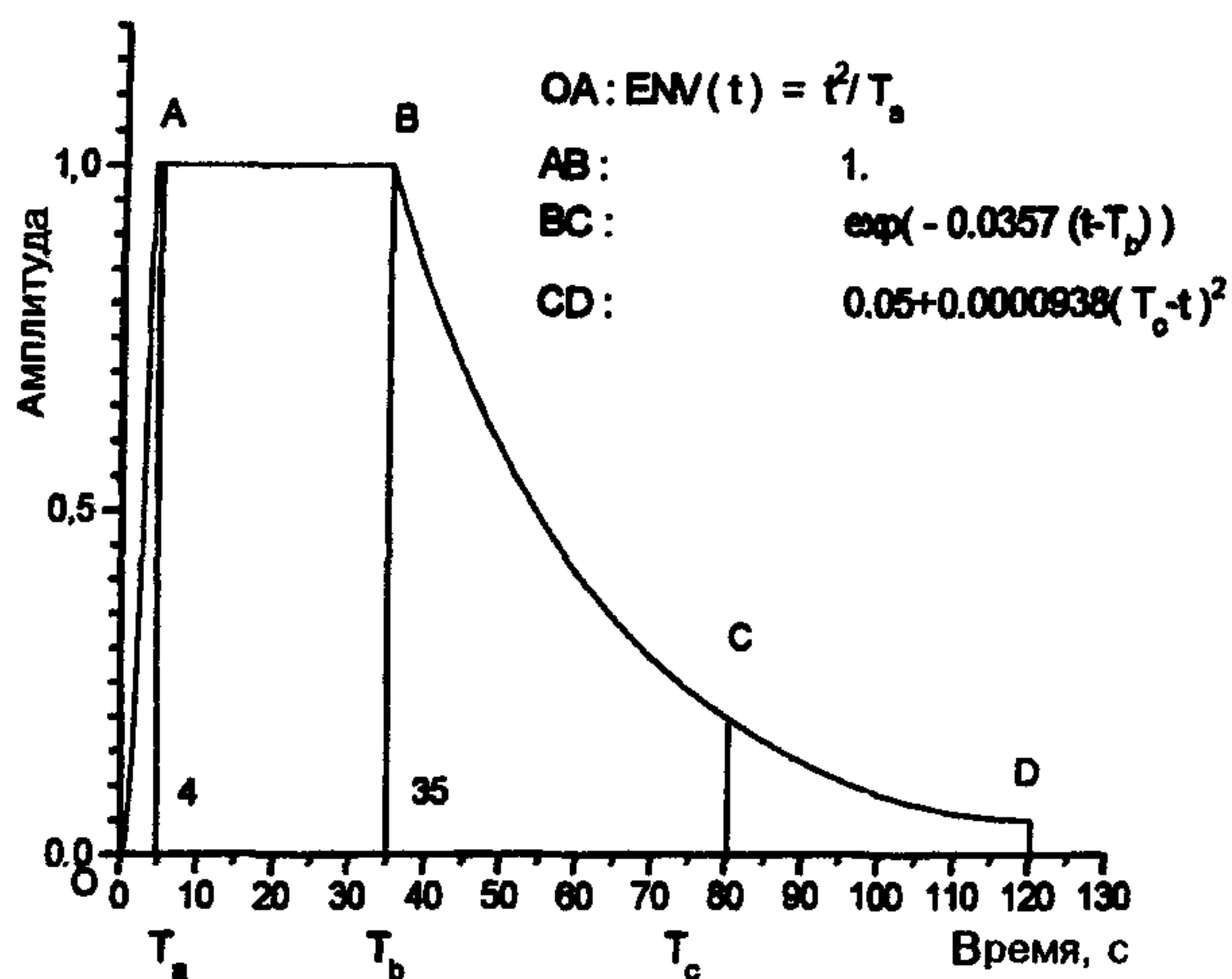
Рис. 3. Форма амплитуды огибающей колебаний
