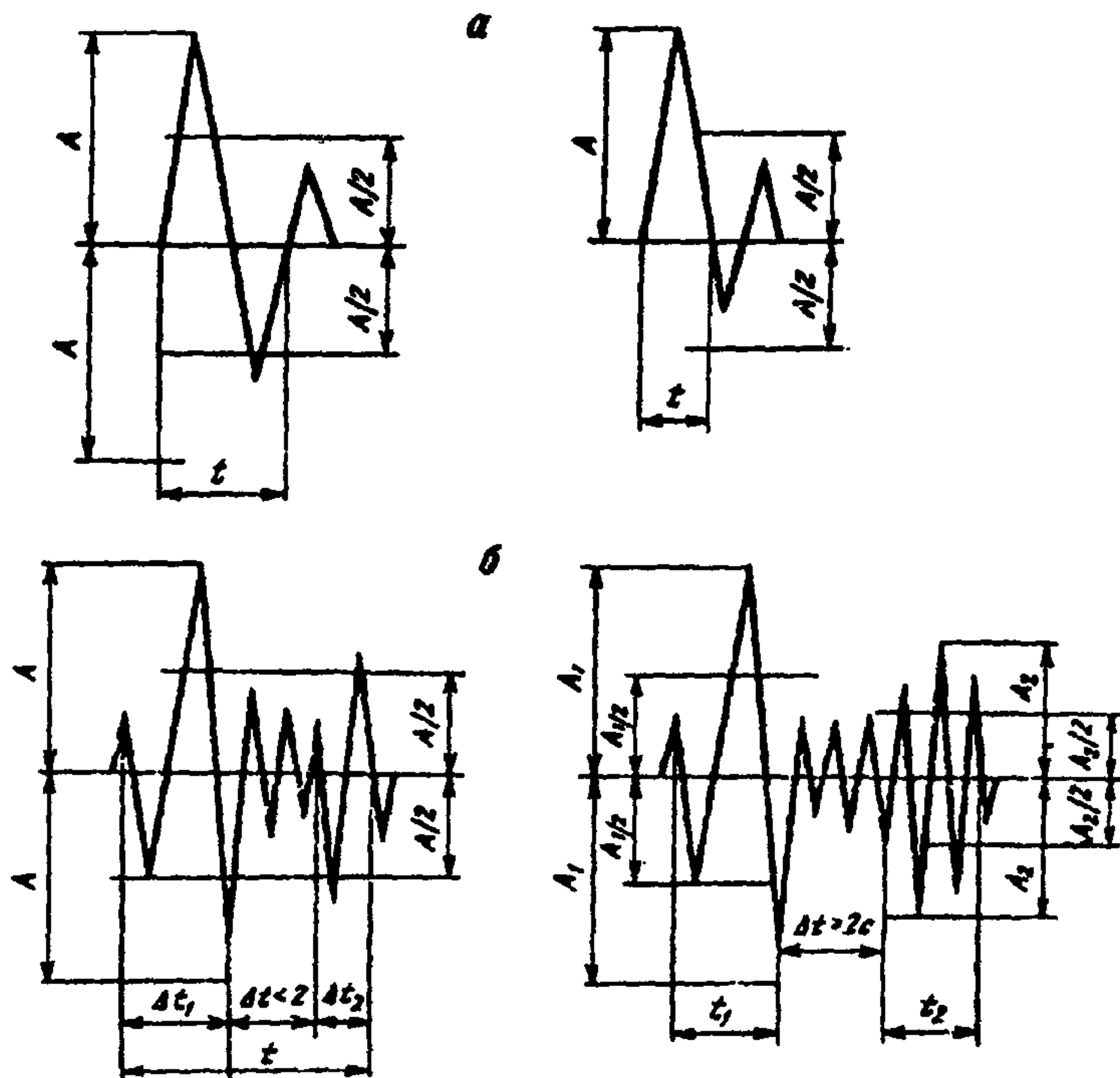
Рис. 1.3. Схема измерения ширины импульса: a — для простых колебаний; б — для колебаний сложной формы
