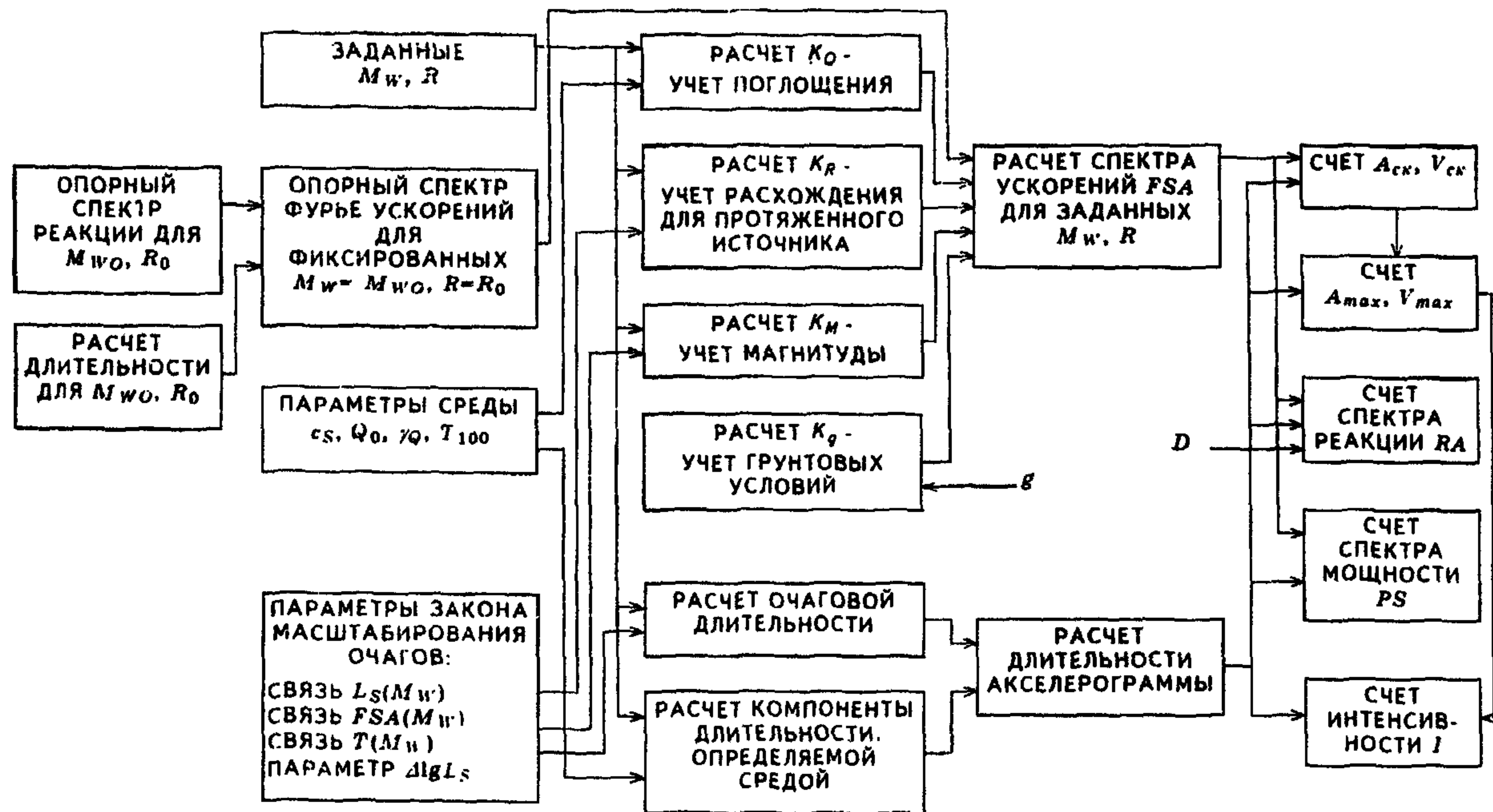
Рис. 2.2. Блок-схема алгоритма моделирования параметров колебаний грунта
