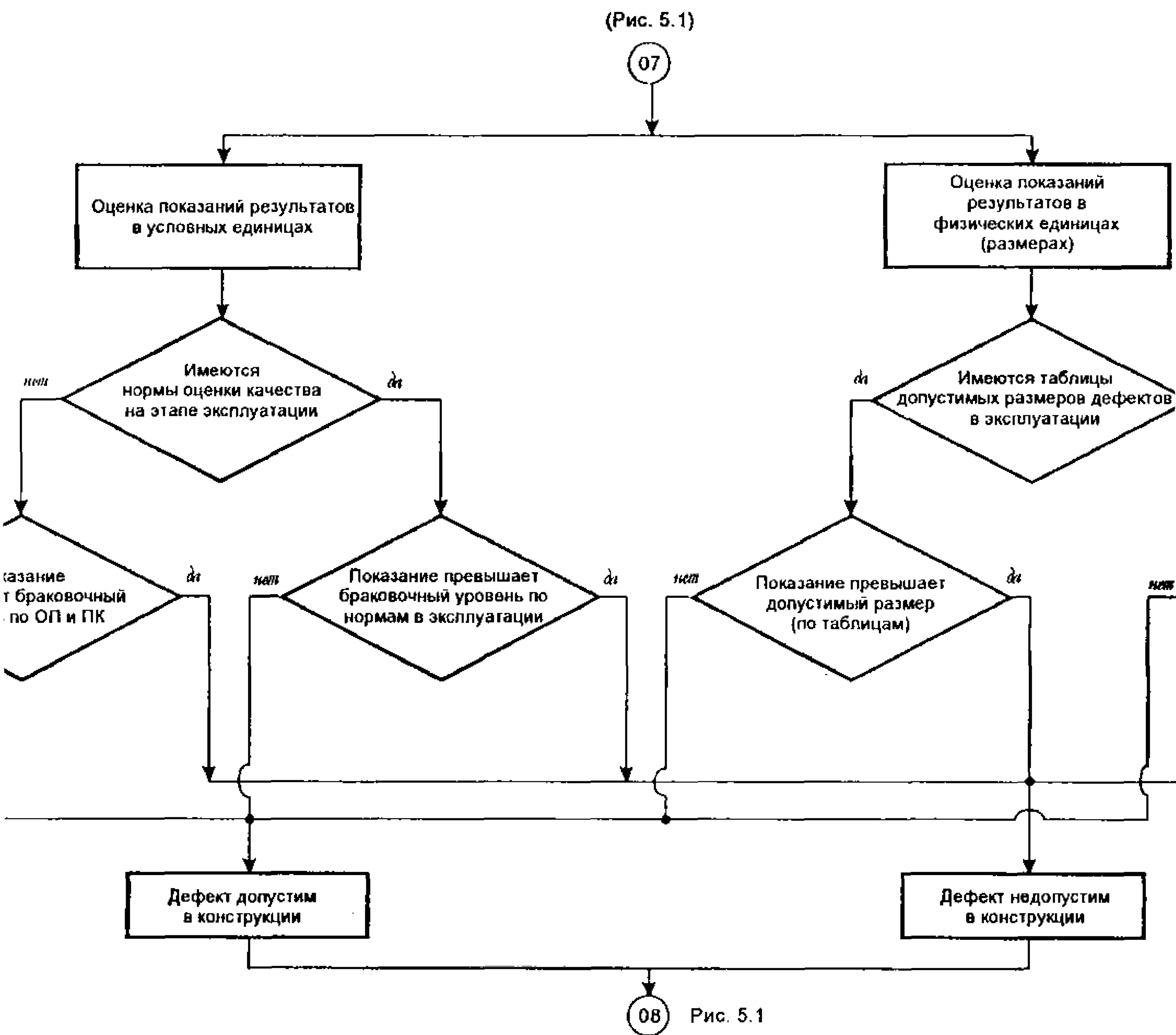
Рис. 5.2. Схема оценки допустимости дефекта по результатам НК (в кружках указаны номера этапов работ)
