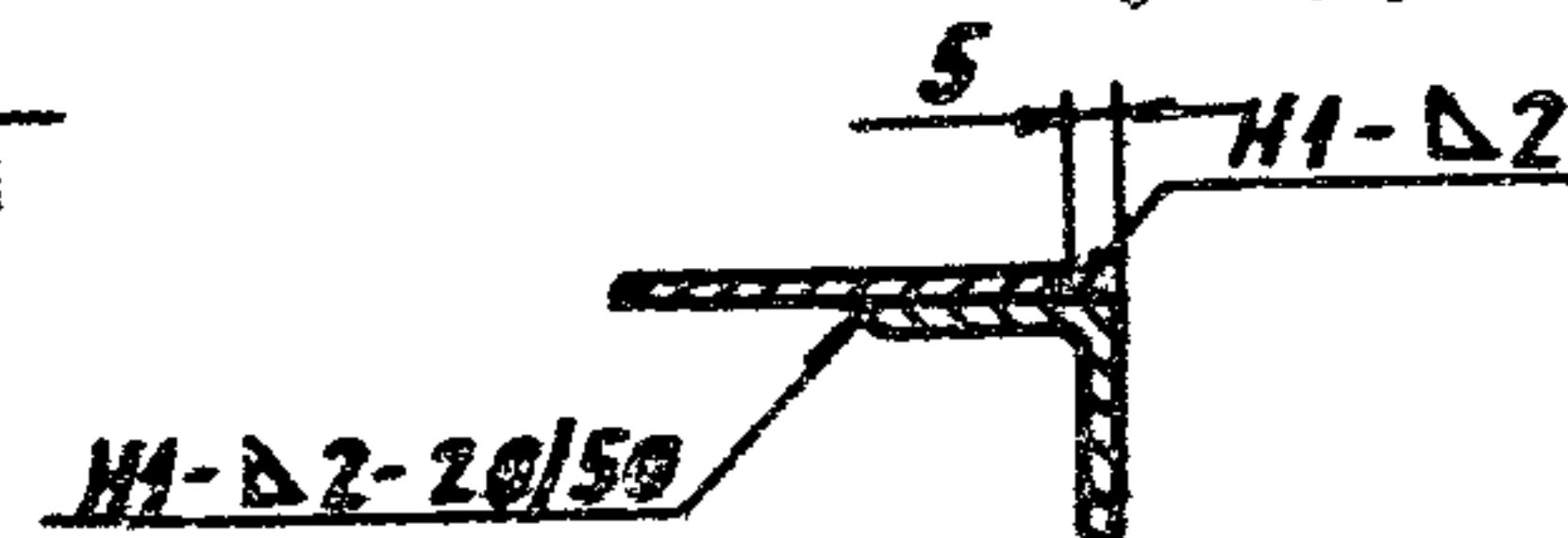
Б-Б (125)
