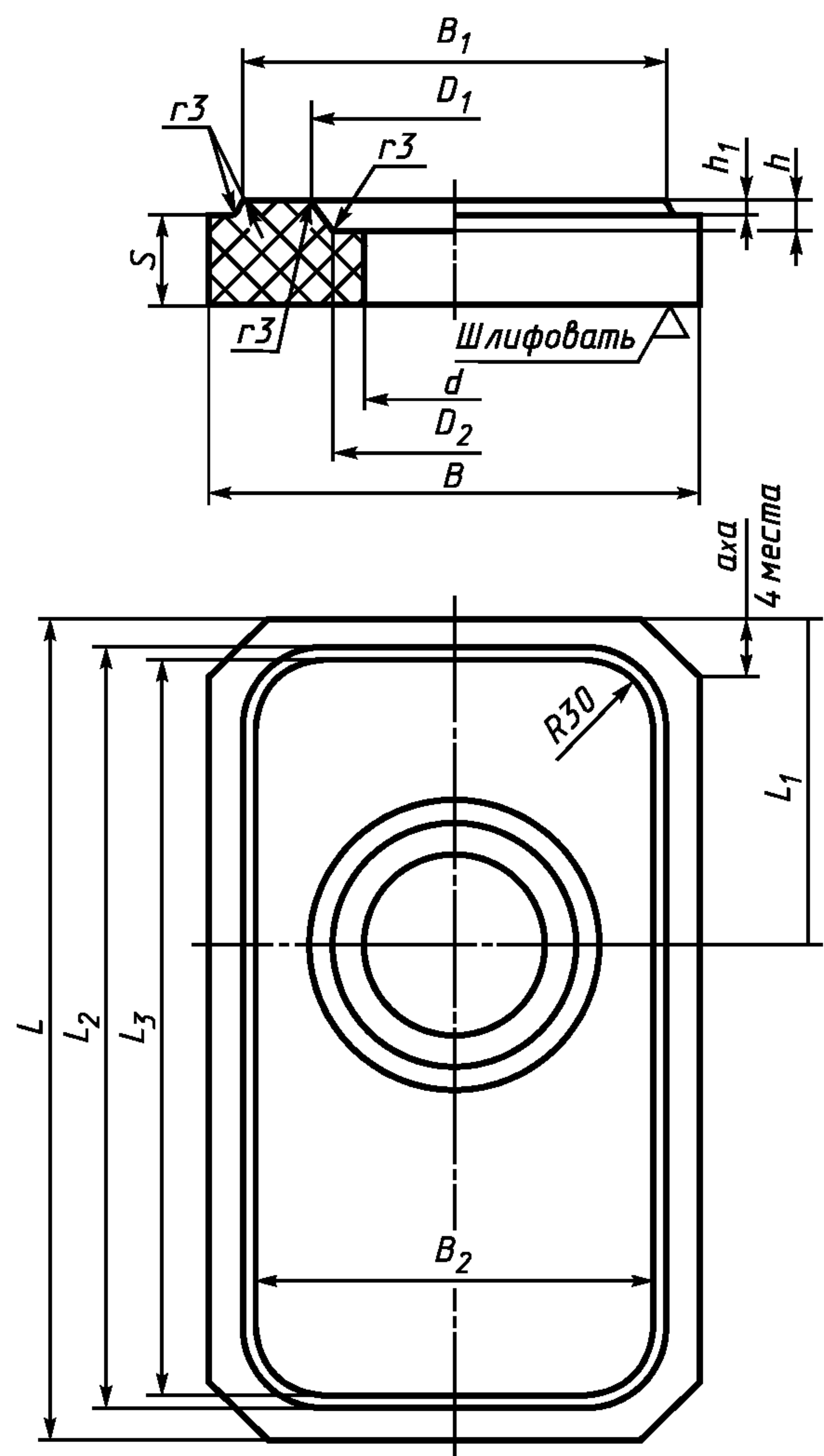
Рисунок 3 — Плита номер 13
