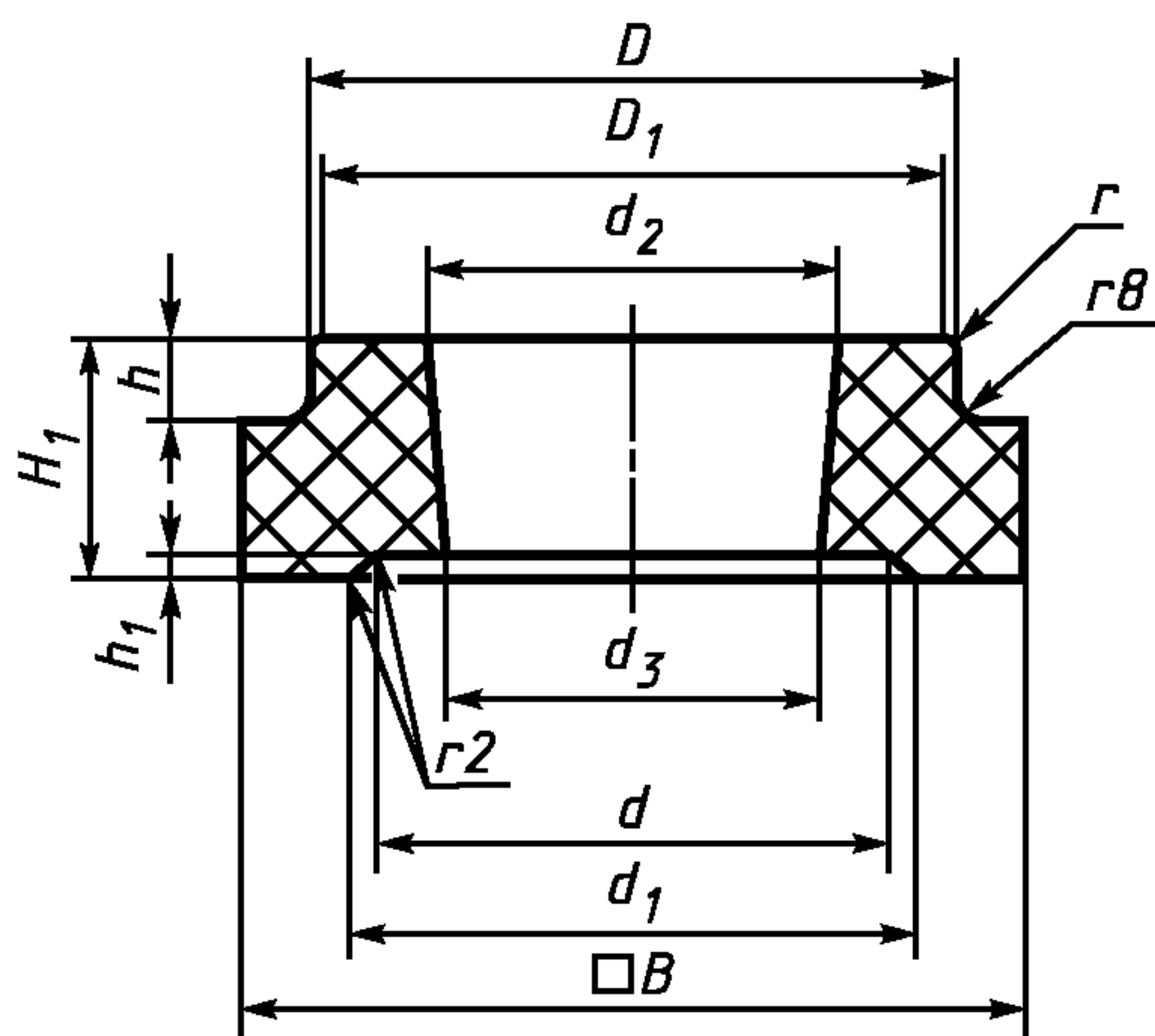
Рисунок 27 — Гнездовой кирпич номер 13 (нижняя часть)
