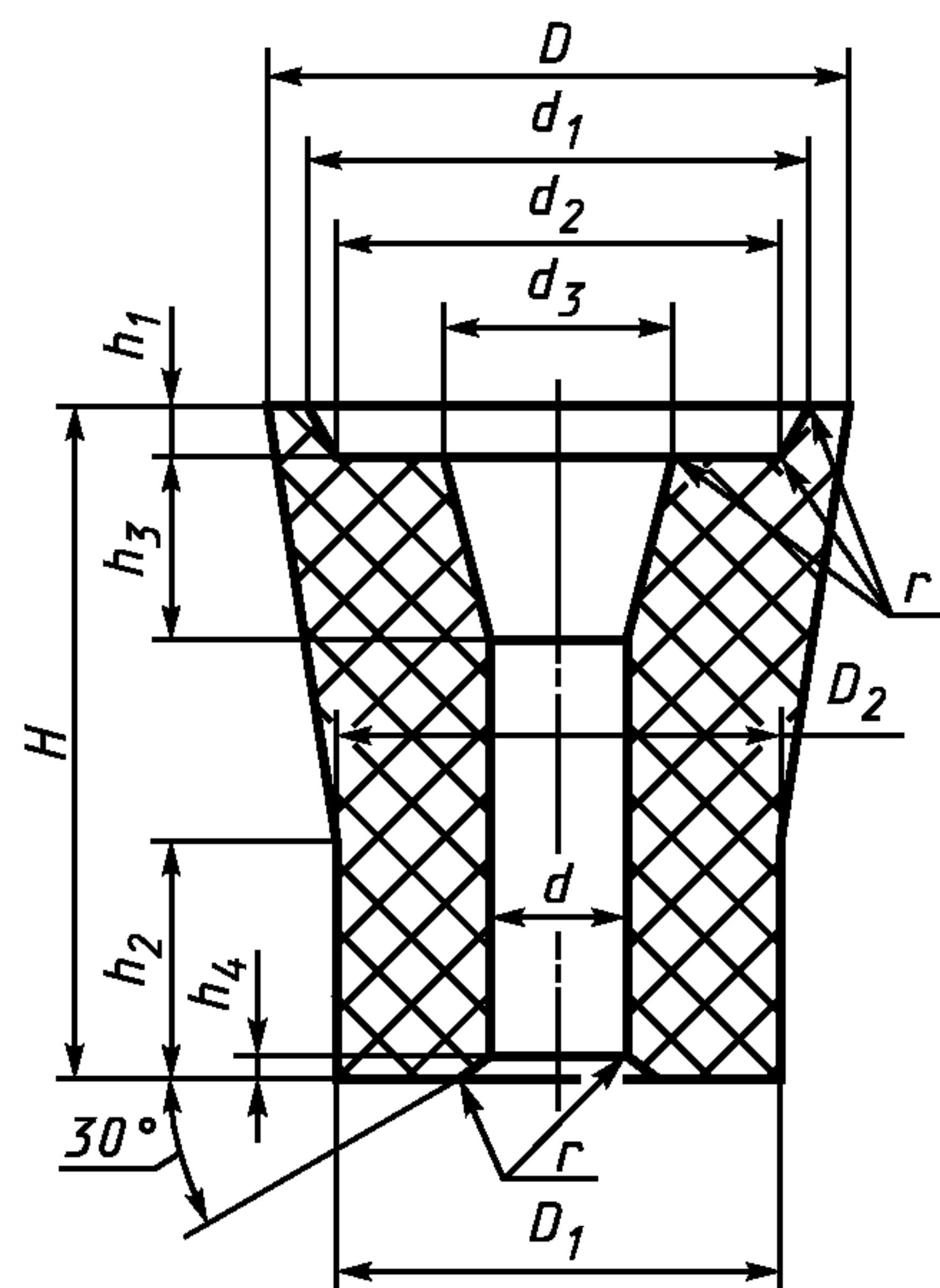
Рисунок 12 — Стакан-коллектор номер 18
