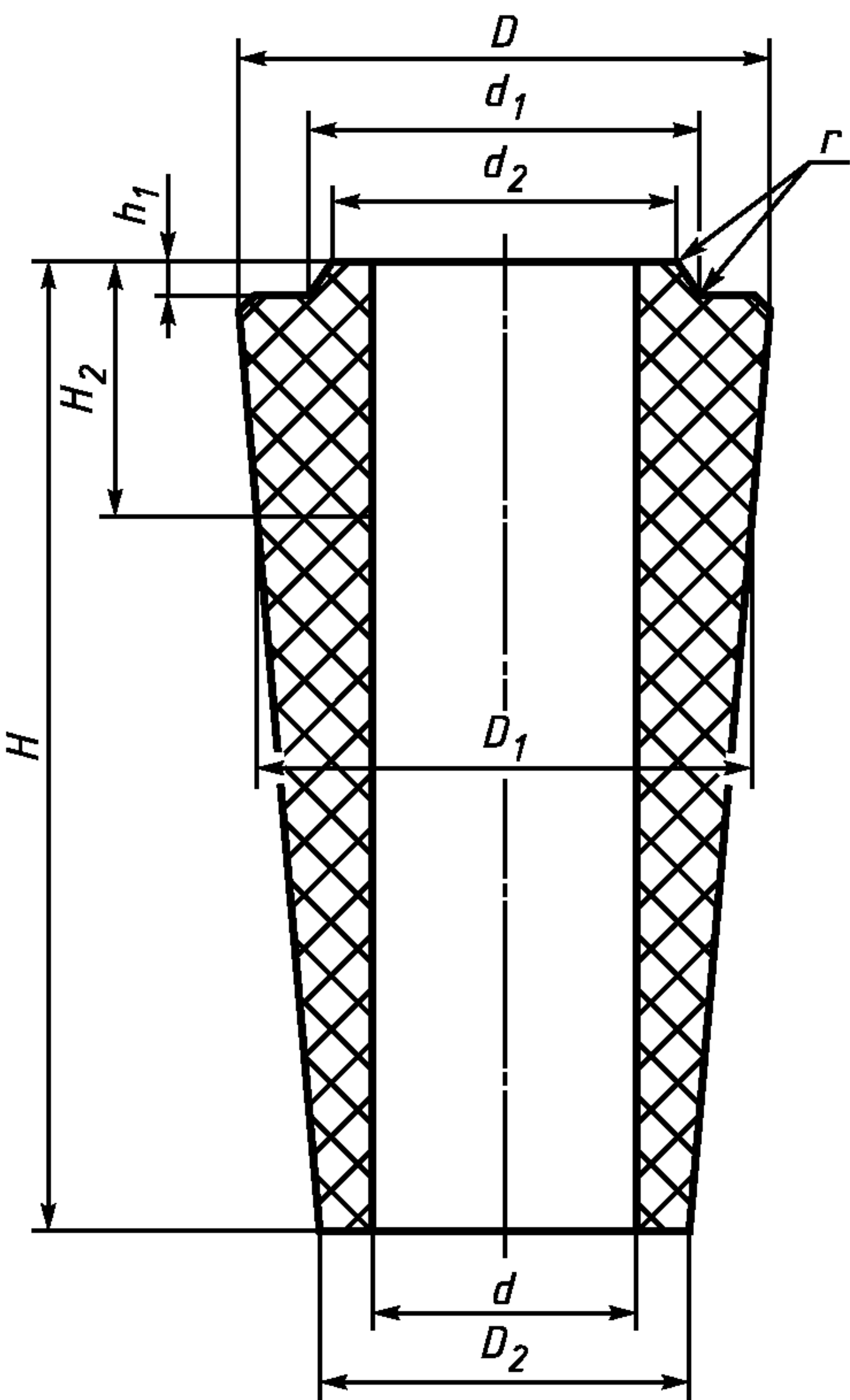
Рисунок 13 — Стакан-коллектор номеров 19 и 20
