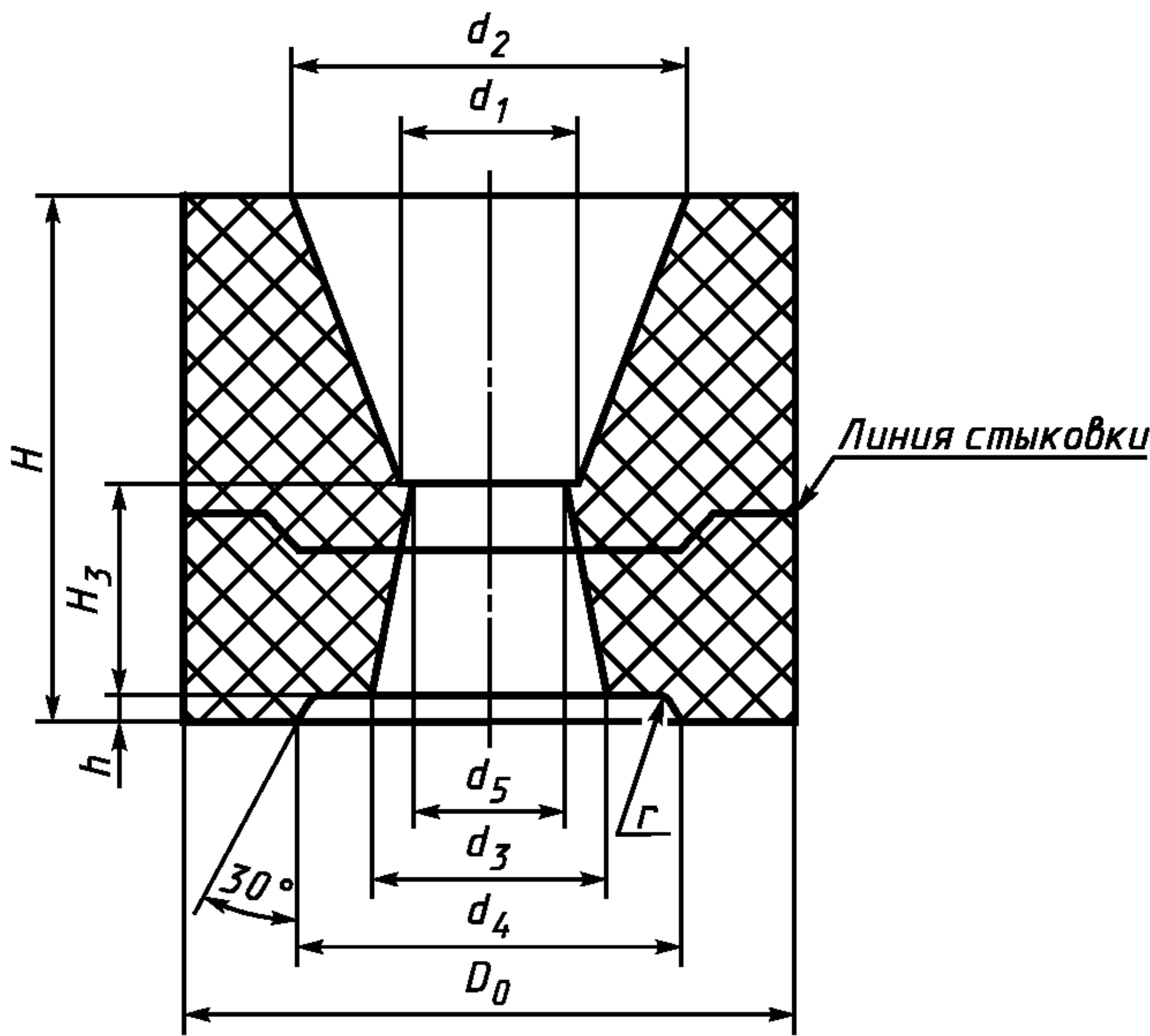
Рисунок 24 — Гнездовой кирпич номер 10
