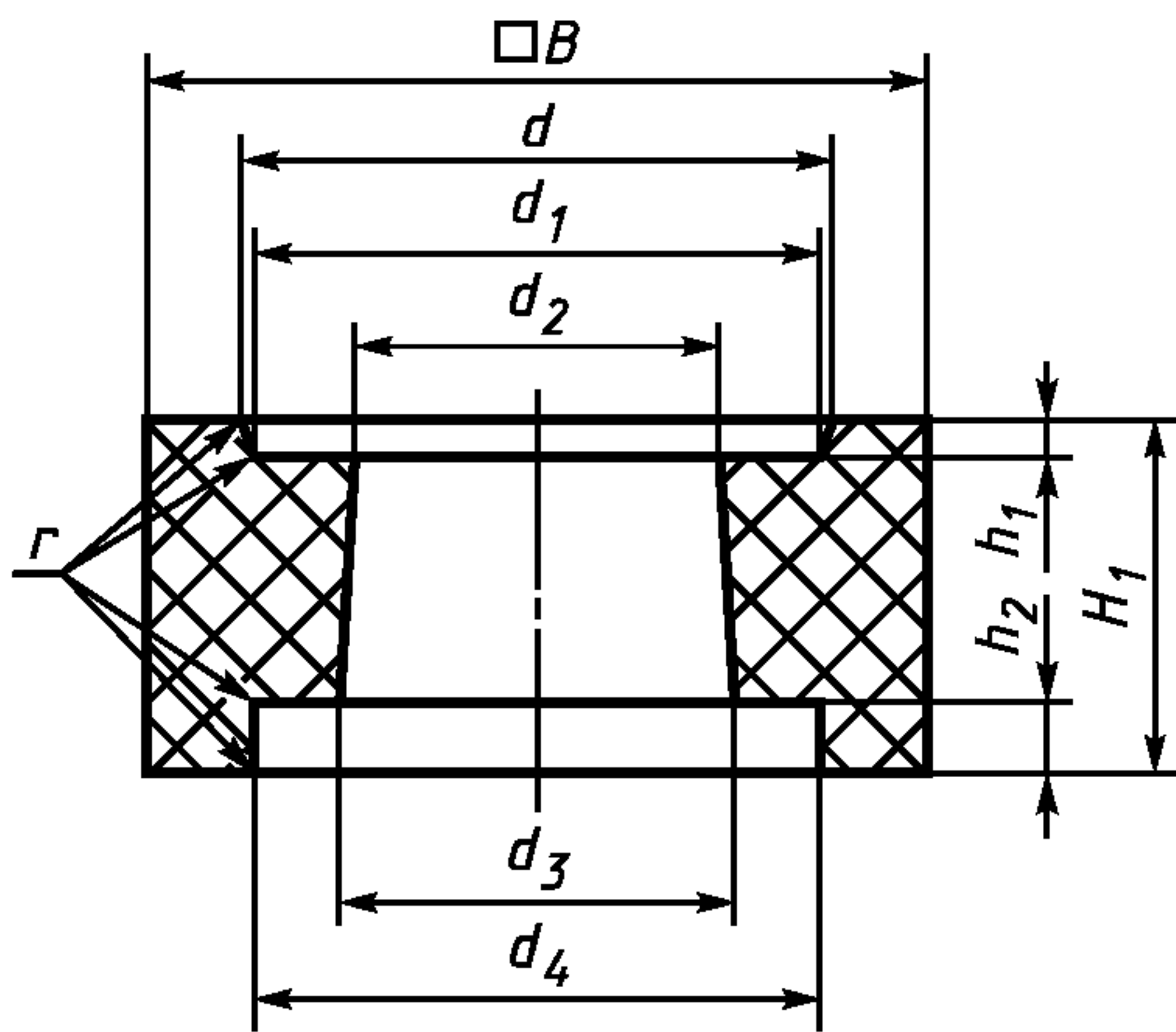
Рисунок 20 — Гнездовой кирпич номер 5 (нижняя часть)
