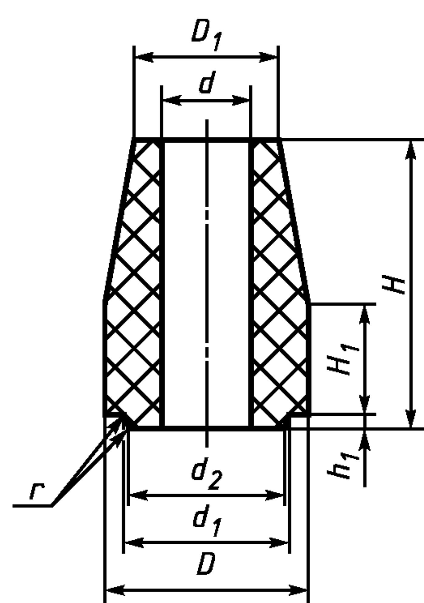
Рисунок 9 — Стакан и стакан-коллектор номеров 9-1 и 9-2
