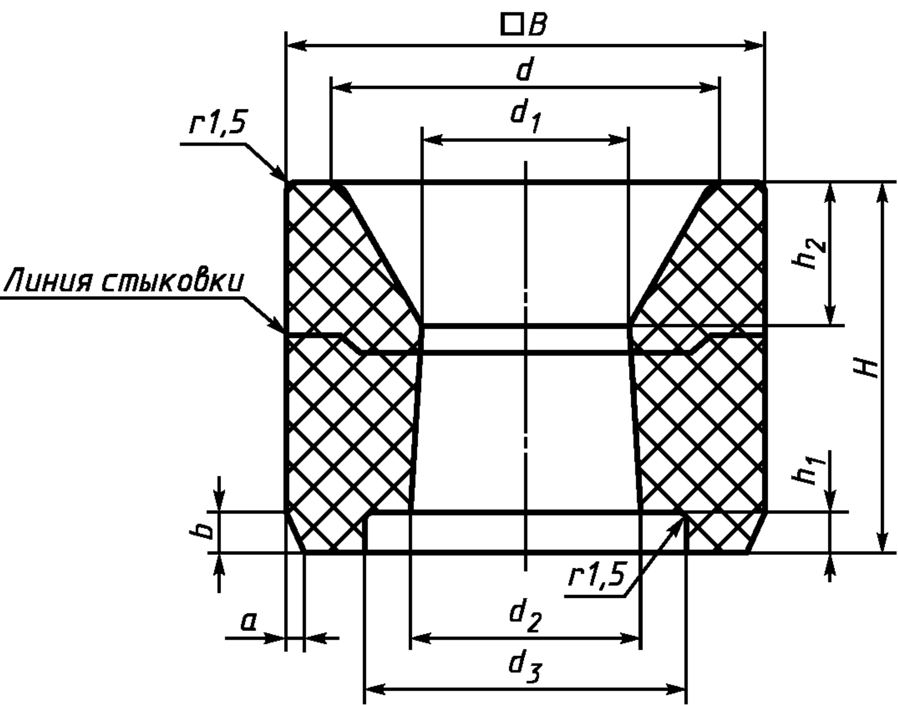
Рисунок 25 — Гнездовой кирпич номер 11
