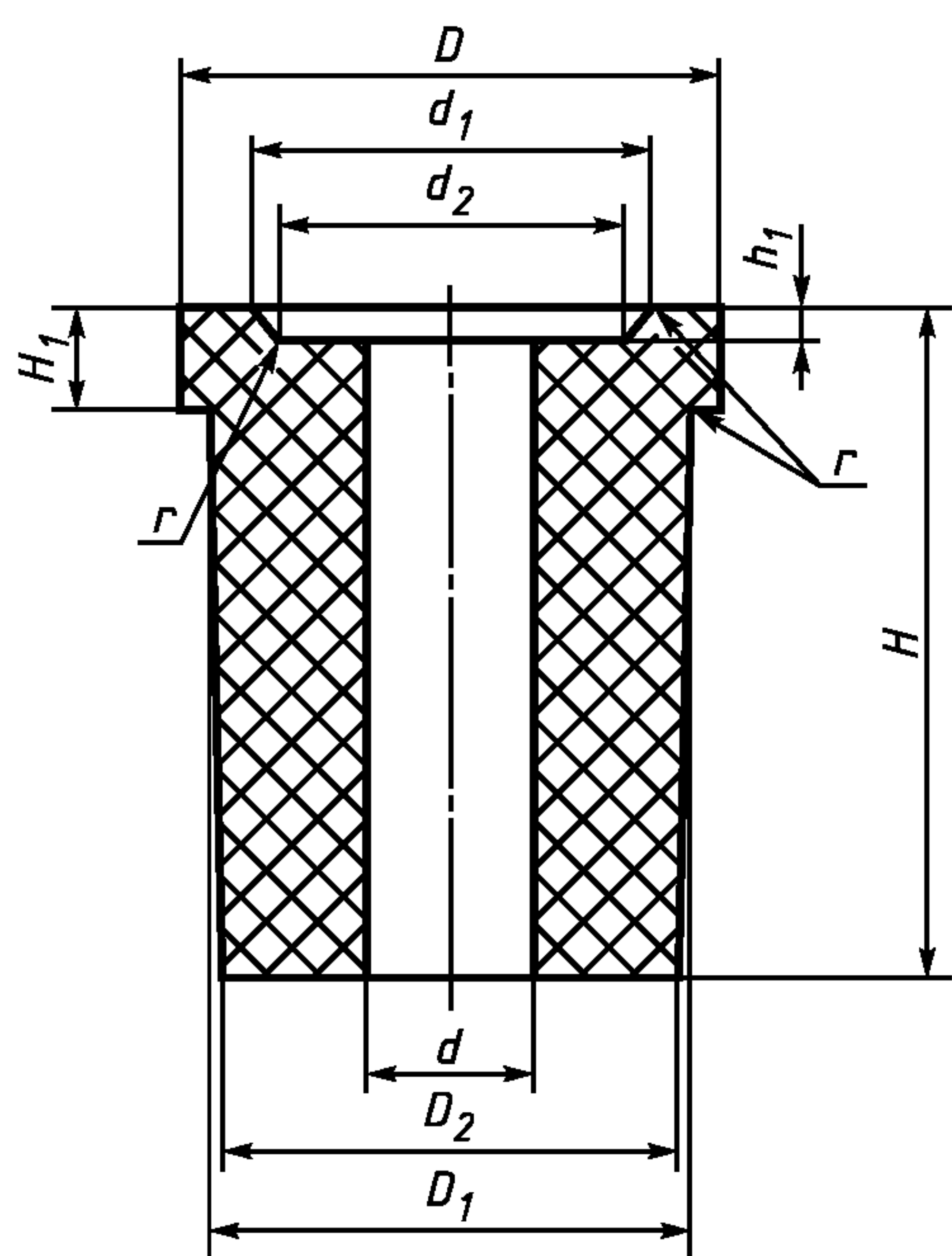
Рисунок 10 — Стакан-коллектор номеров 10—16
