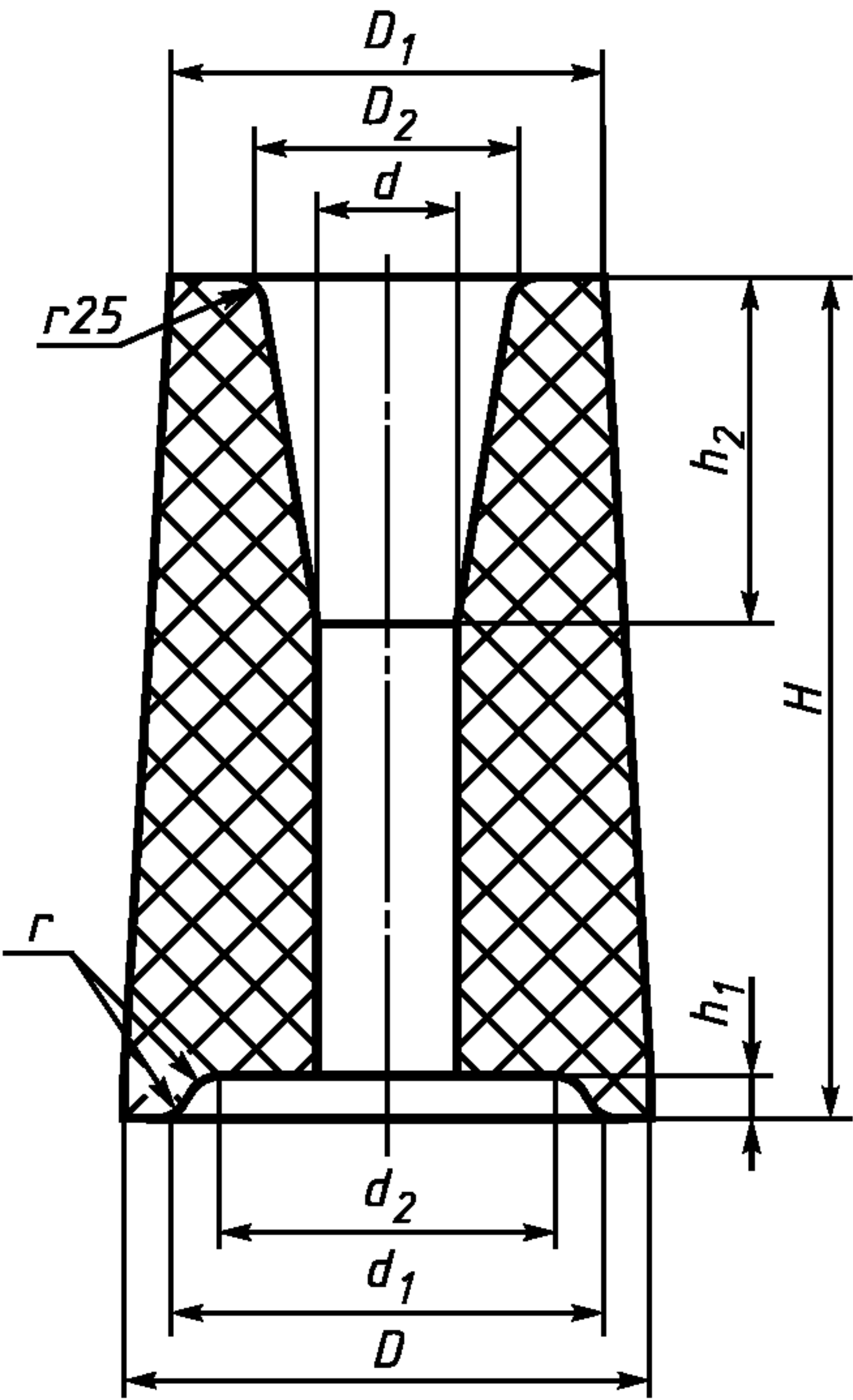
Рисунок 7 — Стакан номеров 8 и 8-1
