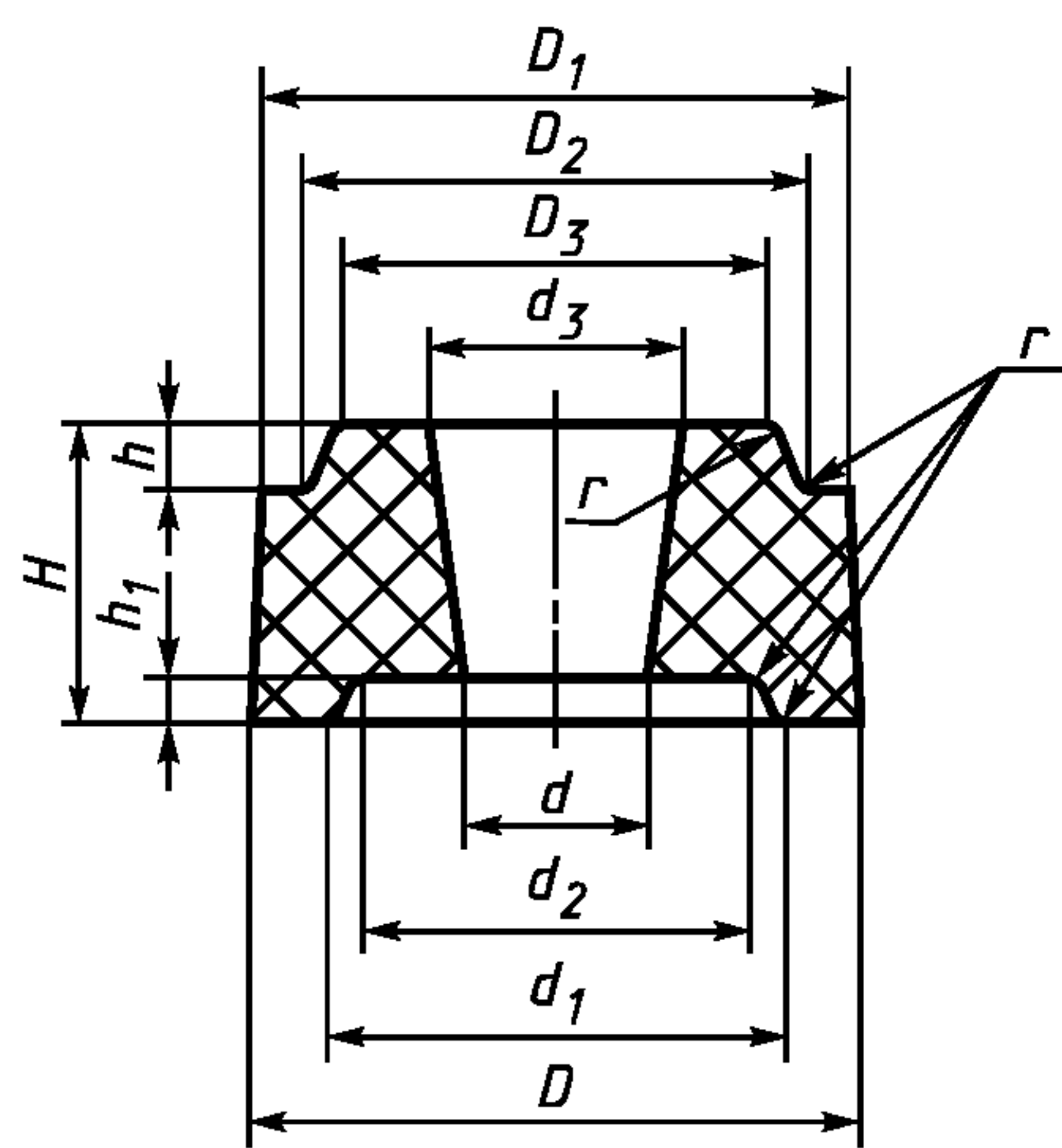
Рисунок 5 — Вставка номеров 1—4
