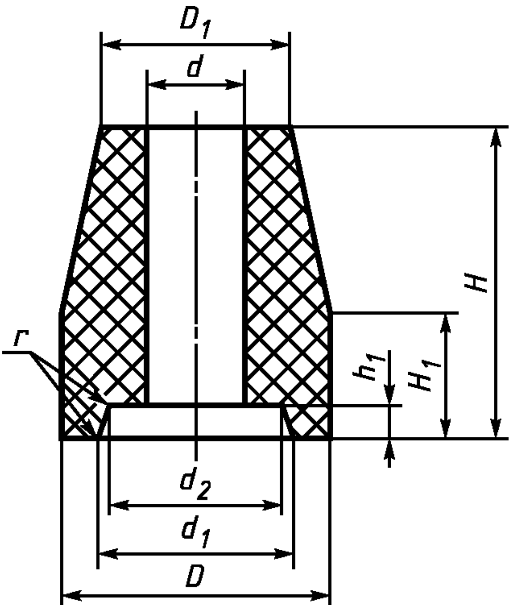
Рисунок 8 — Стакан и стакан-коллектор номер 9
