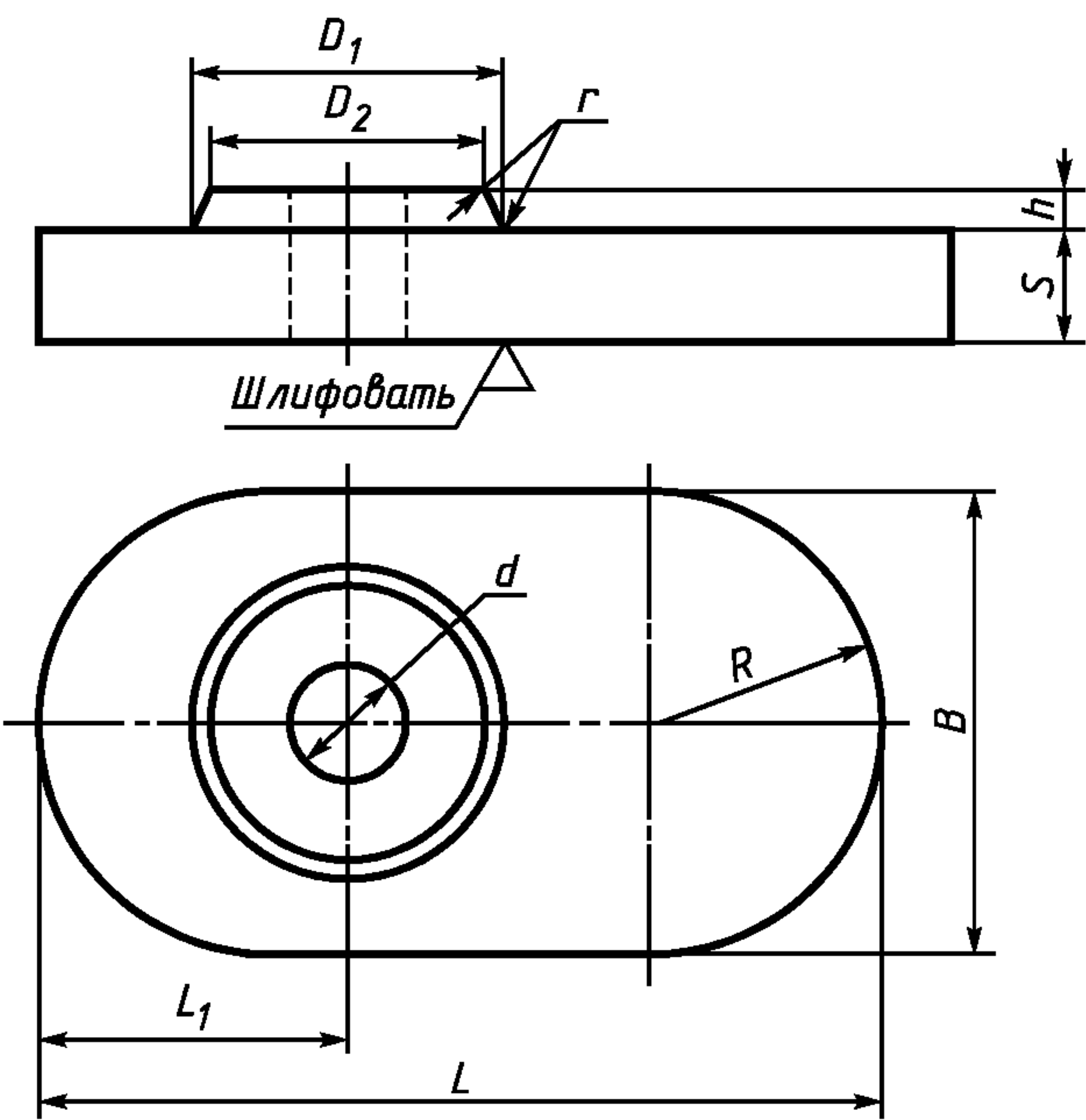
Рисунок 1 — Плита номеров 1—10, 10-1, 10-2, 10-3
