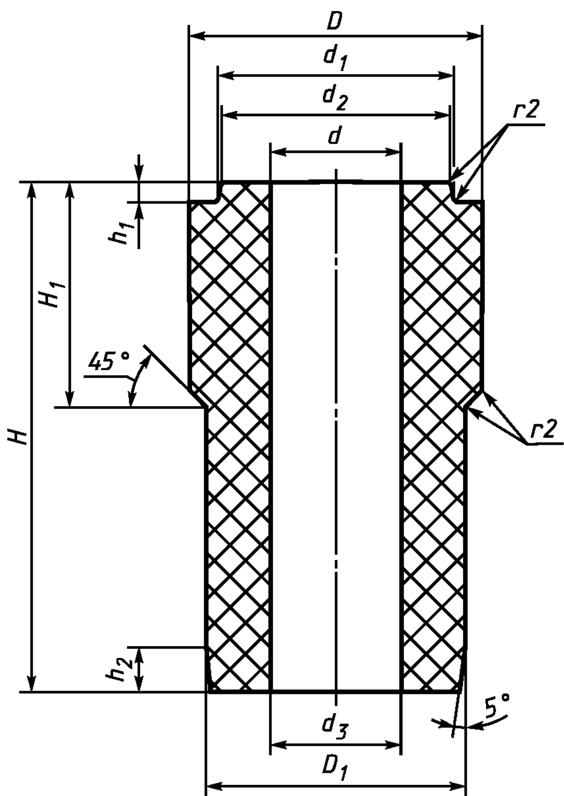
Рисунок 16 — Стакан-коллектор номер 23
