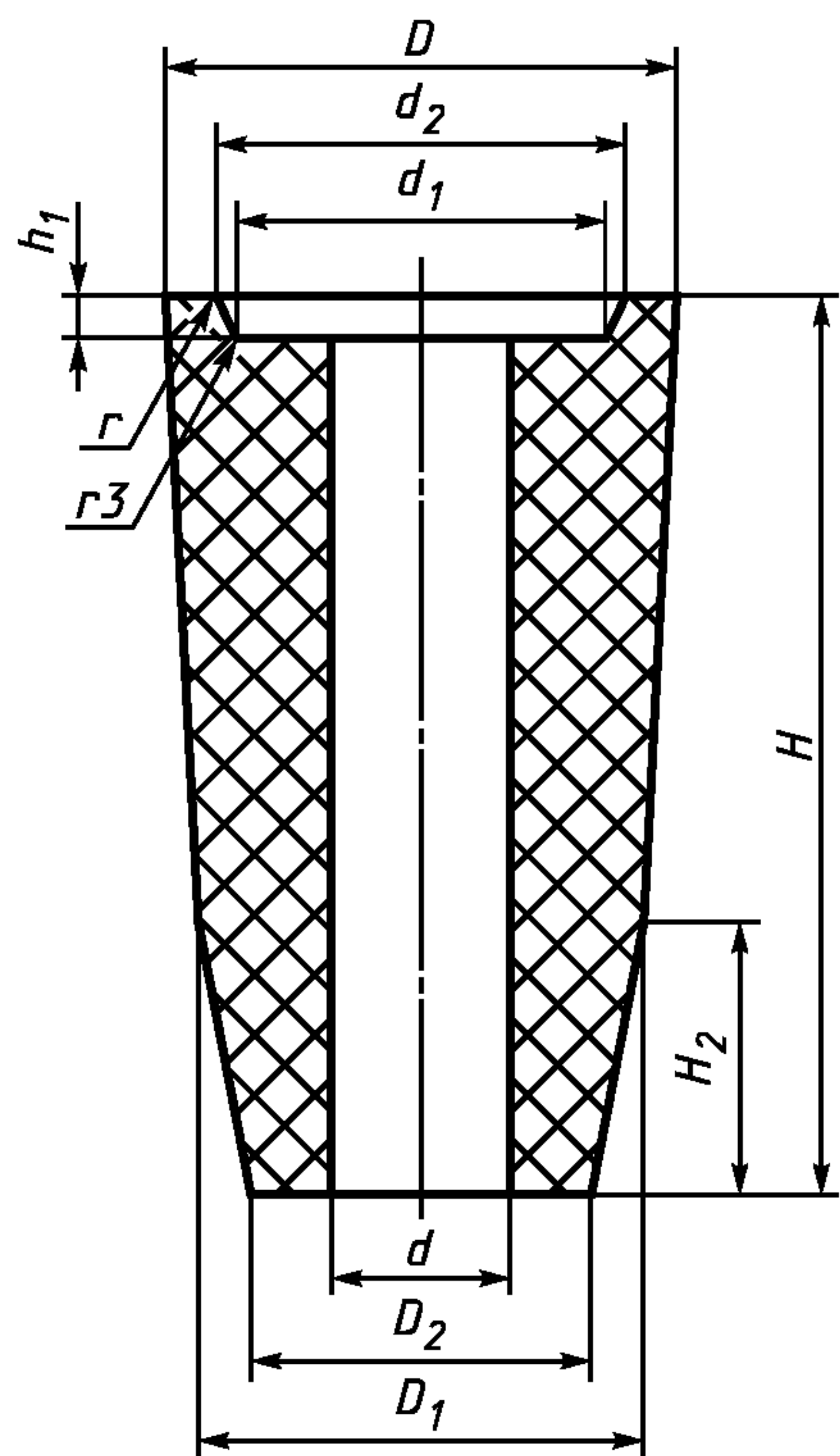
Рисунок 15 — Стакан-коллектор номер 22
