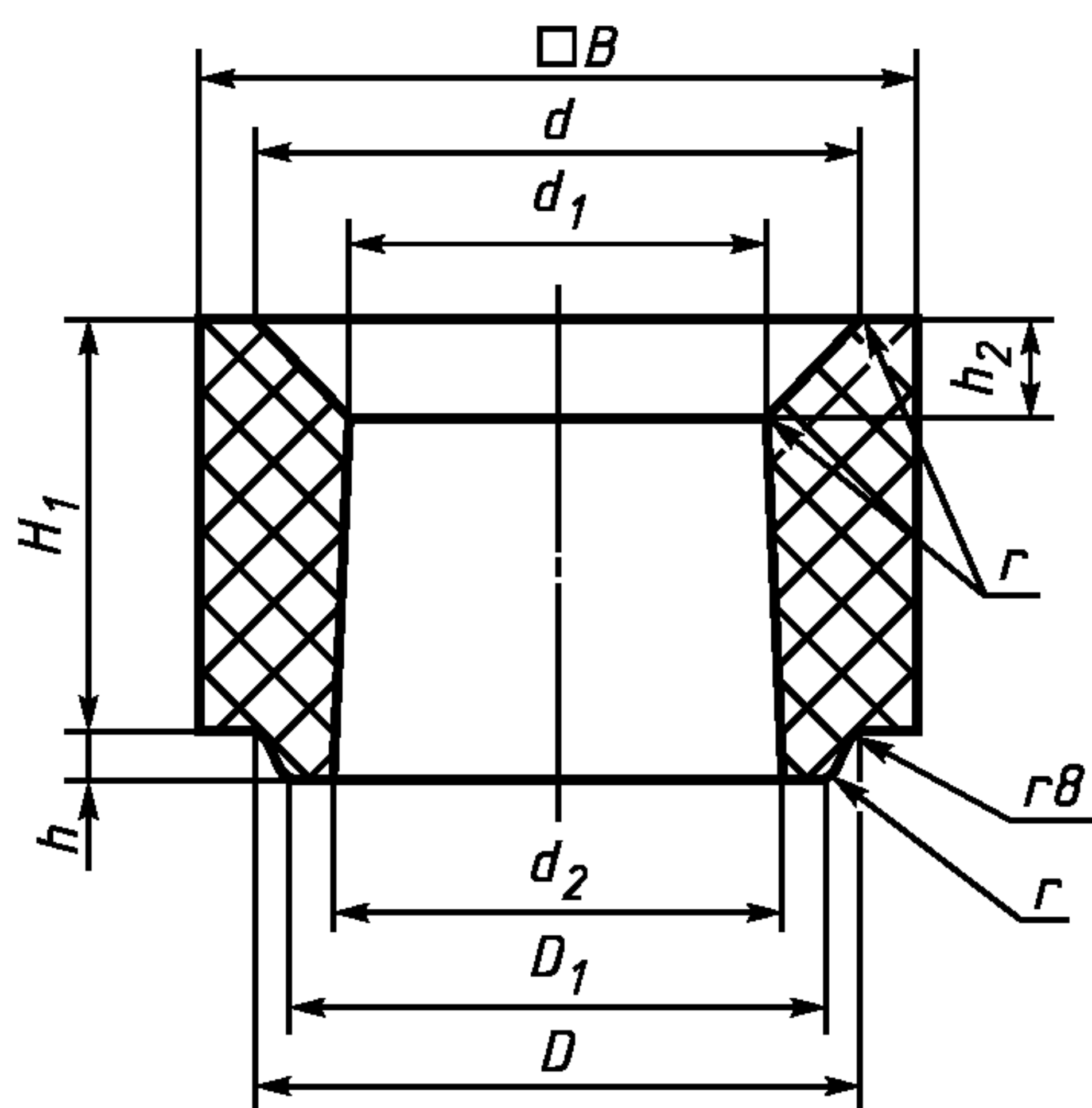
Рисунок 19 — Гнездовой кирпич номеров 3, 4 (верхняя часть)
