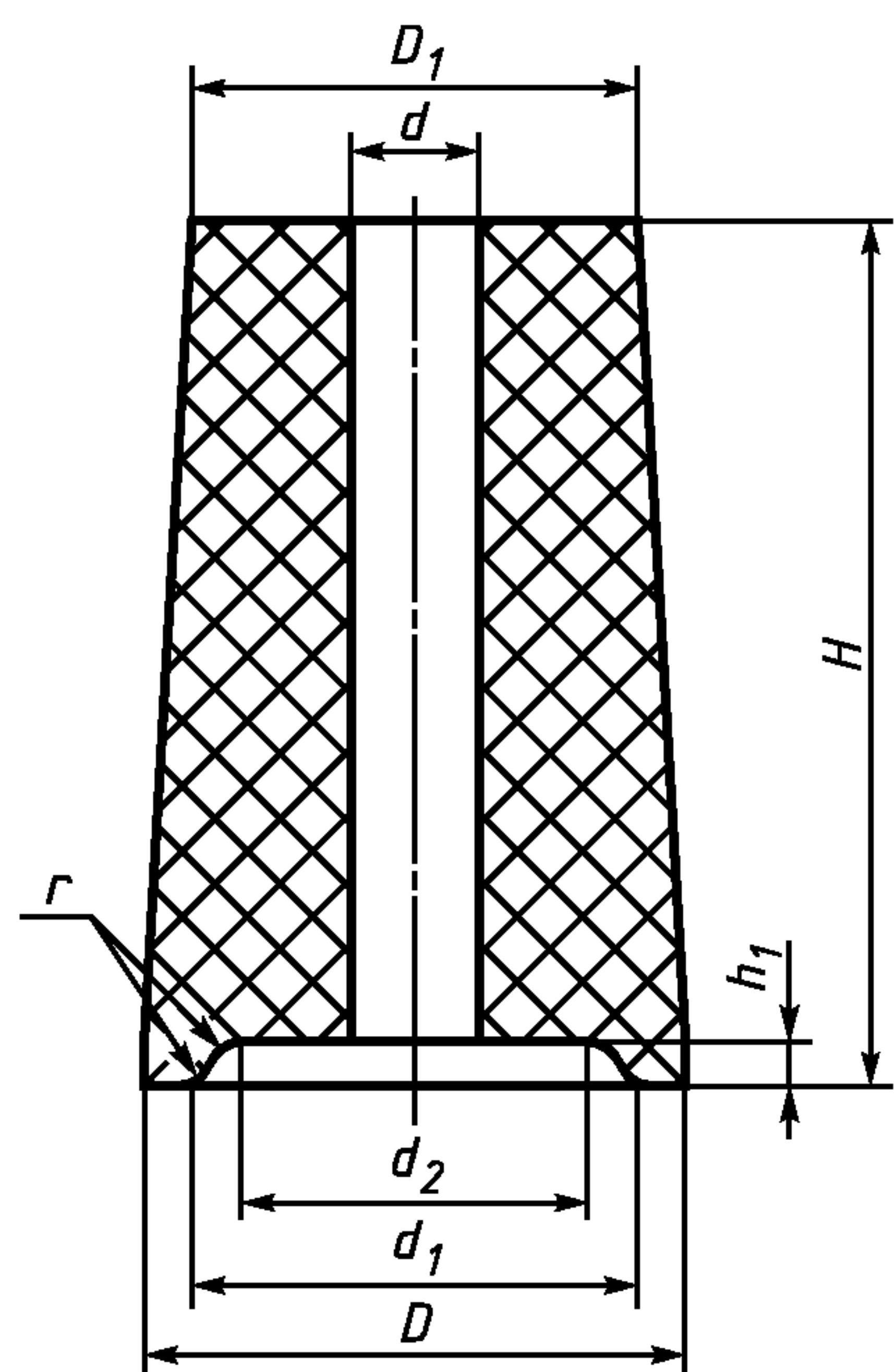
Рисунок 6 — Стакан и стакан-коллектор номеров 1—7, 7-1, 7-2
