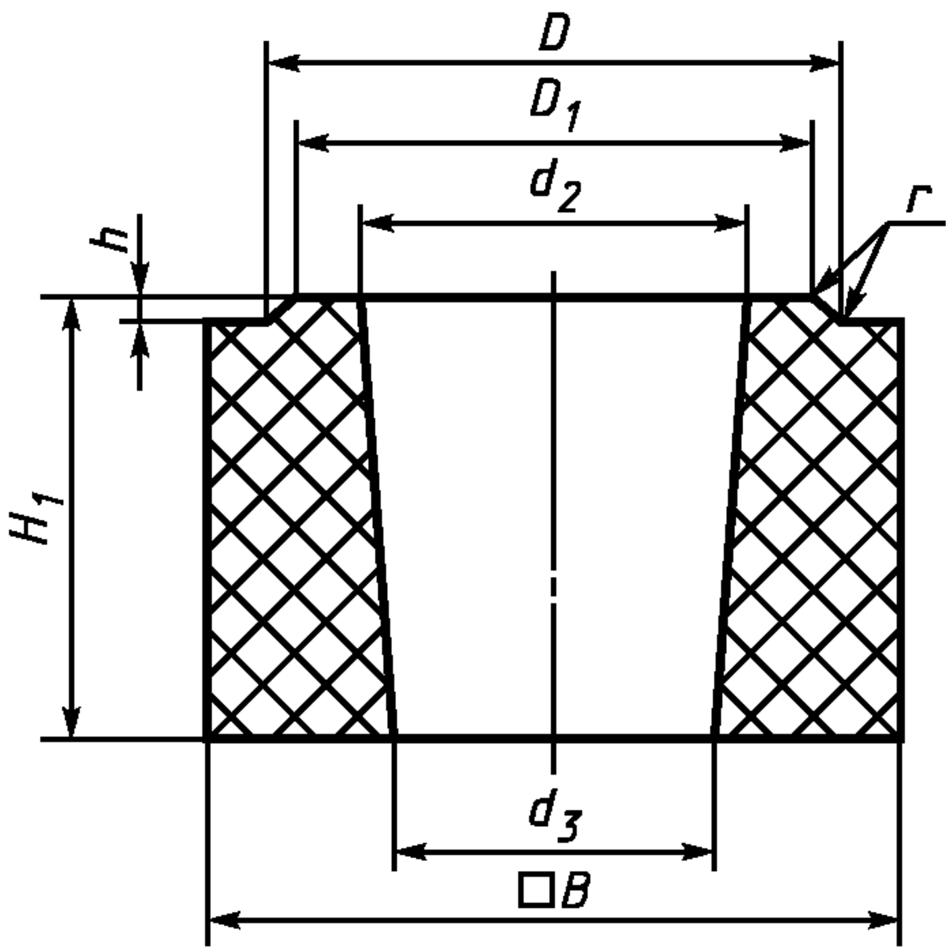
Рисунок 26 — Гнездовой кирпич номер 12 (верхняя часть)
