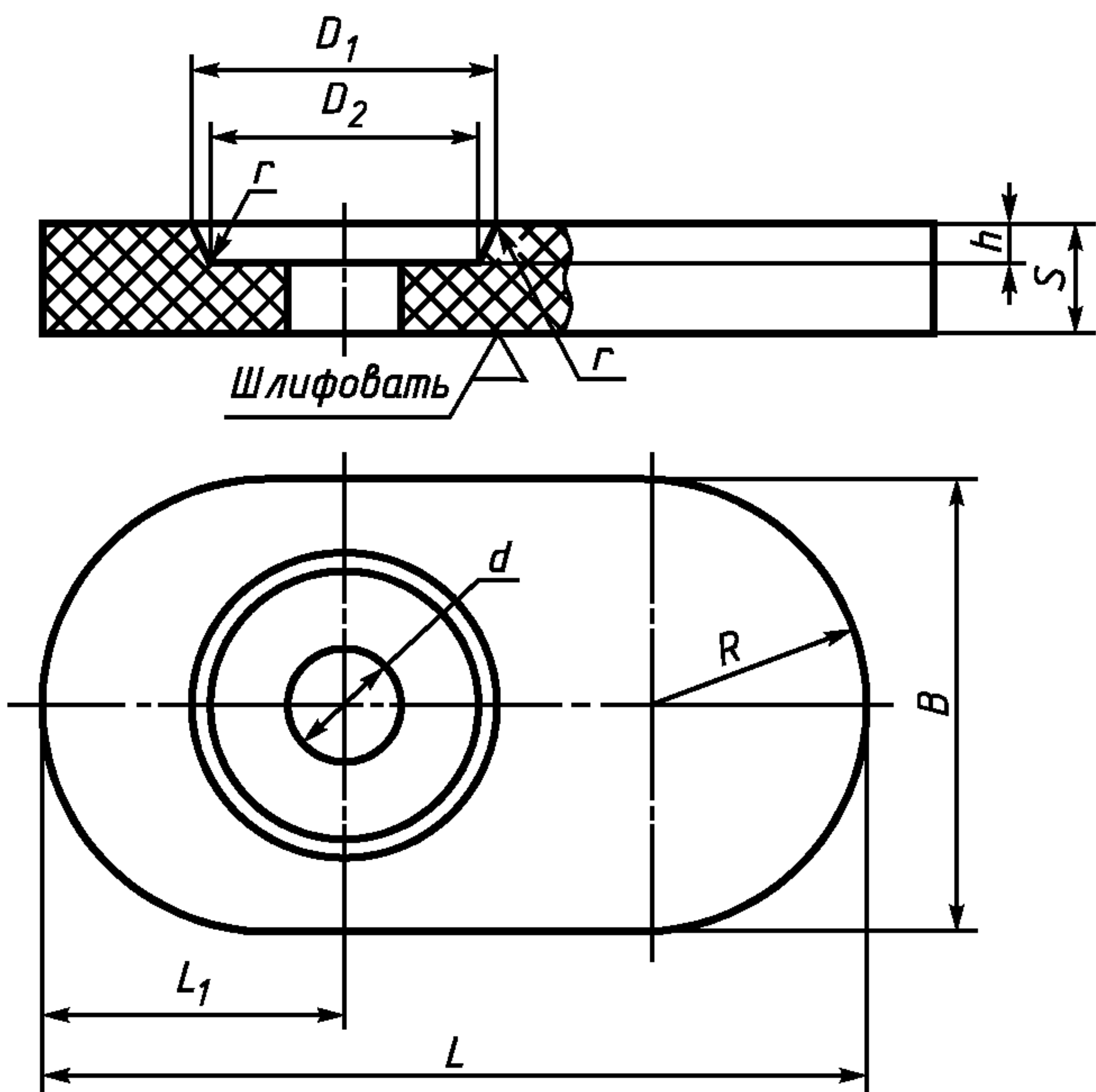
Рисунок 2 — Плита номеров 11 и 12
