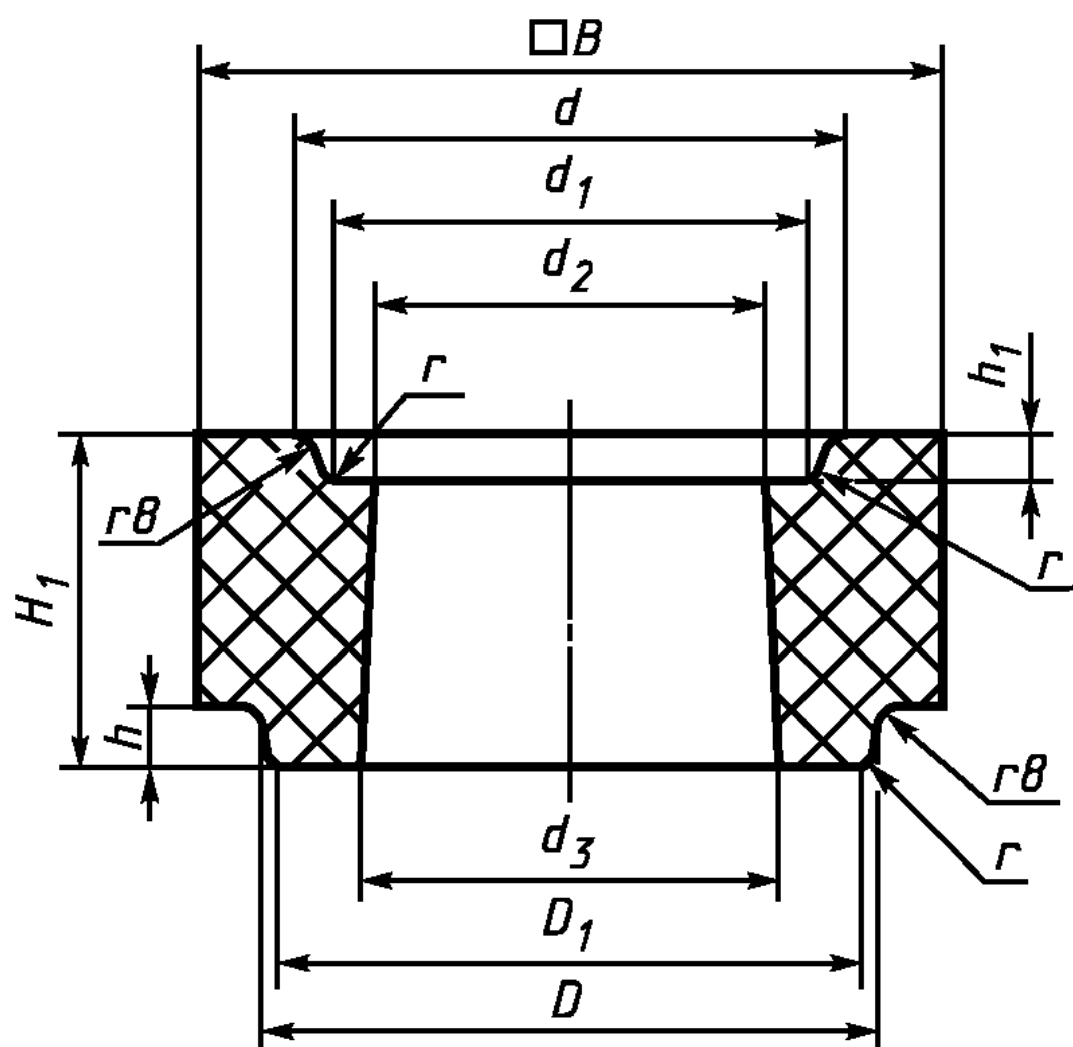
Рисунок 21 — Гнездовой кирпич номеров 6, 7 (нижняя часть)
