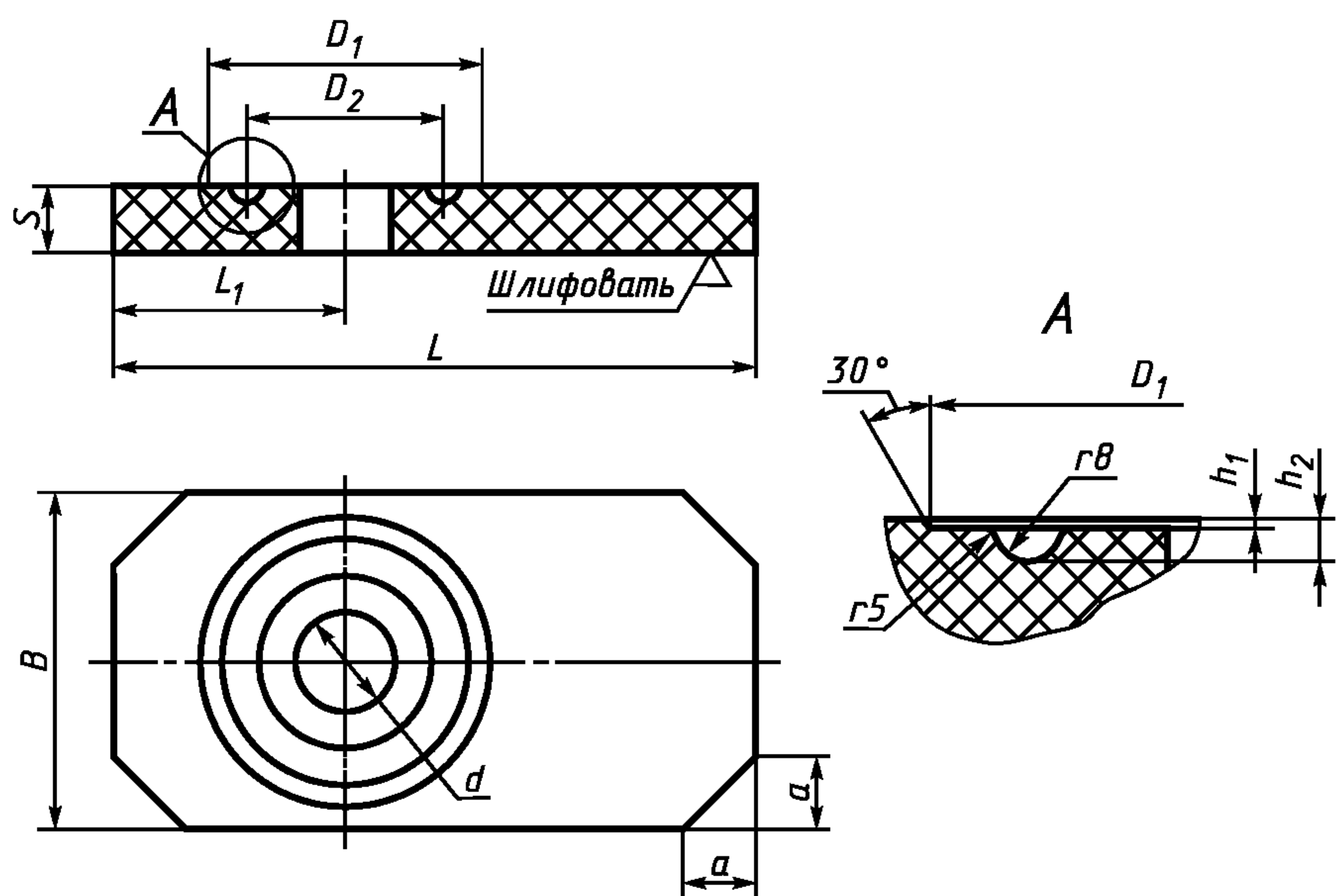
Рисунок 4 — Плита номер 14
