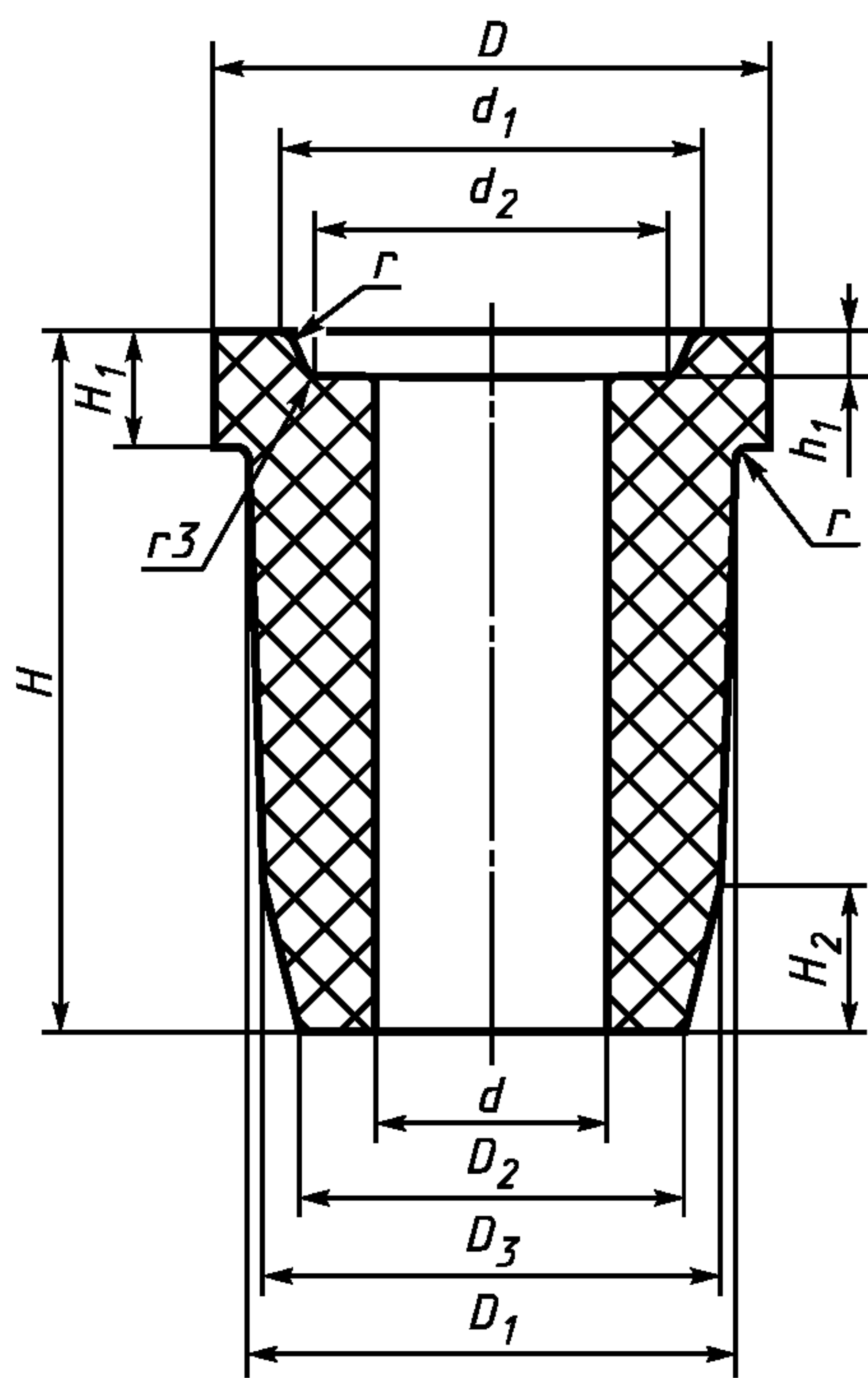
Рисунок 14 — Стакан-коллектор номер 21
