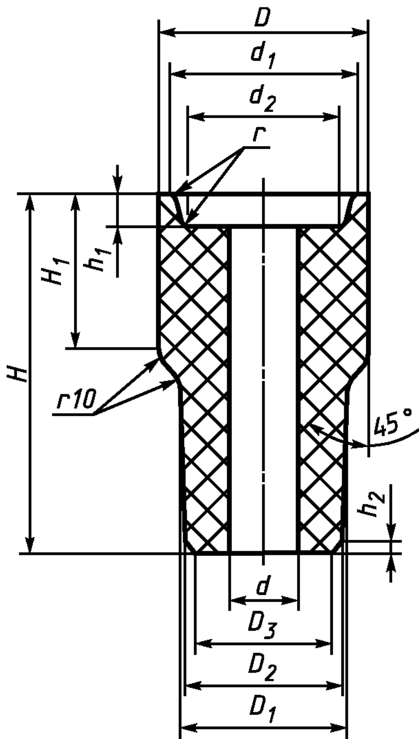
Рисунок 11 —Стакан-коллектор номер 17
