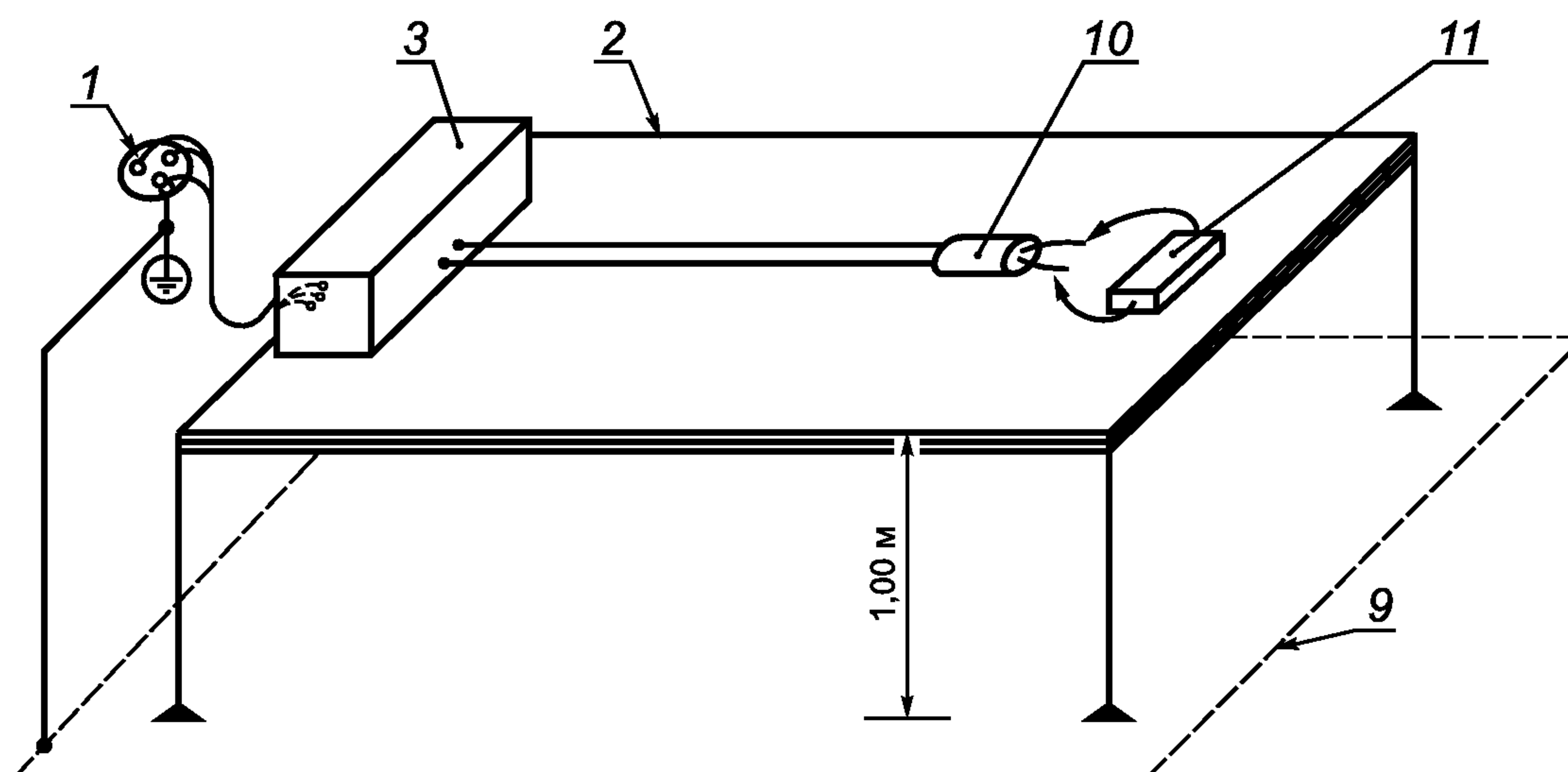
Рисунок 106 — Измерение ВЫХОДНОЙ МОЩНОСТИ. Биполярный выход (пункт 50)
