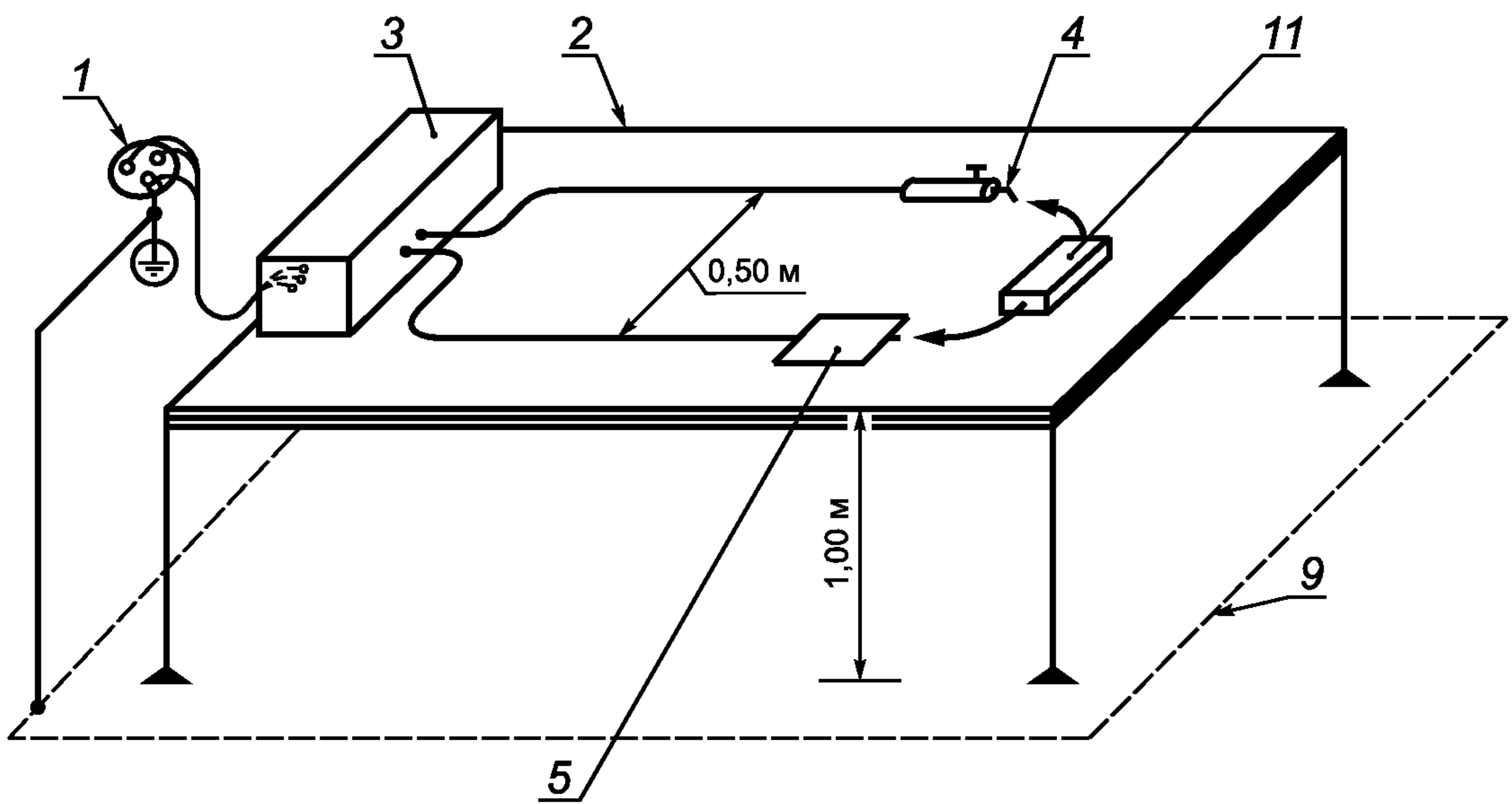
Рисунок 105 — Измерение ВЫХОДНОЙ МОЩНОСТИ. Монополярный выход (пункт 50)
