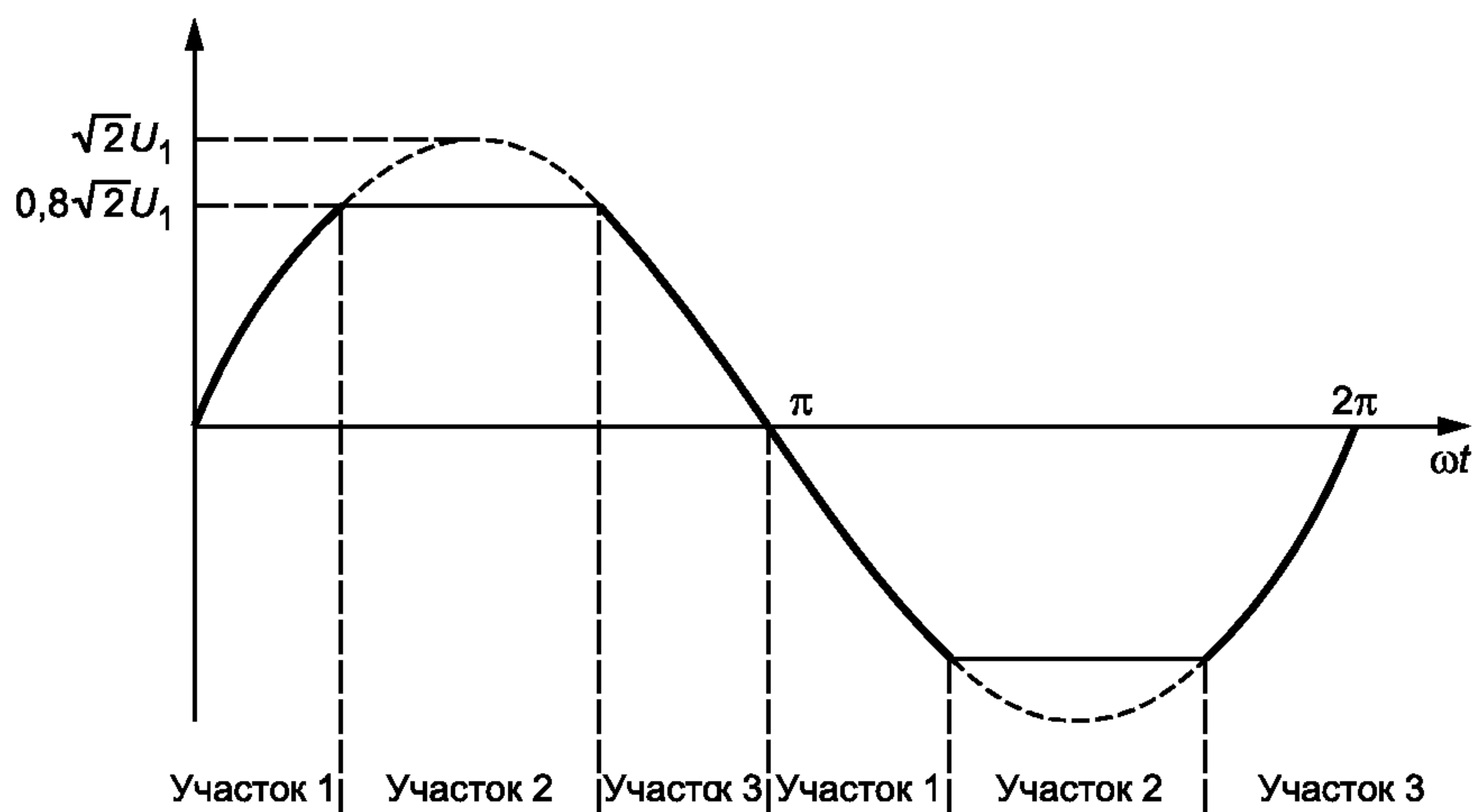
Рисунок 5 — Форма испытательного сигнала при испытаниях «Ограниченная синусоида»
