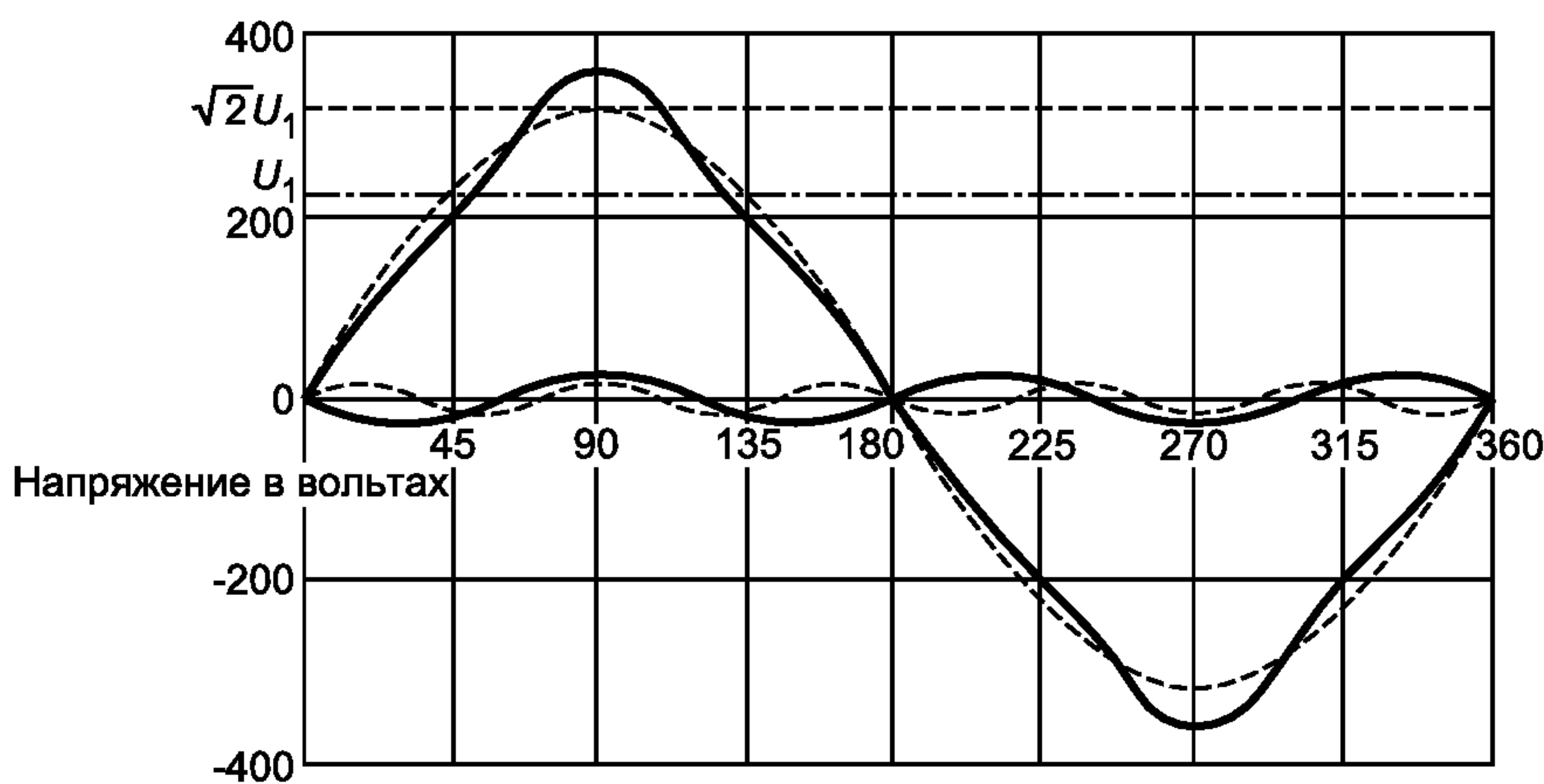
Рисунок 6 — Форма испытательного сигнала при испытаниях «Треугольные импульсы»
