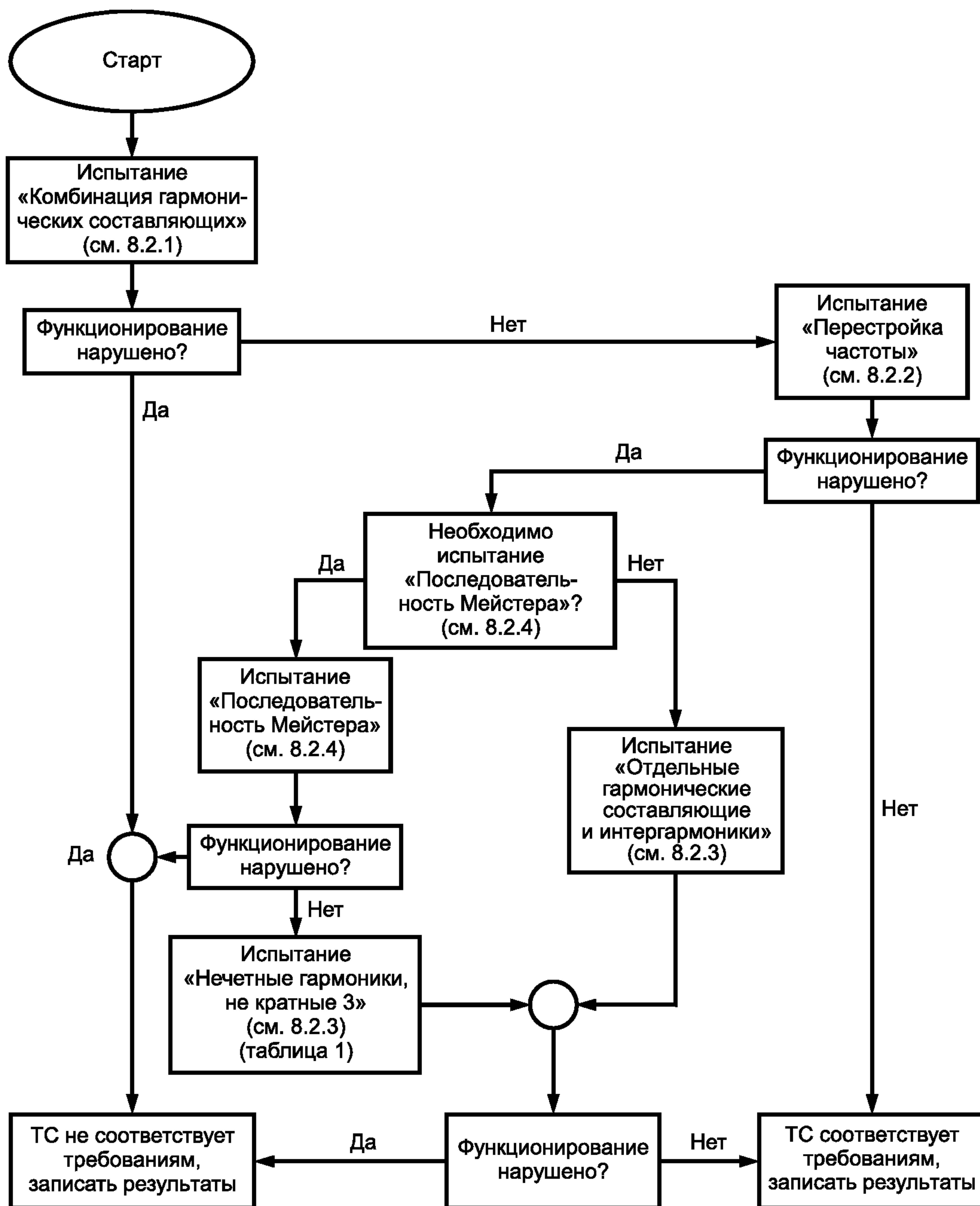
Рисунок 4 — Рекомендуемый алгоритм проведения испытаний (класс электромагнитной обстановки 3)
