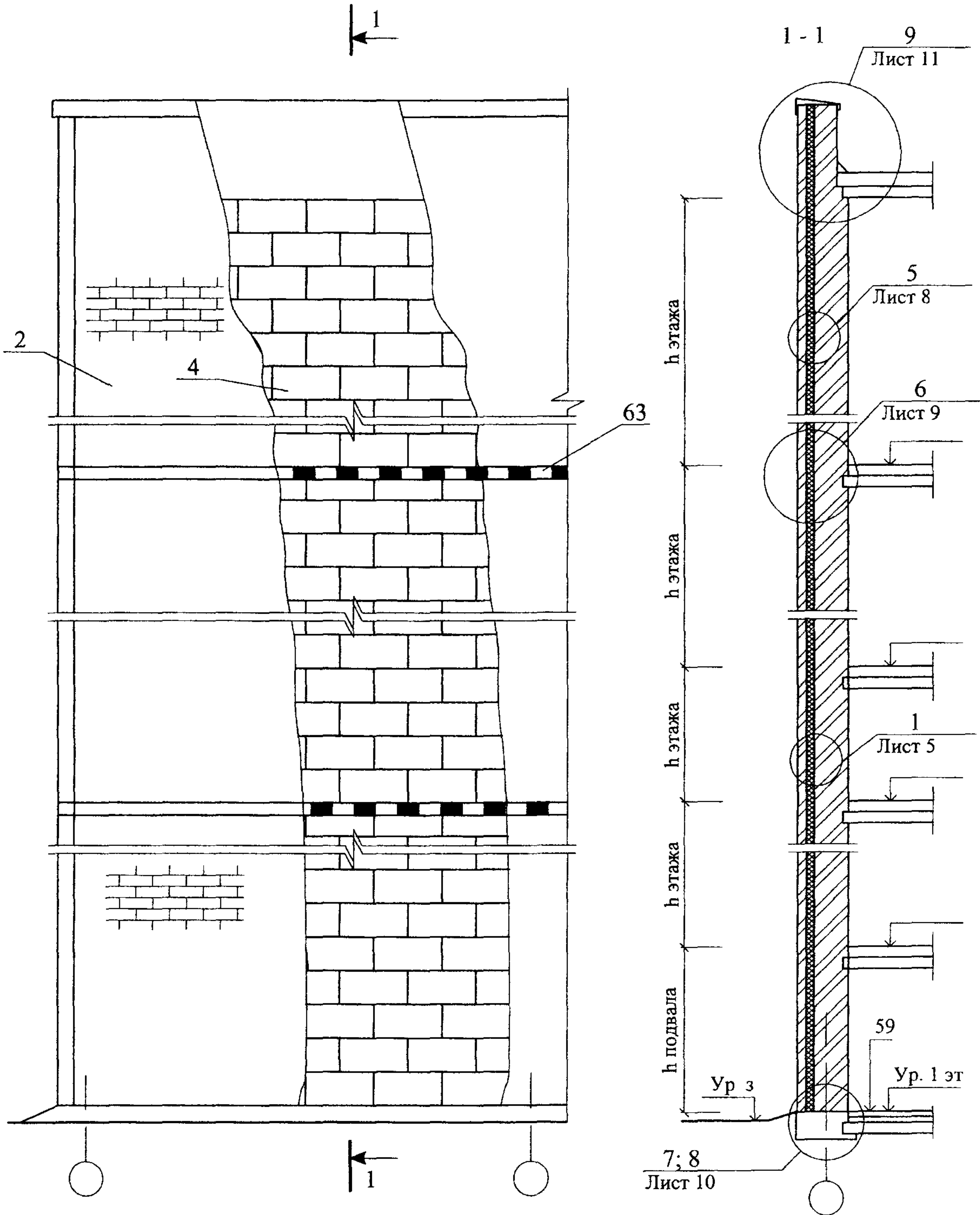
СХЕМА № 1. Расположение плит утеплителя, защитно-декоративной кладки, несущей балки-пояса
