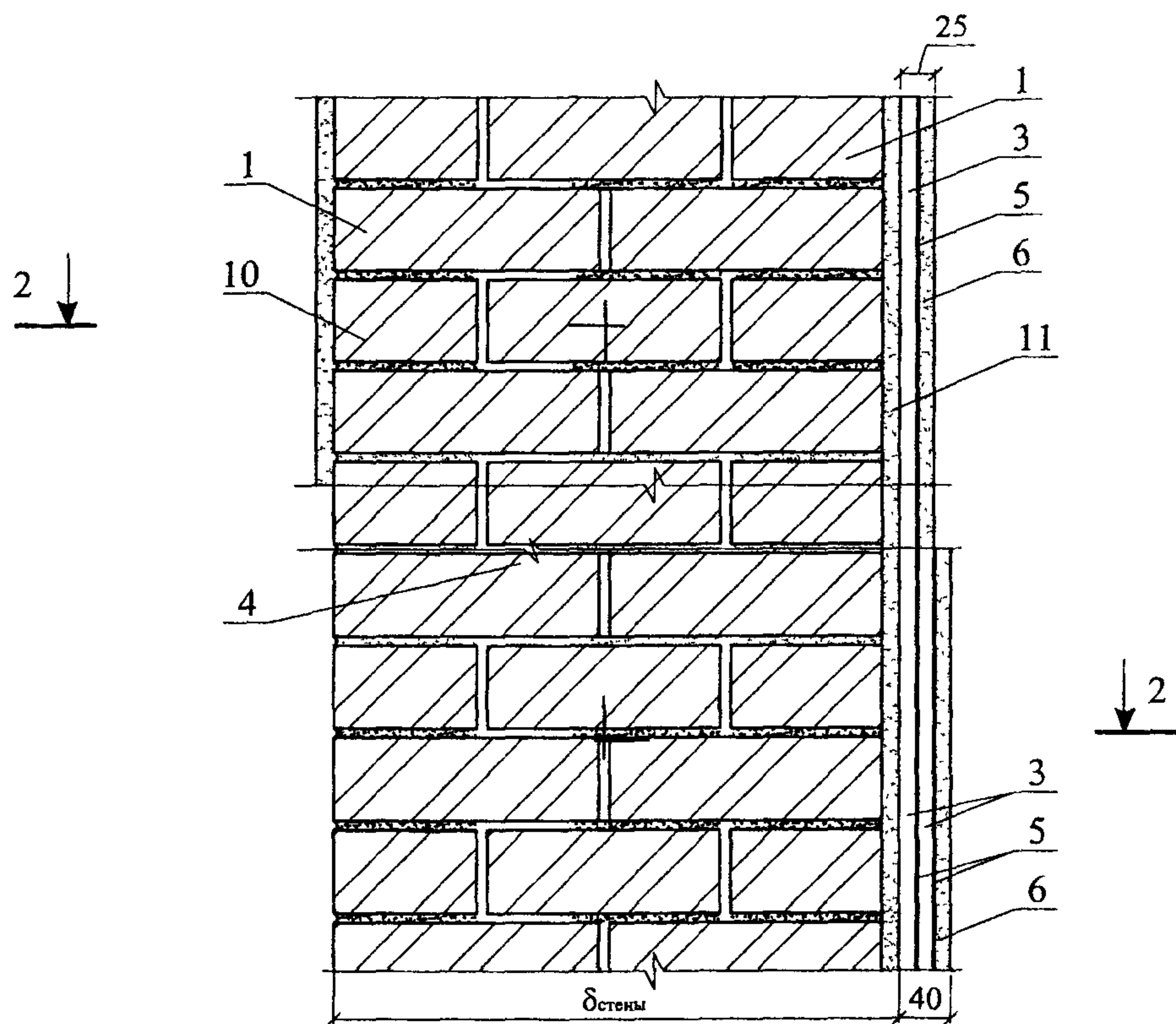
Вариант "А" с одной воздушной прослойкой
