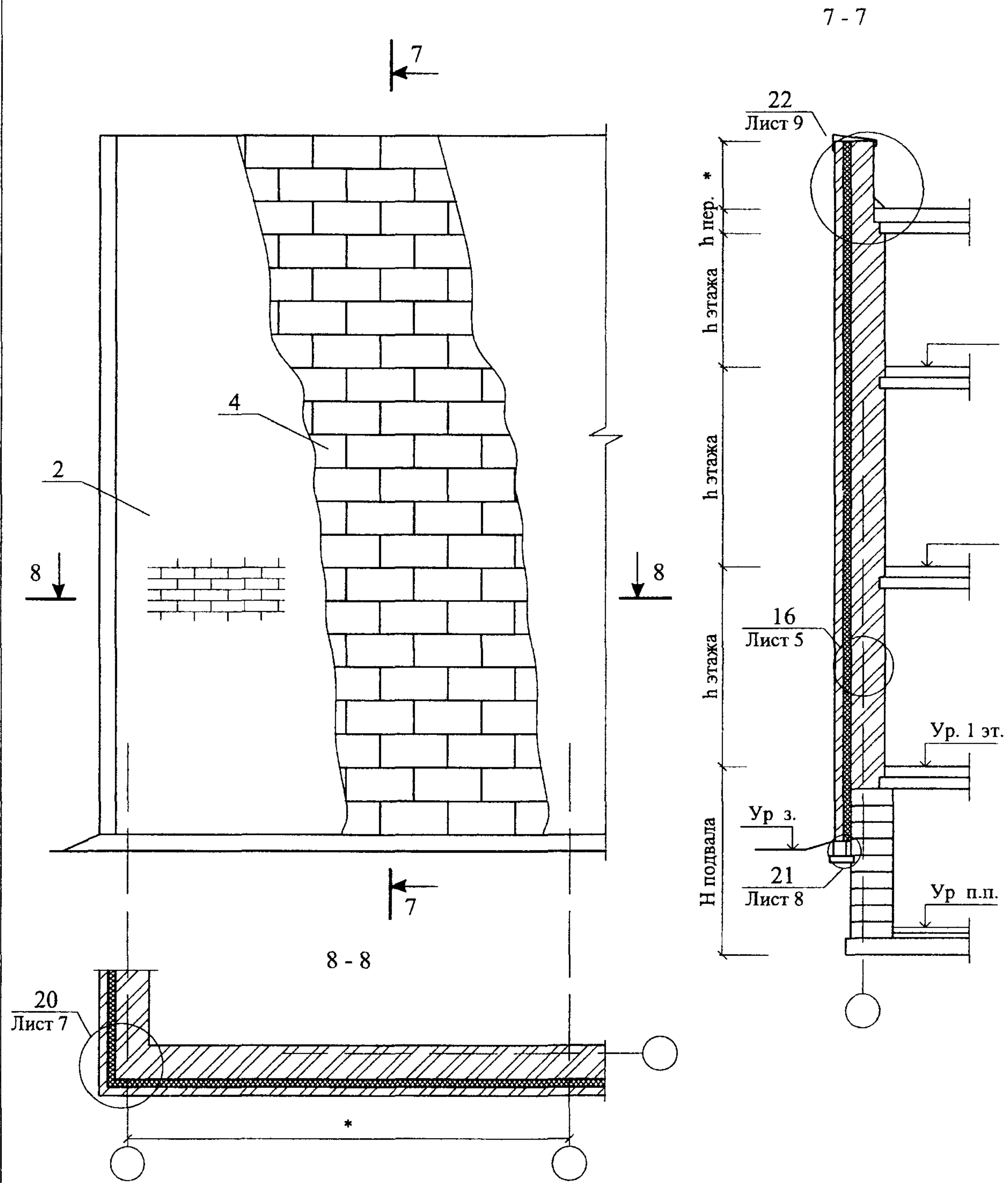
СХЕМА № 5. Расположение плит утеплителя и защитно-декоративной кладки
