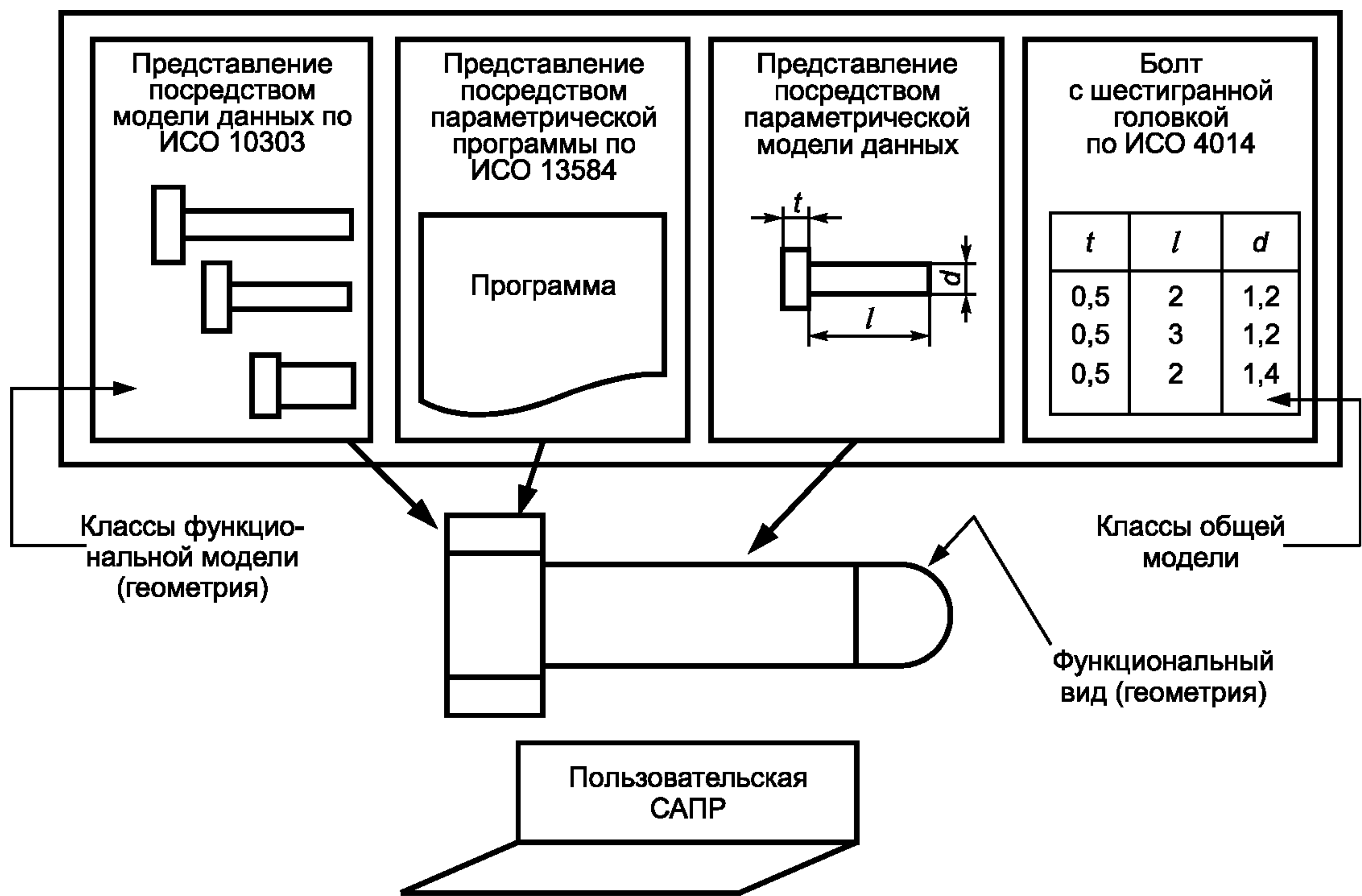
Рисунок 3 — Структура содержимого библиотеки
