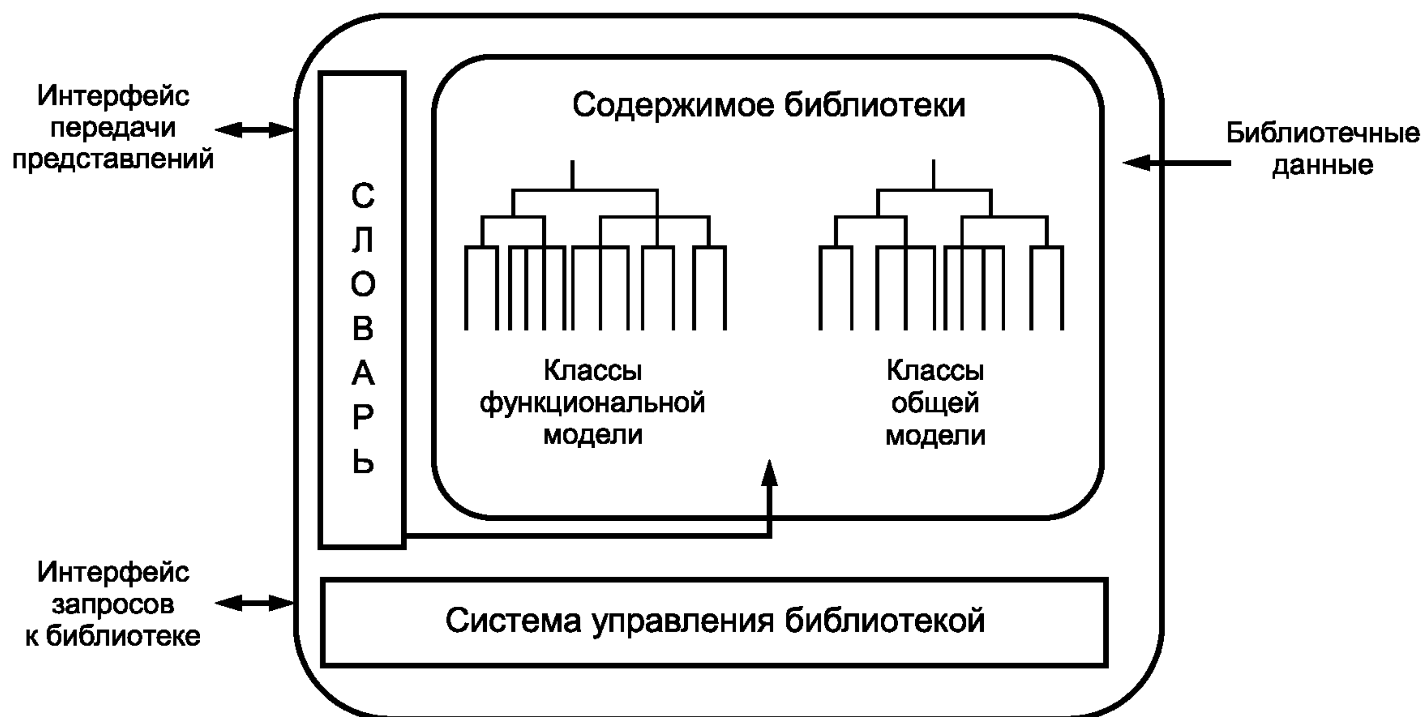
Рисунок 2 — Библиотечная система
