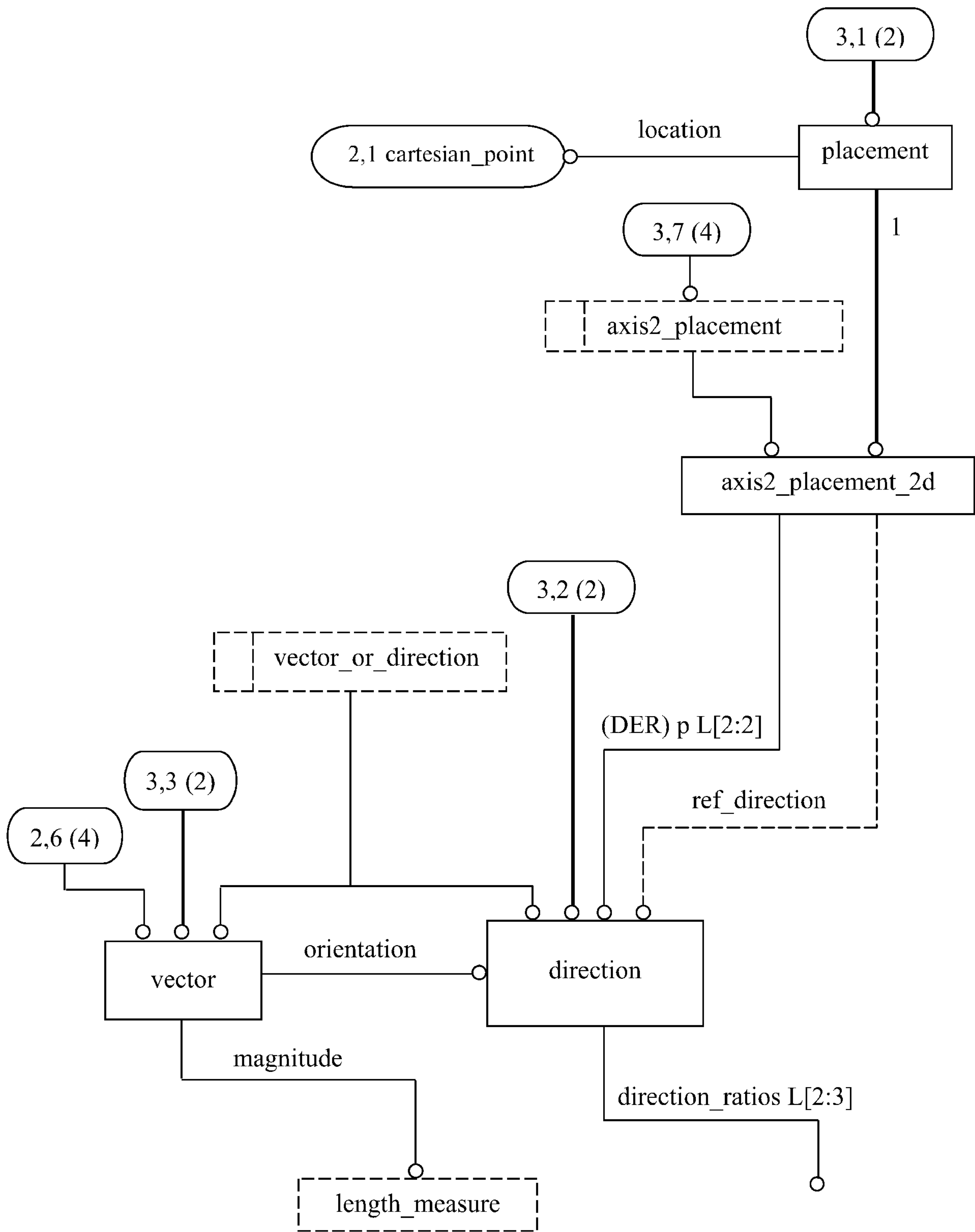
Рисунок С.3 — aic_geometrically_bounded_2d_wireframe — EXPRESS-G диаграмма 3 из 5
