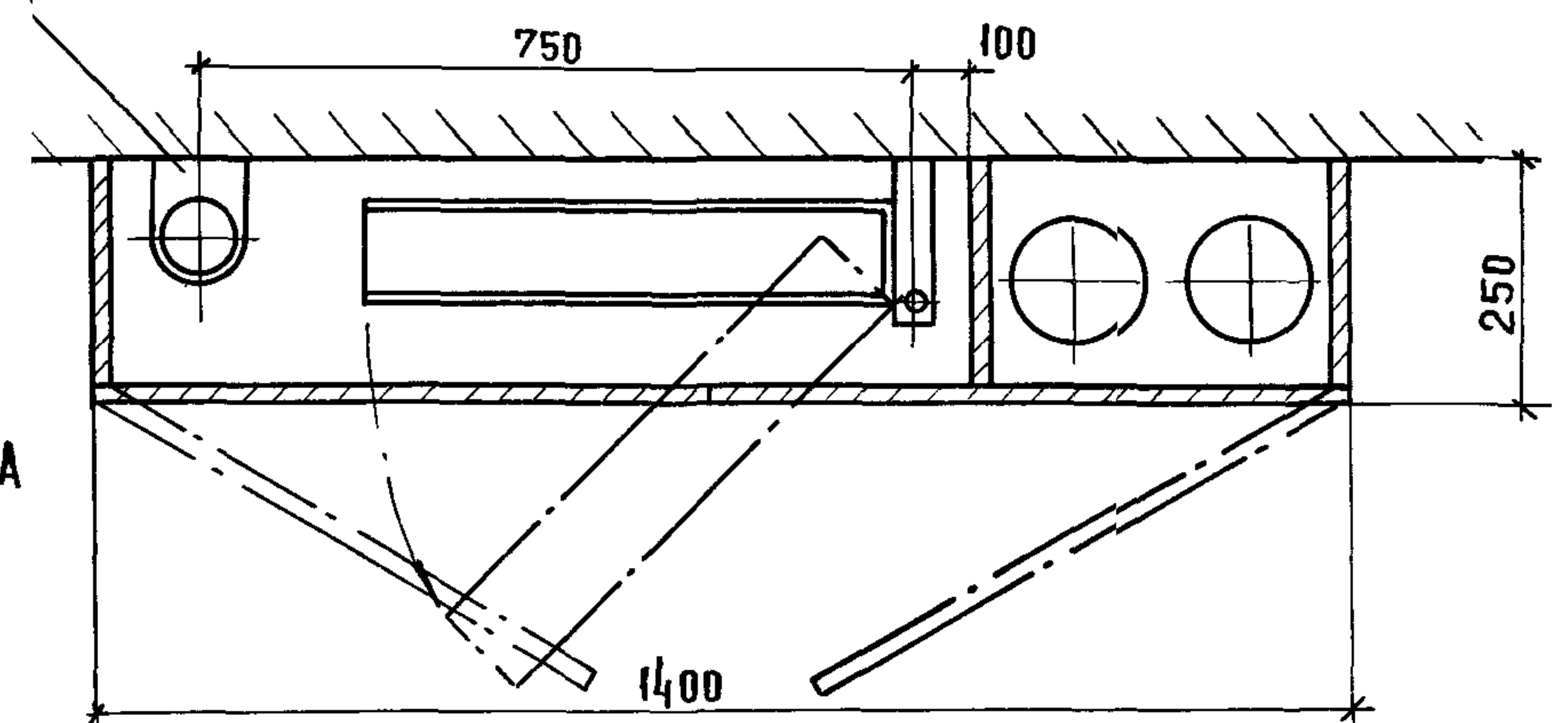
А-А. ВАРИАНТ 2 (ШКАФЫ ШП-13; ШП-16)
