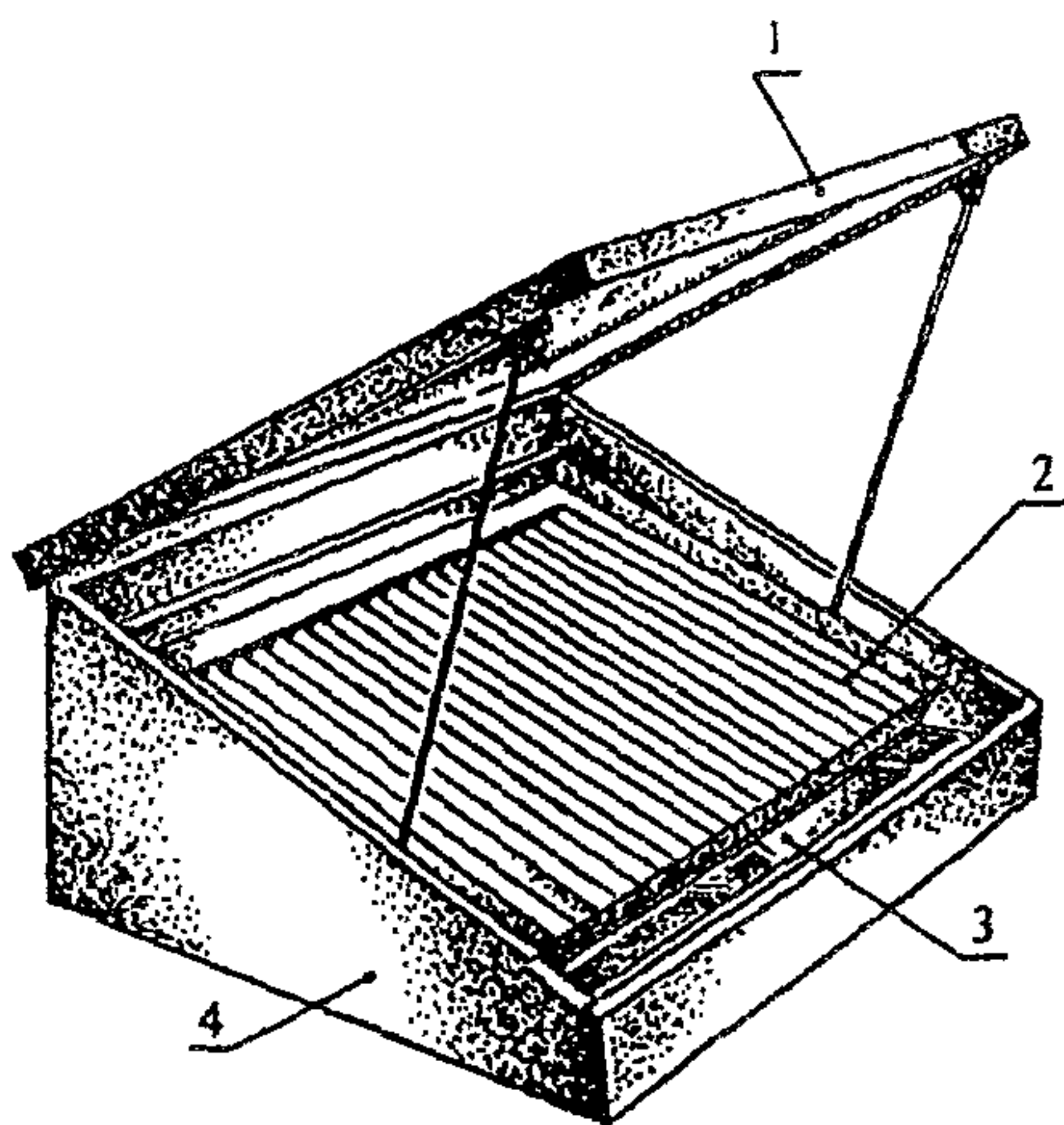
Рис. 1. Воскотопка солнечная. 1 — рама стеклянная; 2 — противень; 3 — корытце; 4 — корпус.
