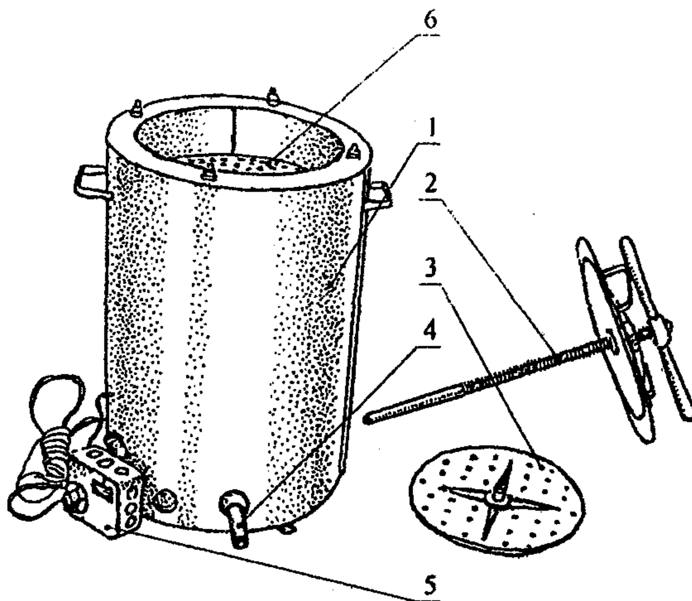
Рис. 5. Воскотопка-воскопресс для переработки воскосырья сухим способом.
