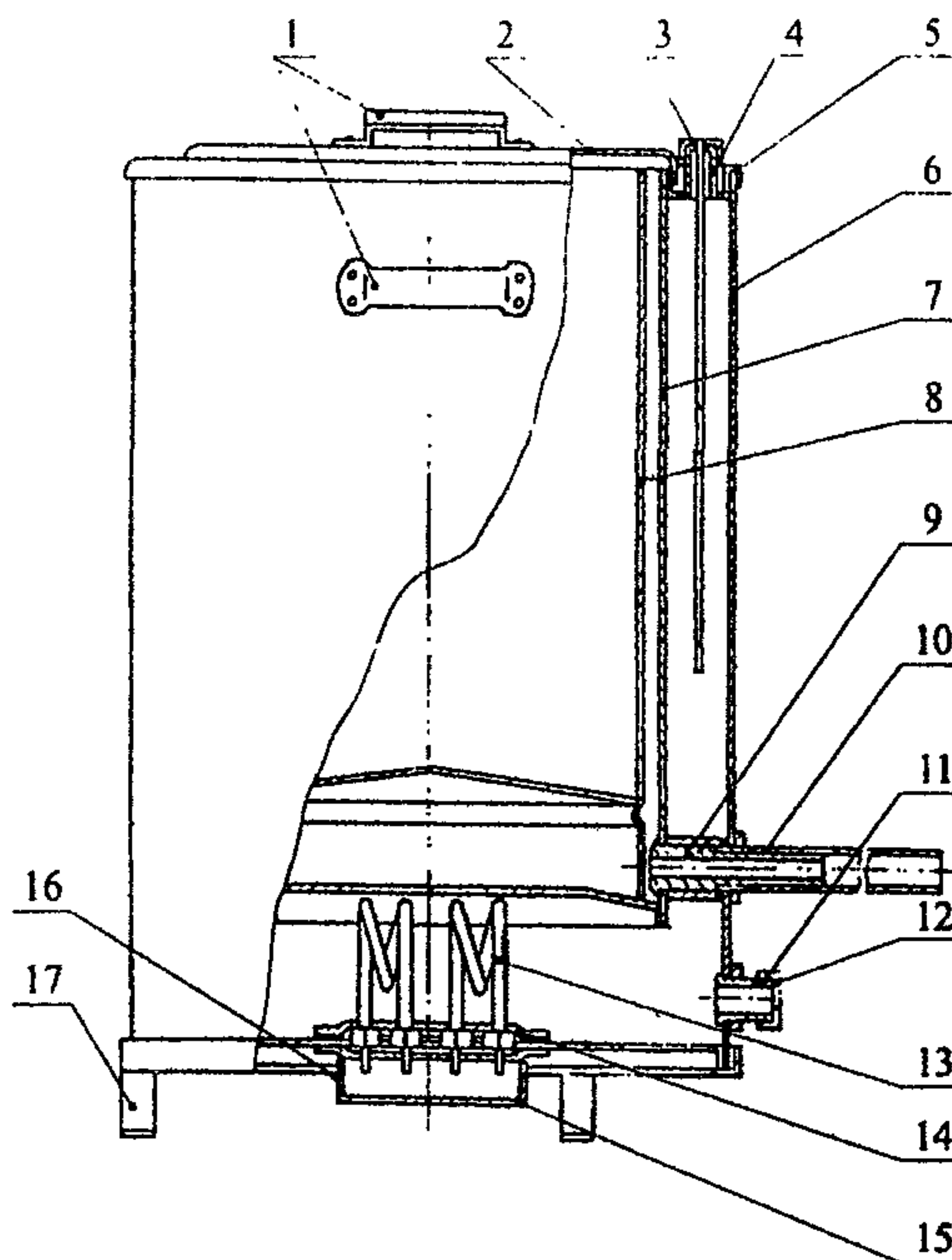
Рис. 3. Воскотопка паровая с электронагревом.
