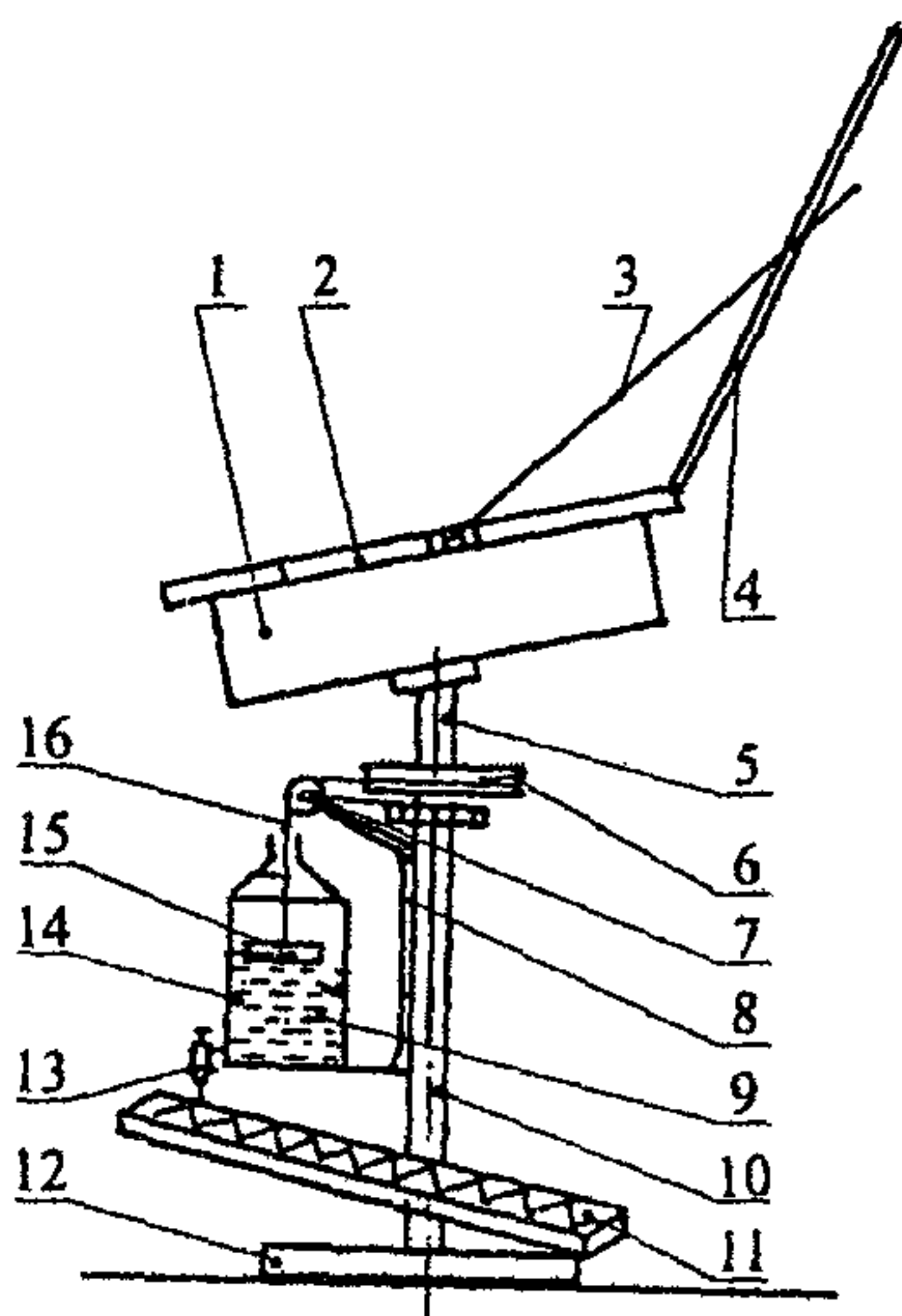
Рис. 2. Схема солнечной воскотопки с поилкой для пчел.
