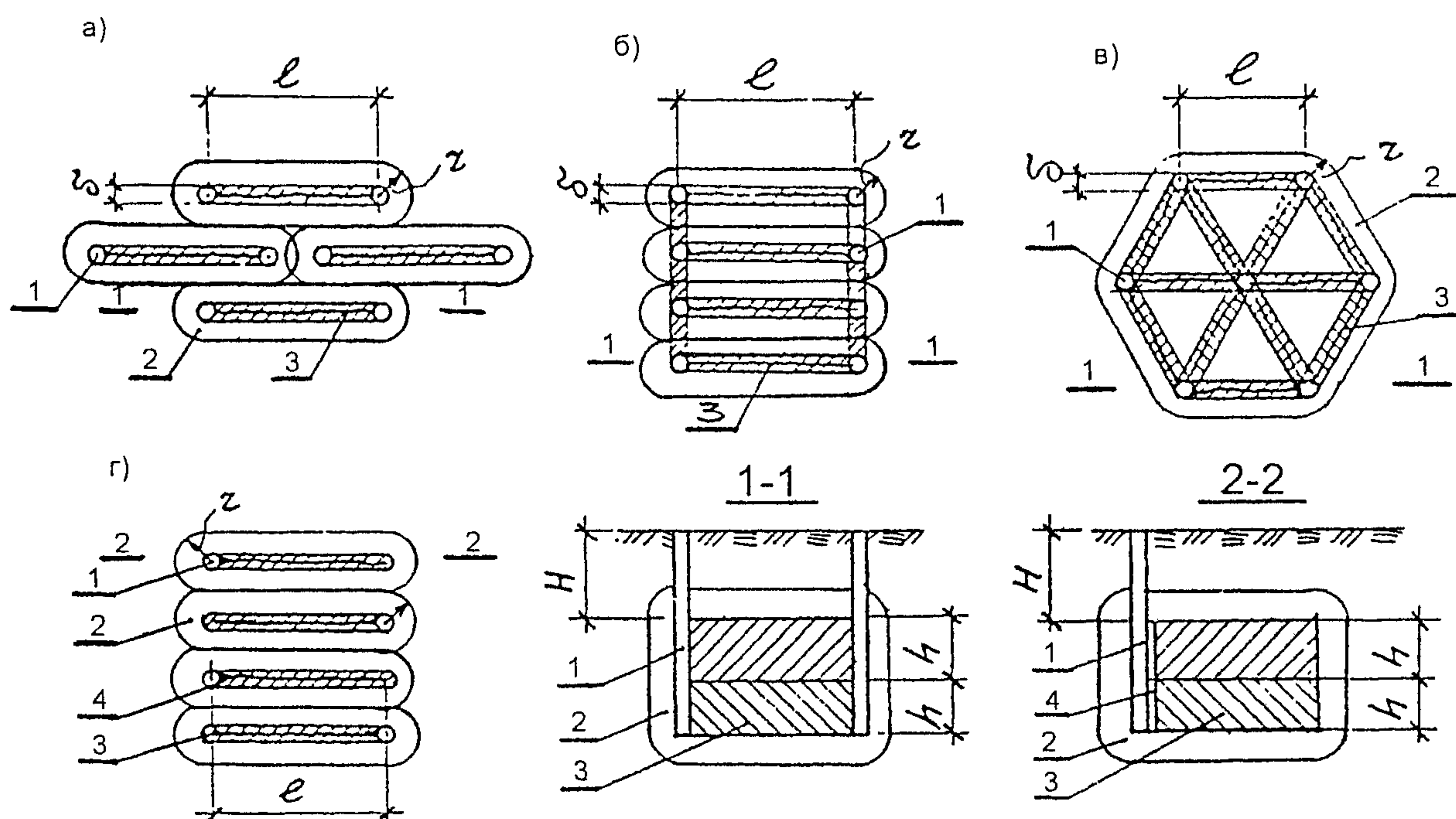
а) для плитного фундамента; б) столбчатого; в) круглого; г) ленточного 1 – скважина; 2 – зона уплотнения; 3 – армоэлемент из цементогрунта; 4 – концентратор напряжения
