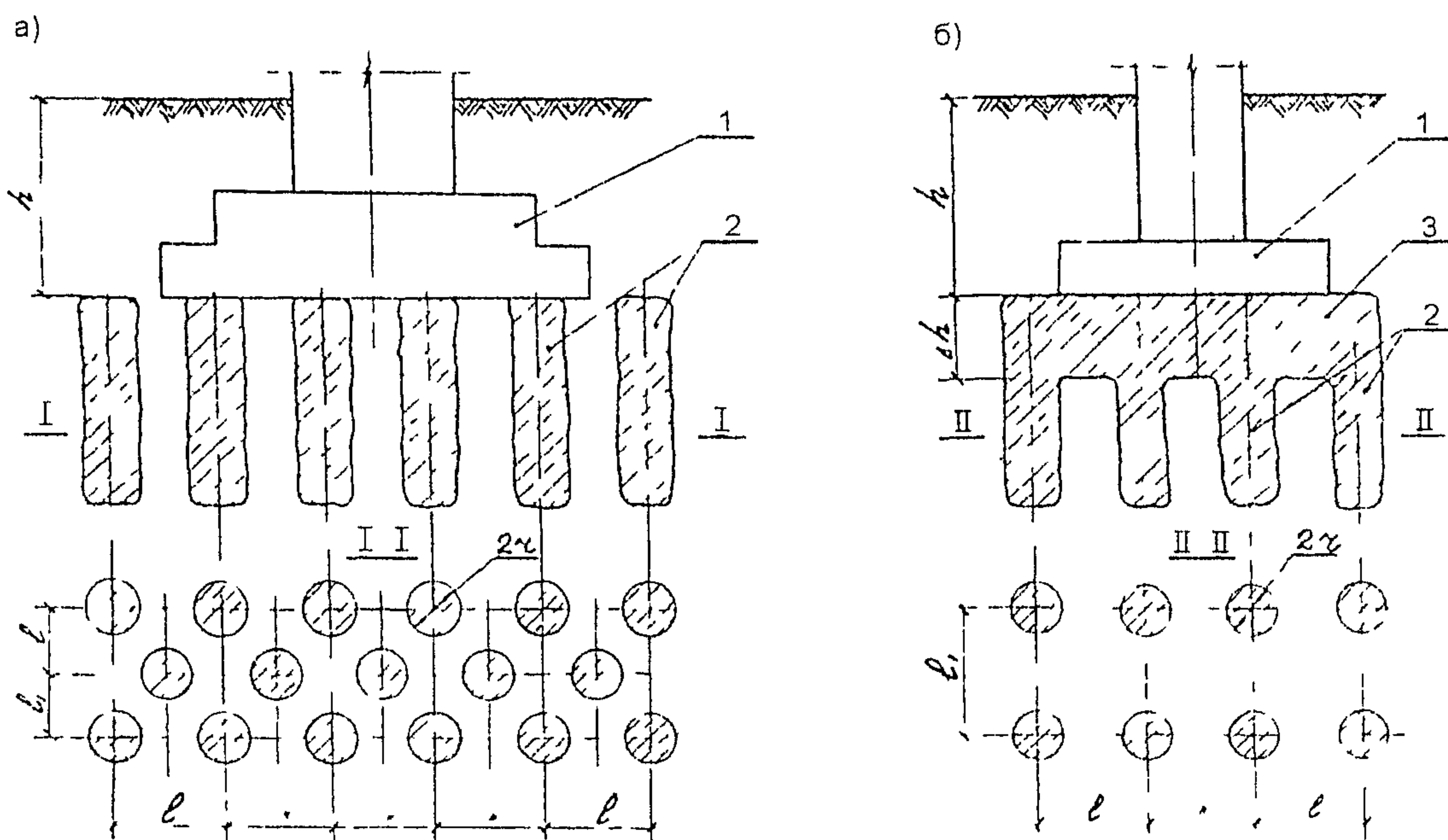
а) сплошное закрепление, б) с разрывом по вертикали, в) стаканного типа, г) с разрывом по горизонтали Рис. Б.1. Конструктивные схемы укрепления грунта в основании фундаментов
