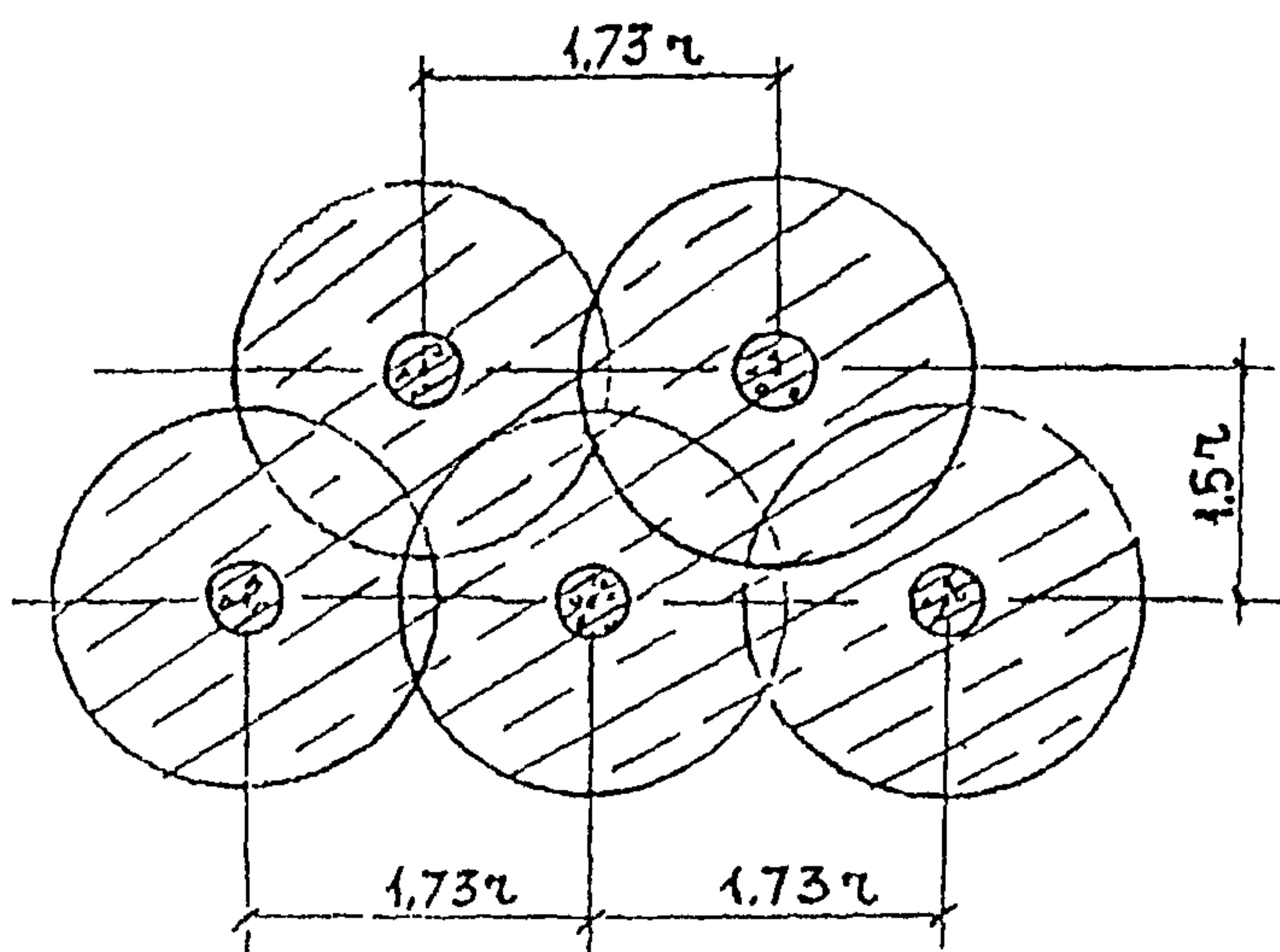
Рис. 6.4. Схема размещения свай-инъекторов при формировании куста
