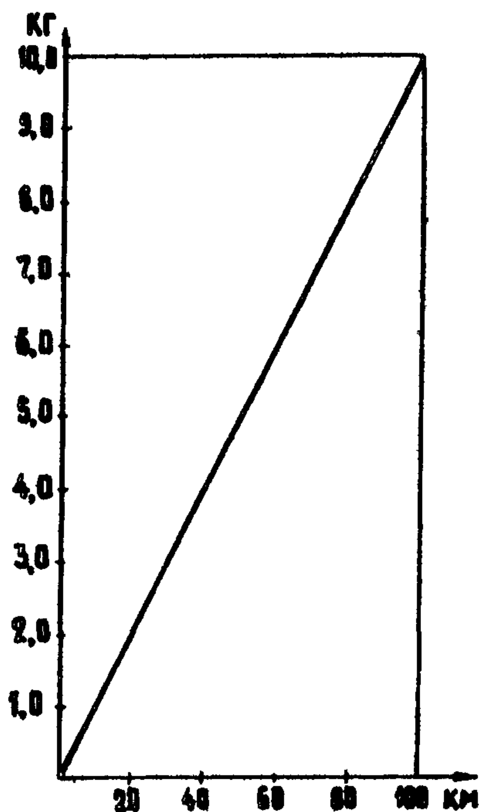
Рис. 2.3. Годовые затраты условного топлива на транспортировку 1 т комбикормов в зависимо- сти от расстояния
