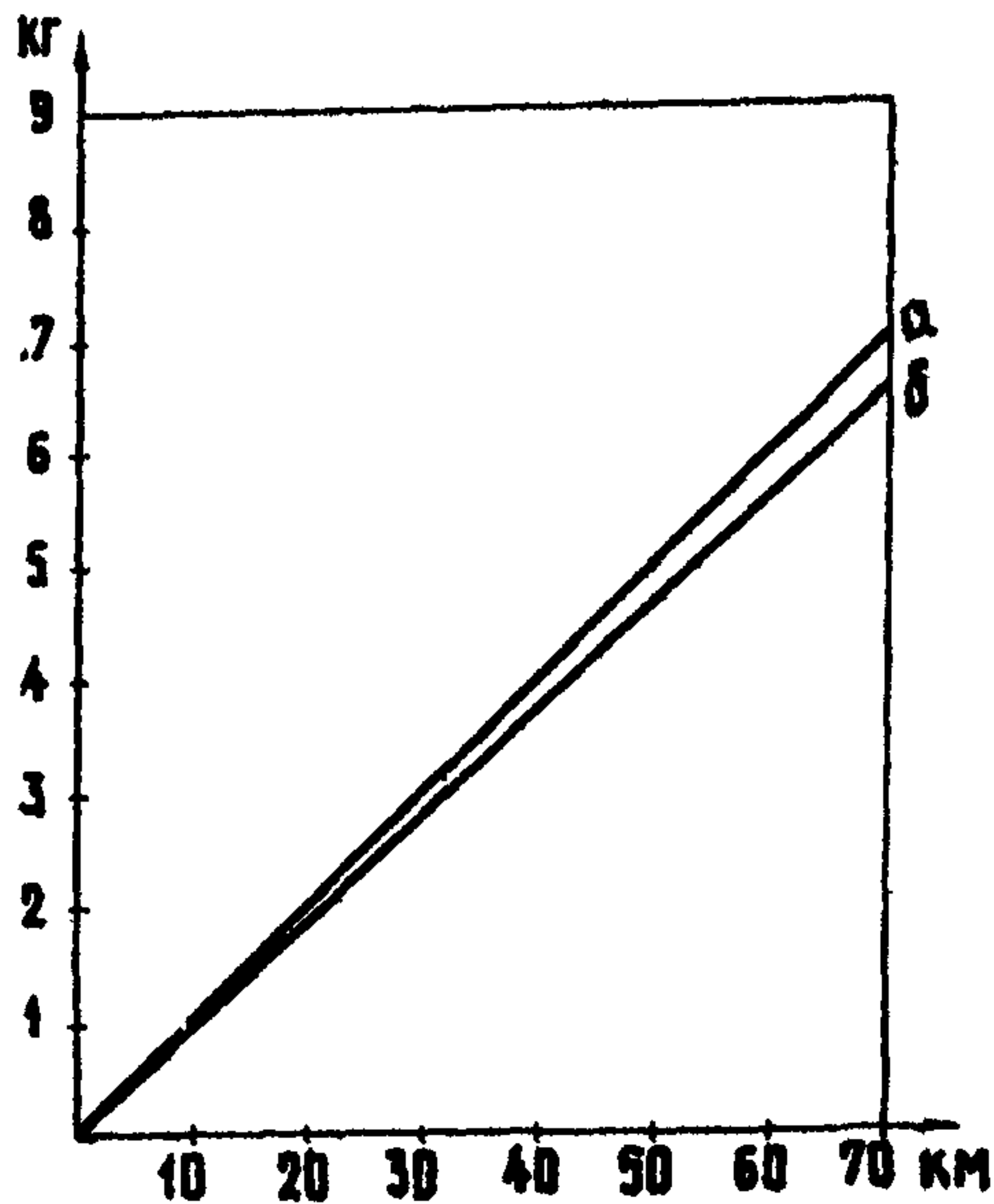
Рис. 2.1. Годовые затраты условного топлива на доставку к ферме I т ЗЦМ (а), соли, монокальция фосфата (б) в зависимости от расстояния перевозки
