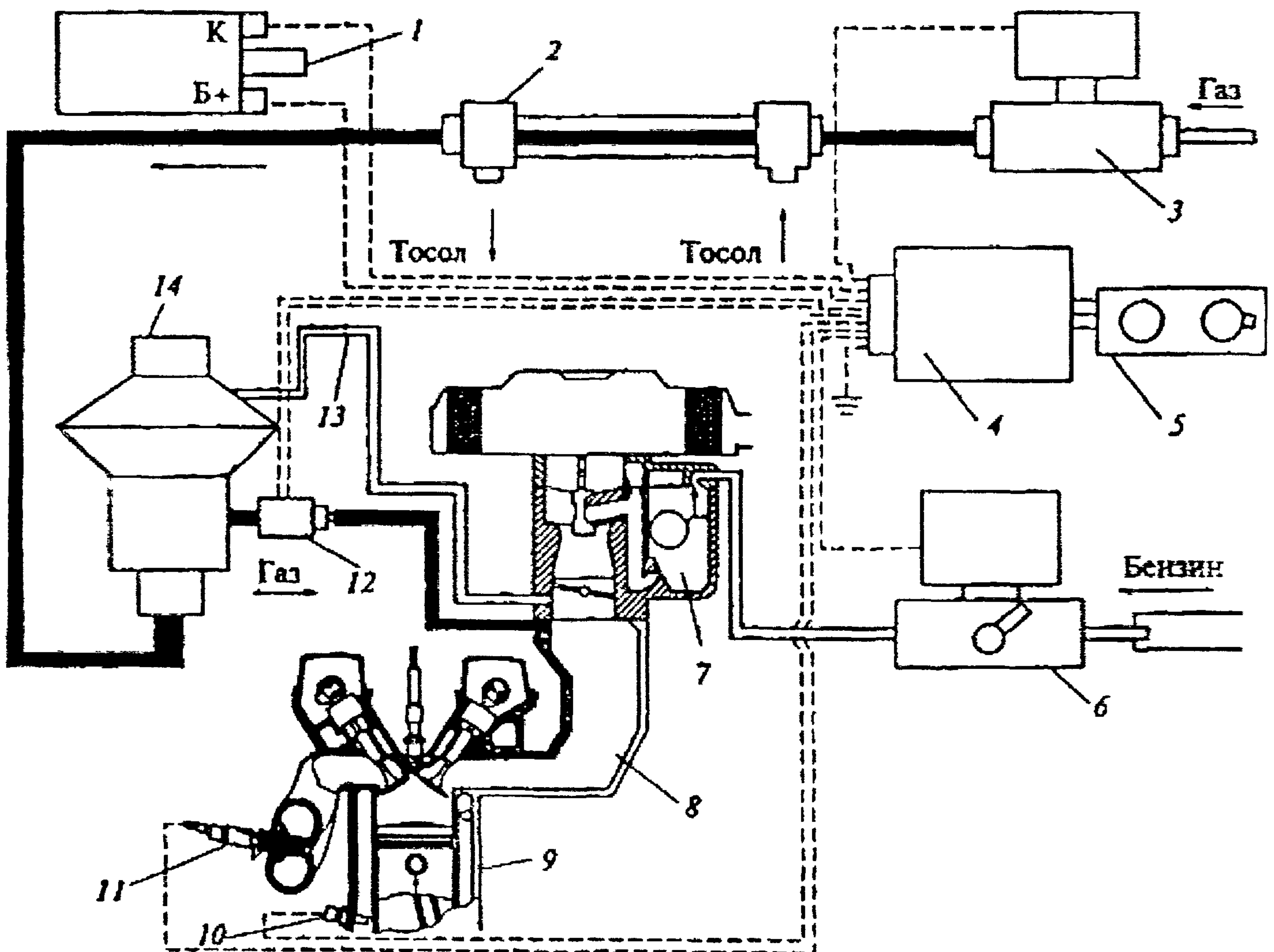
Рис. 3.10. Схема инжекторной системы дозирования газового топлива:
