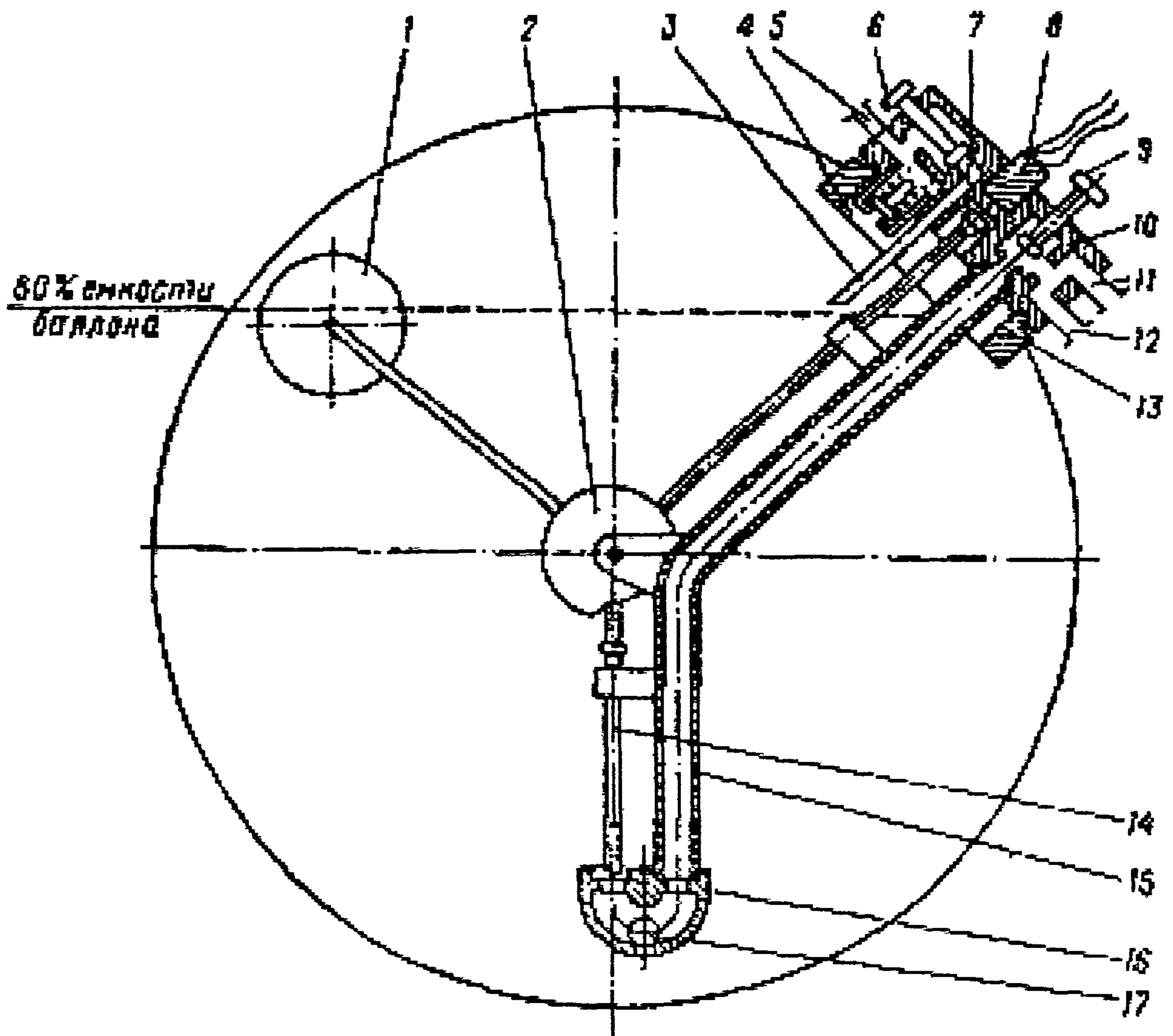
Рис. 3.9. Блок арматуры «САГА - 6»:
