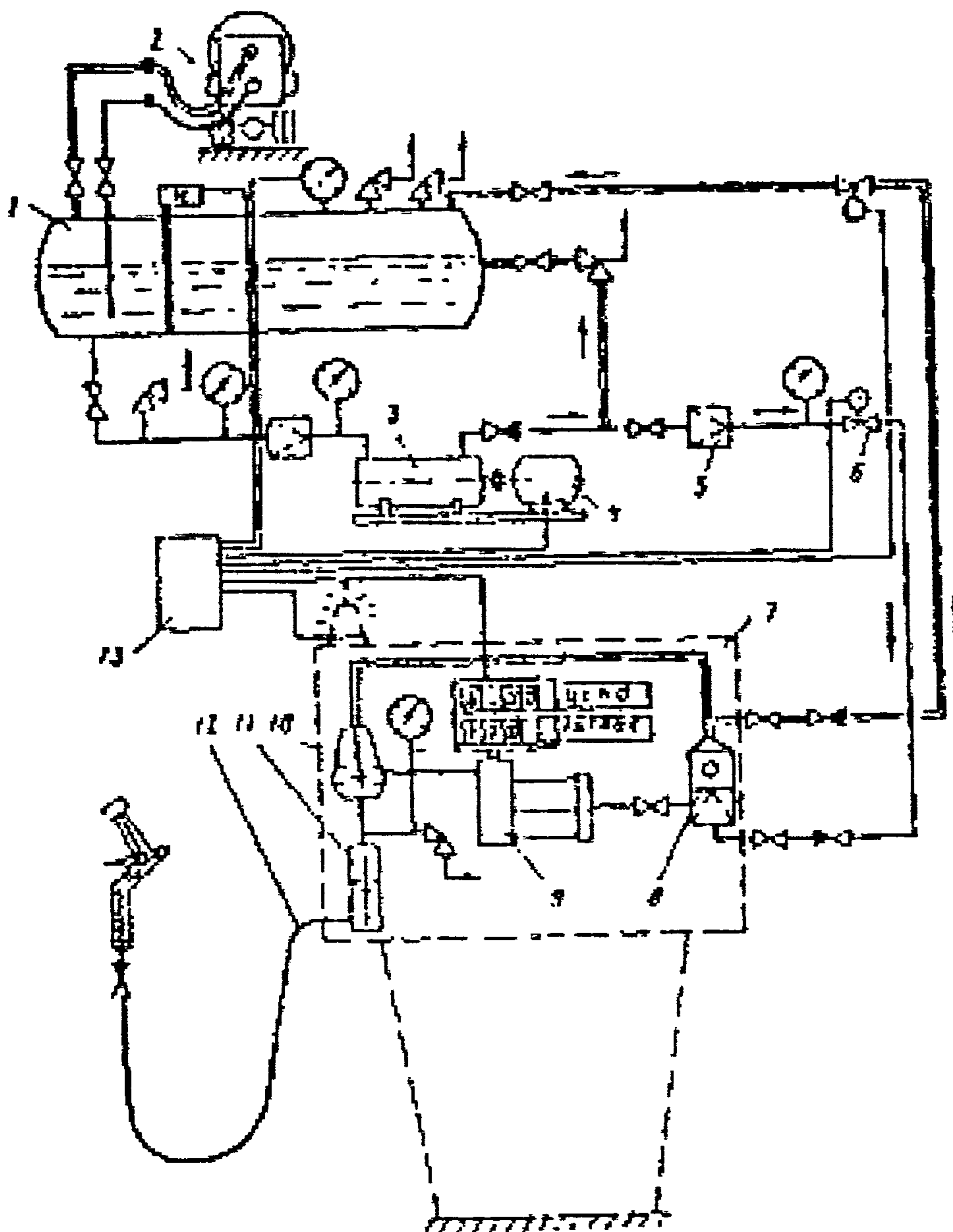
Рис. 7.1. Схема газозаправочной станции для заправки автомобиля сжиженным нефтяным газом:
