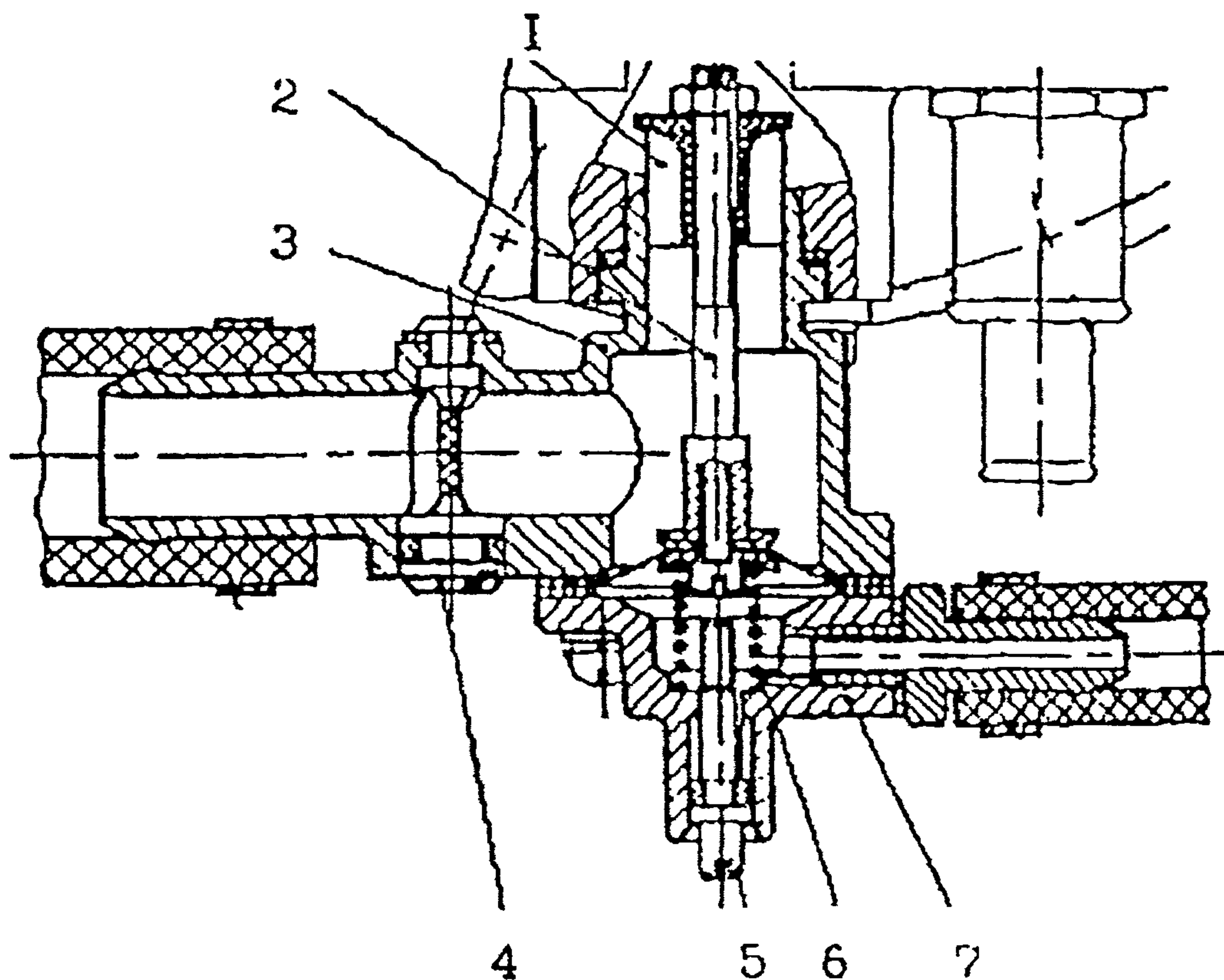
Рис. 4.1. Экономайзер:
