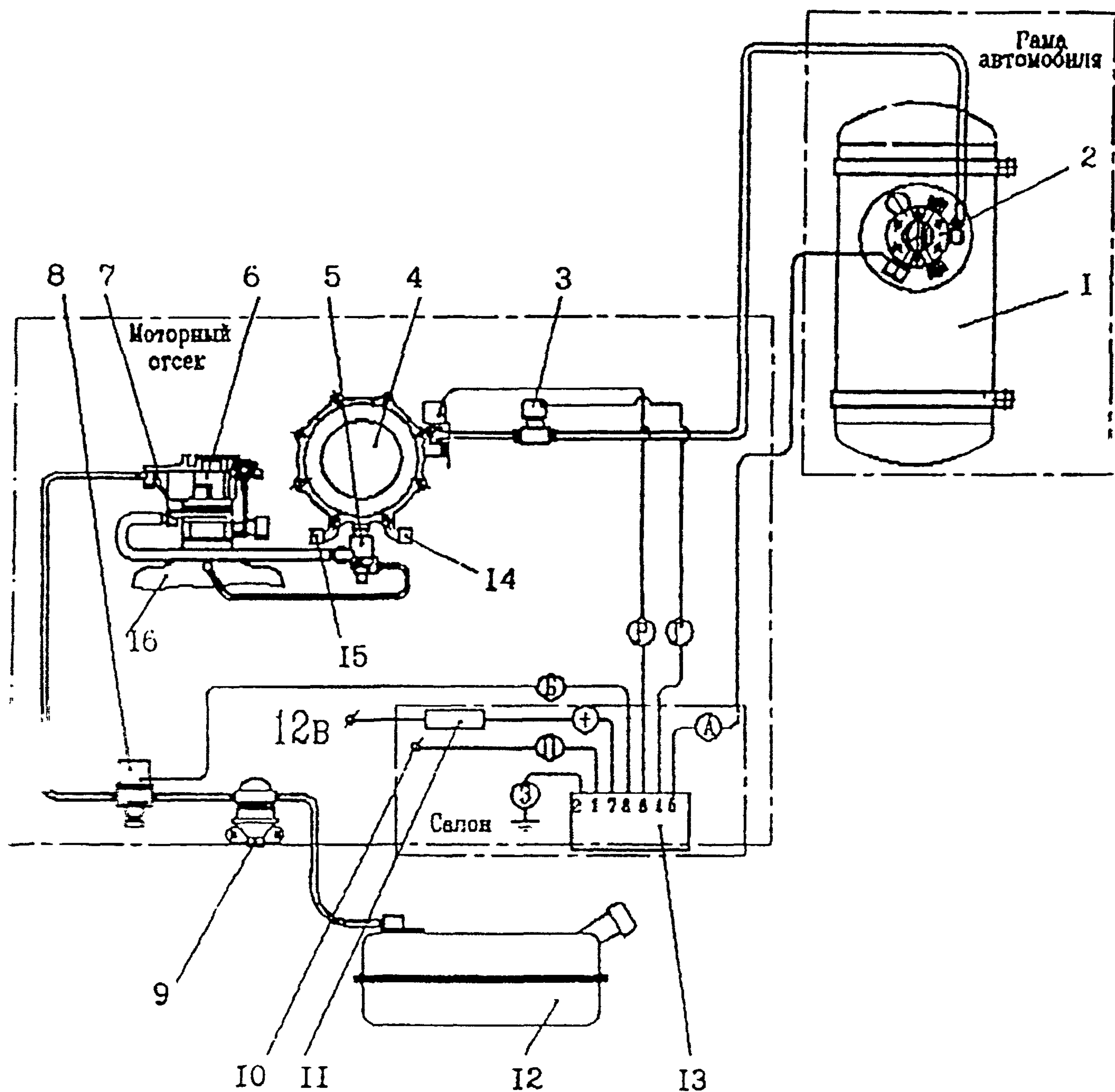
Рис. 3.3. Схема принципиальная газобаллонной установки АО «ЭКОРТ» для грузовых автомобилей: 1 - баллон автомобильный газовый, 2 - блок арматуры, 3 - клапан электромагнитный газовый, 4 - редуктор - испаритель, 5 - экономайзер, 6 - карбюратор, 7 - смеситель, 8 - клапан электромагнитный бензиновый, 9 - бензонасос, 10 - распределитель, 11 - предохранитель, 12 - бензобак, 13 - электронный блок БЕГ-3; 14 - рукав водяной подводящий, 15 - рукав водяной отводящий, 16 - коллектор впускной
