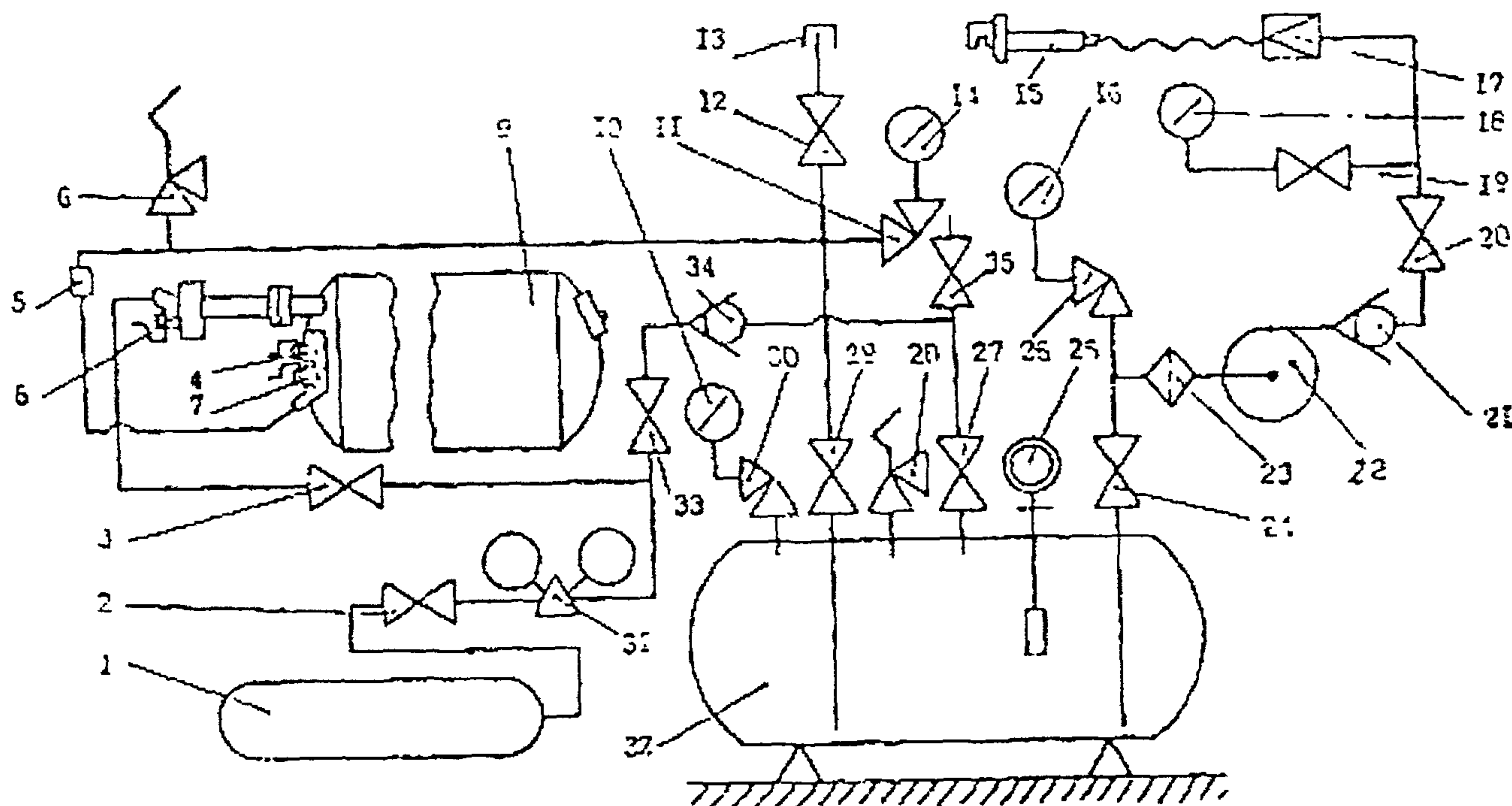
Рис. 5.2. Технологическая схема установки для слива ГСН (вытеснительный вариант):
