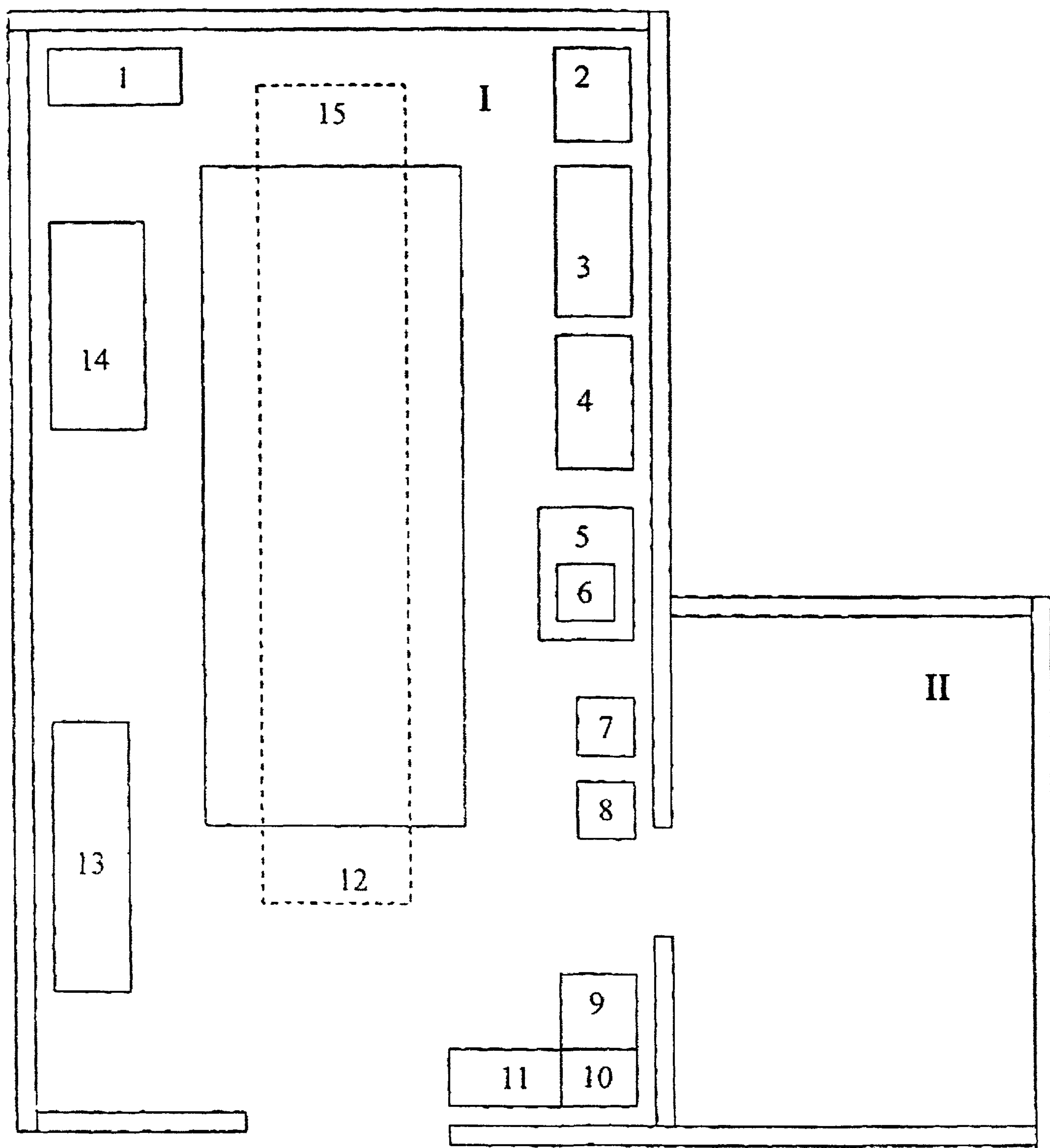
Рис. 5.6. Участок ТО и ТР газобаллонных автомобилей:
