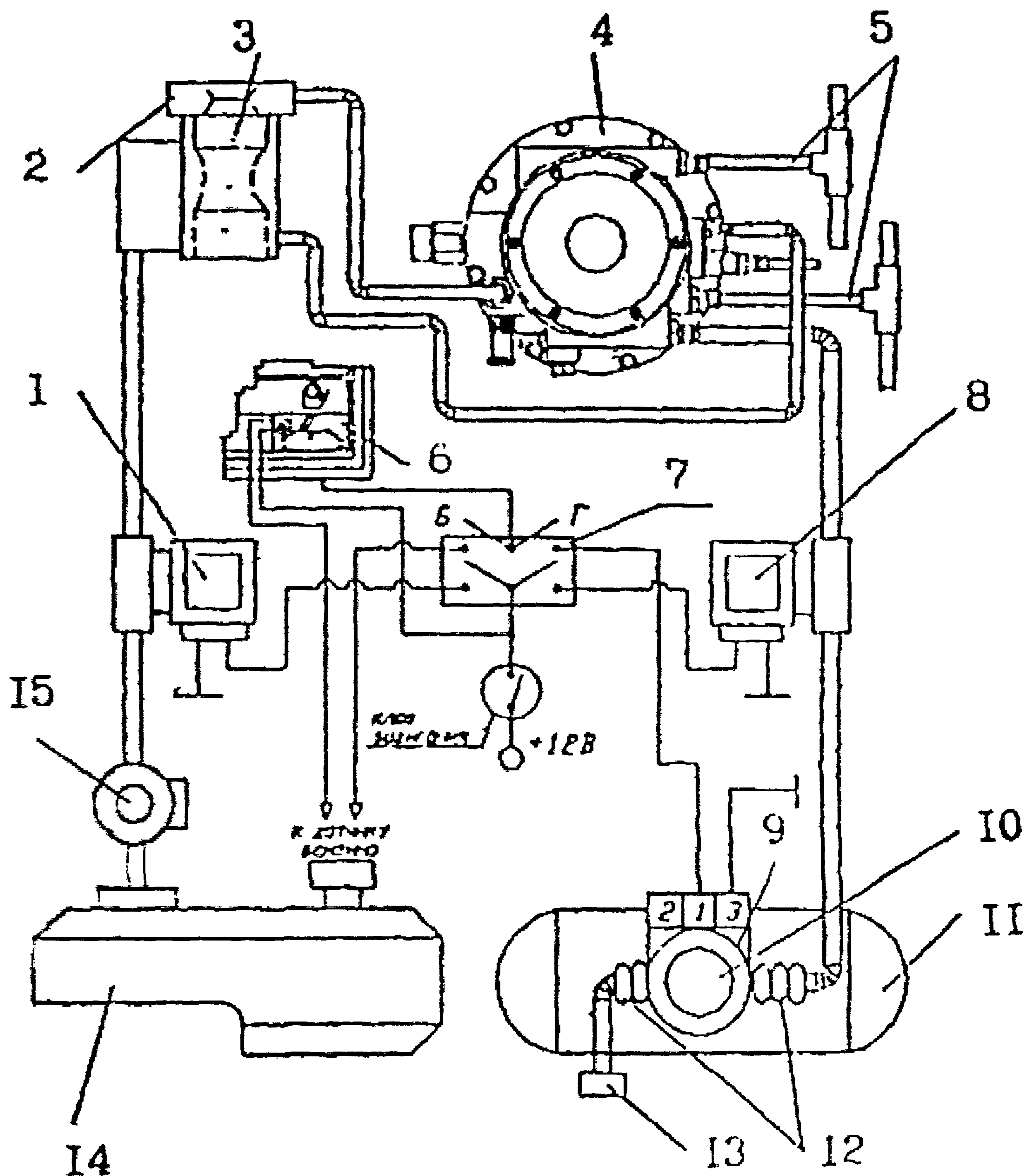
Рис. 3.6. Схема принципиальная газобаллонной установки «САГА-6» для легковых автомобилей:
