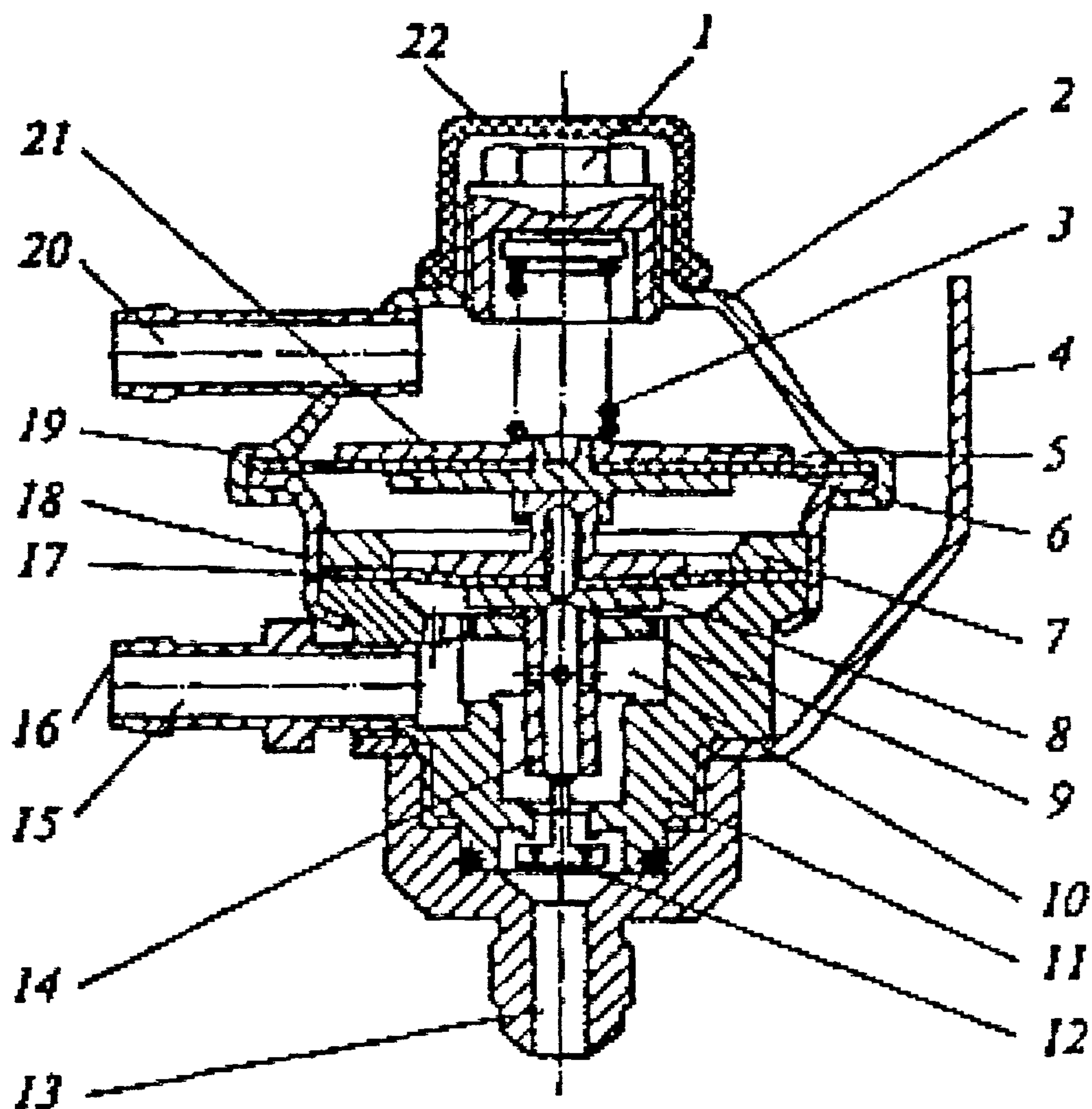
Рис. 3.11. Редуктор дифференциальный:
