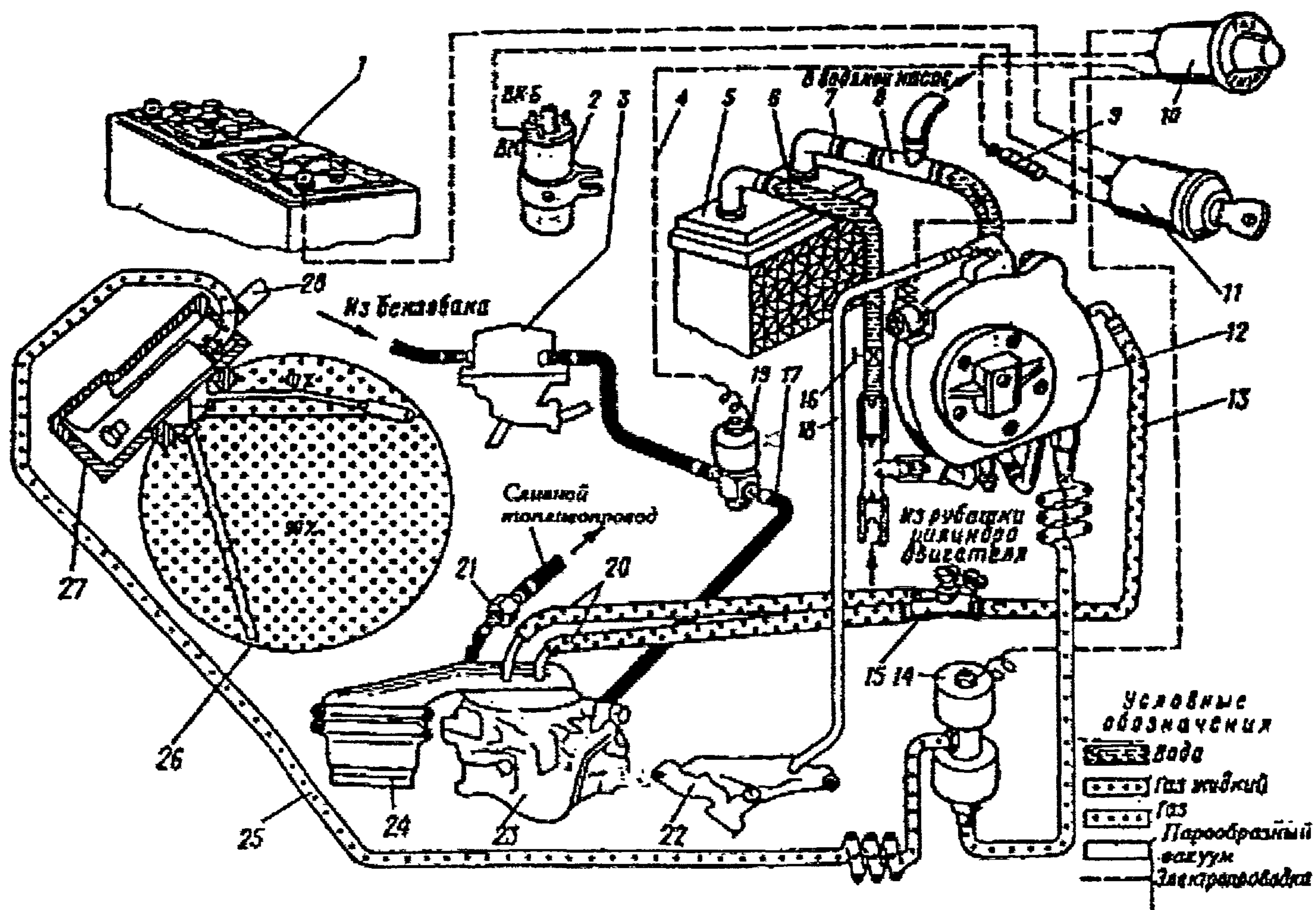
Рис. 3.5. Схема газобаллонной аппаратуры Новоградского завода:
