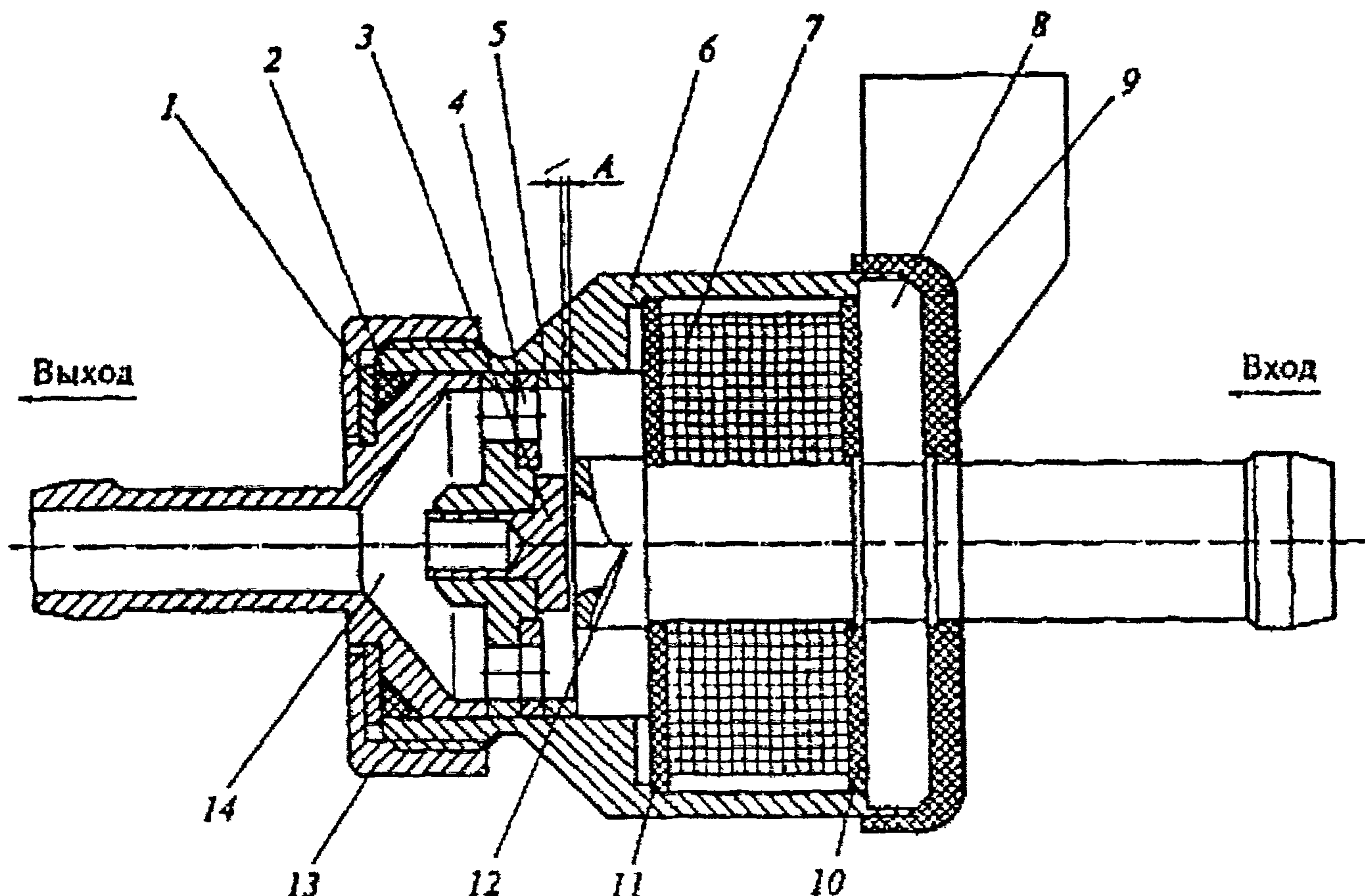
Рис. 3.12. Инжектор газовый:
