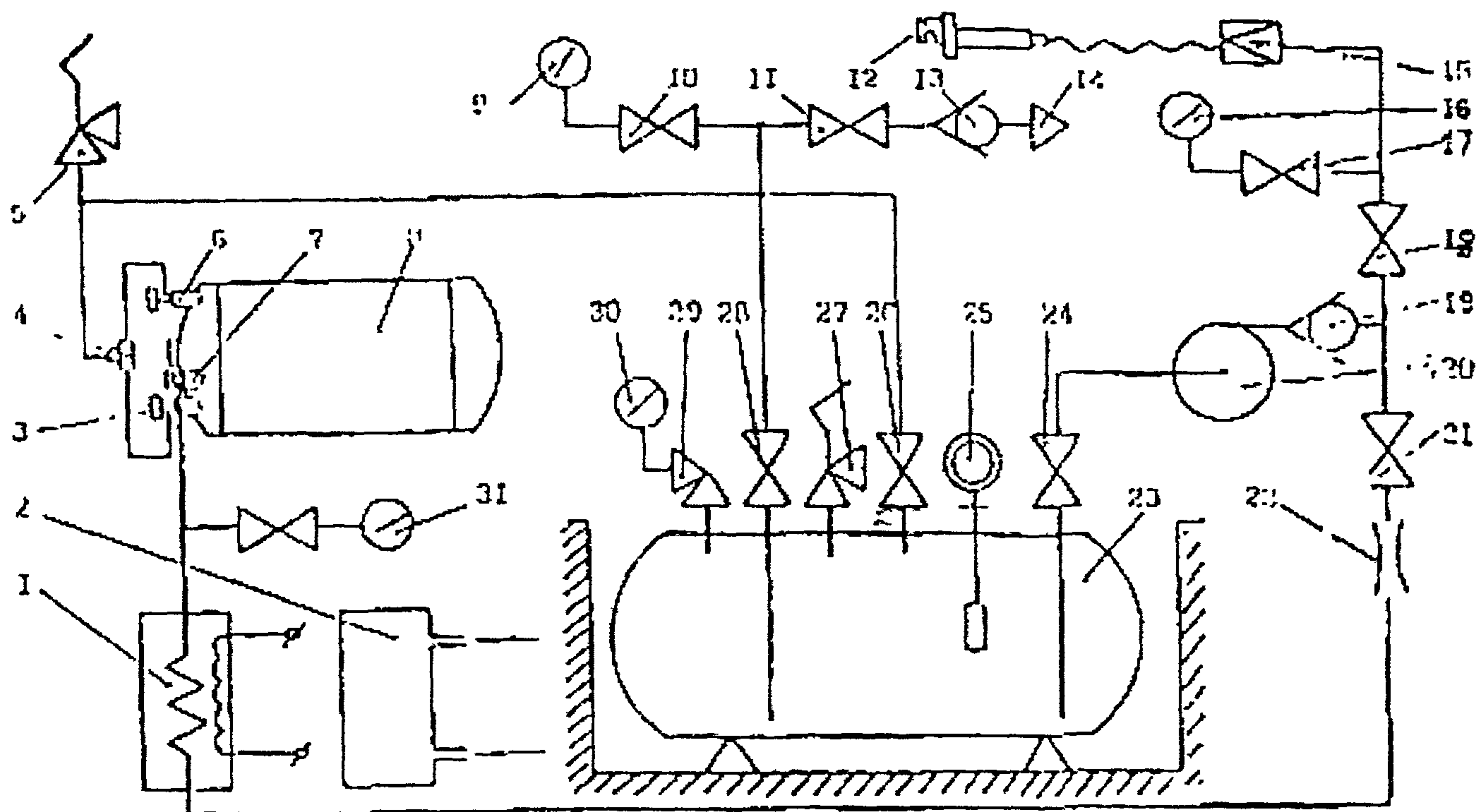
Рис. 5.4. Технологическая схема установки для слива ГСН (теплообменный вариант):
