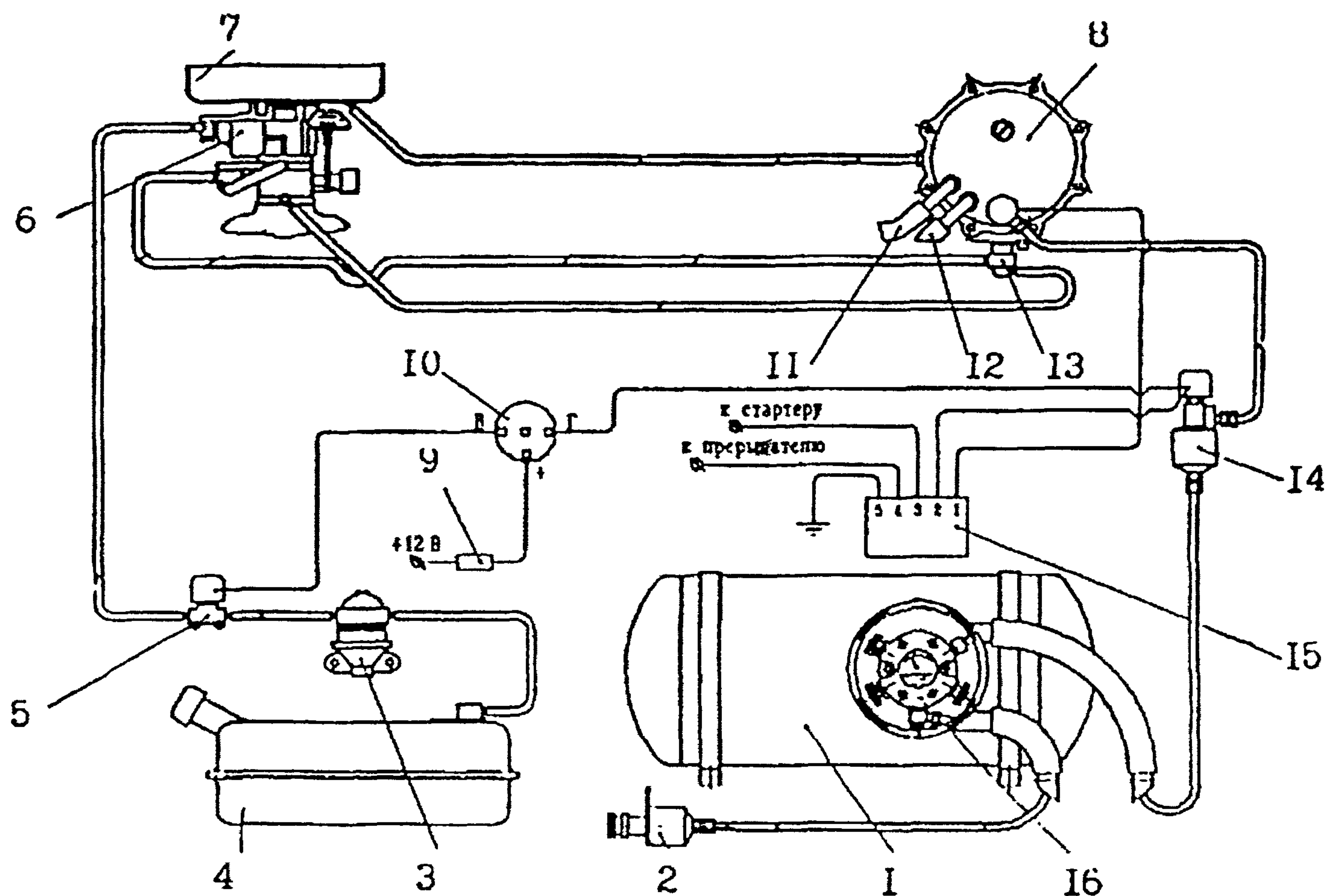
Рис. 3.4. Схема принципиальная газобаллонной установки ПО «УралВЗ» для легковых автомобилей: 1 - баллон автомобильный газовый, 2 - устройство заправочное выносное, 3 - бензонасос, 4 - бензобак, 5 - клапан электромагнитный бензиновый, 6 - карбюратор, 7 - смеситель, 8 - редуктор - испаритель, 9 - предохранитель, 10 - переключатель вида топлива, 11 - рукав водяной подводящий, 12 - рукав водяной отводящий, 13 - экономайзер, 14 - клапан электромагнитный газовый, 15 - блок электронный, 16 - блок арматуры
