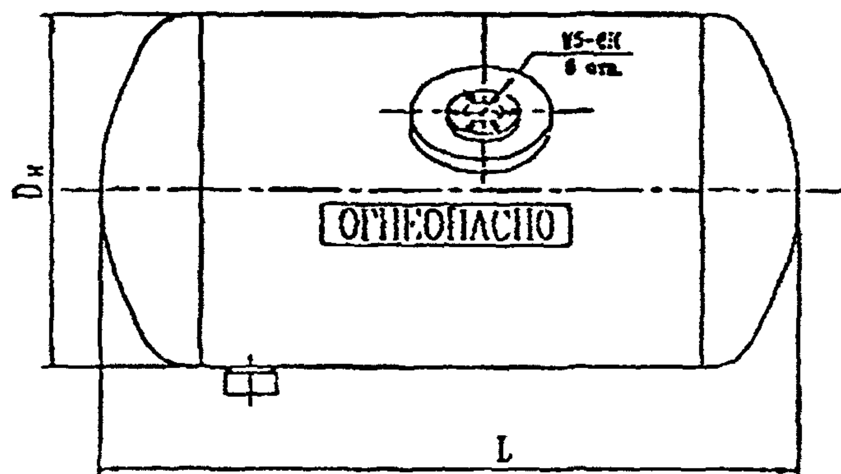
Рис. 3.7. Баллоны автомобильные газовые:
