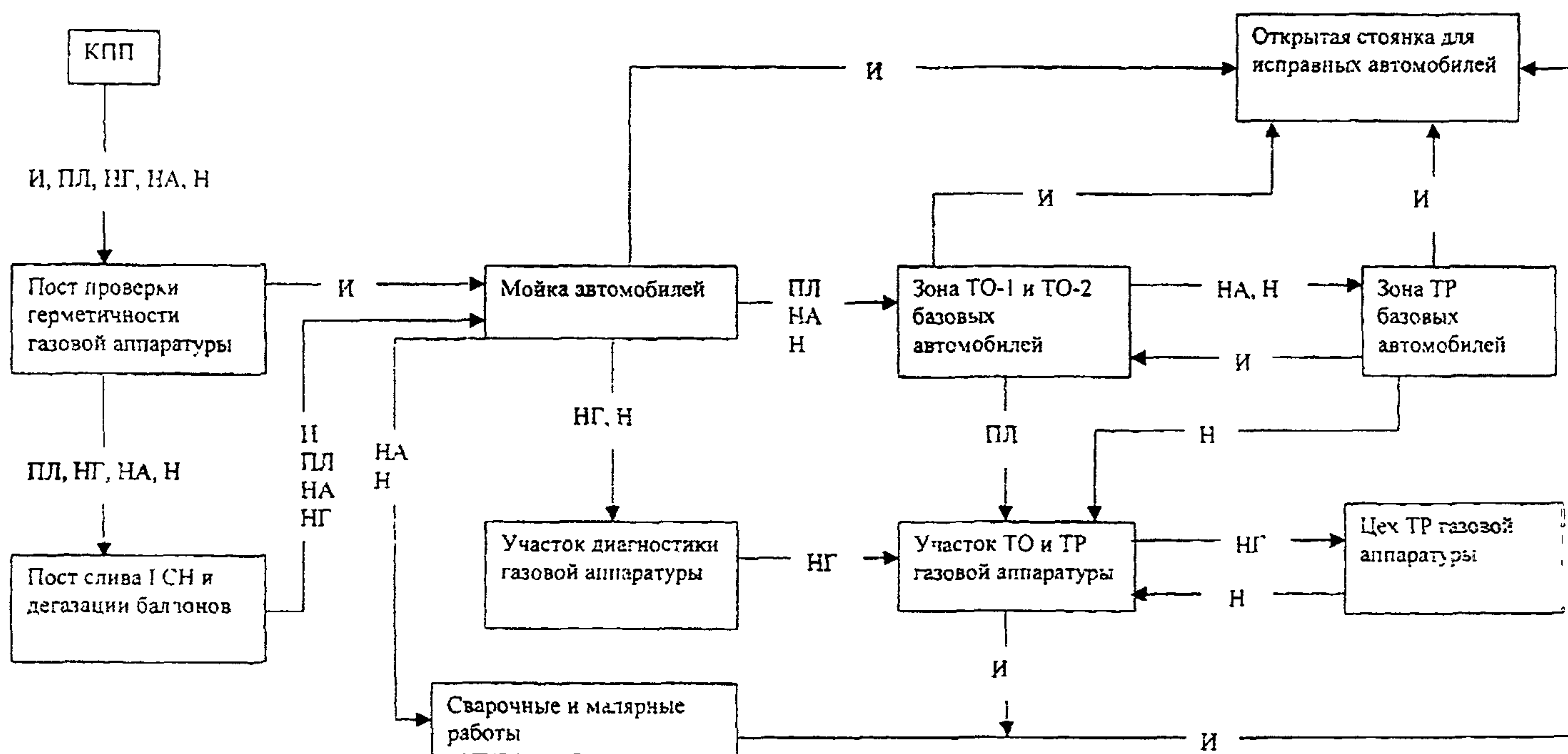
Рис. 5.1. Типовая технологическая схема проведения ТО и ТР газобаллонных автомобилей в условиях АТП:
