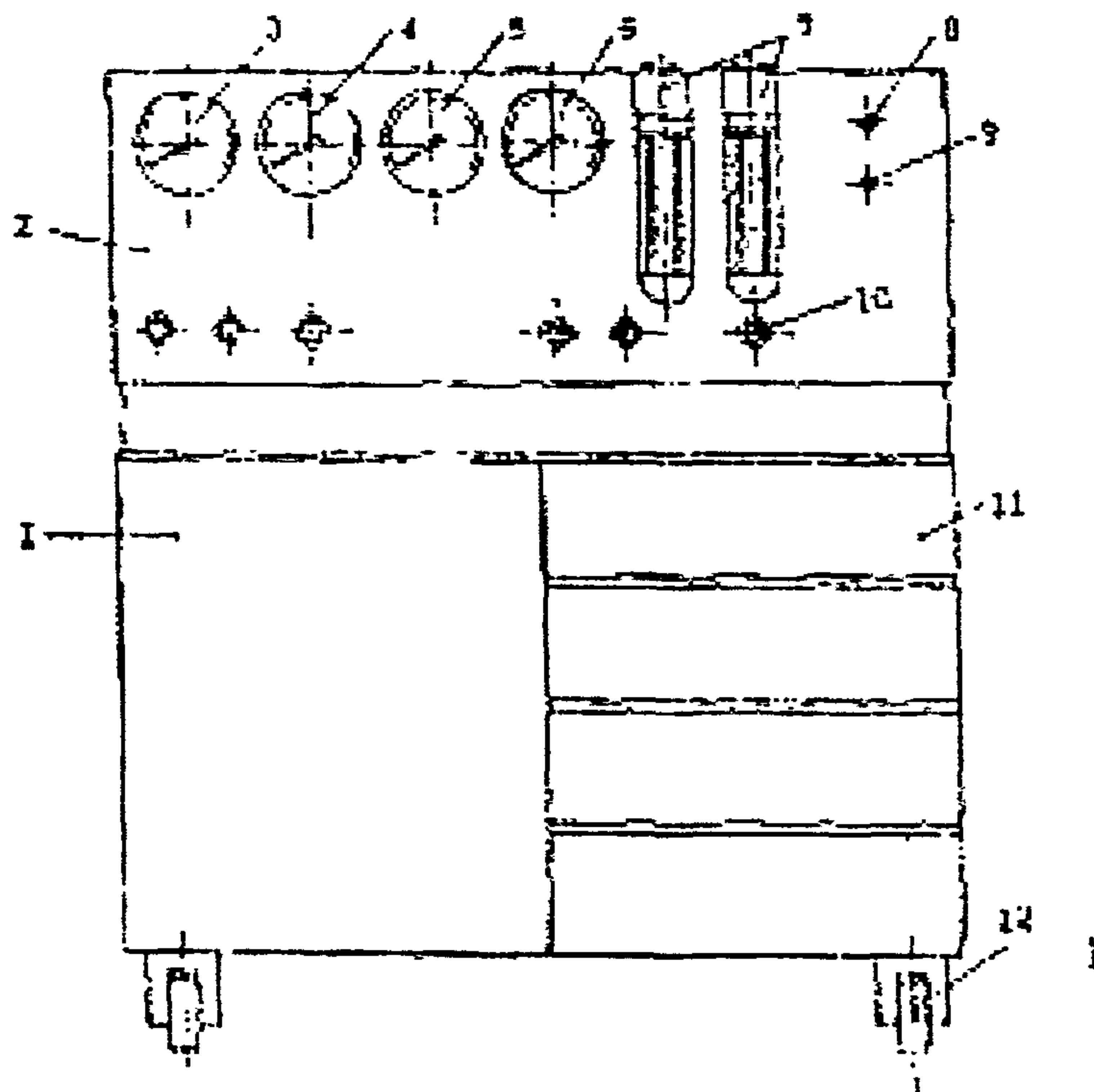
Рис. 6.1. Передвижная установка К-277 для проверки аппаратуры автомобилей:
