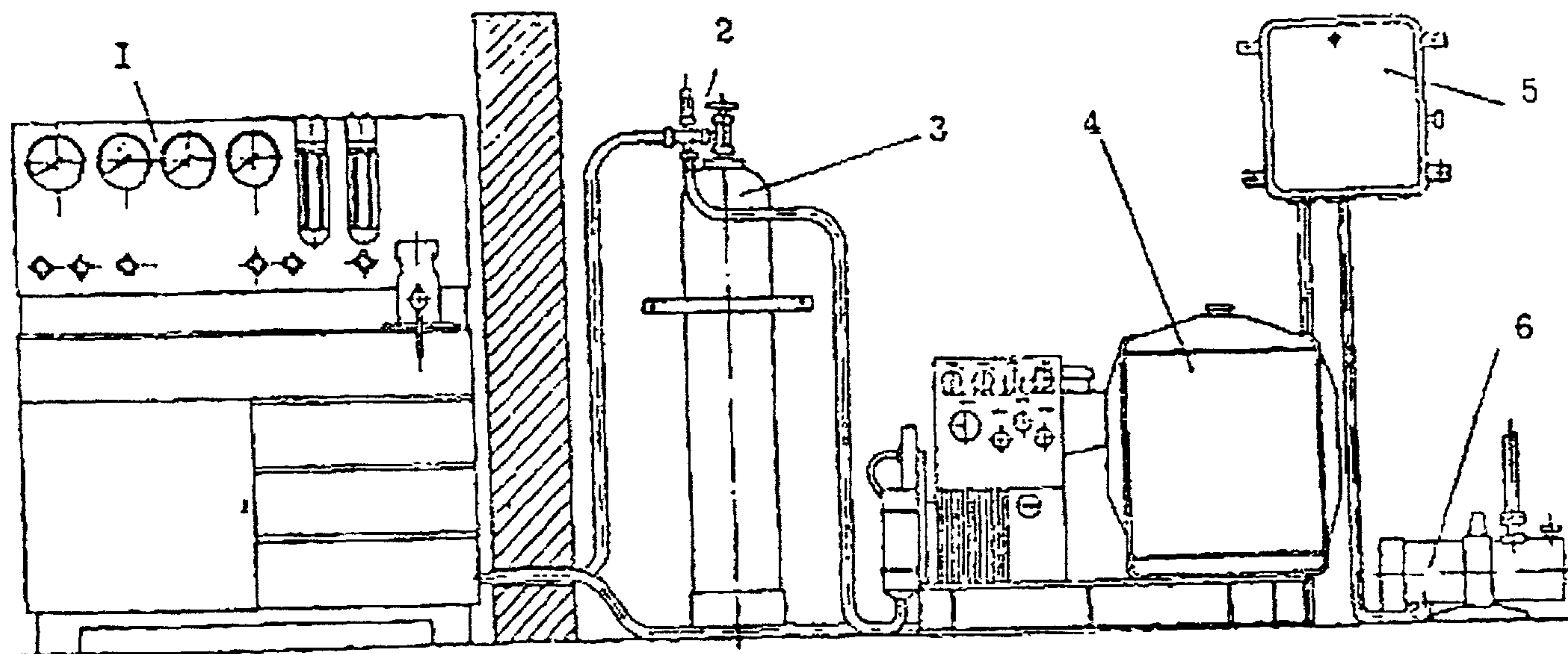
Рис. 6.2. Стенд для проверки газовой аппаратуры автомобилей, мод. К-278:
