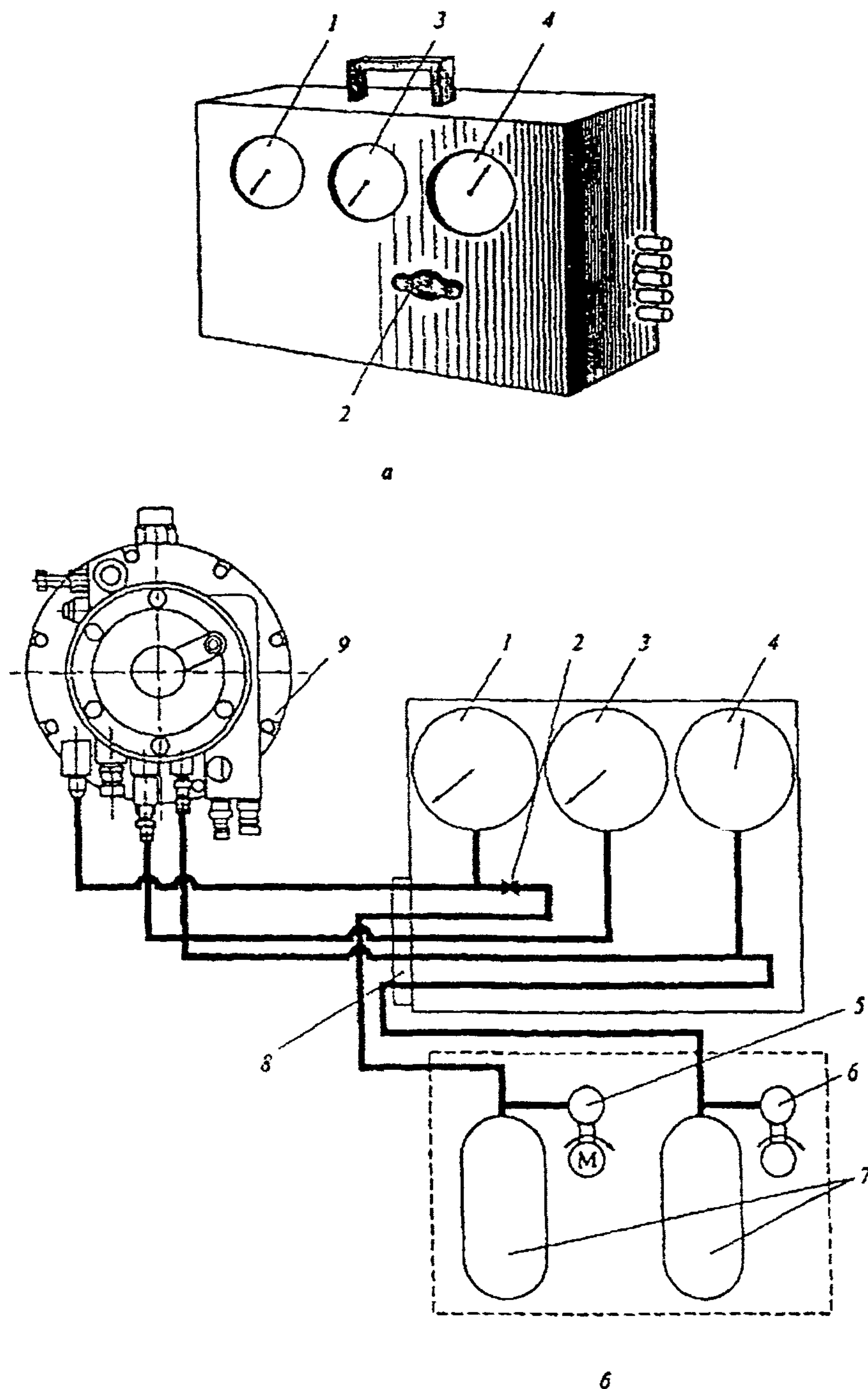
Рис. 6.5. Стенд НПФ «САГА»:
