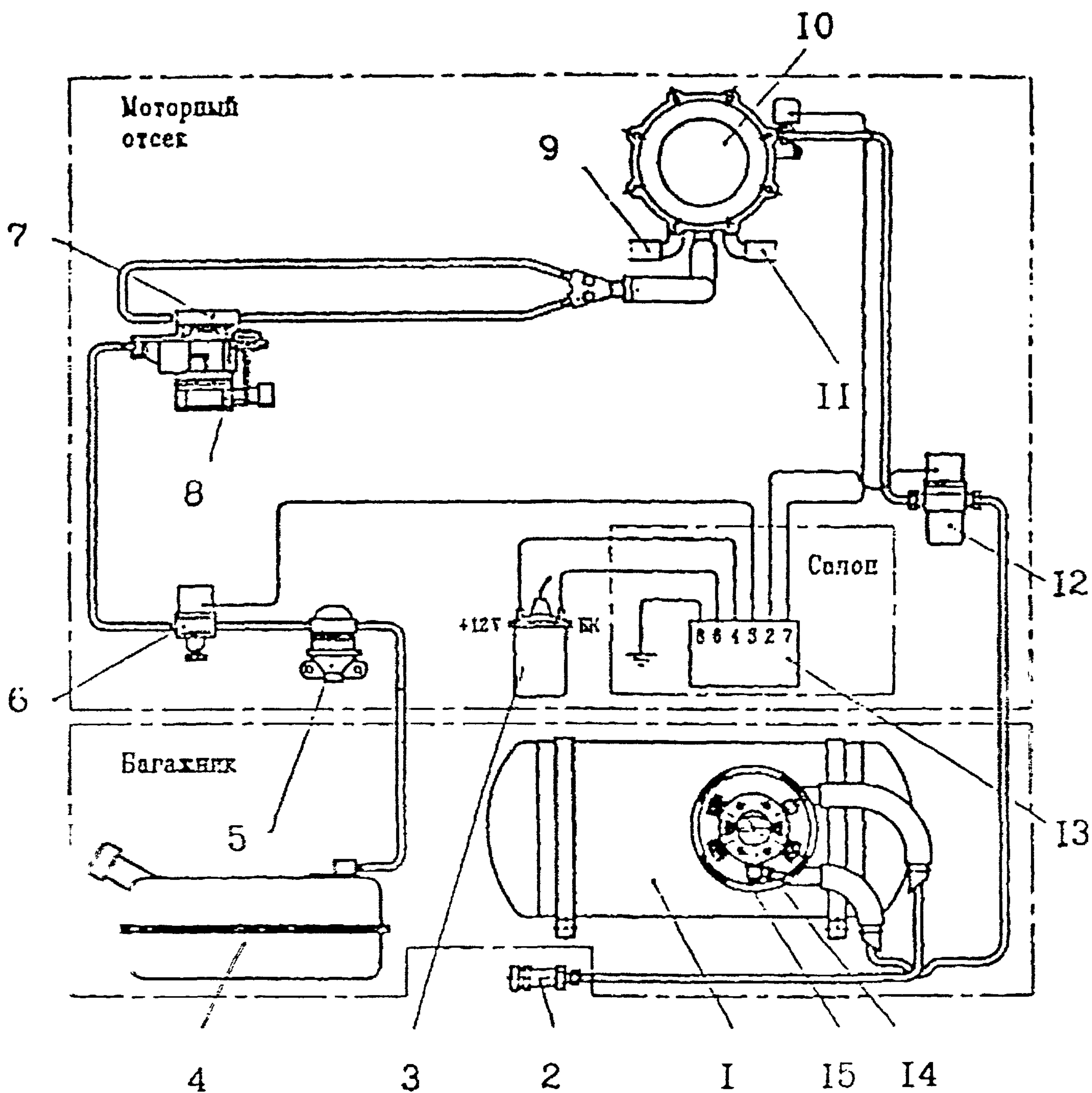
Рис 3.2. Схема принципиальная газобаллонной установки АО «ЭКОРТ» для легковых автомобилей: 1 - баллон автомобильный газовый; 2 - устройство заправочное выносное; 3 - катушка зажигания; 4 - бензобак; 5 - бензонасос; 6 - клапан электромагнитный бензиновый; 7 - смеситель; 8 - карбюратор; 9 - рукав водяной отводящий; 10 - редуктор - испаритель; 11 - рукав водяной подводящий; 12 - клапан электромагнитный газовый; 13 - блок электронный; 14 - блок арматуры; 15 - система вентиляции блока арматуры.
