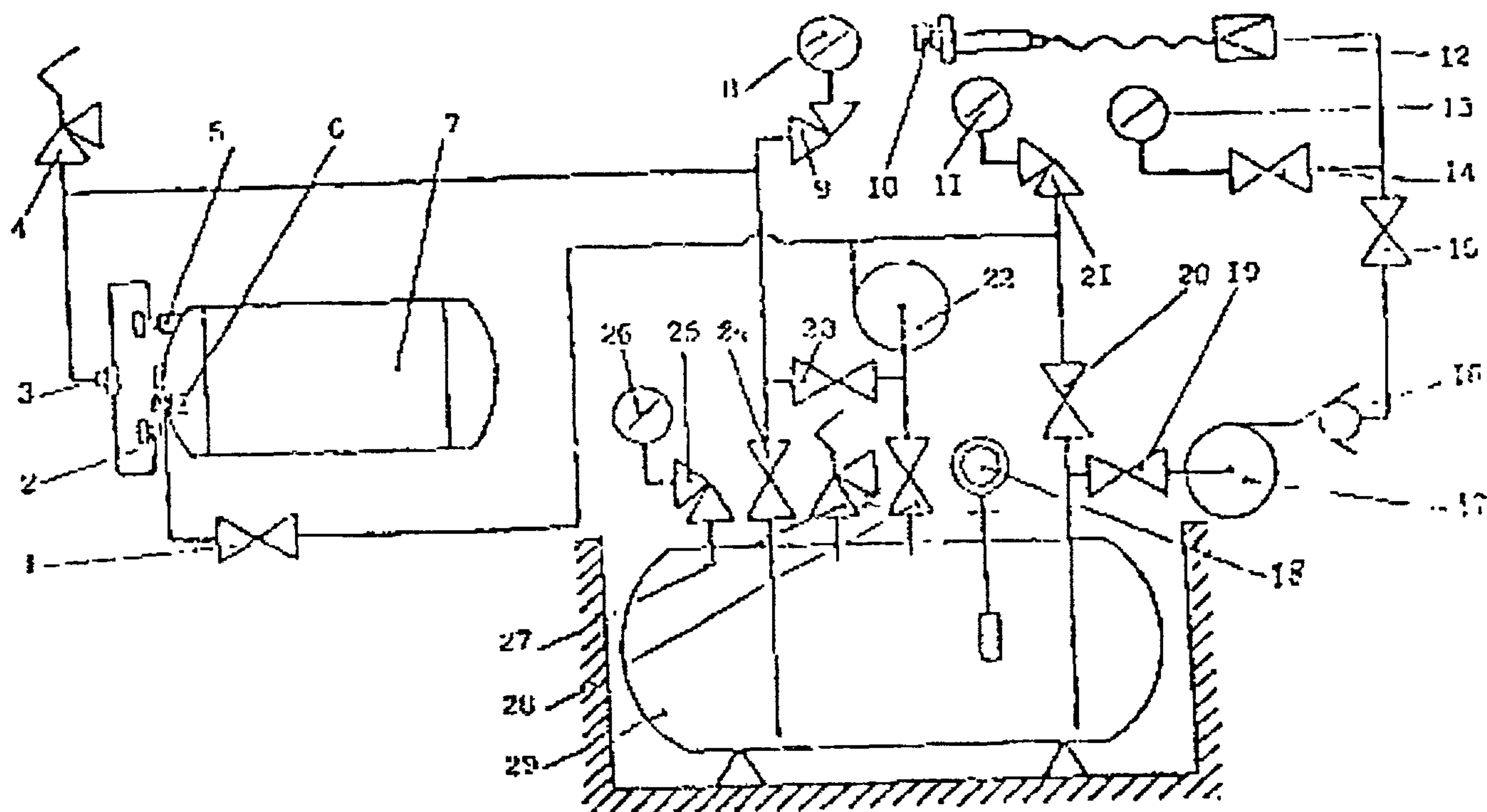
Рис. 5.3. Технологическая схема установки для слива ГСН (компрессорный вариант):
