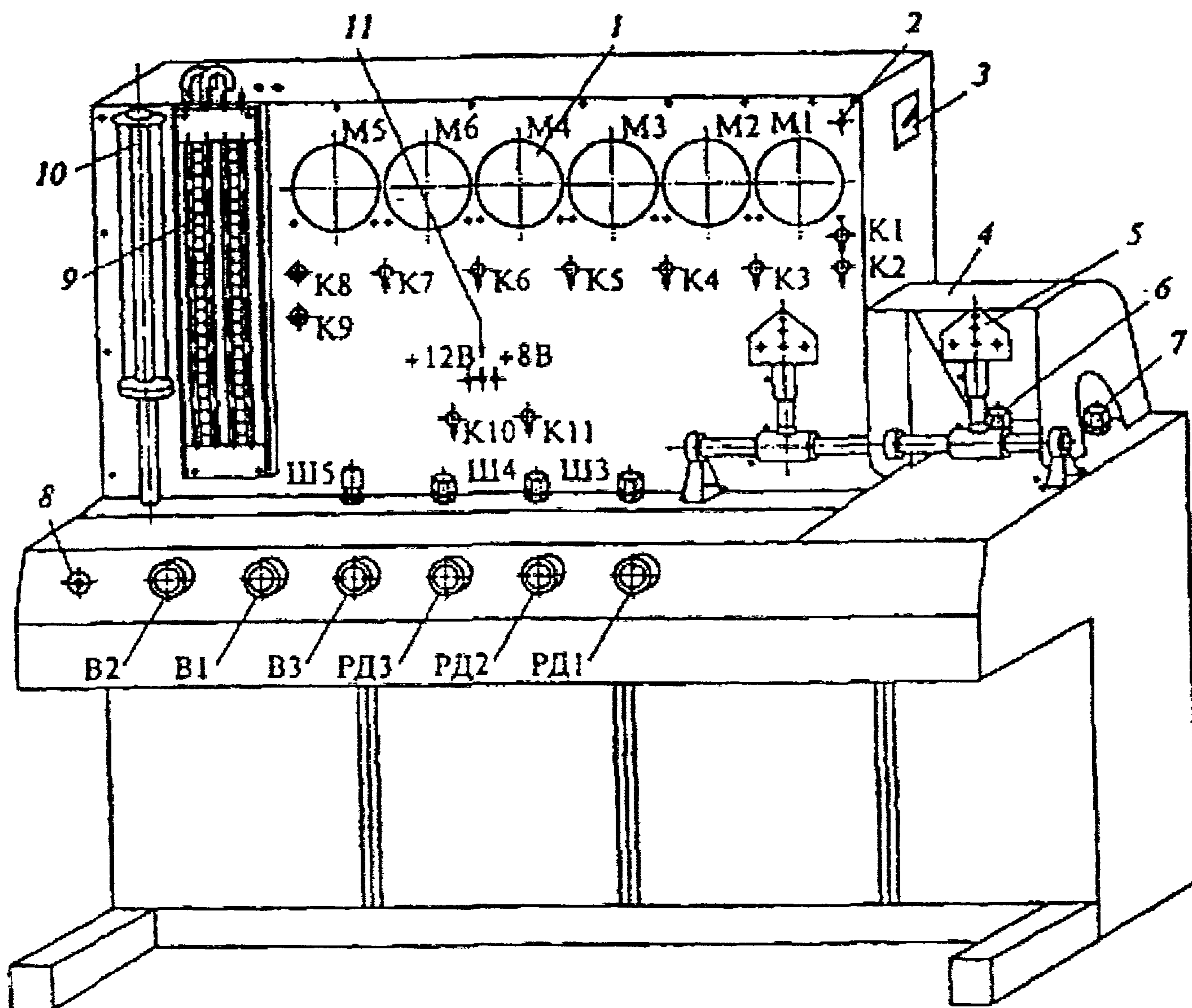
Рис. 6.4. Стенд ИС-001:
