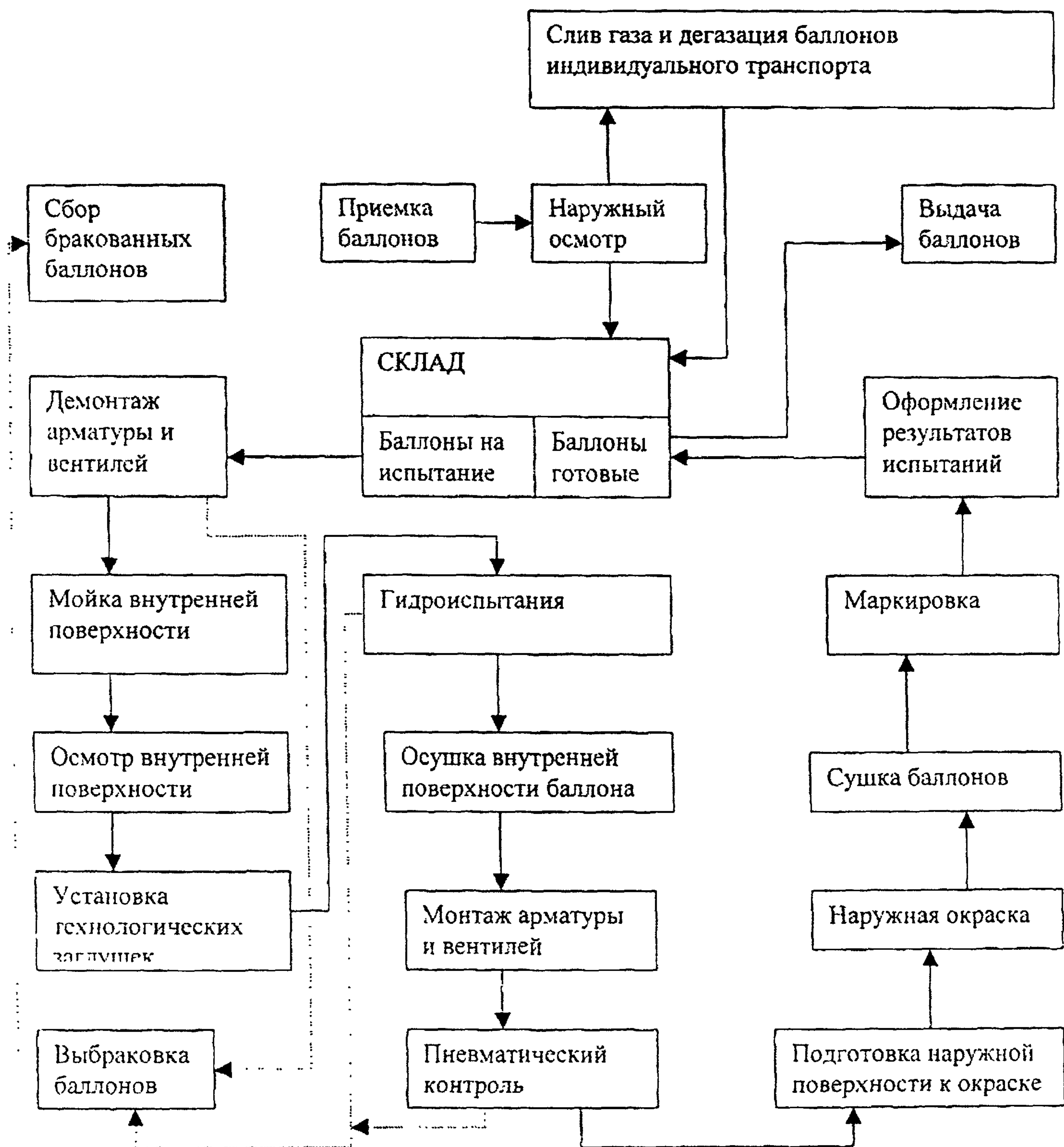
Рис. 9.1. Схема технологического процесса освидетельствования баллонов для ГСН
