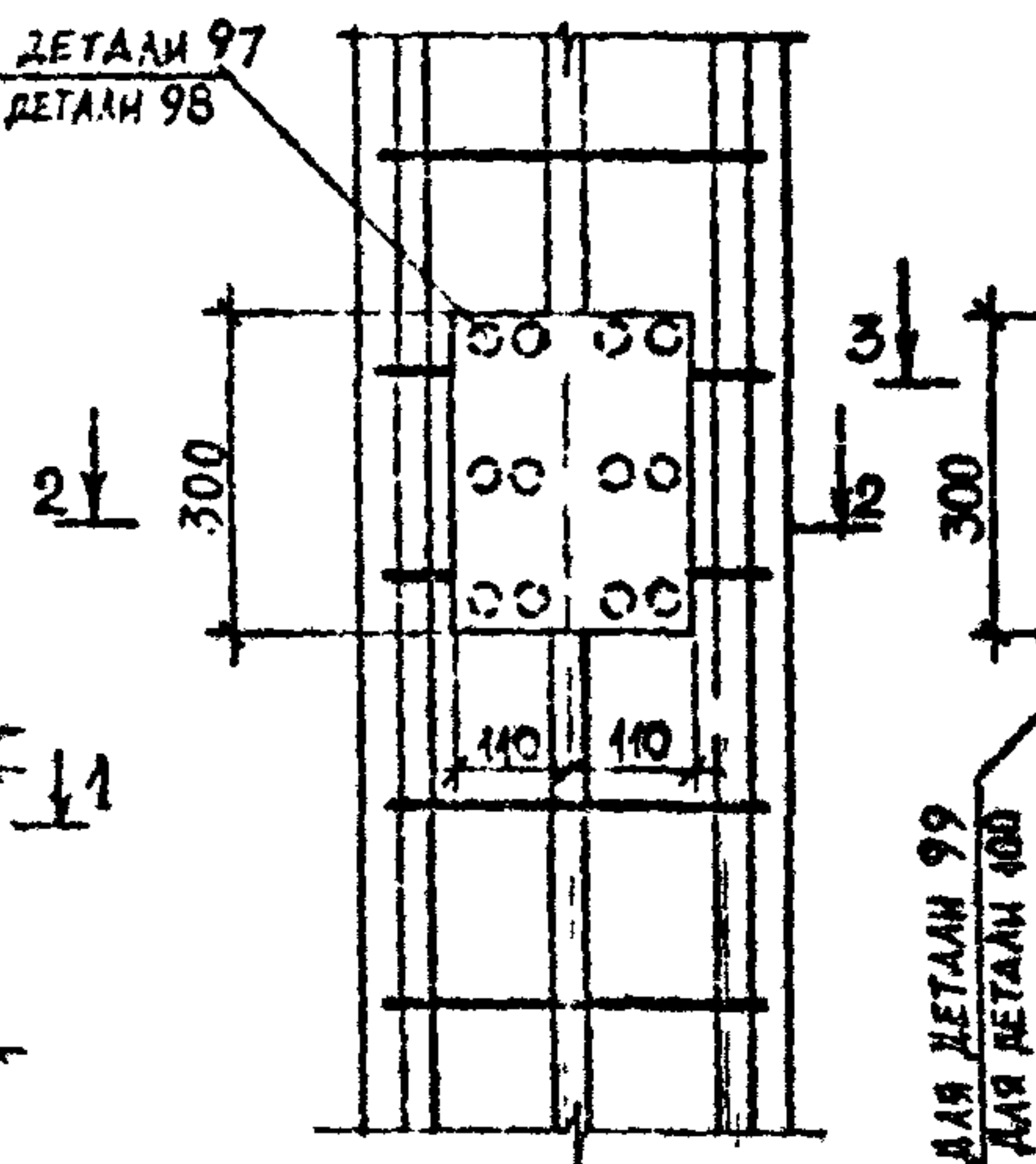
ДЕТАЛЬ 97, 98
