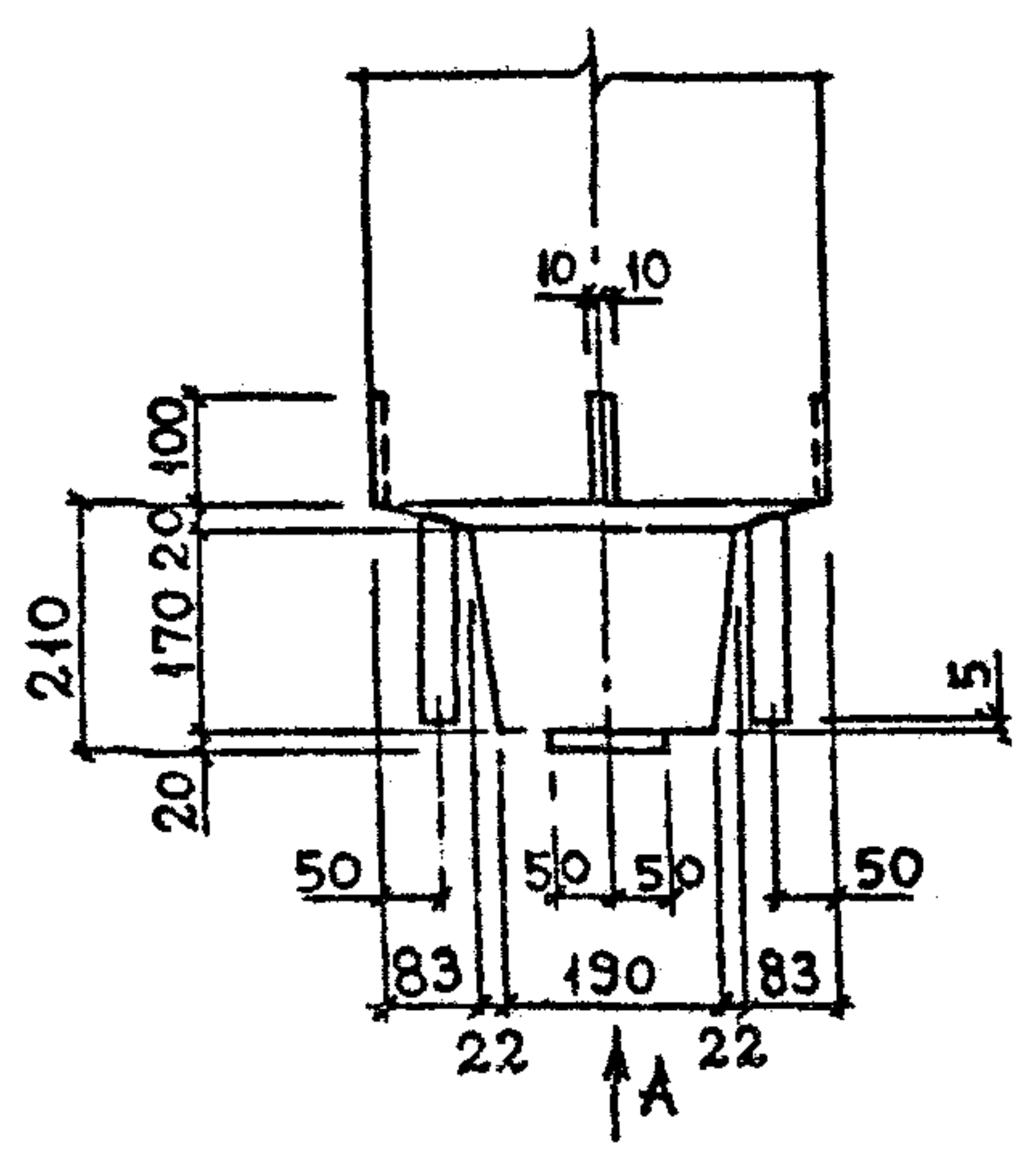
ДЕТАЛЬ 23
