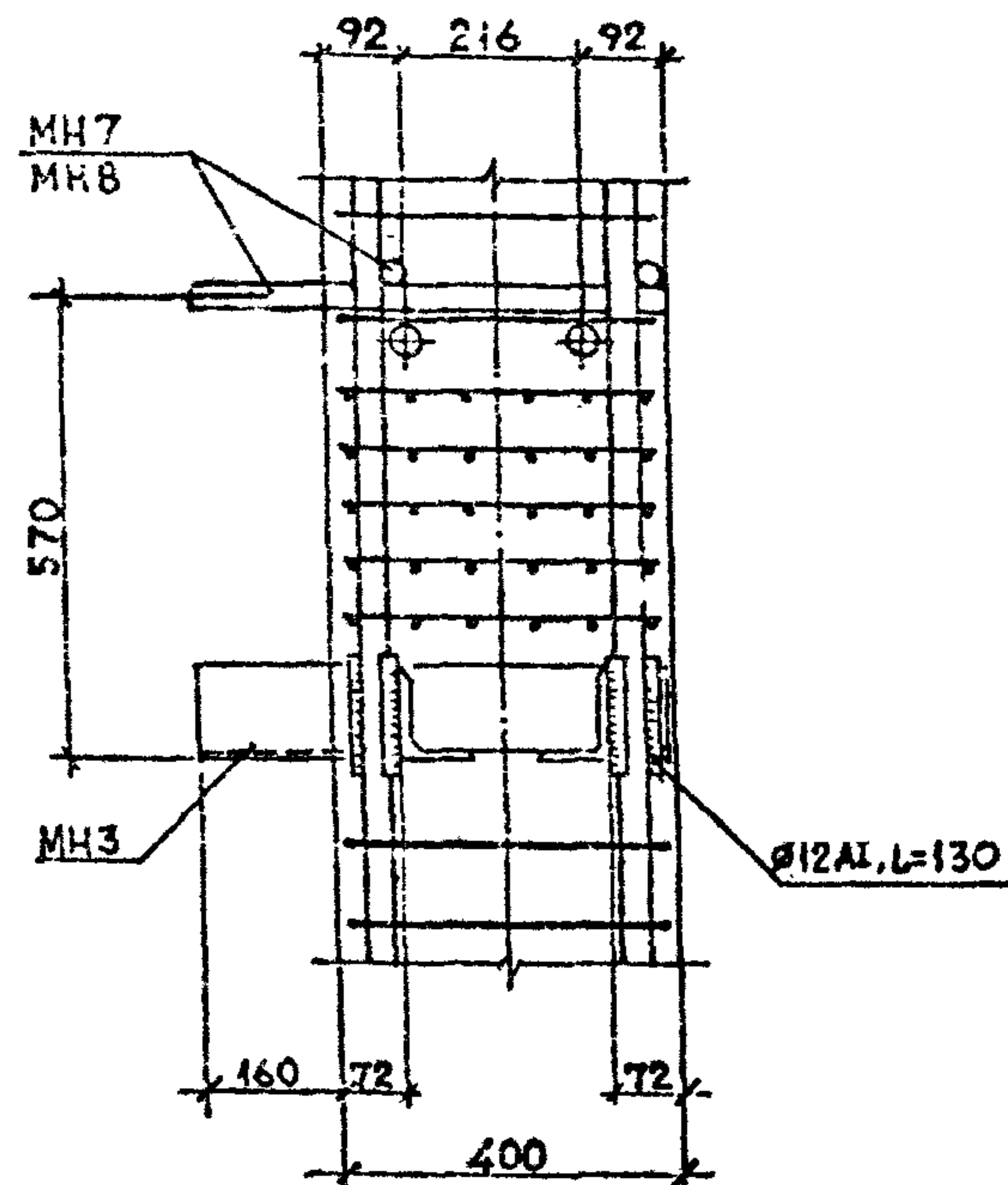
Вид А
