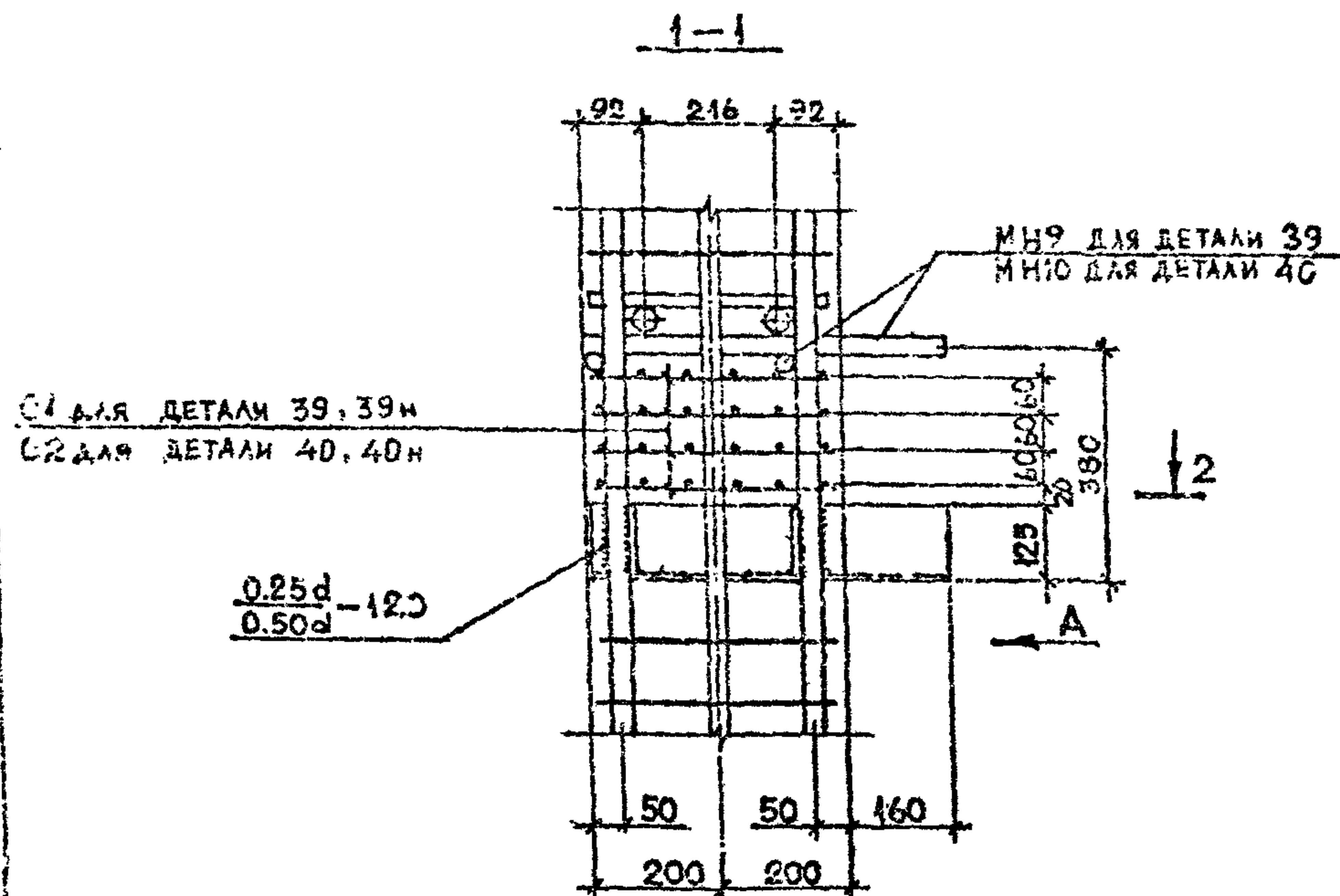
ДЕТАЛЬ 39, 40
