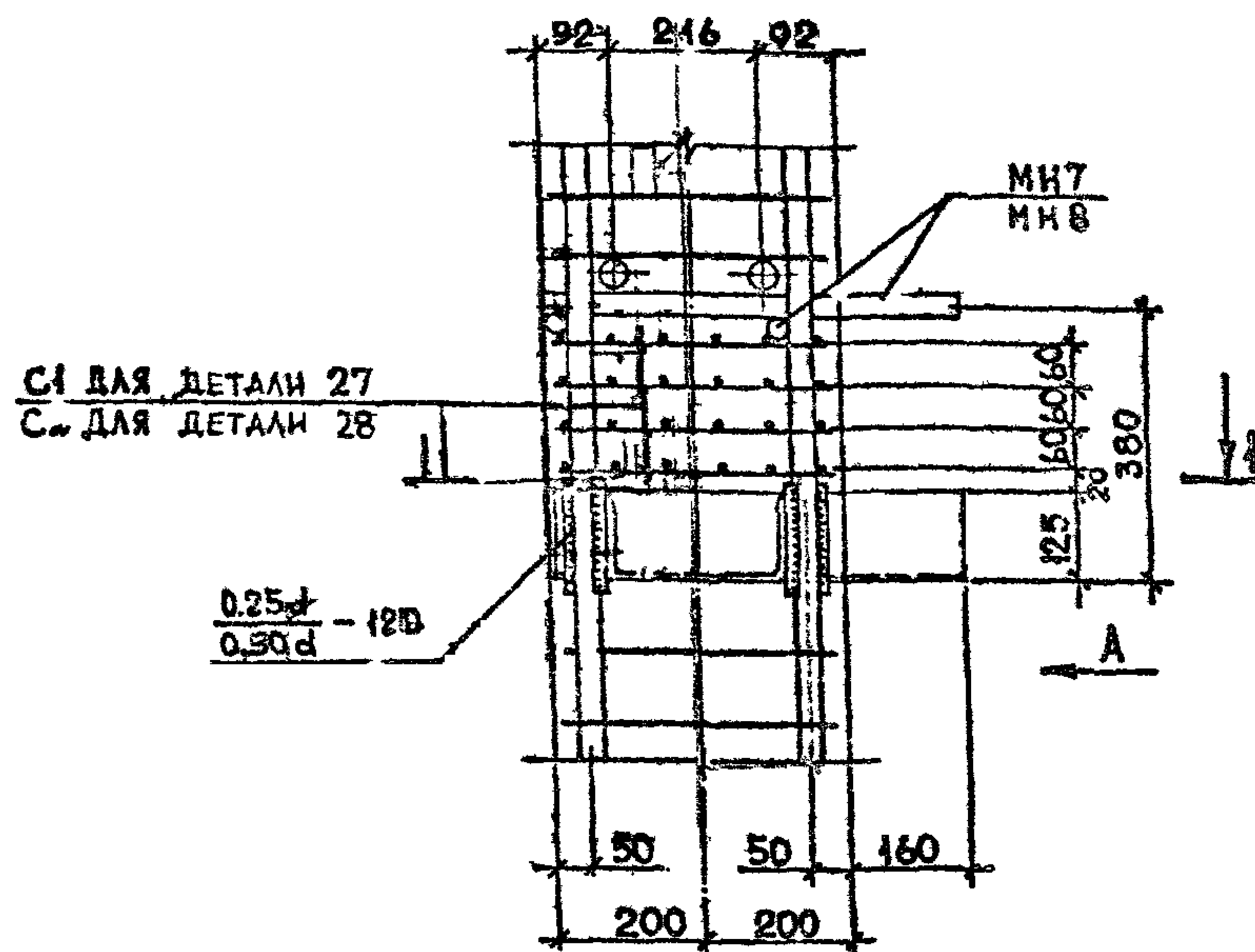
ДЕТАЛЬ 27,28
