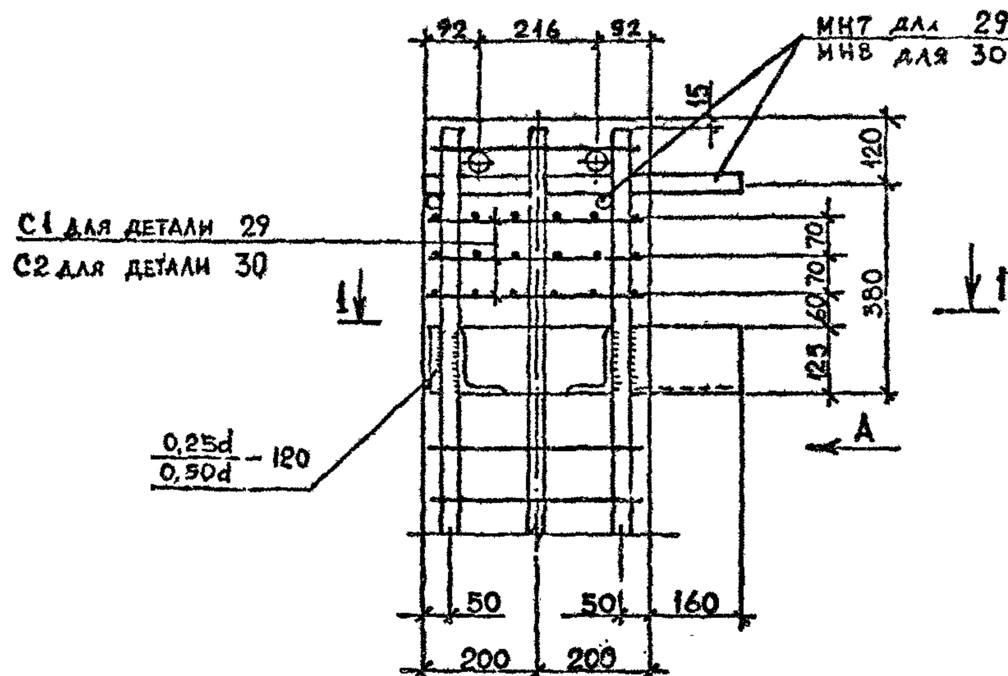
ДЕТАЛЬ 29, 30
