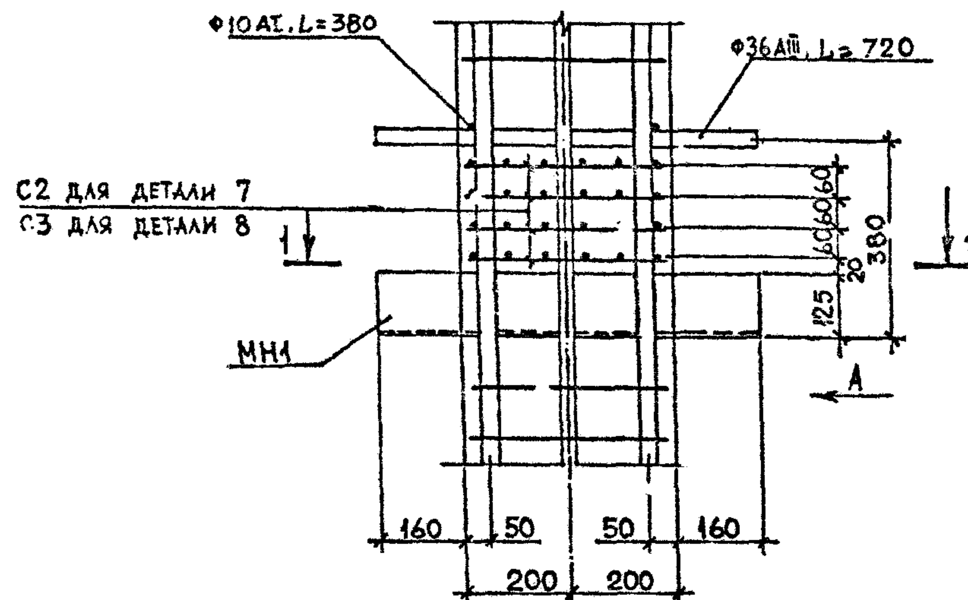
ДЕТАЛЬ 7,8
