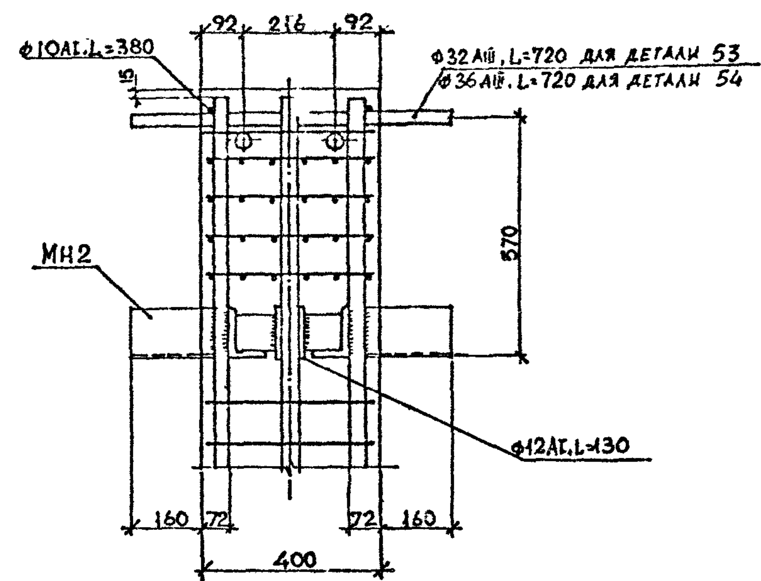
Вид А
