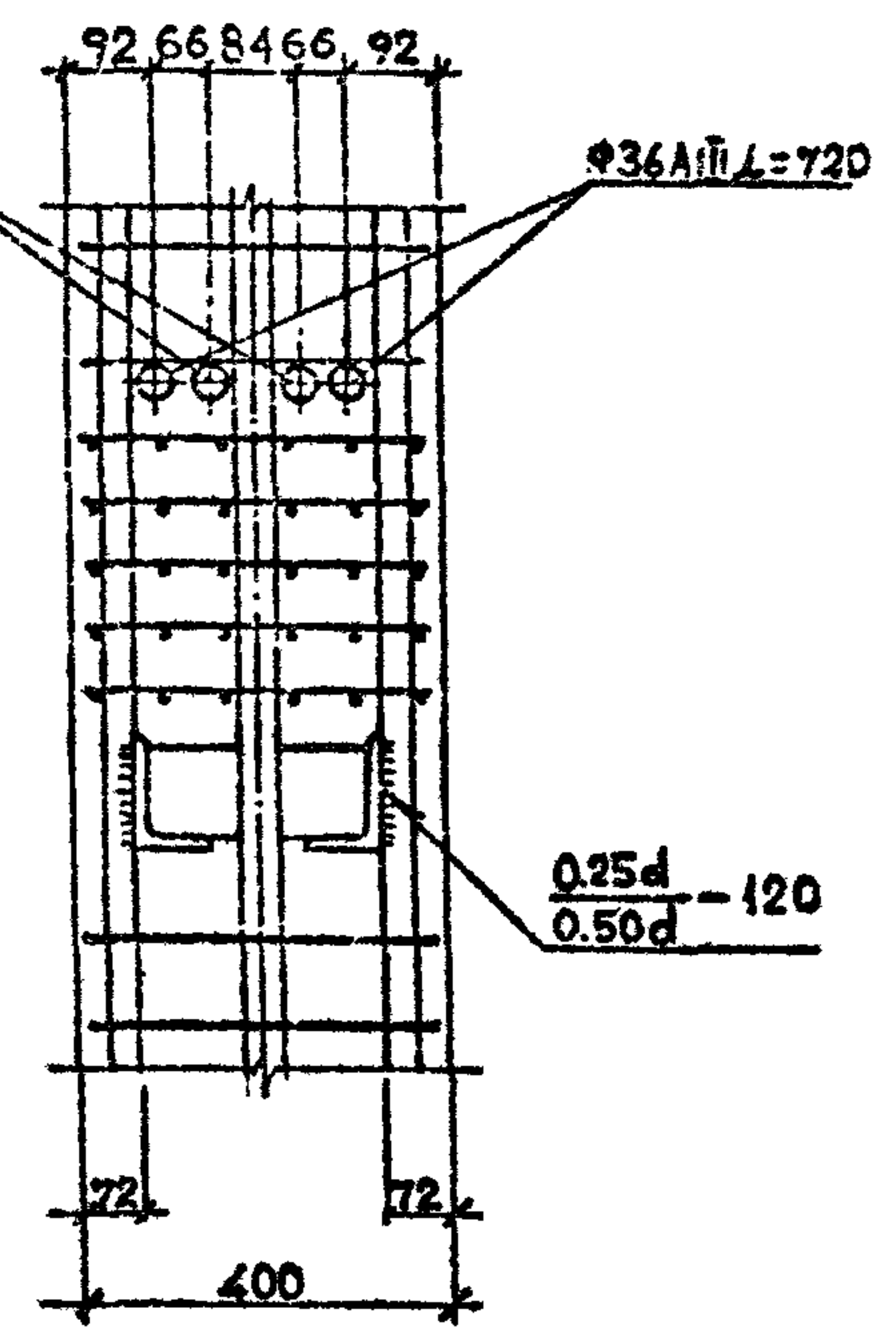
Вид А
