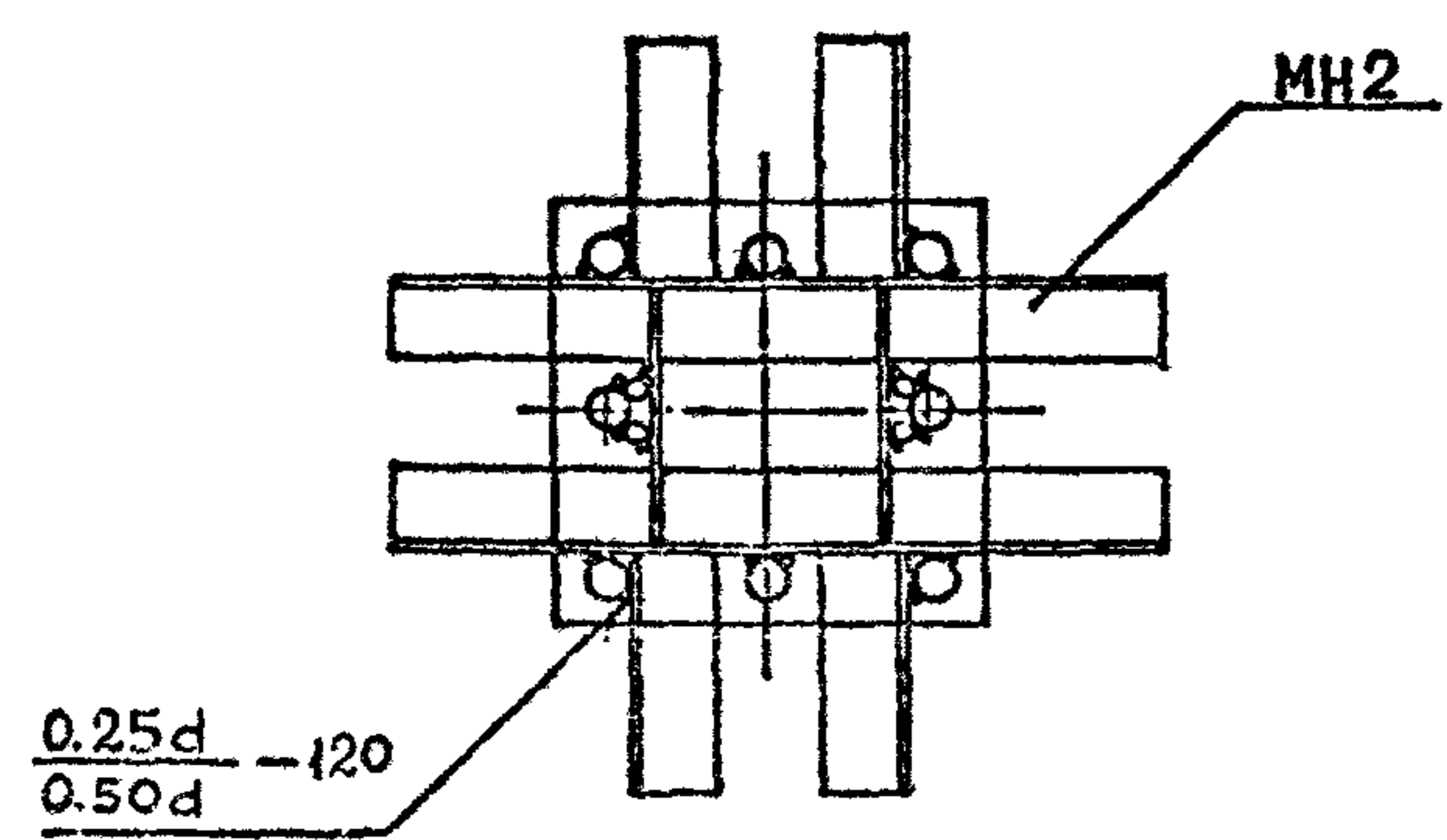
1-1
