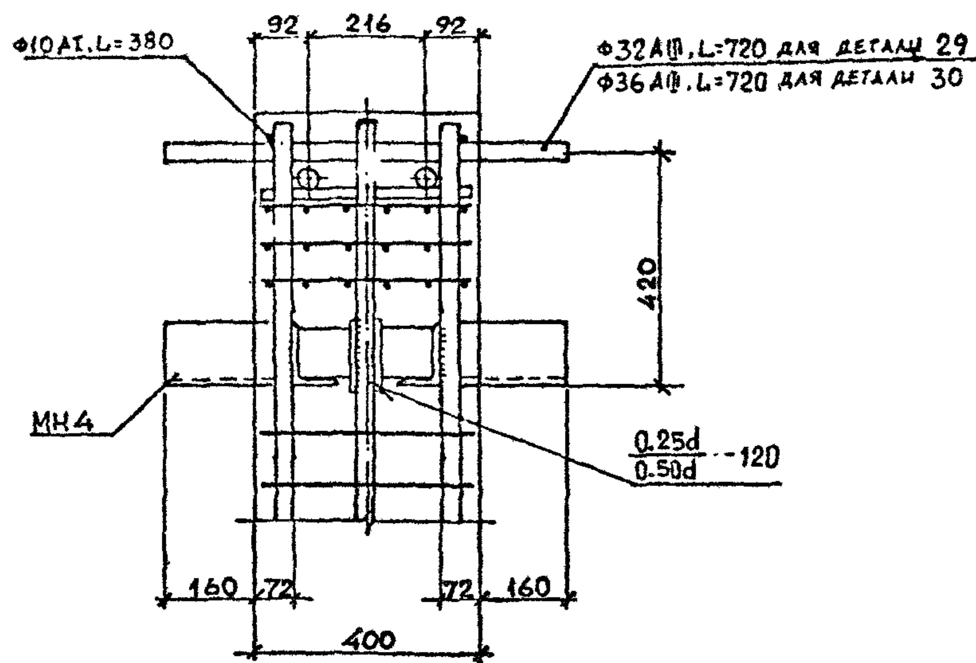
Вид А
