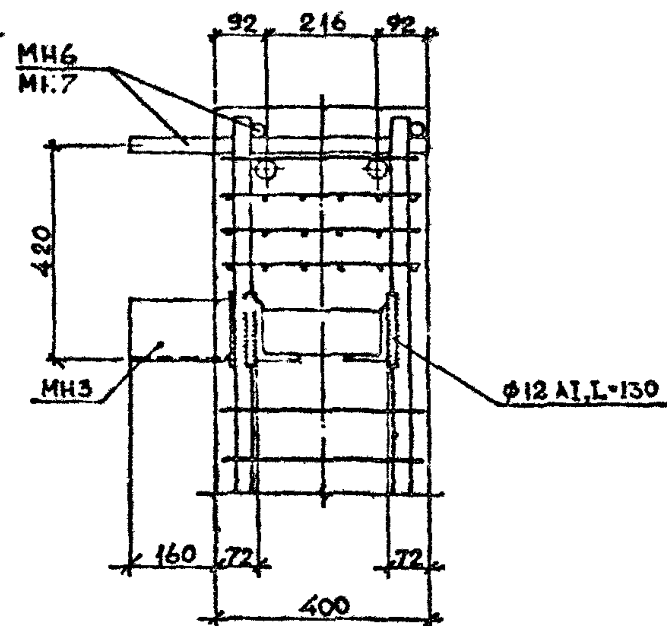
Вид А
