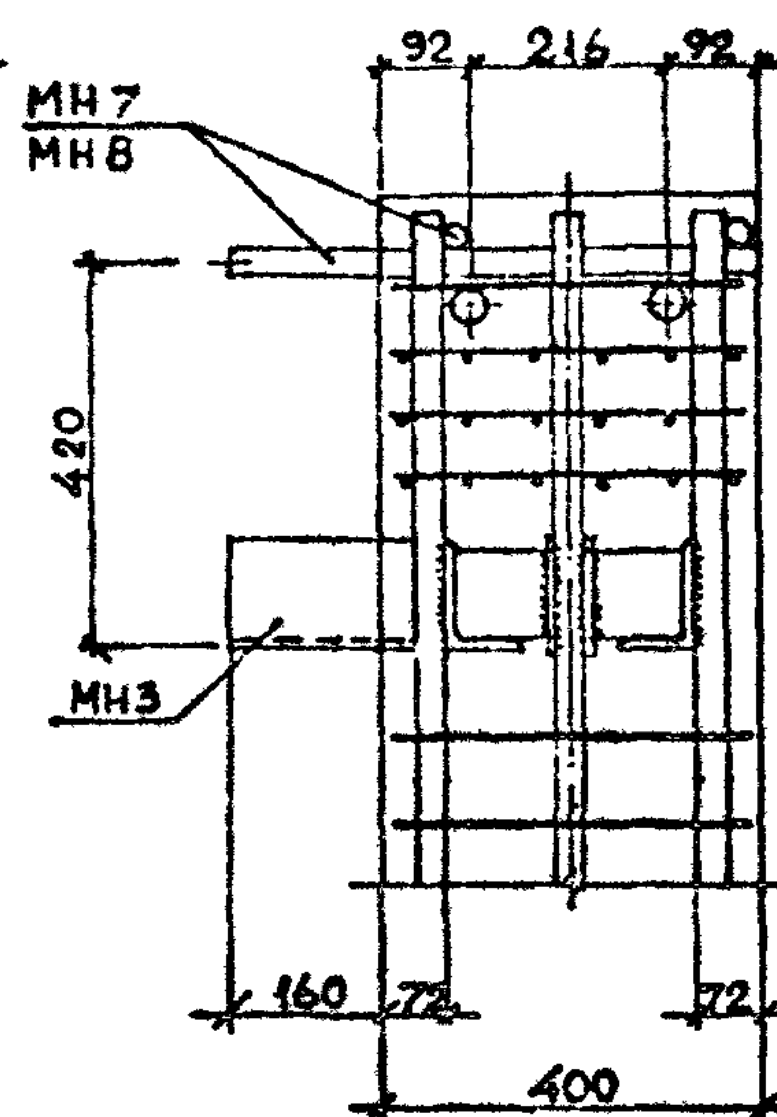
Вид А
