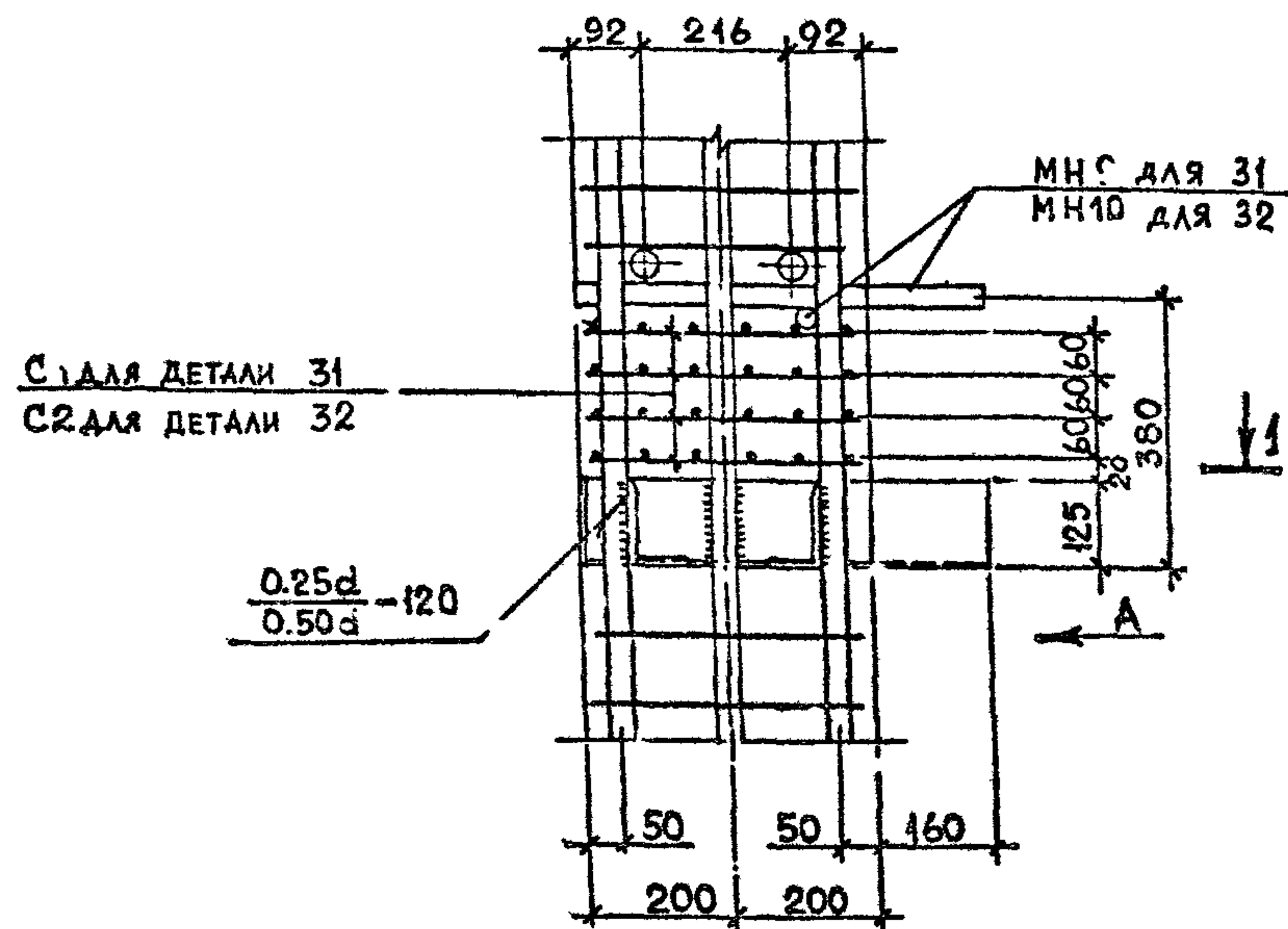
ДЕТАЛЬ 31,32
