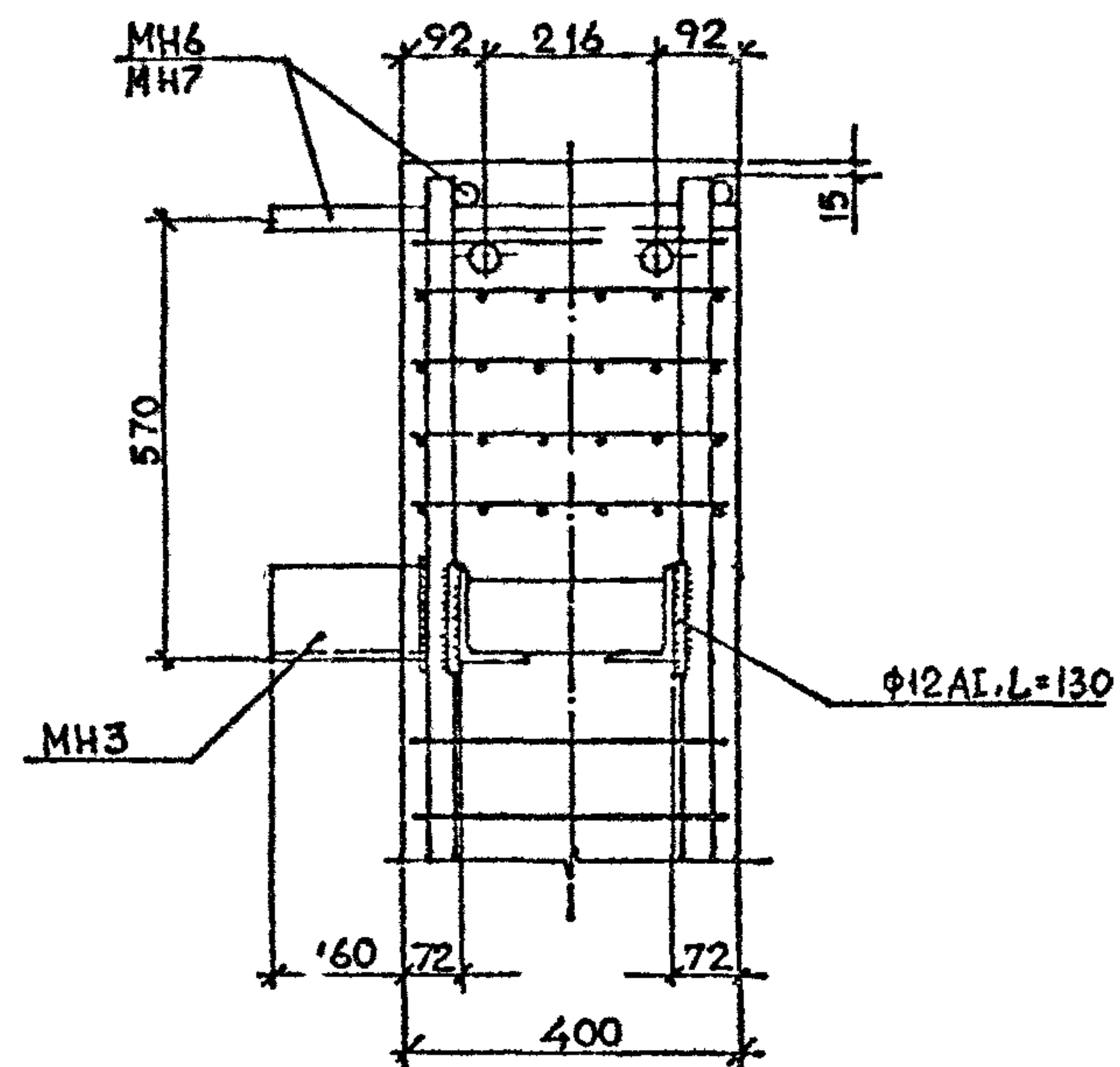
Вид А
