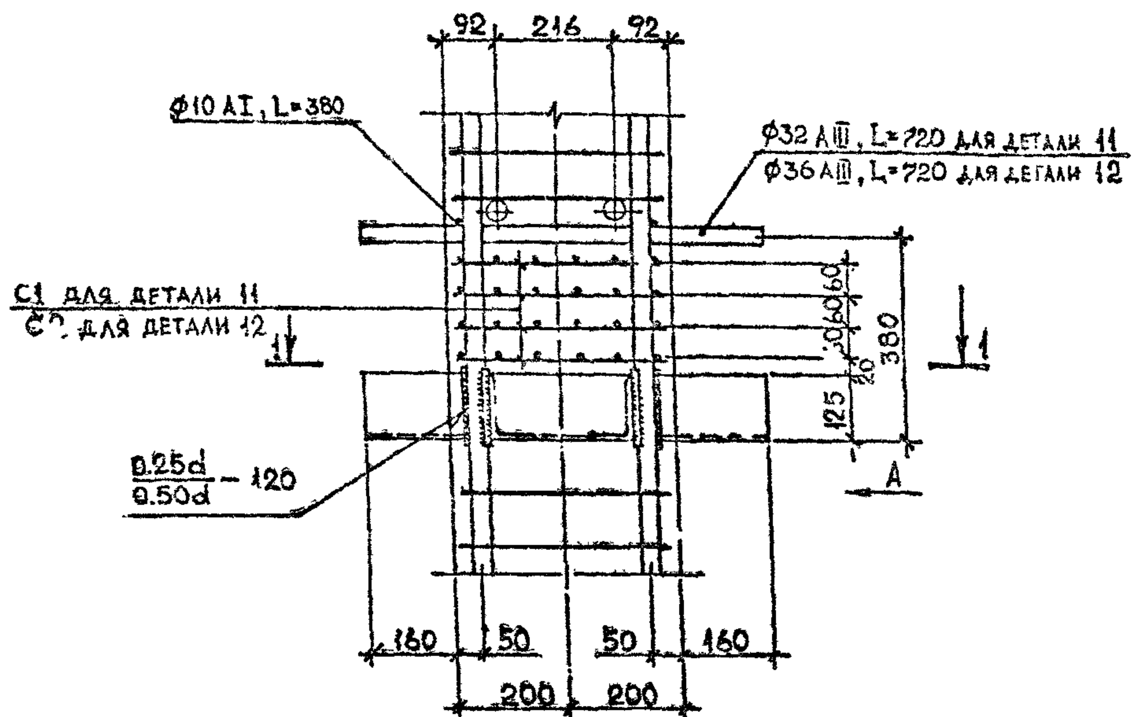
ДЕТАЛЬ 11.12
