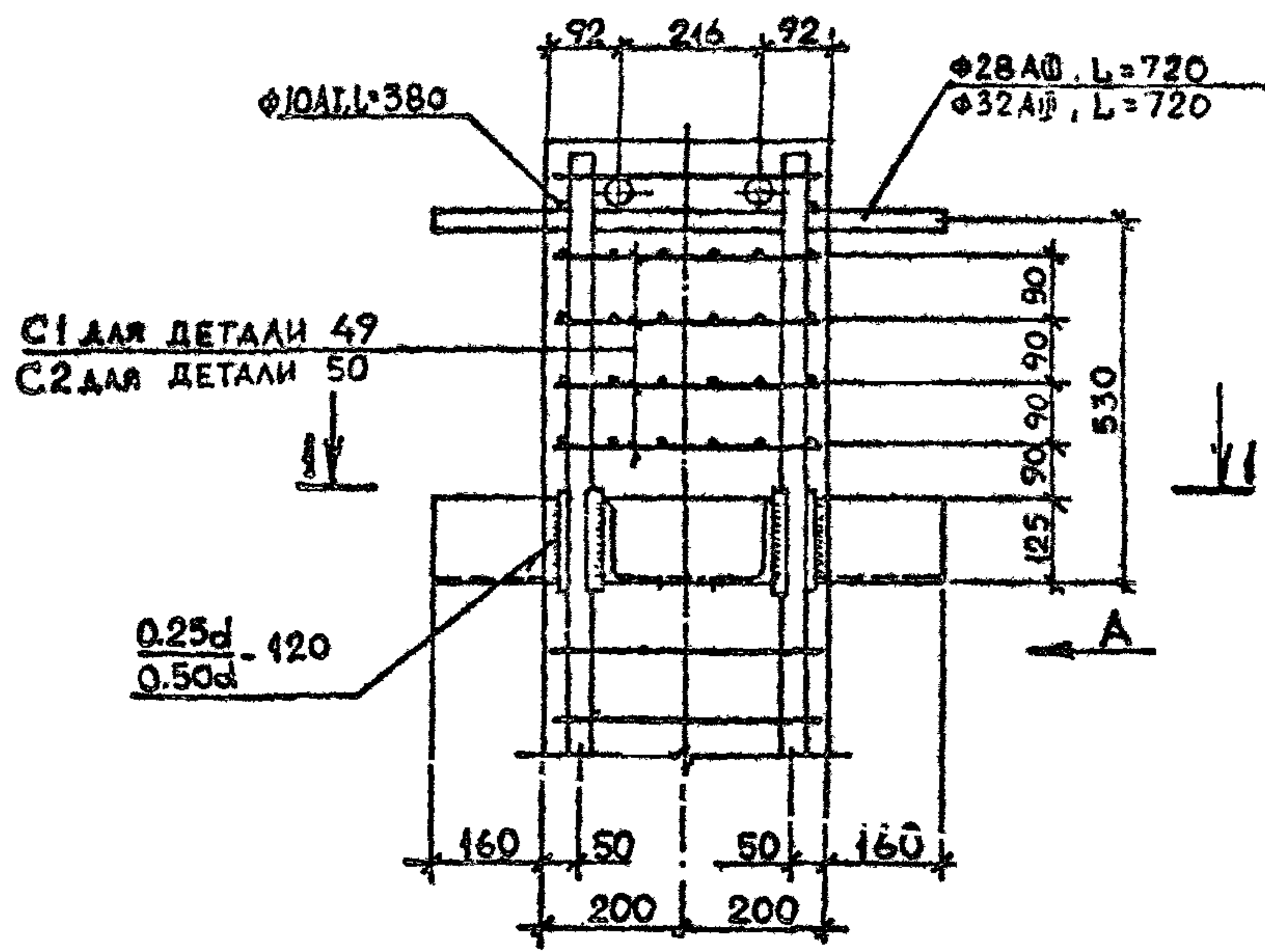
1-1
