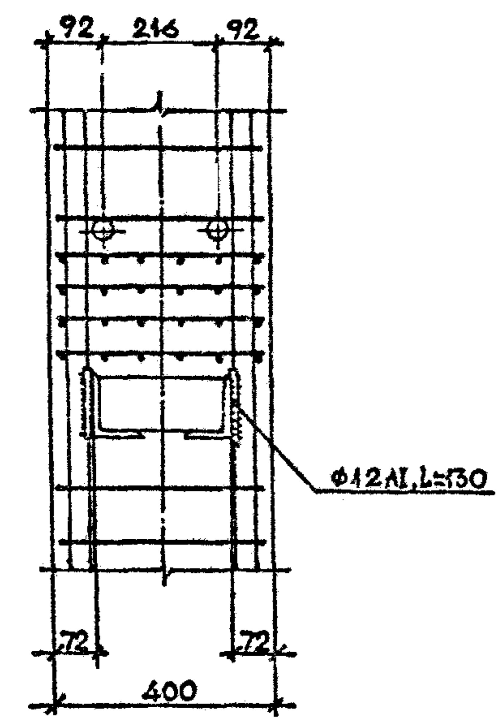
ВИД А
