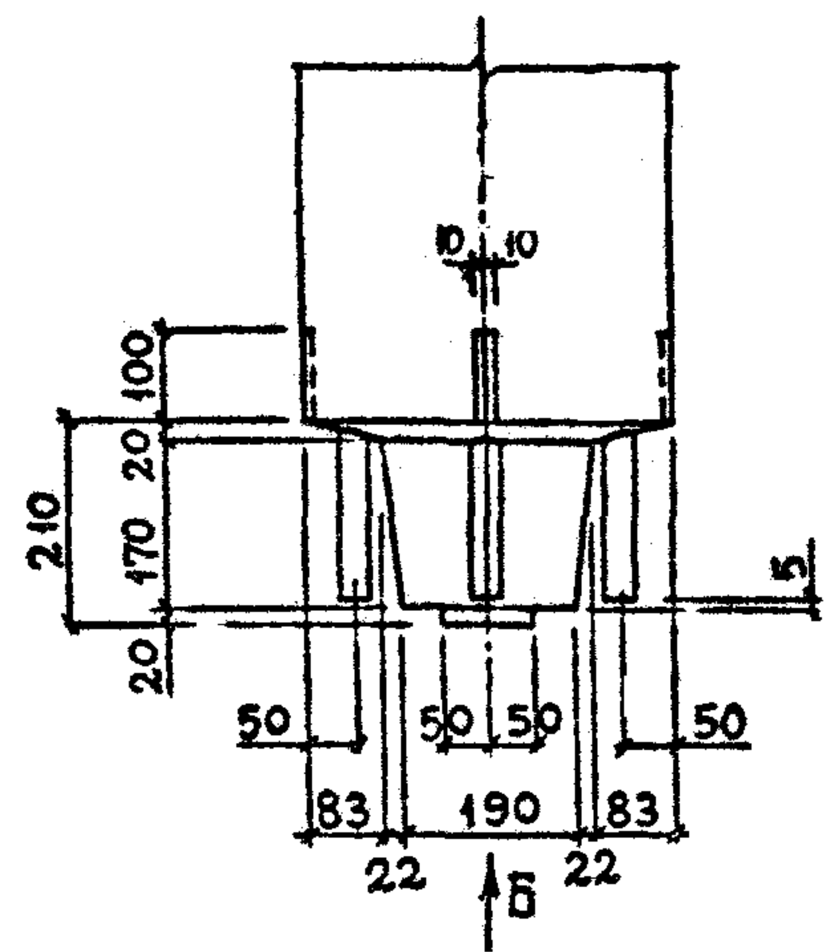
ДЕТАЛЬ 24
