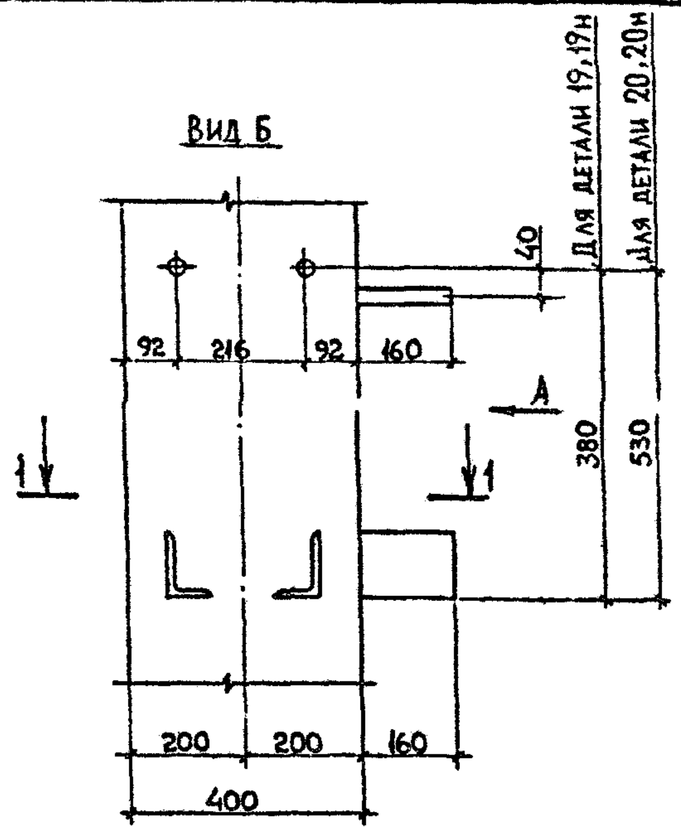
ДЕТАЛЬ 19н, 20н ЗЕРКАЛЬНОЕ ОТРАЖЕНИЕ
