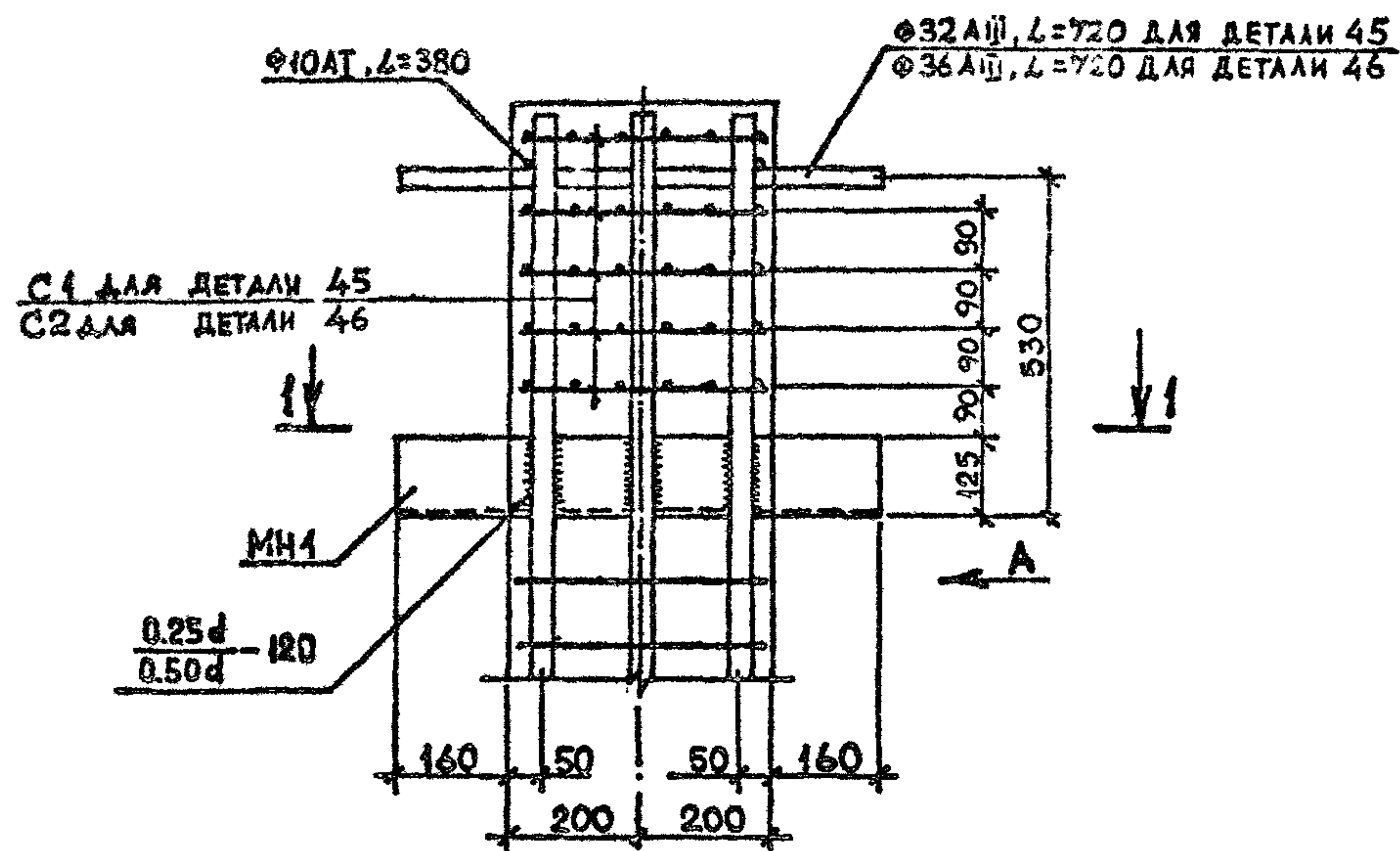
ДЕТАЛЬ 45.46
