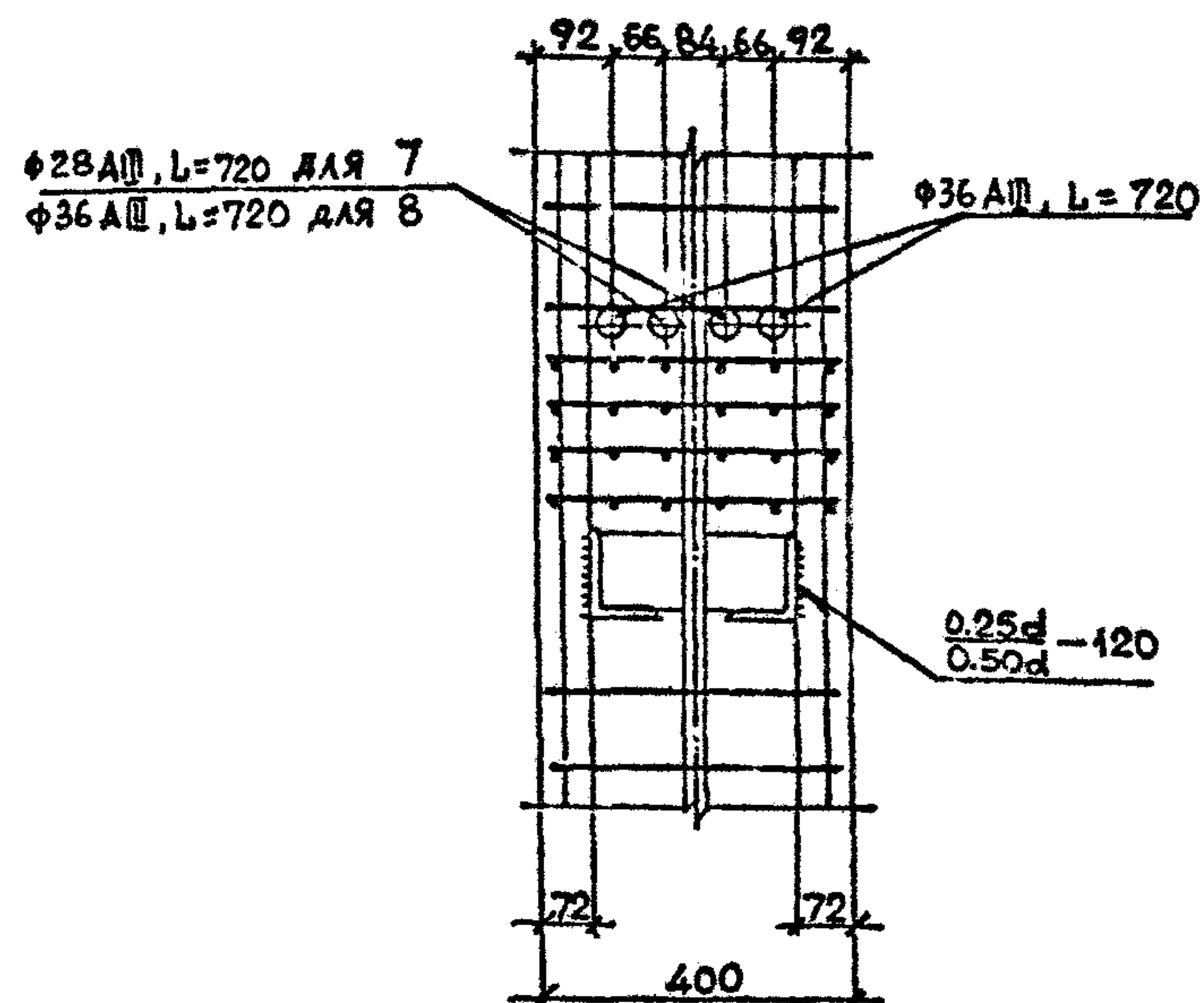
Вид А
