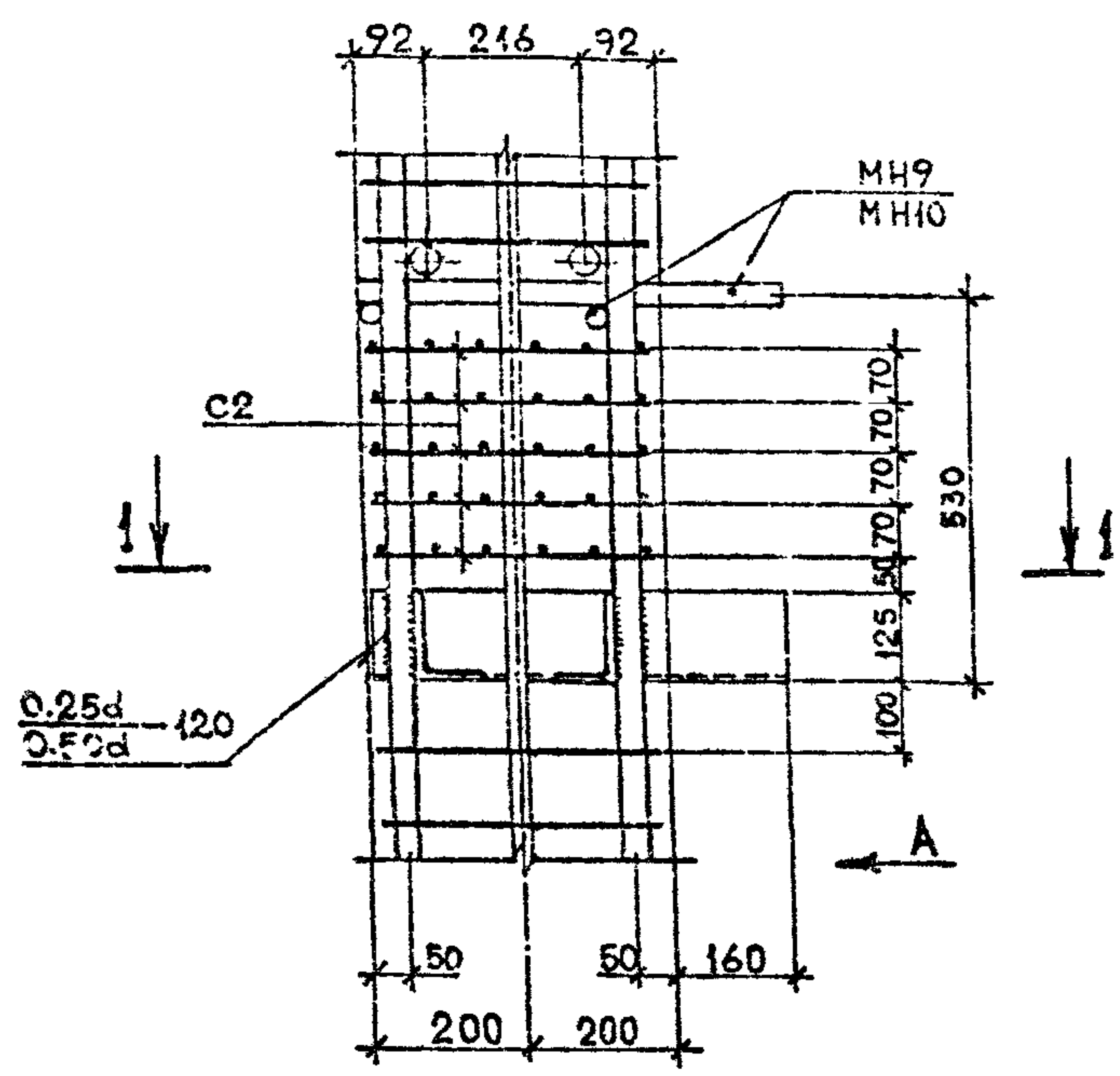
ДЕТАЛЬ 71, 72
