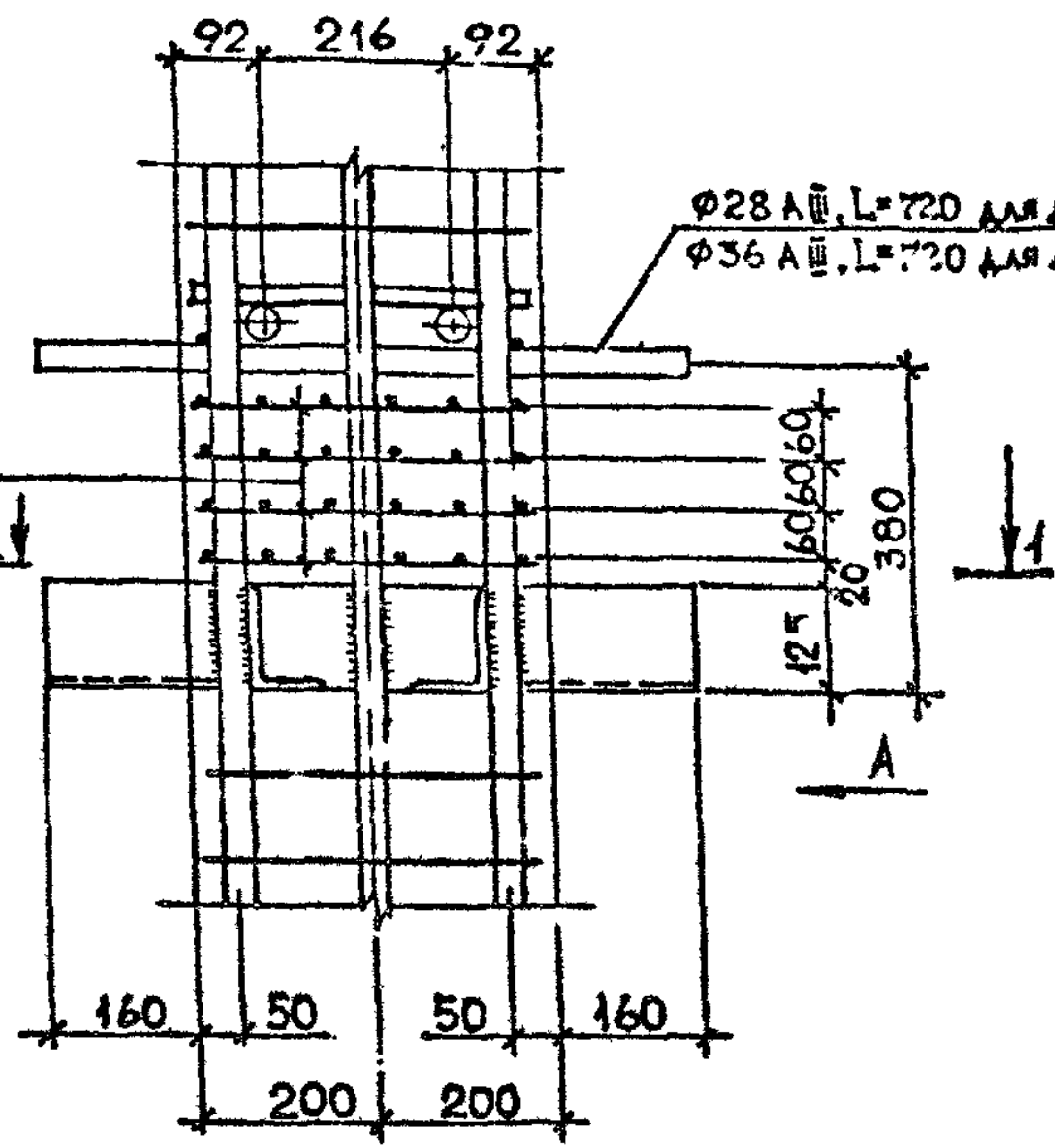
ДЕТАЛЬ 23, 24
