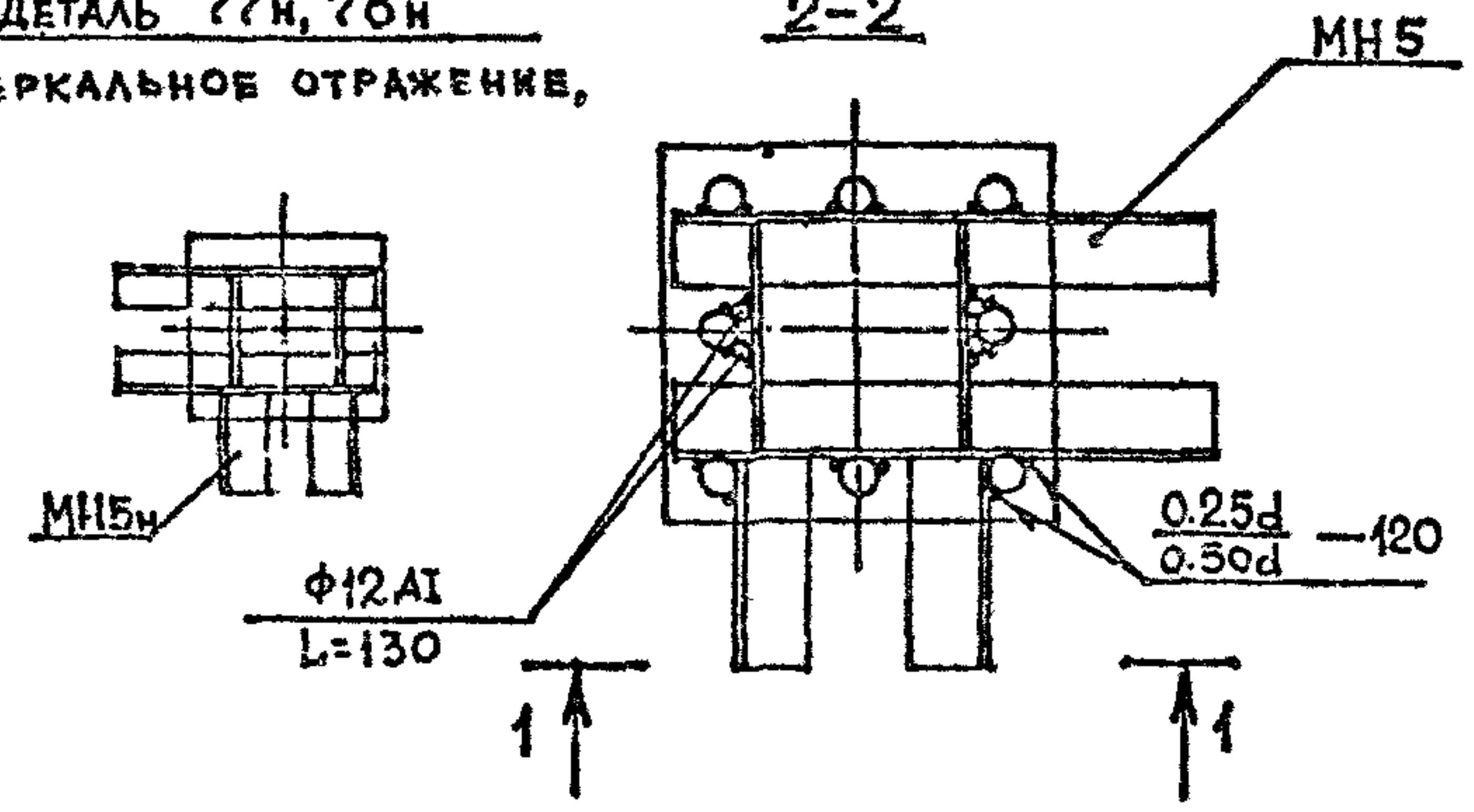
Деталь 77, 78
