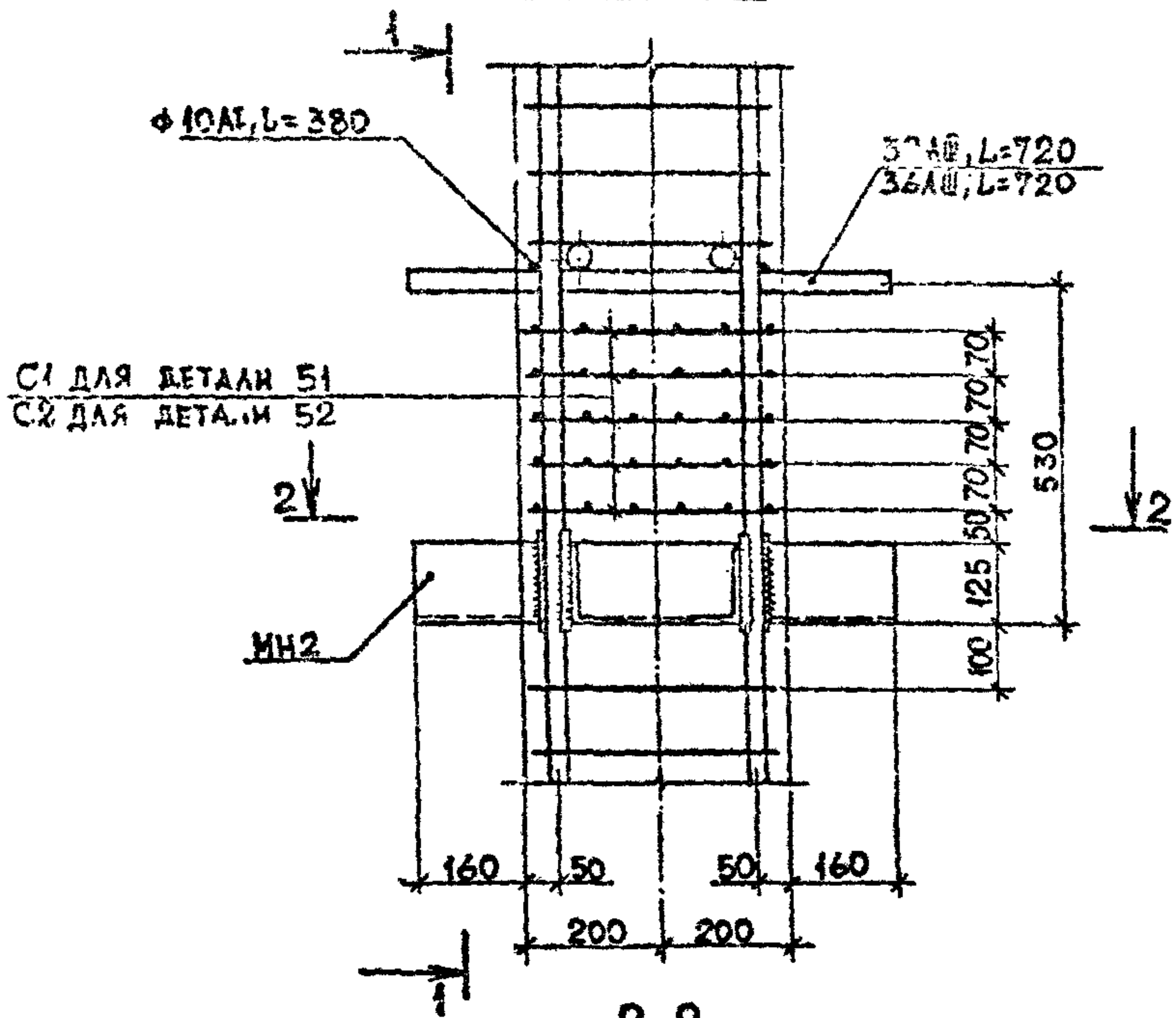
ДЕТАЛЬ 51, 52
