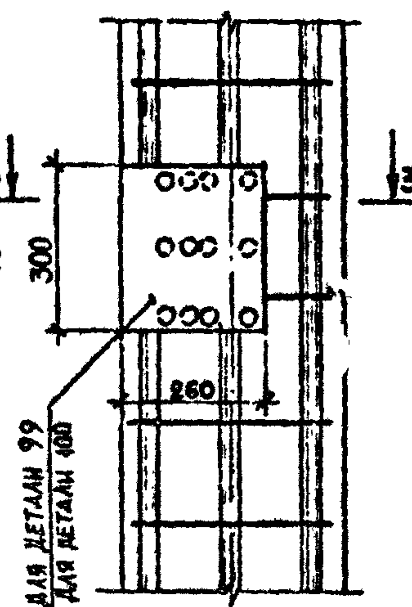
ДЕТАЛЬ 99, 100
