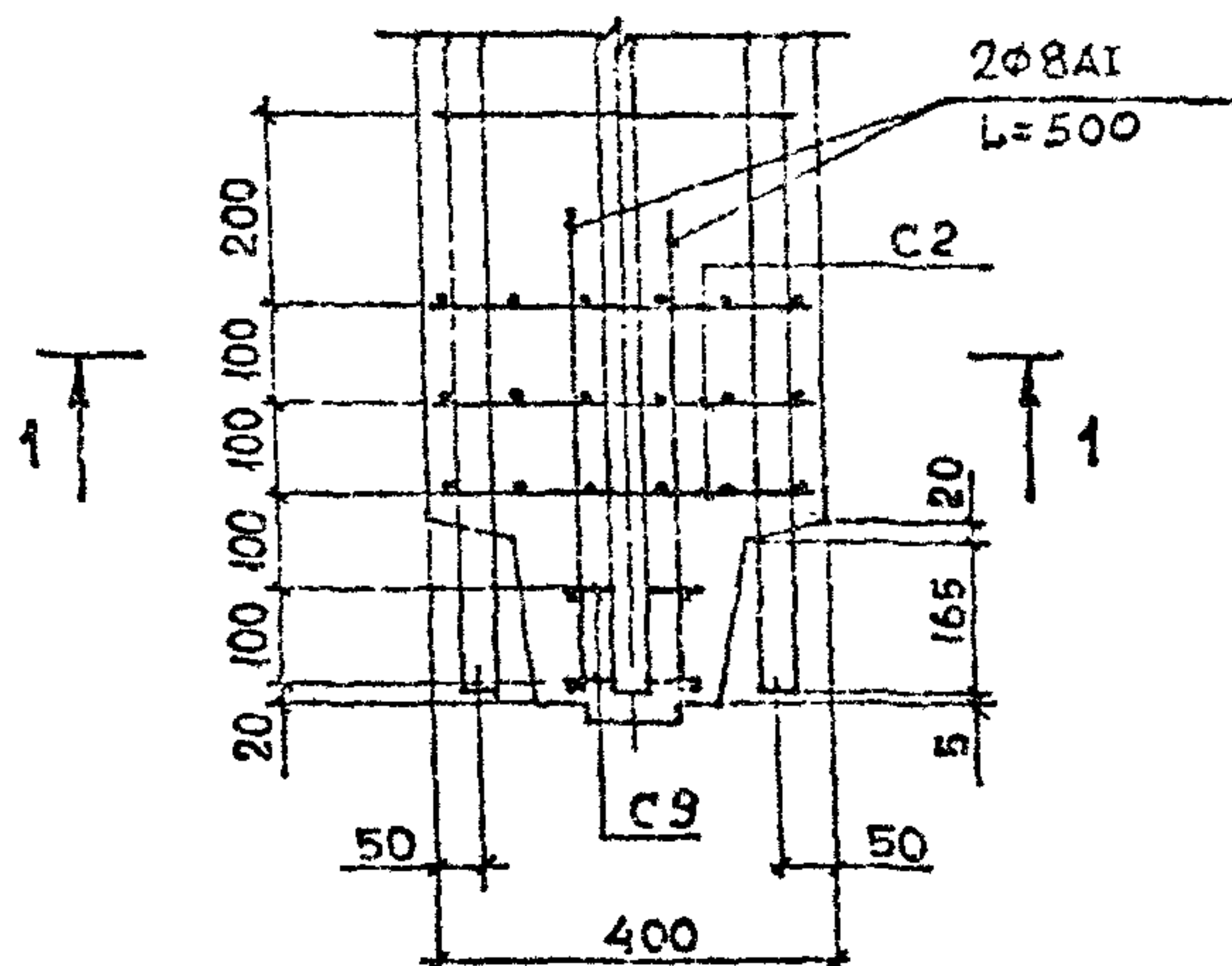
ДЕТАЛЬ 84
