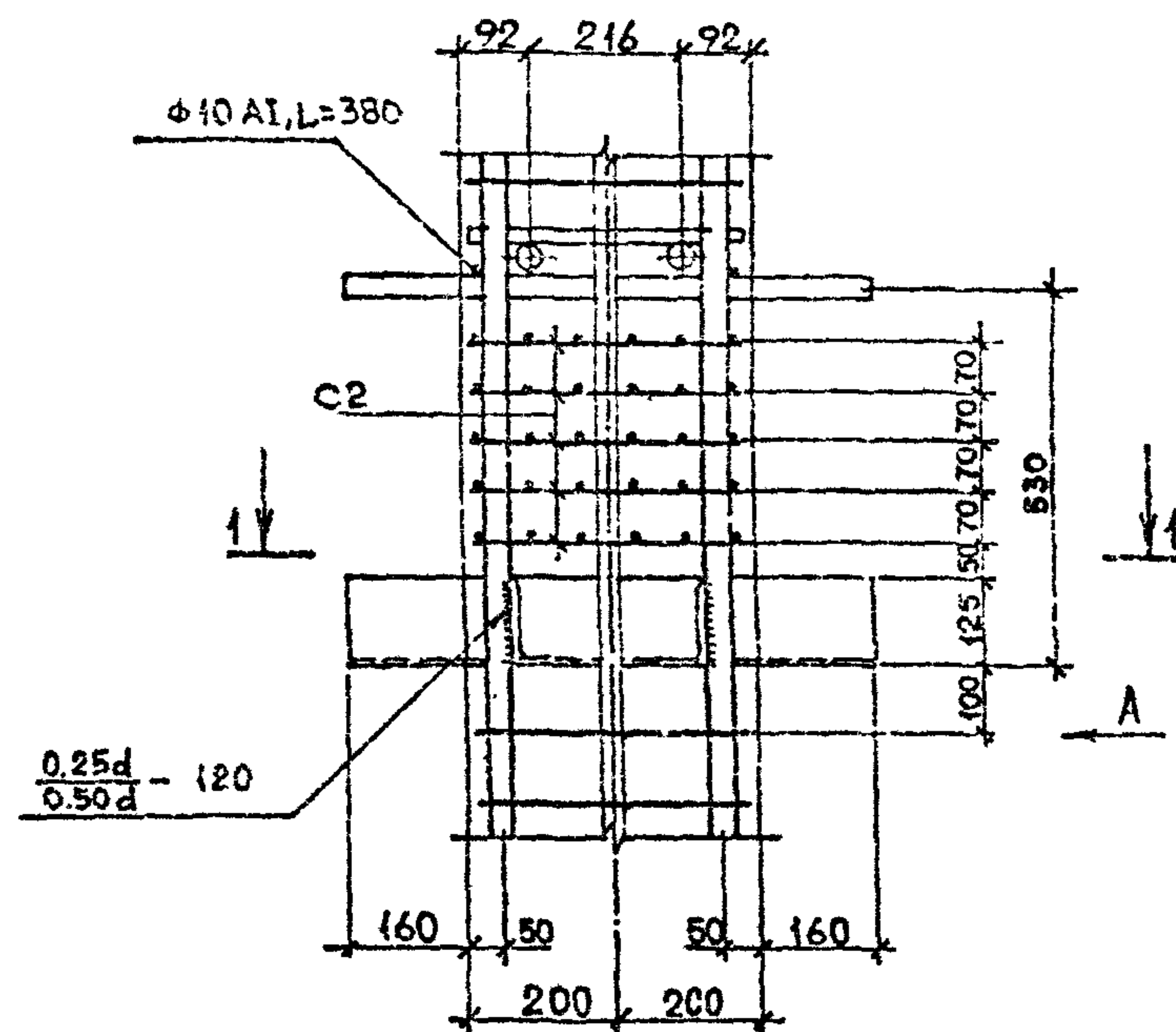
ДЕТАЛЬ 63,64
