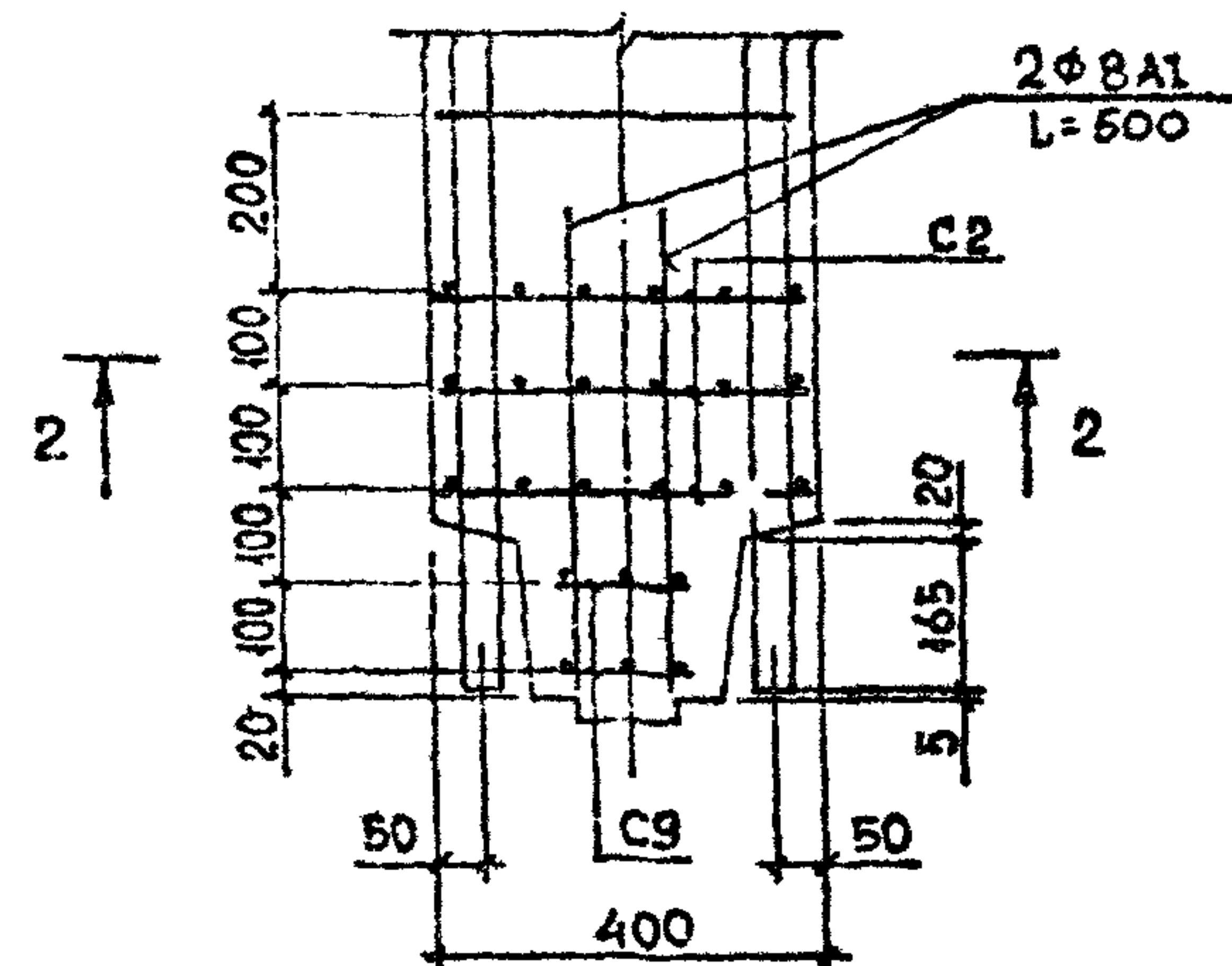
ДЕТАЛЬ 83
