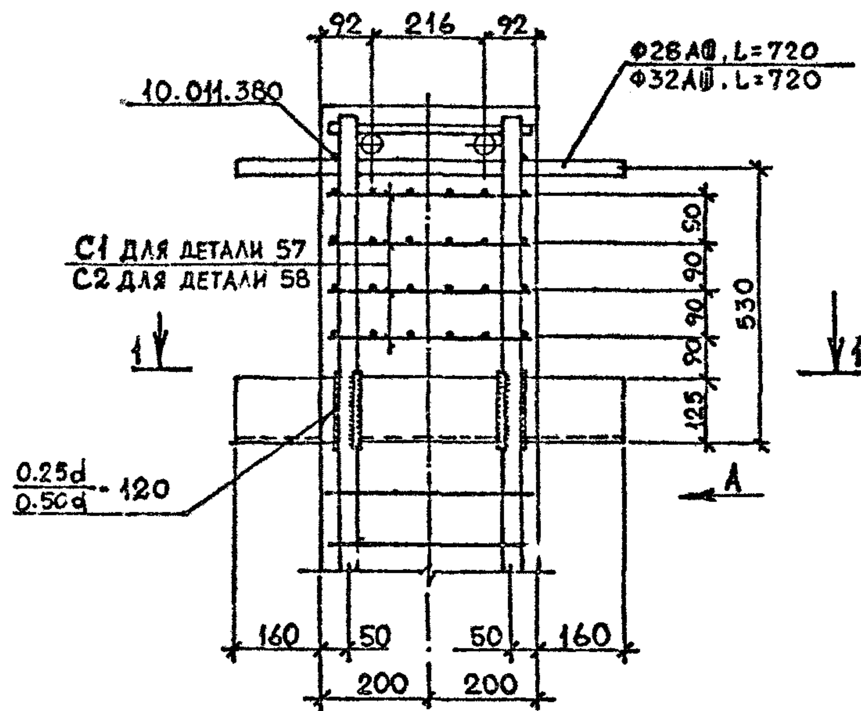
ДЕТАЛЬ 57.58
