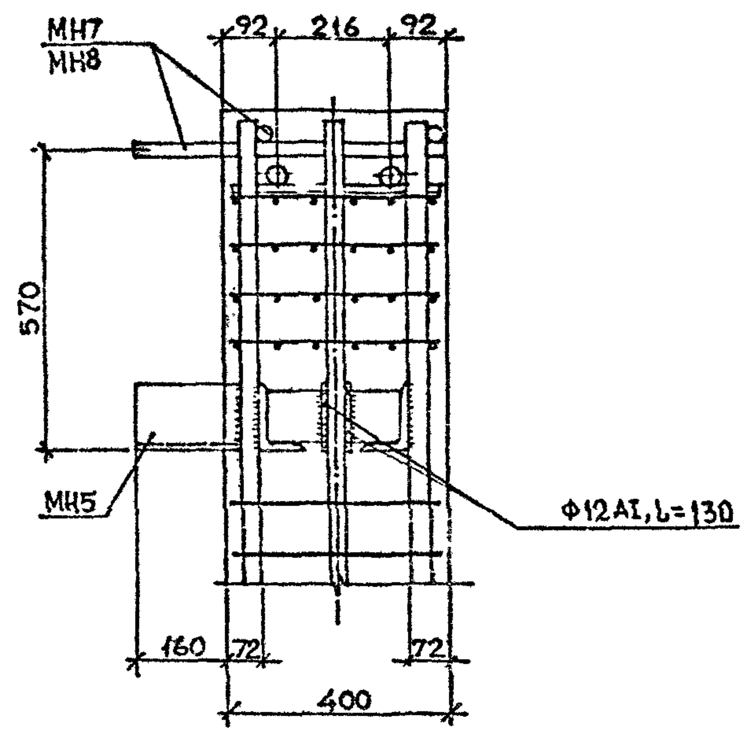
Вид А
