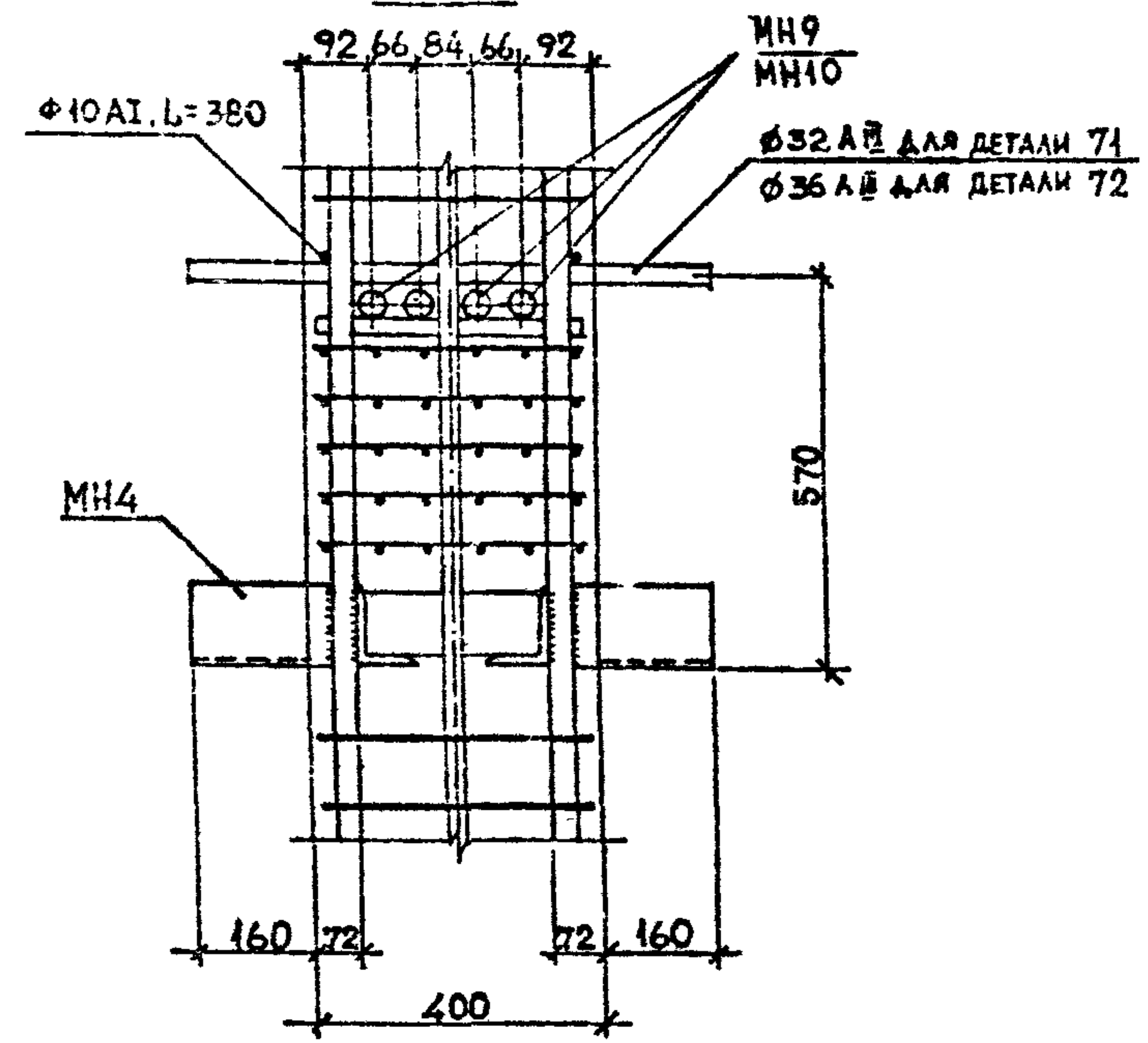
Вид А
