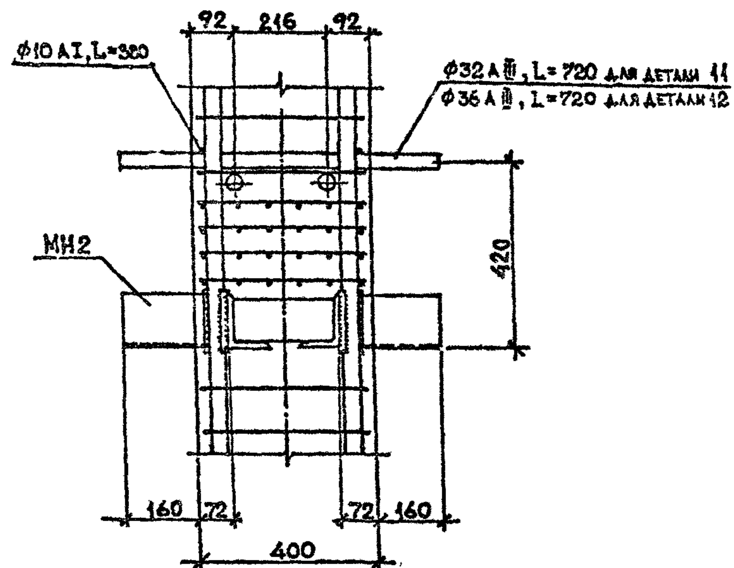
Вид А
