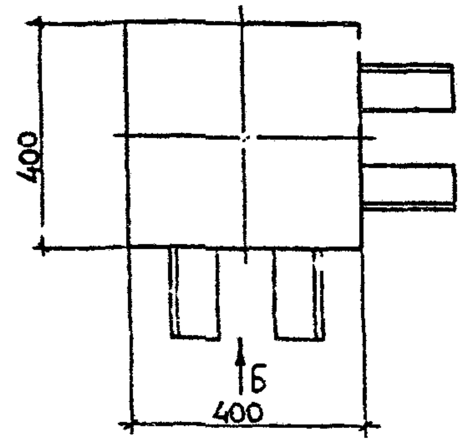
ДЕТАЛЬ 19, 20
