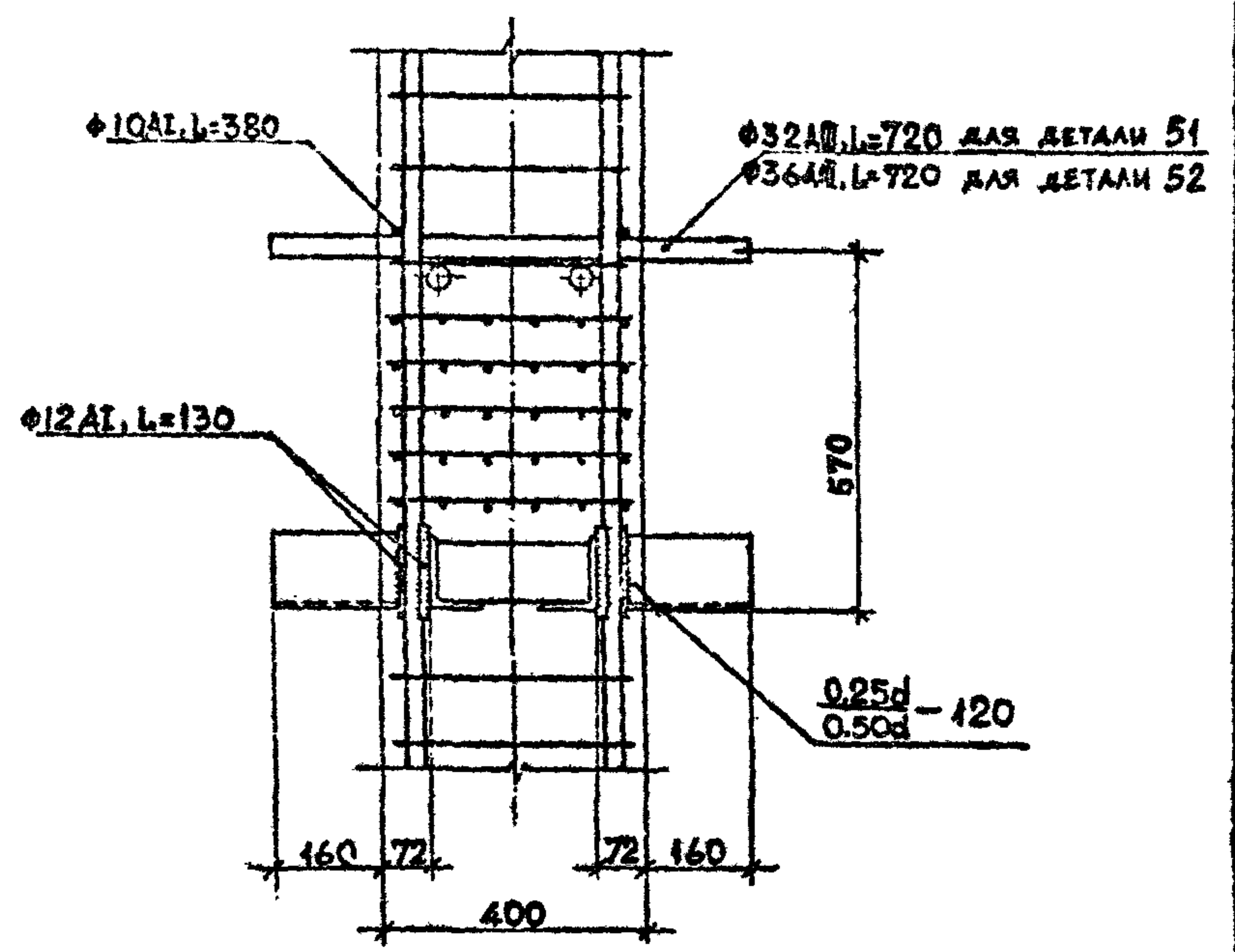
1-1
