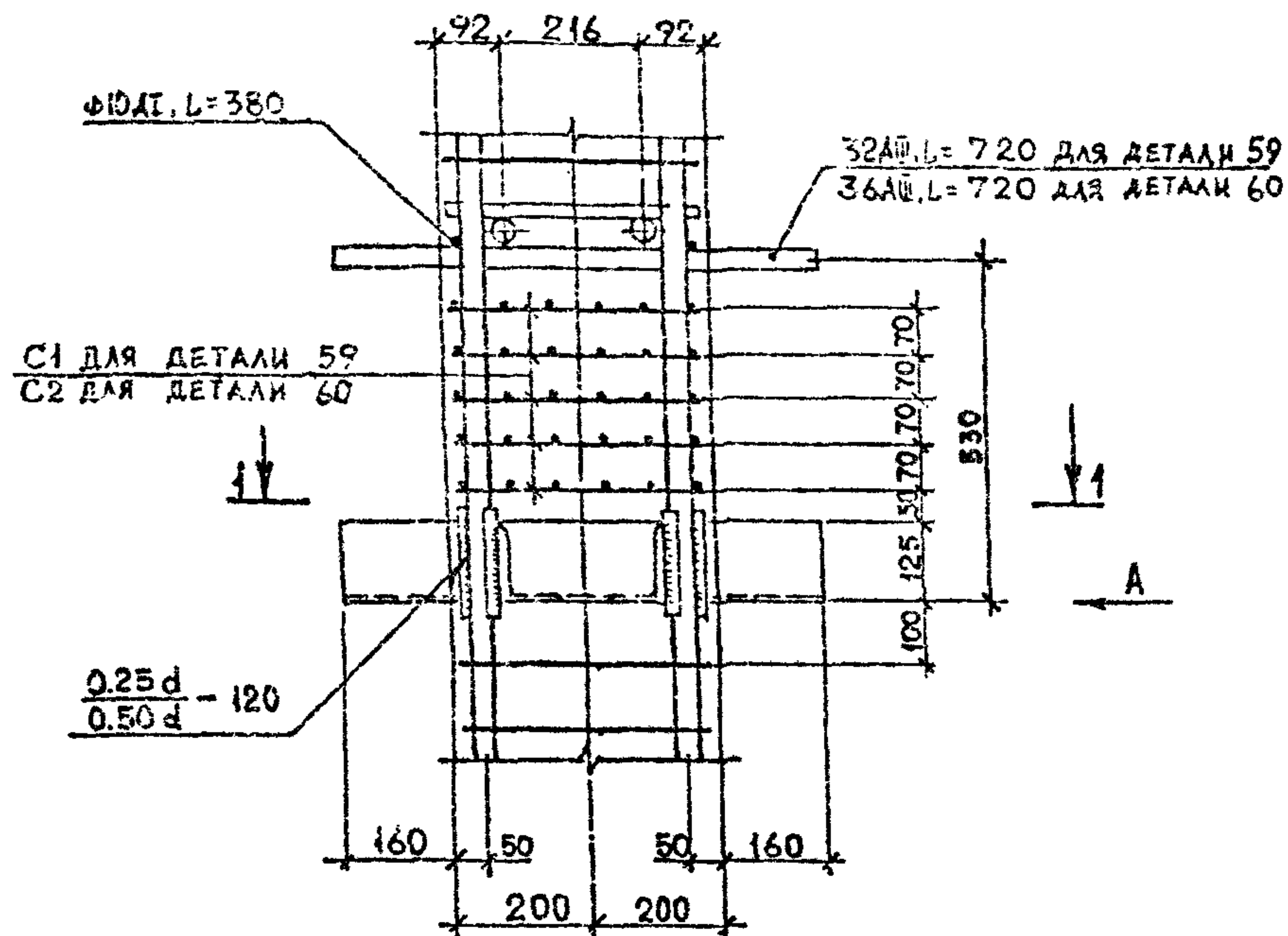
ДЕТАЛЬ 59,60
