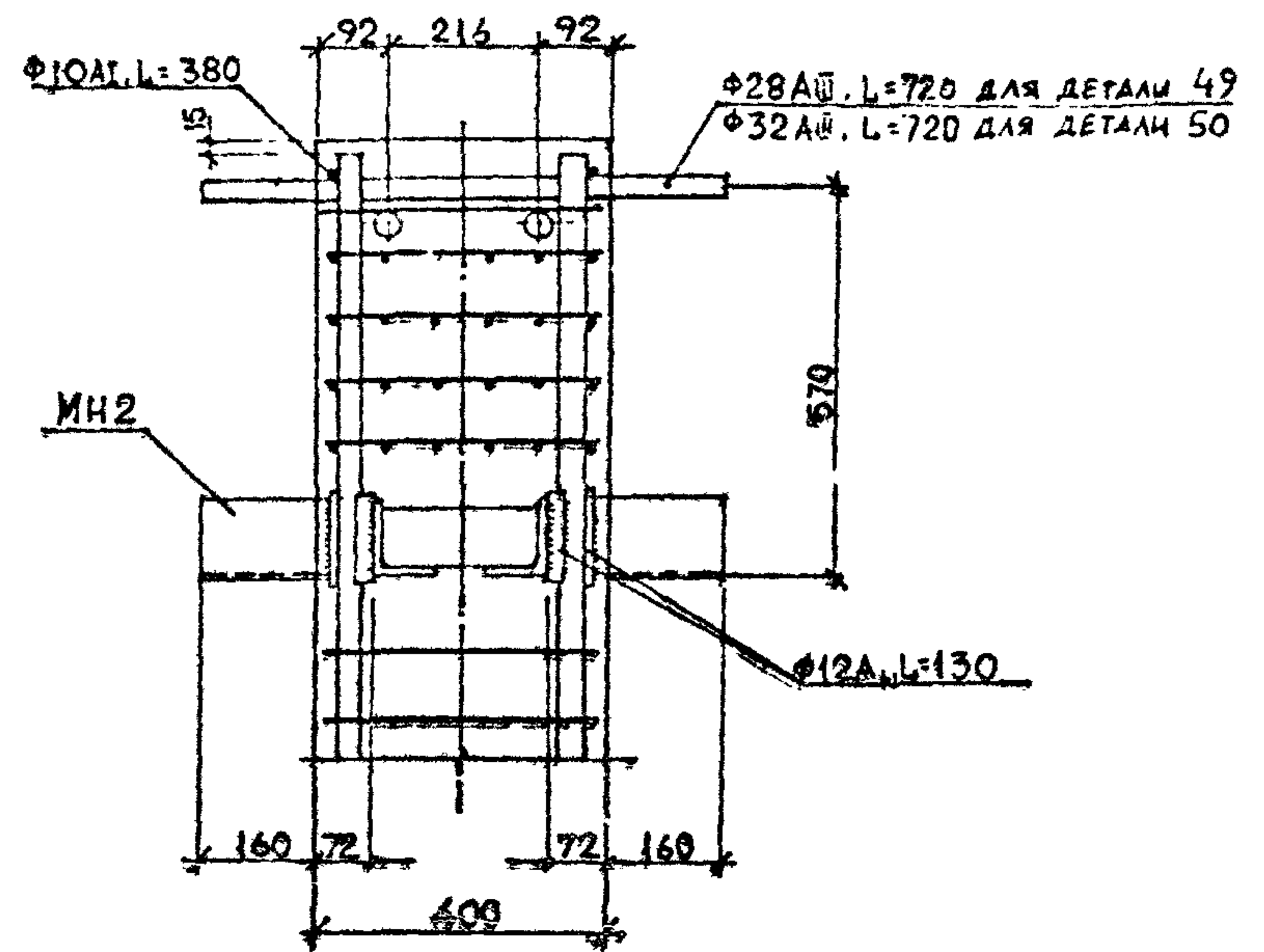
Вид А
