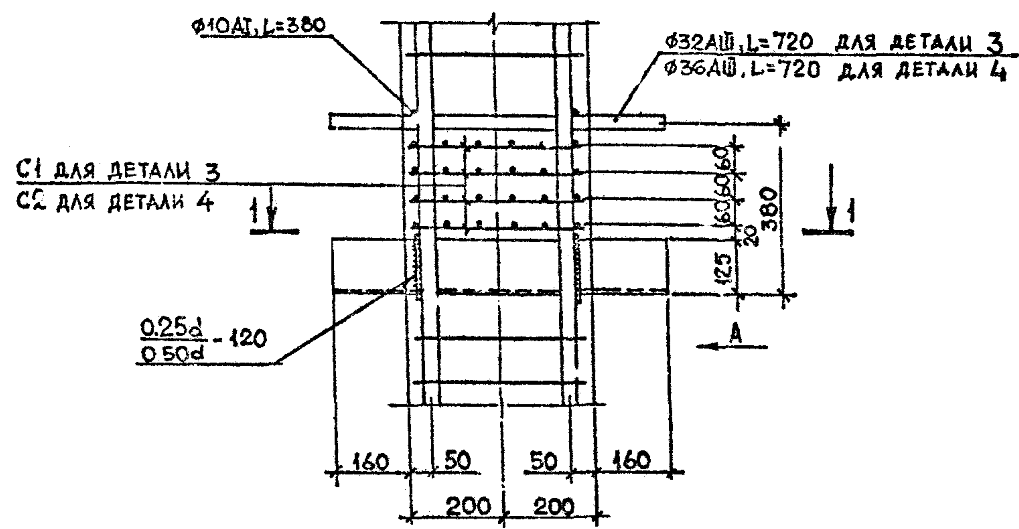
ДЕТАЛЬ 3, 4
