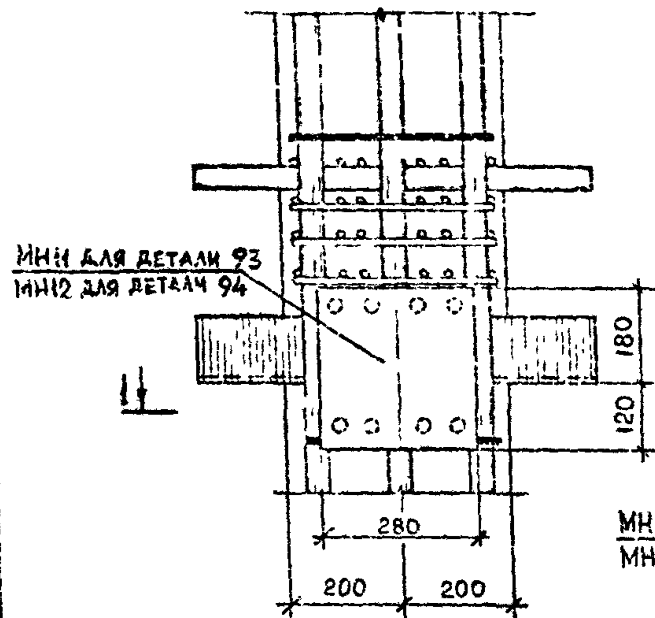
ДЕТАЛЬ 93, 94
