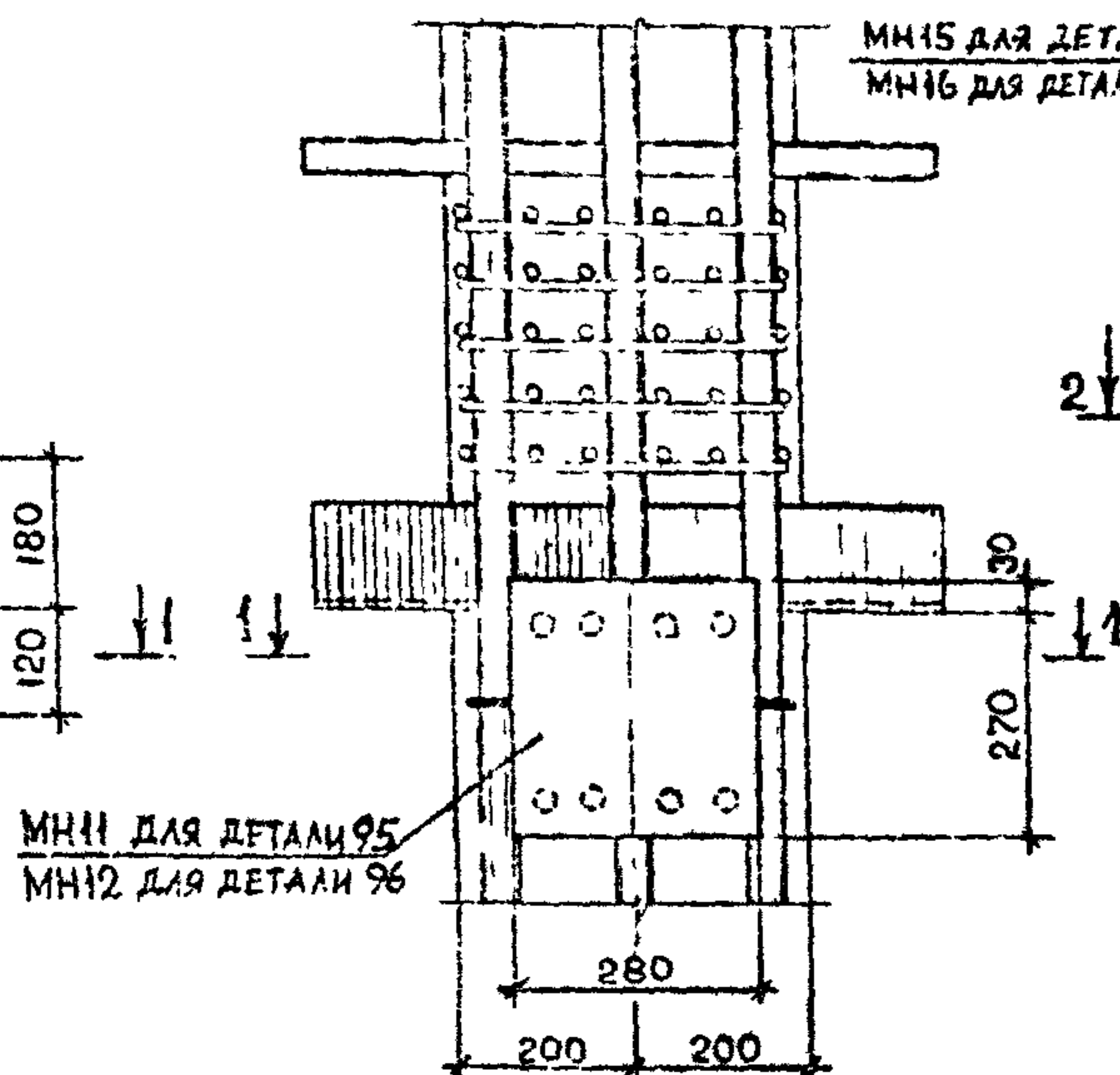
ДЕТАЛЬ 95, 96
