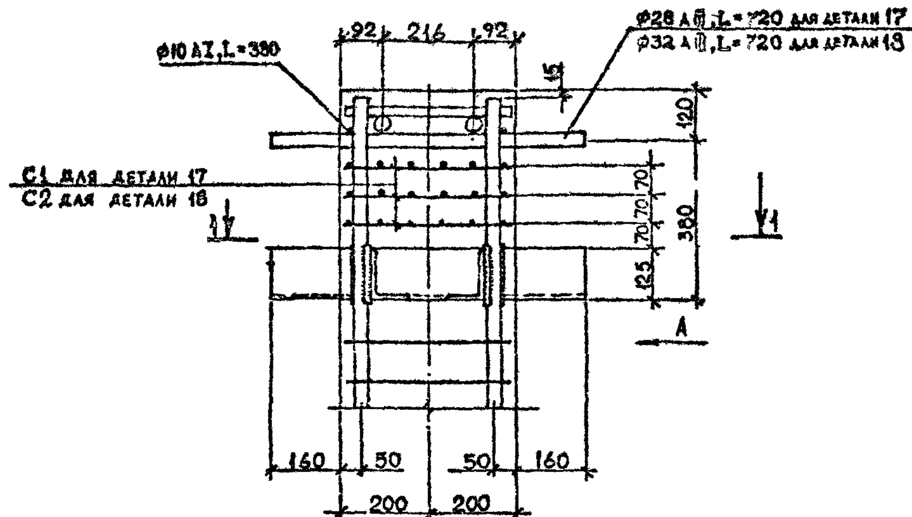
ДЕТАЛЬ 17, 18
