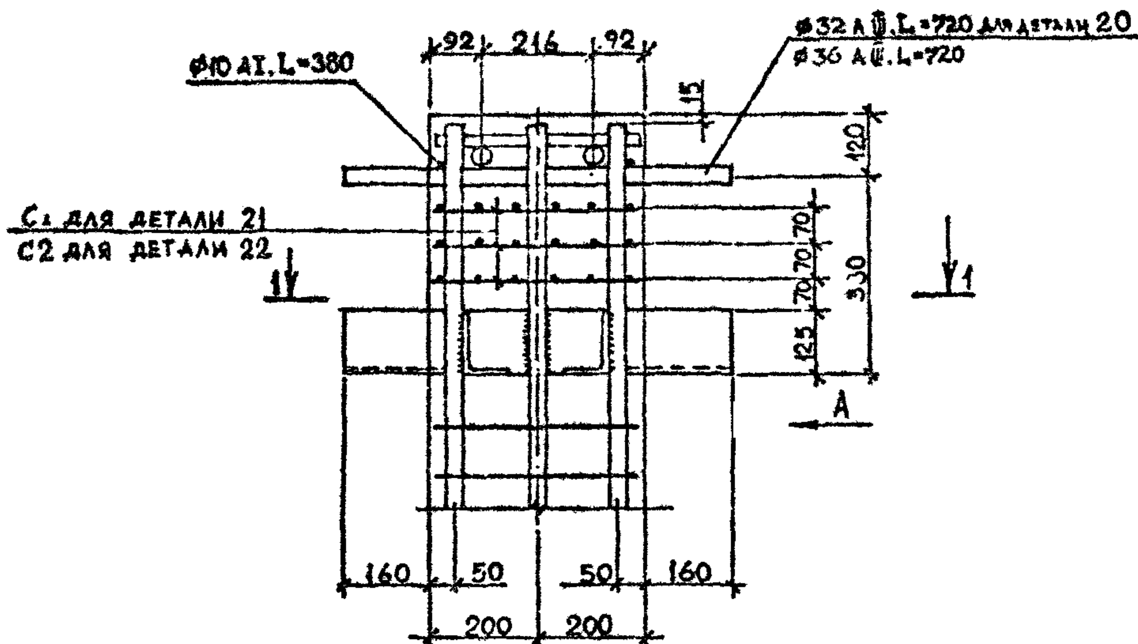
ДЕТАЛЬ 21, 22
