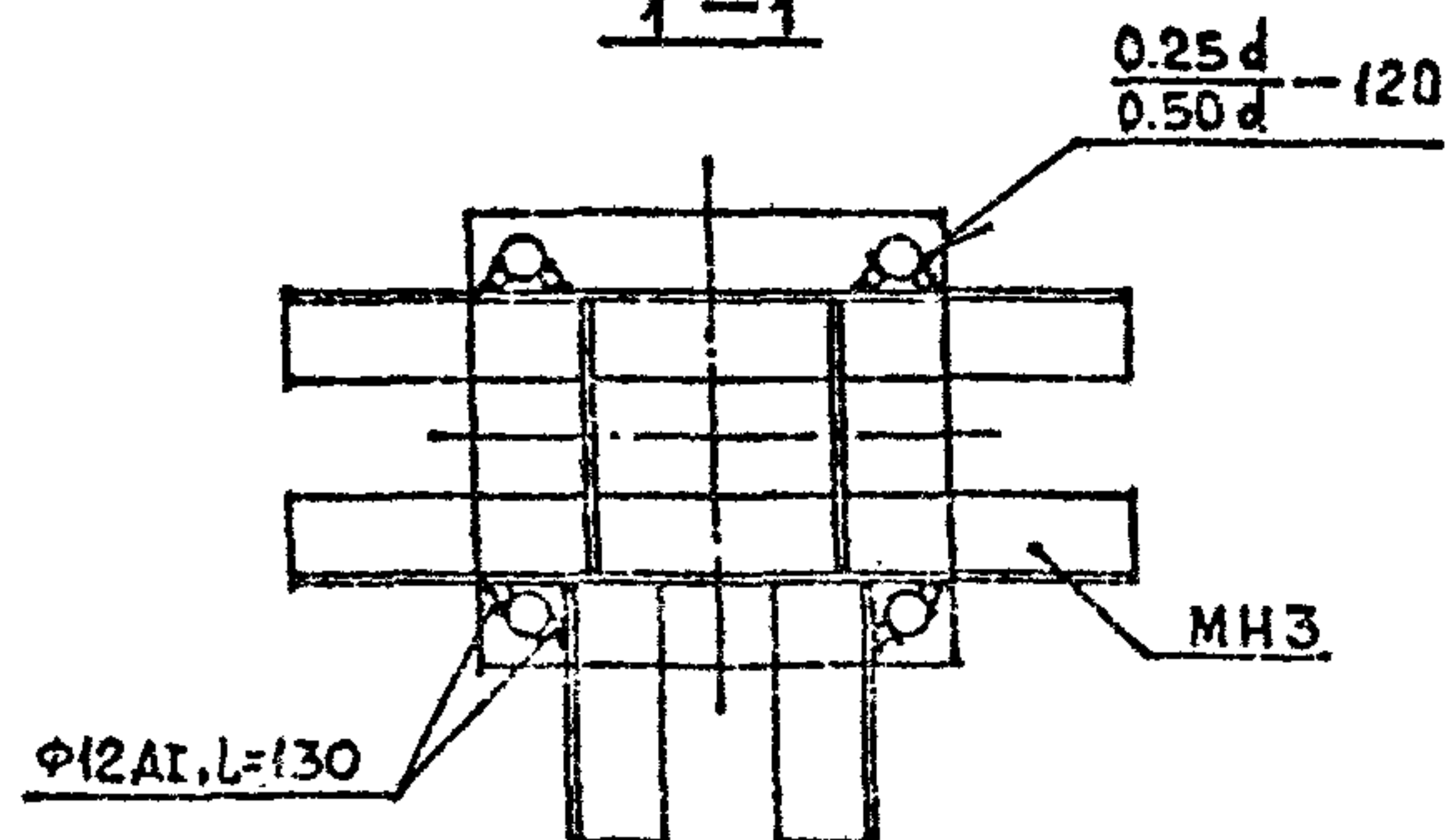
1-1
