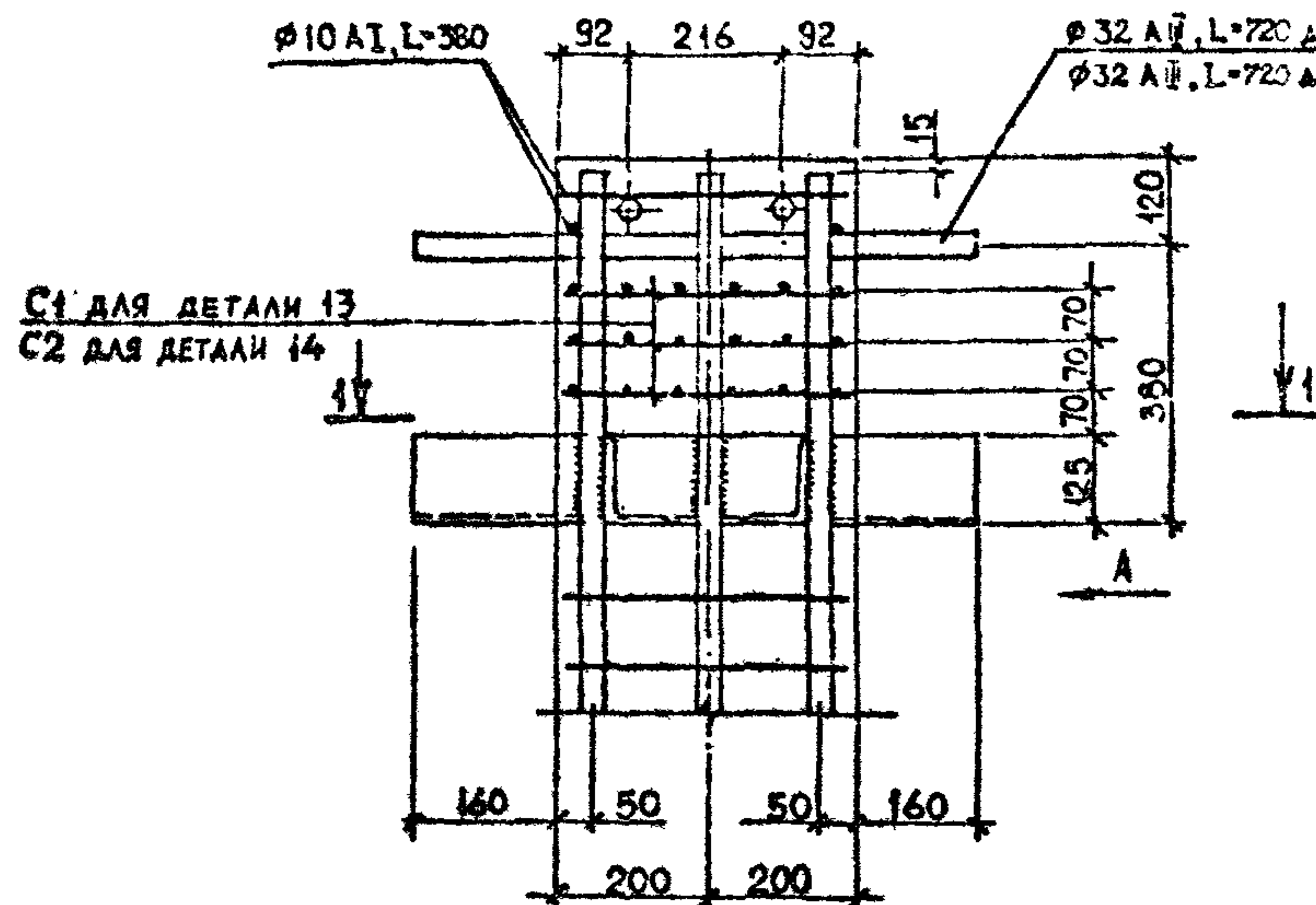
ДЕТАЛЬ 13, 14
