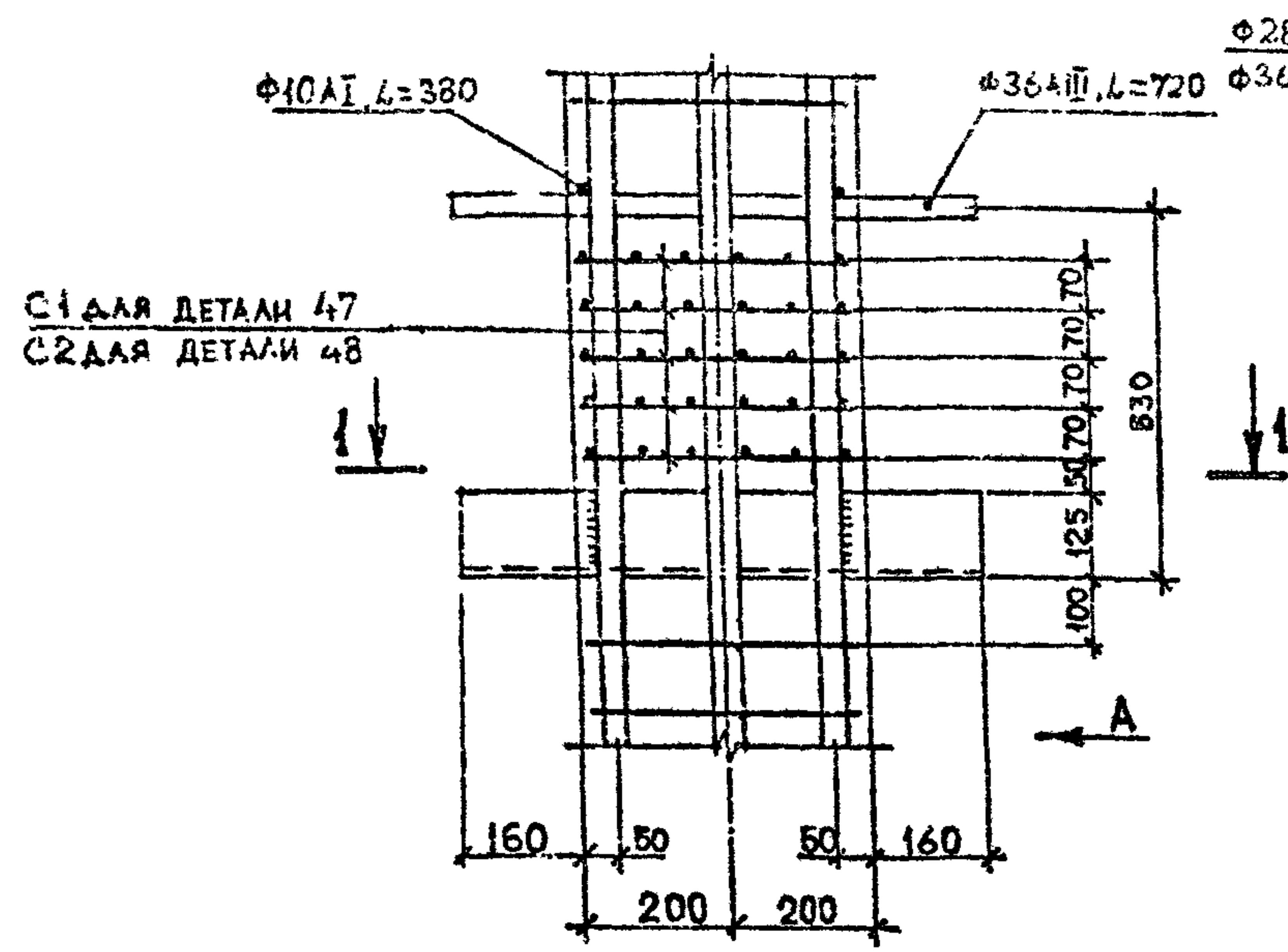
ДЕТАЛЬ 47,48
