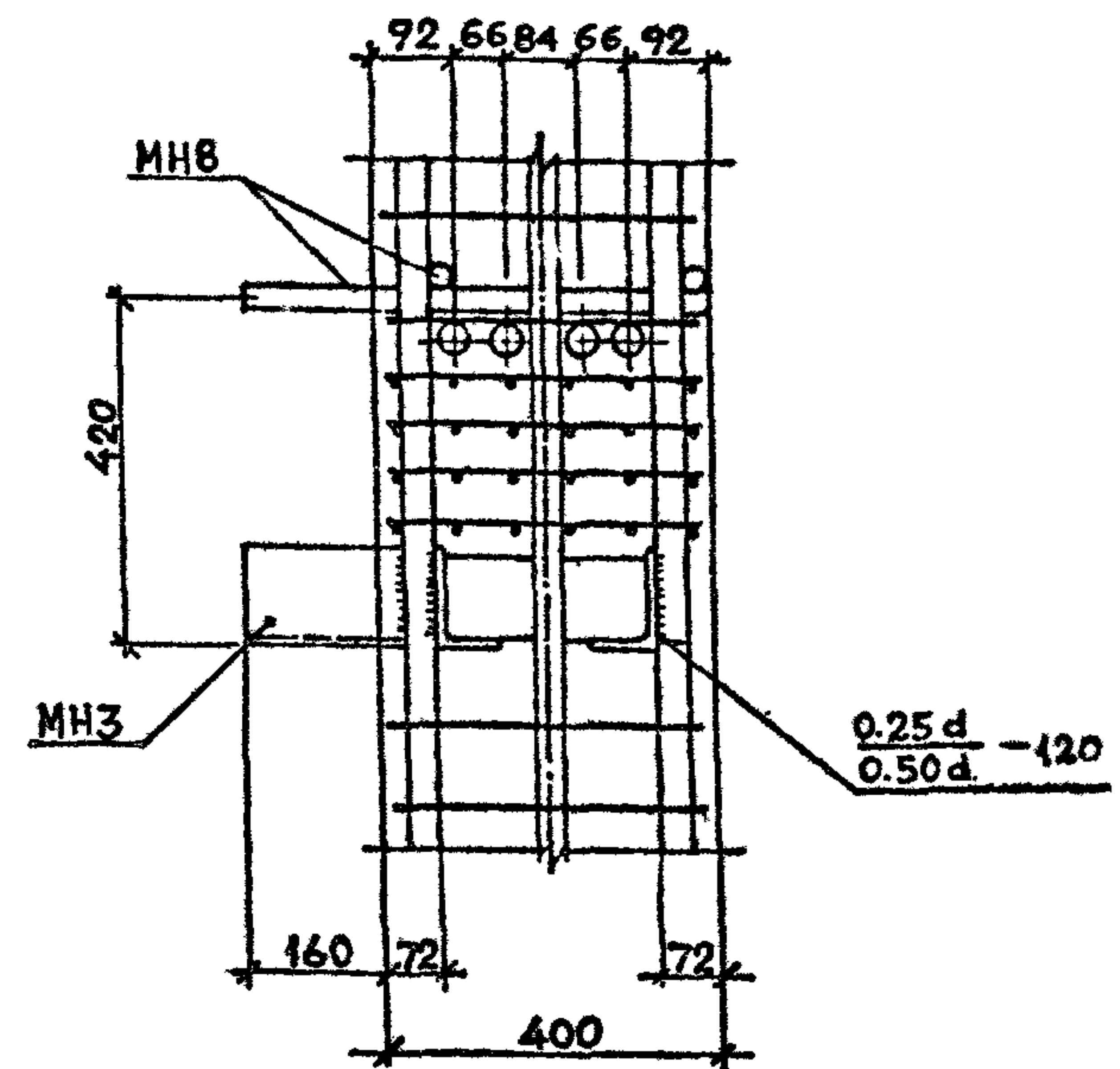
Вид А
