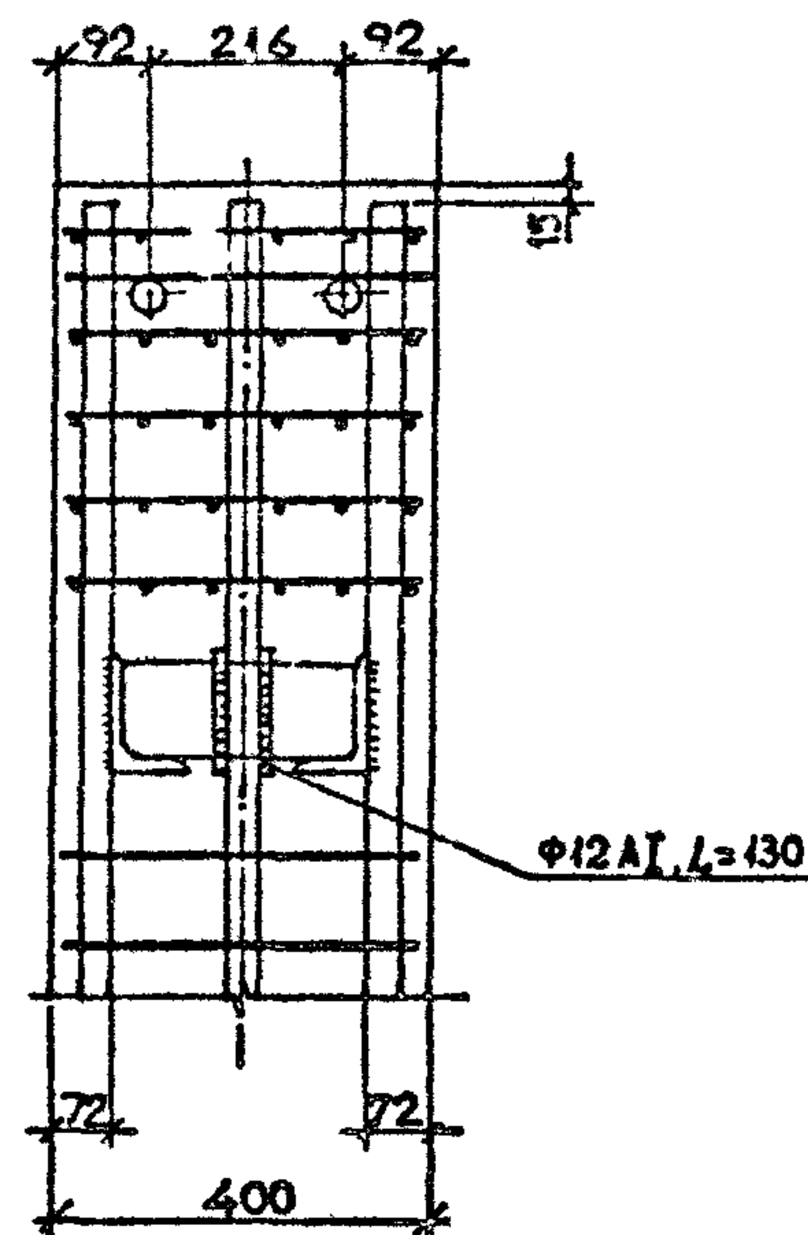
Вид А
