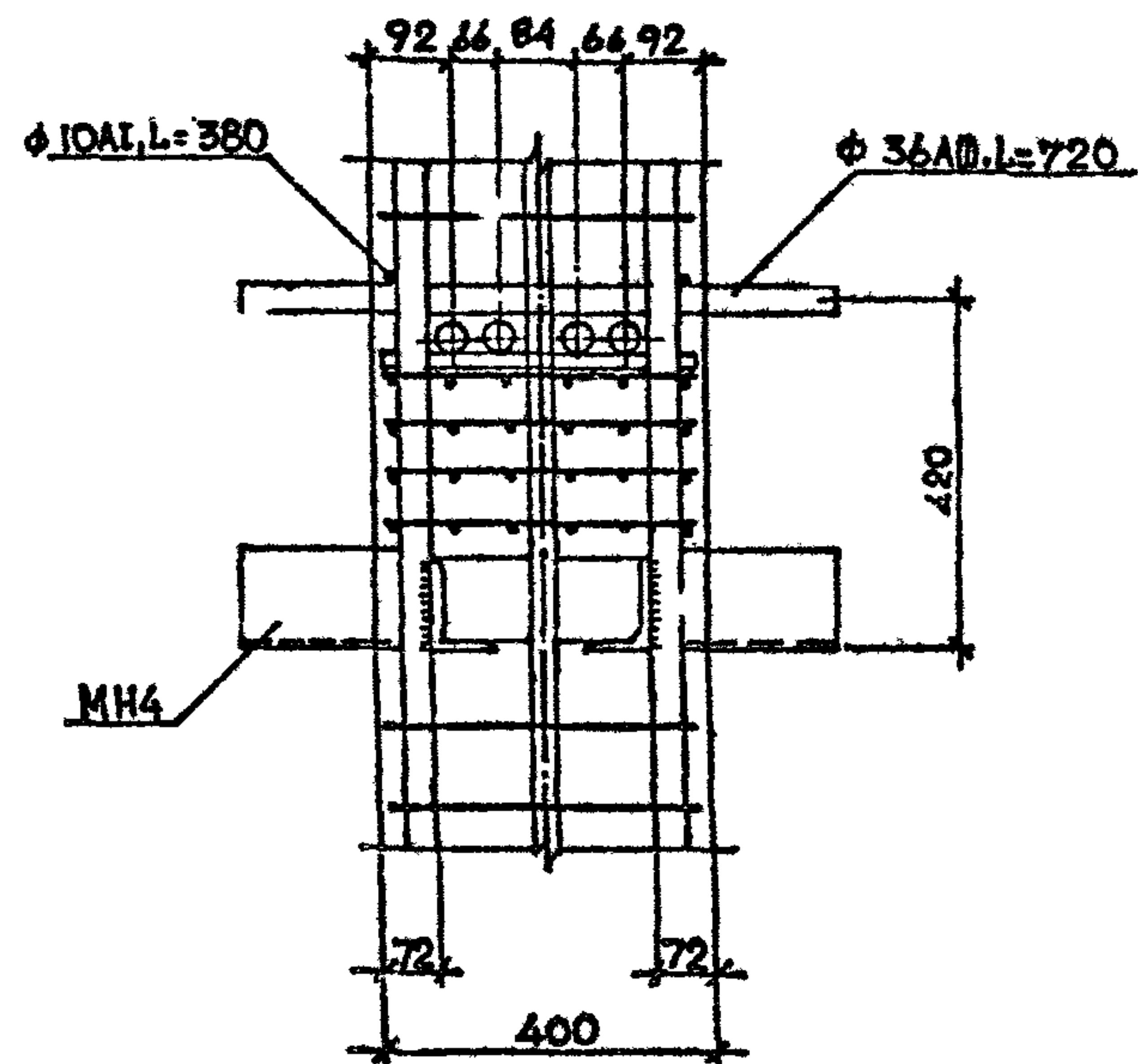
Вид А
