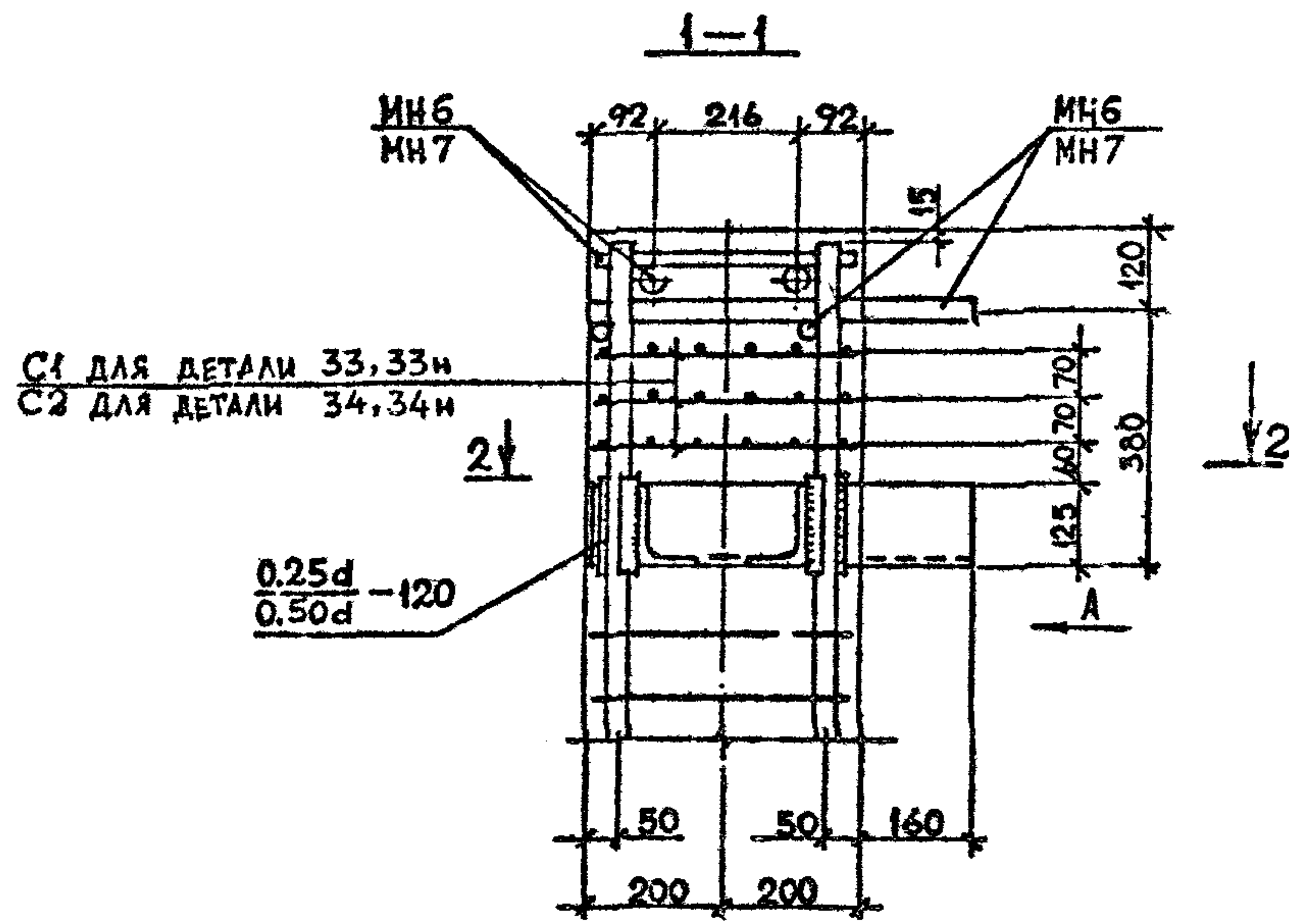
Деталь 33, 34
