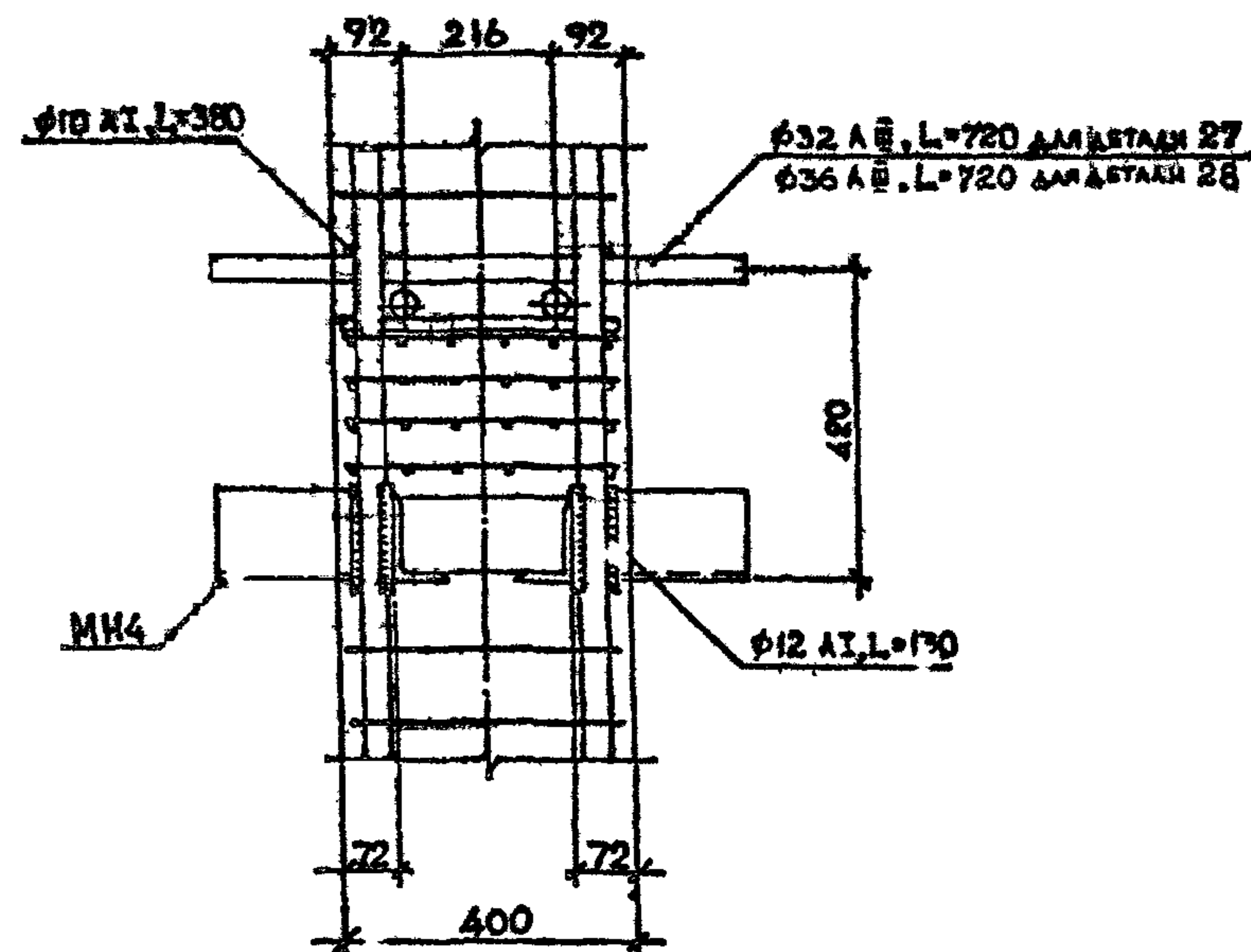
Вид А
