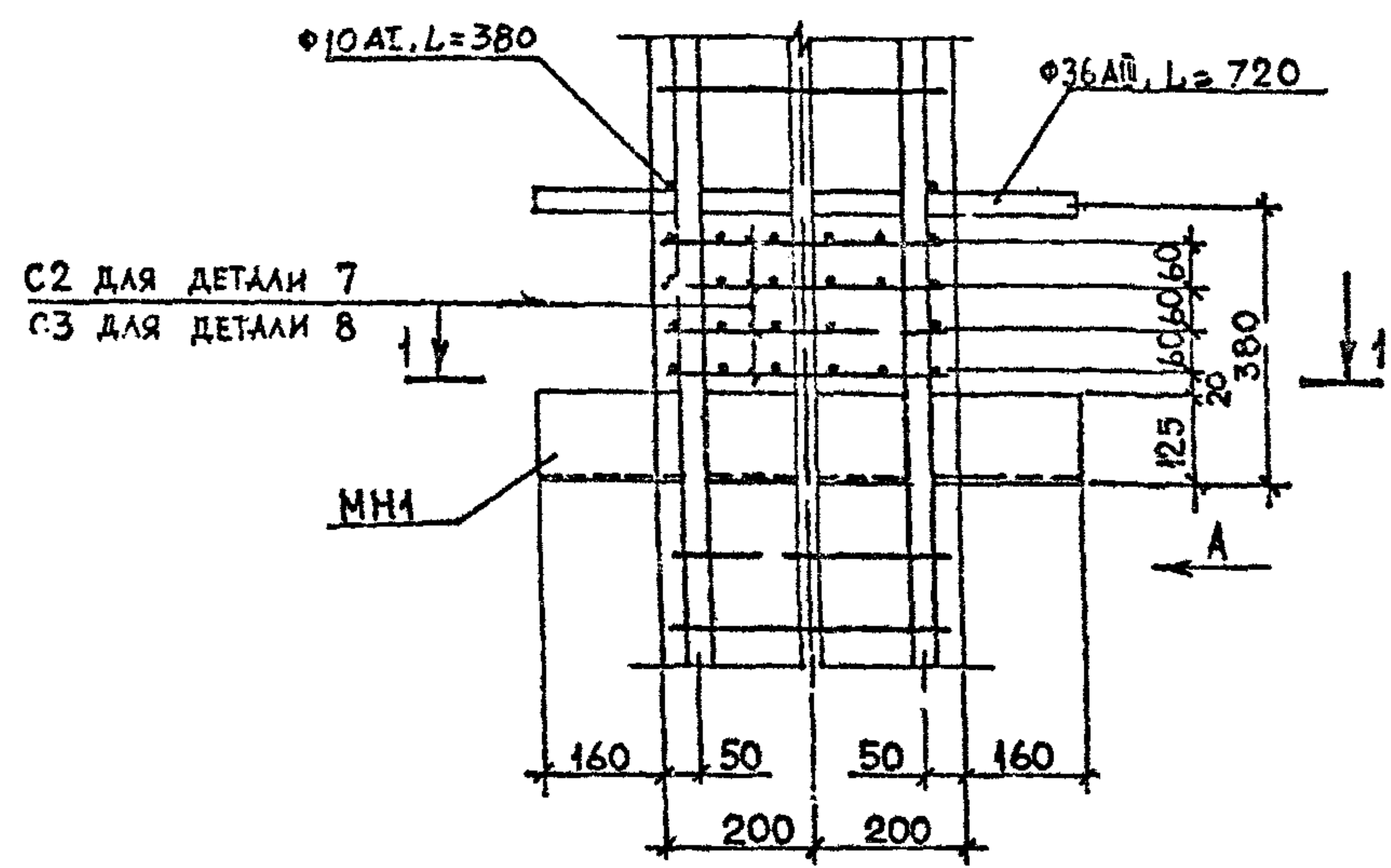
ДЕТАЛЬ 7,8
