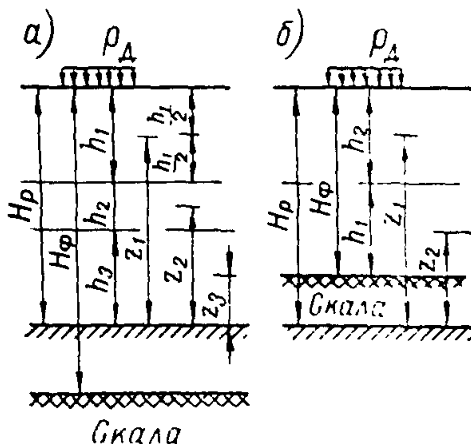
Рис. 3. Схема к определению H_p
