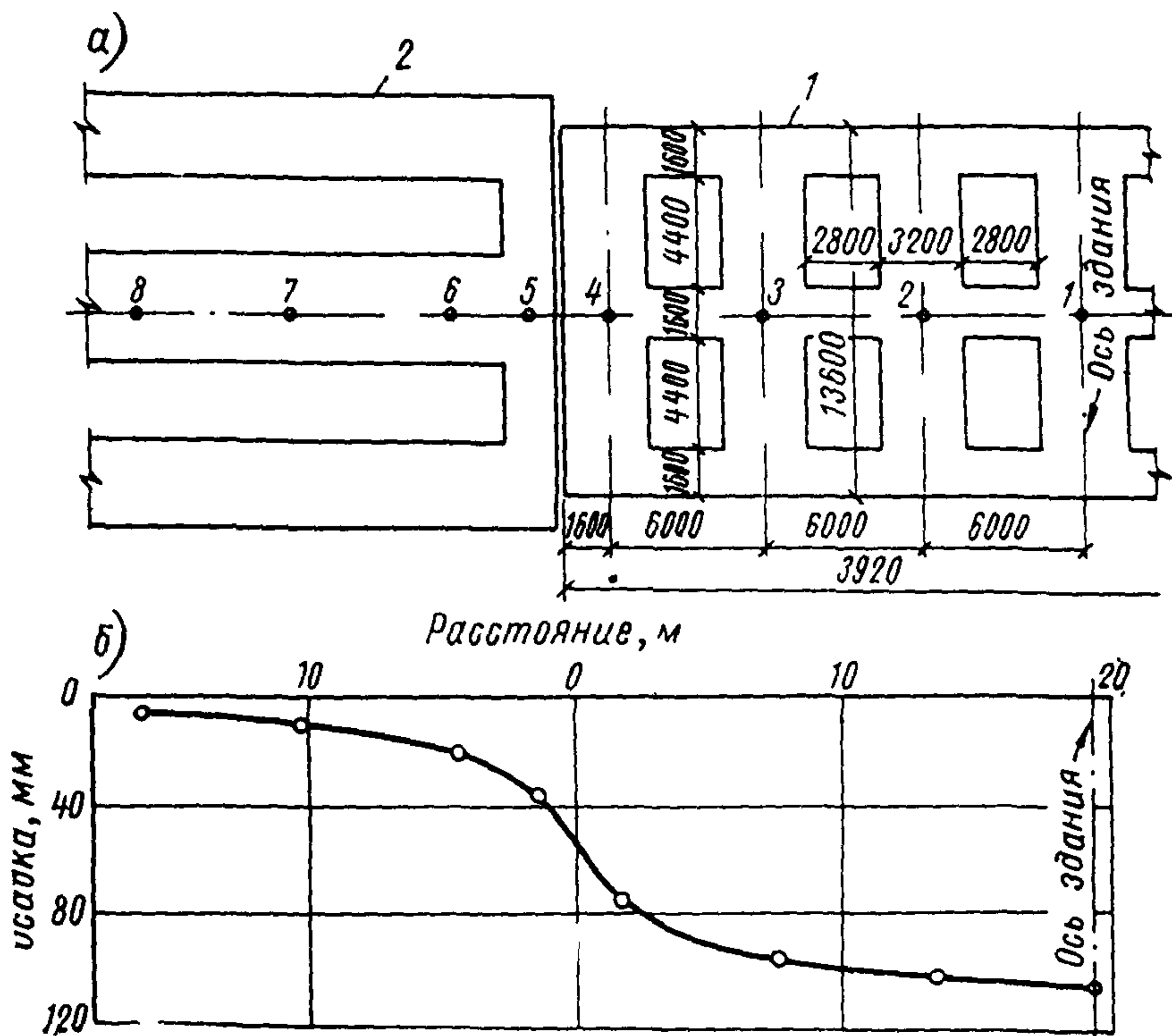
Рис 4 Схема к примеру расчета осадки
