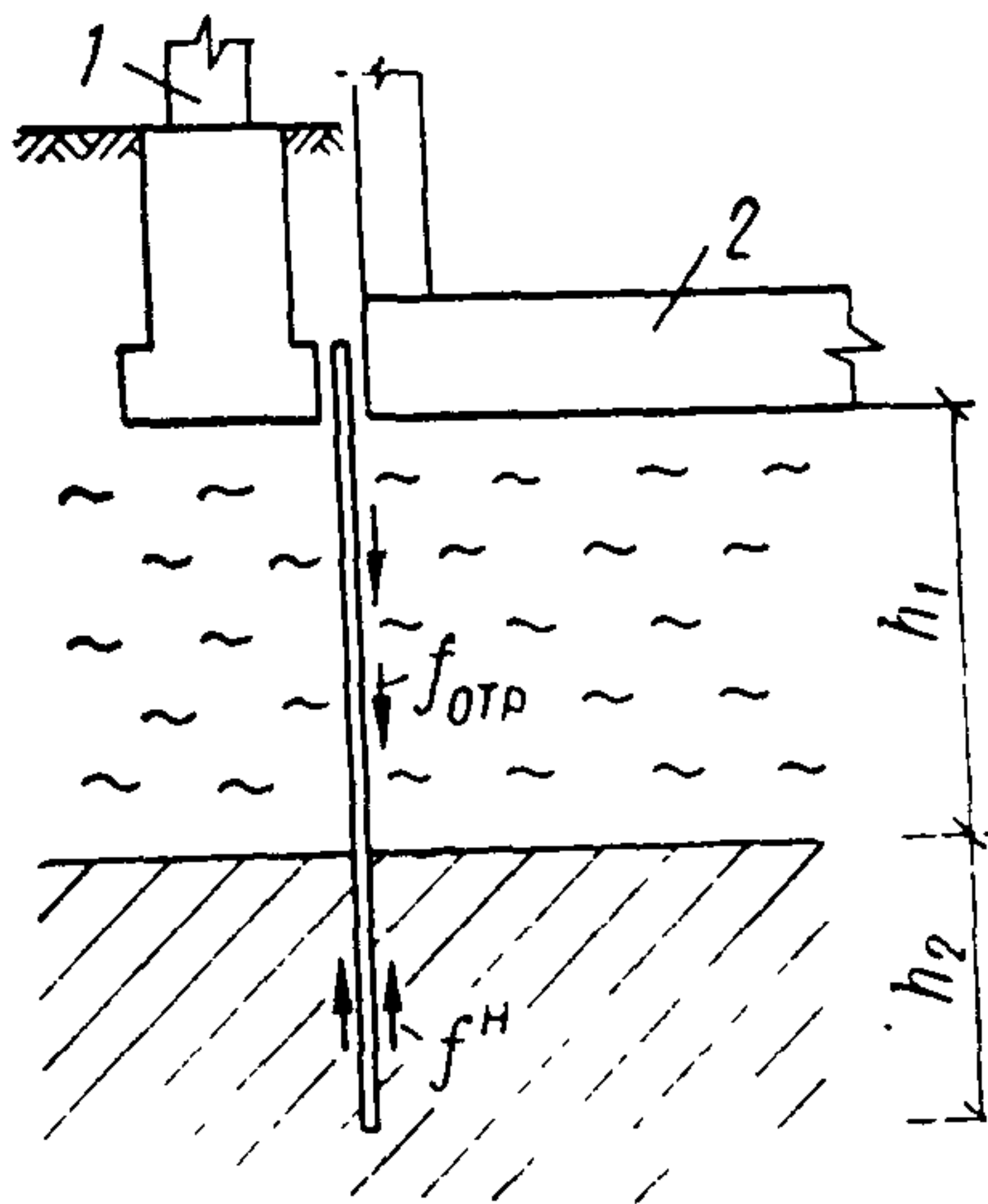
Рис 1. Разъединительная шпунтовая стенка
