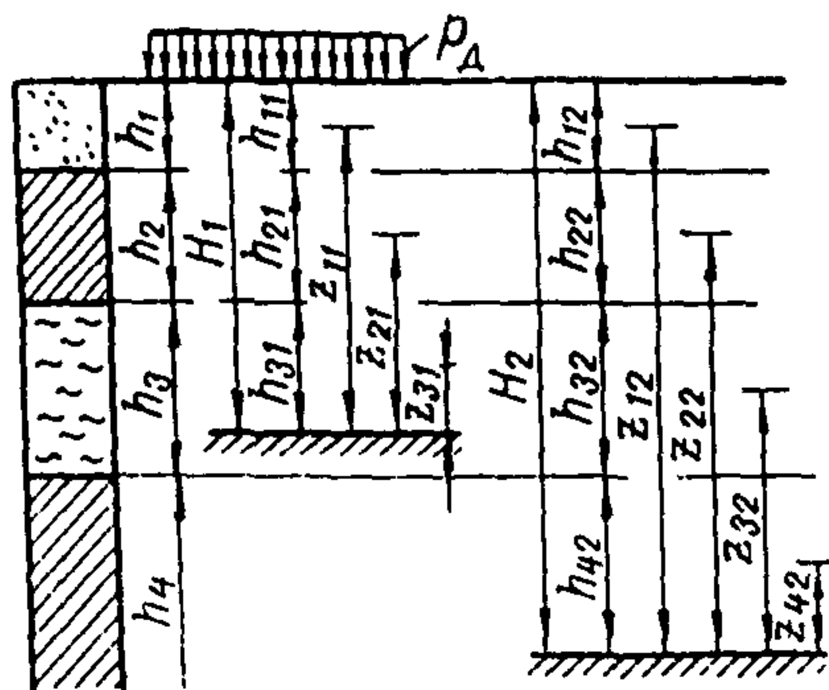
Рис. 2. Схема к определению среднего значения коэффициента относительной сжимаемости
