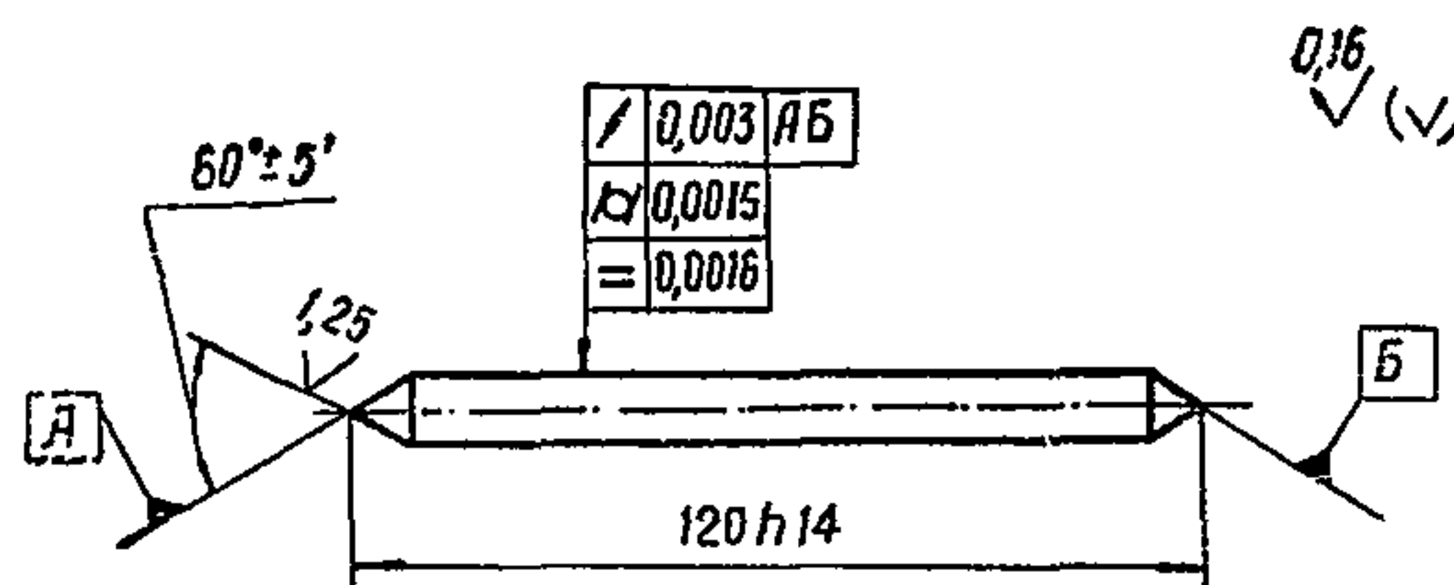
Черт. 14. Валик. Материал — сталь ХВГ ГОСТ 5950—63, НВС58...63
