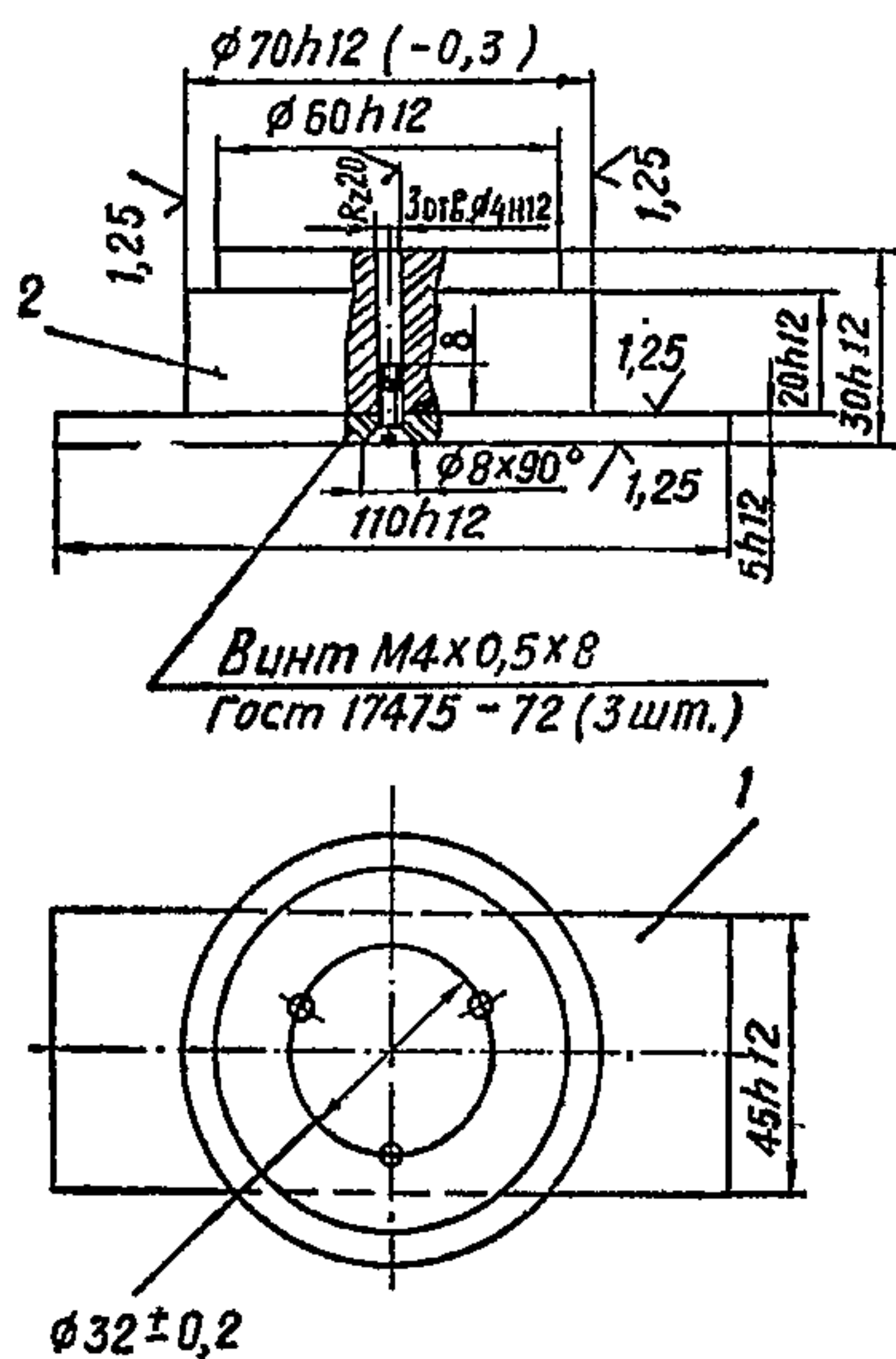
Черт. 1. Приспособление для установки квадранта:
