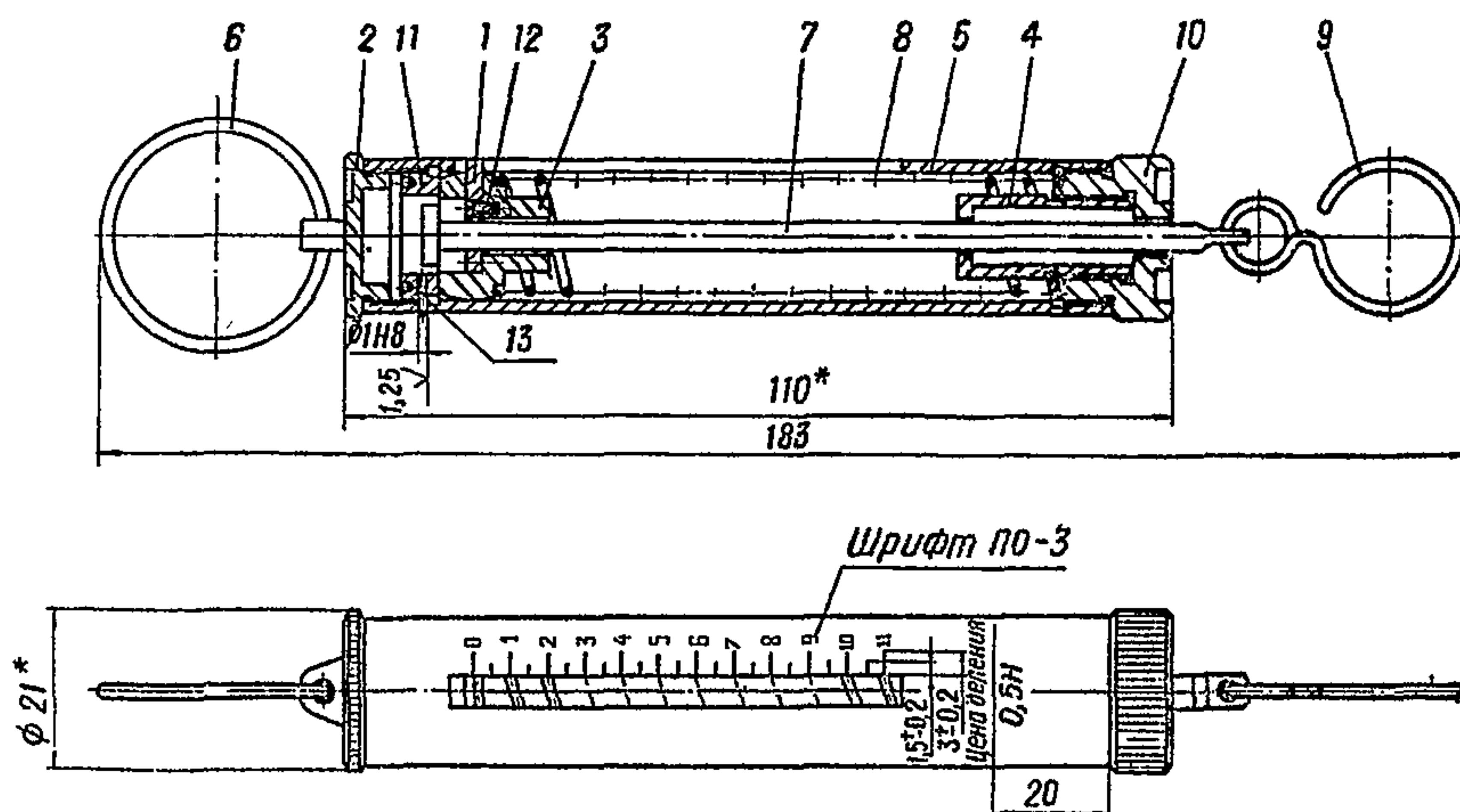
Черт. 8. Динамометр: 1 — указатель; 2 — крышка; 3 — направляющая; 4 — втулка; 5 — гильза; 6 — кольцо; 7 — шток; 8 — пружина; 9 — крючок; 10 — гайка; 11 — гайка; 12 — винт М1,2×5.56.04 ГОСТ 17475—72; 13 — штифт 1h8×5 ГОСТ 3128—70
