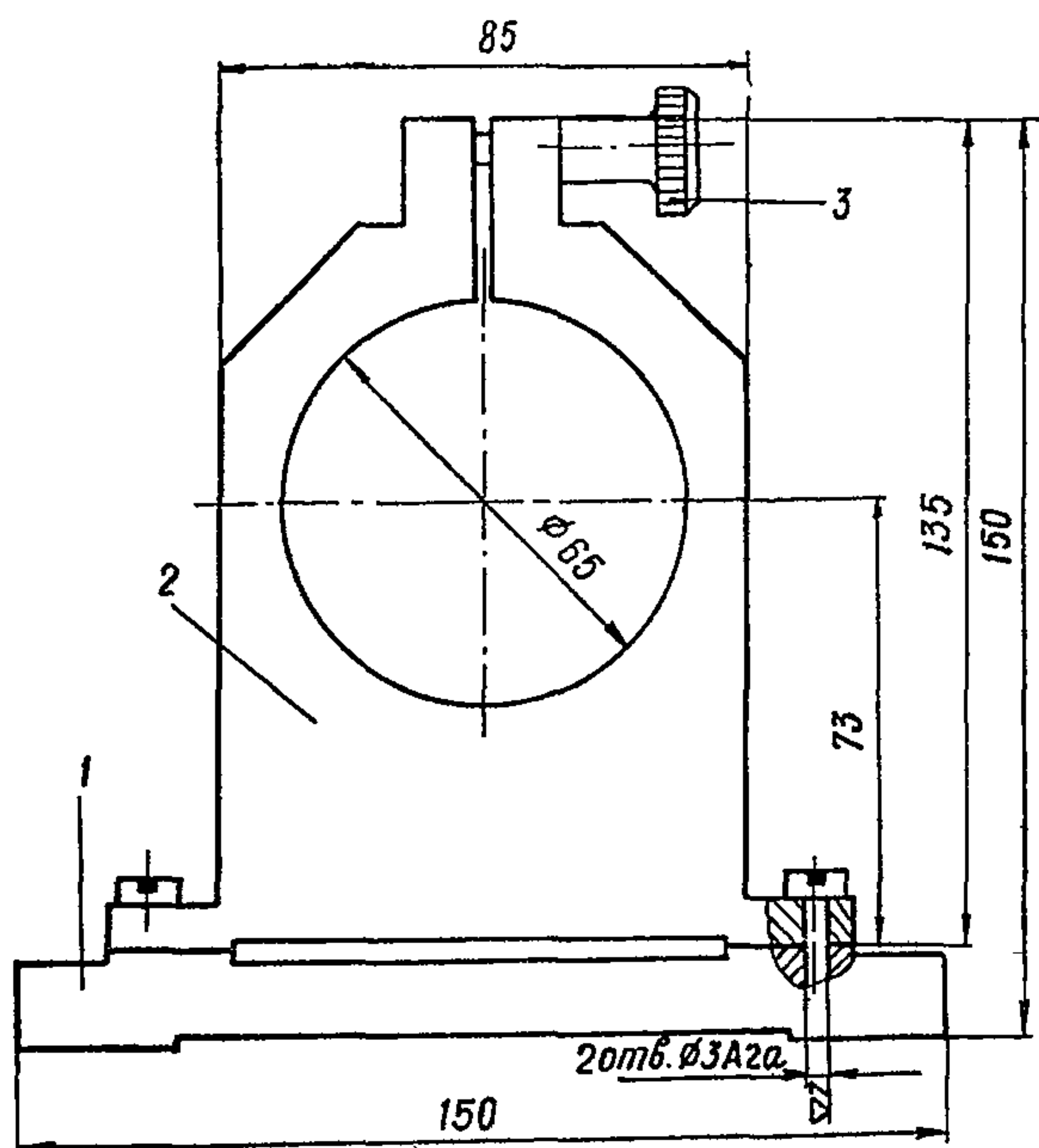
Черт. 5. Кронштейн K_2 : 1 — основание; 2 — крон- штейн; 3 — винт
