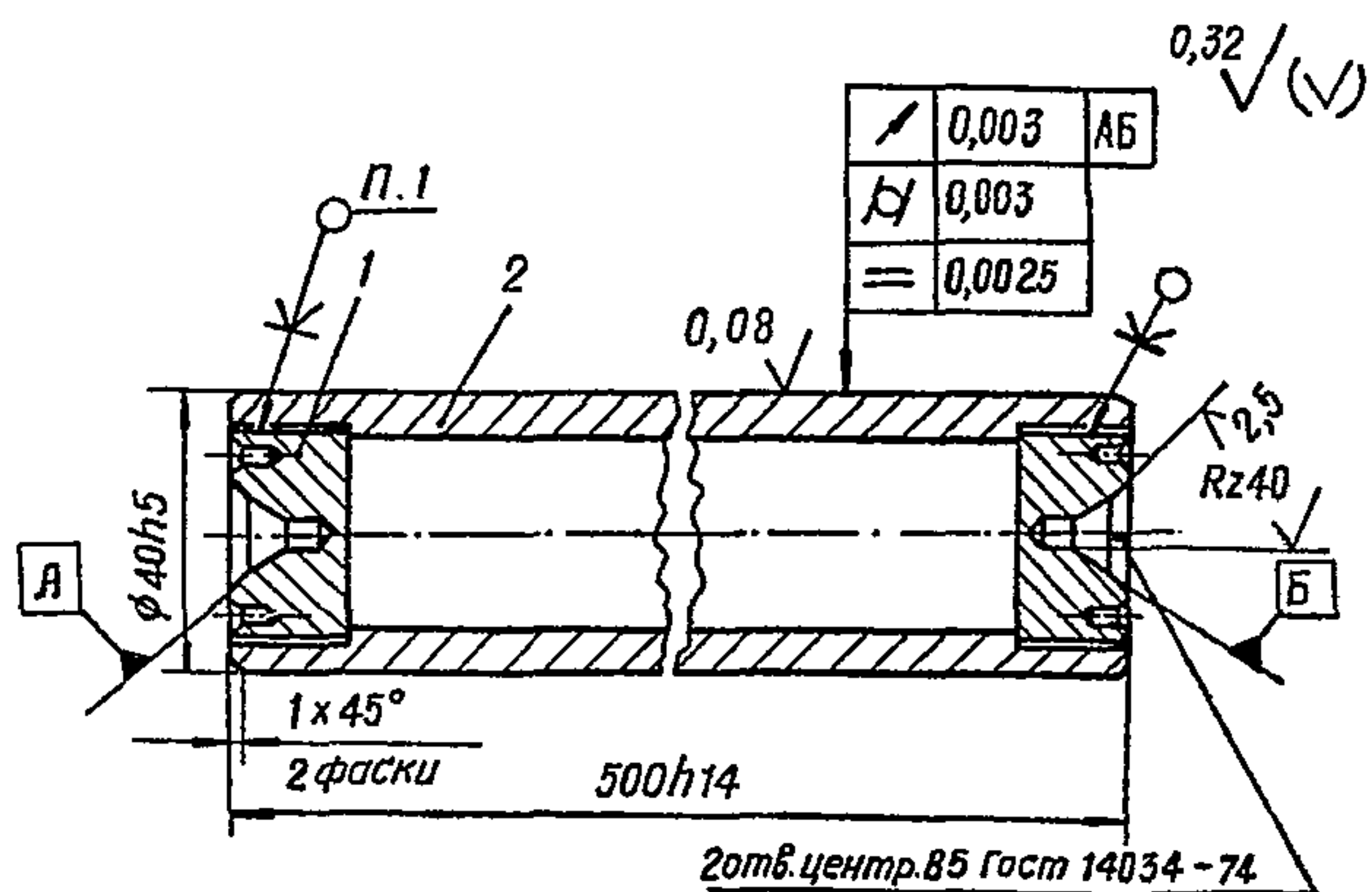
Черт. 13. Валик. Материал — сталь ХВГ ГОСТ 5950—63, НВС58...63:
