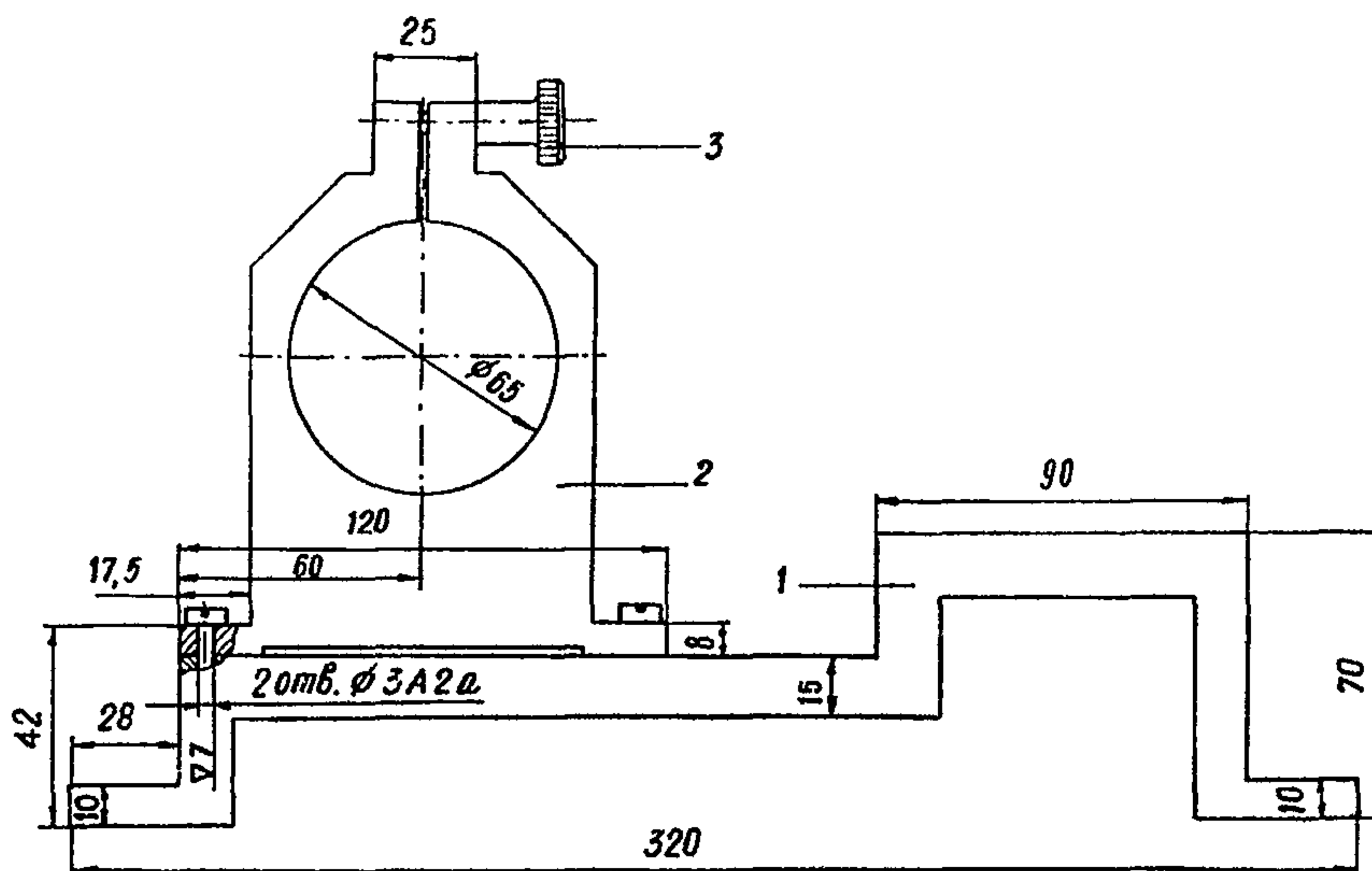
Черт. 7. Кронштейн К 3 : 1 — скоба; 2 — кронштейн; 3 — винт
