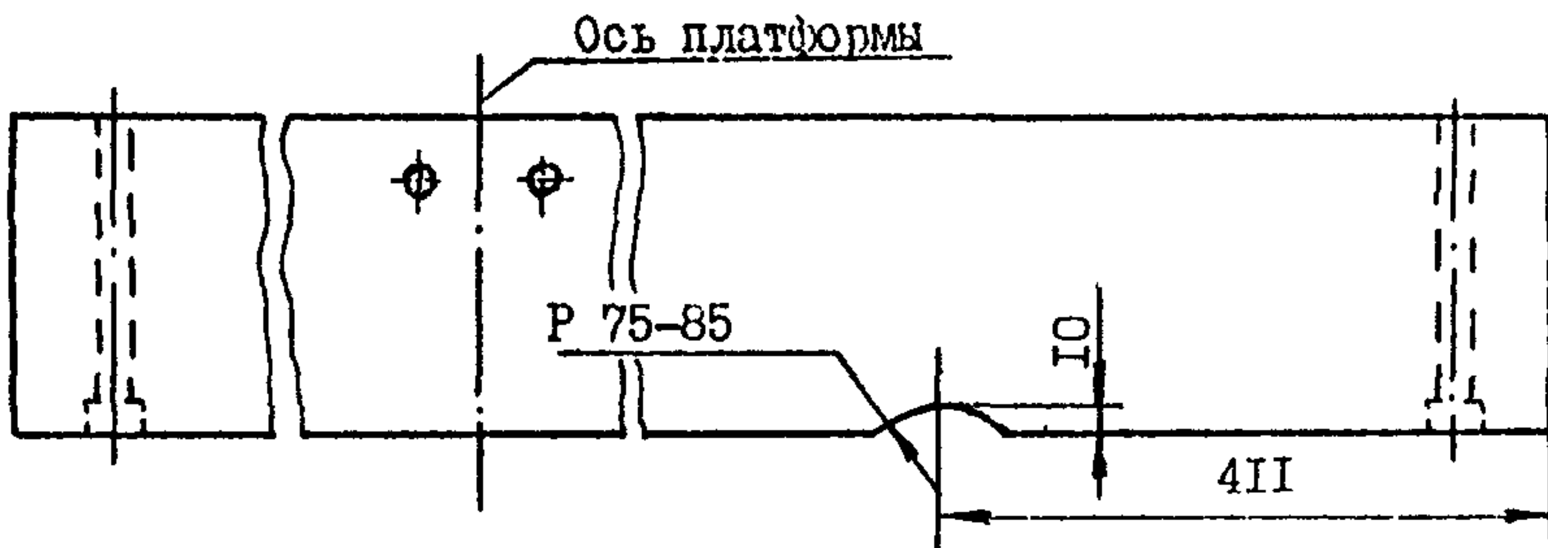
Рис. 5.33 Передний поперечный брус автомобиля ГАЗ-52-07
