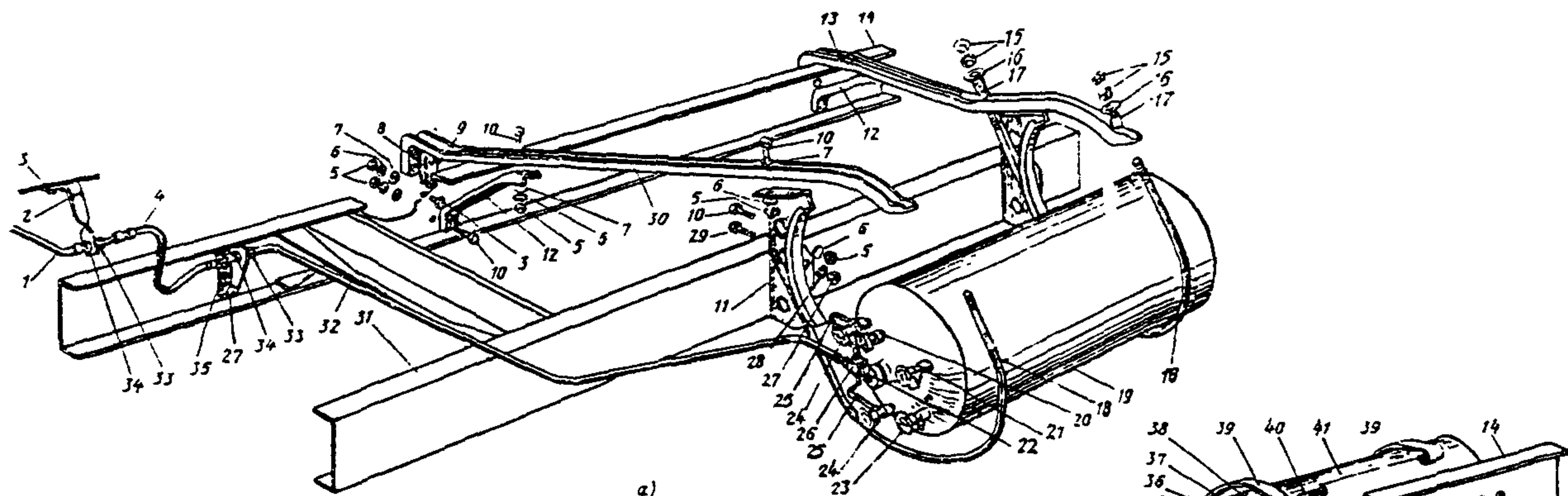
Рис. 5.8 Крепление баллонов на автомобилях
