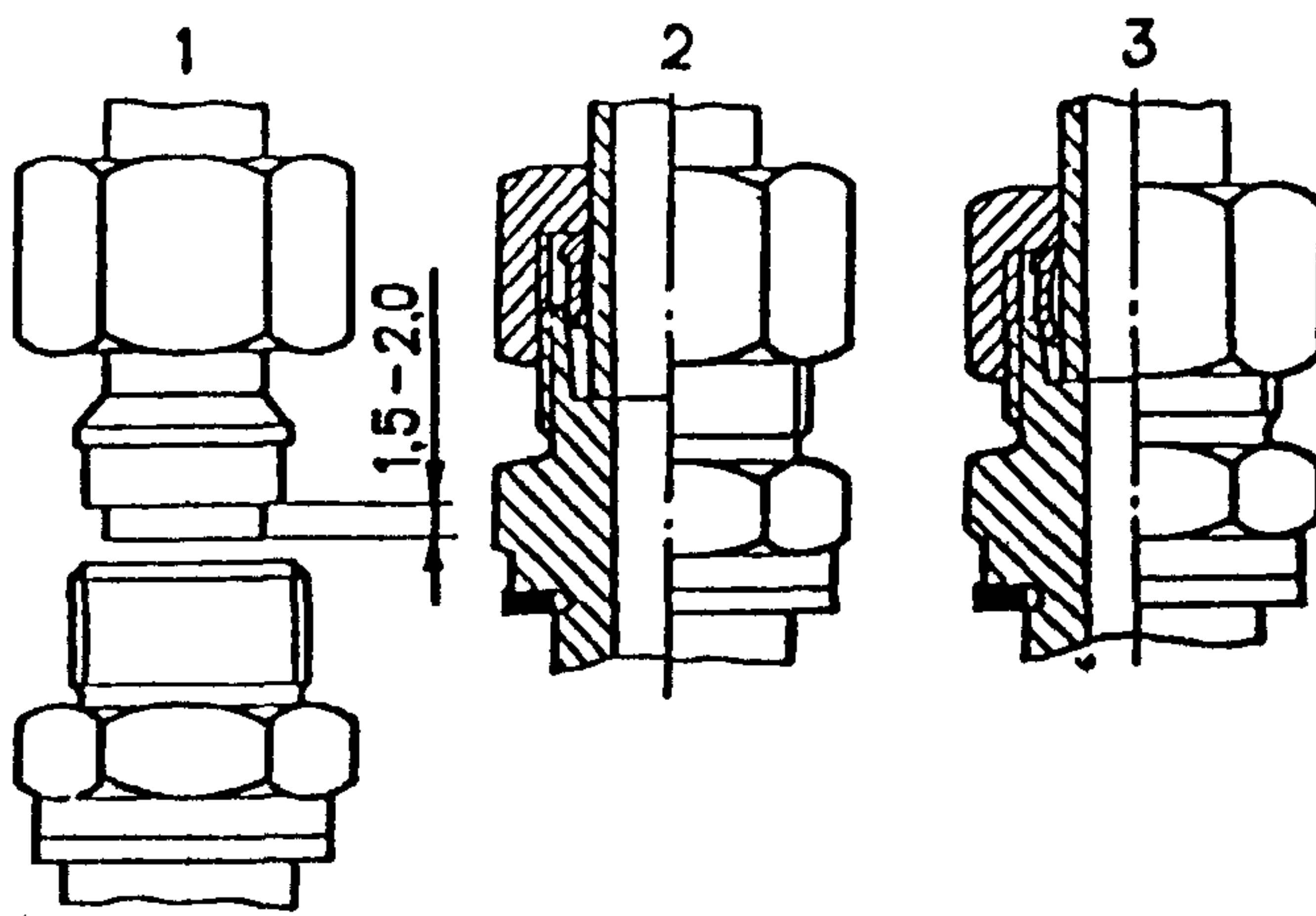
Рис. 5.20 Соединение при помощи врезавшегося кольца
