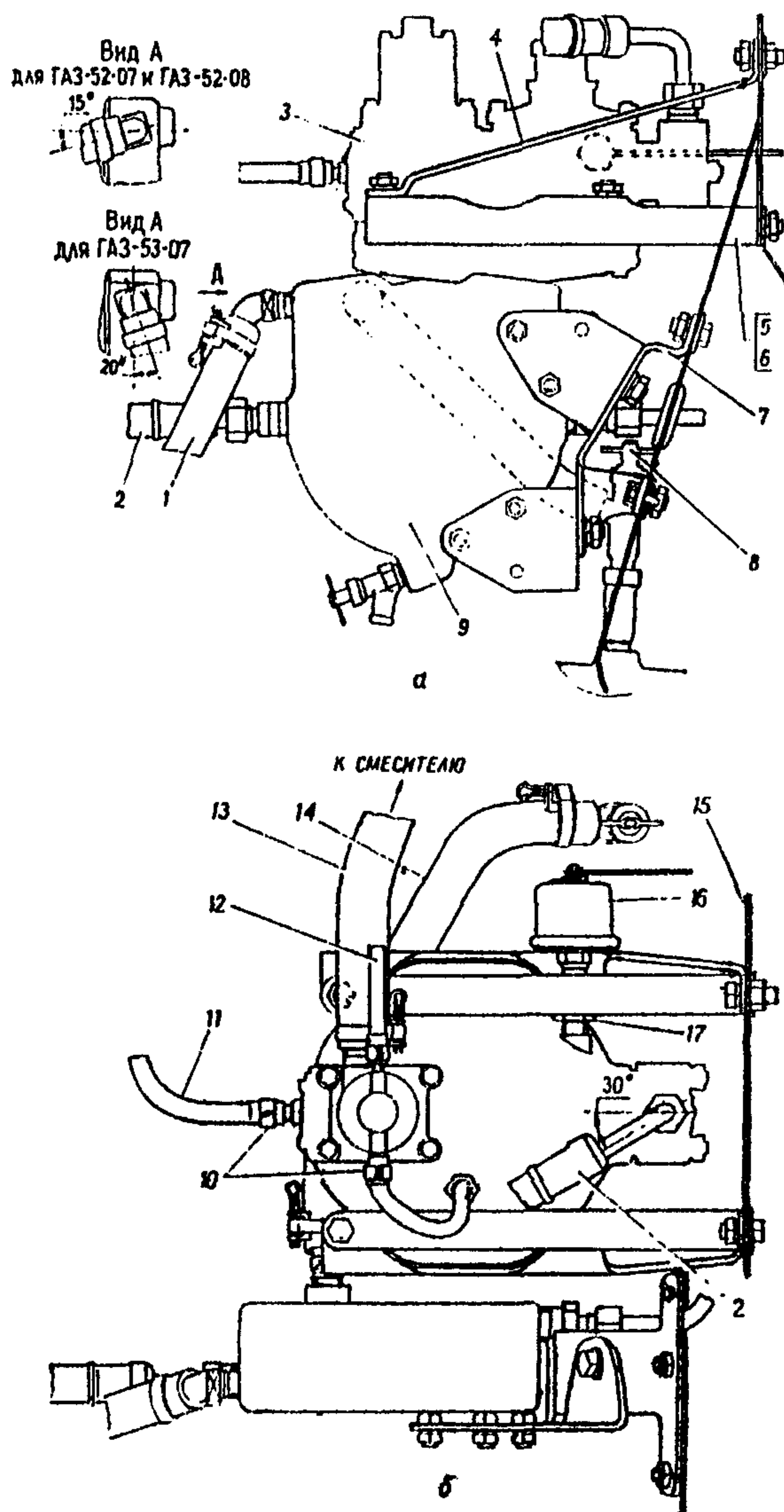
Рис. 5.40. Установка газового оборудования
