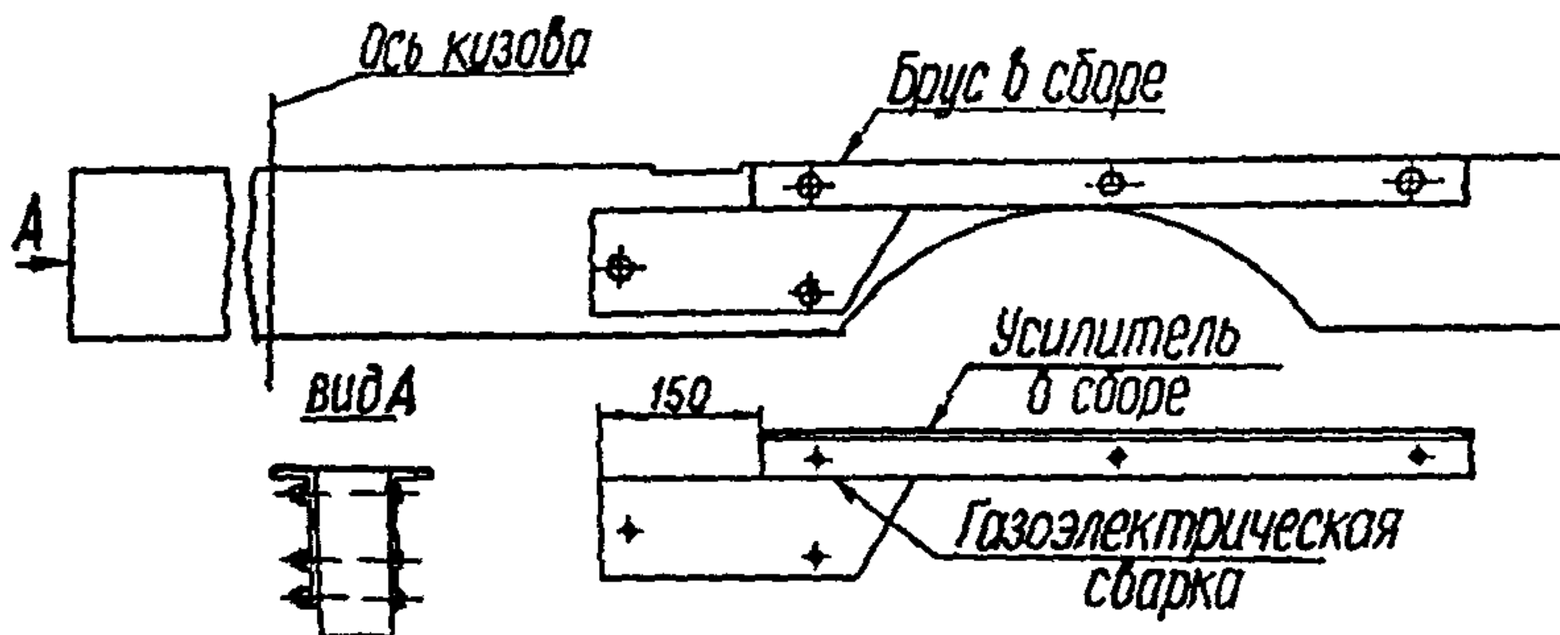
Рис. 5.49. Брус и усилитель в сборе
