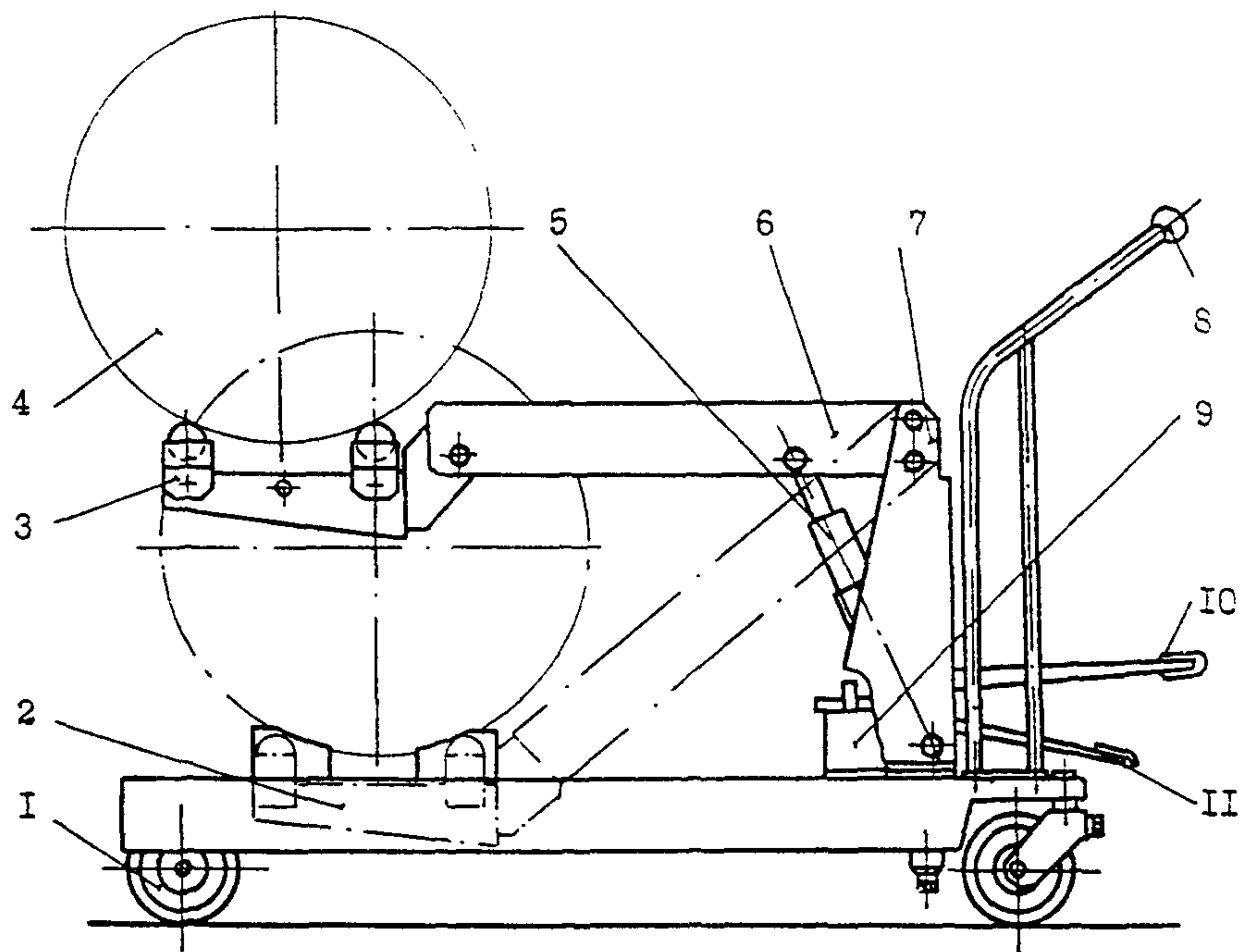
Рис. 6.1. Тележка для снятия, постановки и транспортировки газовых баллонов автомобилей
