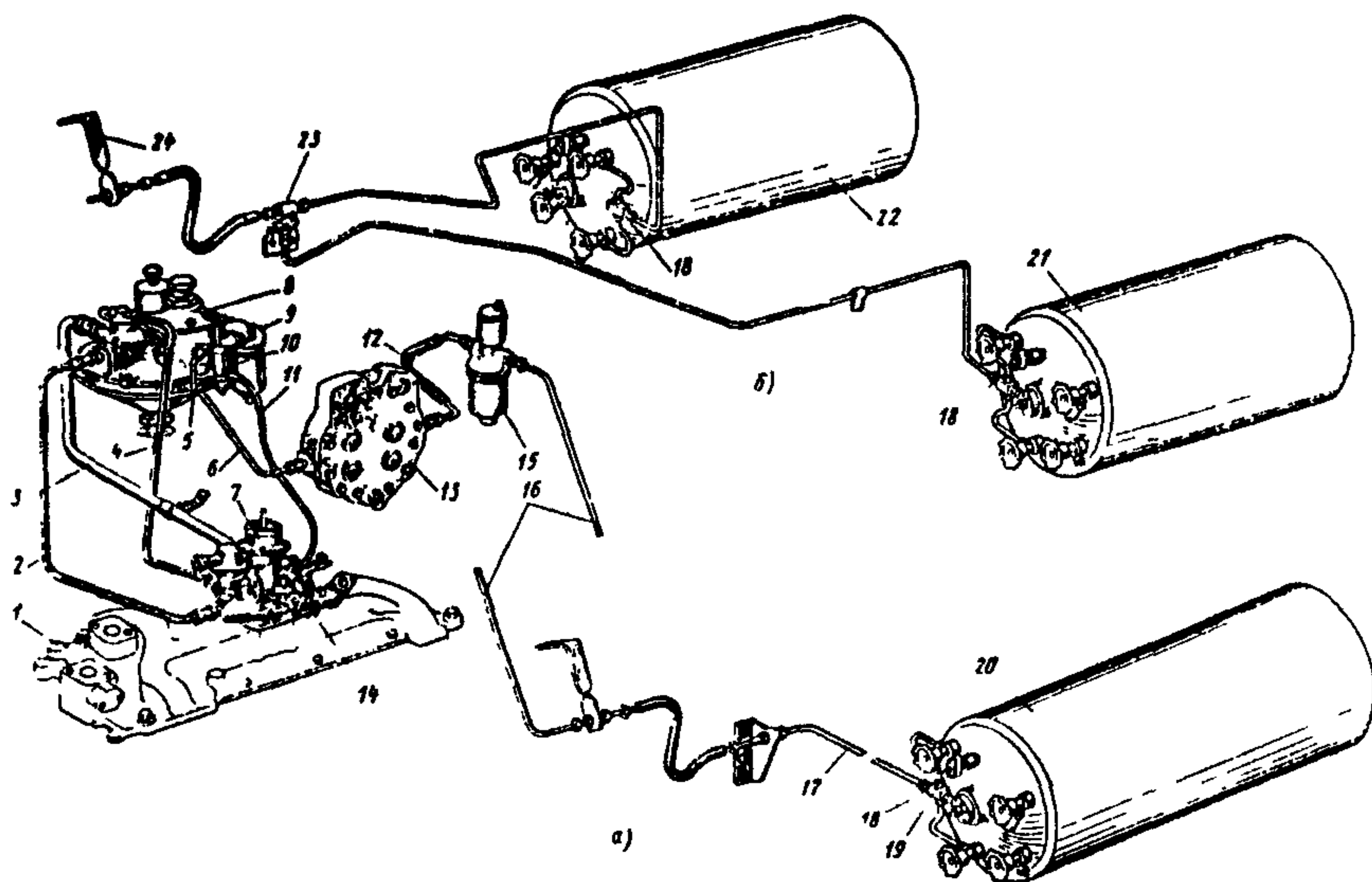
Рис. 5.1 Газовая топливная система автомобилей
