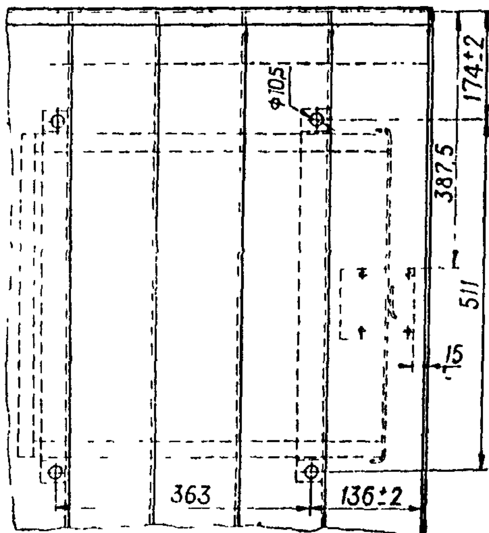
Рис.5.45 Основание платформы автомобиля ГАЗ-52-07
