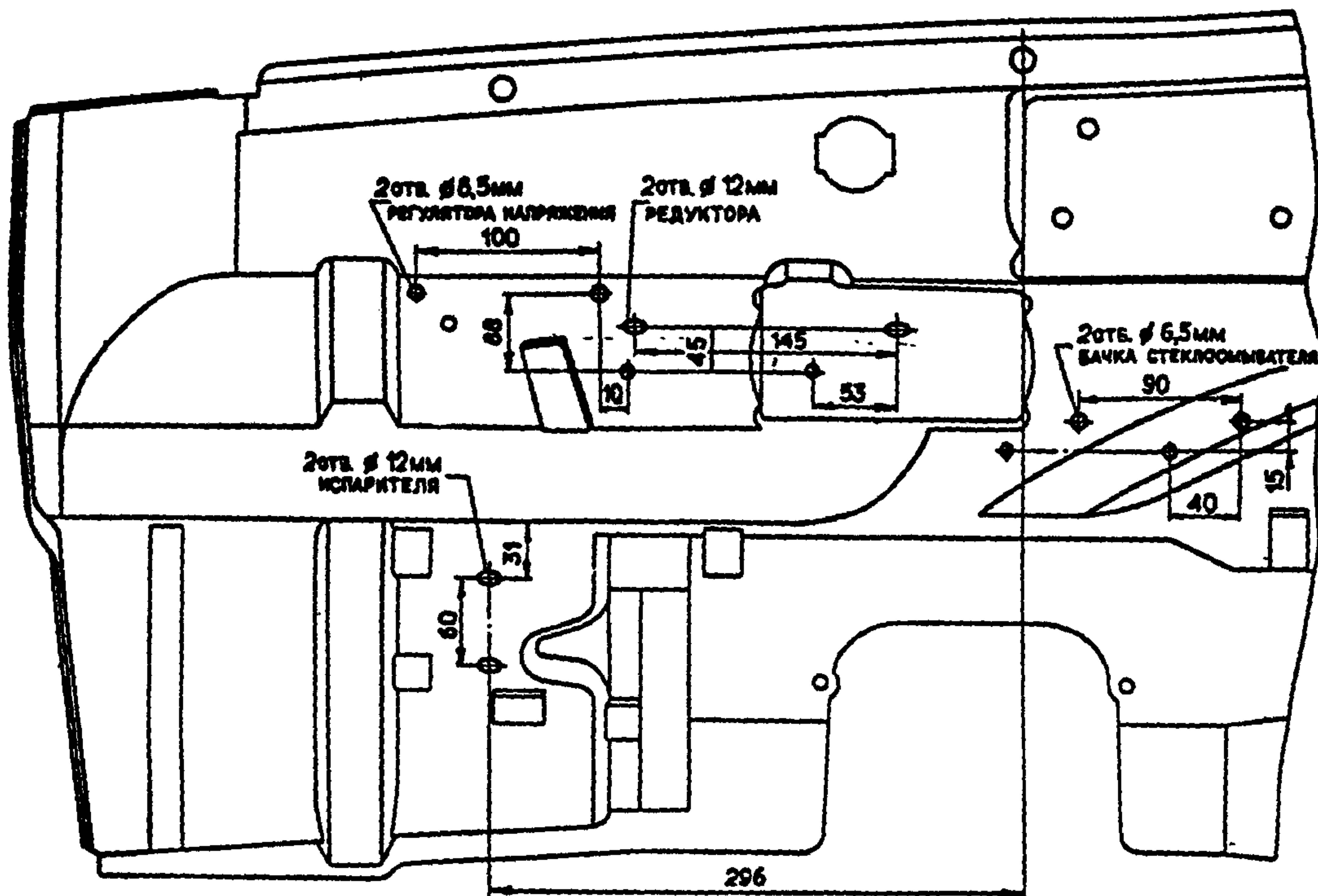
Рис. 5.9 Разметка отверстий на брызговике правого переднего крыла для крепления газового редуктора, испарителя, кронштейна бачка стеклоомывателя и регулятора напряжения
