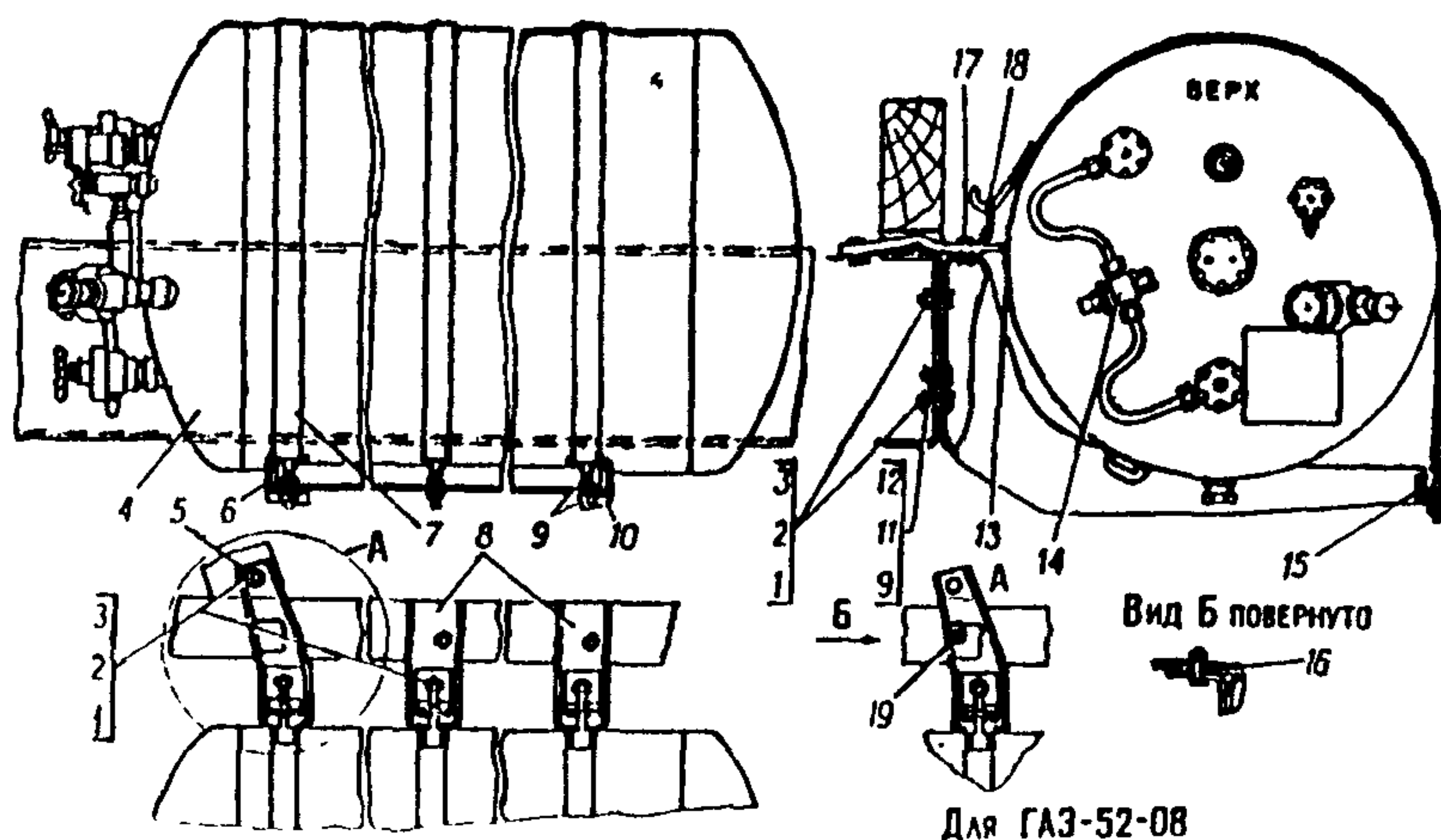
Рис. 5.31. Установка баллона на автомобили ГАЗ-53-07 и ГАЗ-52-08
