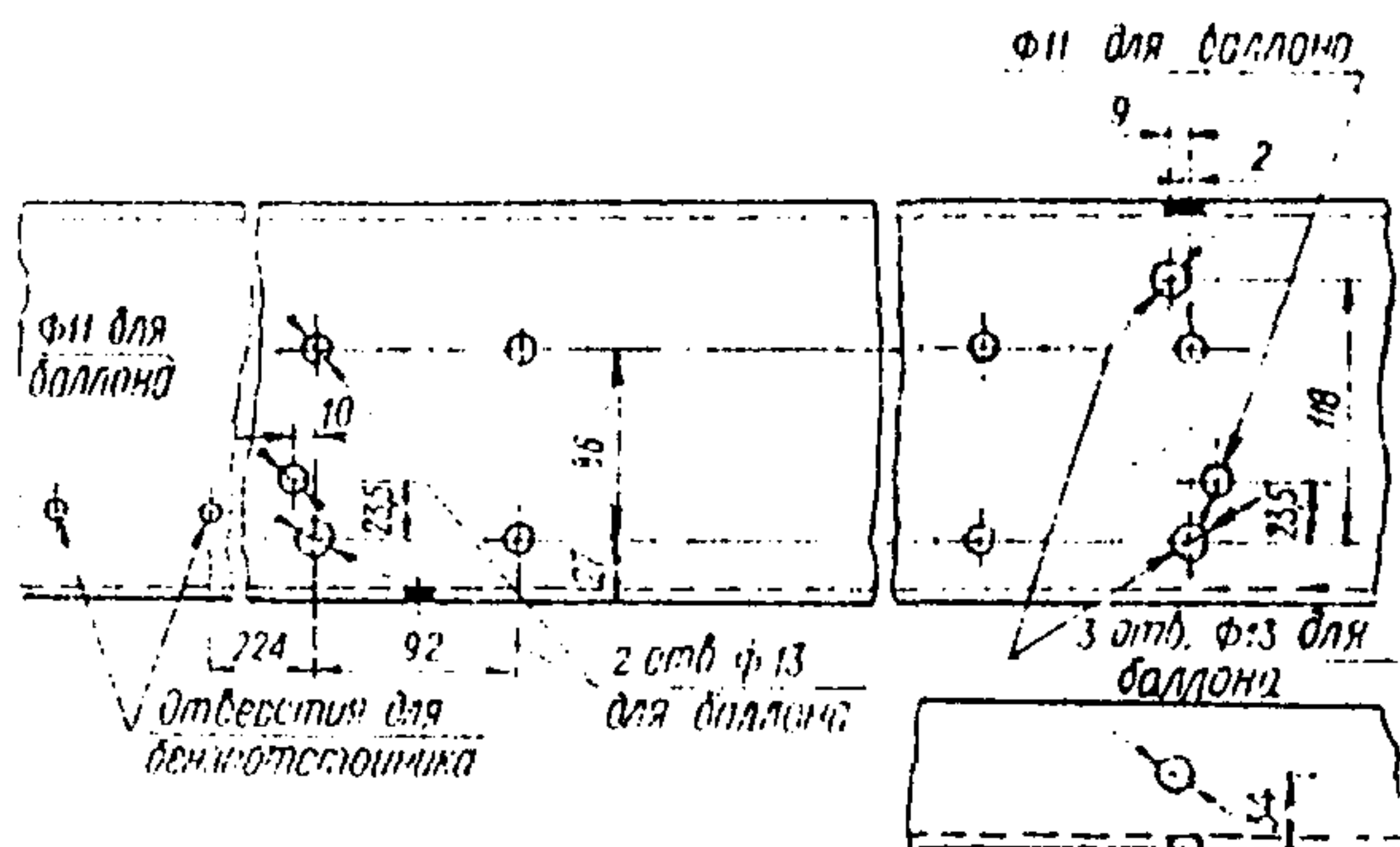
Рис. 5.34. Левый лонжерон рамы автомобиля ГАЗ-52-07
