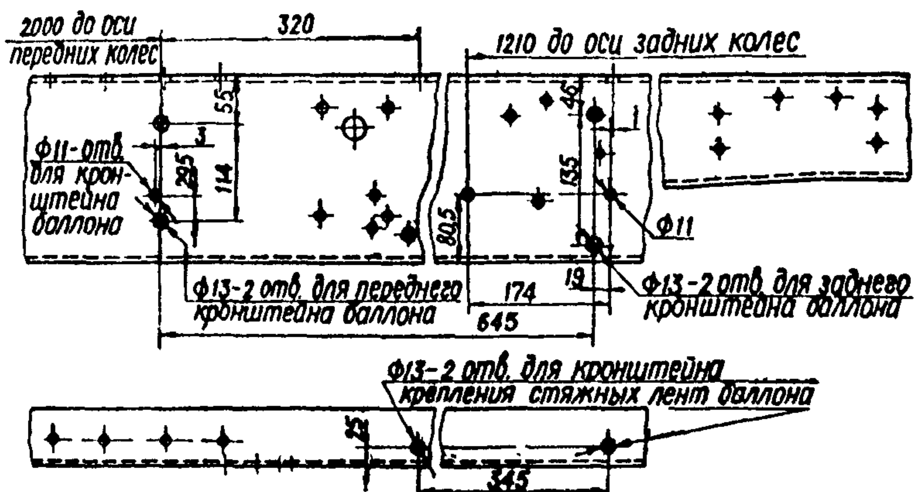
Рис. 5.32. Левый лонжерон рамы автомобилей ГАЗ-53-07 и ГАЗ-52-08
