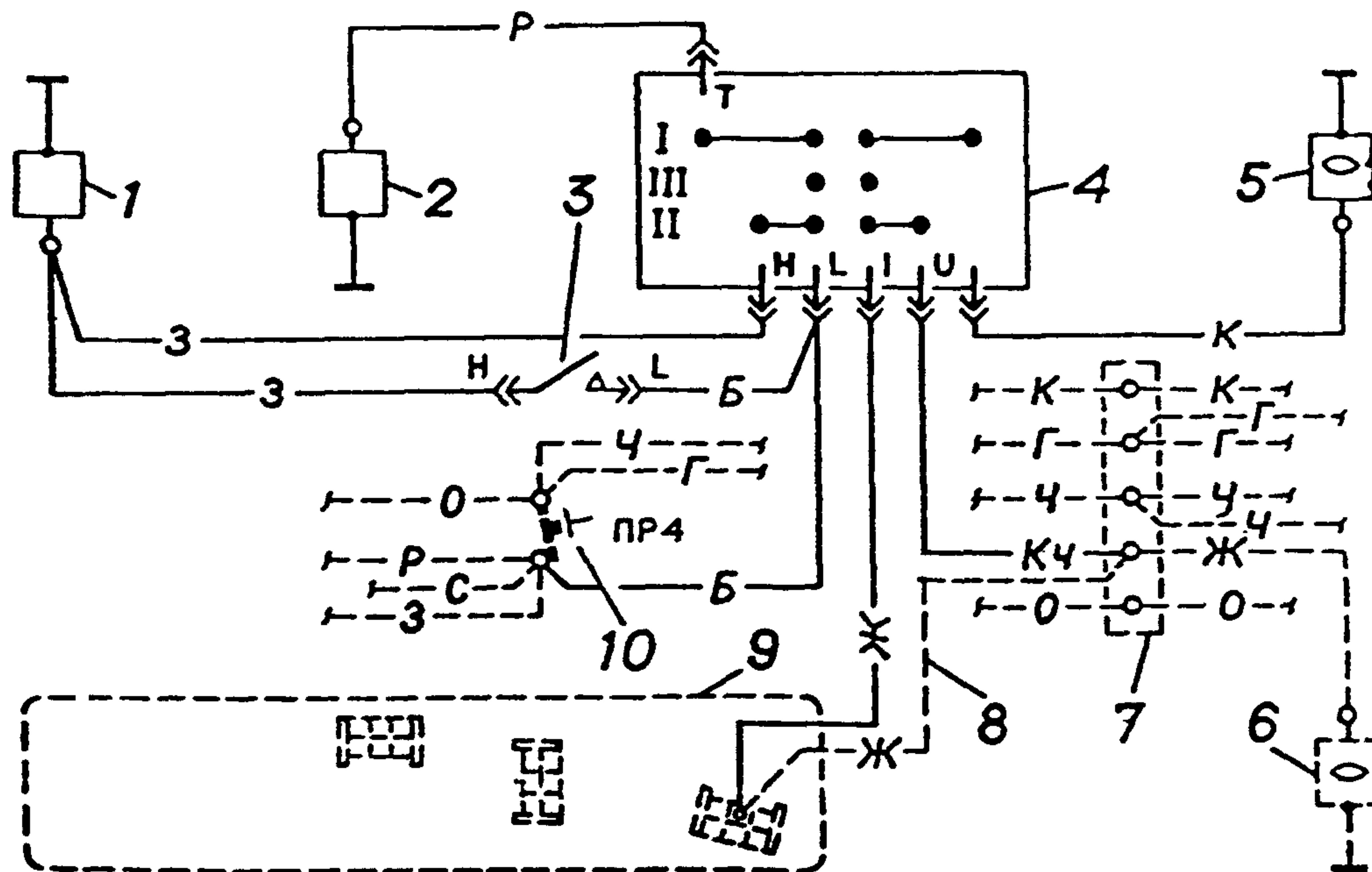
Рис. 5.23 Изменения в схеме электрооборудования для автомобилей ГАЗ-24 и ГАЗ-24-01 выпуска 1985 г., дооборудуемых газовой аппаратурой
