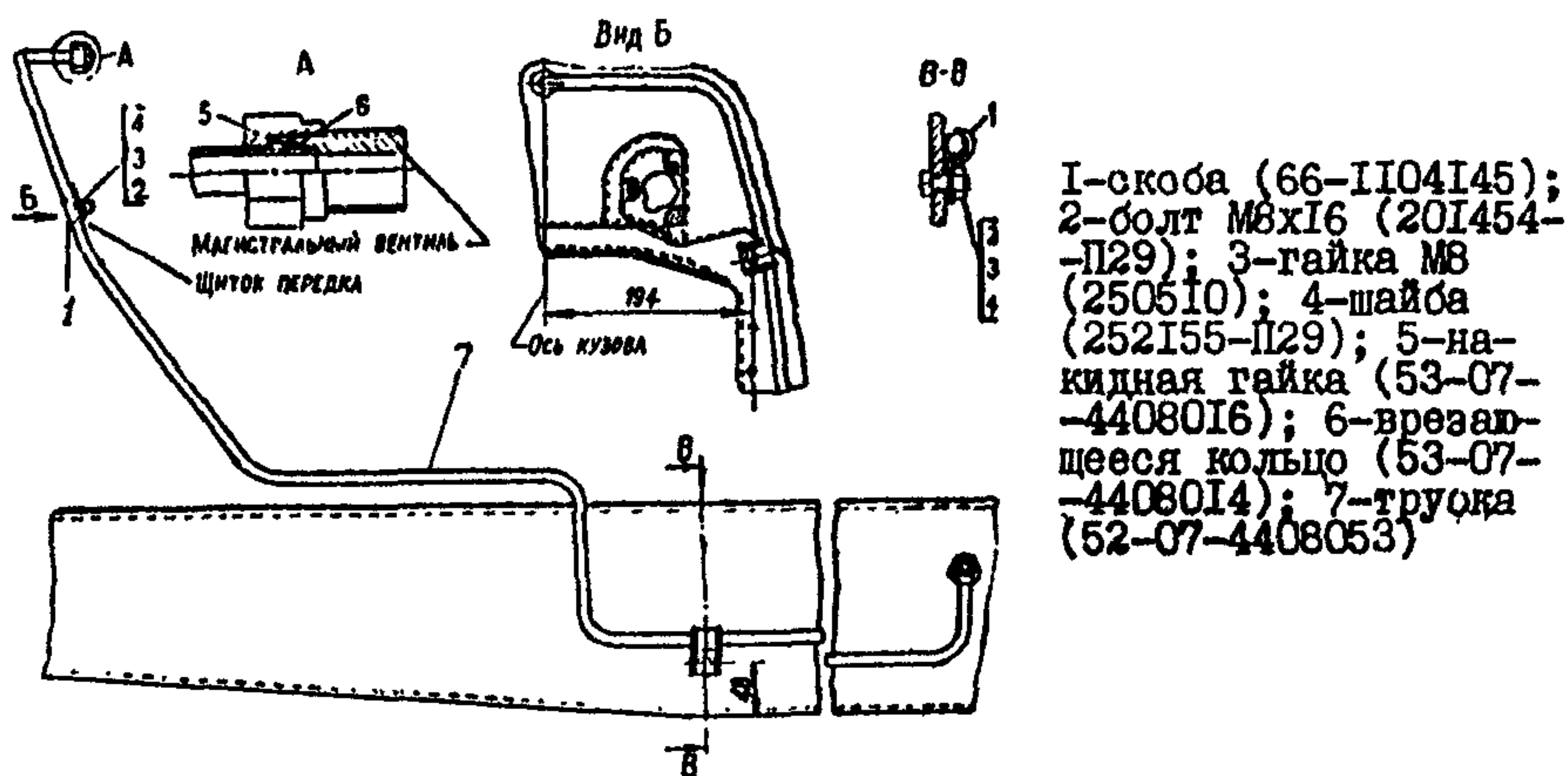
Рис. 5.41. Установка трубки от баллона к магистральному вентилю
