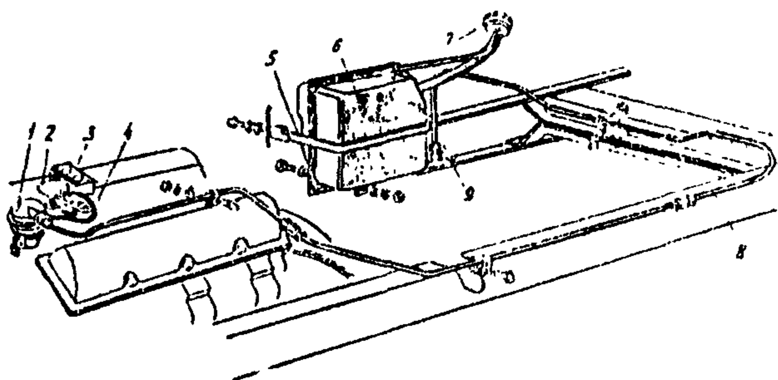
Рис. 5.7 Бензиновая резервная топливная система автомобилей ЗИЛ
