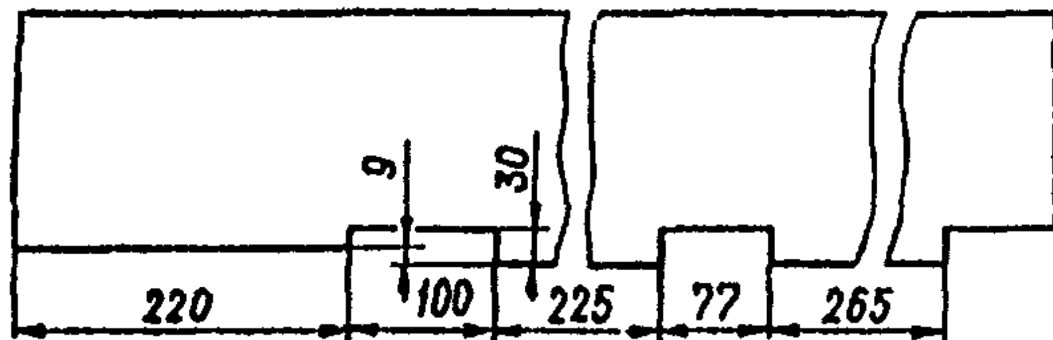
Рис. 5.42. Надставка продольного бруса автомобиля ГАЗ-53-07
