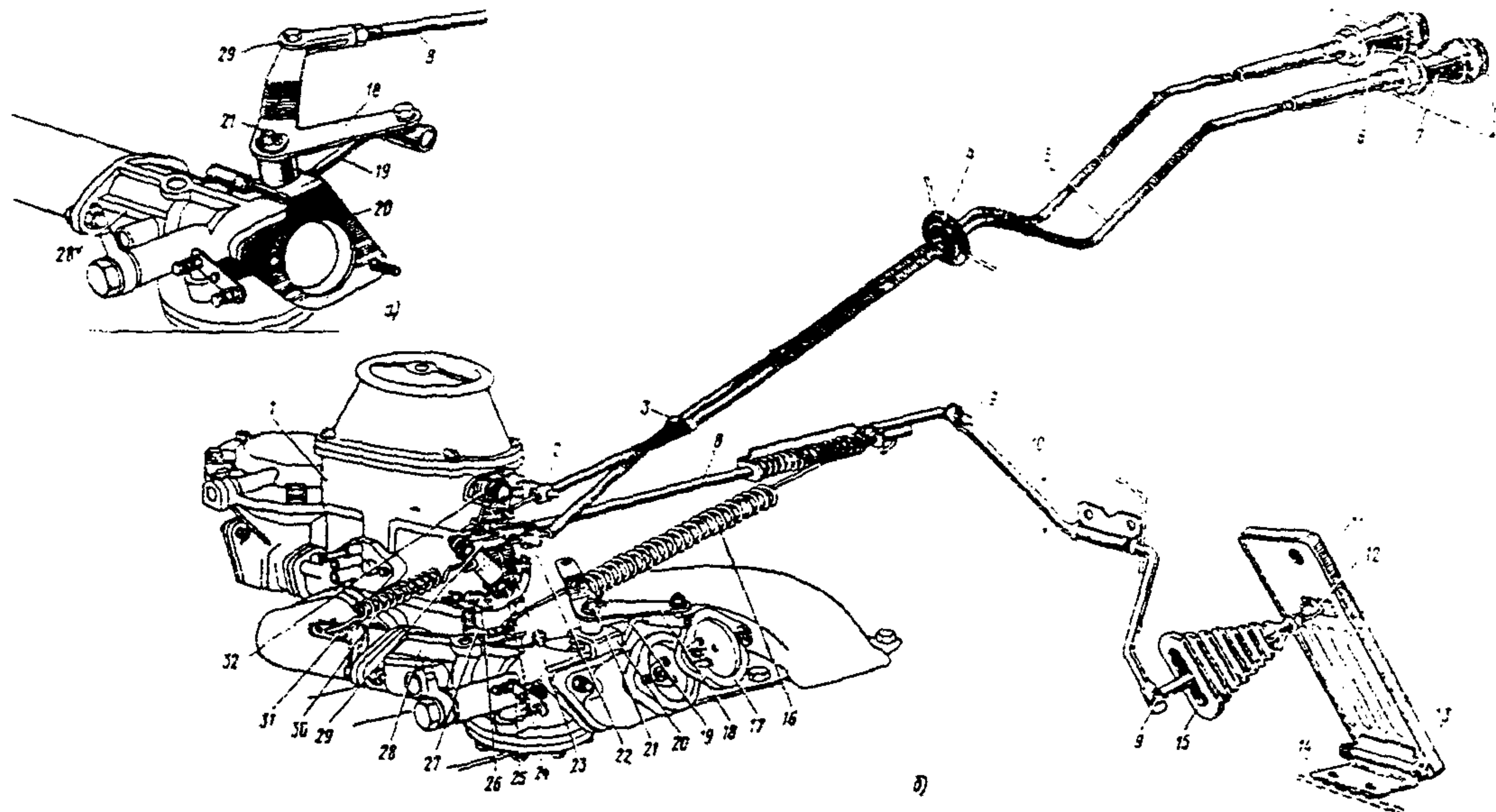
Рис. 5.6 Схема механизма управления подачей топлива при работе двигателя ЗИЛ-130 а - на газе; б - на бензине; 1 - смеситель; 2, 23 и 24 - рычаги пусковой системы; 3 - хомут; 4 - заглушка; 5 - тросы; 6 - рукоятка управления рычагом дроссельных заслонок смесителя; 7 - рукоятка управления рычагами пусковой системы; 8 - тяга; 9 - пальцы со шпильками; 10 - валик; 11 - педаль; 12 - толкатель; 13 - ось педали; 14 - кронштейн педали; 15 - уплотнитель; 16, 30 и 32 - оттяжные пружины; 17 - крышка патрубка карбюратора в открытом положении при работе двигателя на бензине; 18 - двуплечий рычаг привода дроссельной заслонки карбюратора; 19 - тяга привода дроссельной заслонки карбюратора; 20 - кронштейн двуплечего рычага; 21 - ось рычага; 22 - зажим троса; 25 - рычаг воздушной заслонки карбюратора; 26 - рычаг привода дроссельных заслонок смесителя; 27 и 31 - кронштейны пружин; 28 - карбюратор; 29 - наконечник тяги
