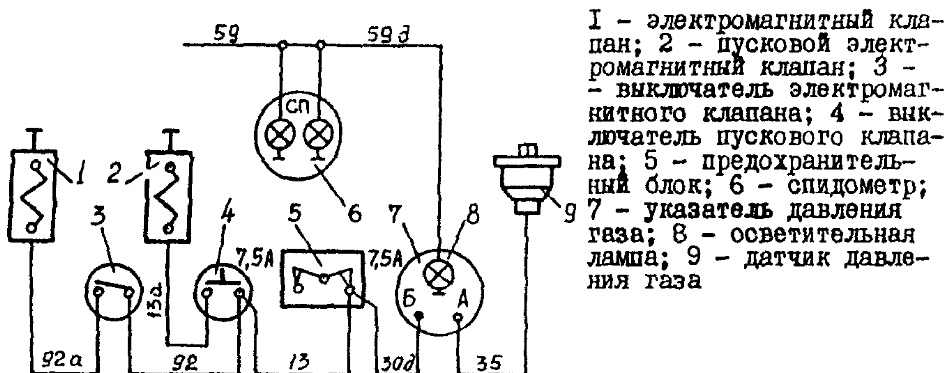
Рис. 5.5 Схема дополнительного электрооборудования
