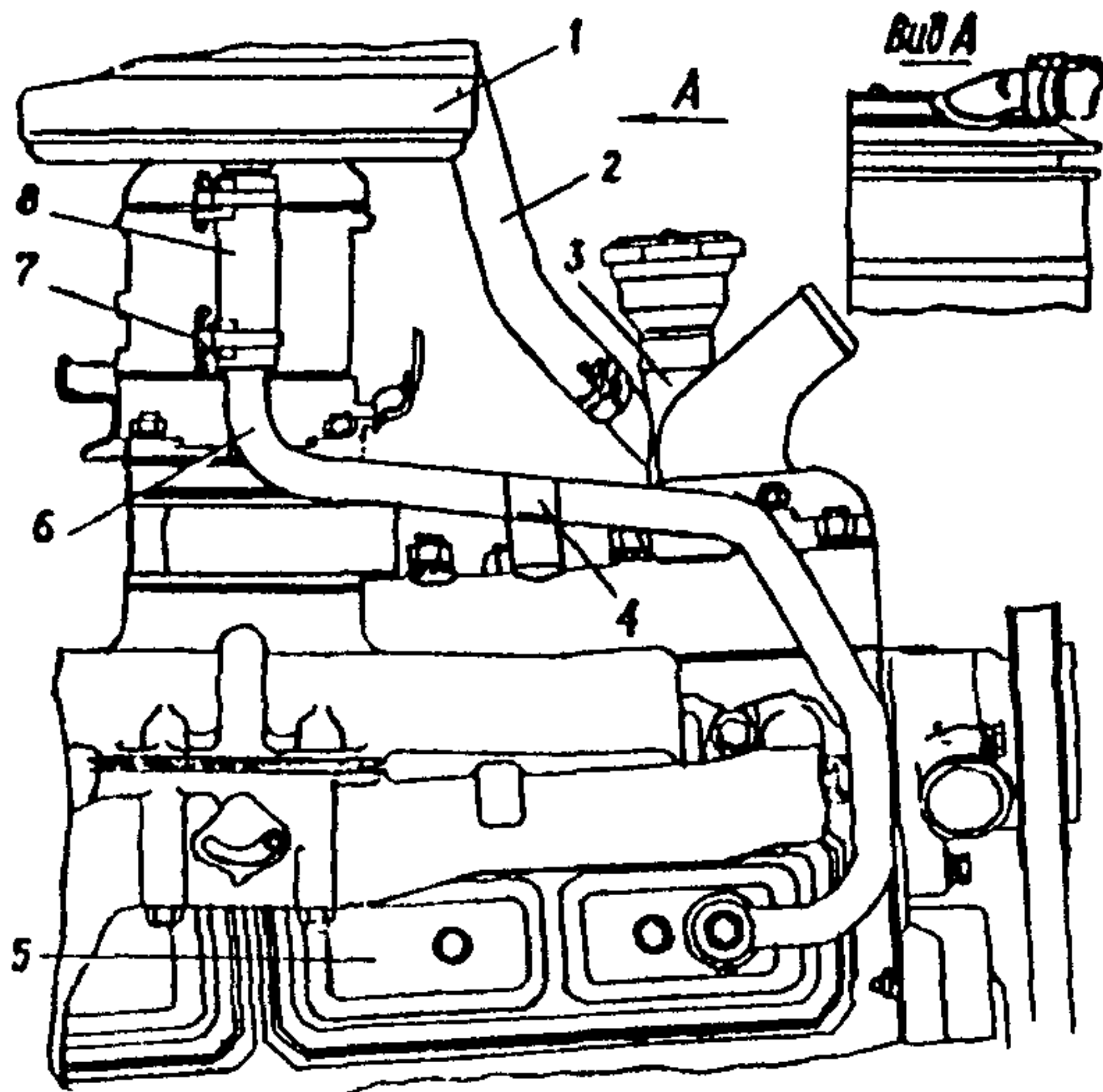
Рис. 5.30. Установка деталей закрытой вентиляции картера двигателя ГАЗ-52-08
