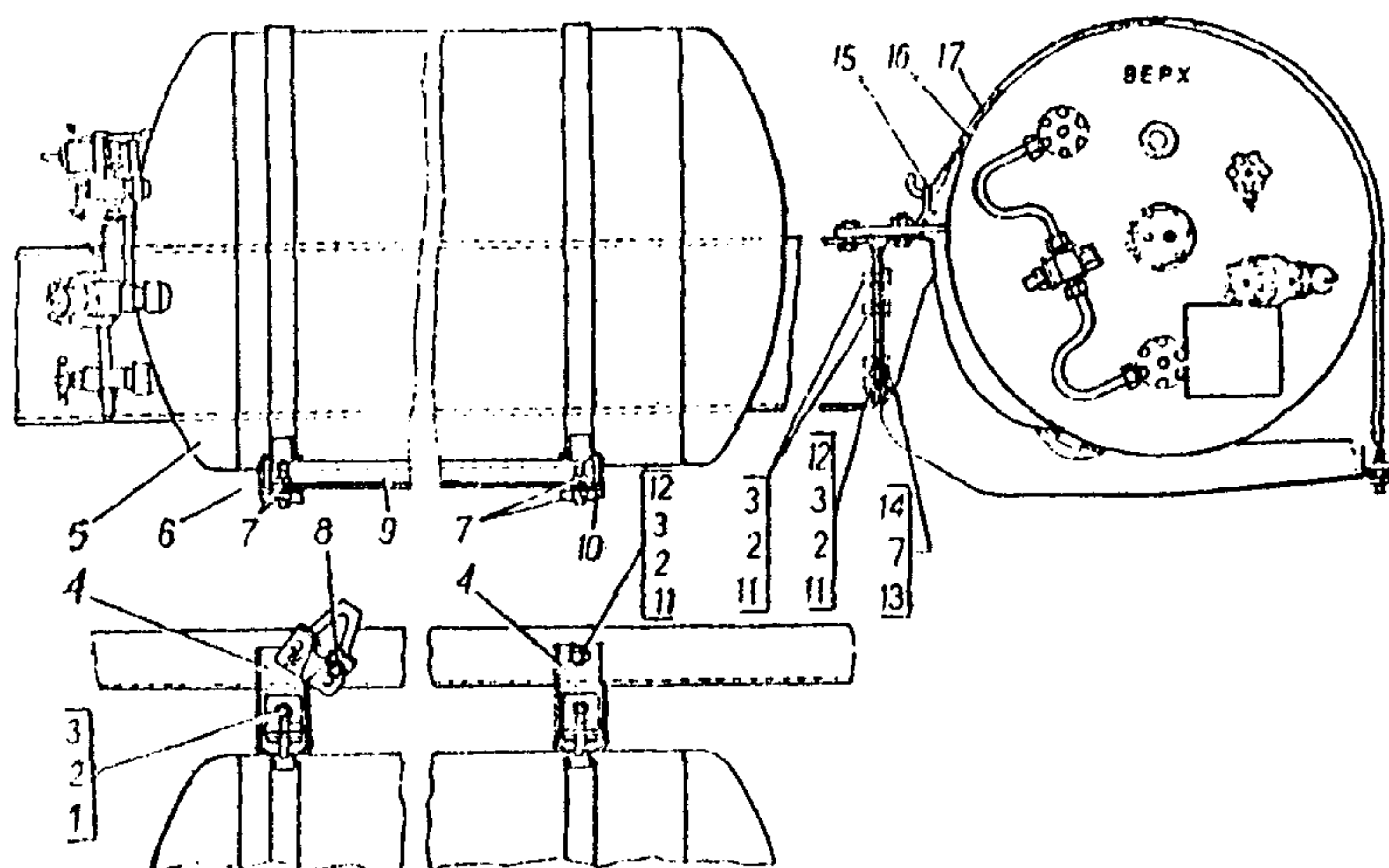
Рис. 5.35. Установка баллона на автомобиль ГАЗ-52-07
