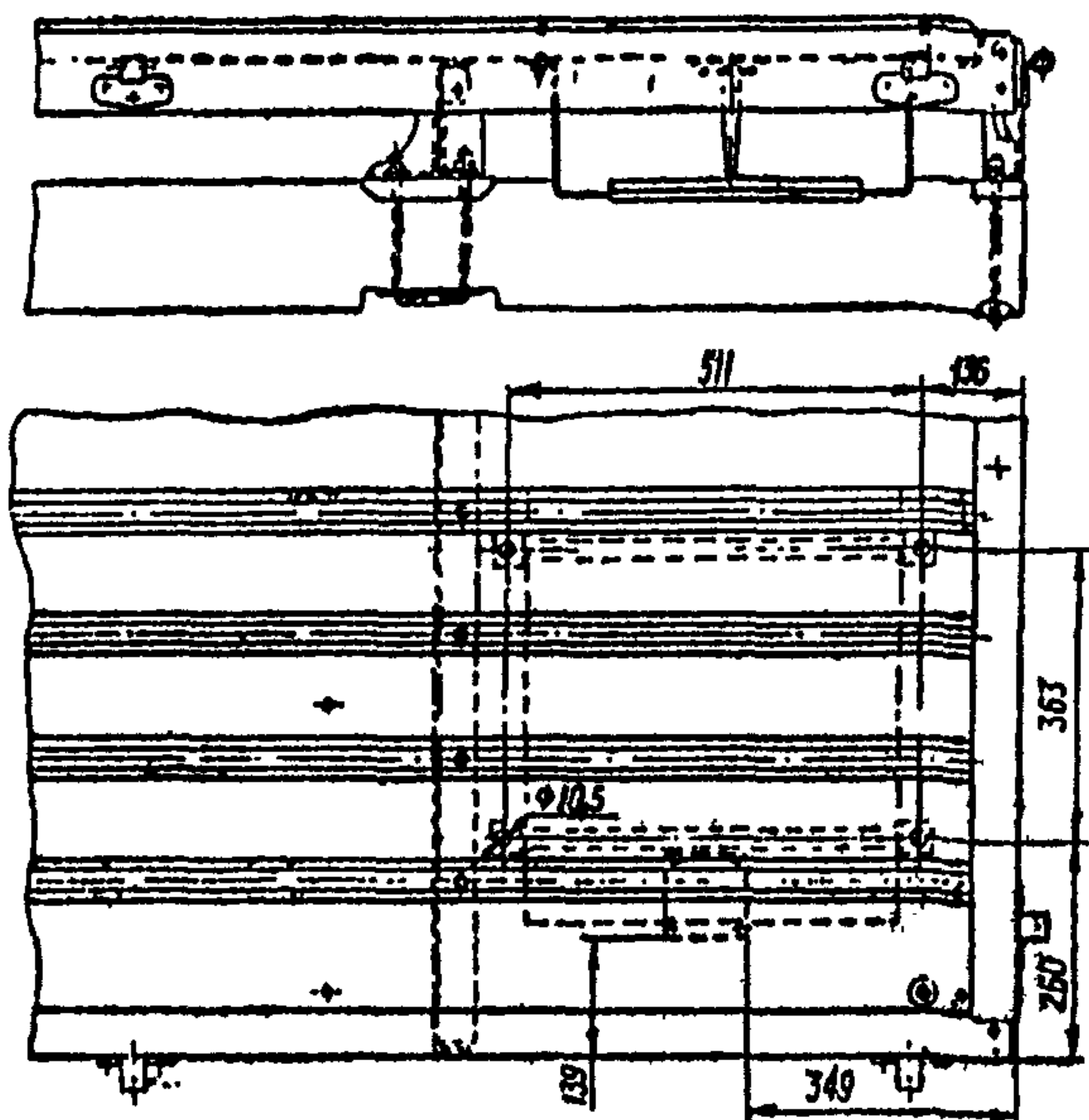
Рис. 5.44. Установка инструментального ящика на автомобилях ГАЗ-53-07 и ГАЗ-52-08
