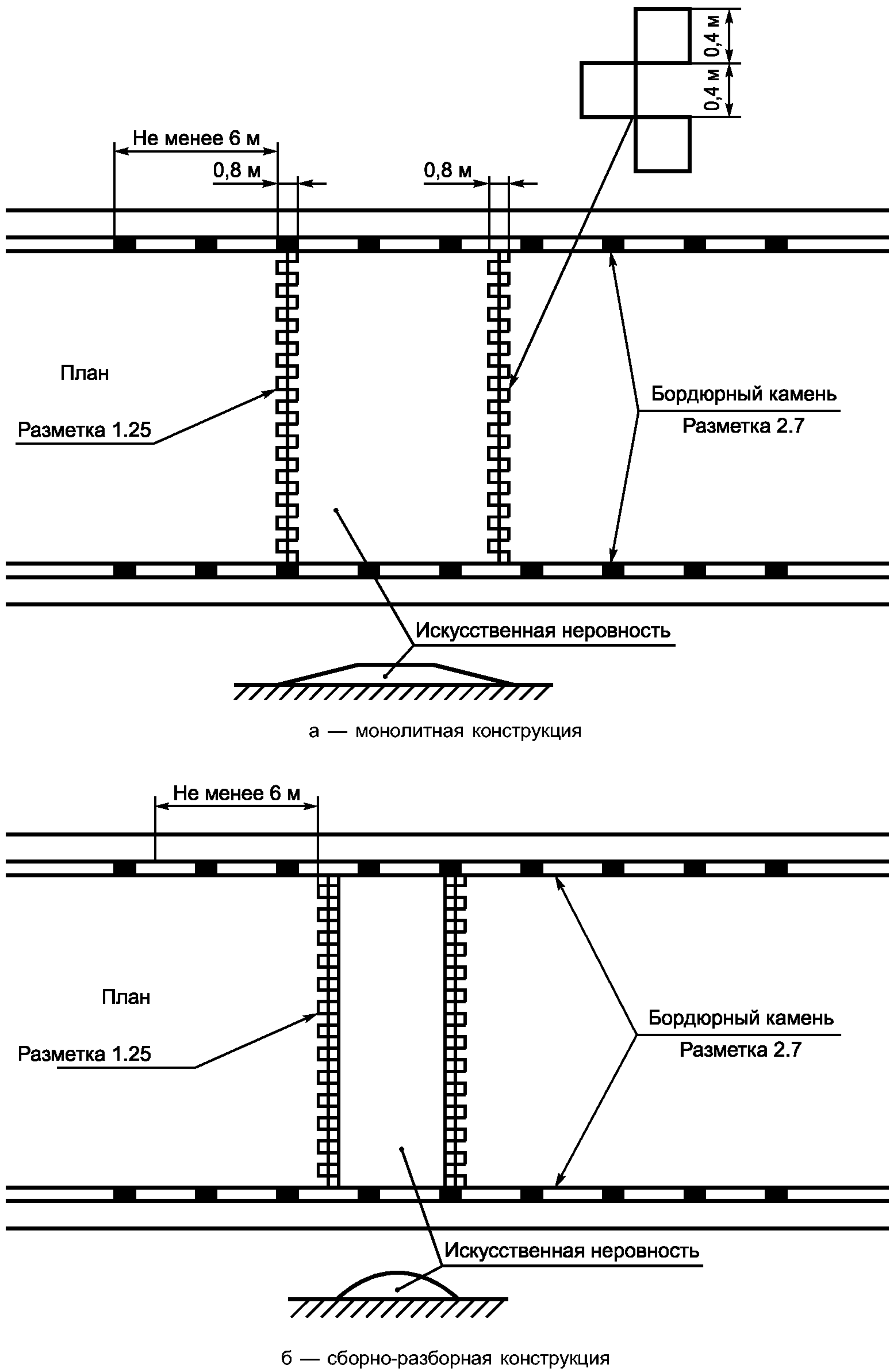
Рисунок 4 — Пример нанесения разметки 1.25 и 2.7 при устройстве ИН
