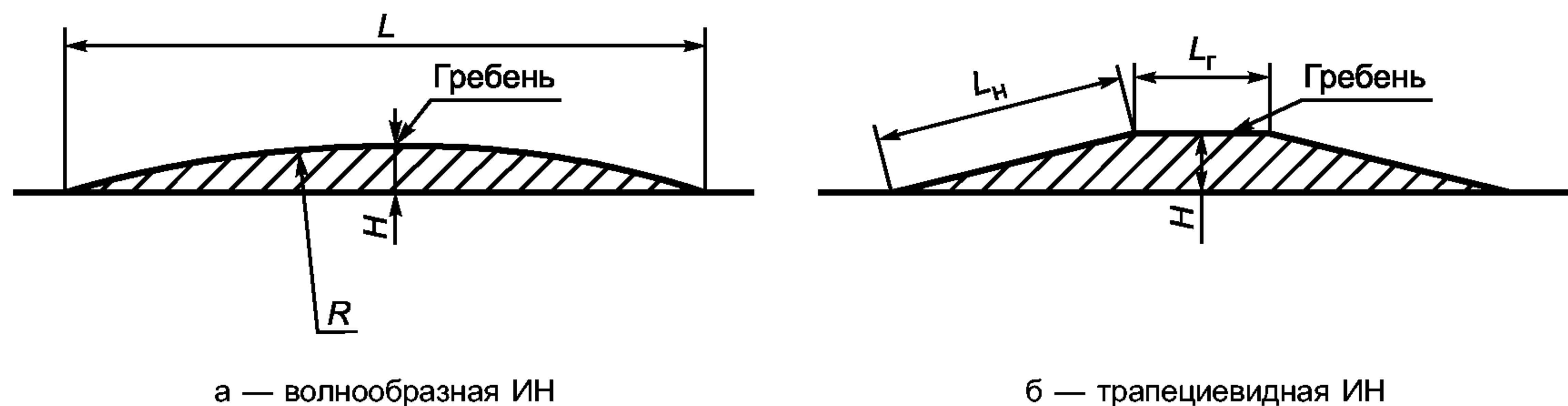
Рисунок 1 — Поперечные профили ИН
