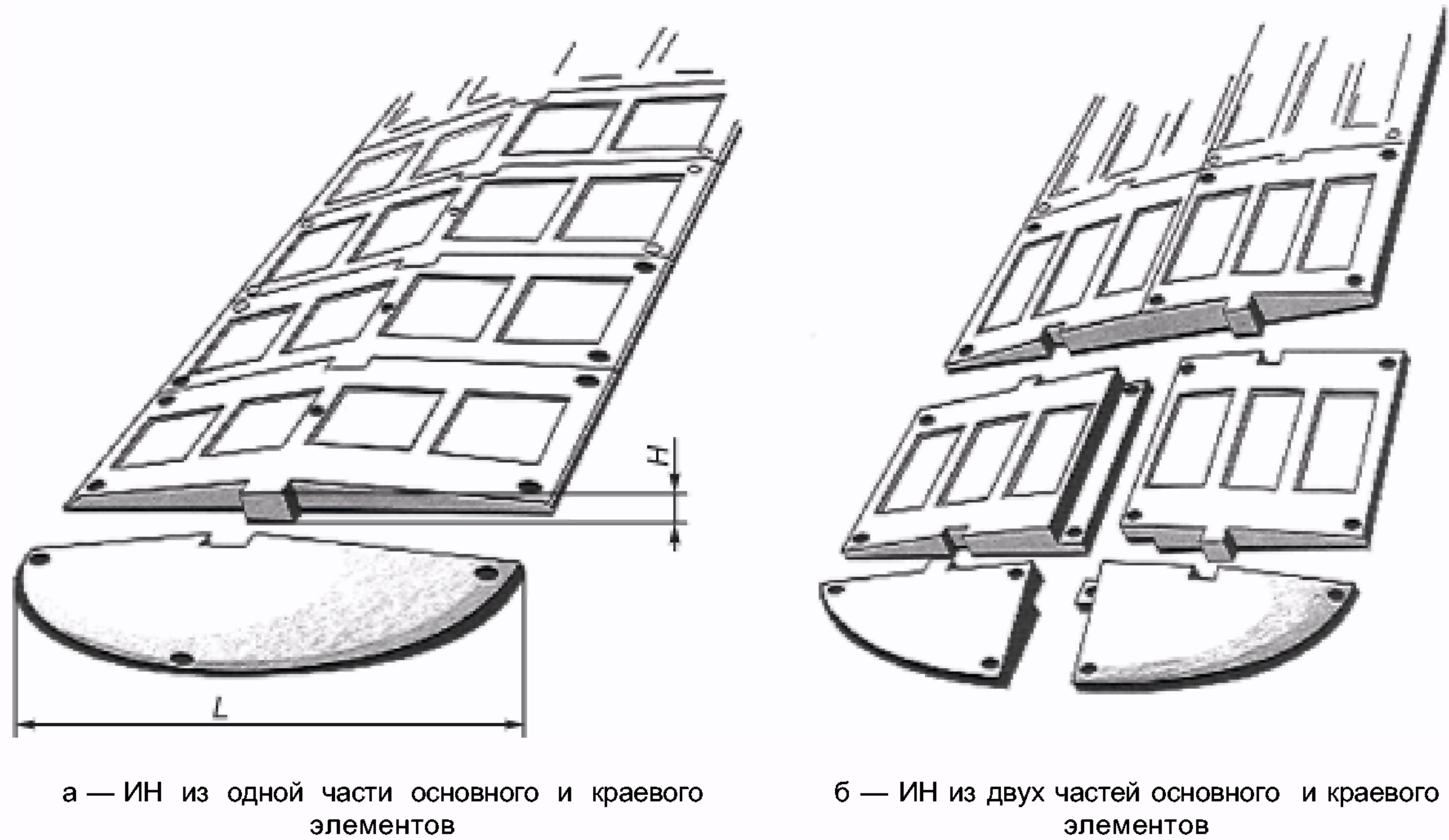
Рисунок 3 — Конструкция сборно-разборной ИН
