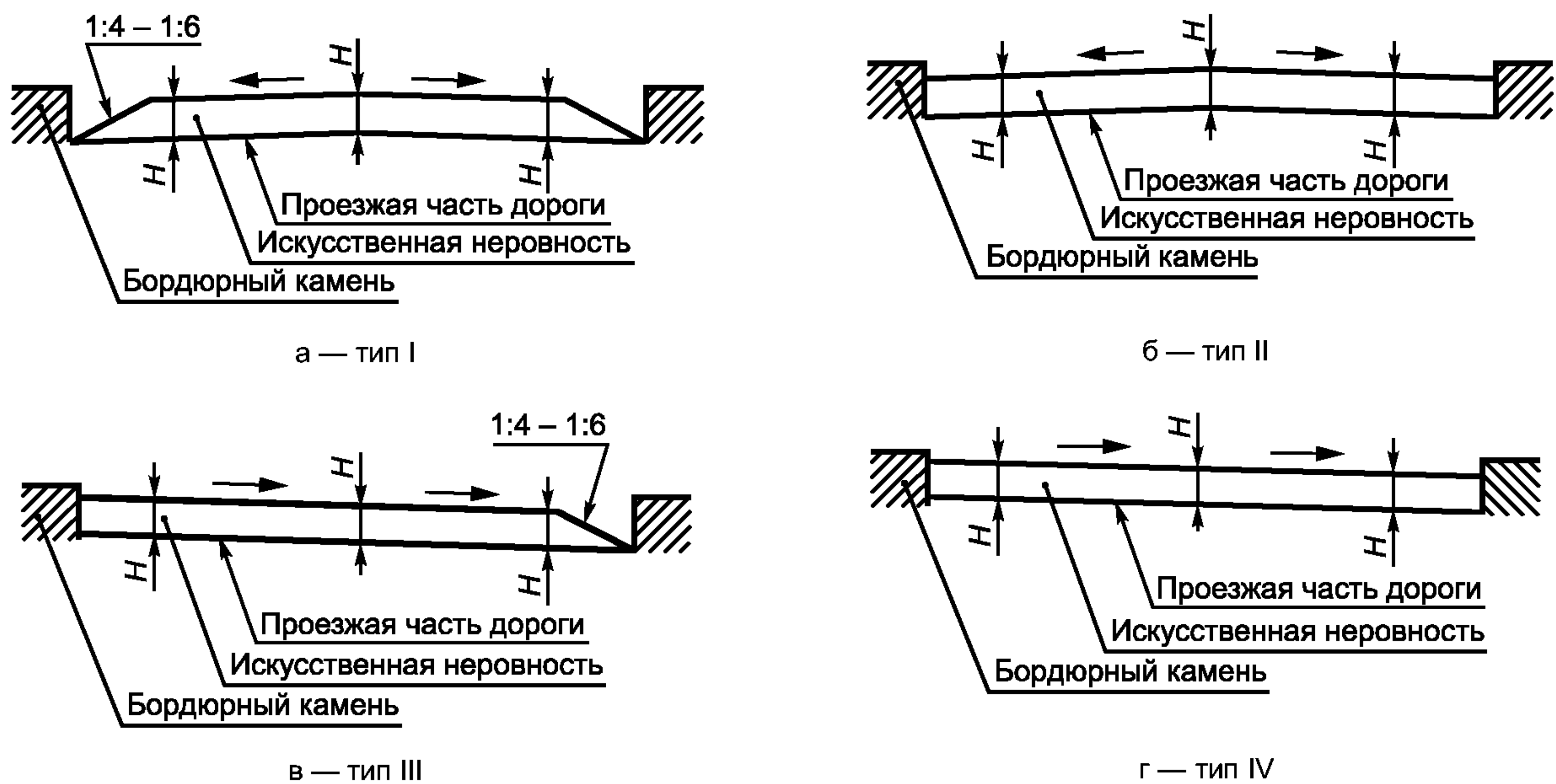
Рисунок 2 — Продольные профили ИН
