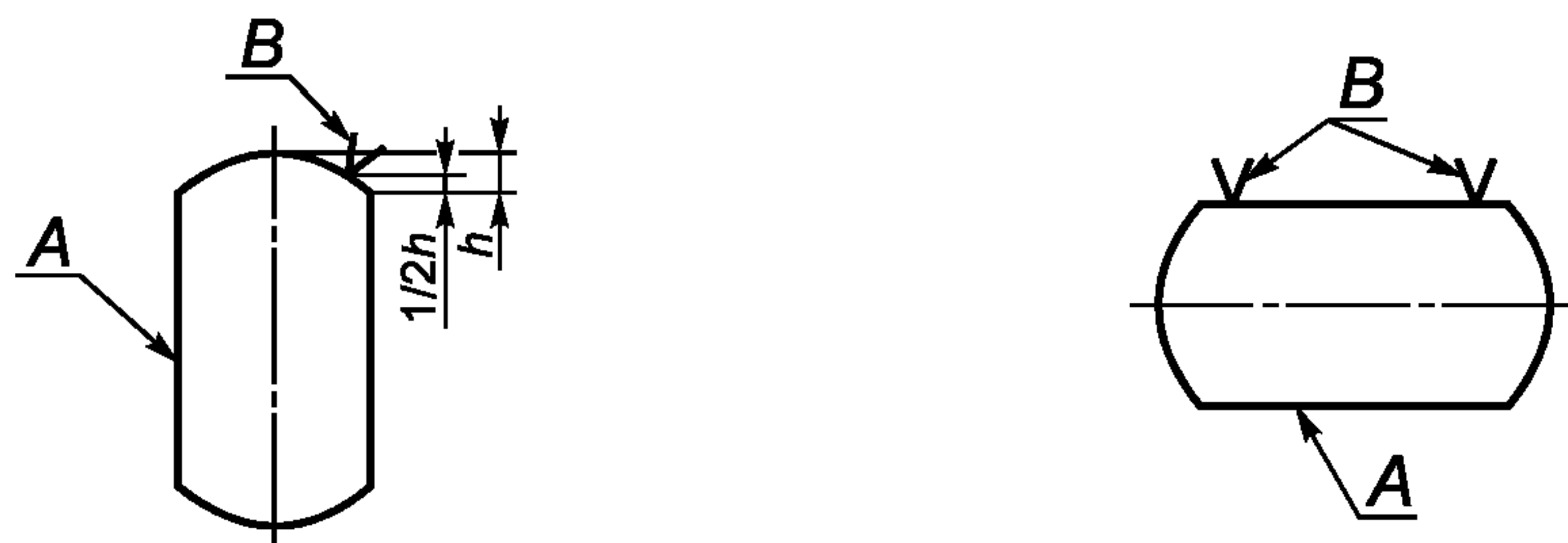
а — Положение термодпар для металлических баков
