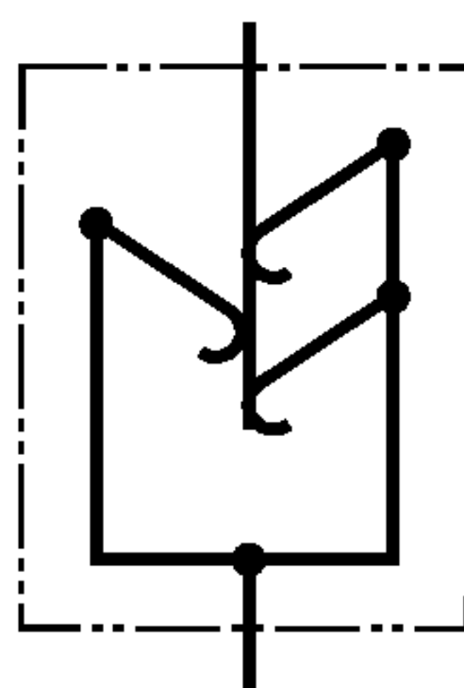
Рисунок 5b — Три соединительных элемента, не являющихся независимыми
