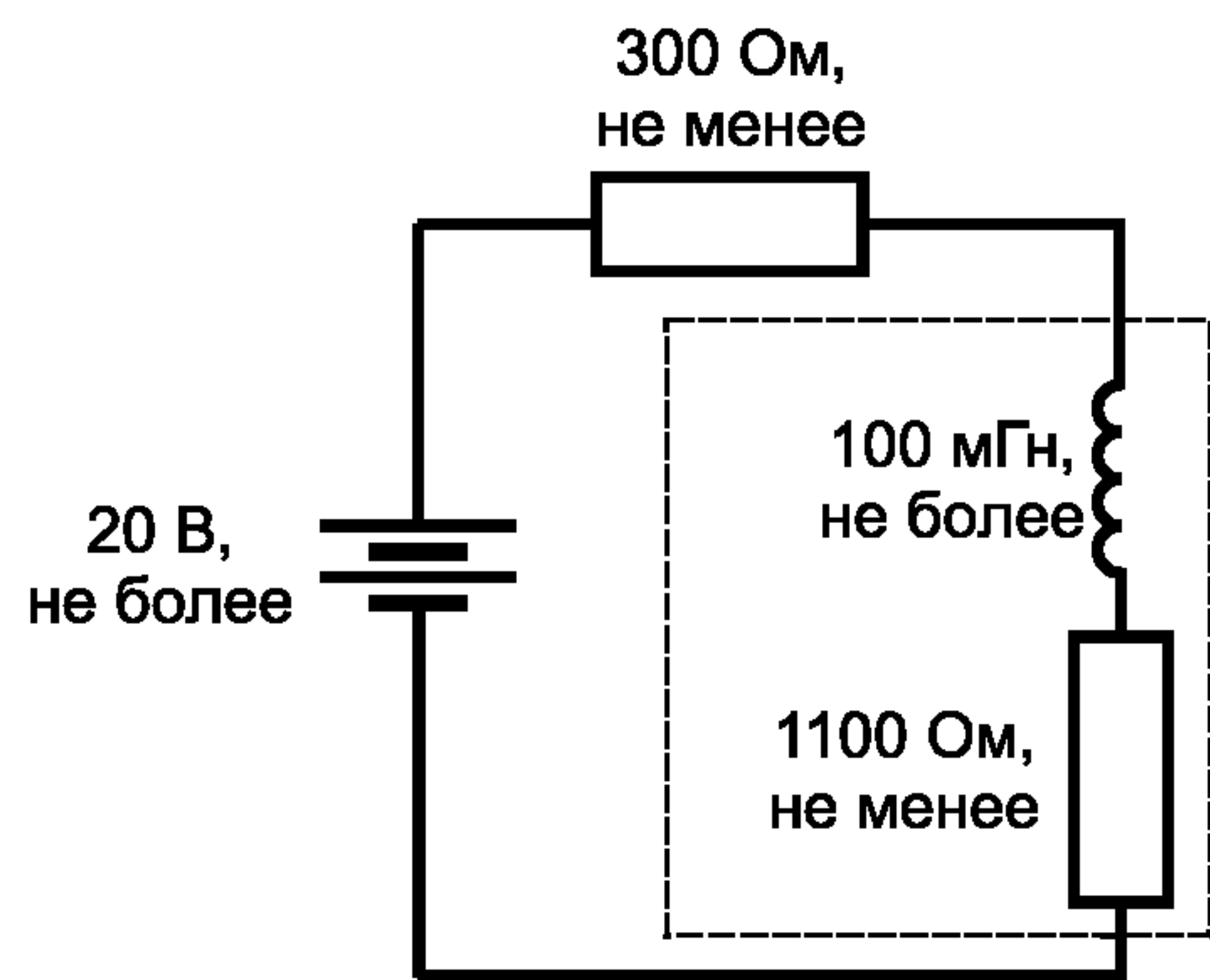
Рисунок А.7 — Простая индуктивная цепь
