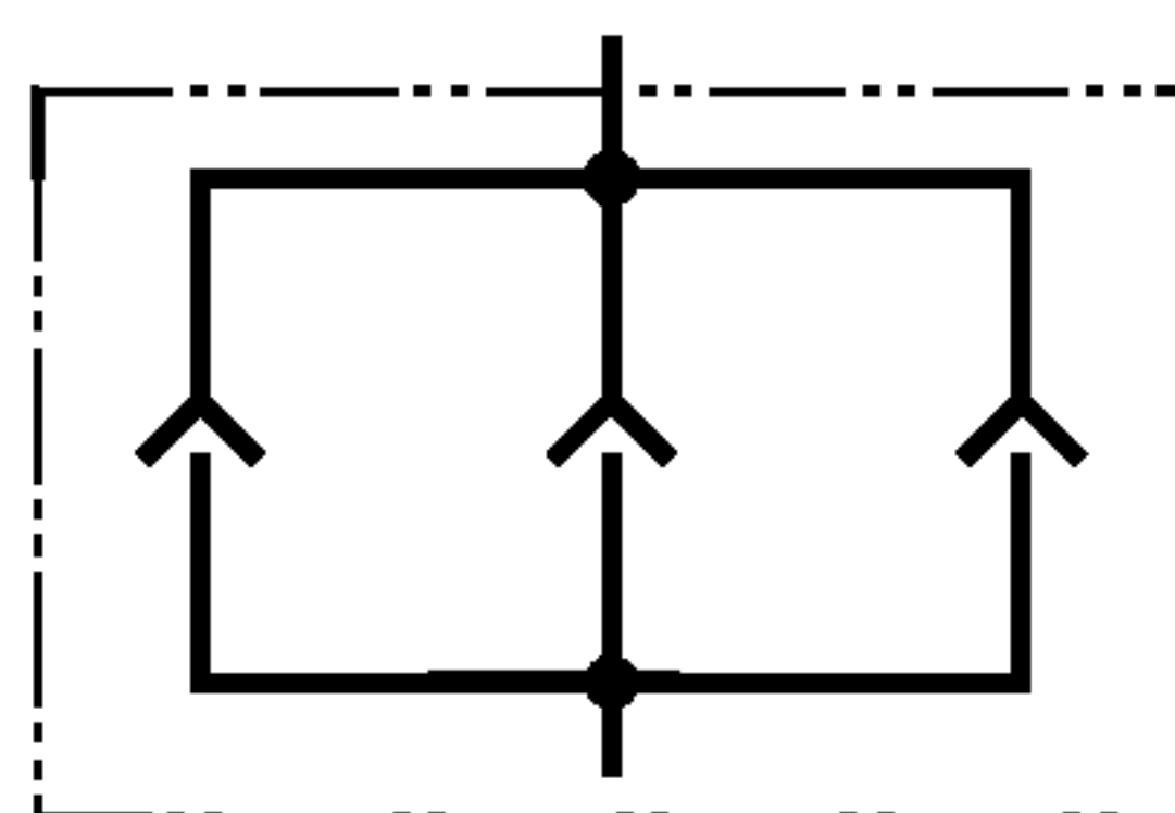
Рисунок 5а — Три независимых соединительных элемента
