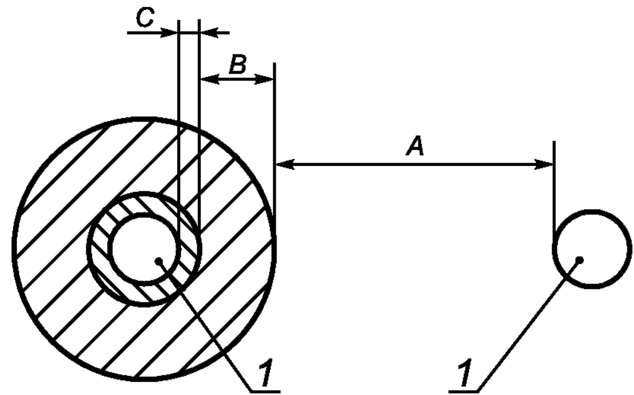
Рисунок С.2 — Измерение сложных расстояний
