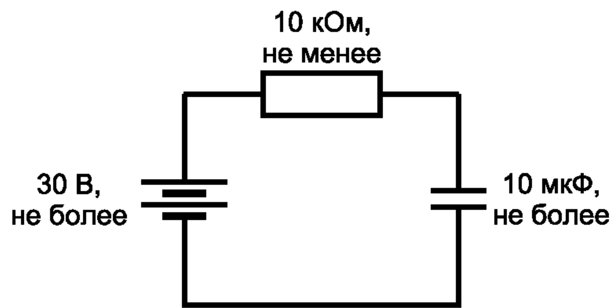
Рисунок А.8 — Простая емкостная цепь
