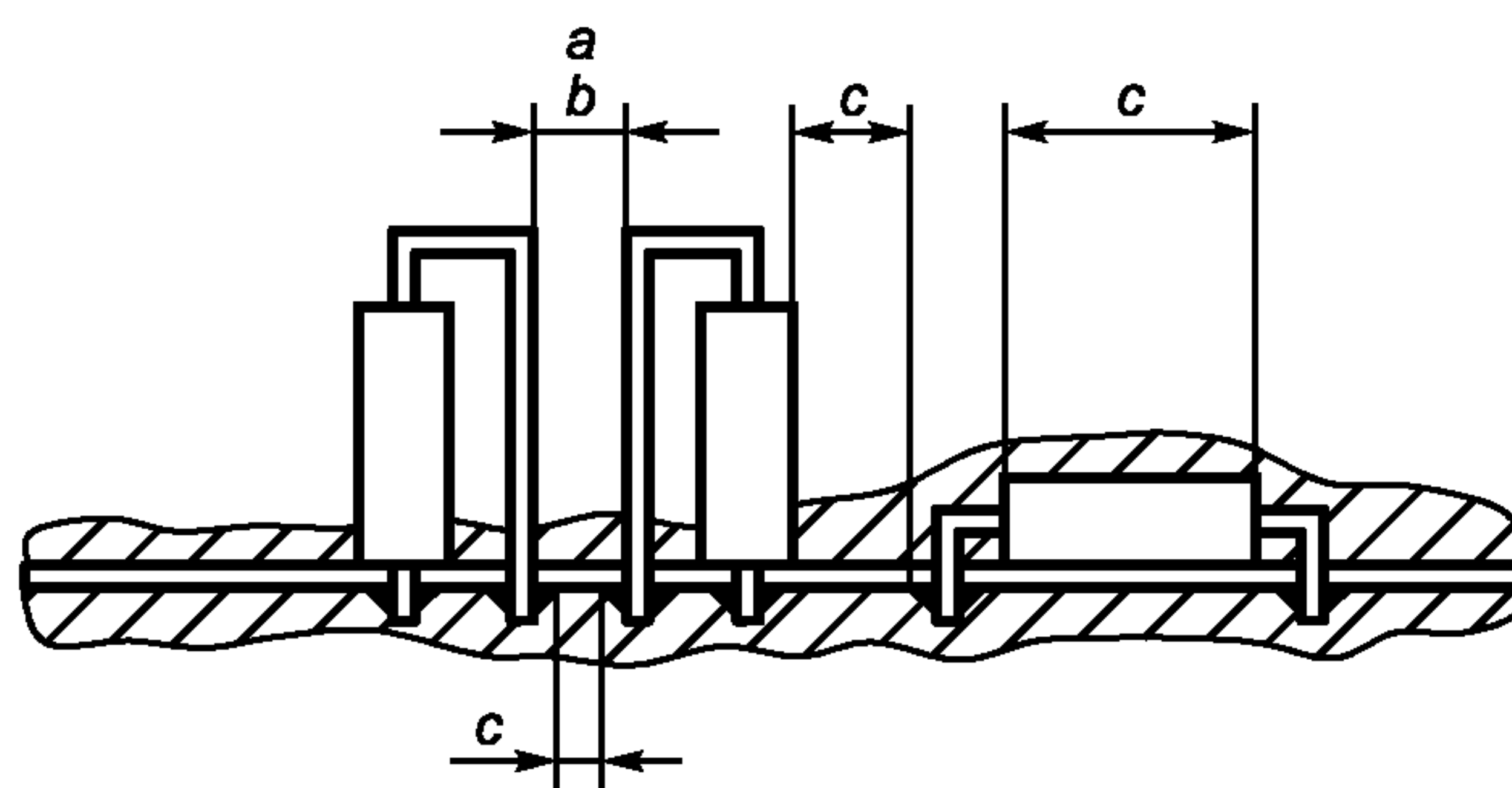
Рисунок в) — Плата с пайкой обрезанных или подогнутых выводов резисторов
