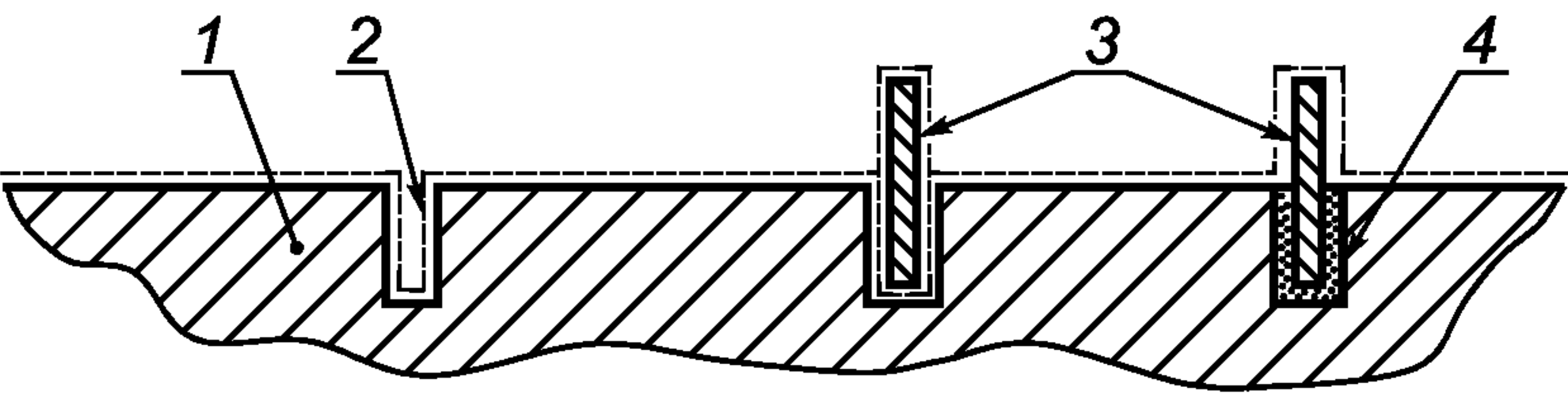
1 — подложка; 2 — бороздка; 3 — перегородка; 4 — клей
