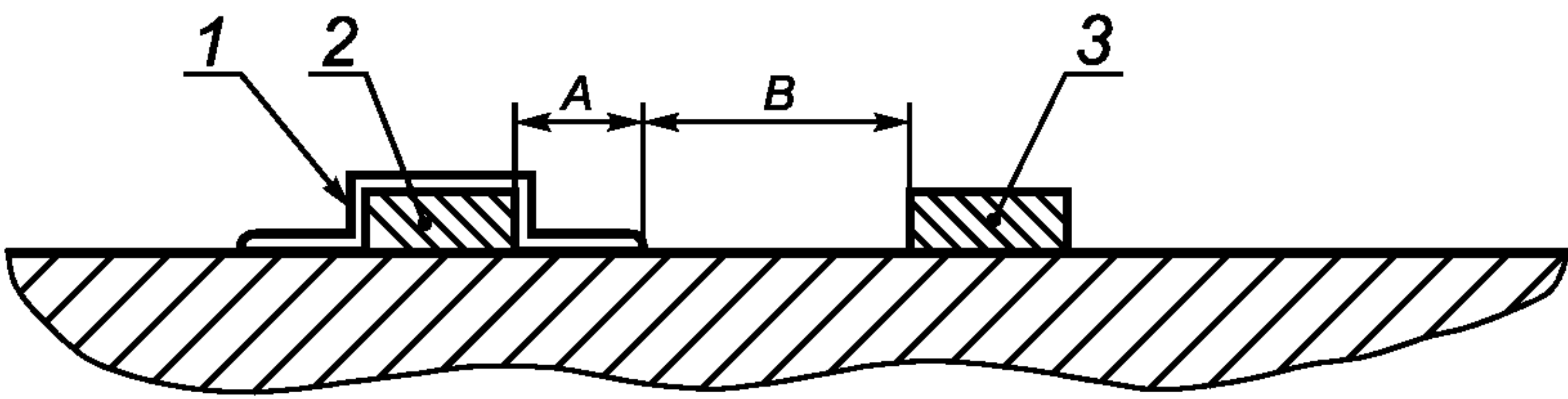
1 — лак; 2 — проводник; 3 — подложка
