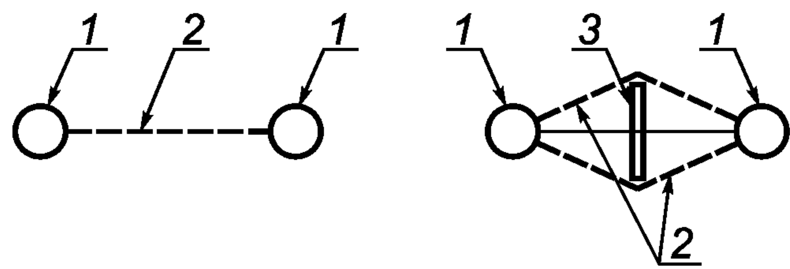
Рисунок С.1 — Измерение зазора
