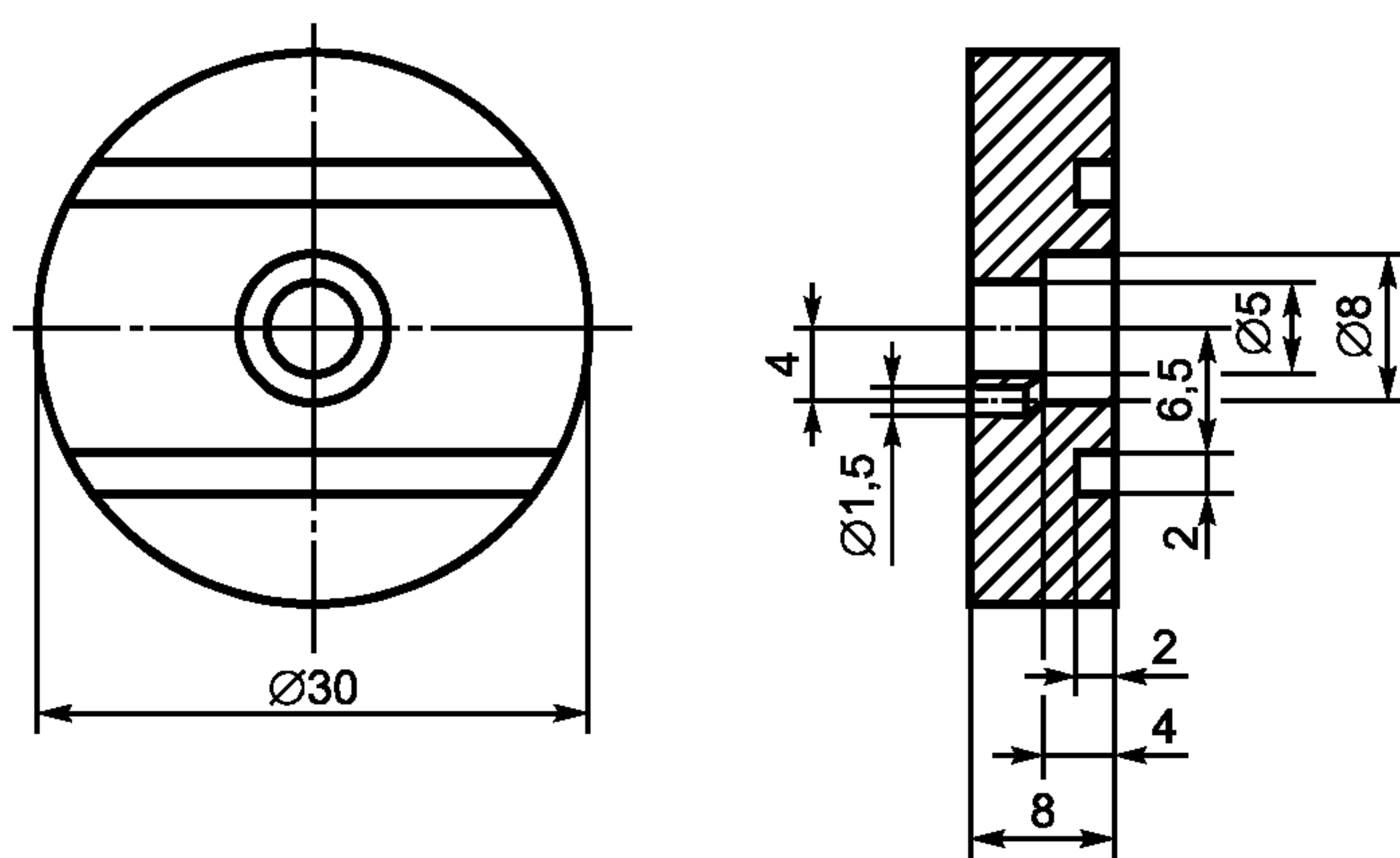
Рисунок В.2 — Кадмиевый контактный диск
