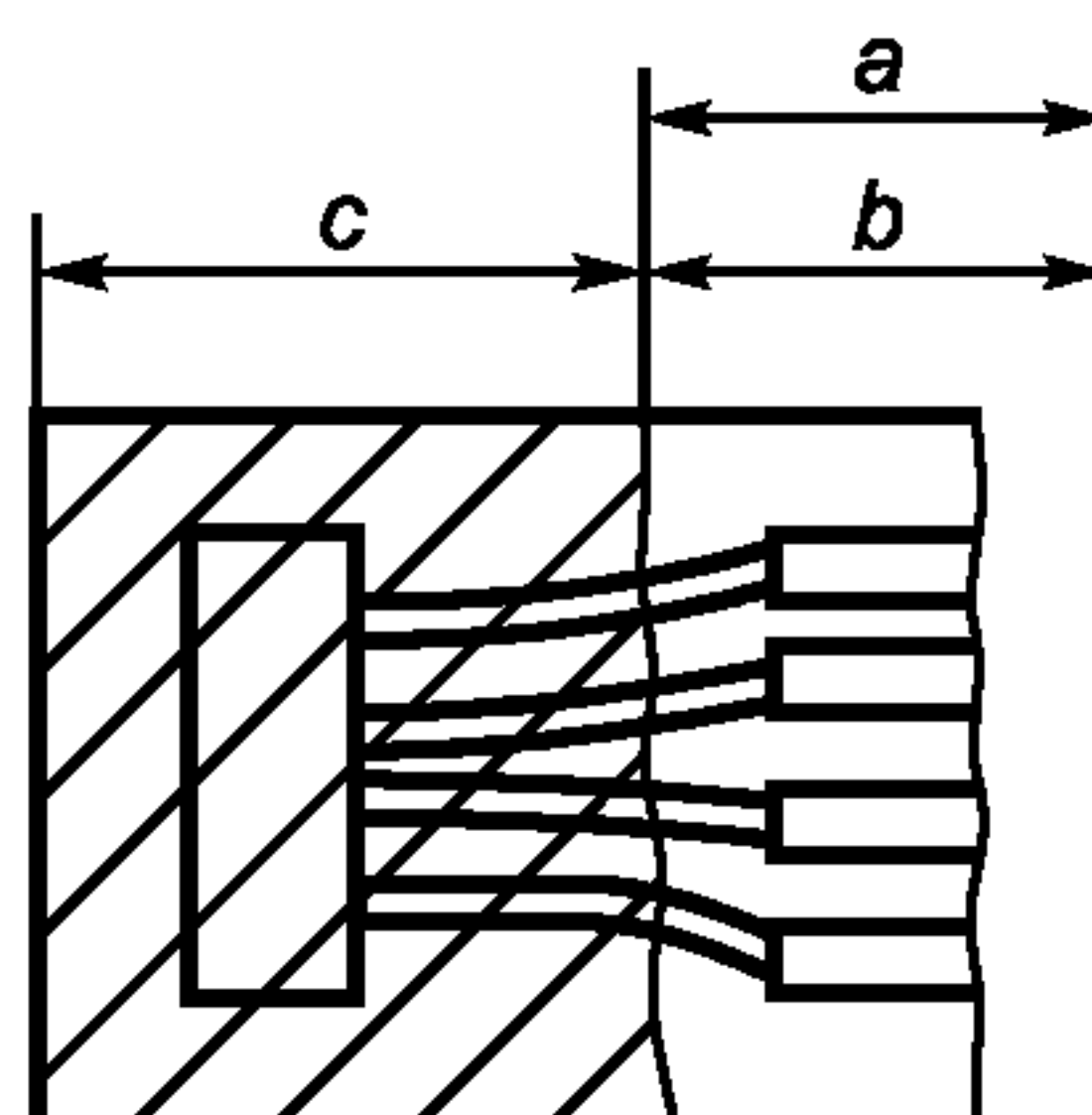
Рисунок а) — Плата с частичным покрытием
