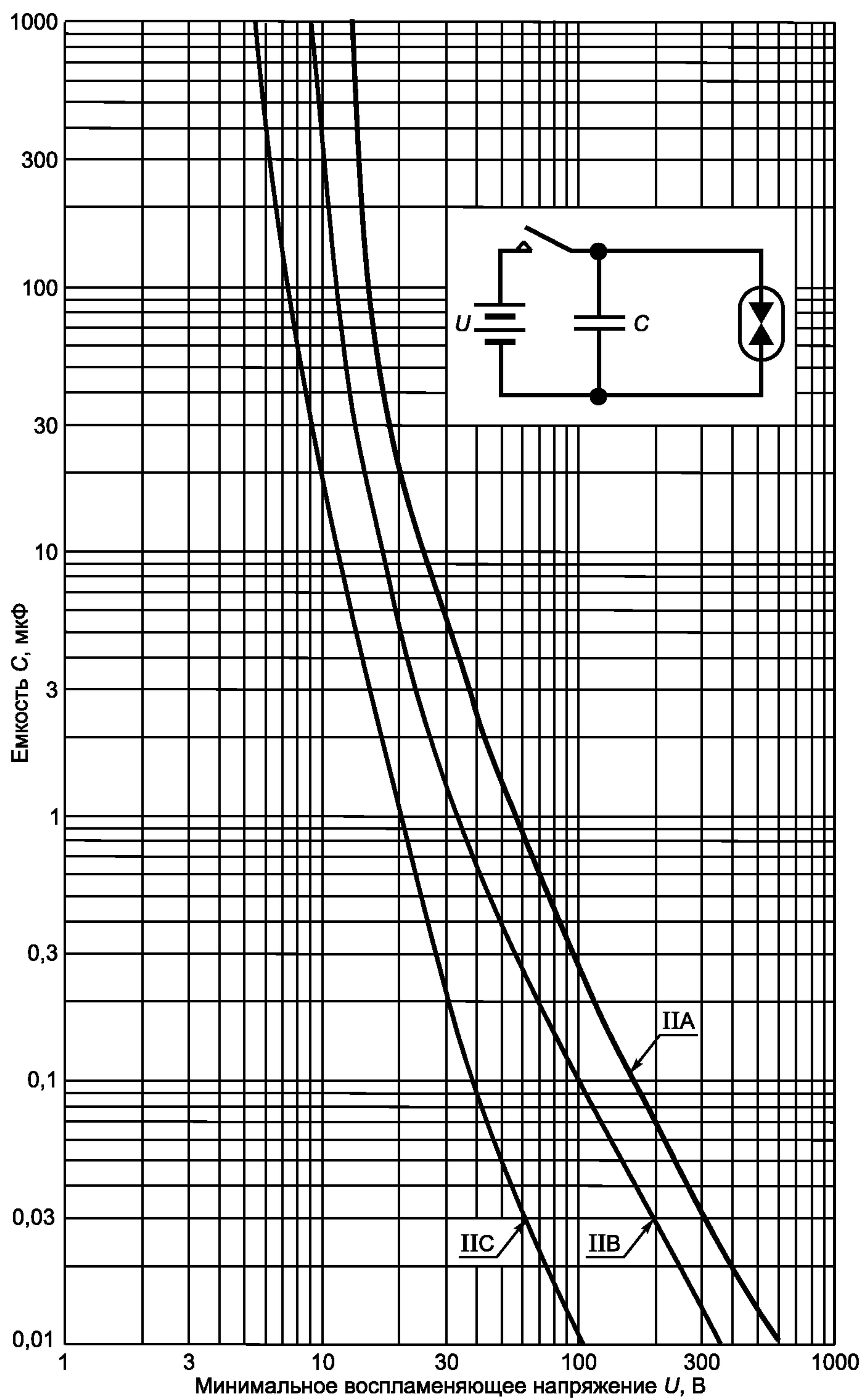
Рисунок А.3 — Емкостные цепи группы II
