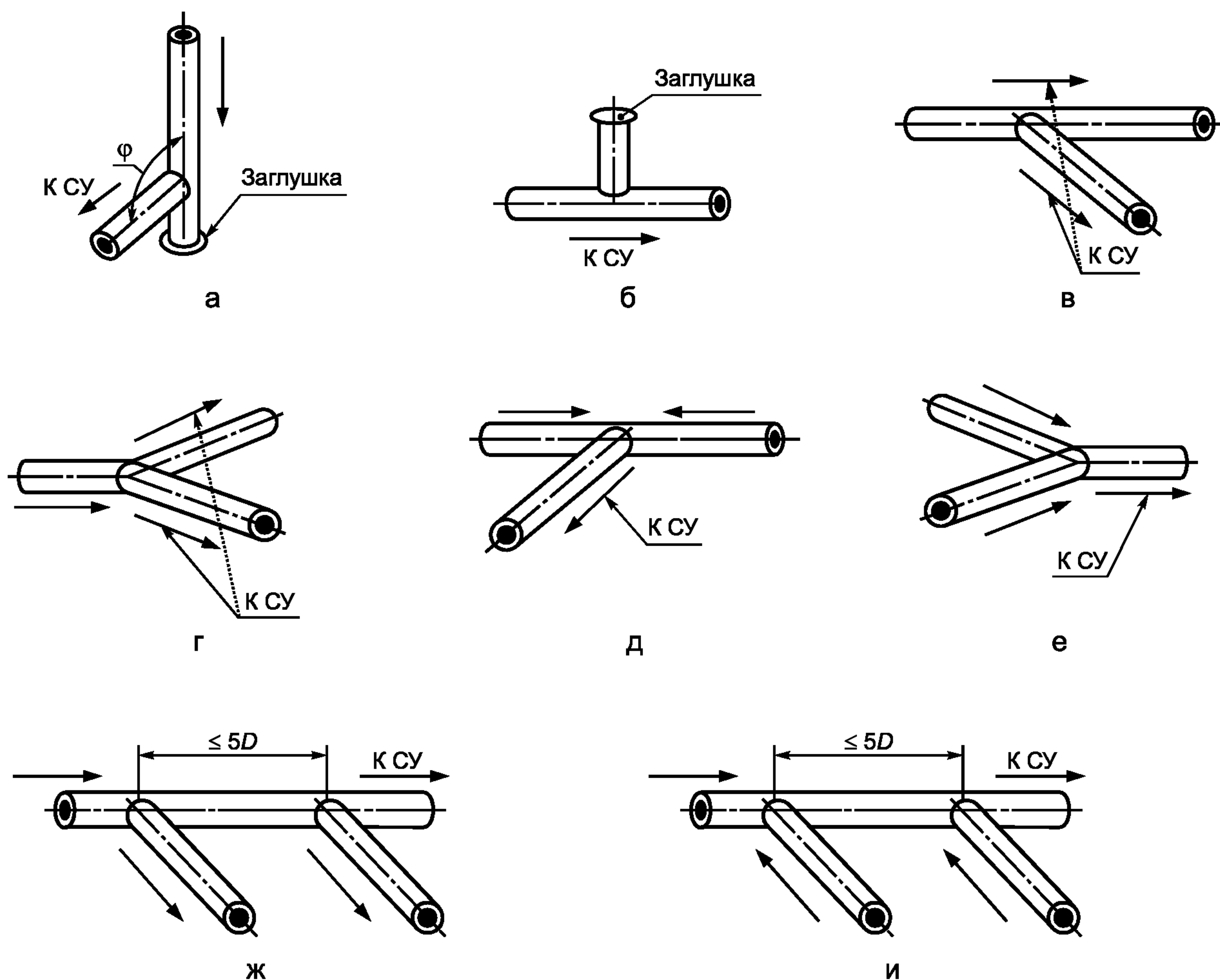
Рисунок А.2 — Тройники
