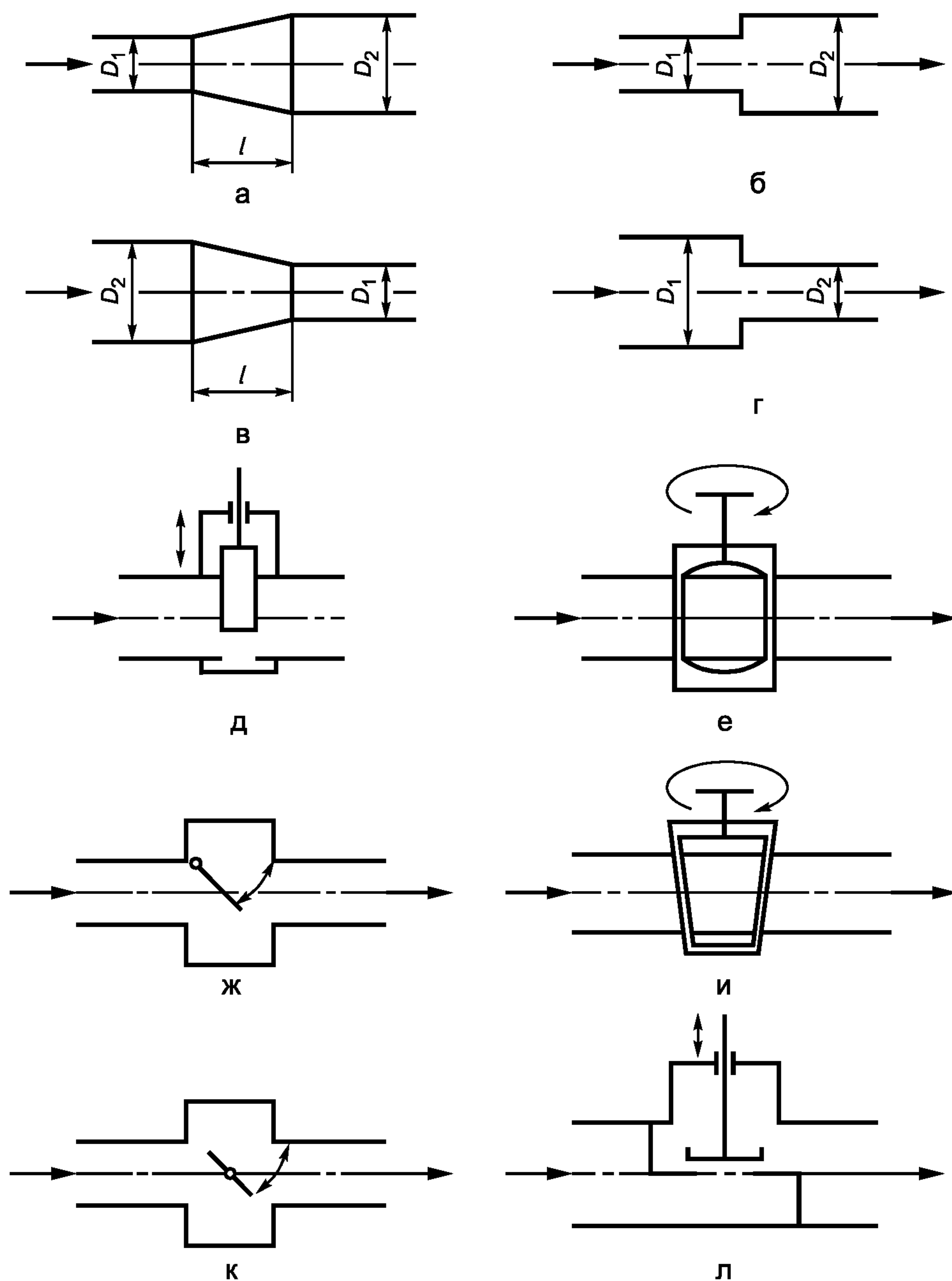
Рисунок А.3 — Переходные участки и запорная арматура
