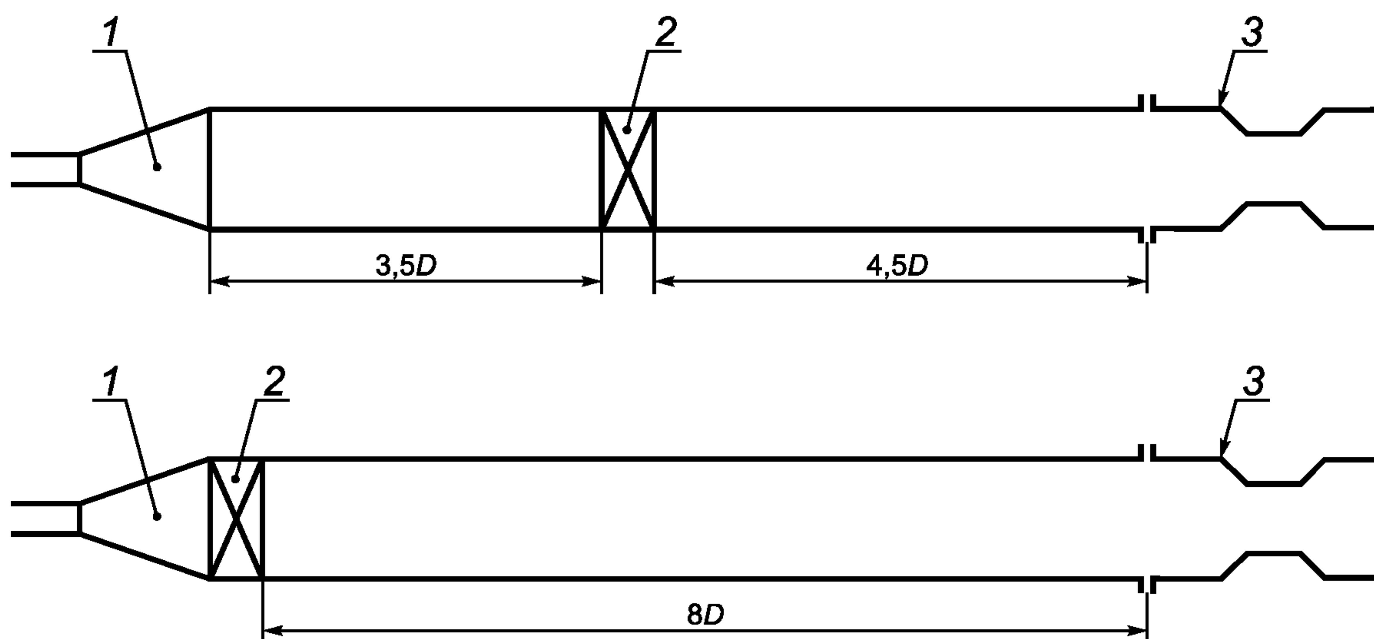
1 — диффузор; 2 — шаровой кран или задвижка; 3 — труба Вентури
