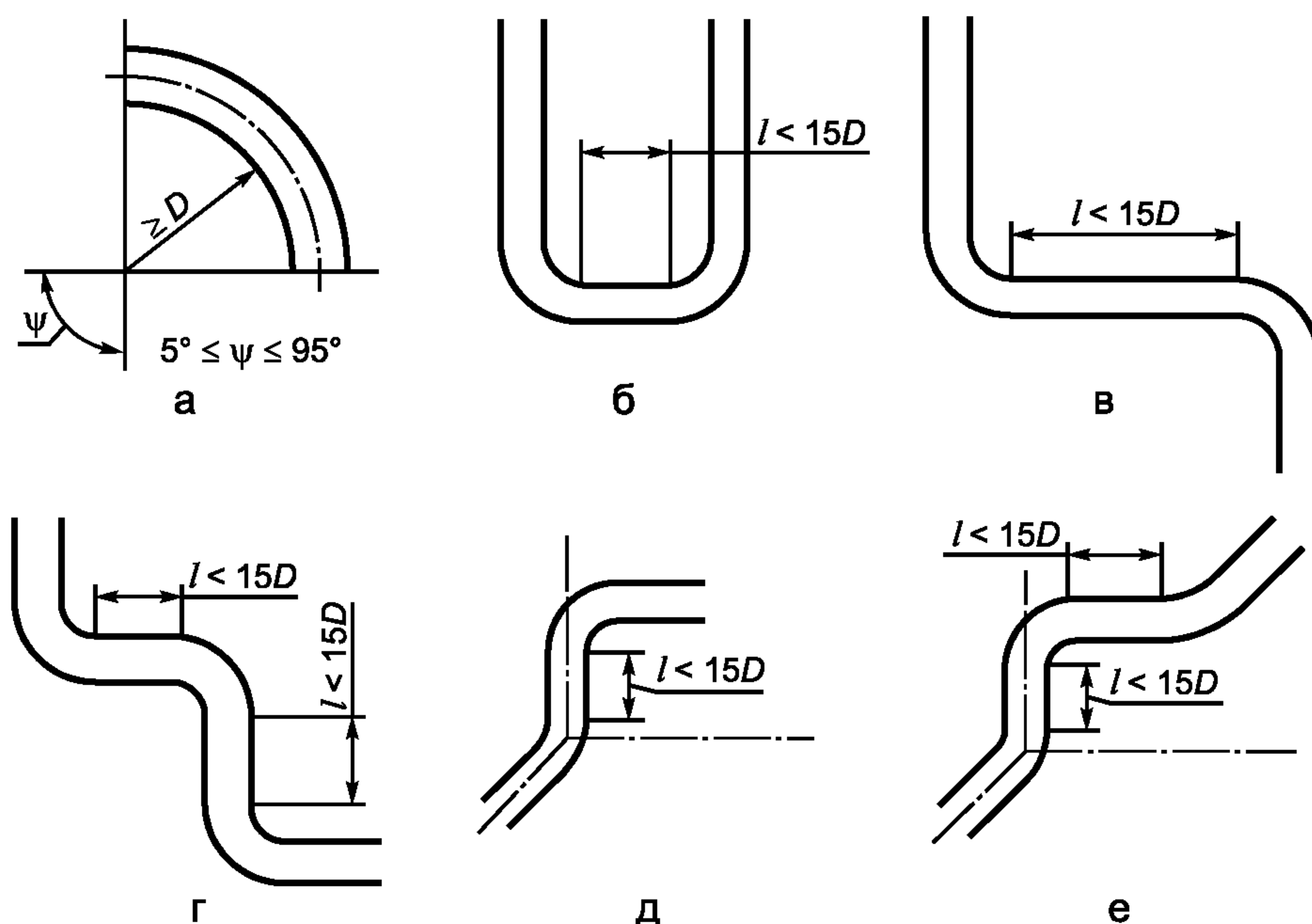
Рисунок А.1 — Колено и группы колен
