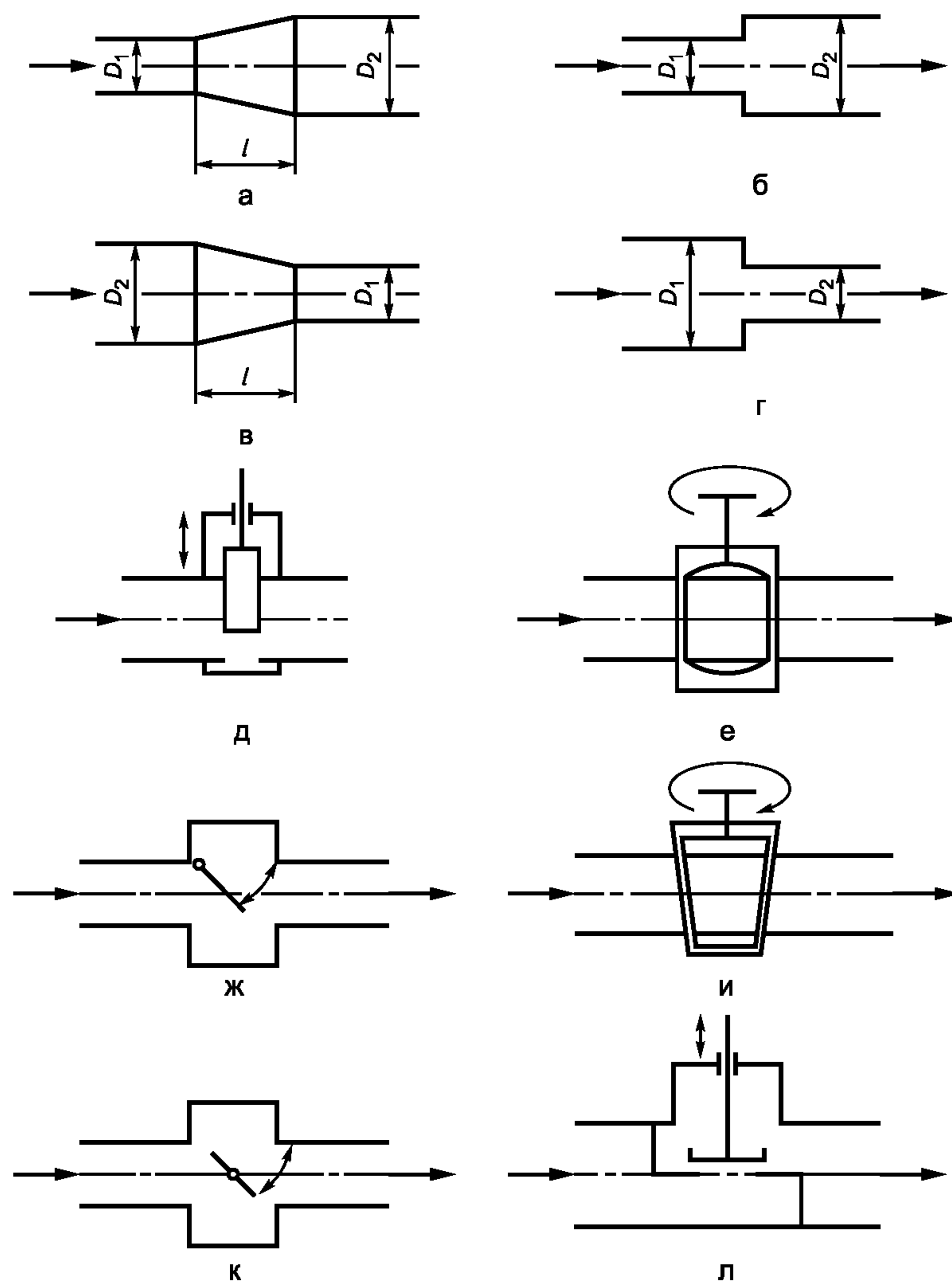
Рисунок А.3 — Переходные участки и запорная арматура
