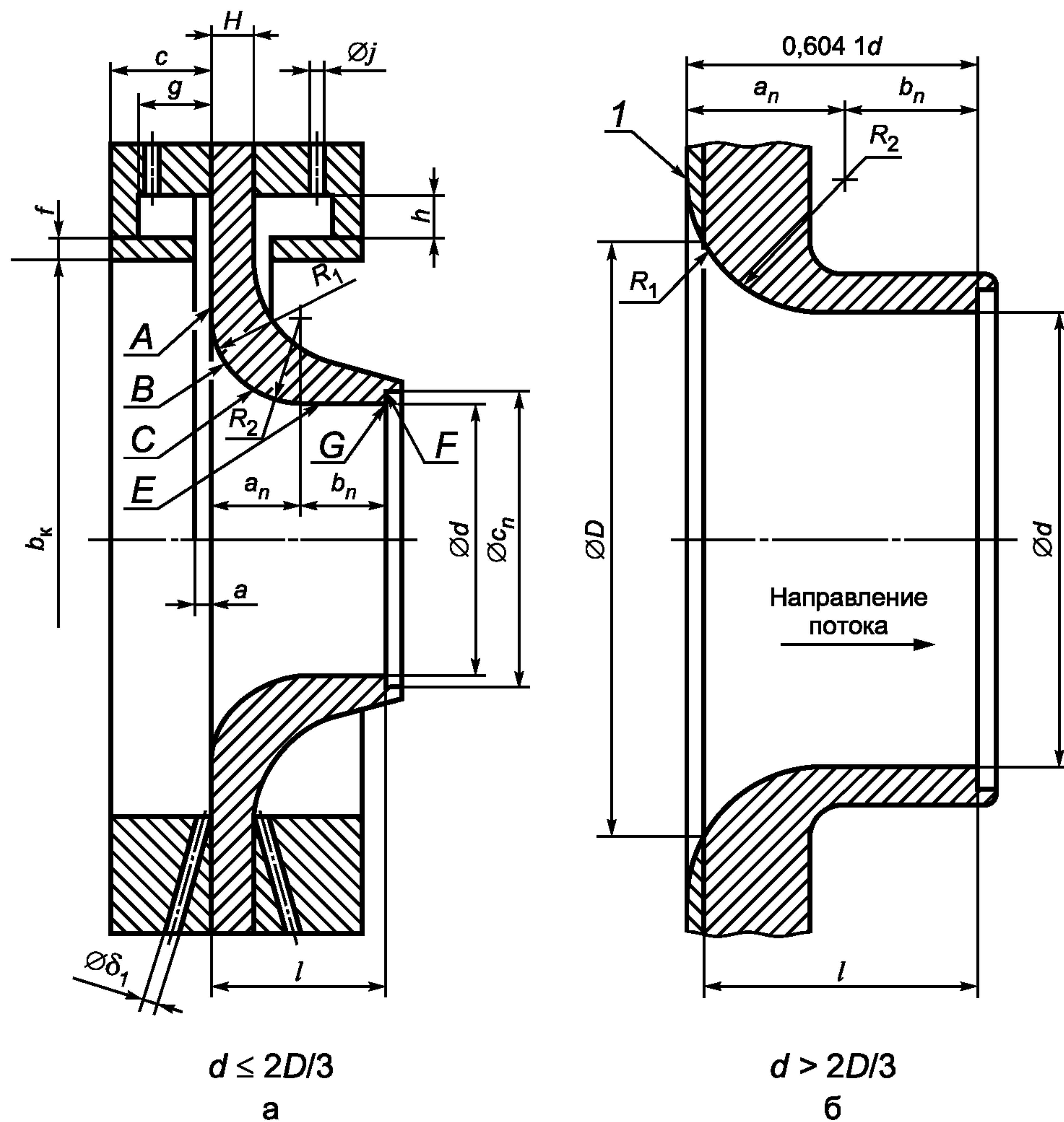
Рисунок 1 — Сопло ИСА 1932
