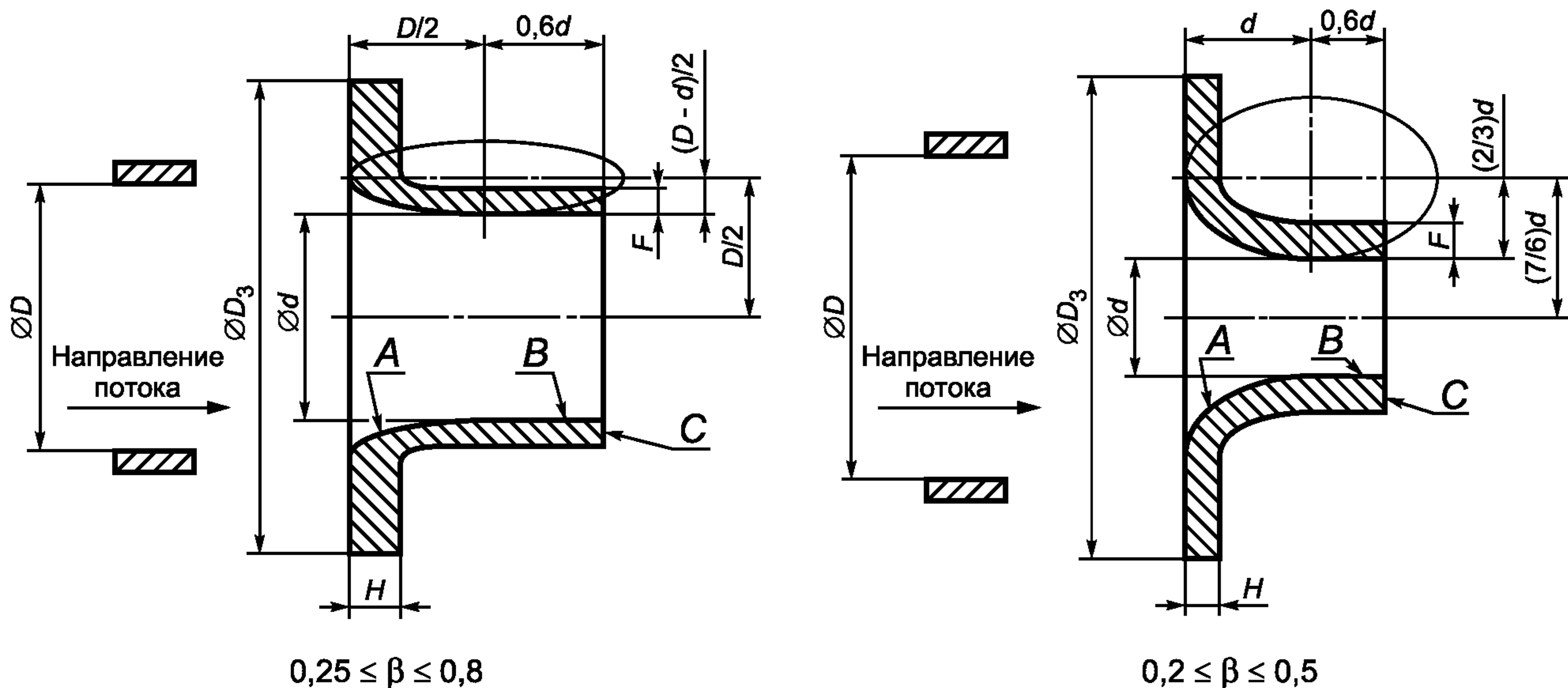
Рисунок 2 — Эллипсное сопло
