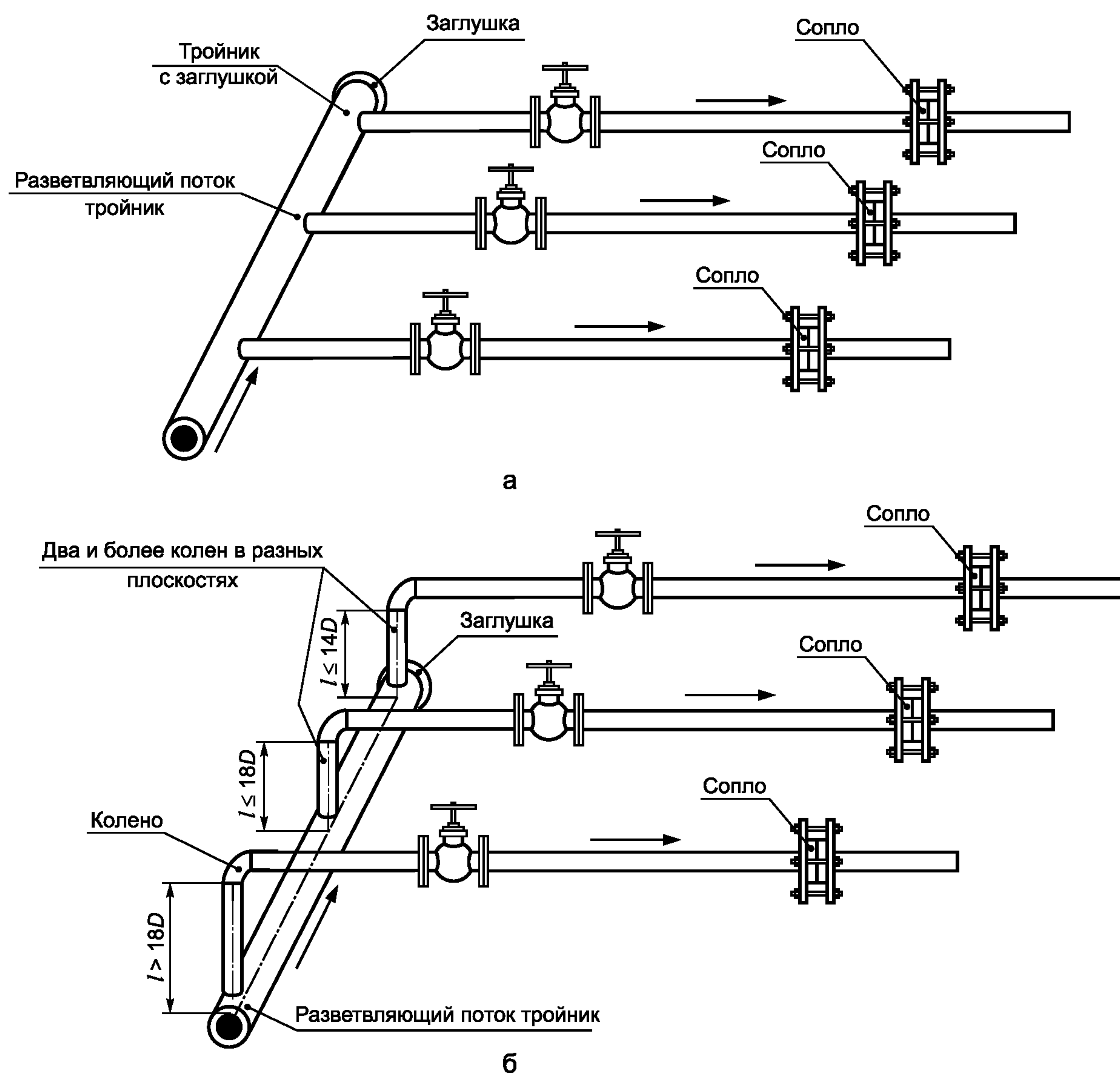
Рисунок 5 — Схемы коллектора
