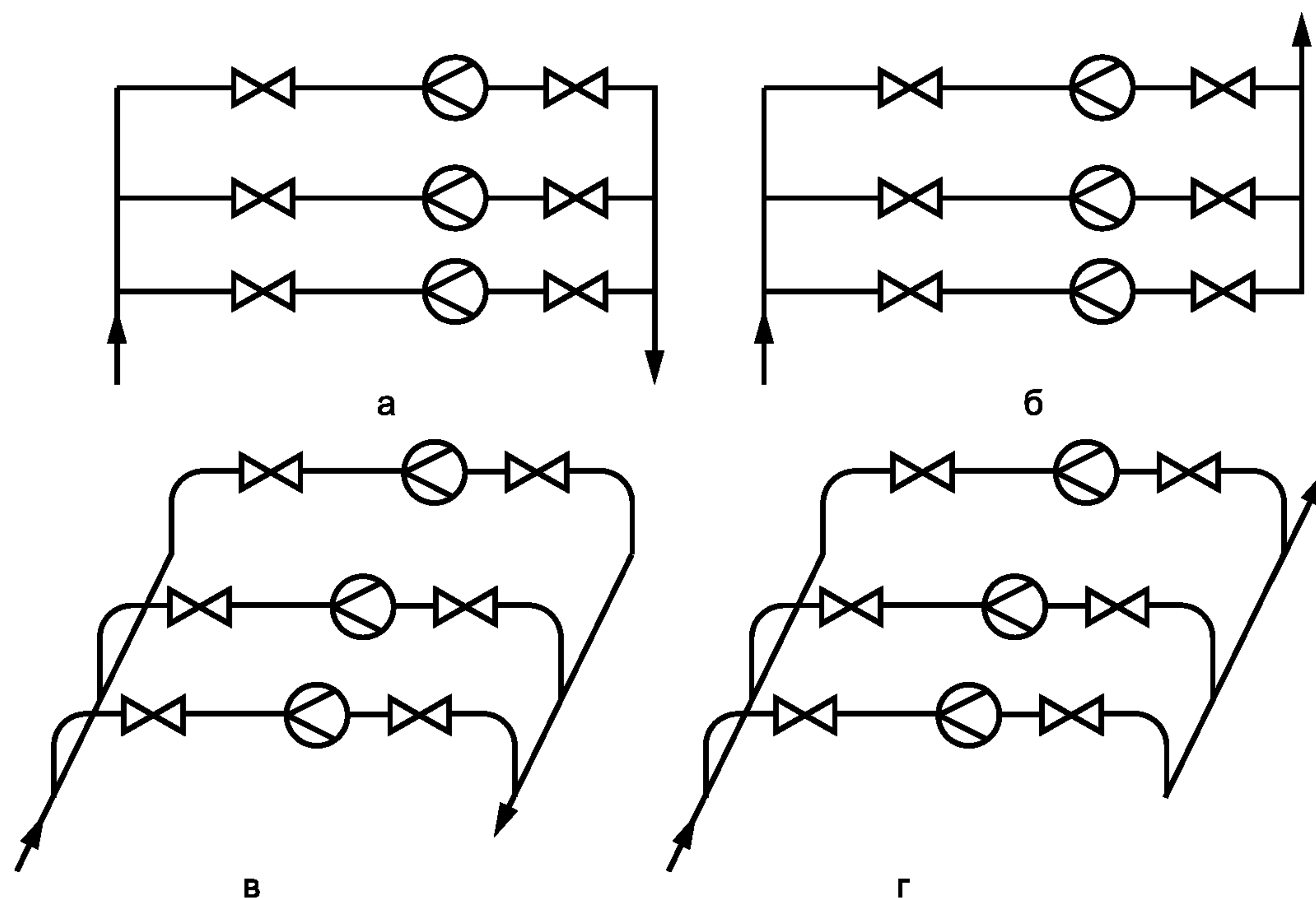
Рисунок А.4 — Схемы коллекторных систем
