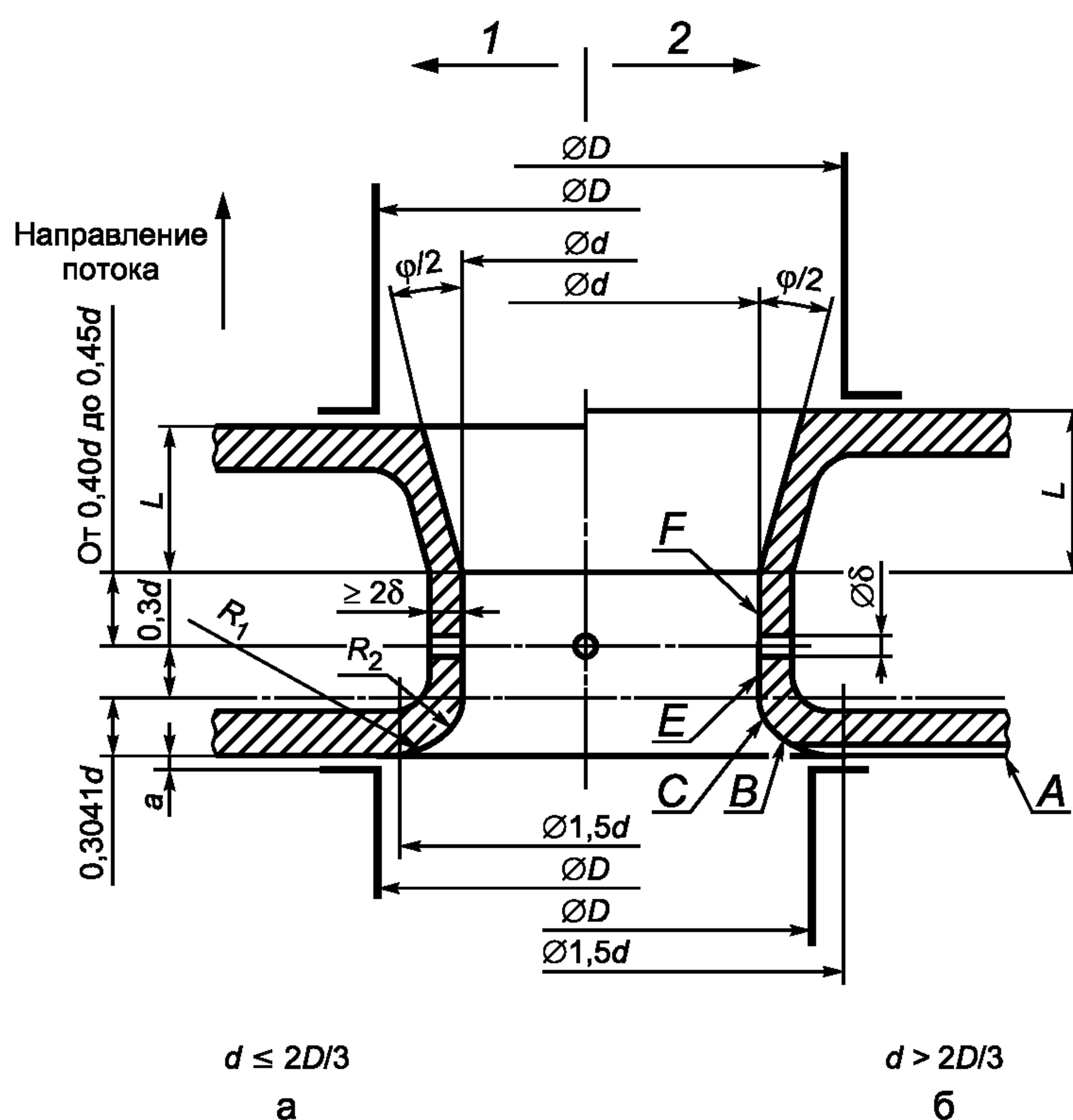
1 — укороченное сопло Вентури; 2 — неукороченное сопло Вентури
