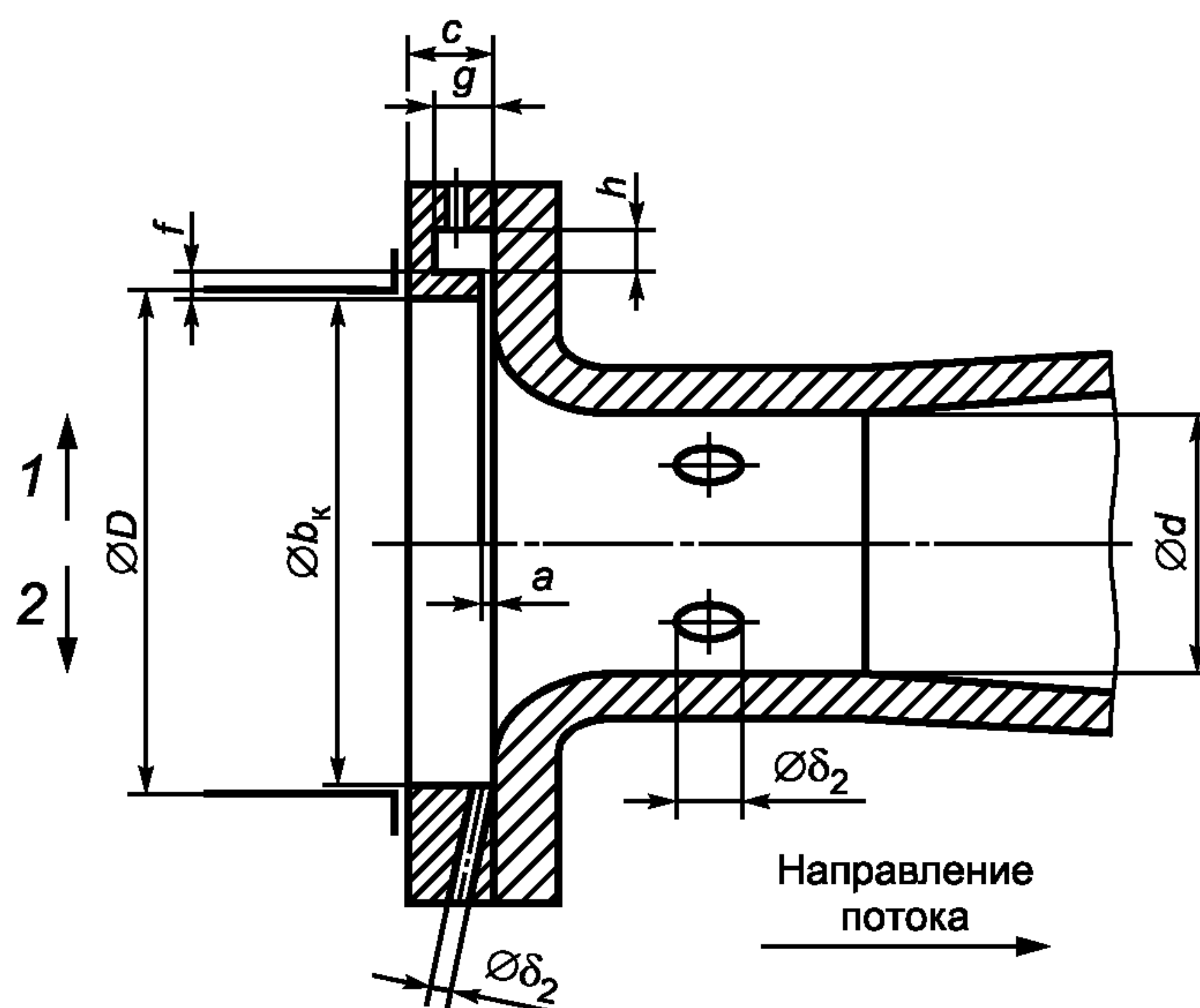
Рисунок 4 — Способы отбора давления, используемые для сопел Вентури
