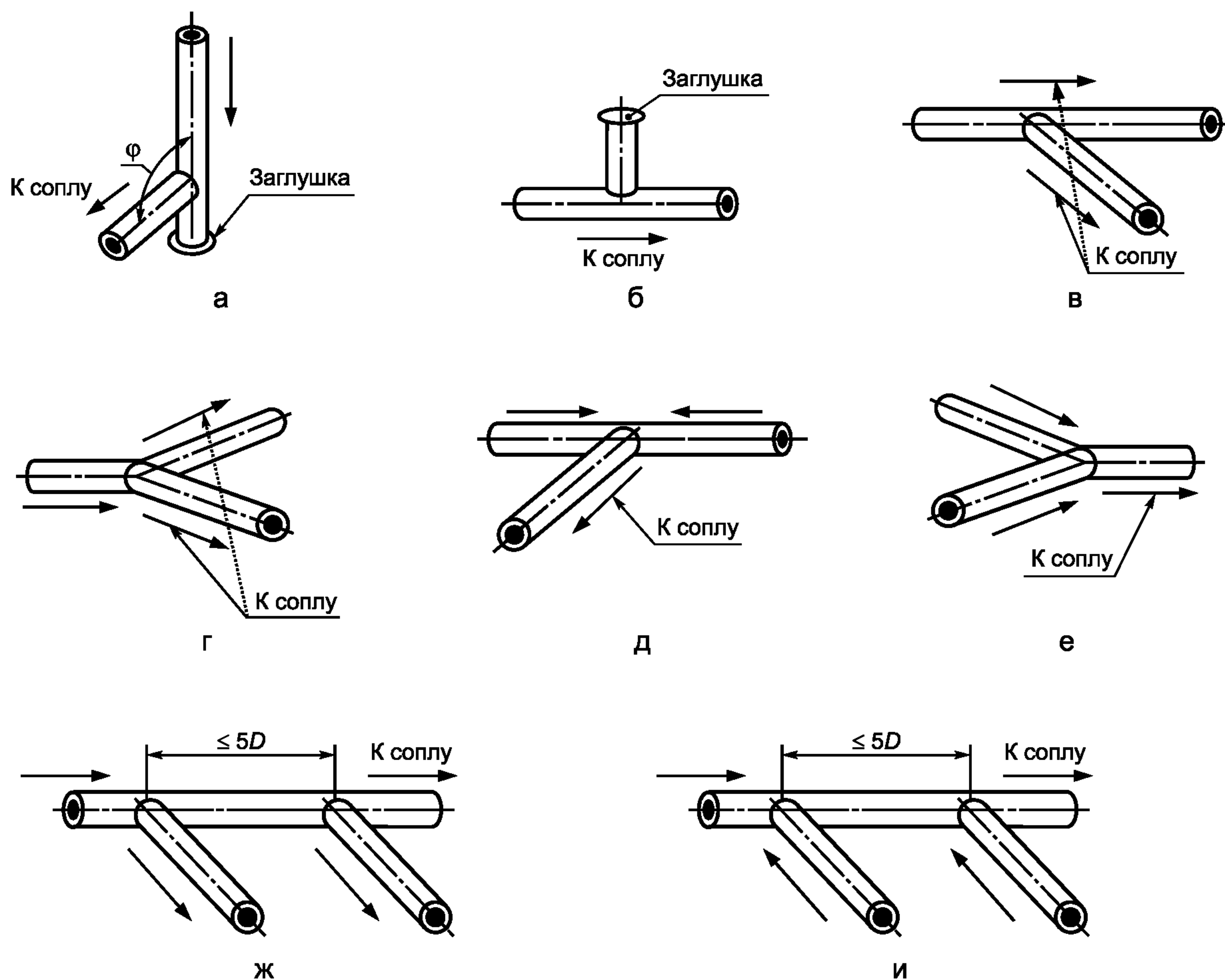
Рисунок А.2 — Тройники
