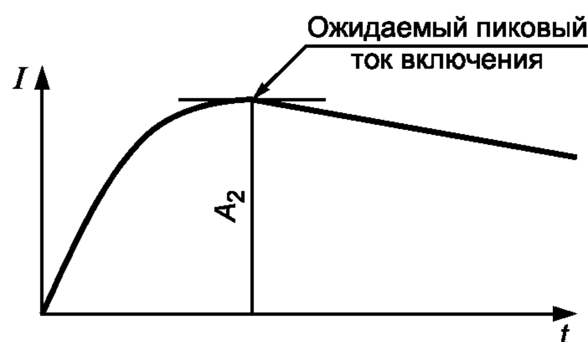
Рисунок 7b — Калибровка испытательной цепи для постоянного тока
