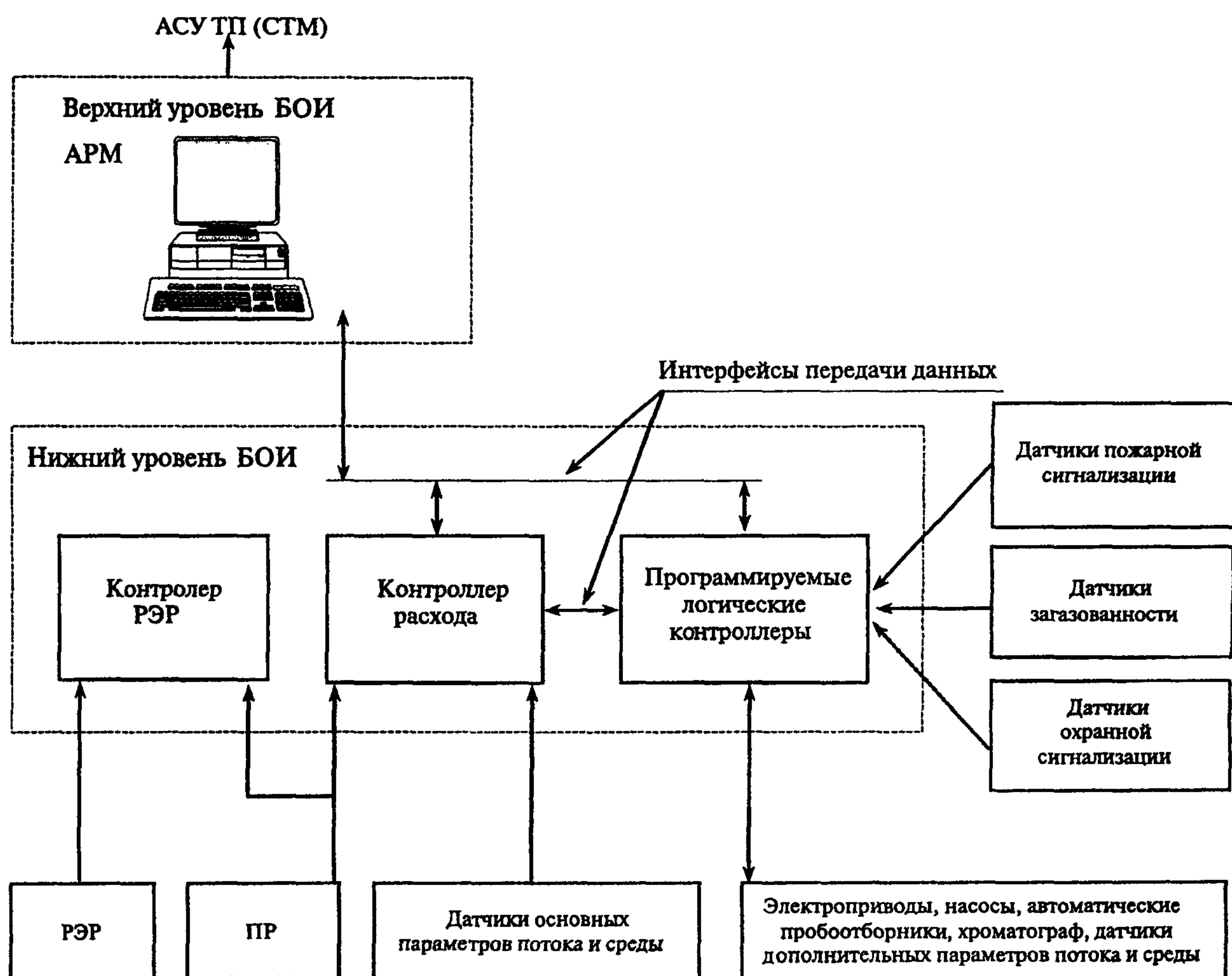
Рисунок Д.1 – Структура ПТС БОИ
