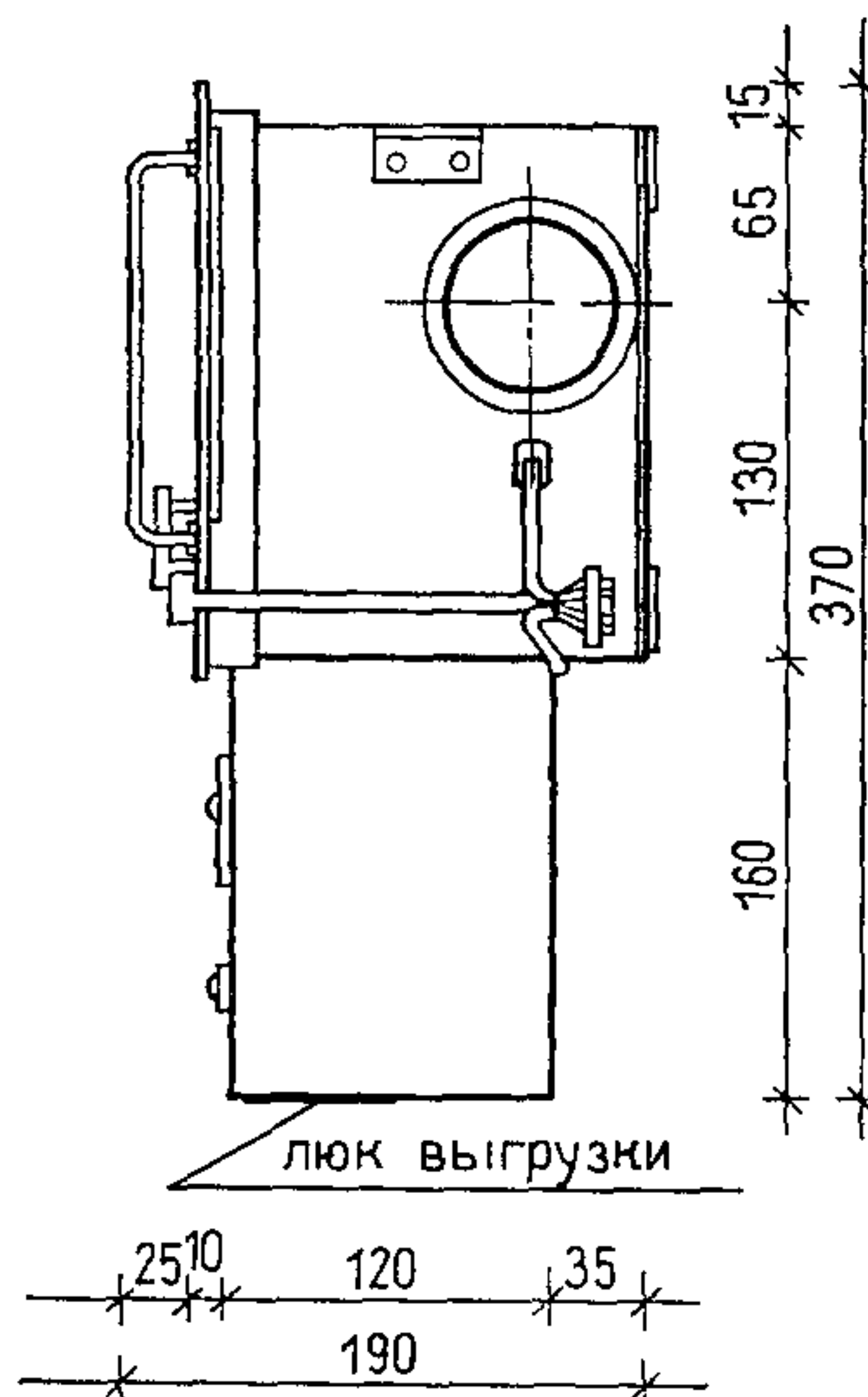
ПРИЕМНО-ОТПРАВНАЯ СТАНЦИЯ ПНЕВМОПОЧТЫ ПТУ-2
