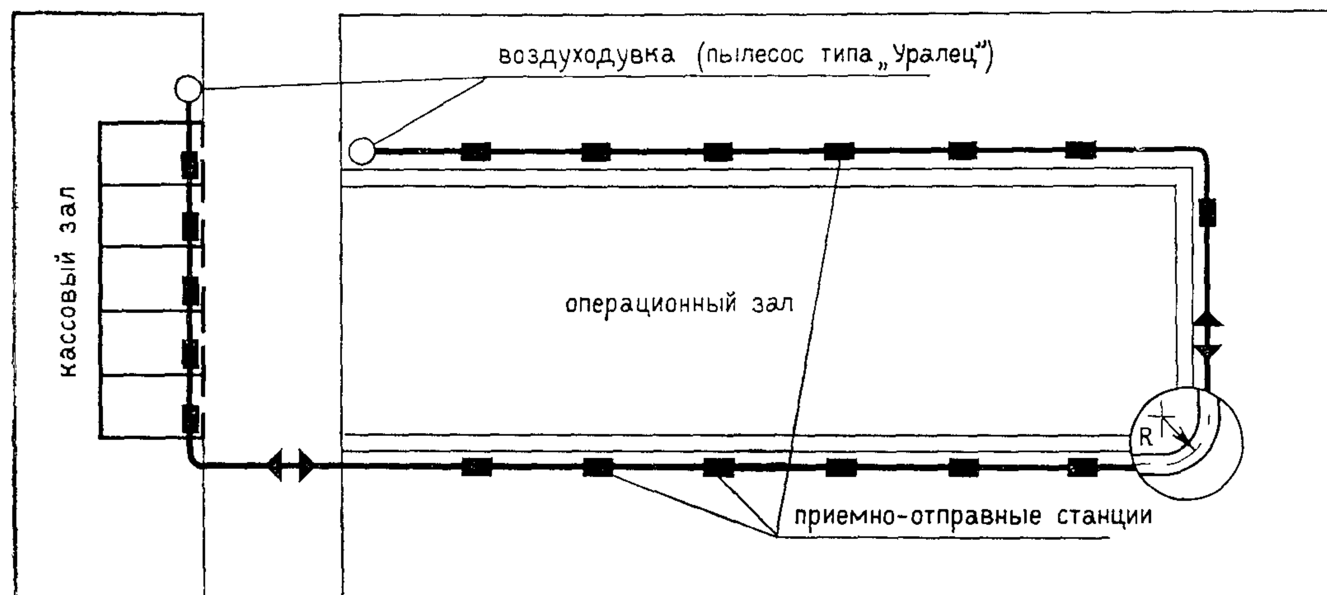
СХЕМА ОДНОТРУБНОЙ ДВУХСТОРОННЕЙ АВТОМАТИЧЕСКОЙ ПНЕВМОПОЧТЫ ПТУ-2
