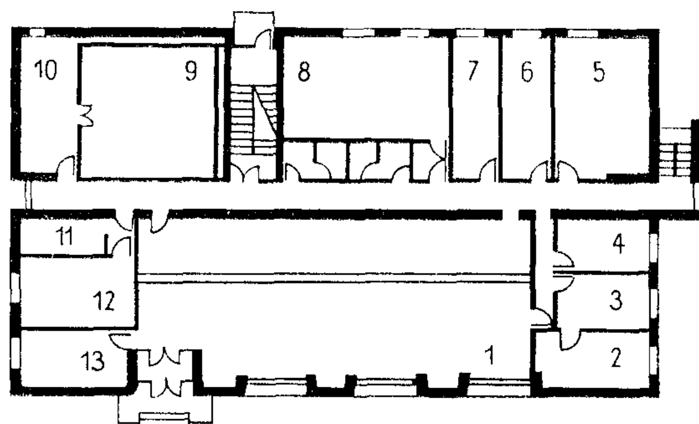
План I этажа
