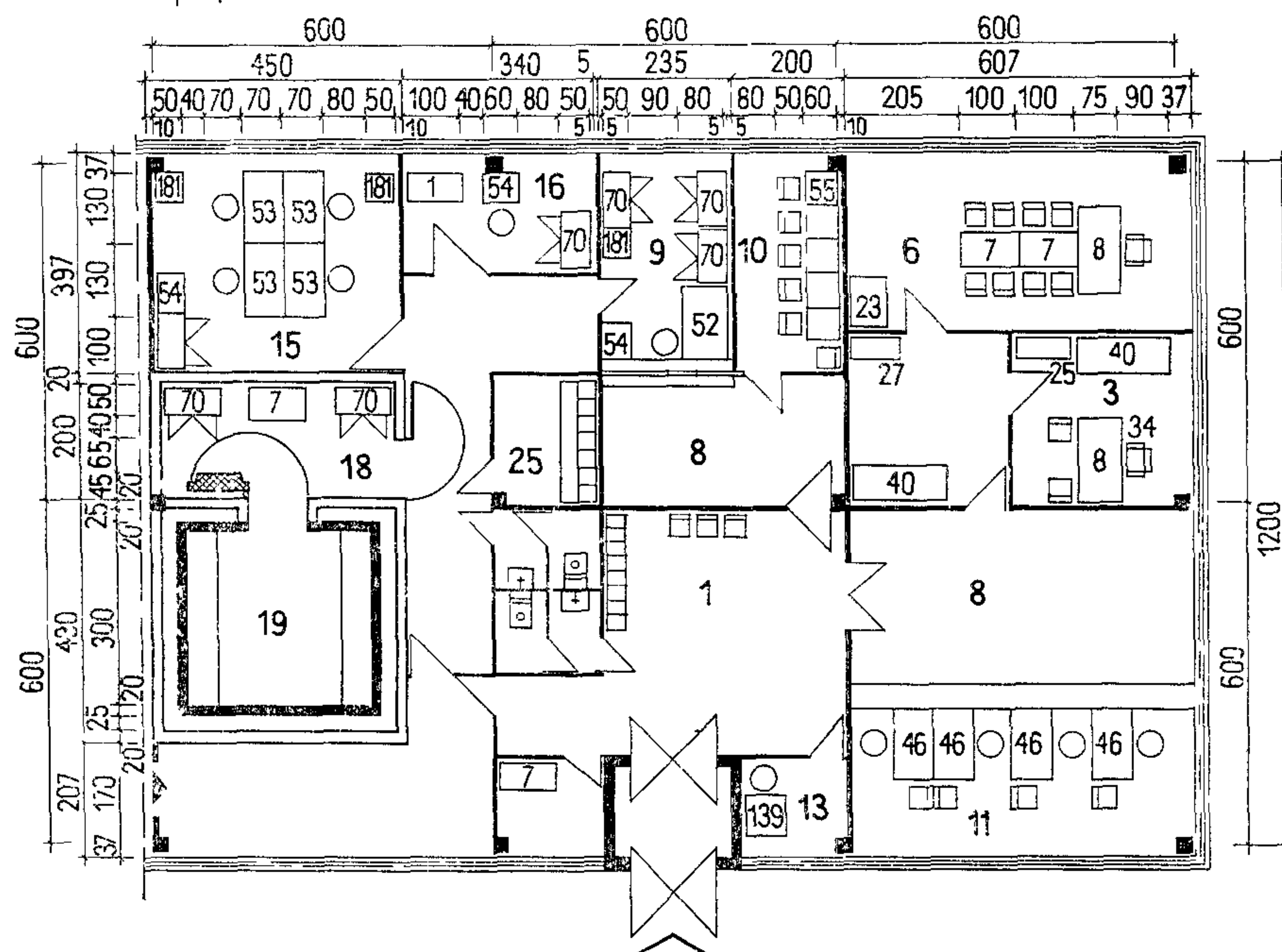
Районное отделение Госбанка при одной операционной кассе, отдельных кассовом и операционном залах
