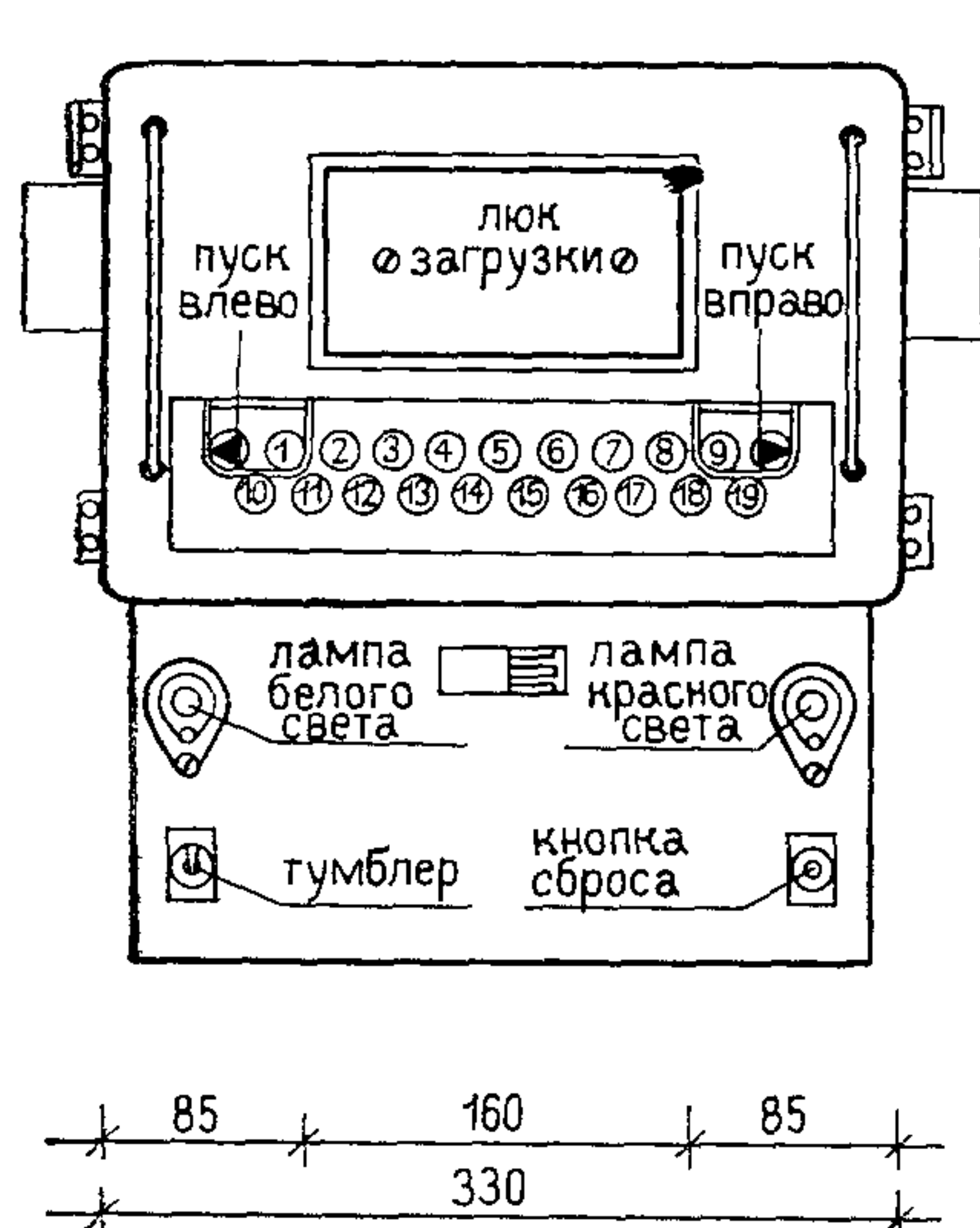
ПРИЕМНО-ОТПРАВНАЯ СТАНЦИЯ ПНЕВМОПОЧТЫ ПТУ-2
