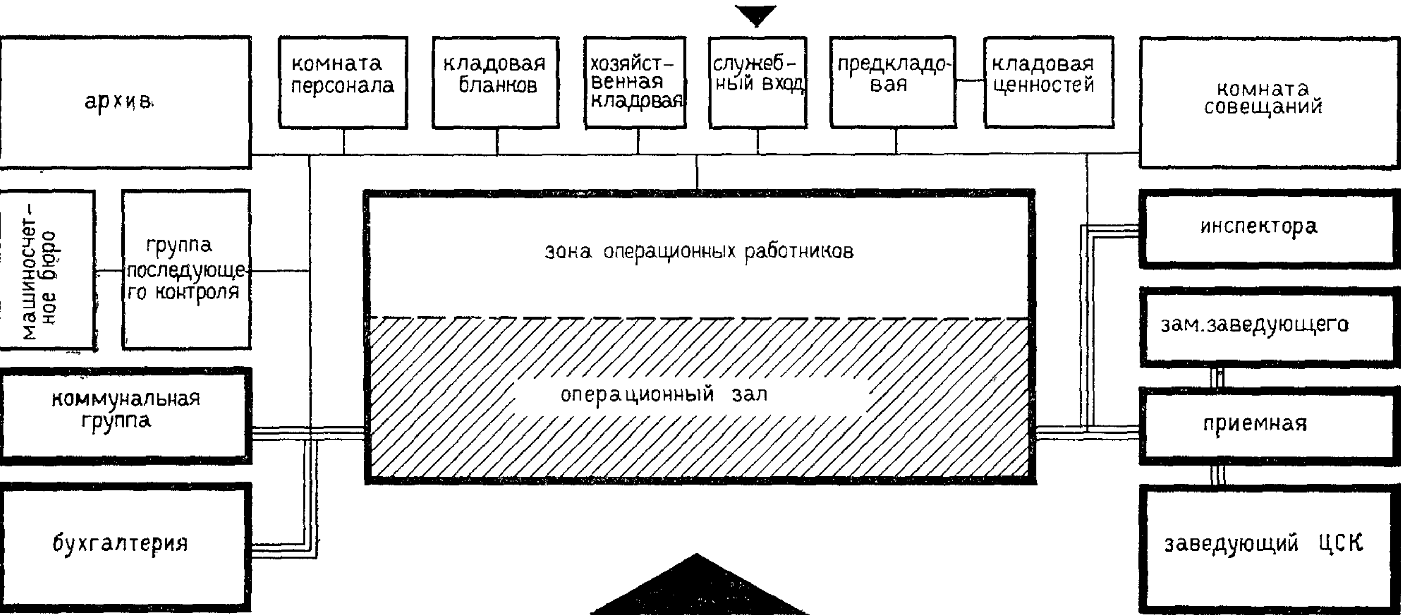
СХЕМА ВЗАИМОСВЯЗИ ПОМЕЩЕНИЙ ЦЕНТРАЛЬНОЙ СБЕРЕГАТЕЛЬНОЙ КАССЫ
