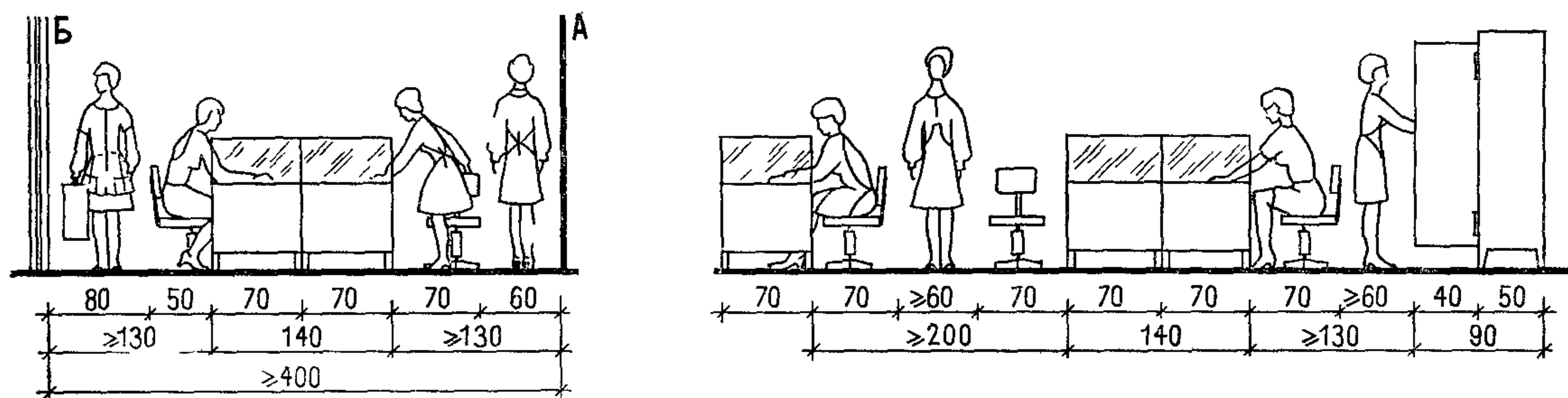
Помещение для пересчета денежных билетов (касса пересчета)
