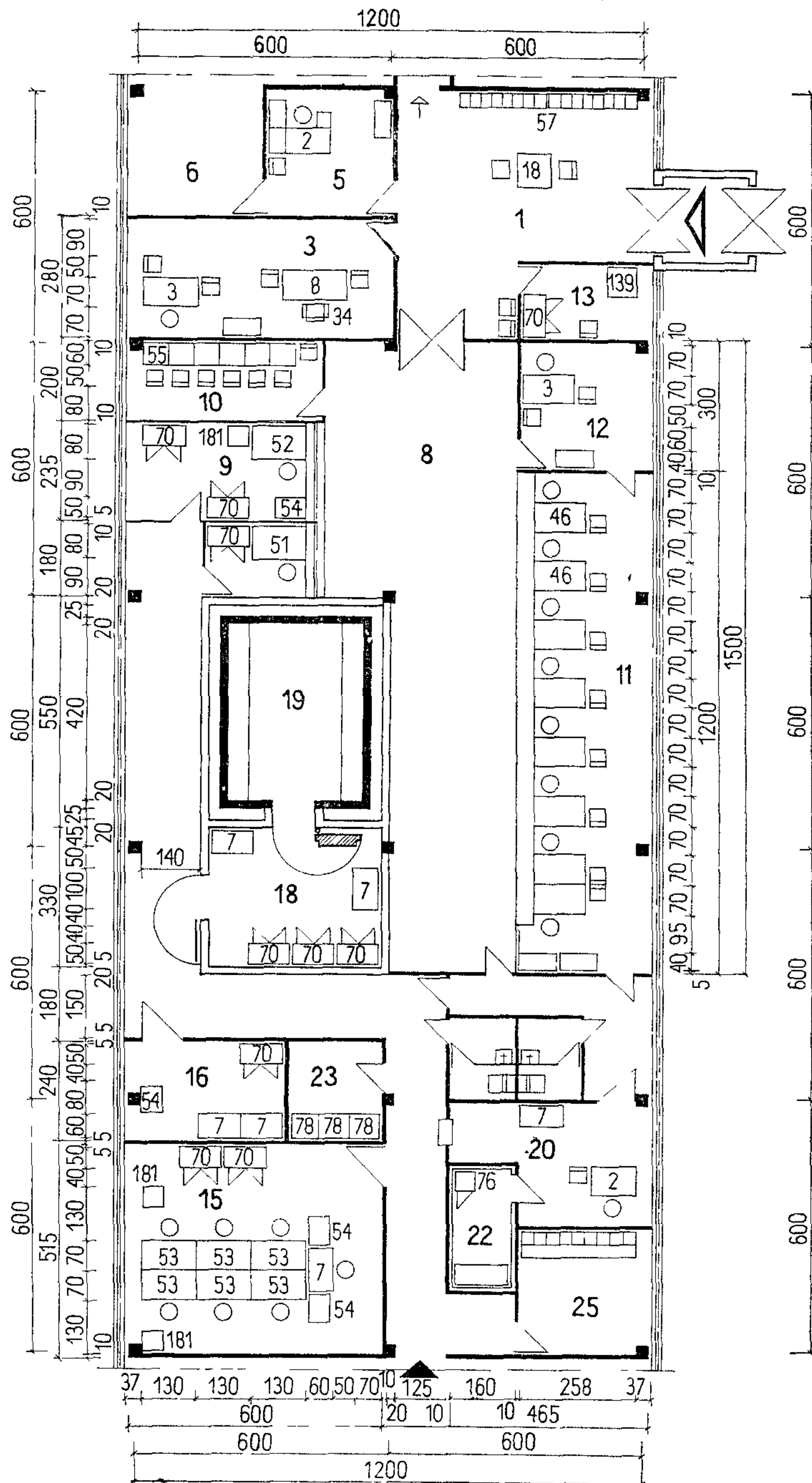
РАЙОННОЕ ОТДЕЛЕНИЕ ГОСБАНКА ПРИ ДВУХ ОПЕРАЦИОННЫХ КАССАХ
