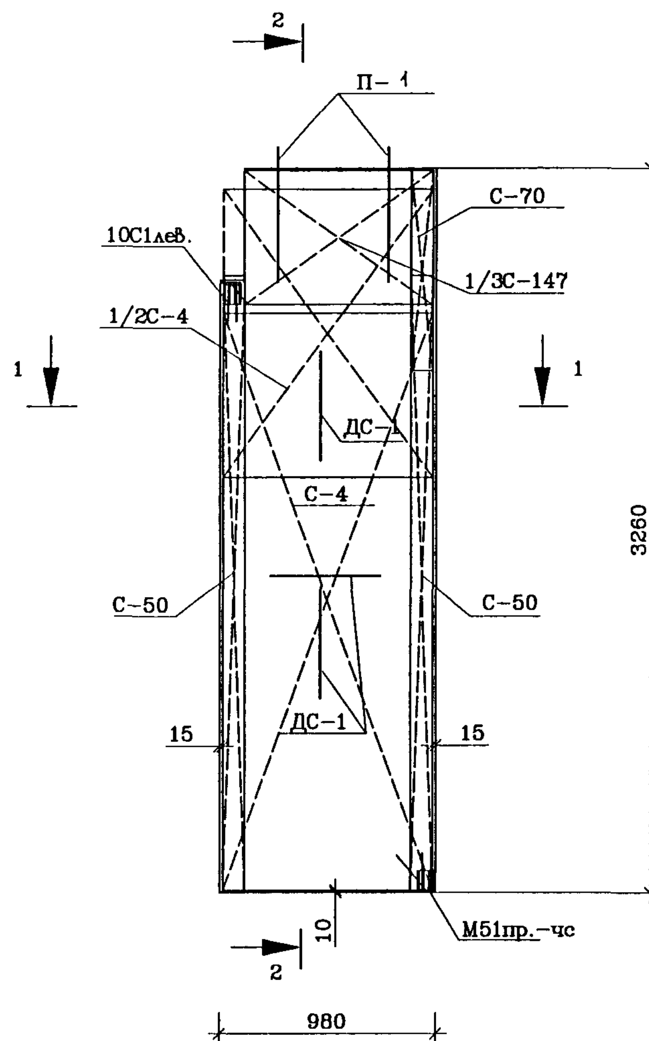
Армирование панели 1ЛНФЧ 10-1
