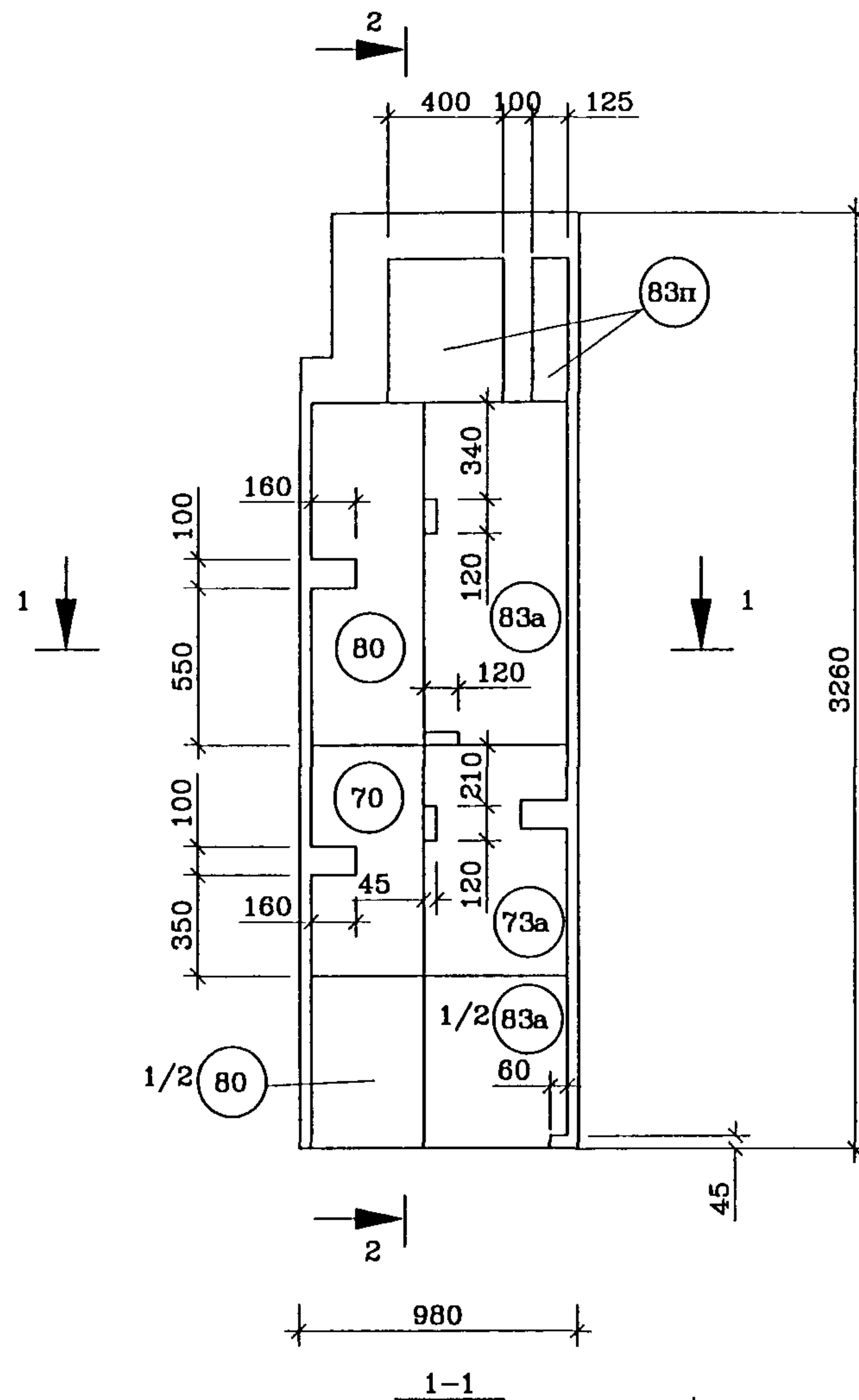
Раскладка утеплителя 1ЛНФЧ 10-1
