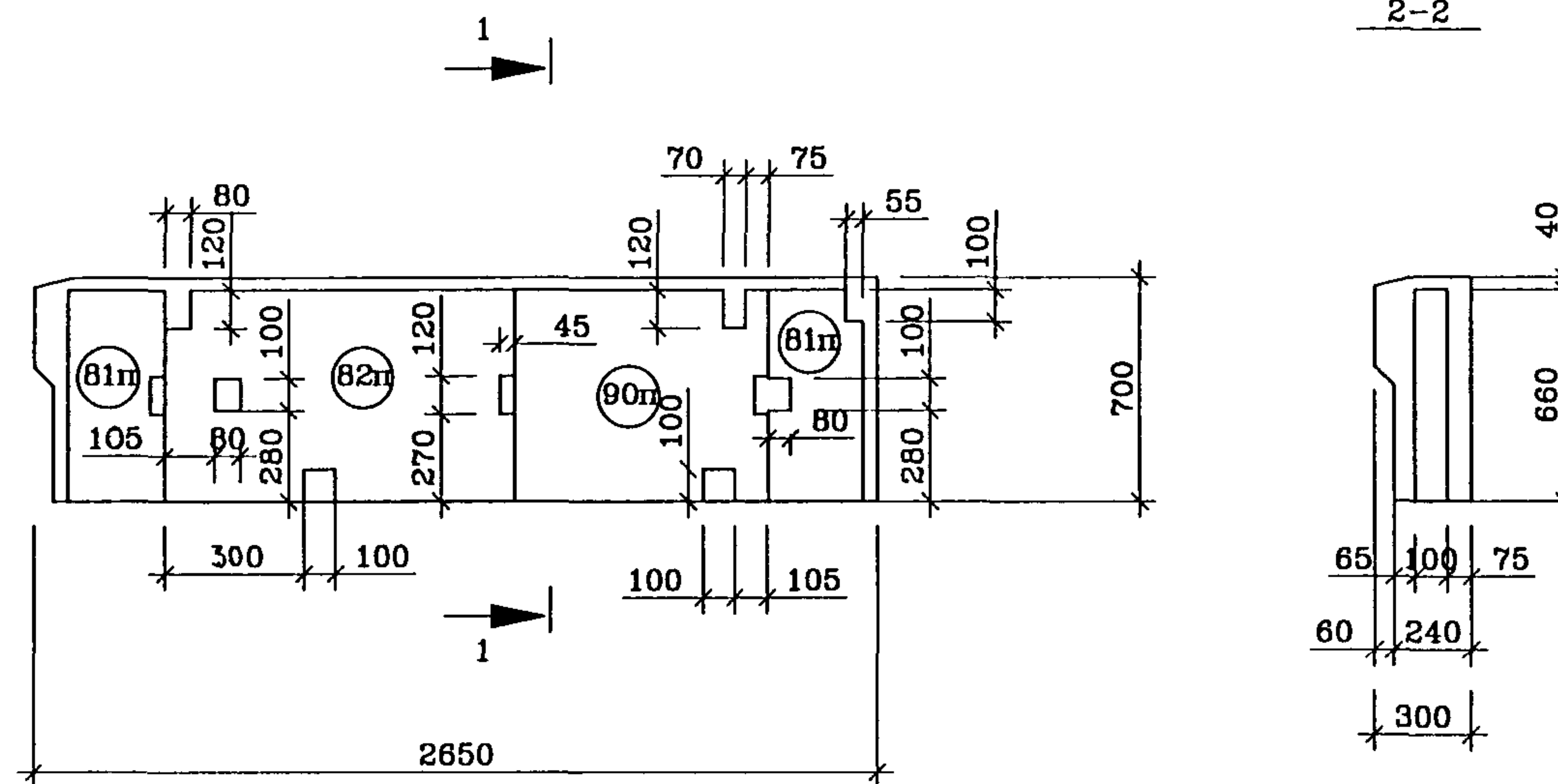
Раскладка утеплителя панели ЛНФЧ 26-1
