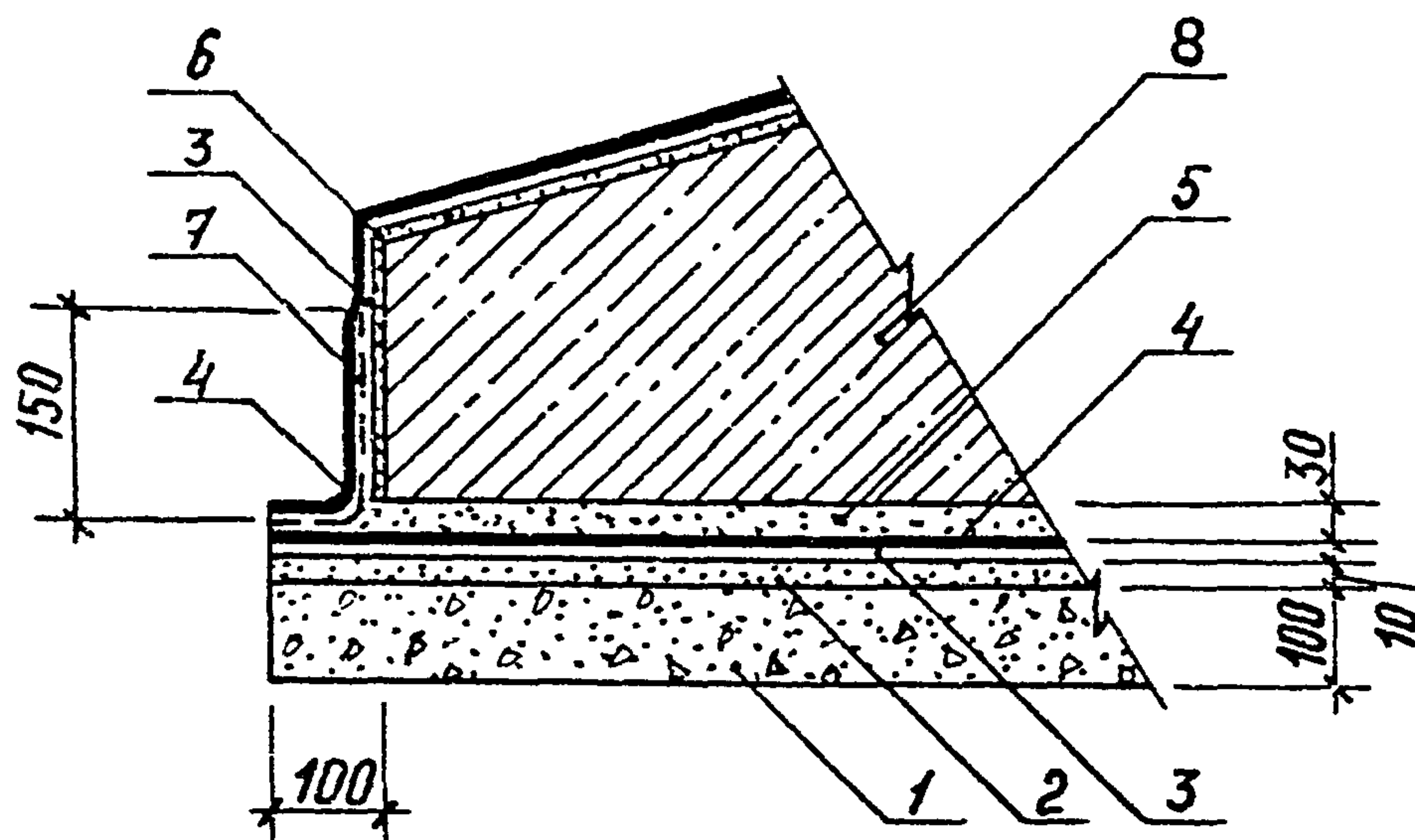
Рис. 9. Узел 5. Окрашенная гидроизоляция
