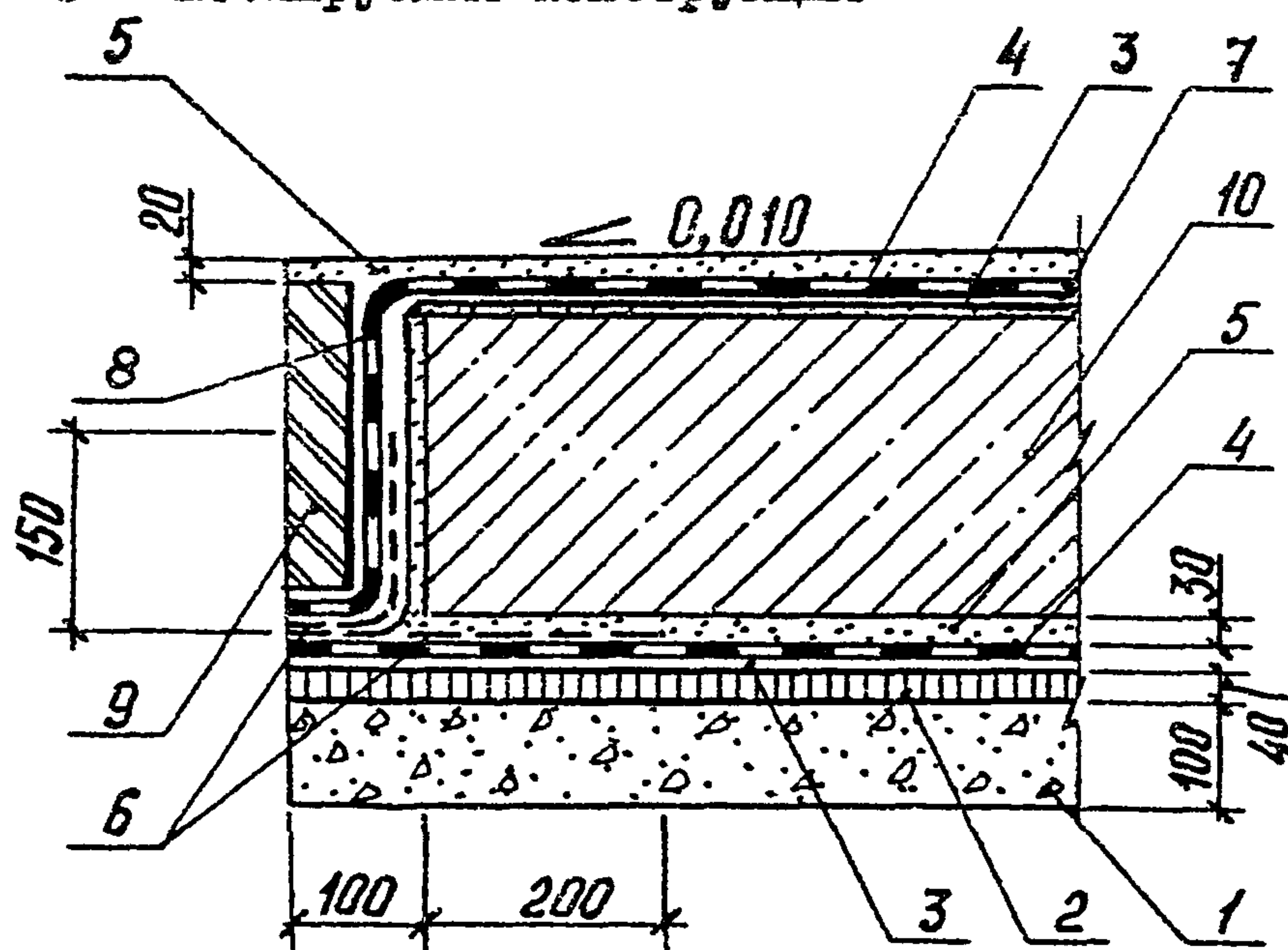
Рис. 20. Узел I6. Оклеечная гидроизоляция
