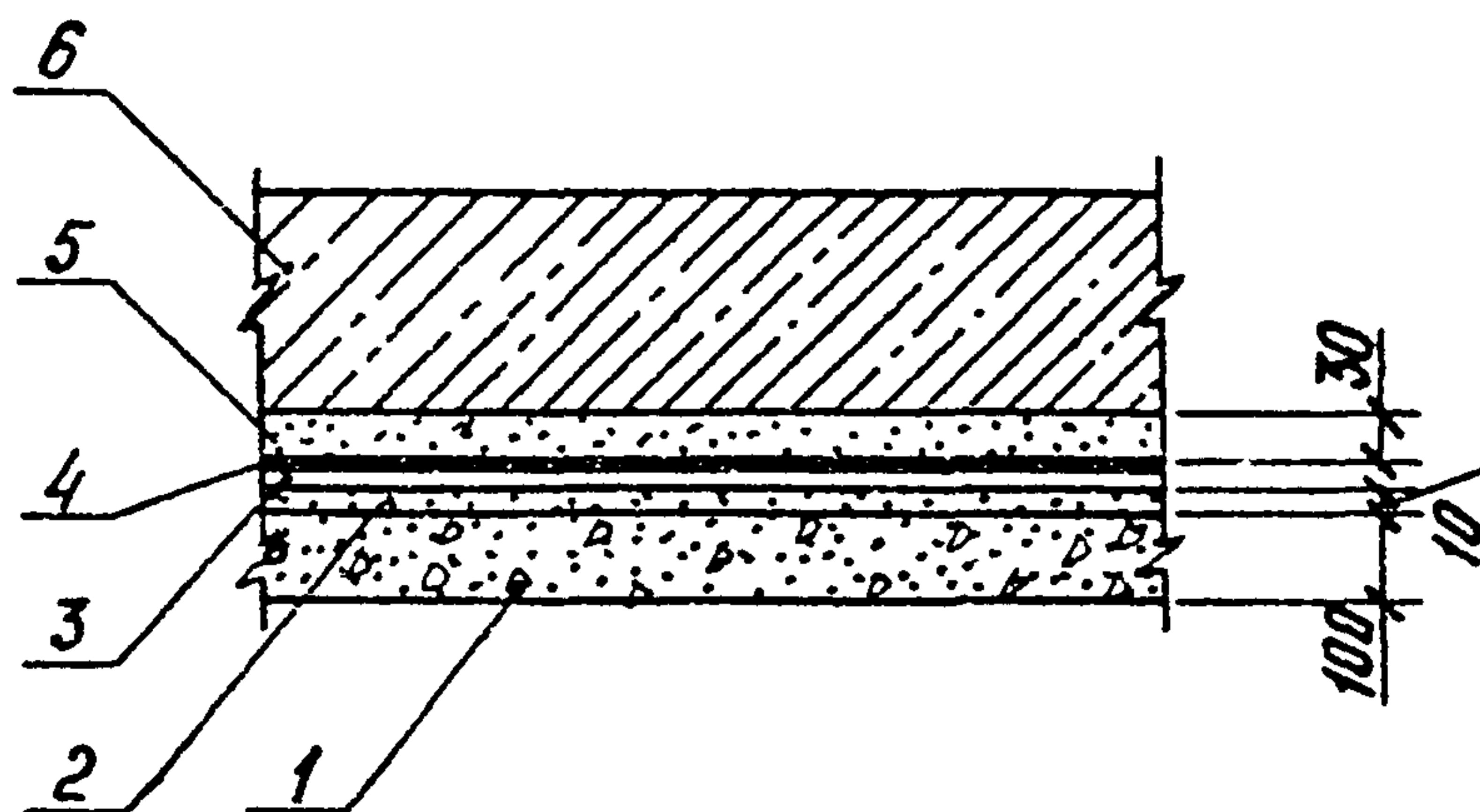
Рис. 5. Узел I. Окрасочная гидроизоляция
