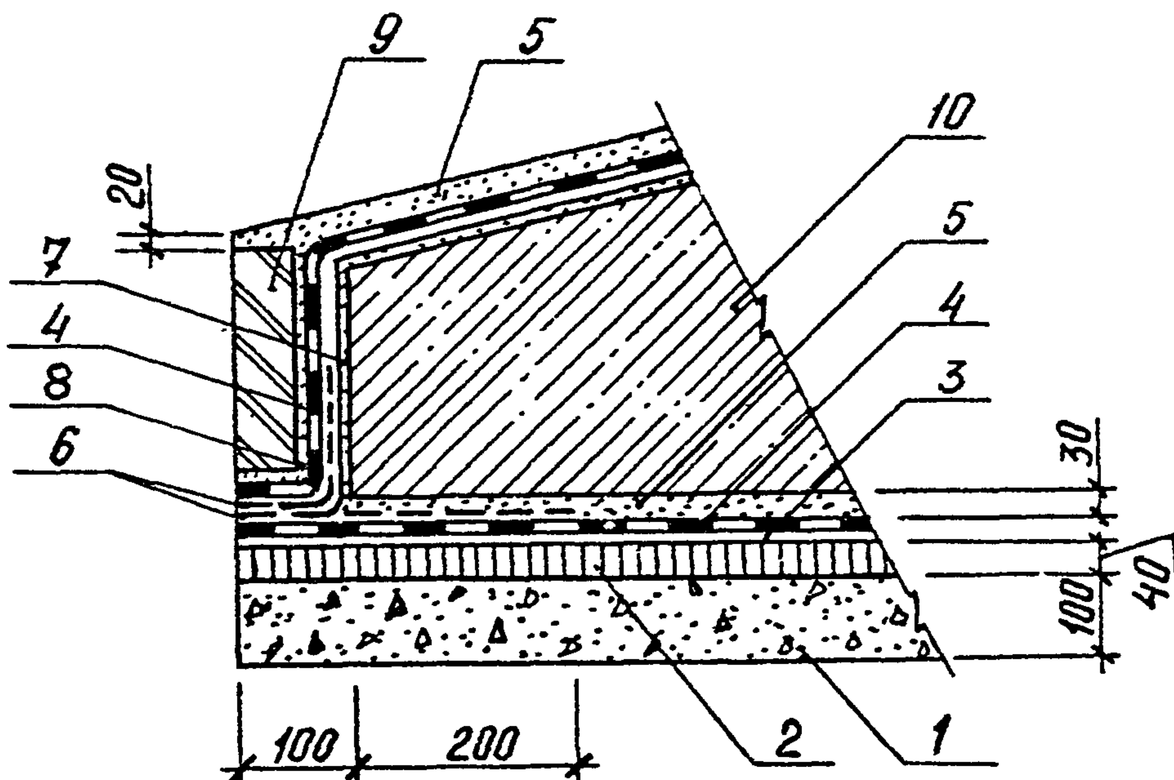
Рис. I2. Узел 8. Оклеечная гидроизоляция
