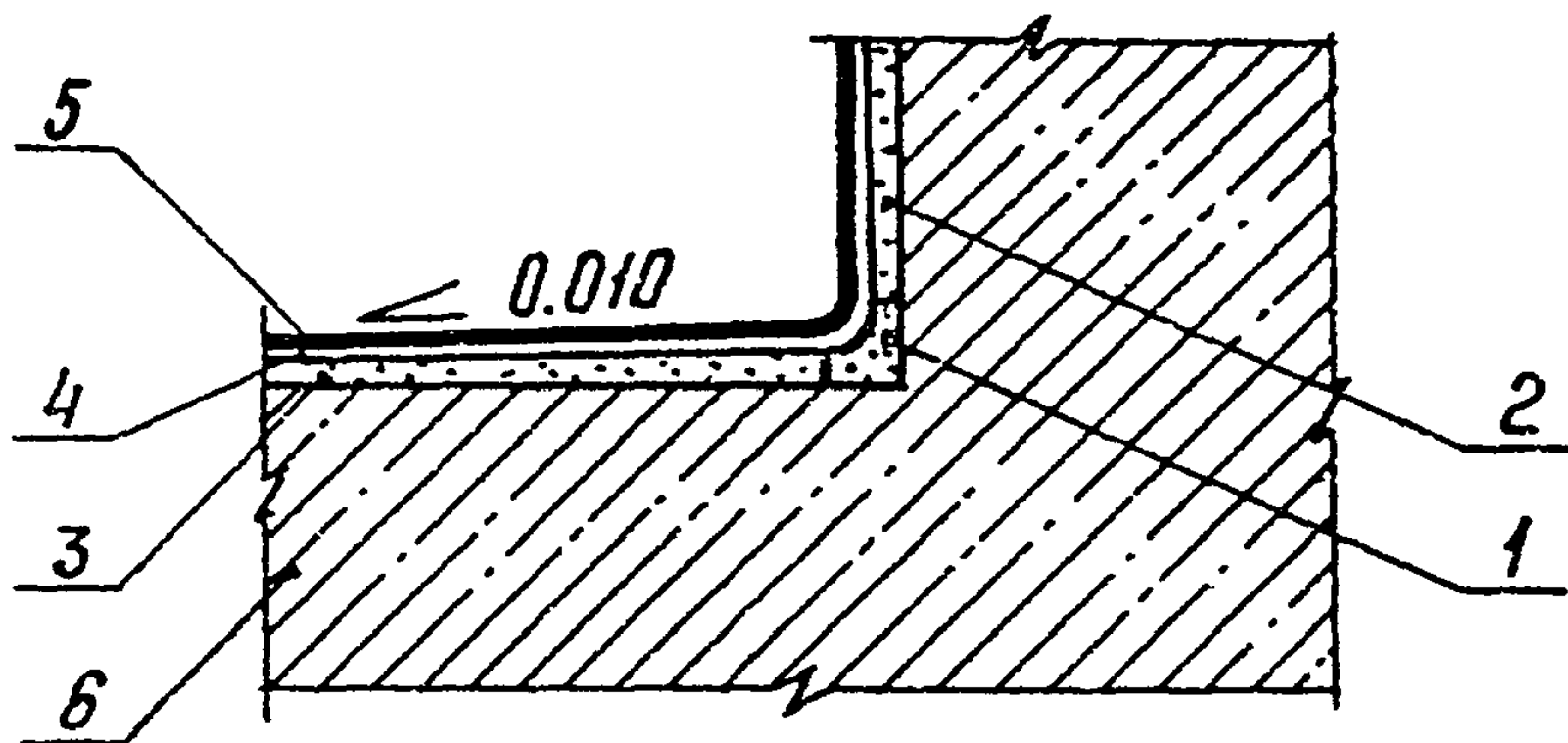
Рис. 13. Узел 9. Окрасочная гидроизоляция
