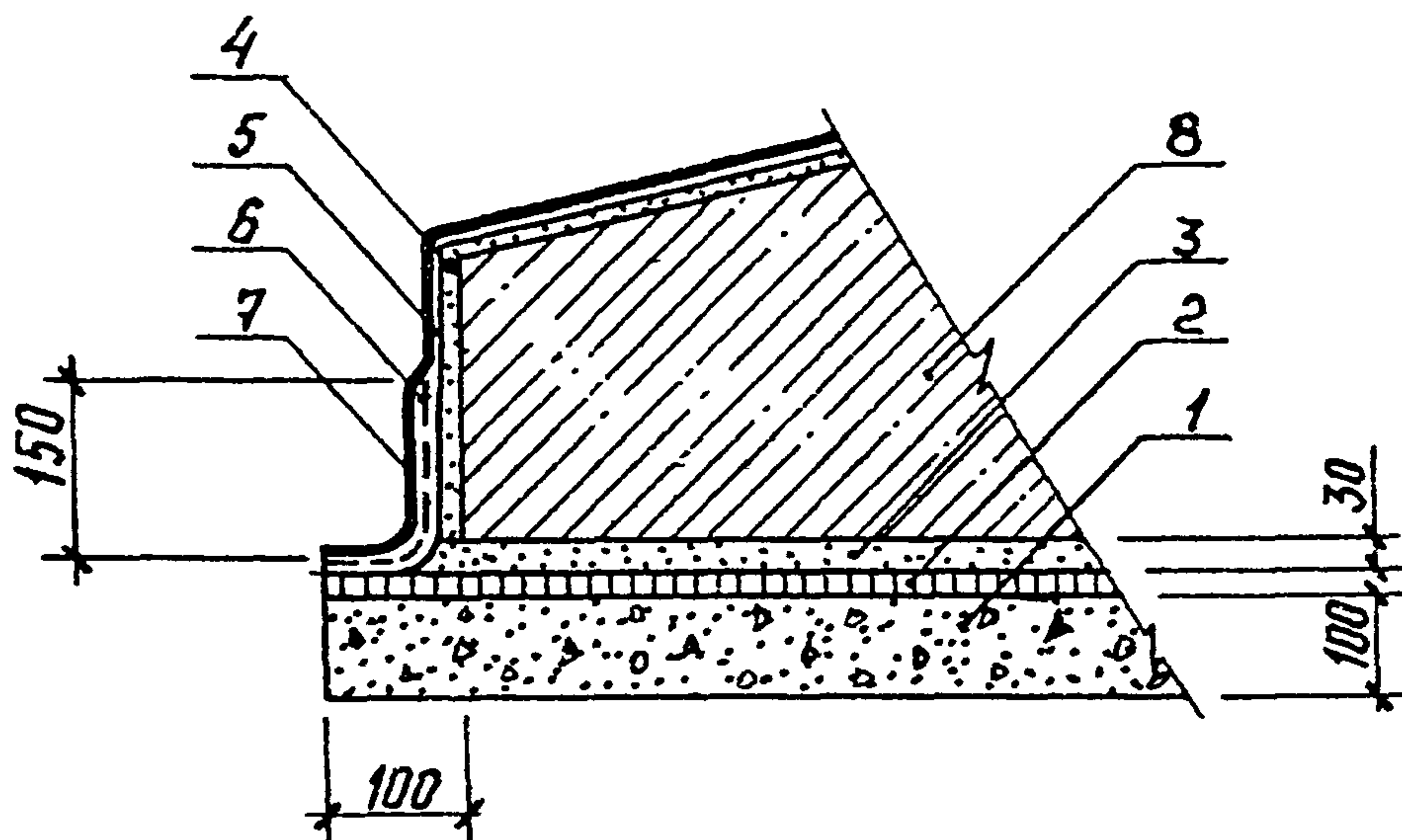
Рис. II. Узел 7. Литая и окрасочная гидроизоляция
