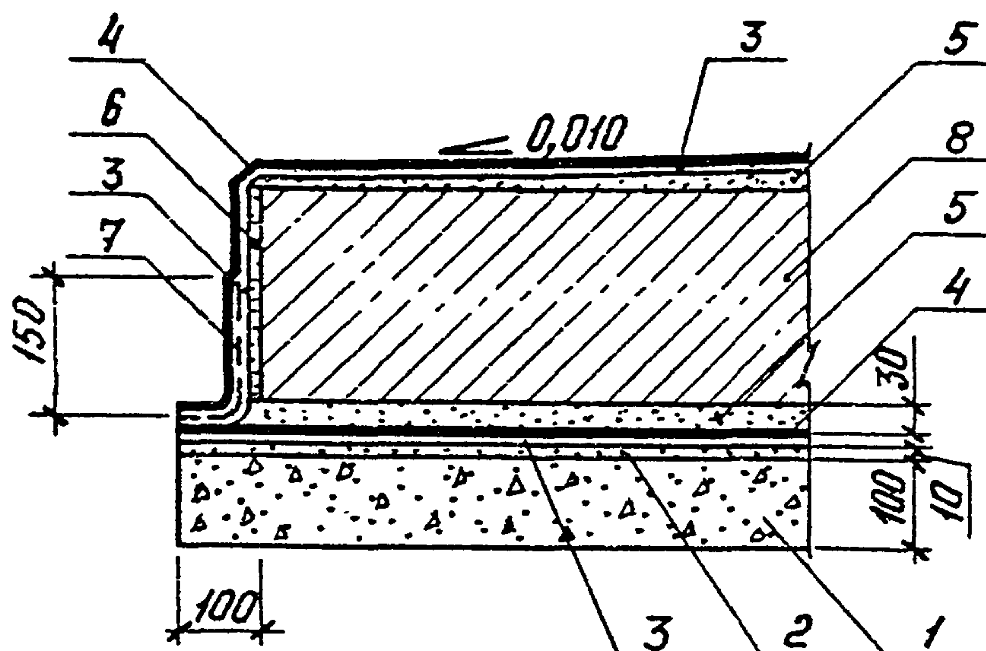
Рис. I7. Узел I3. Окрасочная гидроизоляция
