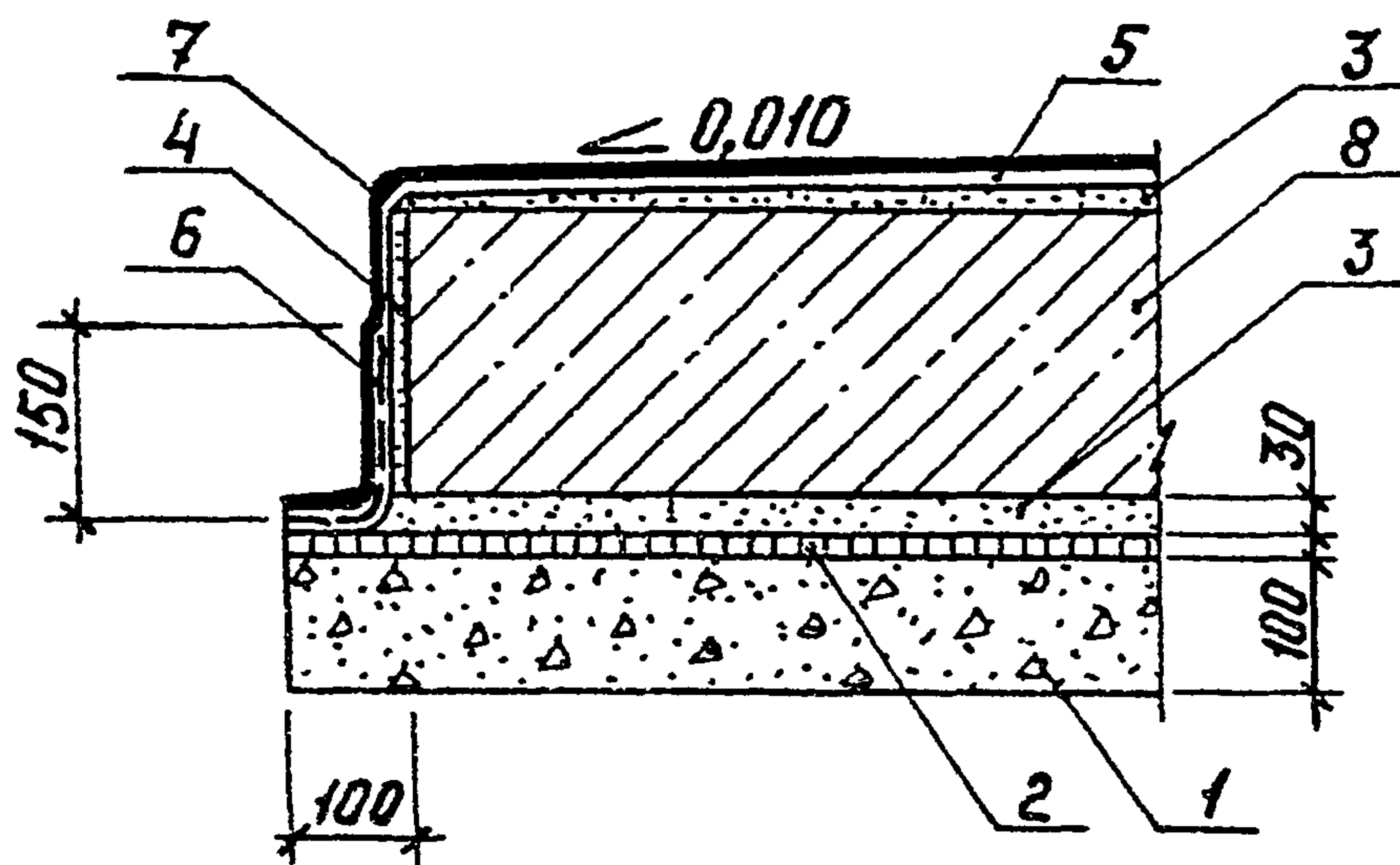
Рис. 19. Узел I5. Литая и окрасочная гидроизоляция
