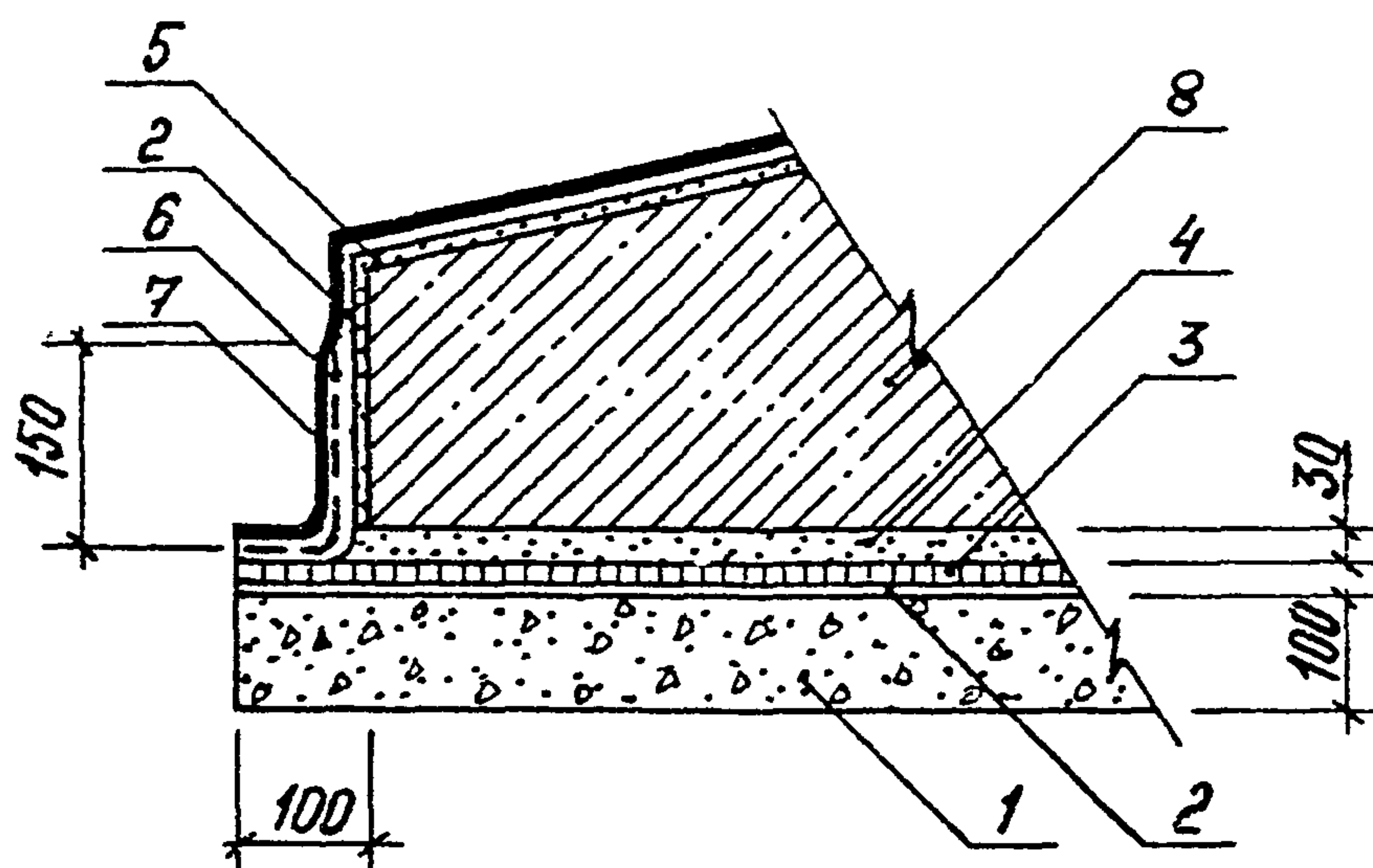
Рис. 10. Узел 6. Асфальтовая и окрасочная гидроизоляция
