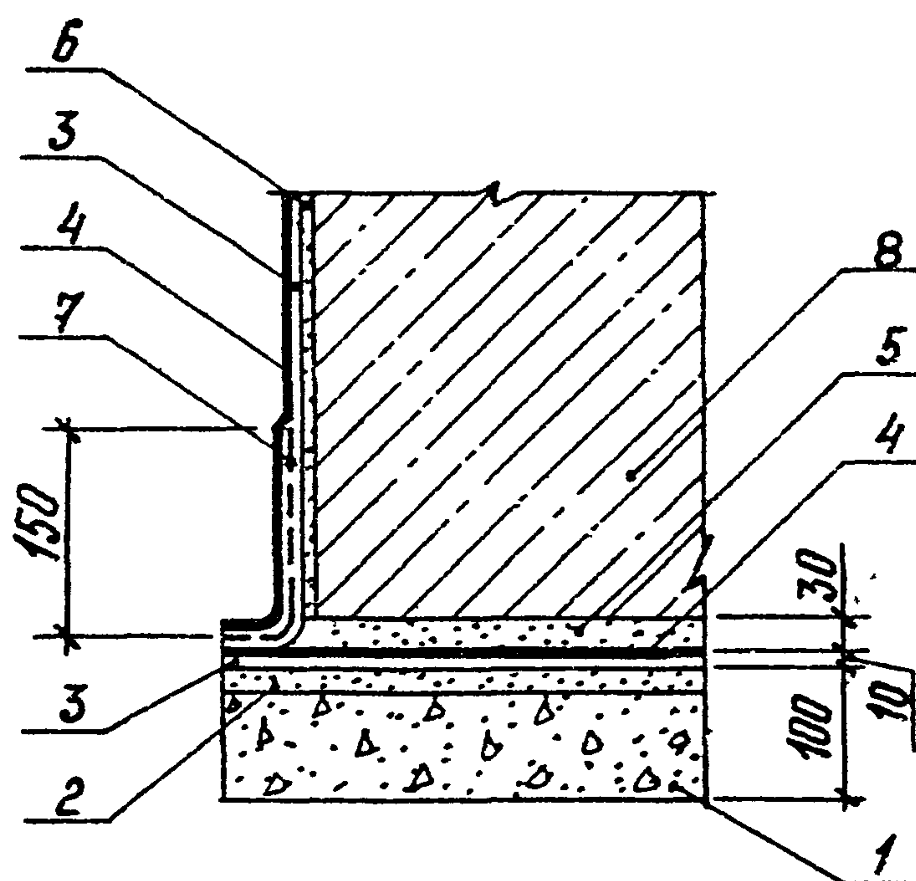
Рис. 24. Узел 20. Окрасочная гидроизоляция
