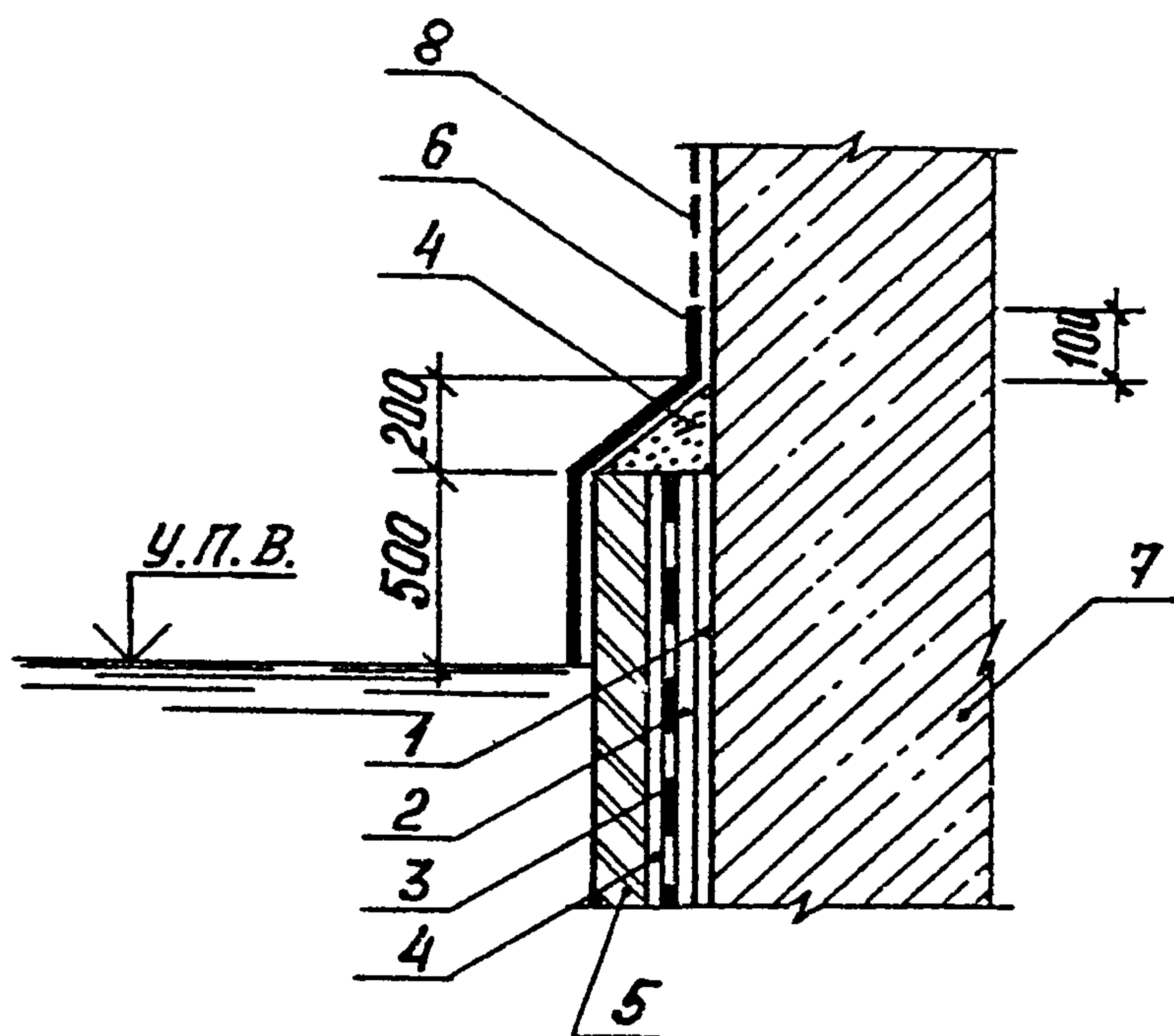
Рис. 16. Узел I2. Оклеечная гидроизоляция
