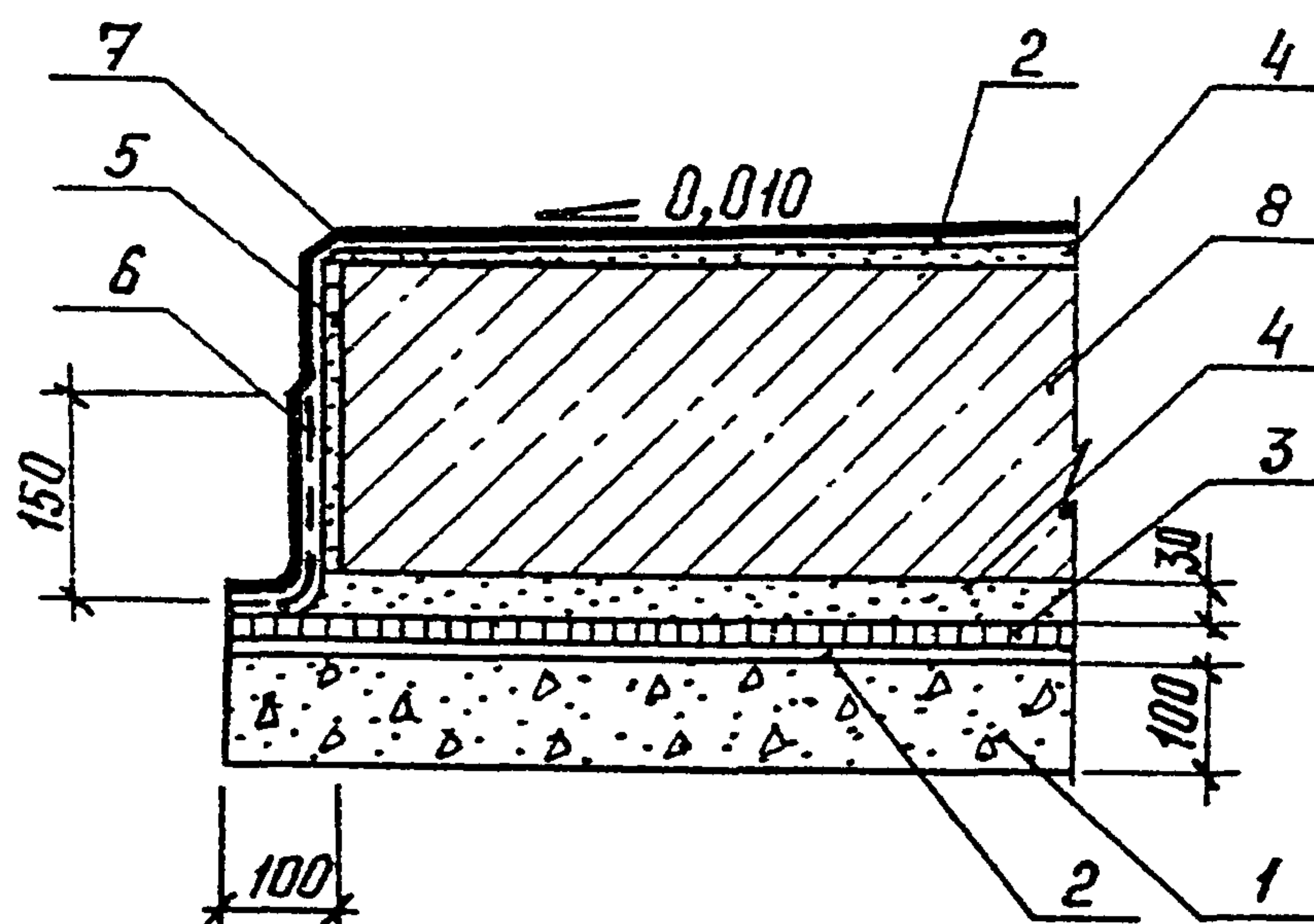
Рис. I8. Узел I4. Асфальтовая и окрасочная гидроизоляция
