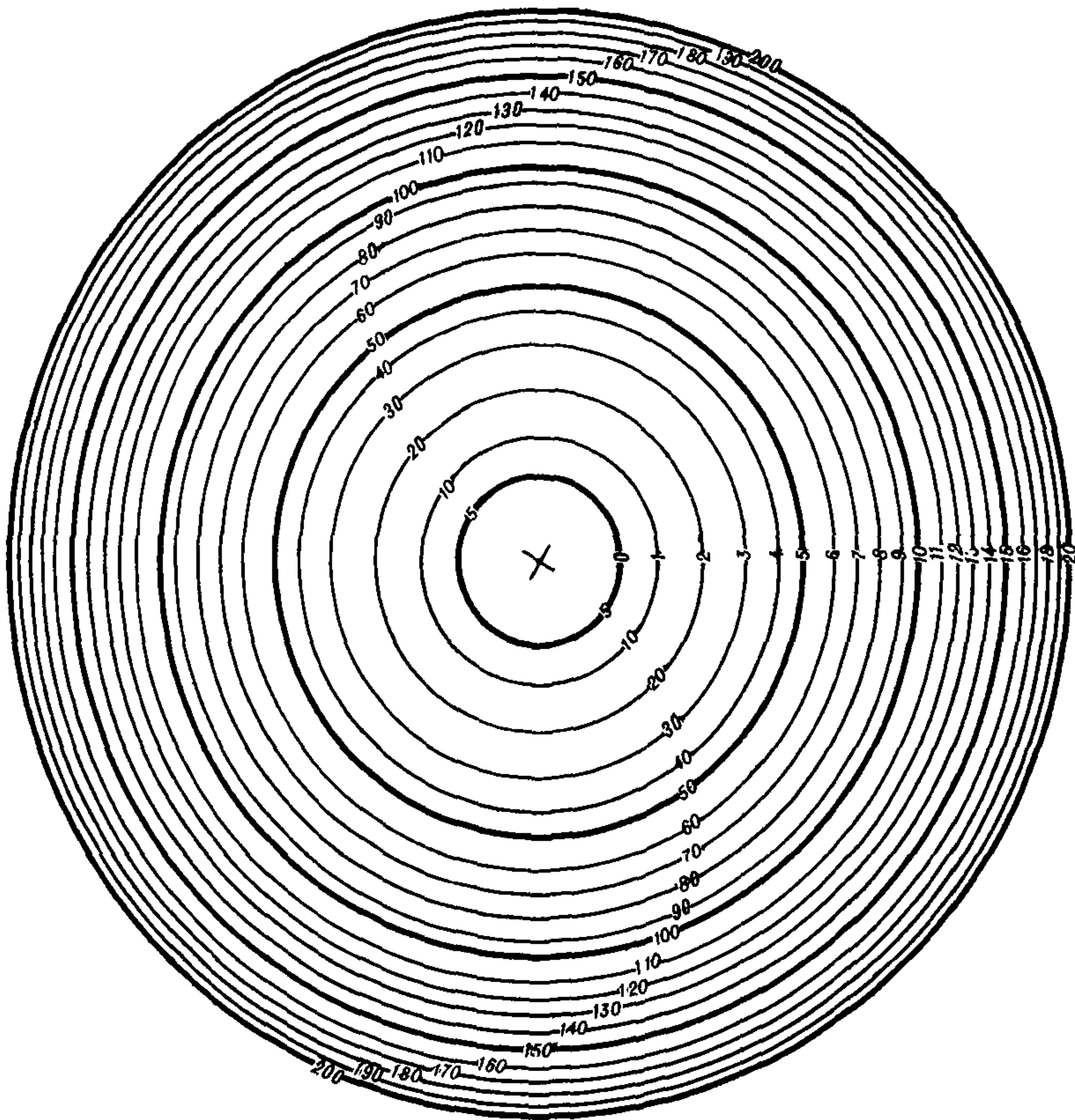
Палетка для определения поправок в показания радиовысотомера
