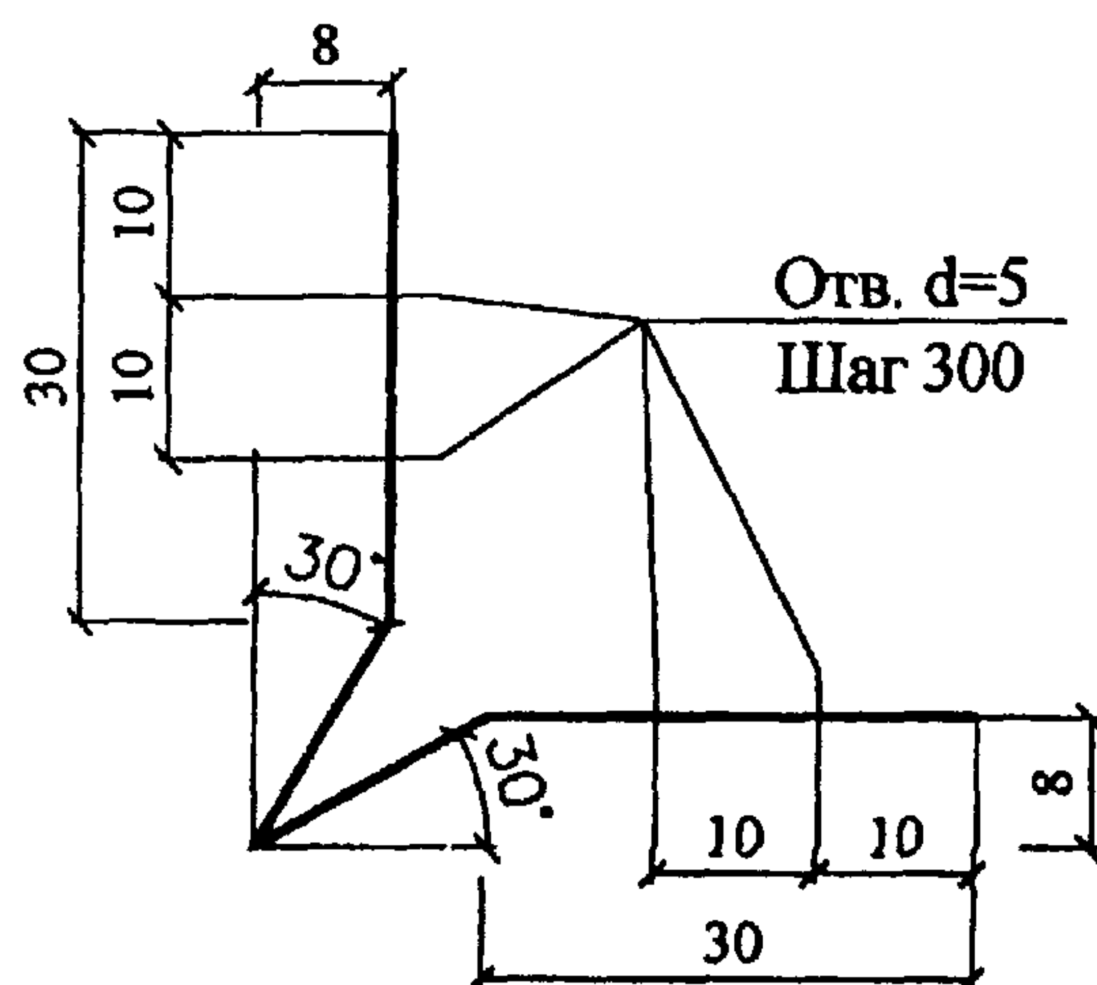
УГОЛОК С5
