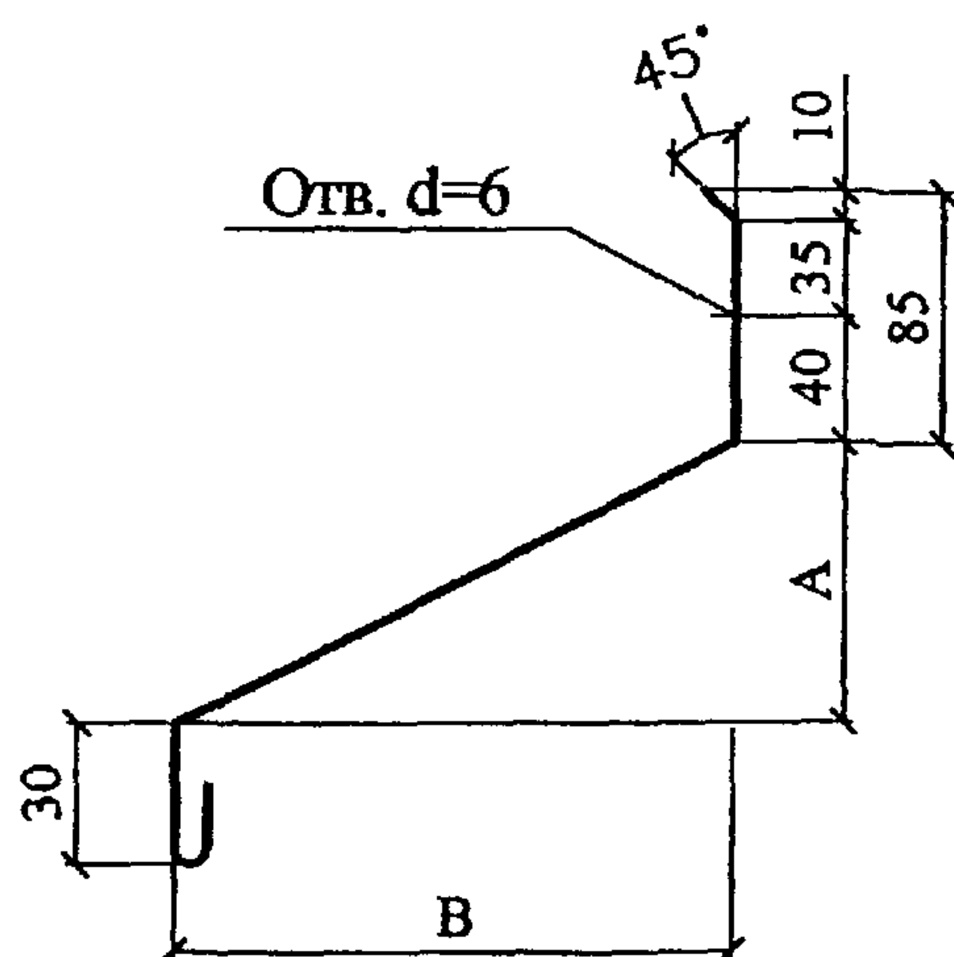
СЛИВ СЗ
