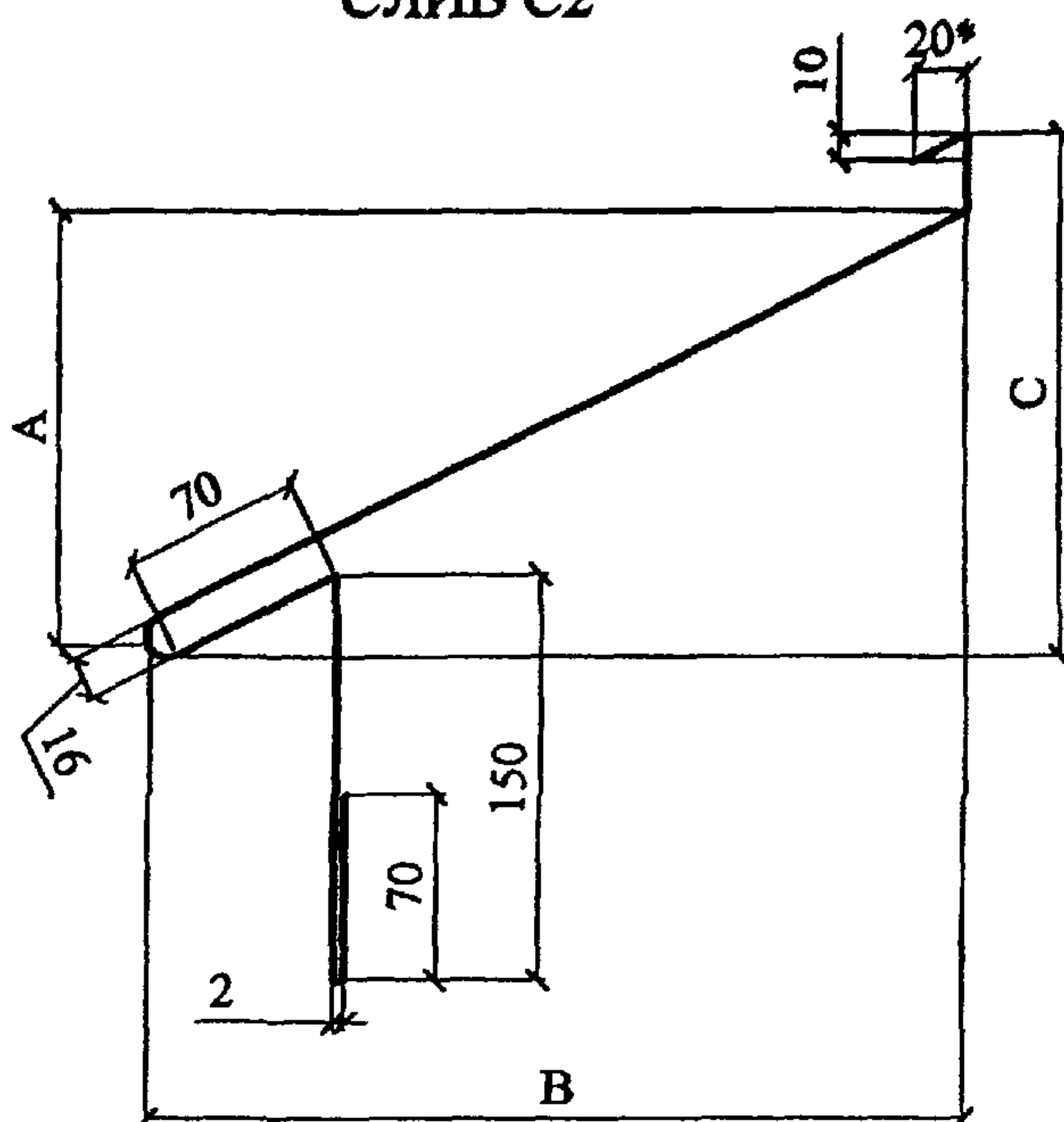
СЛИВ С2
