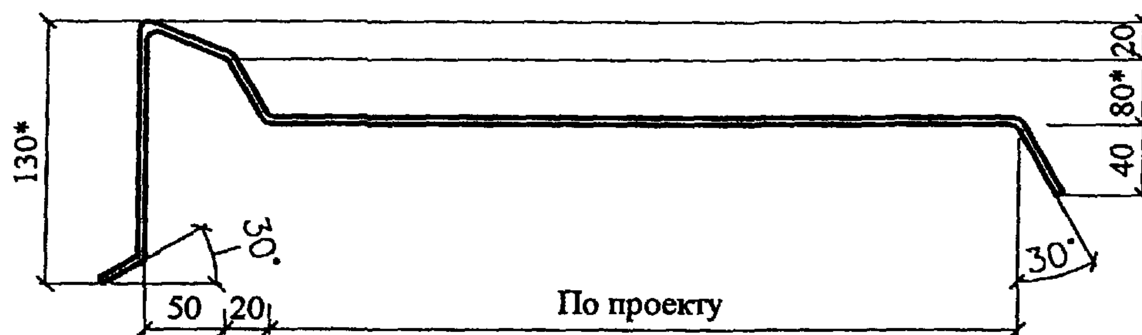
КОСТЫЛЬ К3
