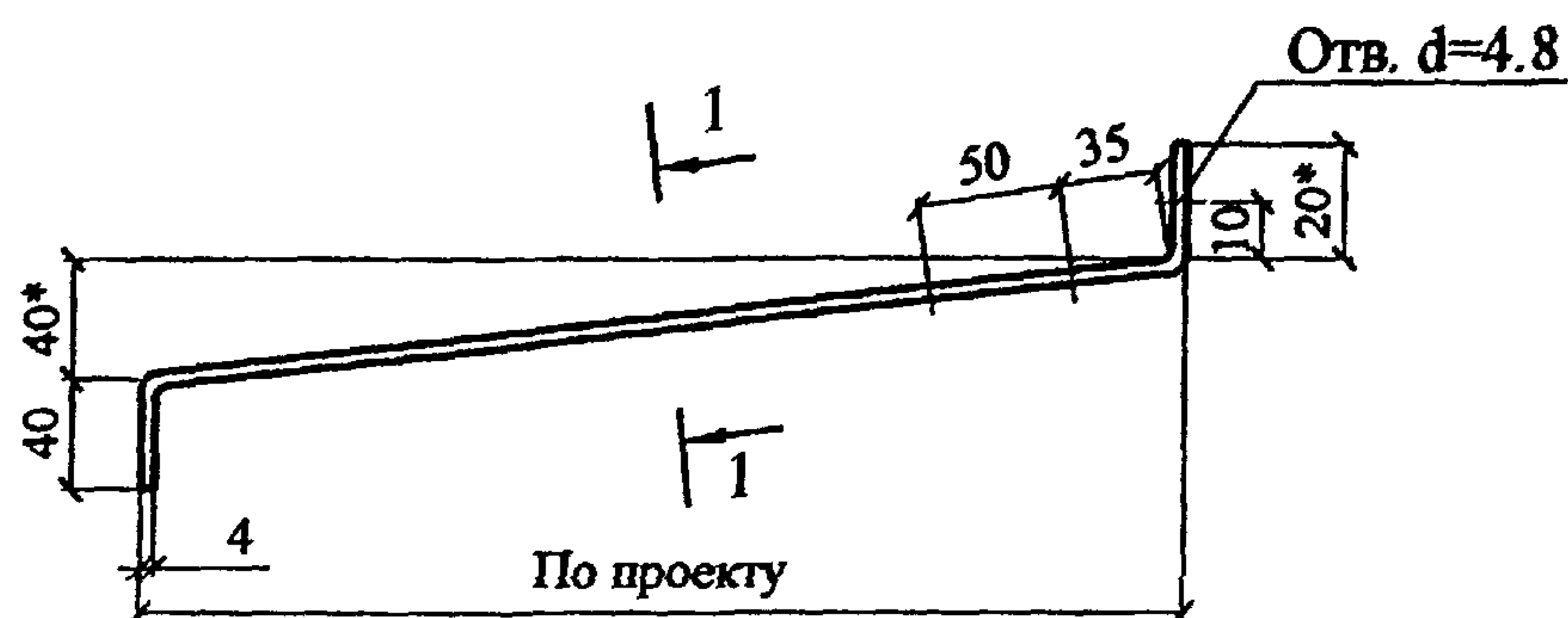
КОСТЫЛЬ К2
