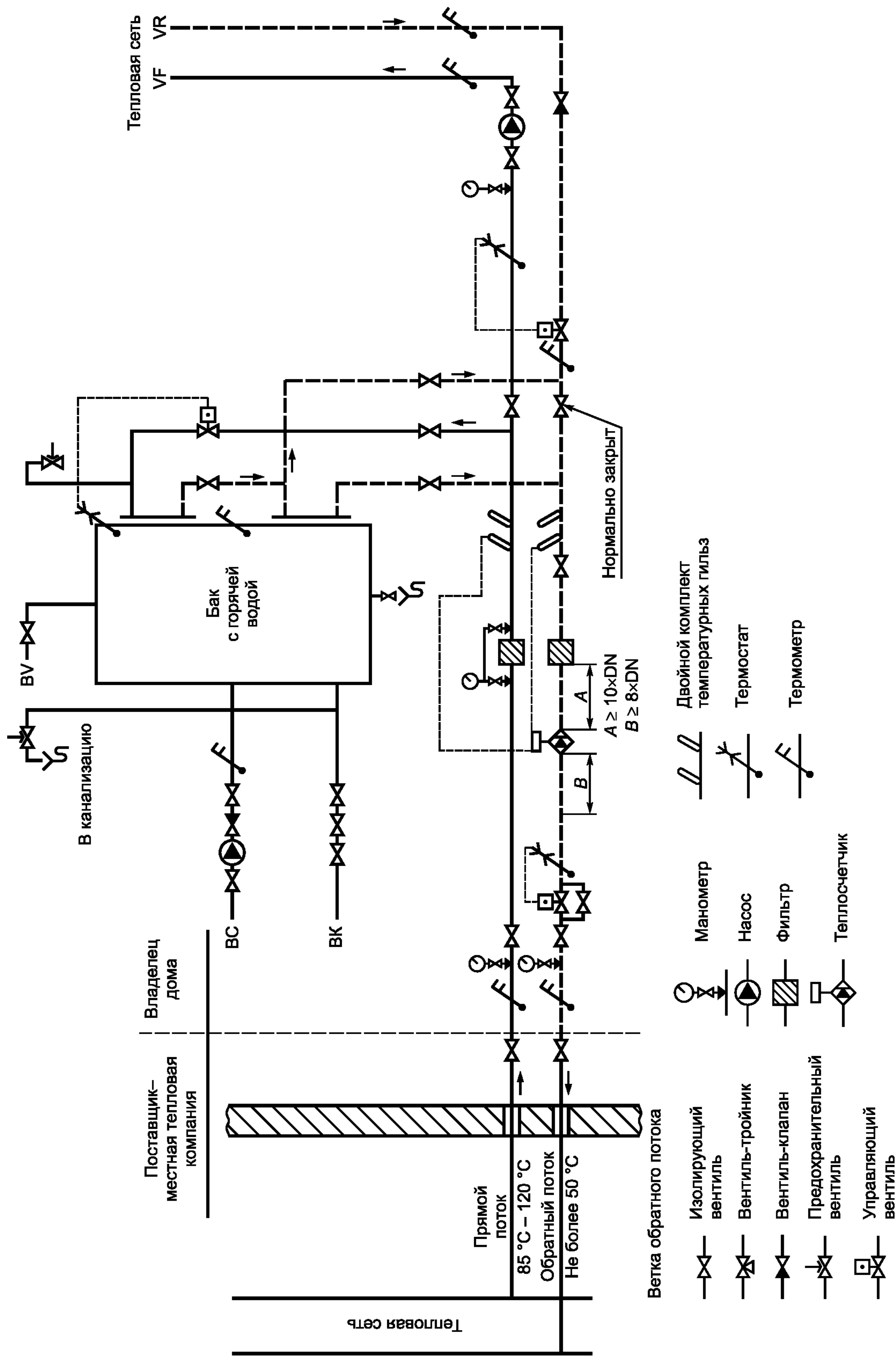
Рисунок А.3 — Отопительная система, прямой тип
