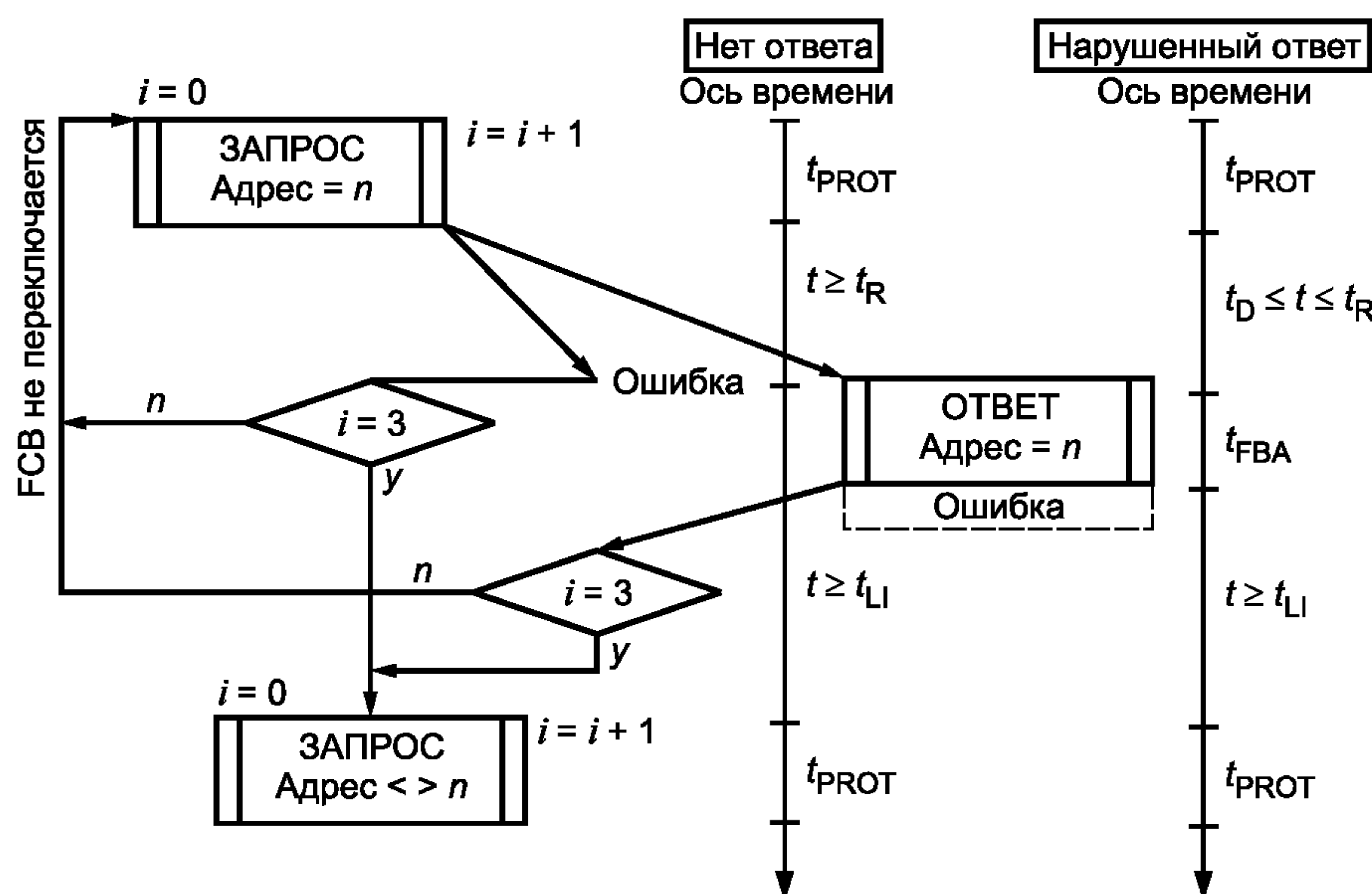
Рисунок 7 — Передача с ошибкой в направлении ответа
