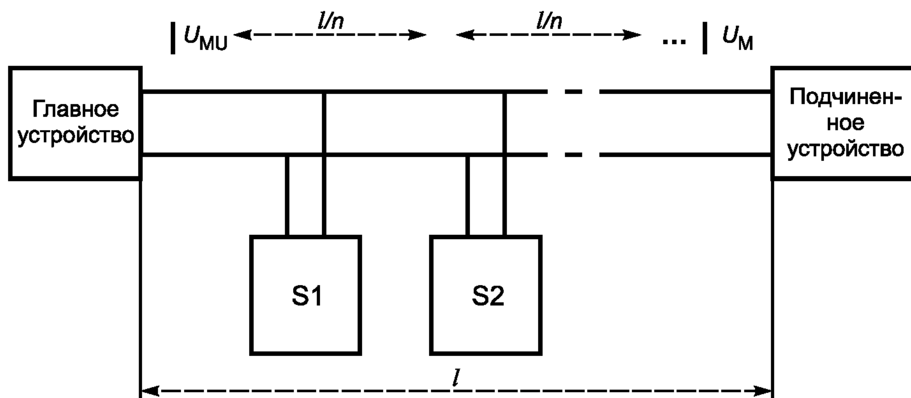
Рисунок В.3 — Тестовое оборудование для M-Bus ( l )
