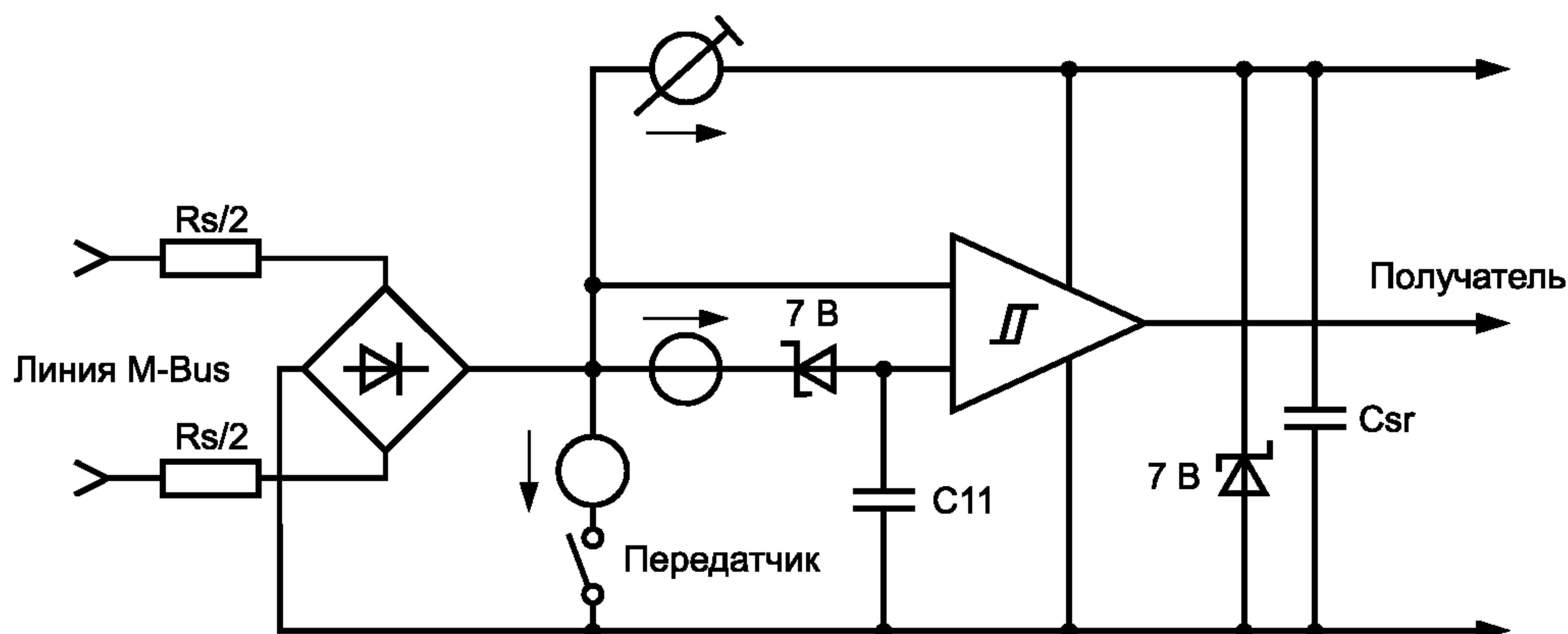
Рисунок 2 — Схема для интерфейса M-Bus
