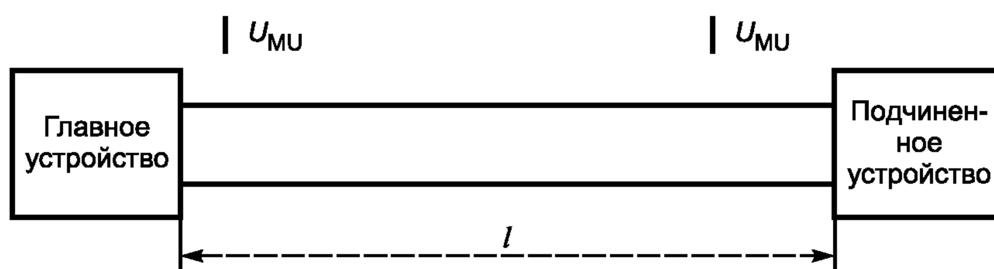
Рисунок В.2 — Тестовое оборудование для M-Bus ( l )
