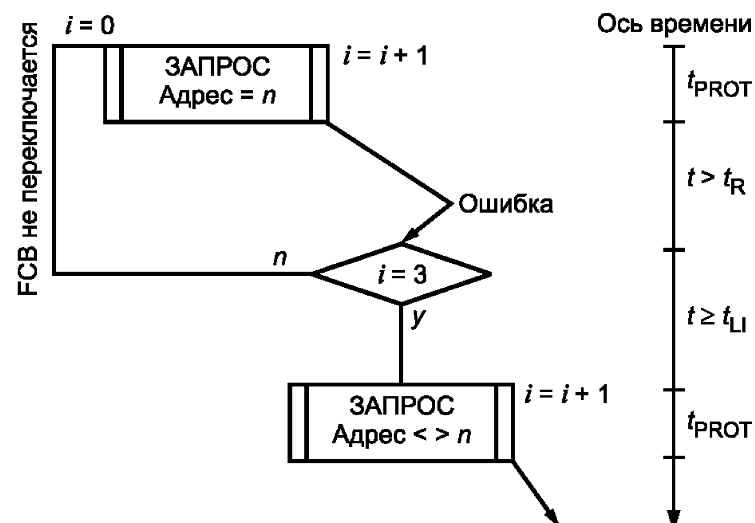
Рисунок 6 — Передача с ошибкой в направлении запроса
