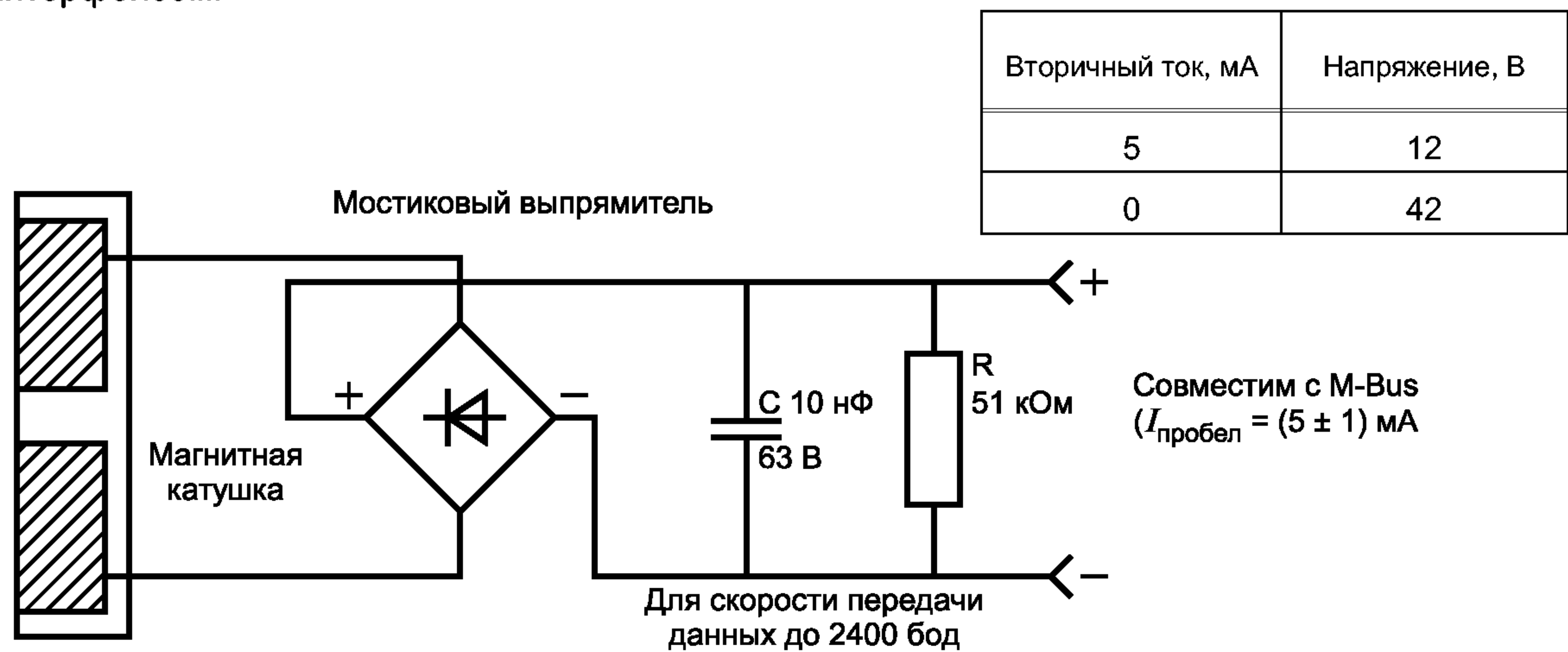
Рисунок 4 — Электрические элементы в теплосчетчике
