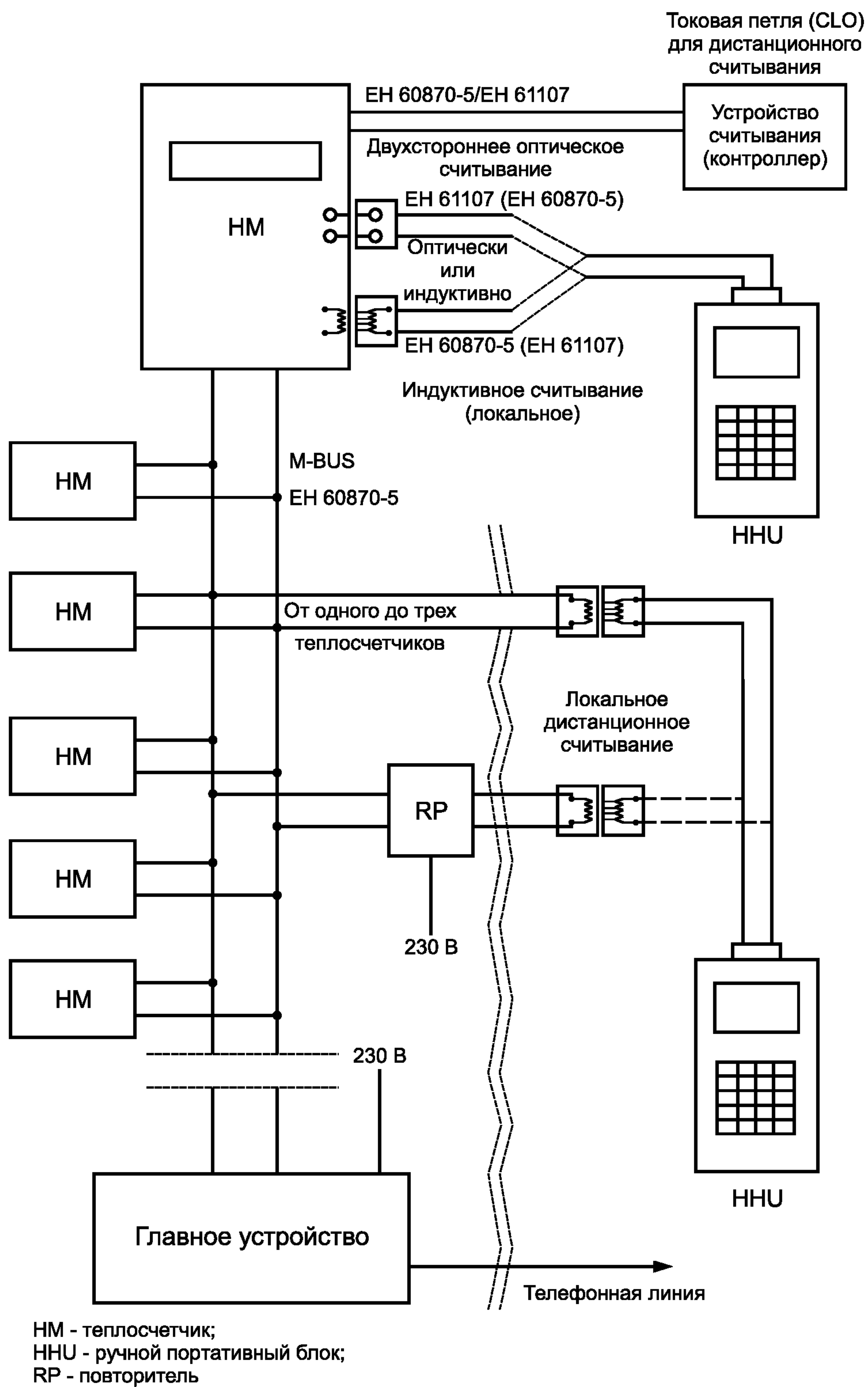
Рисунок 1 — Интерфейсы связи теплосчетчиков
