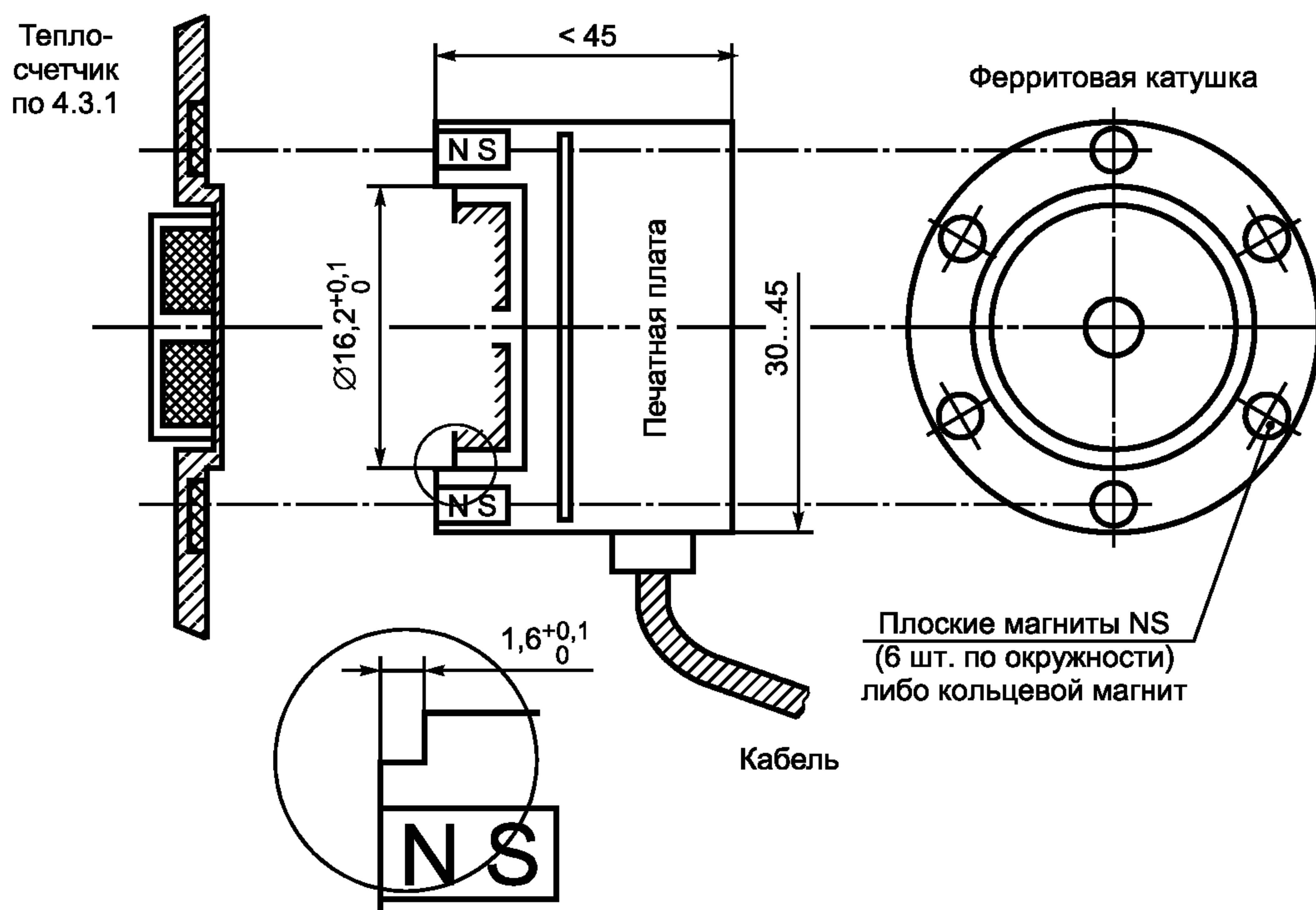
Рисунок D.1 — Расположение компонентов и размеры
