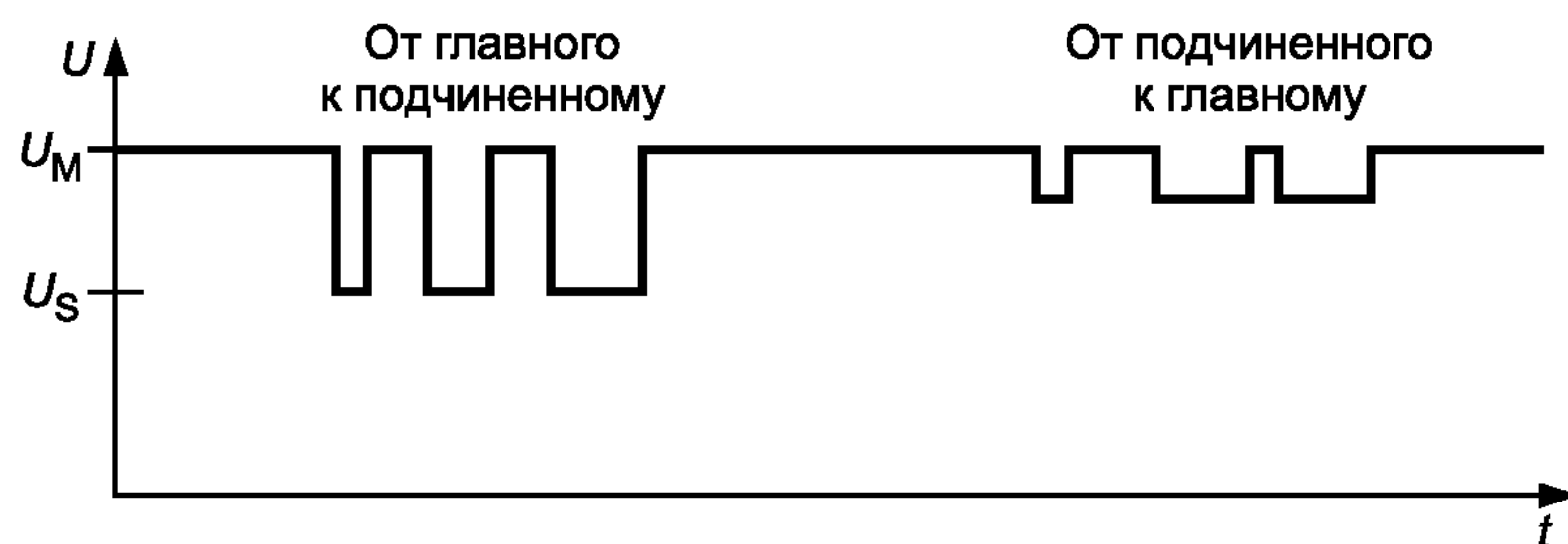
Рисунок В.1 — Зависимость напряжения от времени
