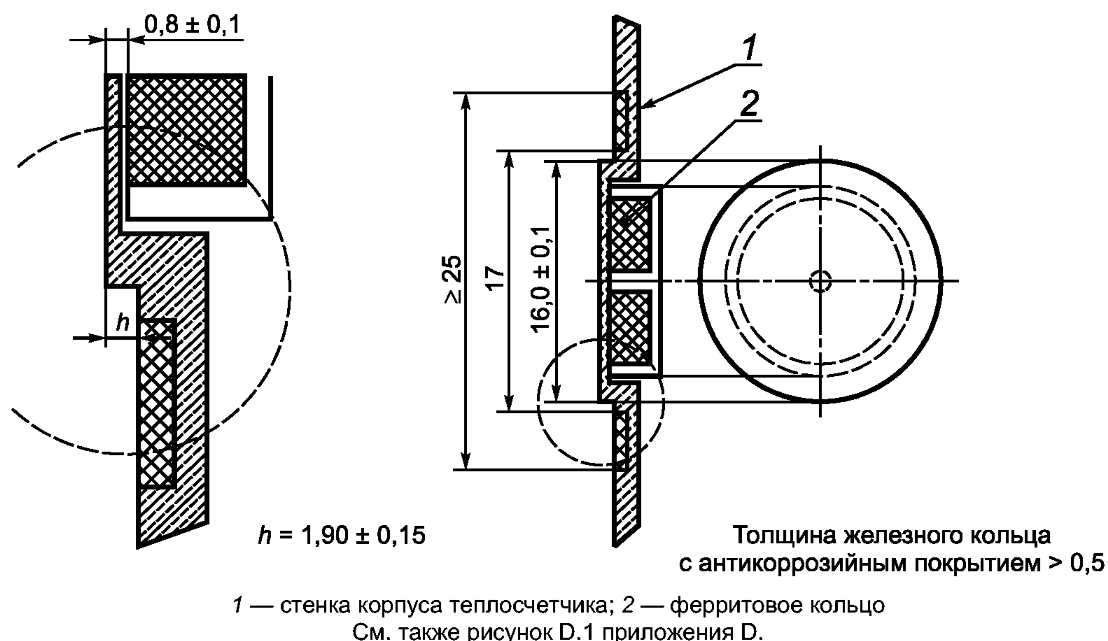
Рисунок 3 — Размеры индуктивного интерфейса в теплосчетчике
