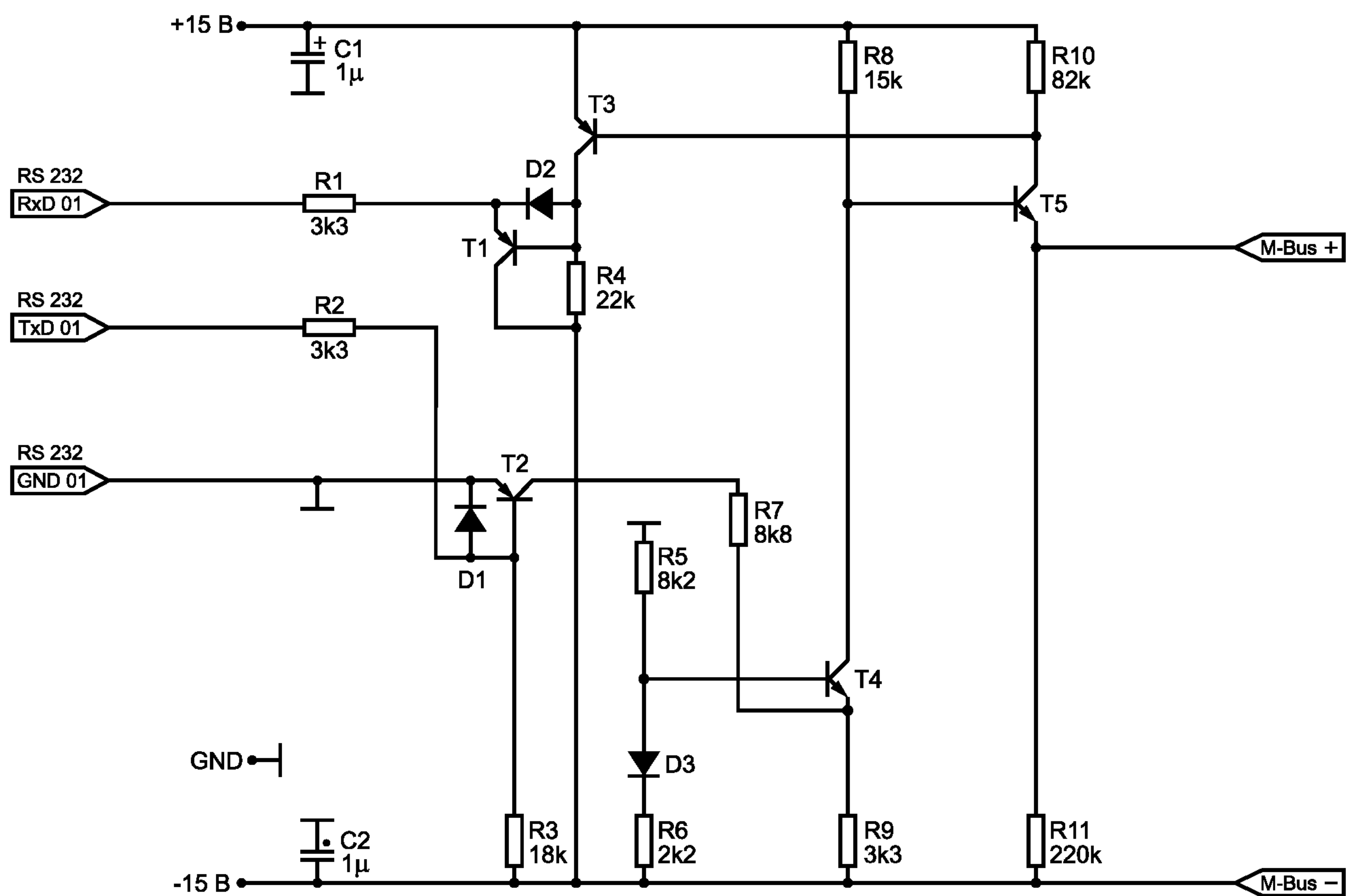
Рисунок С.1 — Конвертер уровня для главного устройства
