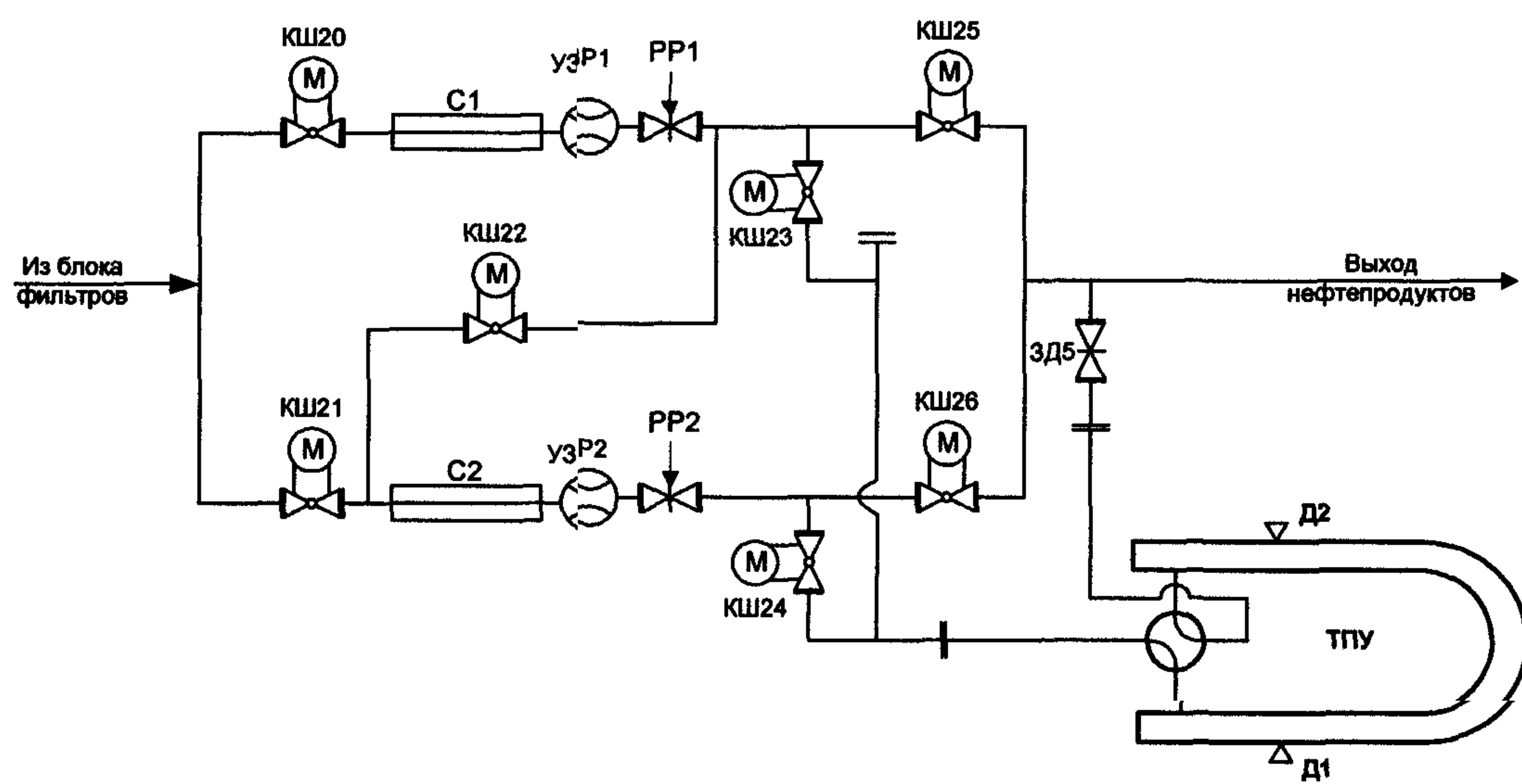
Рисунок Г.1 Принципиальная технологическая схема УУНП
