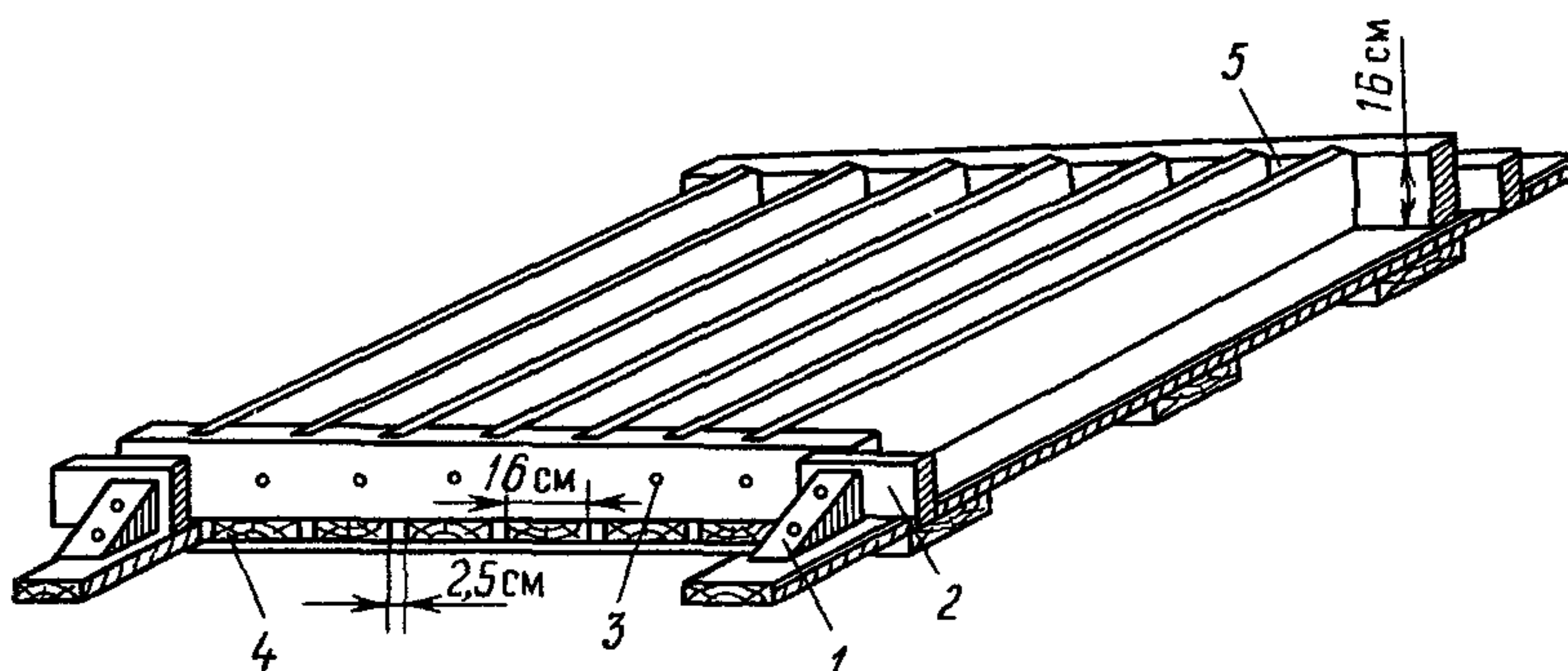
Многоячейковая опалубка.
