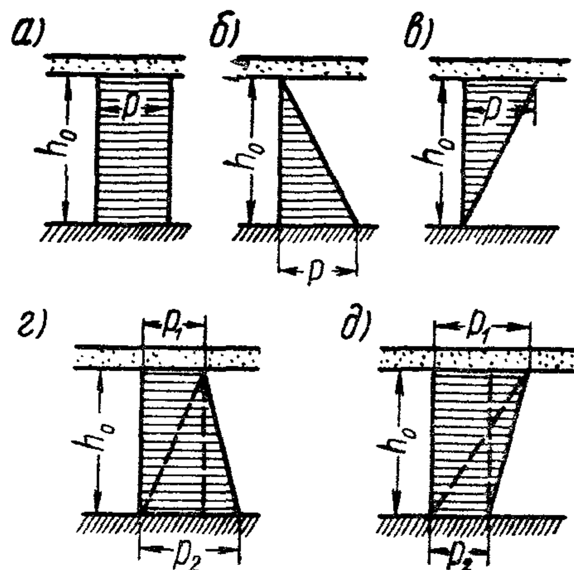
Рис. 7. Эпюры уплотняющих давлений
