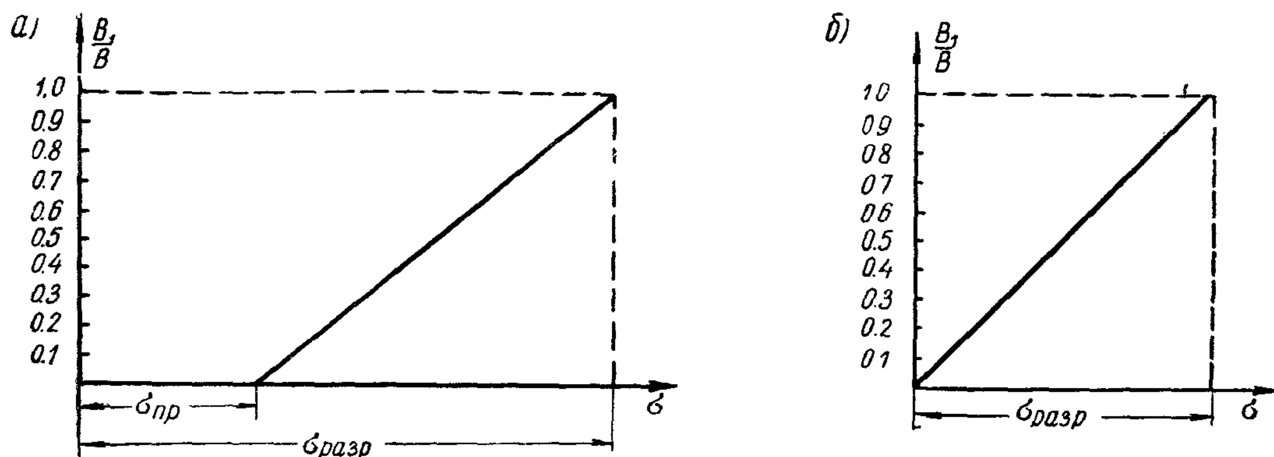
Рис. 3. Графики для определения ширины участка подошвы фундамента B_1 , на котором имеет место сдвиг с выпором грунта основания
