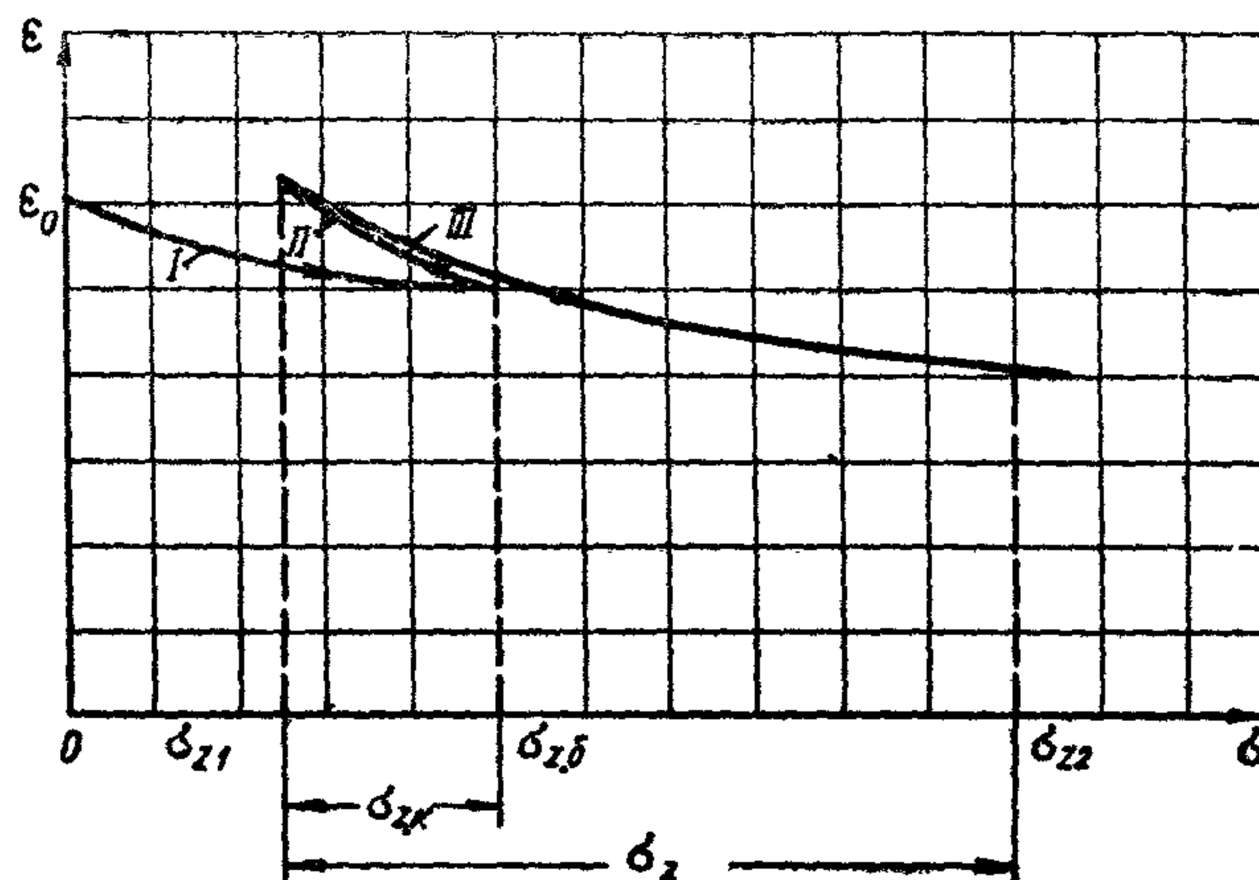
Рис. 2. Компрессионная кривая по опыту по схеме II
