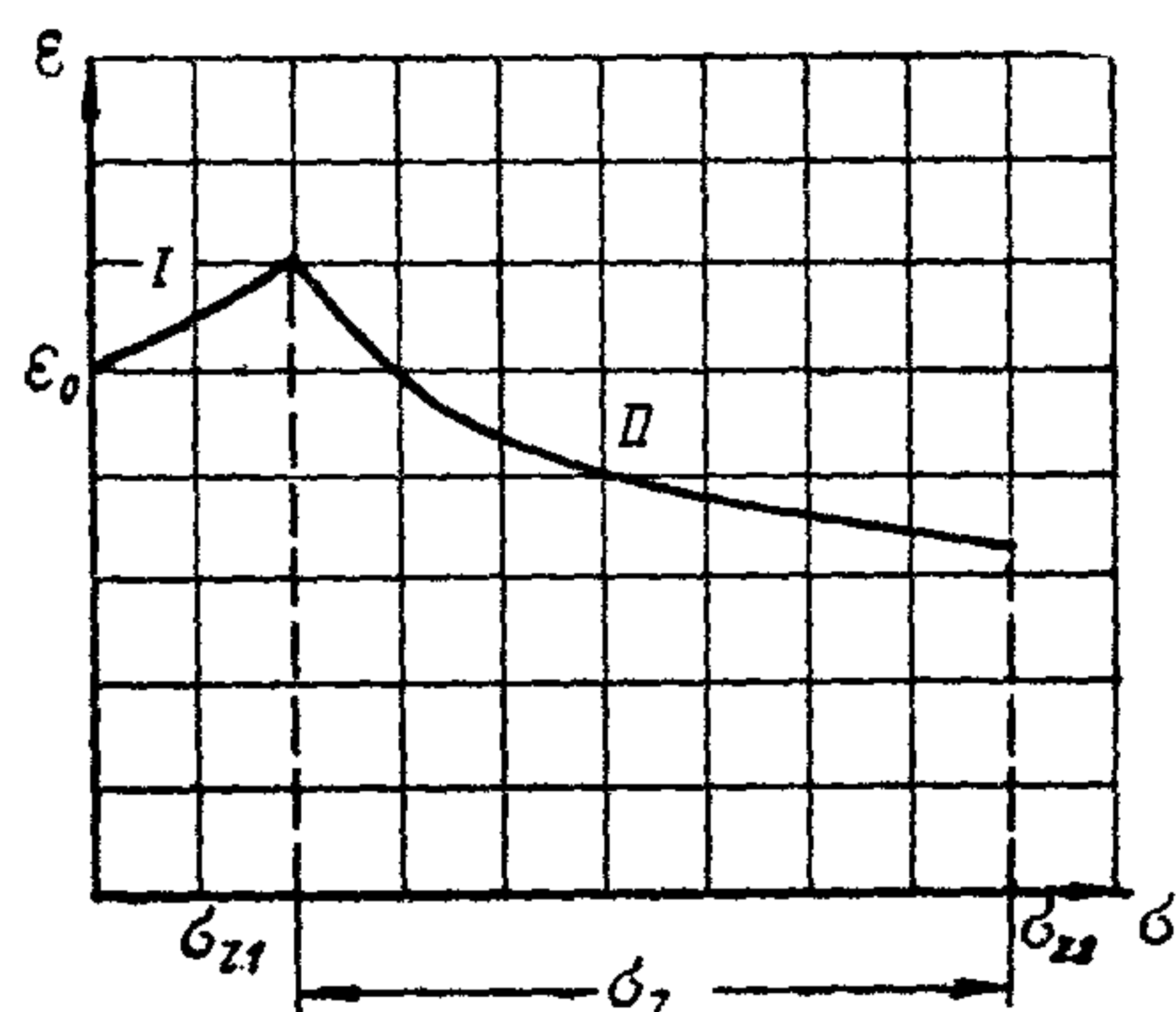
Рис. 1. Компрессионная кривая по опыту по схеме I
