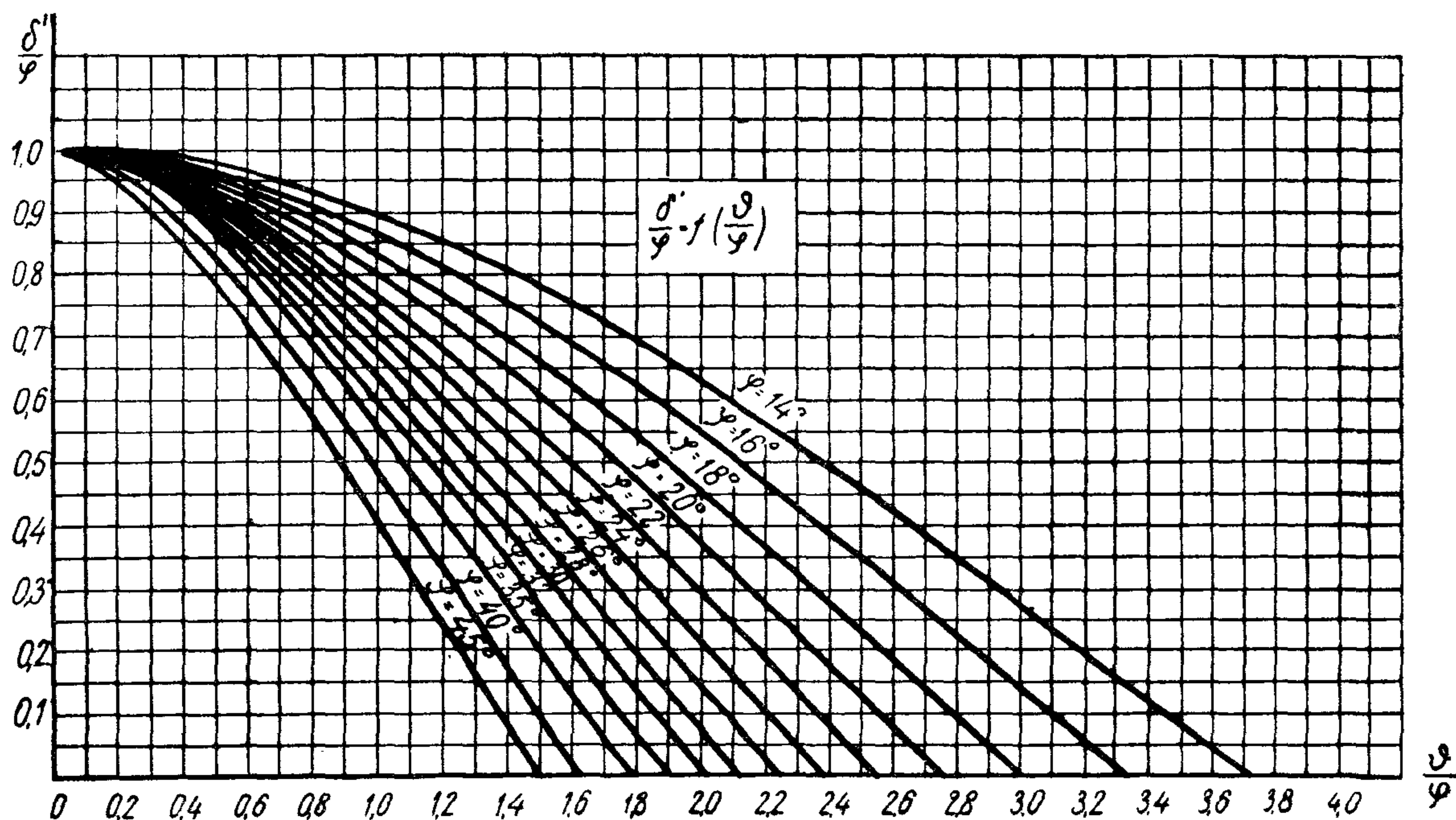
Рис. 2. График зависимости \frac{\delta'}{\varphi} = f\left(\frac{\vartheta}{\varphi}\right)
