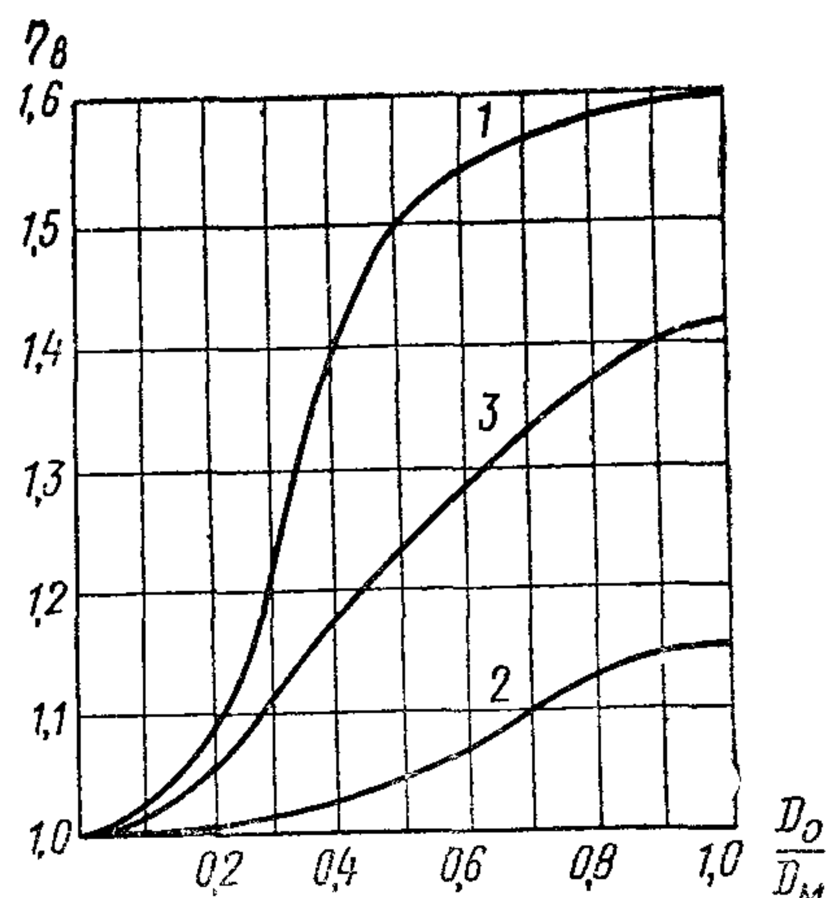
График для определения коэффициента несущей способности тройников
