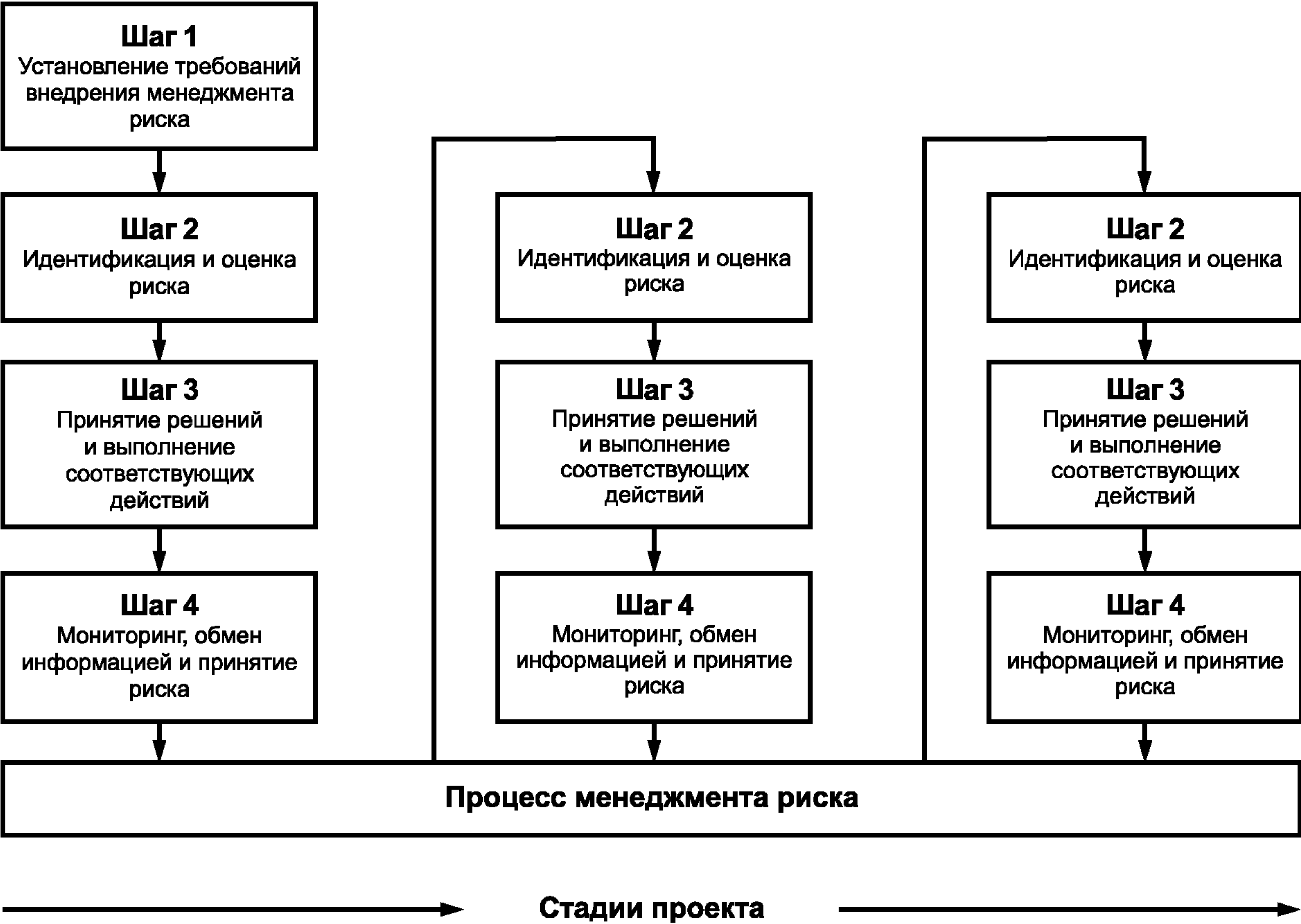
Рисунок 1 — Шаги и циклы процесса менеджмента риска
