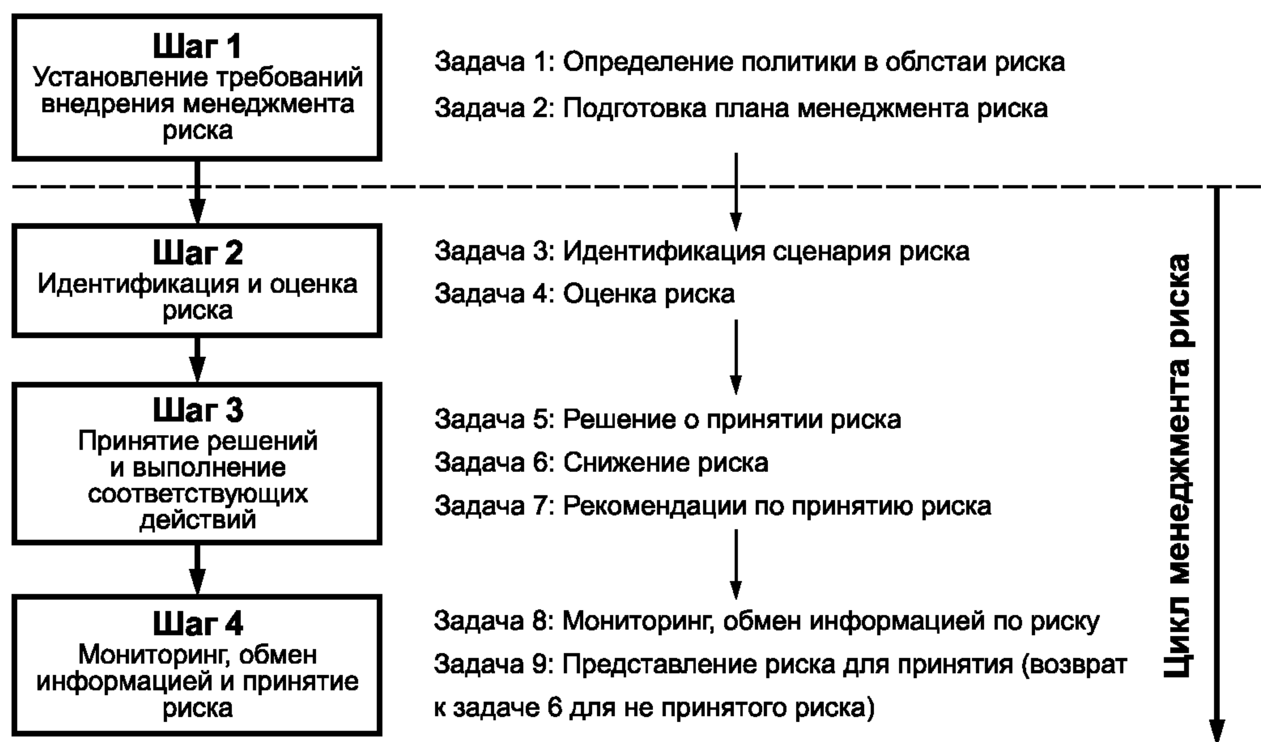
Рисунок 2 — Задачи, соответствующие шагам процесса менеджмента риска в пределах цикла менеджмента риска
