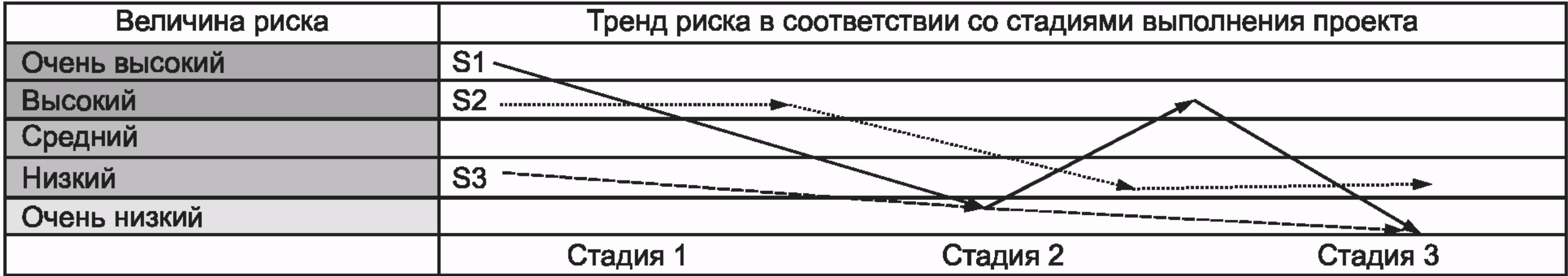
Рисунок 7 — Пример изображения тренда риска
