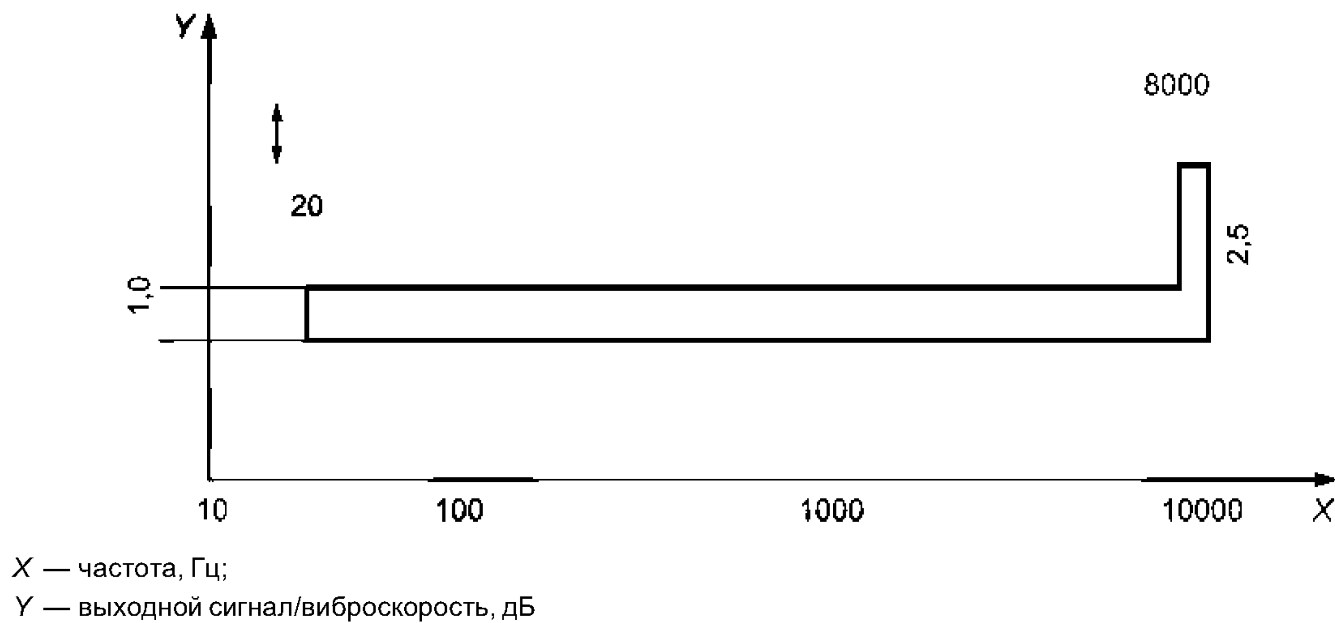
Рисунок 3 — Поле допуска АЧХ вибропреобразователя
