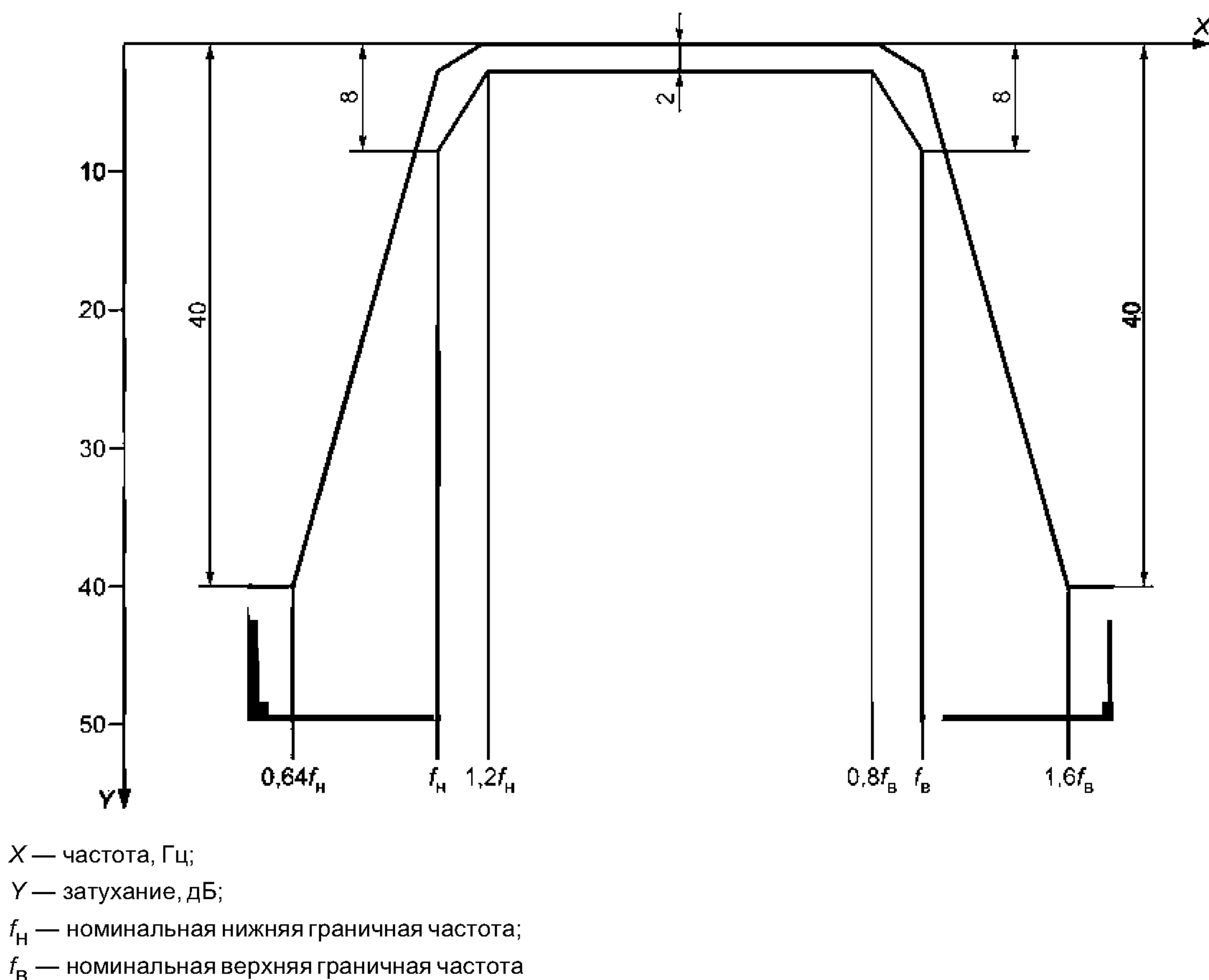
Рисунок 4 — Поле допуска АЧХ полосовых фильтров
