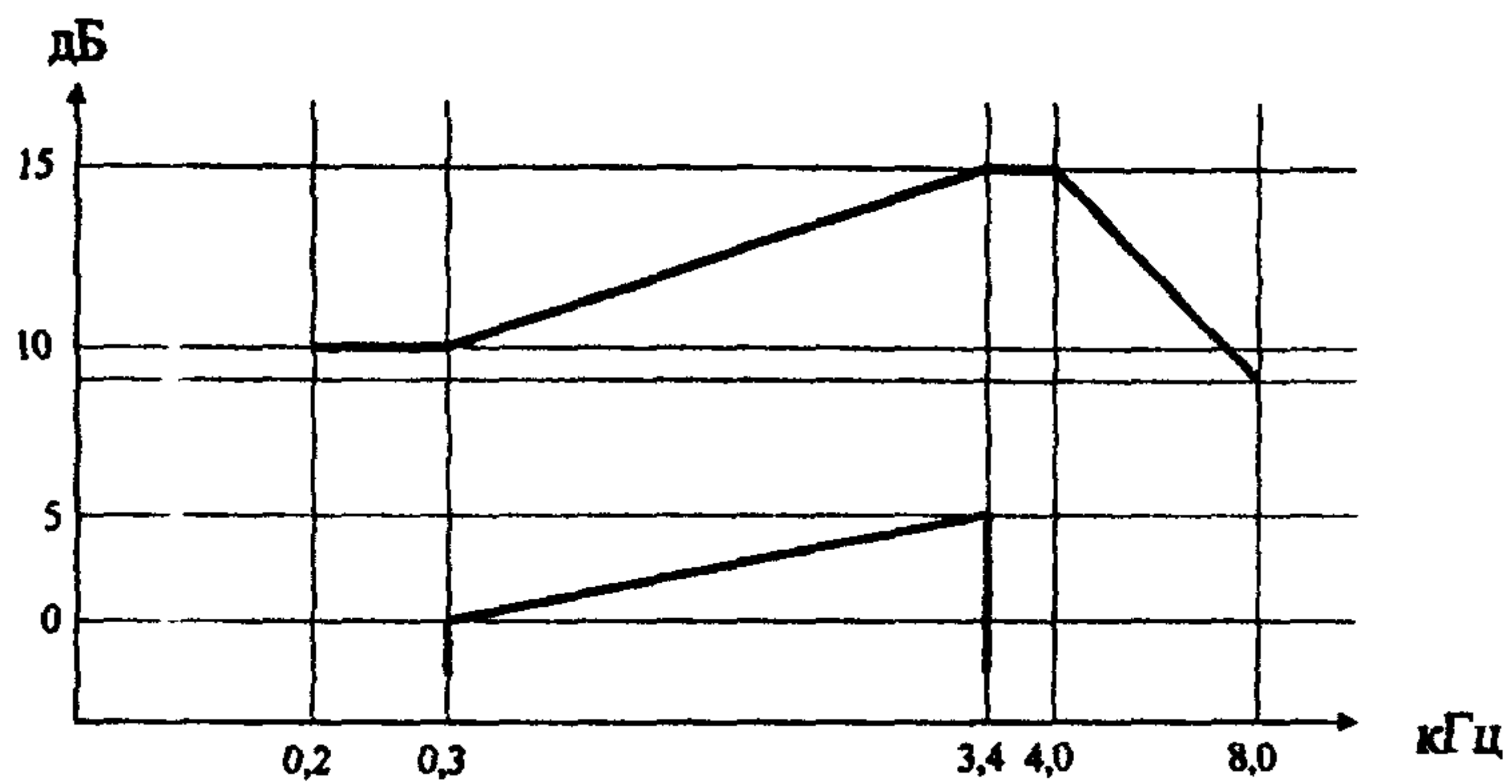
Рисунок 2 - Частотная характеристика коэффициента передачи
