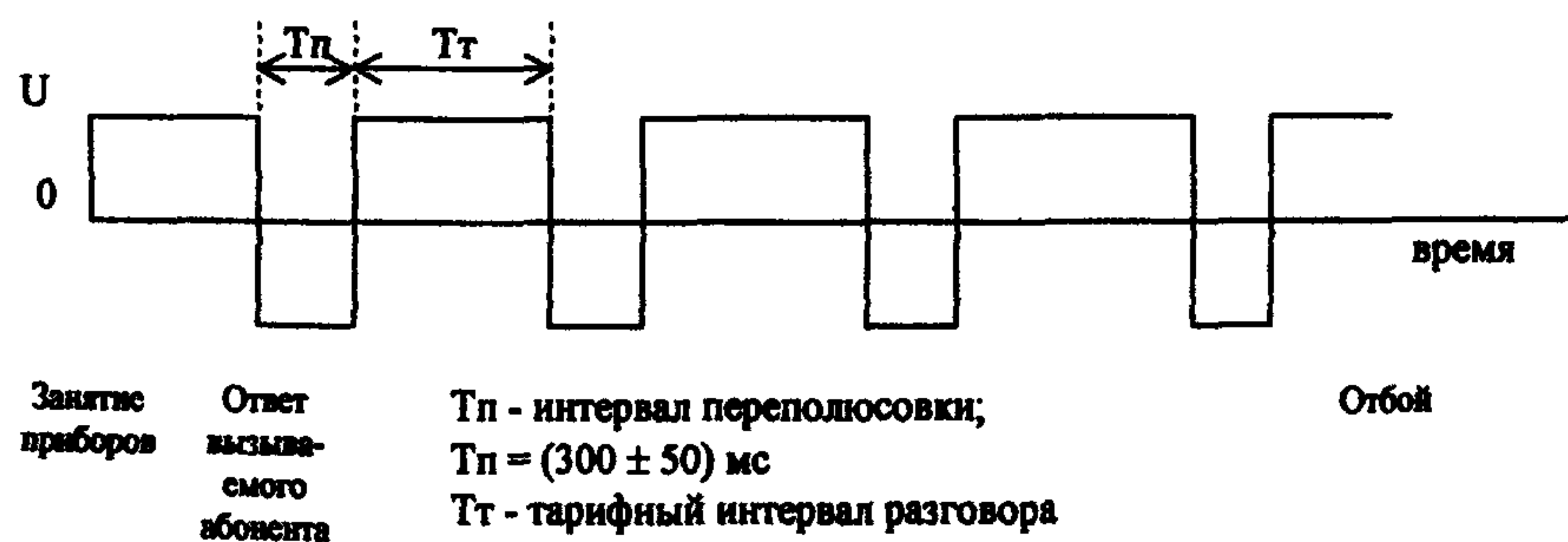
Рисунок 5 - Однократная переполусовка напряжения при ответе вызываемого абонента с многократным восстановлением исходной полярности напряжения при тарификации
