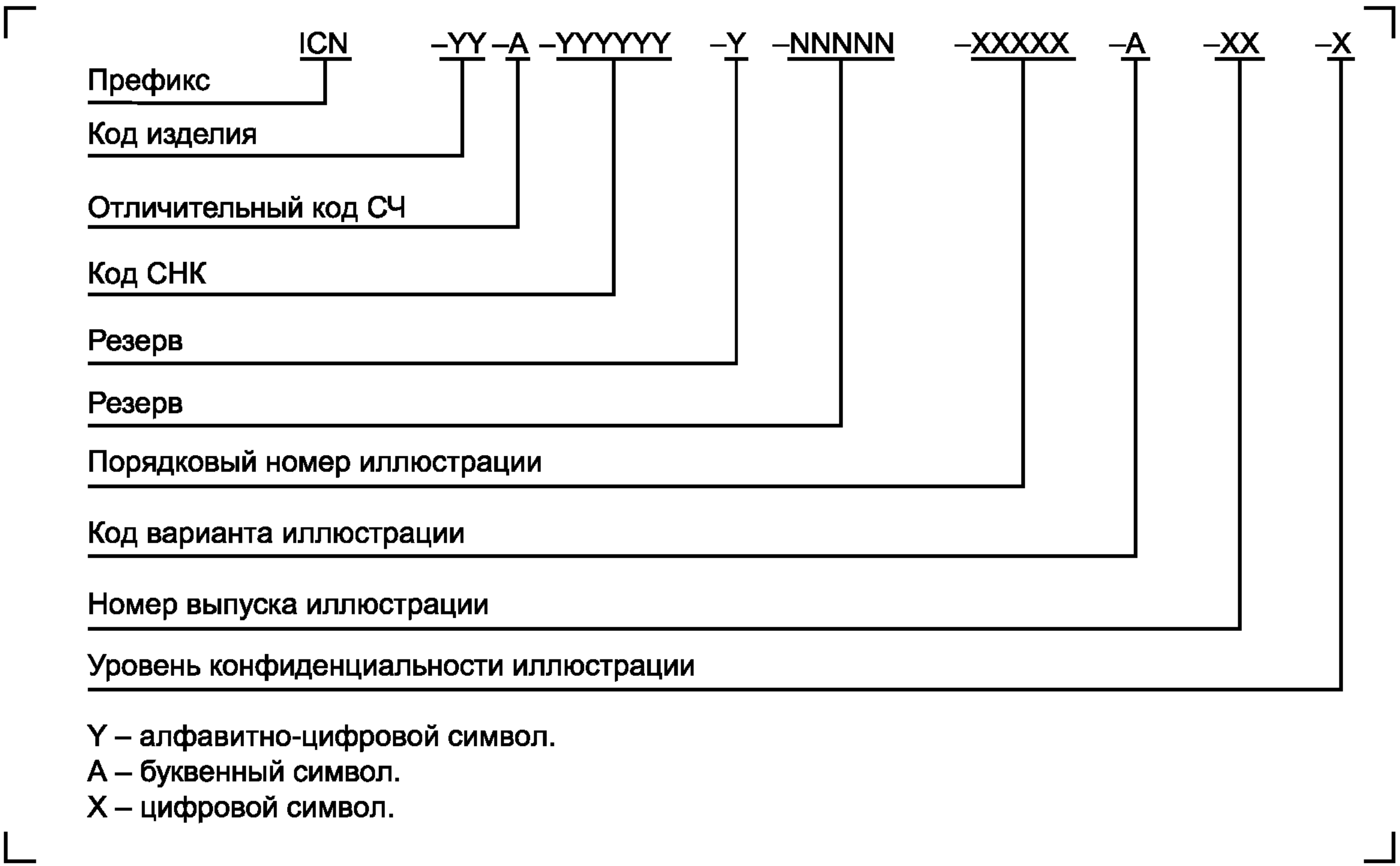
Рисунок Г.2 — Структура обозначения иллюстрации
