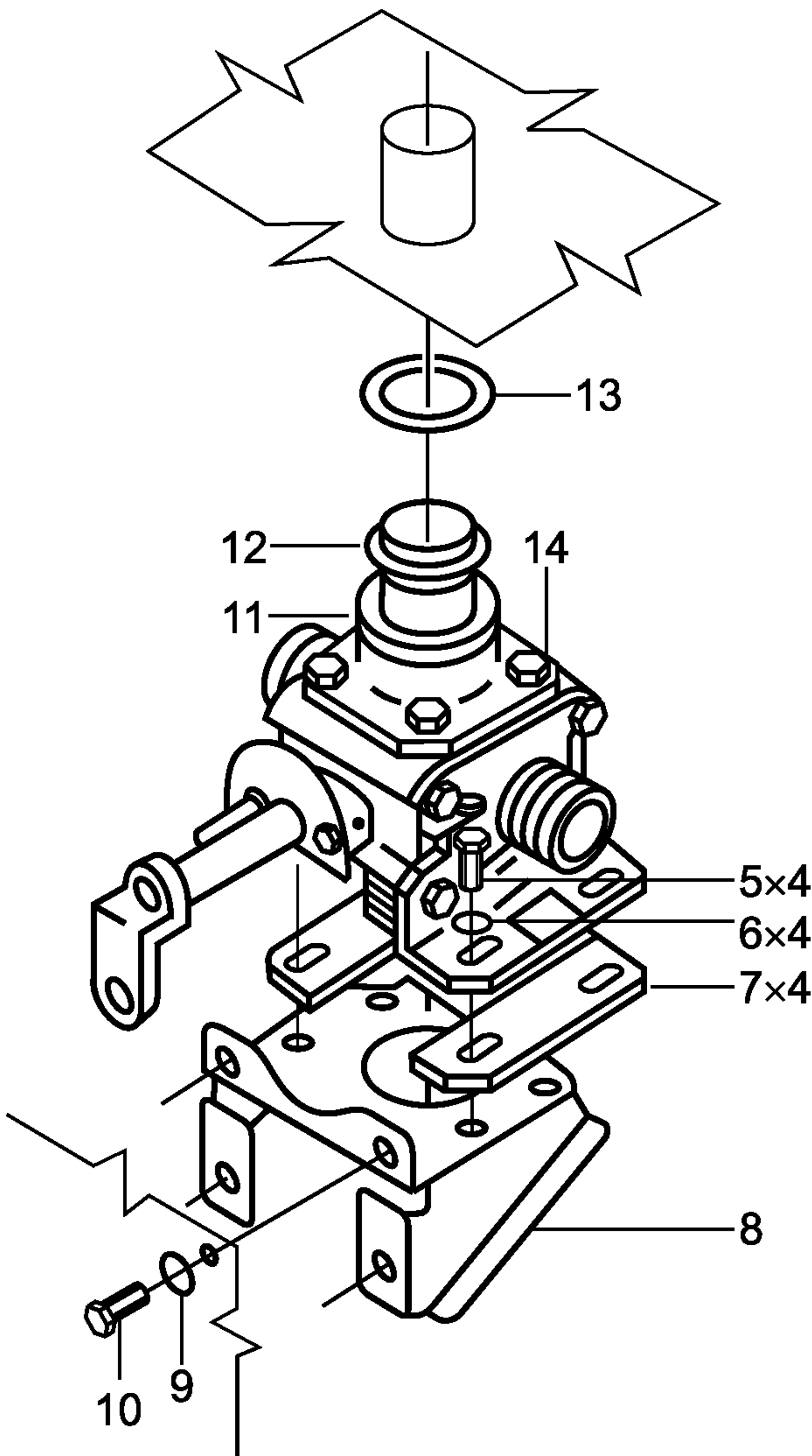
Рисунок А.1 — Пример указания количества одинаковых деталей
