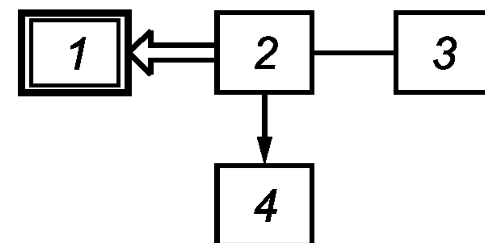
Рисунок 4 — Схема подключения оборудования при проверке пределов и определении погрешности измерения ширины полосы частот
