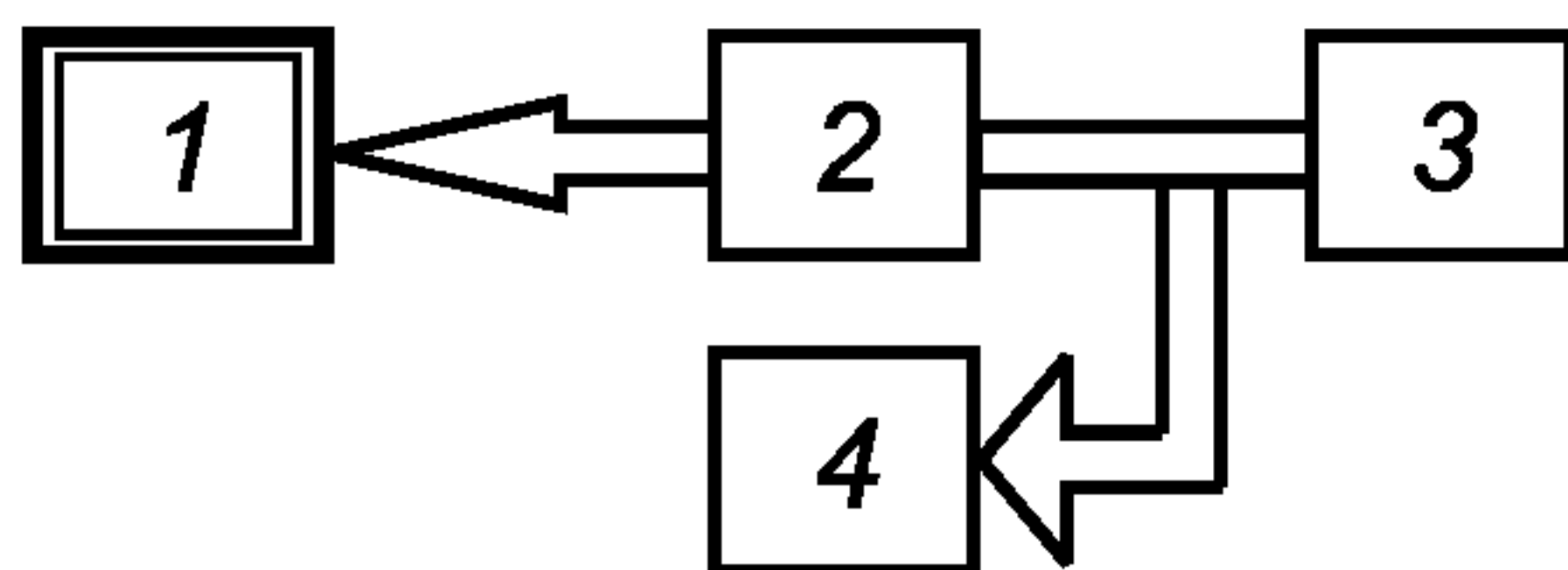
Рисунок 1 — Схема подключения оборудования при определении погрешности измерения частоты
