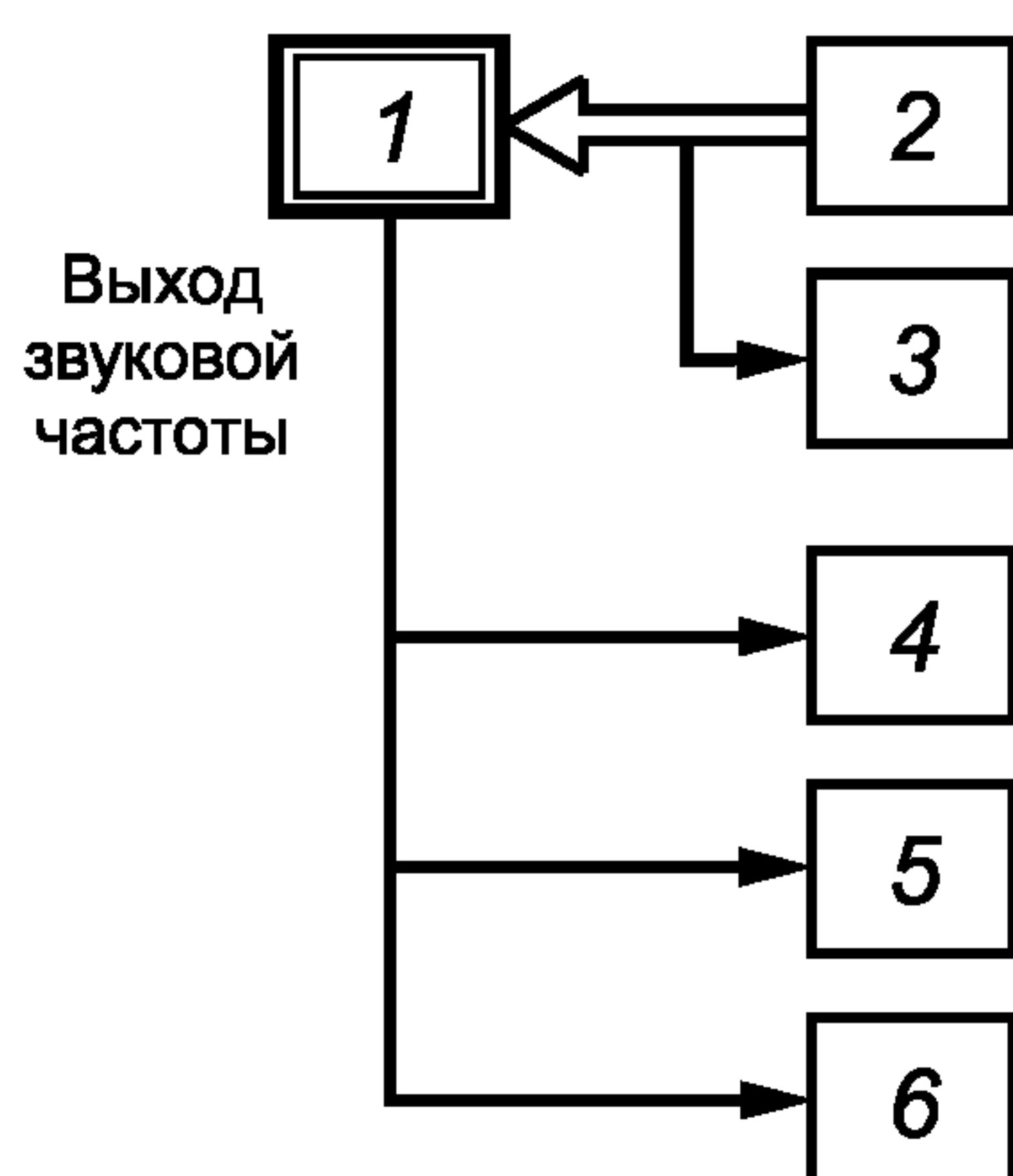
Рисунок 10 — Схема подключения оборудования при определении чувствительности приемника
