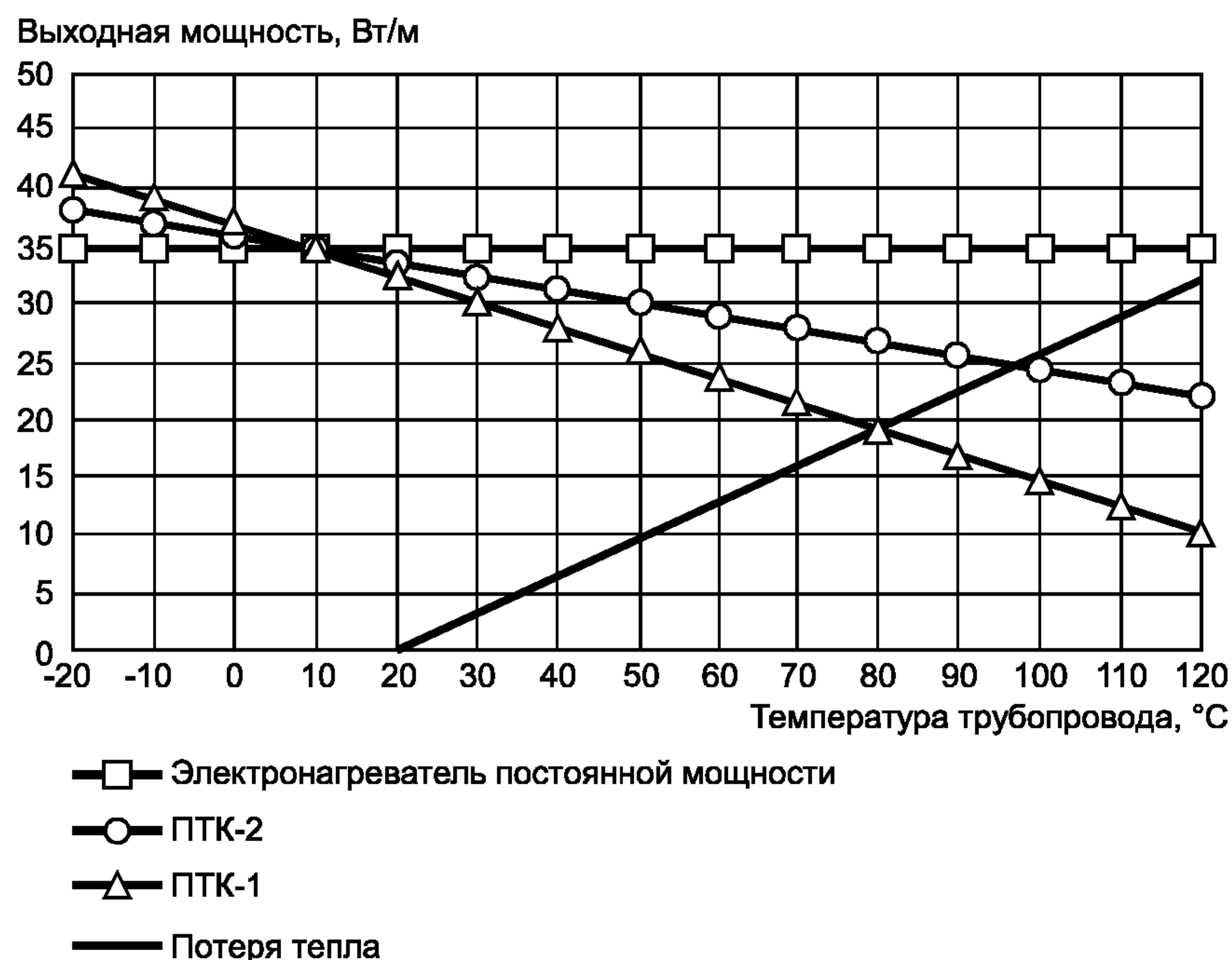
Рисунок 4 — Условия равновесия для оценки верхнего предела
