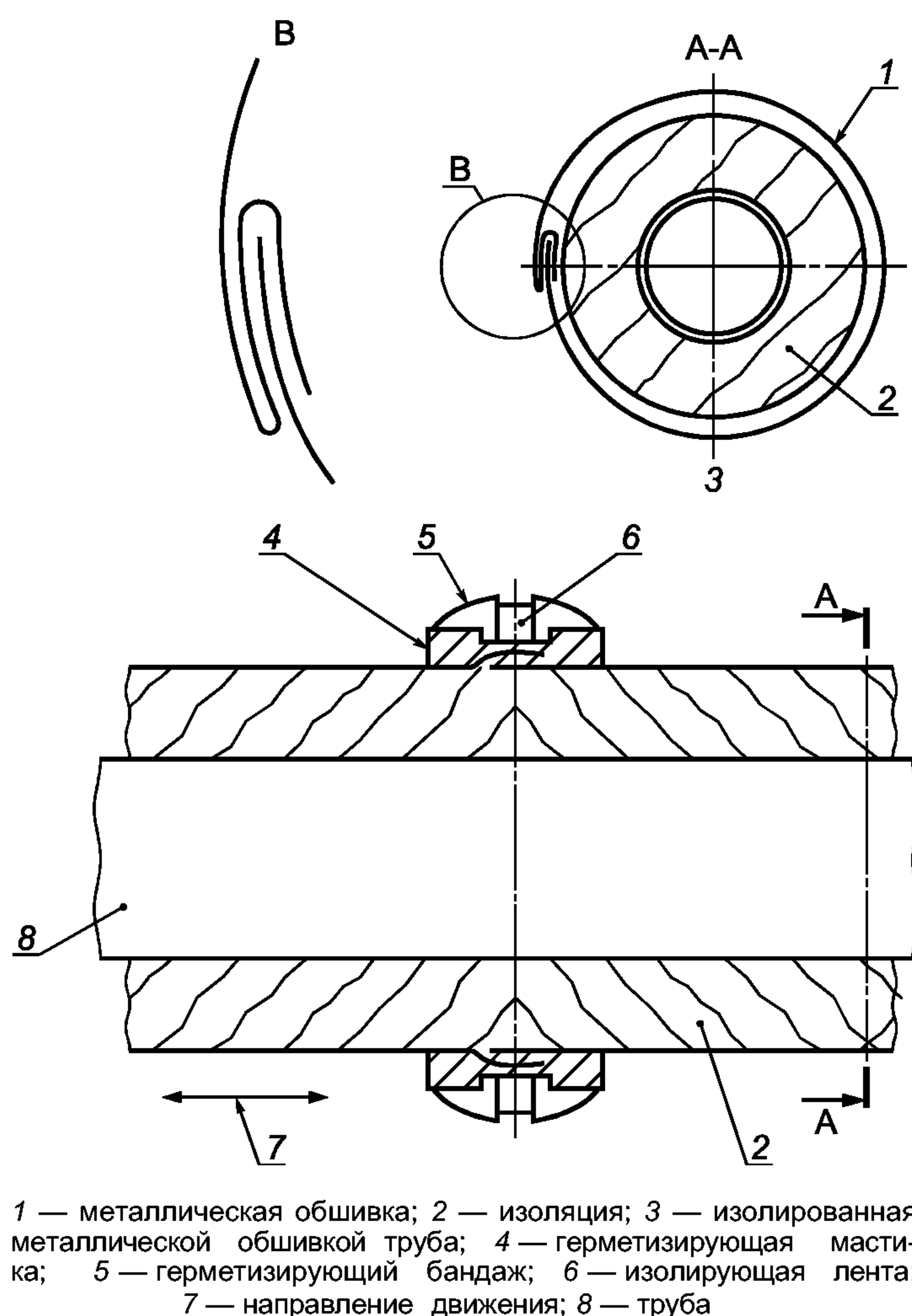
Рисунок 1 — Теплоизоляция: установка климатического барьера
