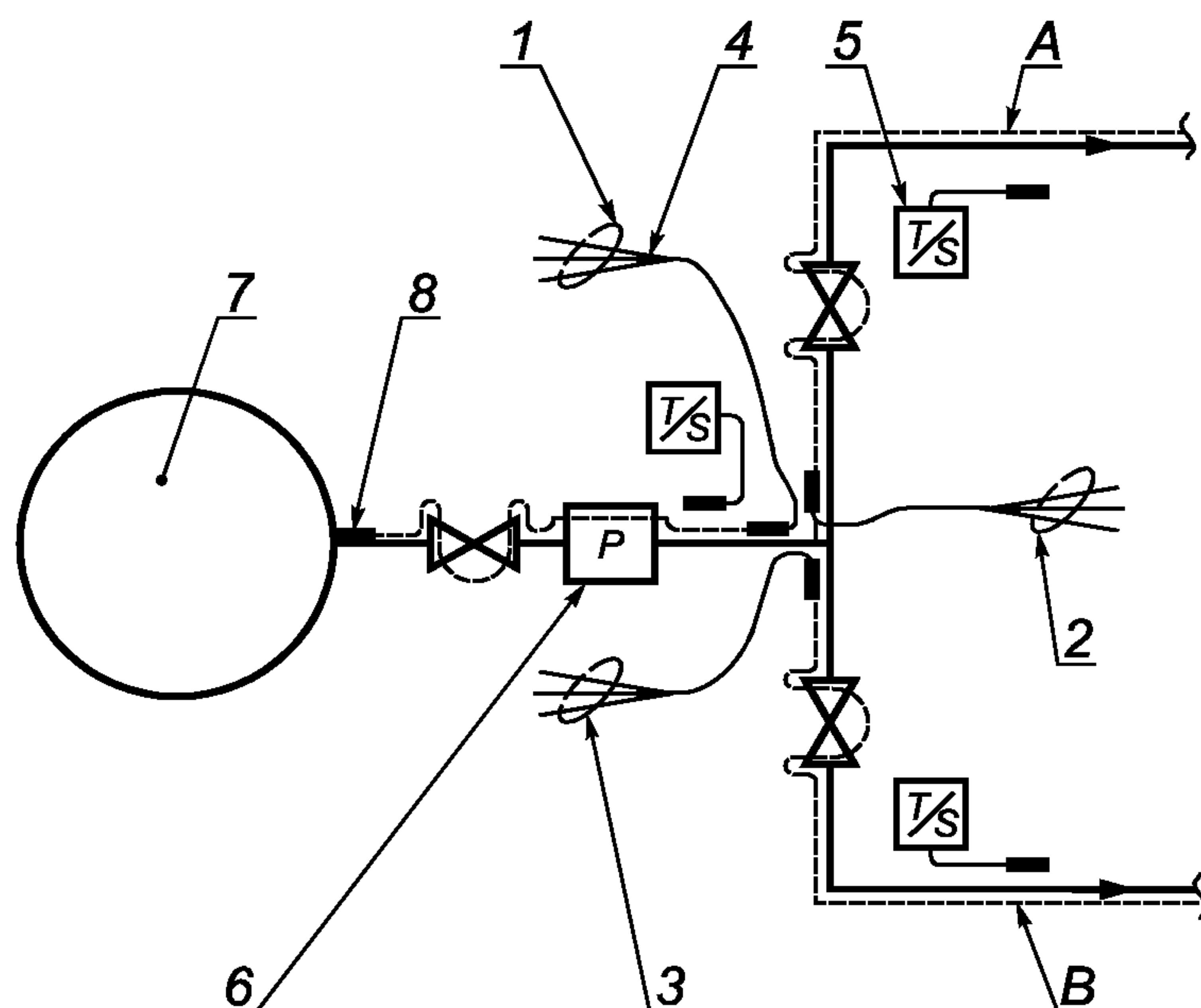
A — труба A; B — труба B; 1 — цепь № 1; 2 — цепь № 2; 3 — цепь № 3; 4 — заделка холодного конца; 5 — температурный датчик; 6 — насос; 7 — обогреваемый резервуар; 8 — заделка горячего конца
