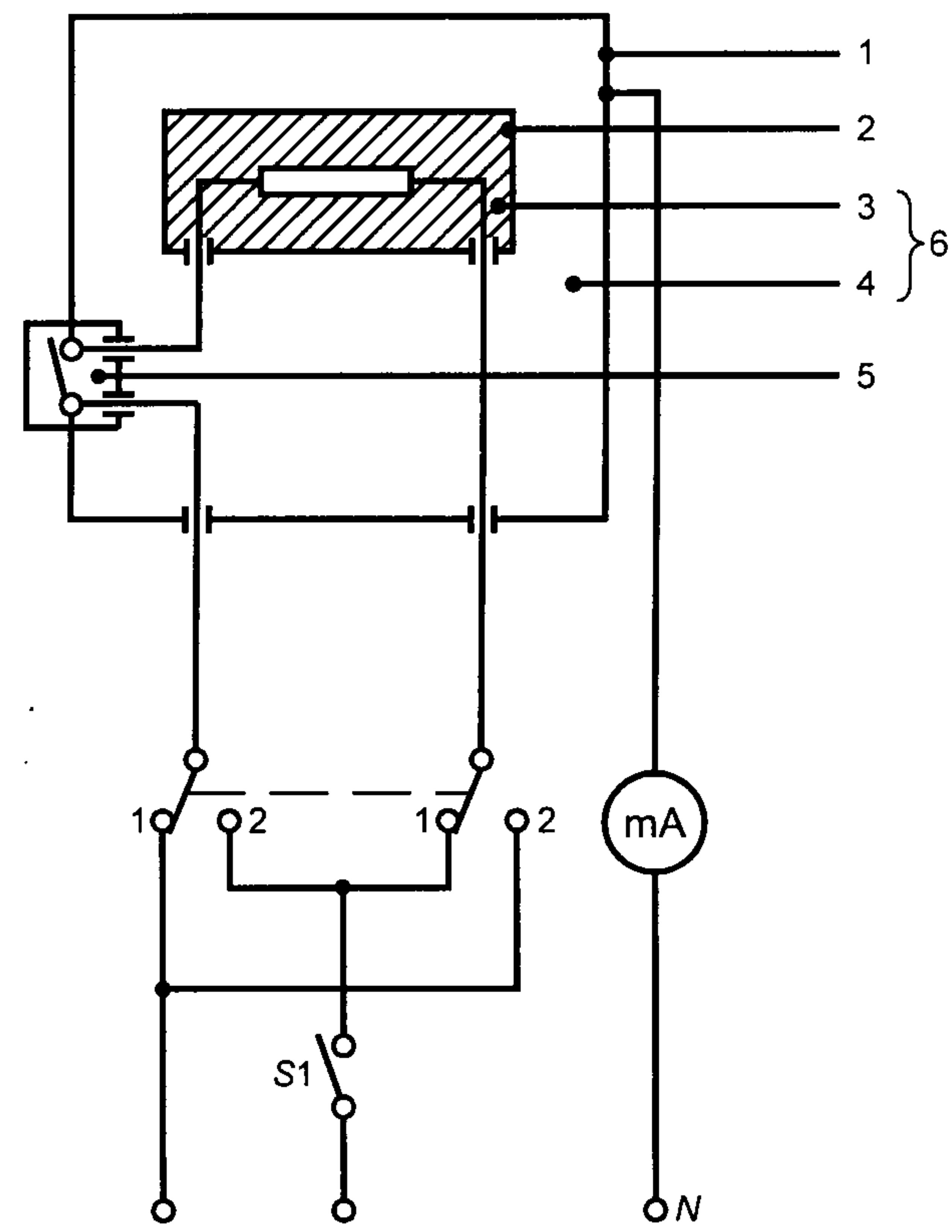
1 — доступная часть; 2 — недоступная металлическая часть; 3 — основная изоляция; 4 — дополнительная изоляция; 5 — усиленная изоляция; 6 — двойная изоляция
