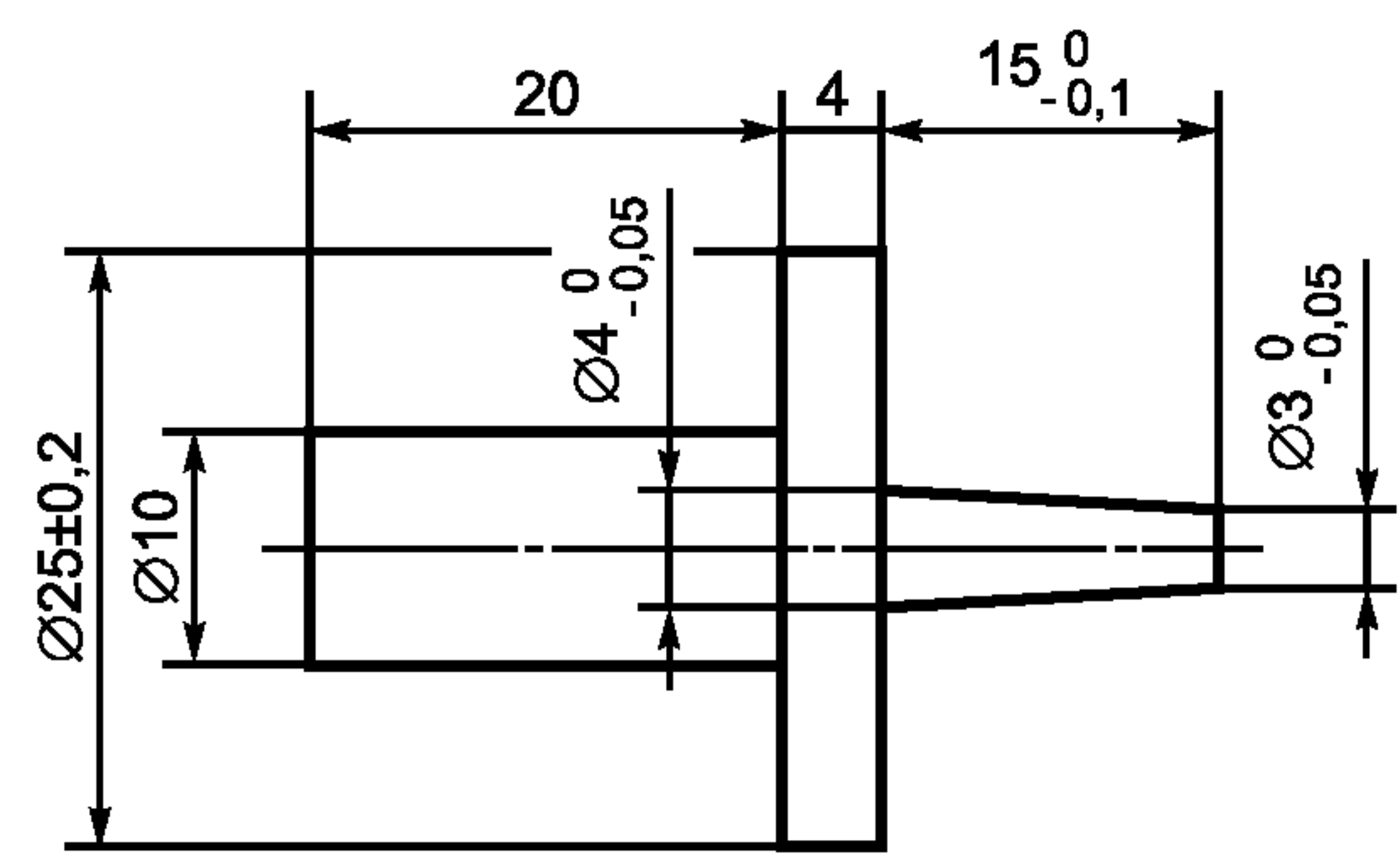
Рисунок 2 — Испытательный щуп
