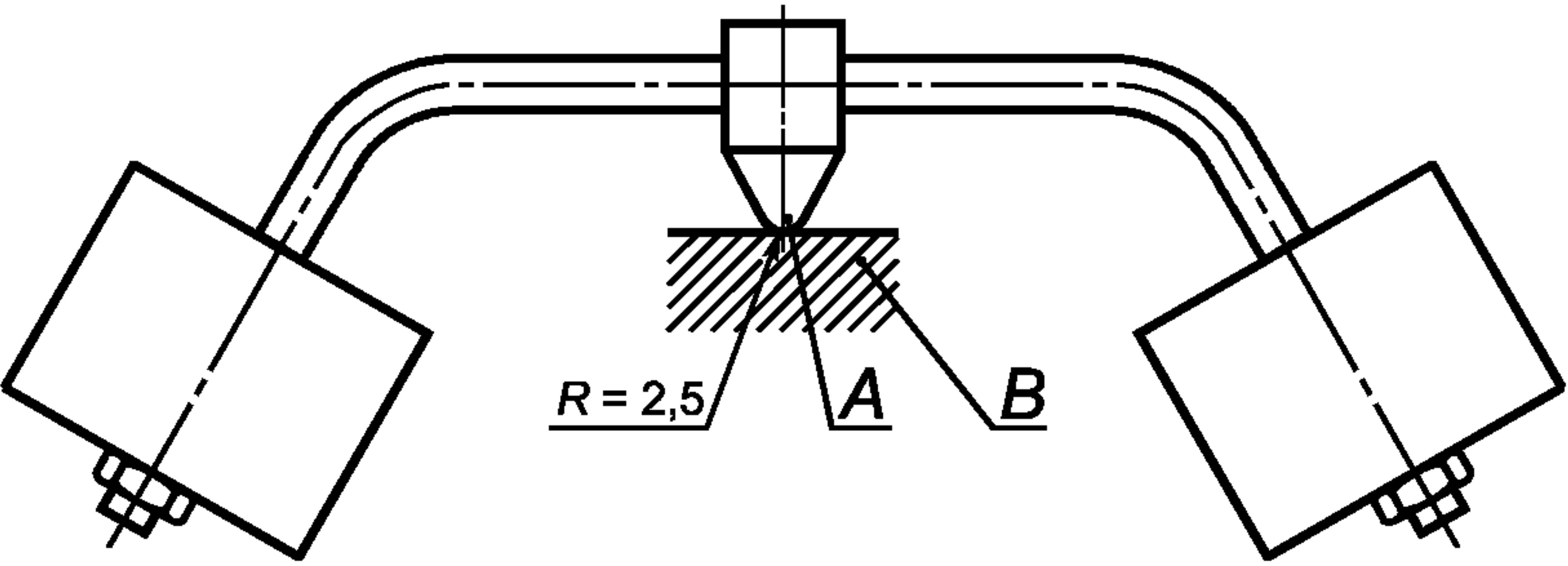
A — сферическая часть; B — испытуемый образец
