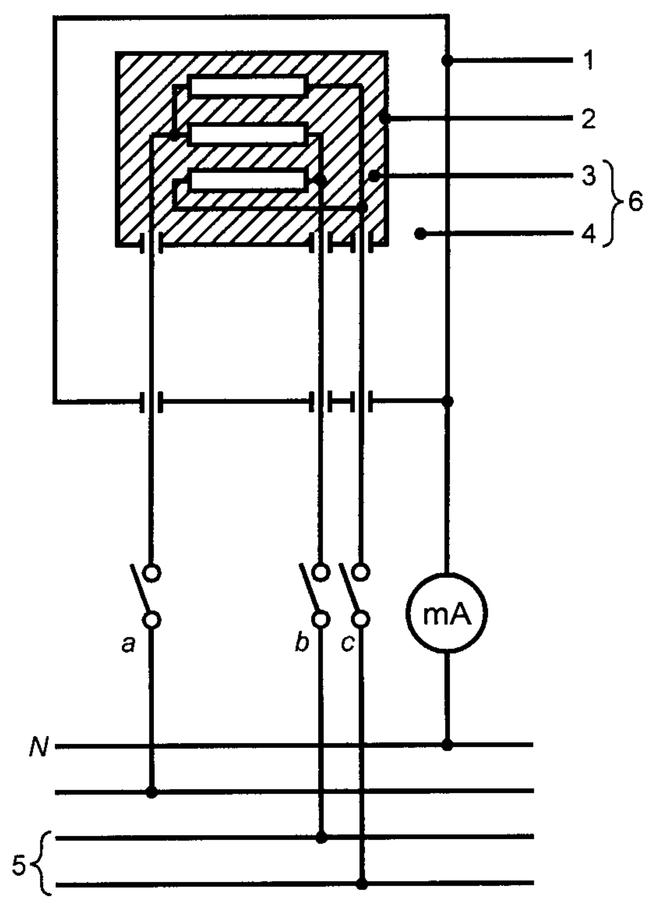
1 — доступная часть; 2 — недоступная металлическая часть; 3 — основная изоляция; 4 — дополнительная изоляция; 5 — трехфазное питание; 6 — двойная изоляция
