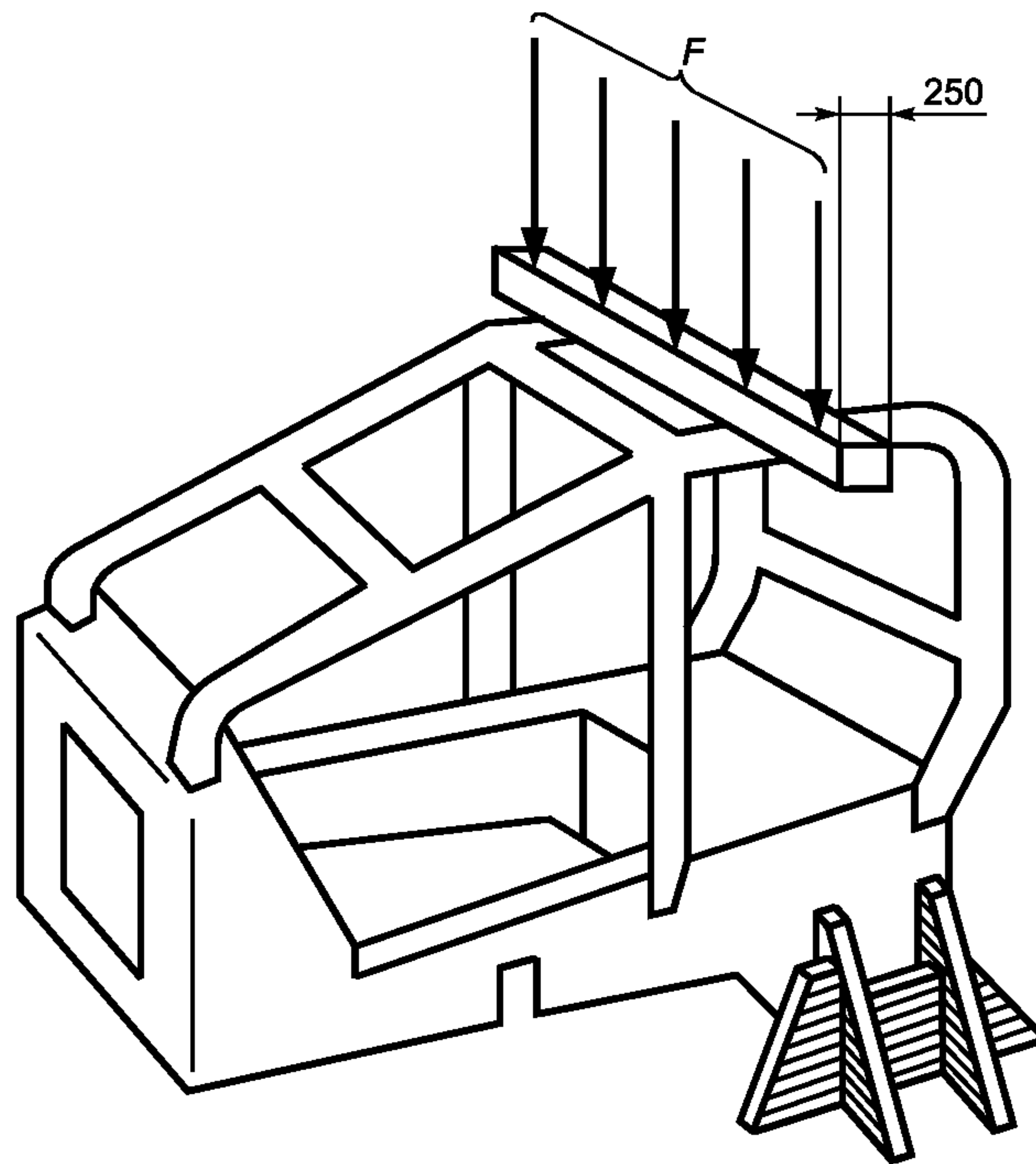
Рисунок 6 — Устройство распределения нагрузки при вертикальном нагружении
