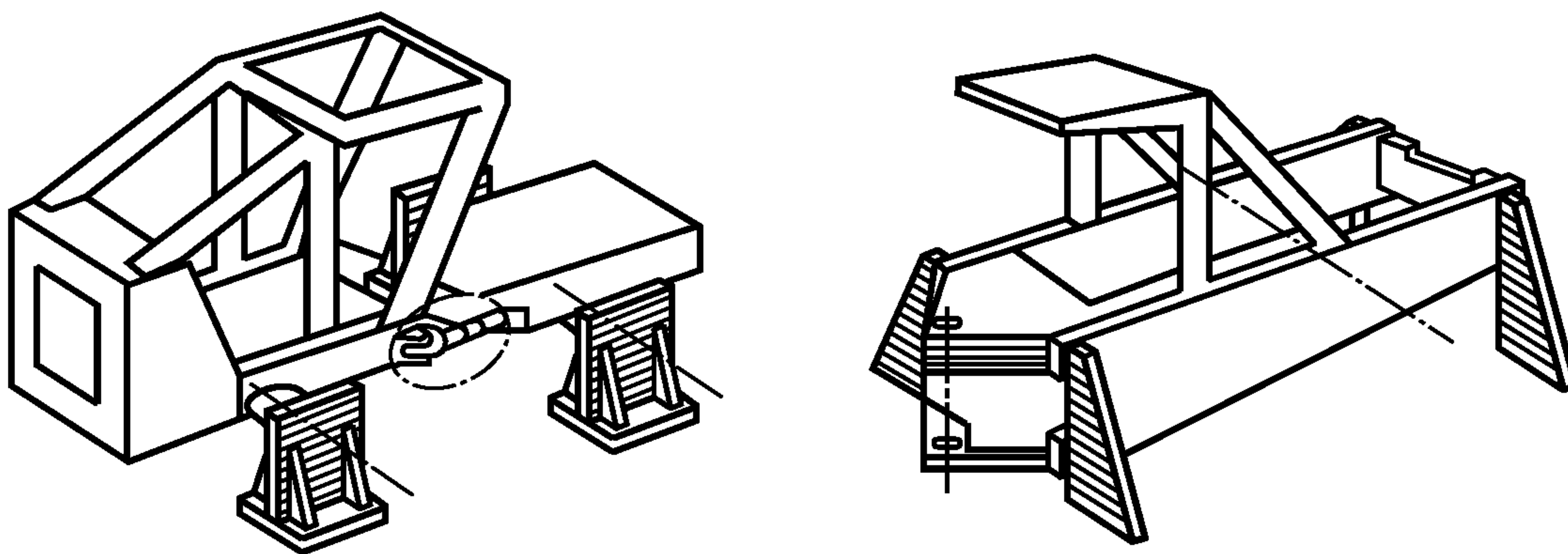
Рисунок 2 — Крепление машины на платформе стенда
