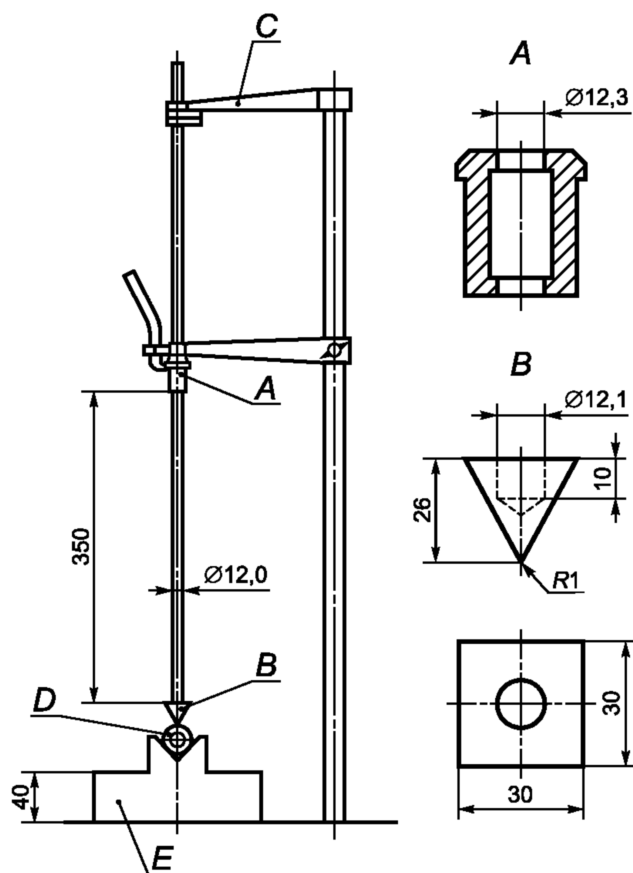
A — груз; B — закаленный стальной резец; C — фиксирующий кронштейн; D — образец; E — основание массой 10 кг
