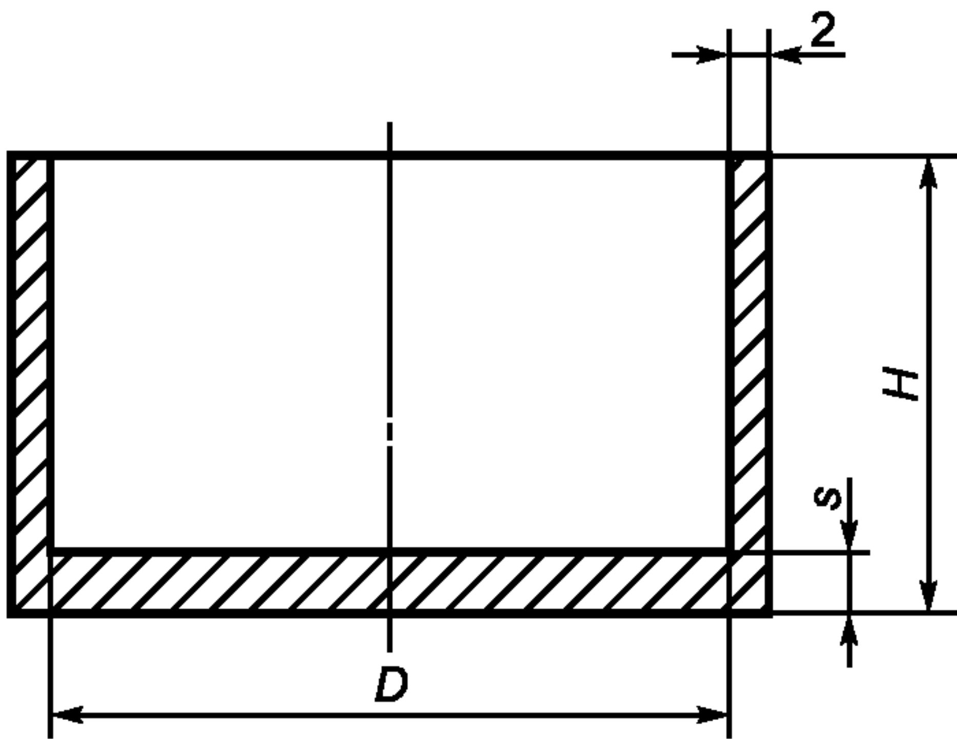
D — наружный диаметр; H — высота; s — толщина дна
