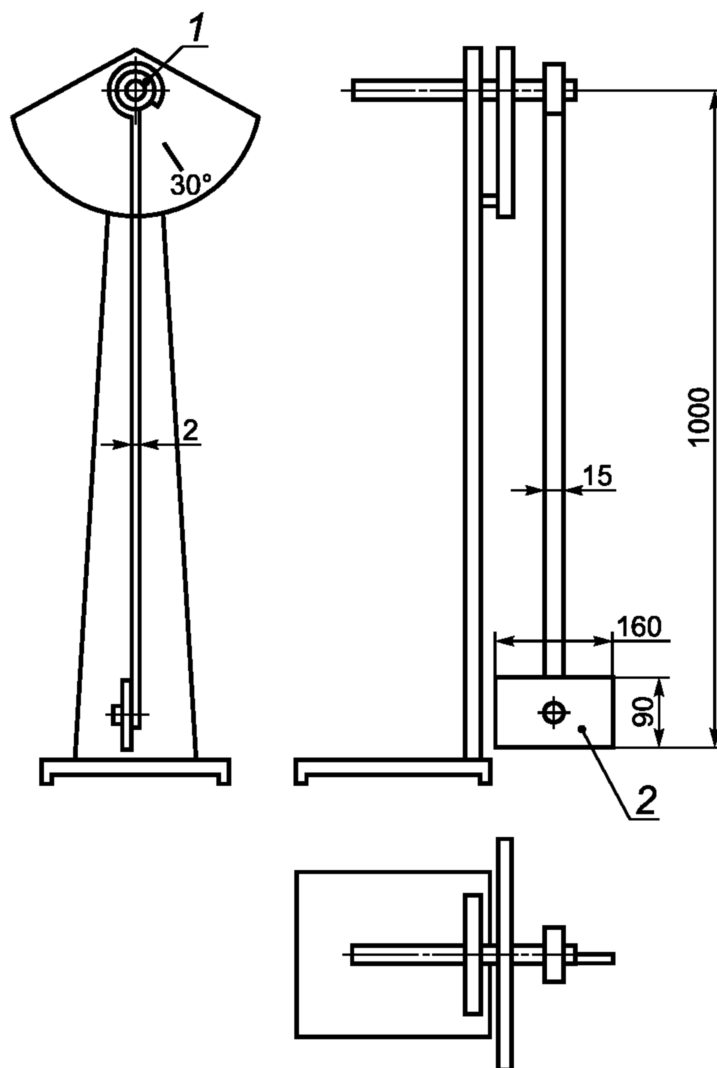
1 — подшипник; 2 — пластина из нержавеющей стали толщиной 2 мм
