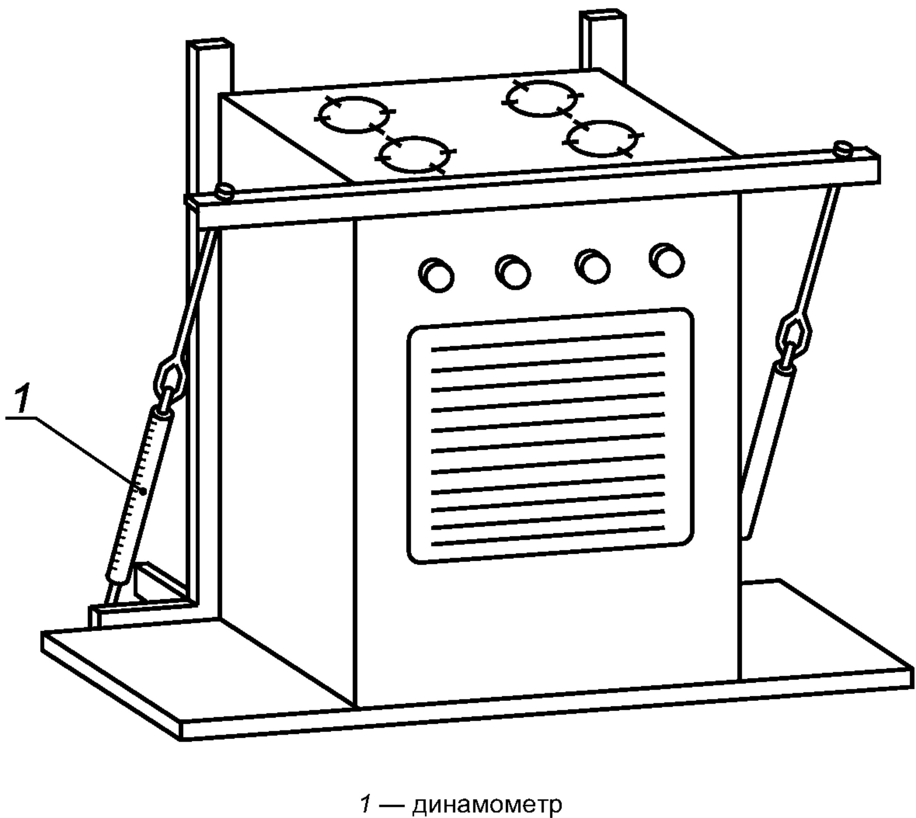
Рисунок 5 — Испытание корпуса прибора на прочность
