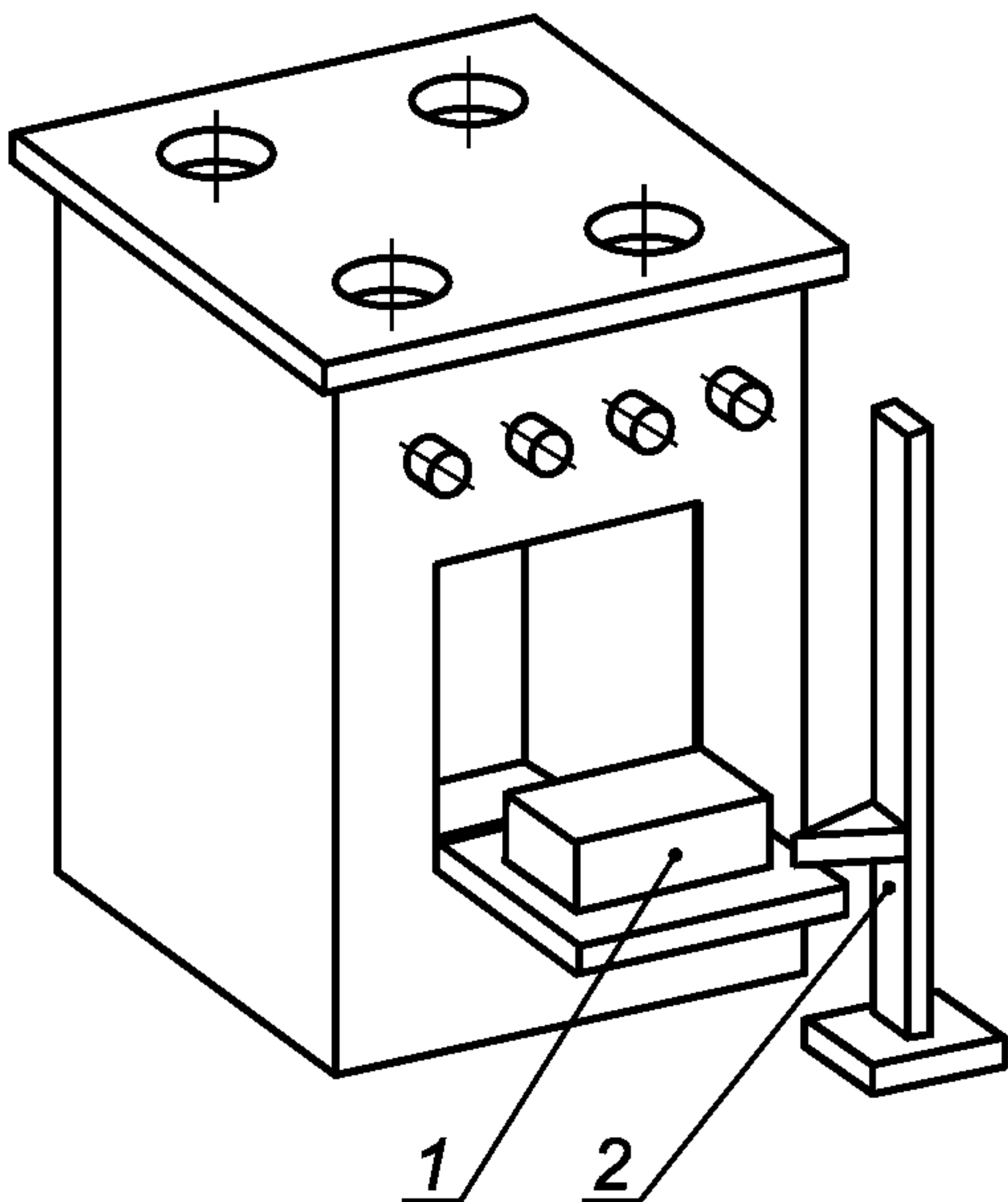
1 — испытательный груз; 2 — измерительное устройство
