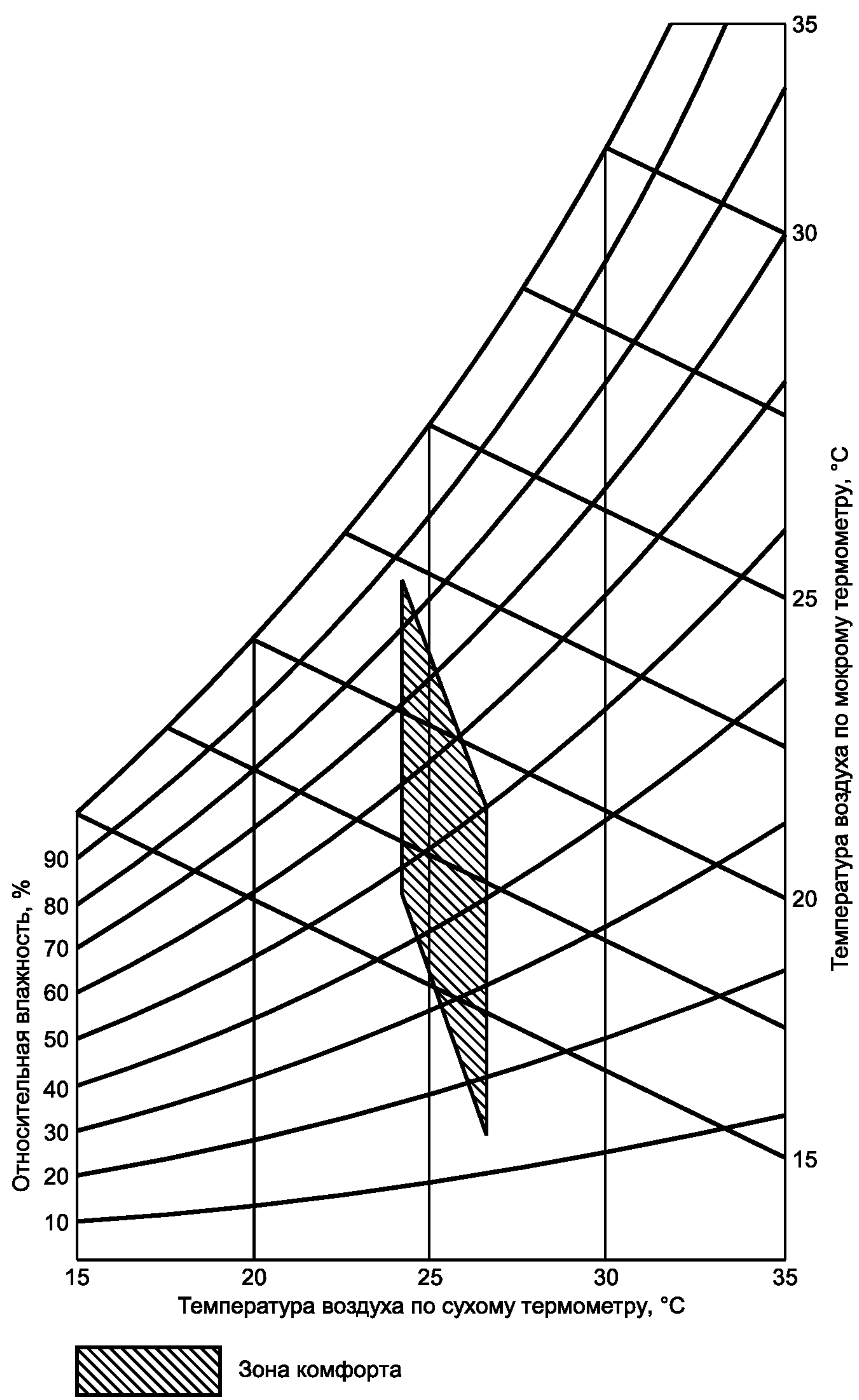
Рисунок 1 — Диаграмма эффективных температур
