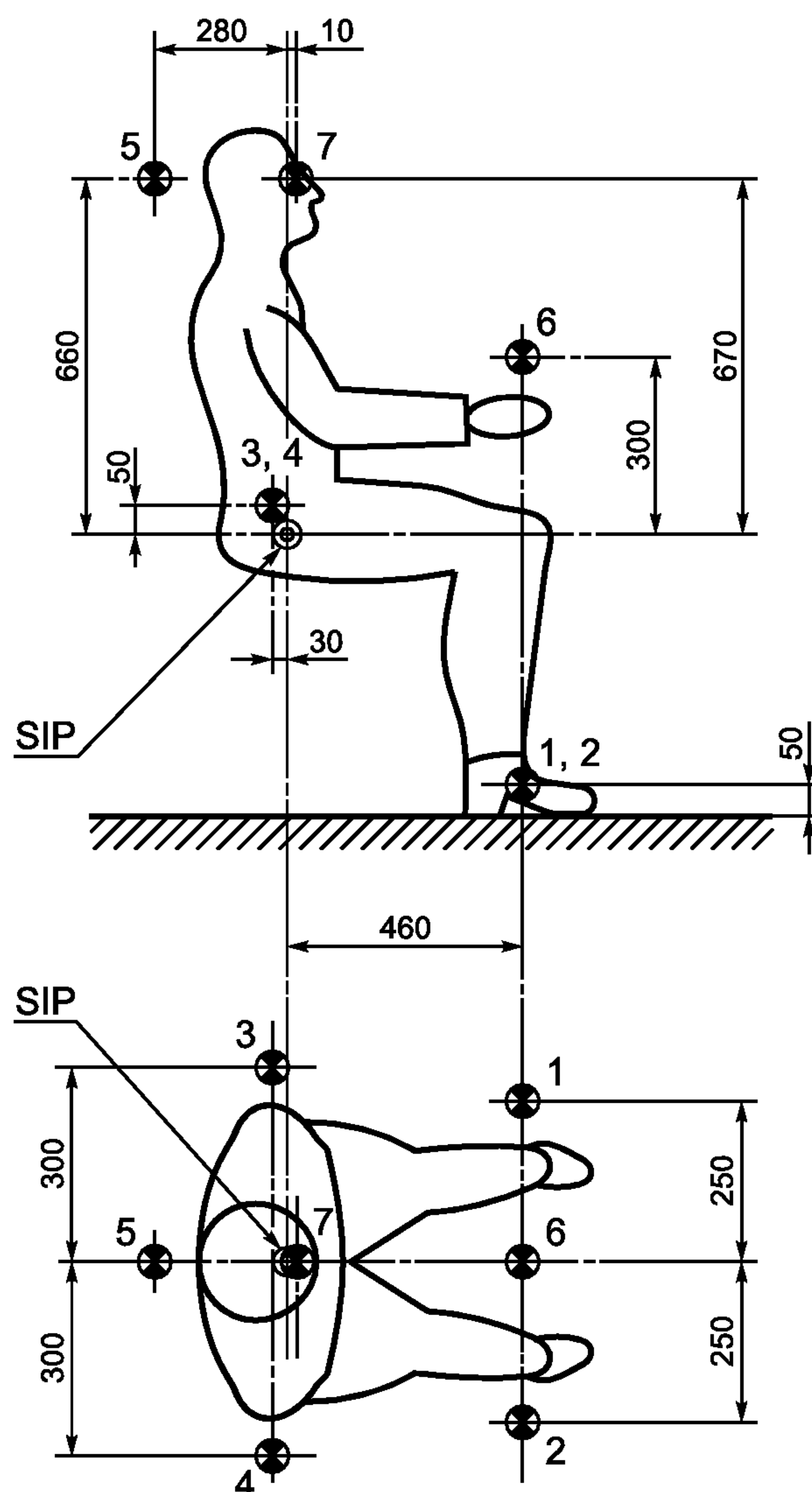
Рисунок 2 — Расположение точек измерения
